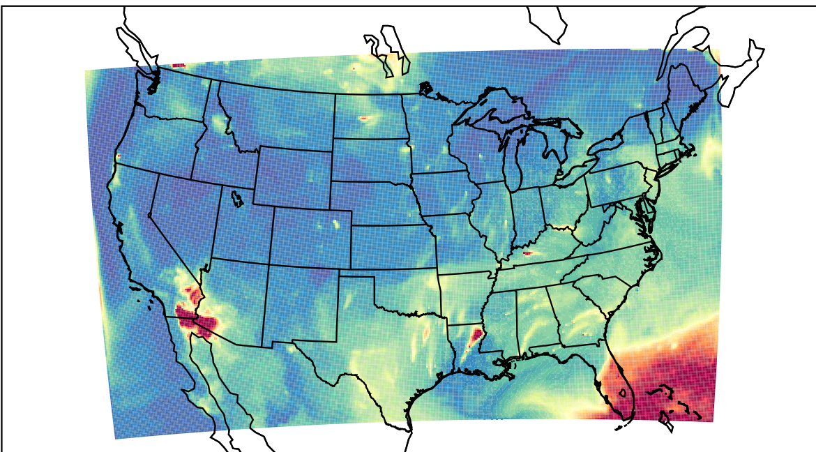
WRF 2023-07-21_08:00:00
