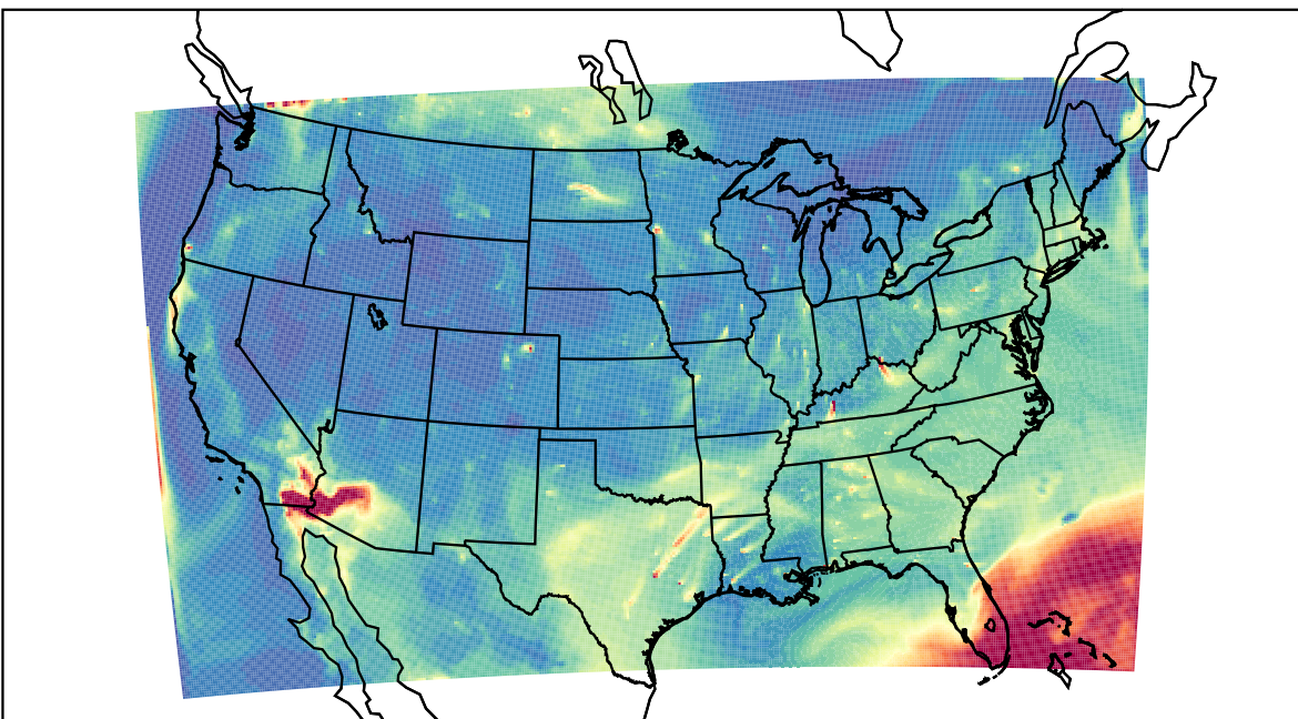
WRF 2023-07-21_13:00:00
