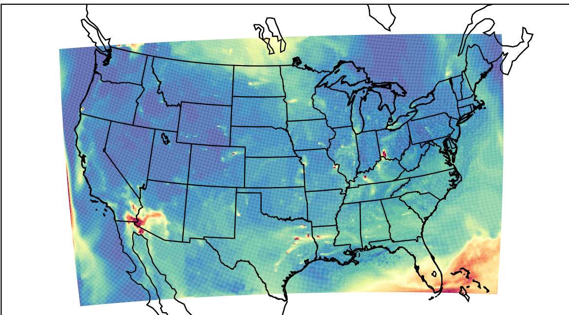
WRF 2023-07-22_15:00:00
