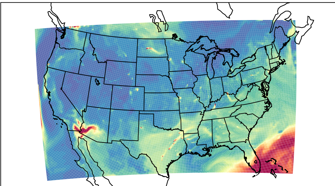
WRF 2023-07-21_15:00:00
