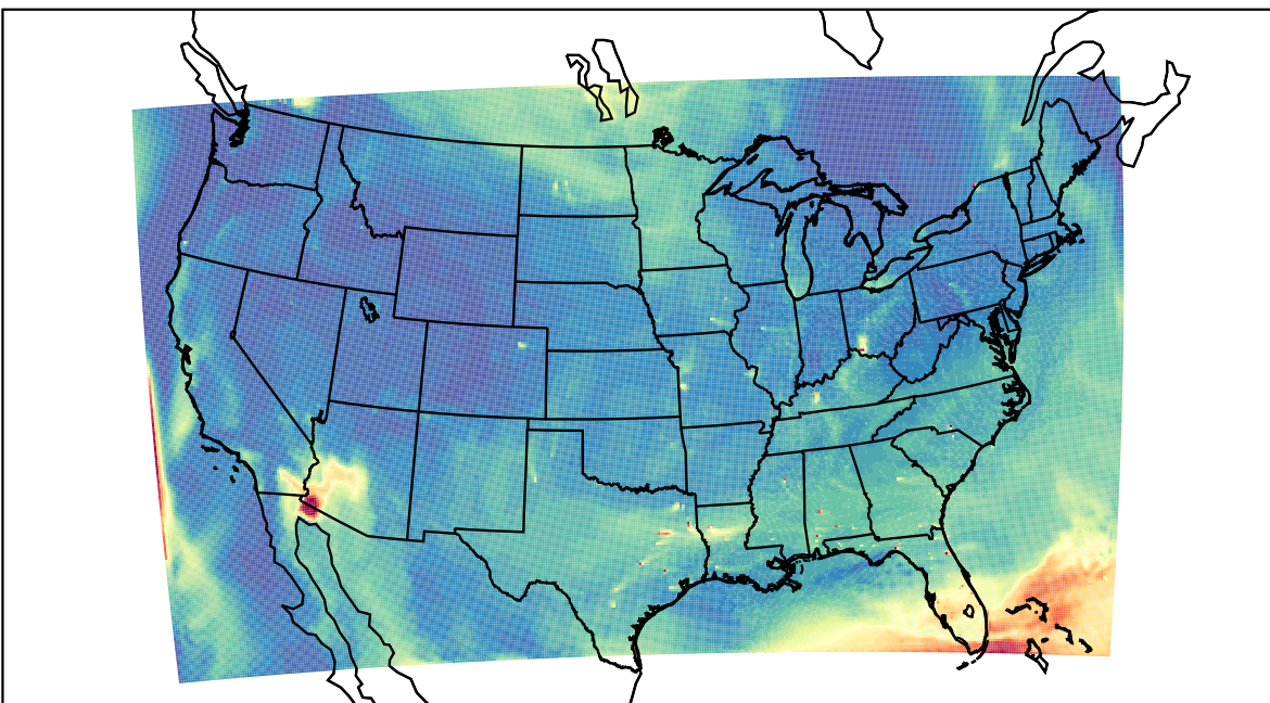
WRF 2023-07-22_18:00:00
