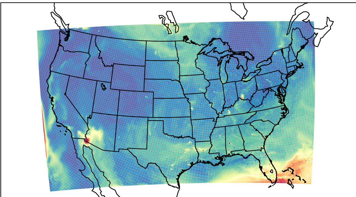
WRF 2023-07-22_19:00:00
