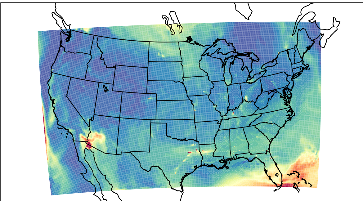
WRF 2023-07-22_17:00:00
