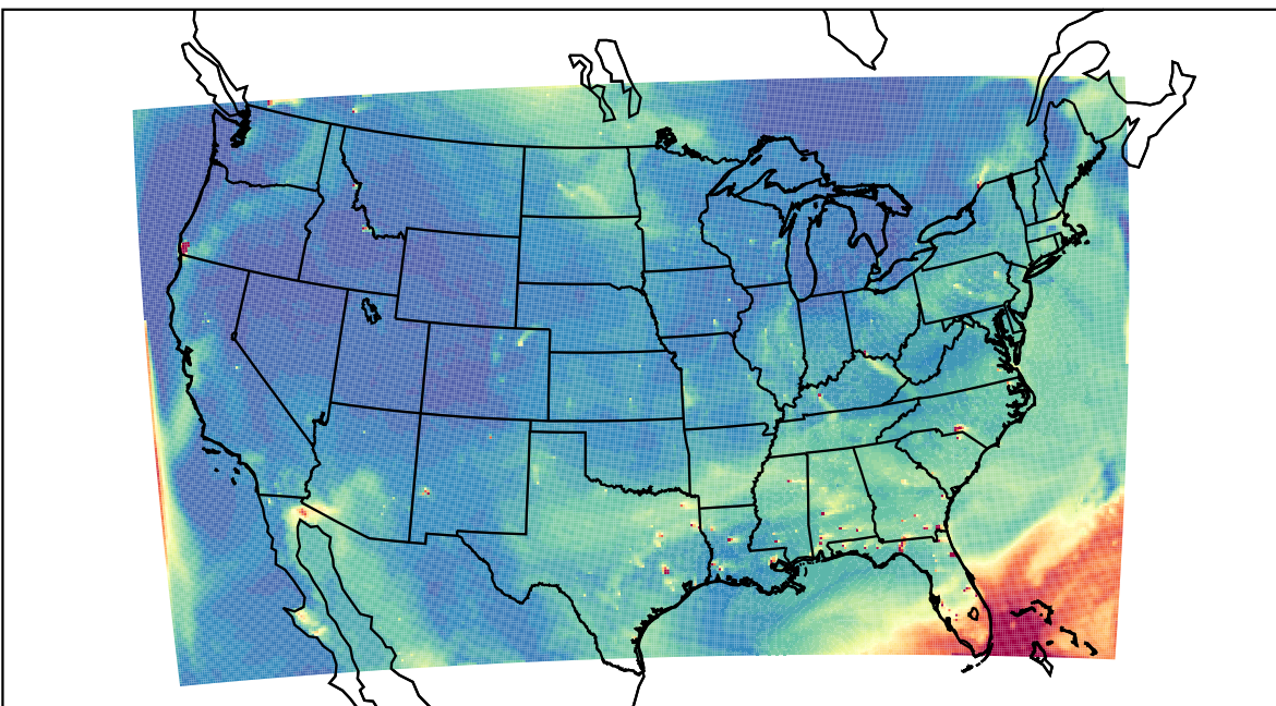
WRF 2023-07-21_23:00:00
