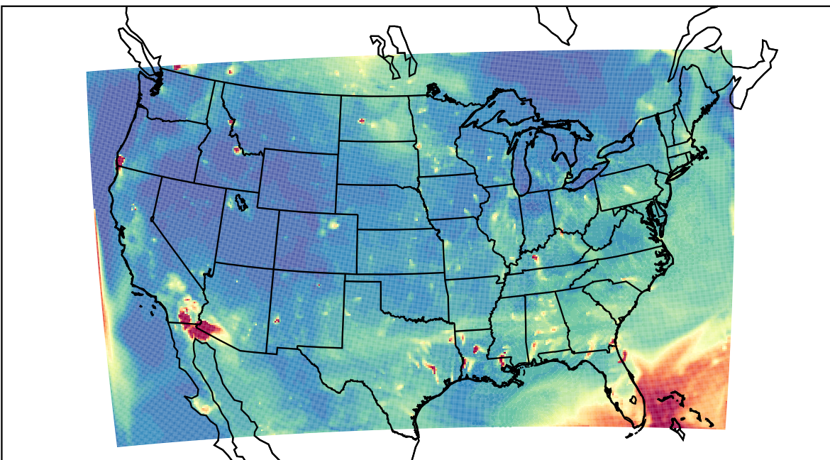
WRF 2023-07-22_03:00:00
