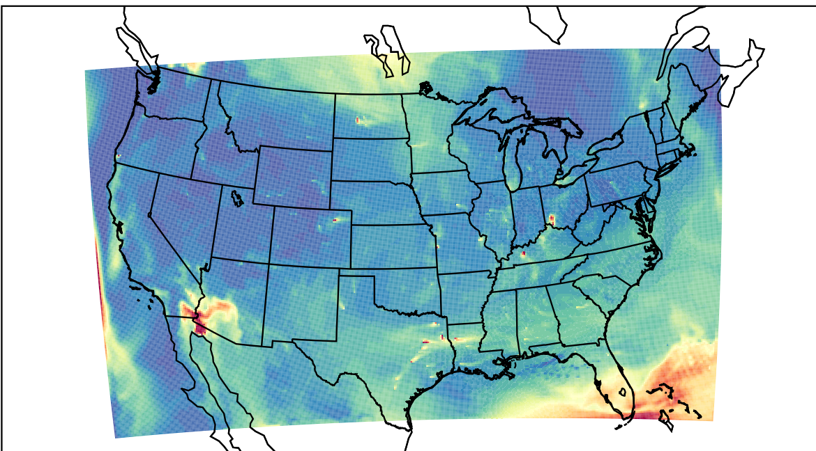
WRF 2023-07-22_16:00:00
