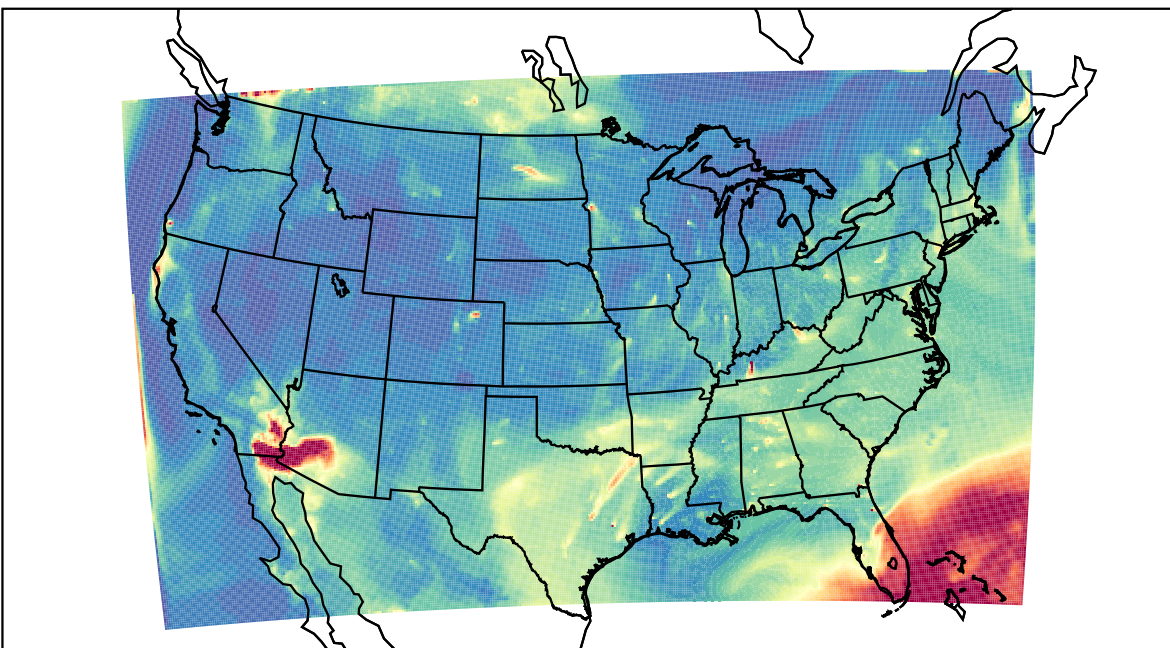
WRF 2023-07-21_12:00:00
