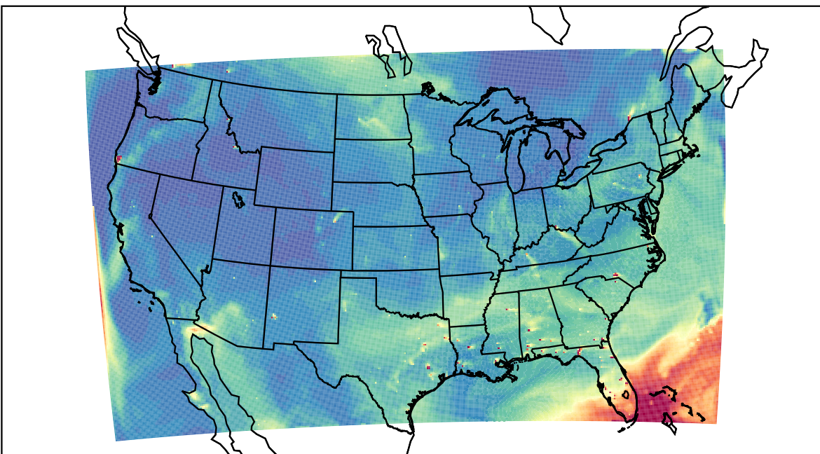
WRF 2023-07-21_22:00:00
