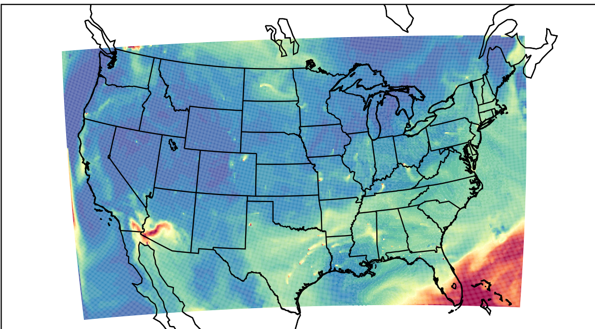
WRF 2023-07-21_17:00:00
