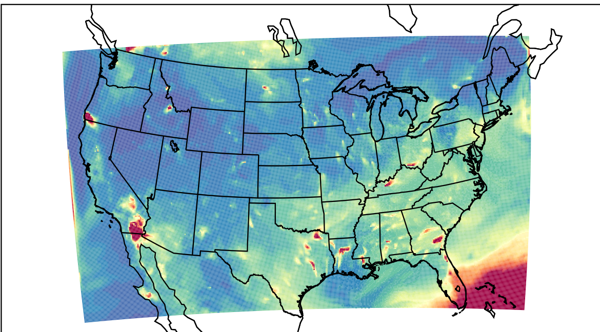
WRF 2023-07-21_04:00:00
