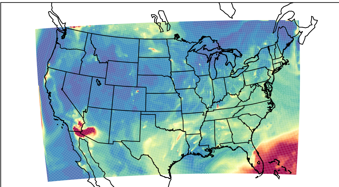
WRF 2023-07-21_11:00:00
