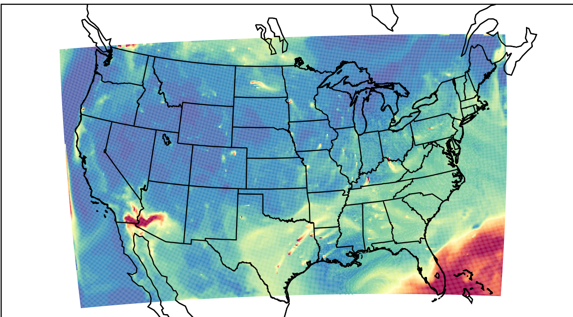
WRF 2023-07-21_14:00:00
