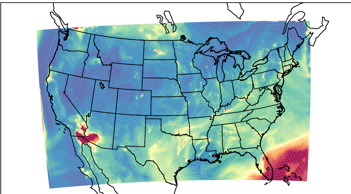
WRF 2023-07-21_10:00:00
