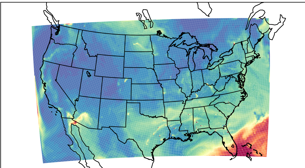
WRF 2023-07-21_19:00:00
