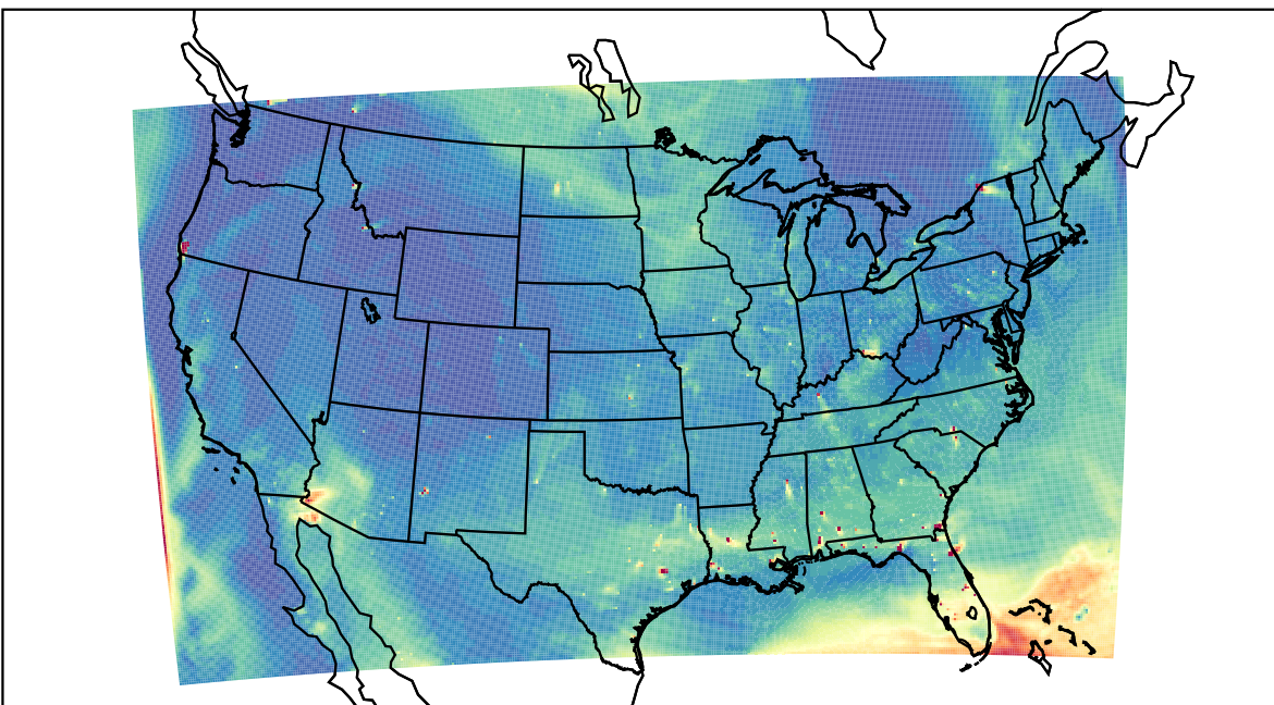
WRF 2023-07-22_23:00:00
