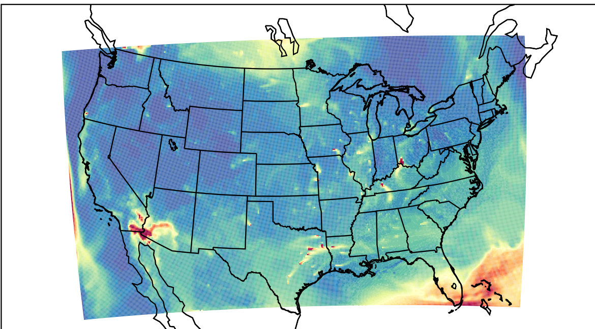
WRF 2023-07-22_14:00:00
