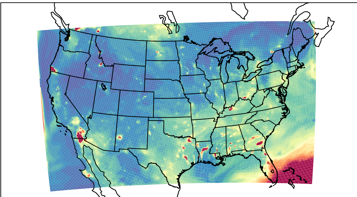
WRF 2023-07-21_03:00:00
