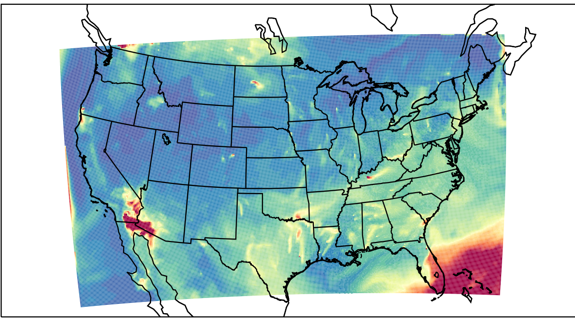
WRF 2023-07-21_08:00:00
