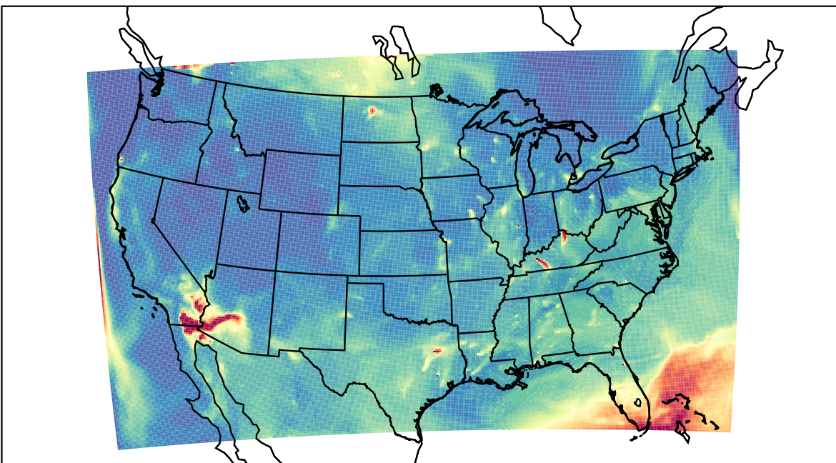
WRF 2023-07-22_10:00:00
