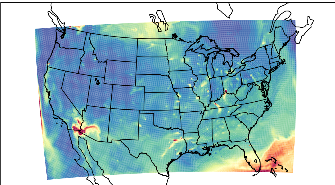
WRF 2023-07-22_13:00:00
