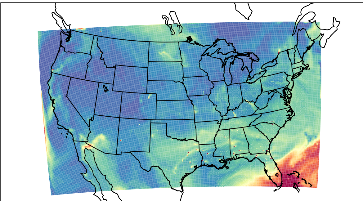
WRF 2023-07-21_20:00:00
