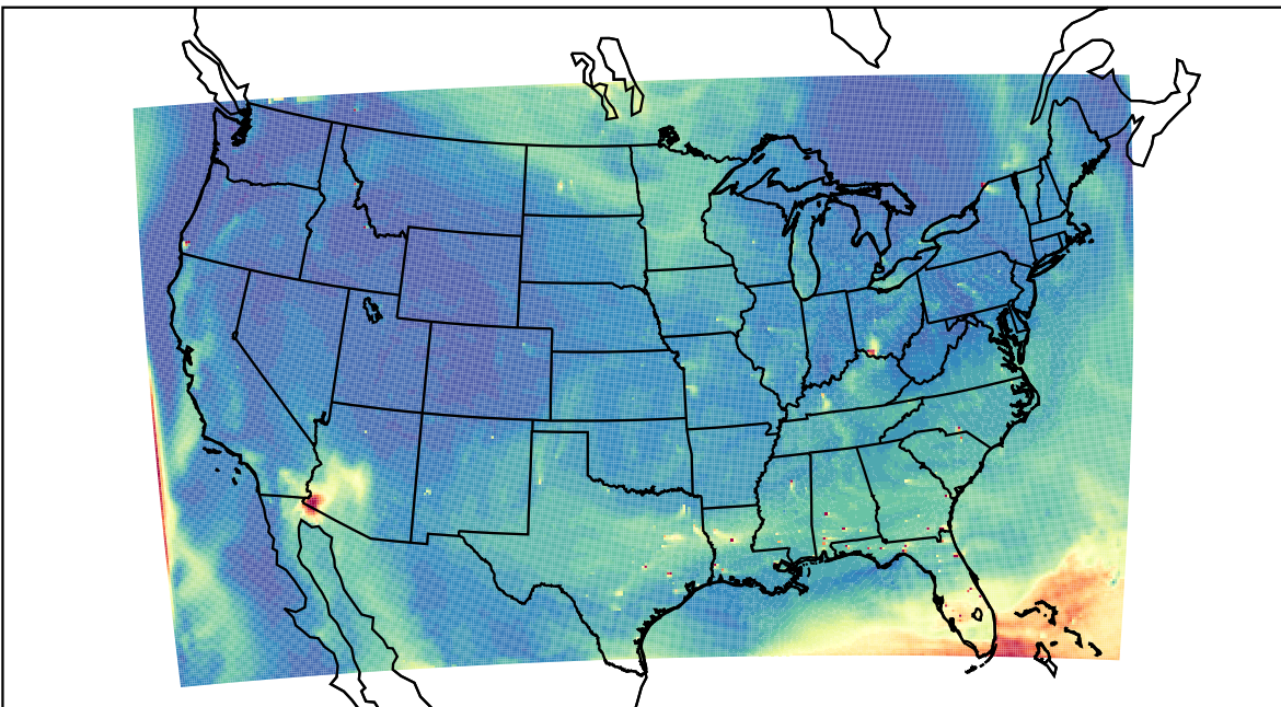
WRF 2023-07-22_20:00:00
