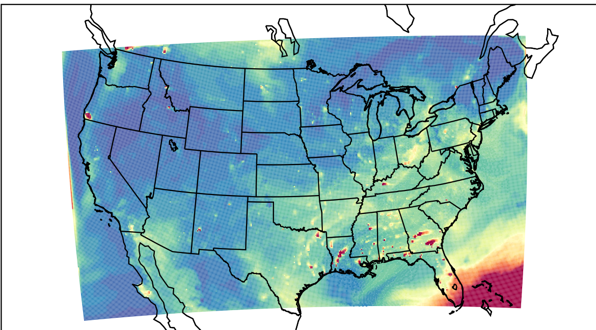
WRF 2023-07-21_01:00:00
