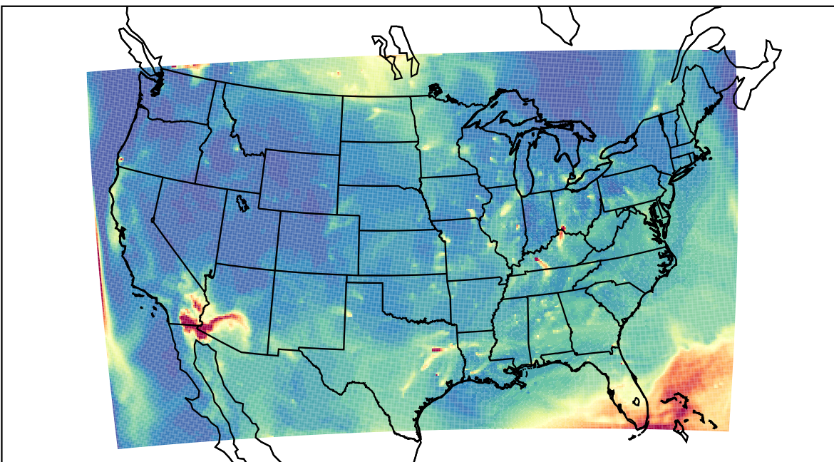
WRF 2023-07-22_12:00:00
