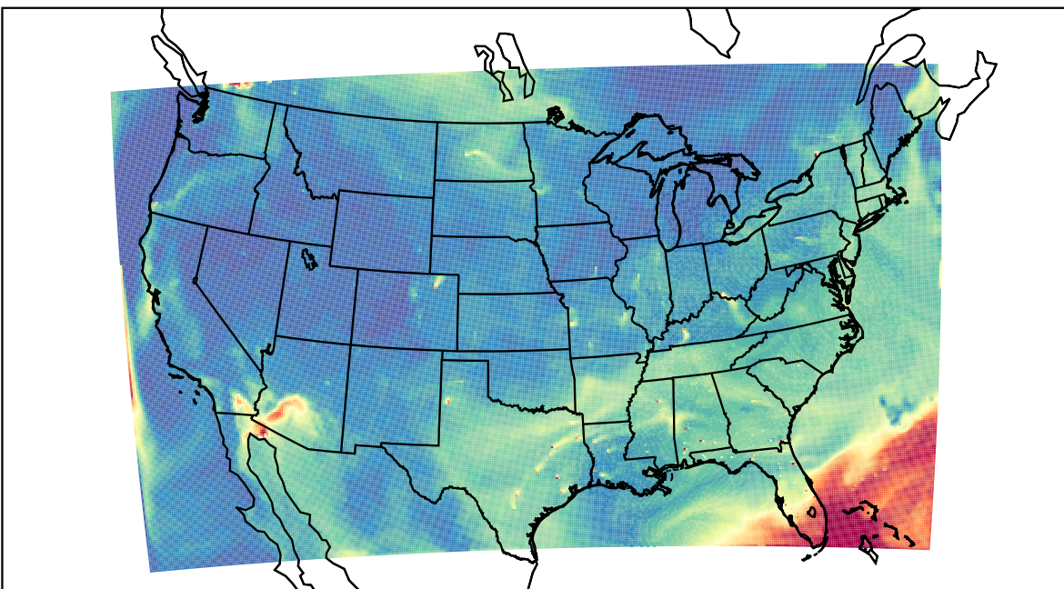
WRF 2023-07-21_18:00:00
