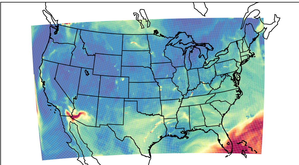
WRF 2023-07-21_16:00:00
