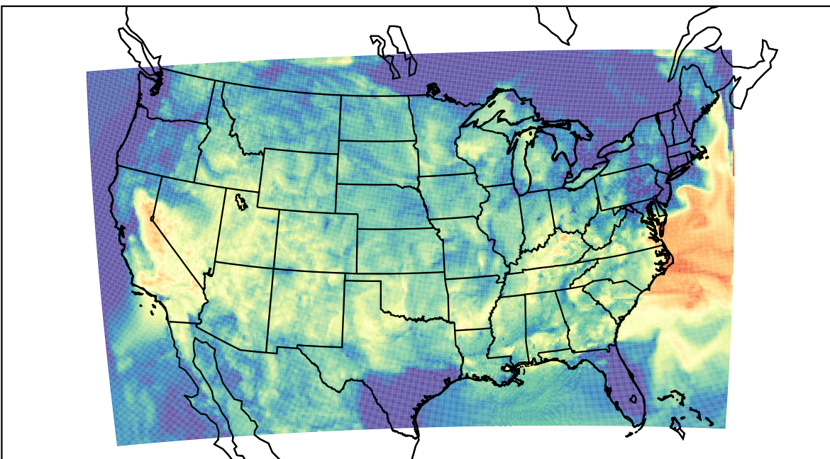
WRF (2023-07-23_10:00:00)
