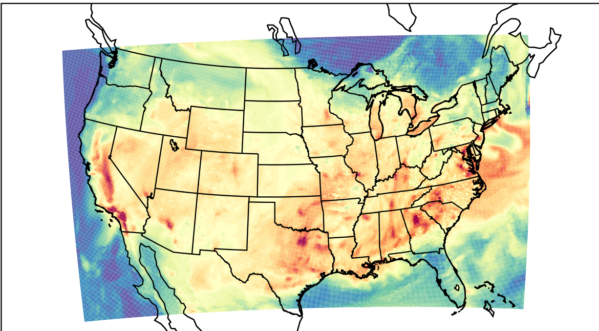
WRF (2023-07-23_20:00:00)
