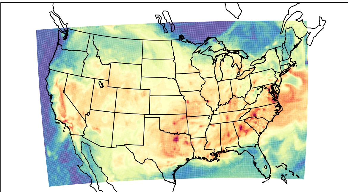
WRF (2023-07-23_18:00:00)
