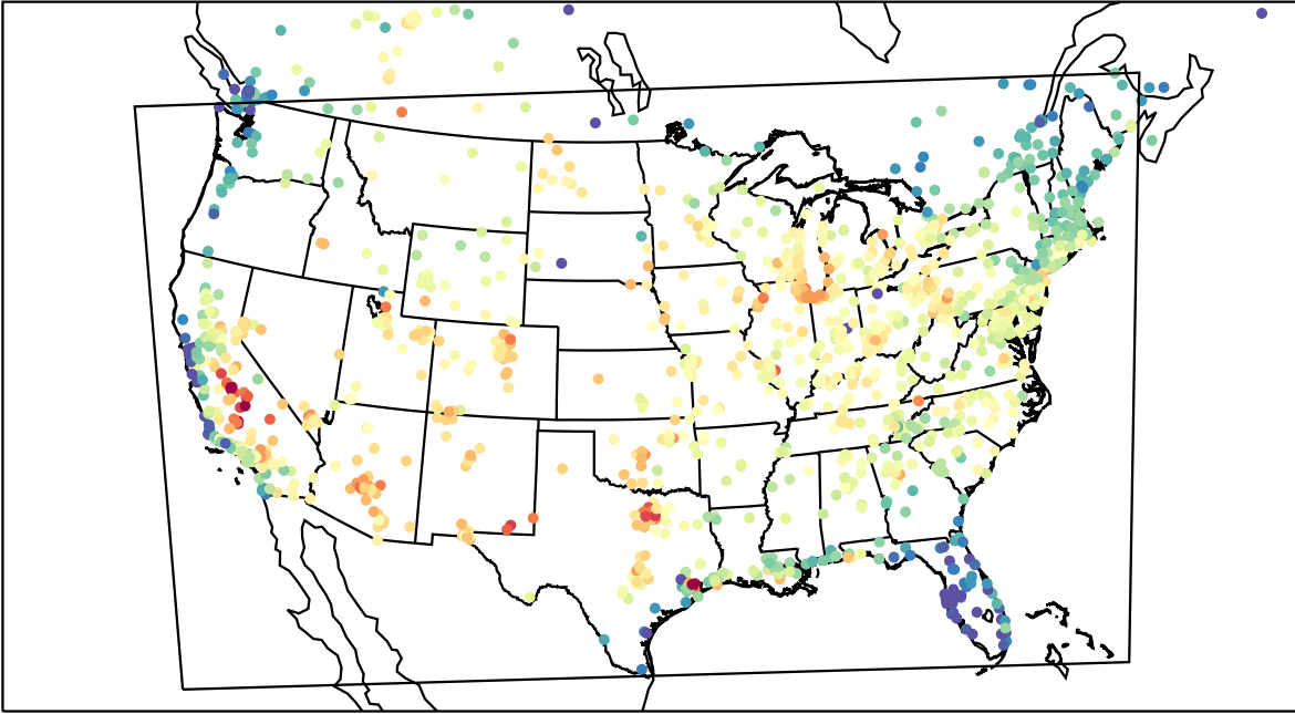
AirNOW (2023-07-23_18:00:00)
