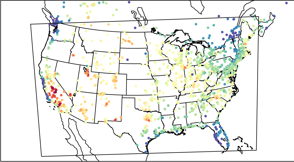
AirNOW (2023-07-22_18:00:00)
