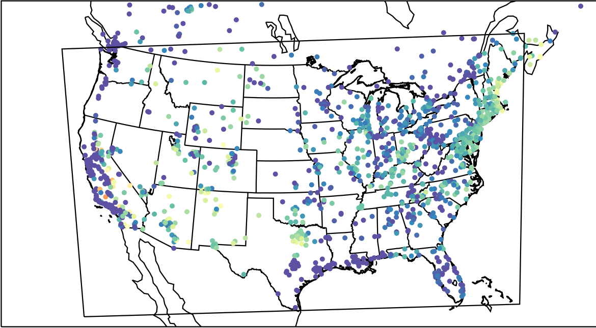
AirNOW (2023-07-22_13:00:00)
