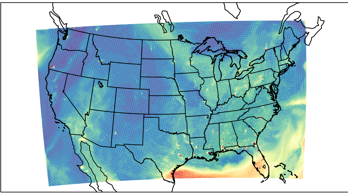
WRF 2023-07-24_23:00:00
