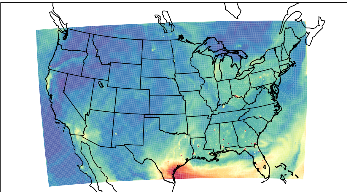
WRF 2023-07-25_20:00:00
