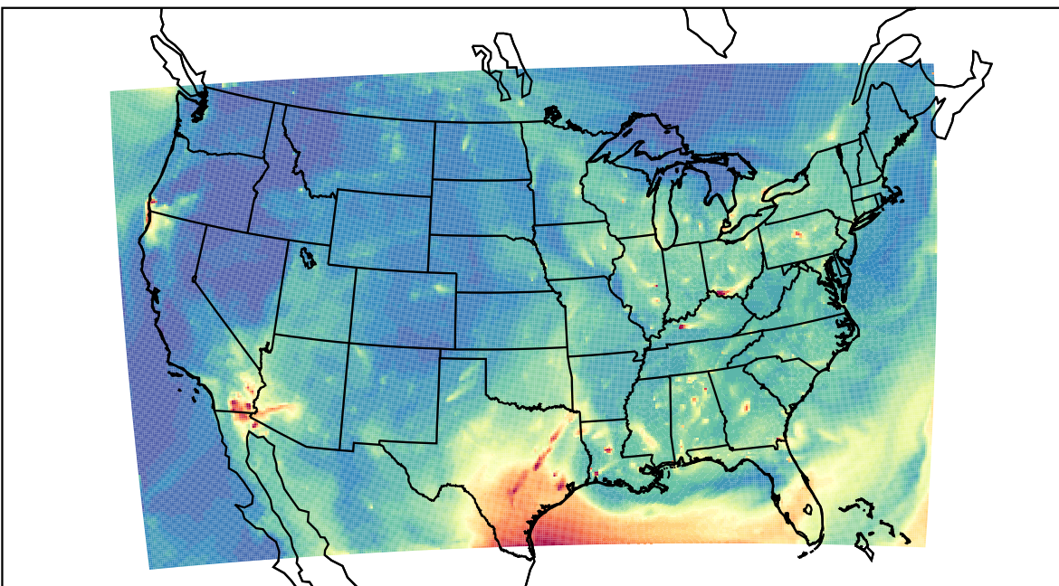
WRF 2023-07-25_13:00:00
