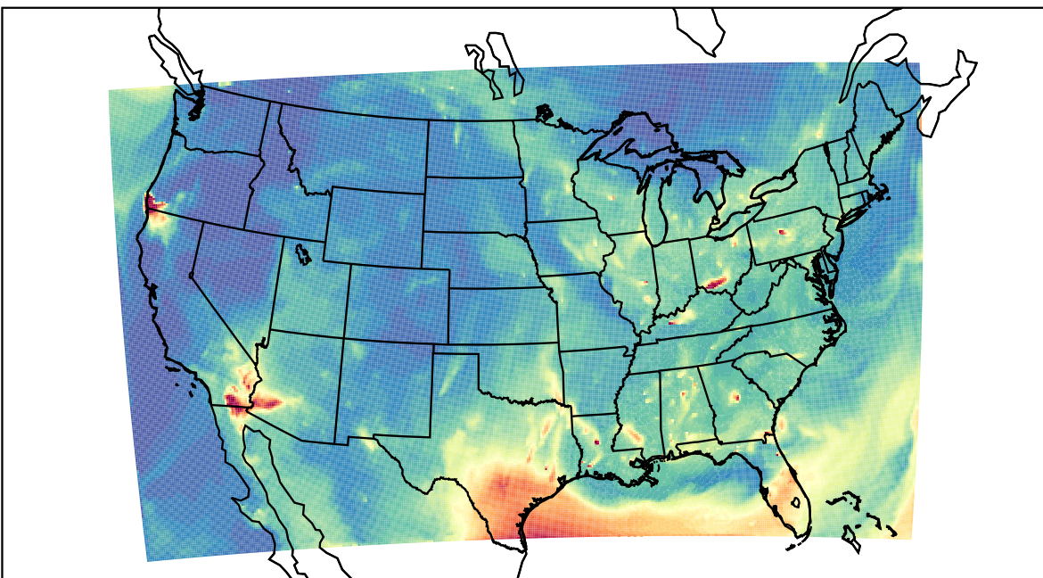
WRF 2023-07-25_10:00:00
