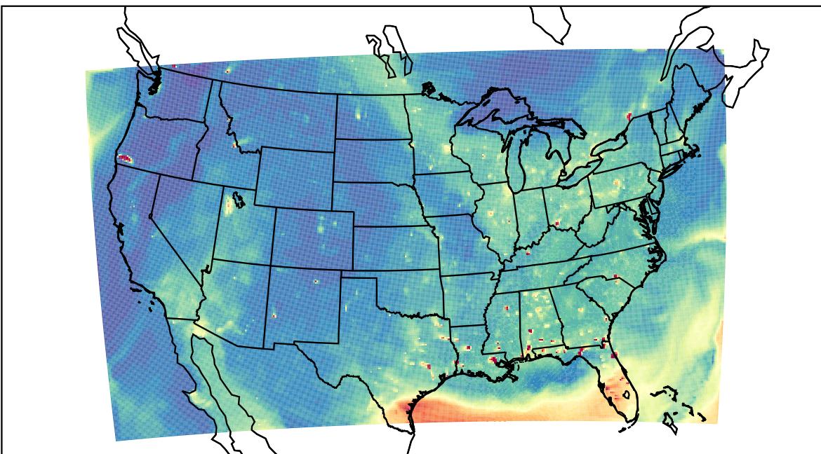
WRF 2023-07-25_01:00:00
