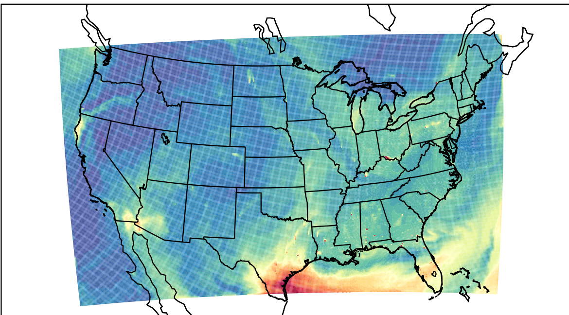
WRF 2023-07-25_18:00:00
