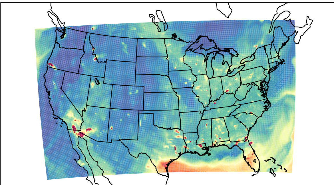
WRF 2023-07-25_03:00:00
