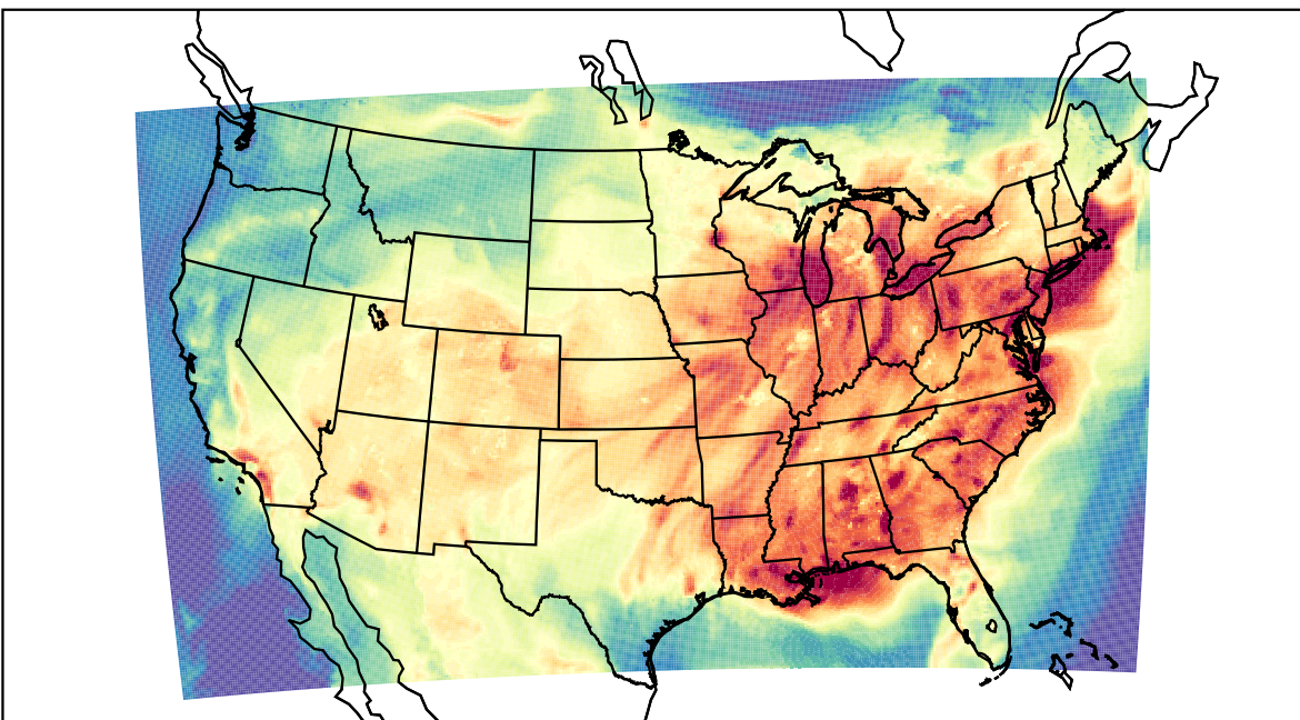
WRF (2023-07-26_19:00:00)
