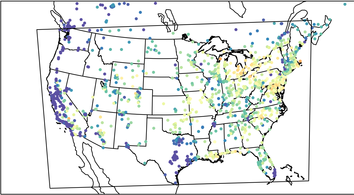
AirNOW (2023-07-26_14:00:00)
