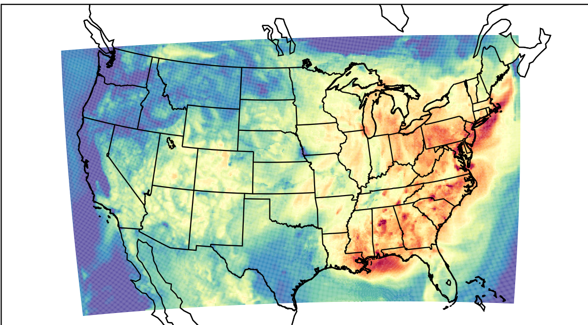
WRF (2023-07-26_15:00:00)
