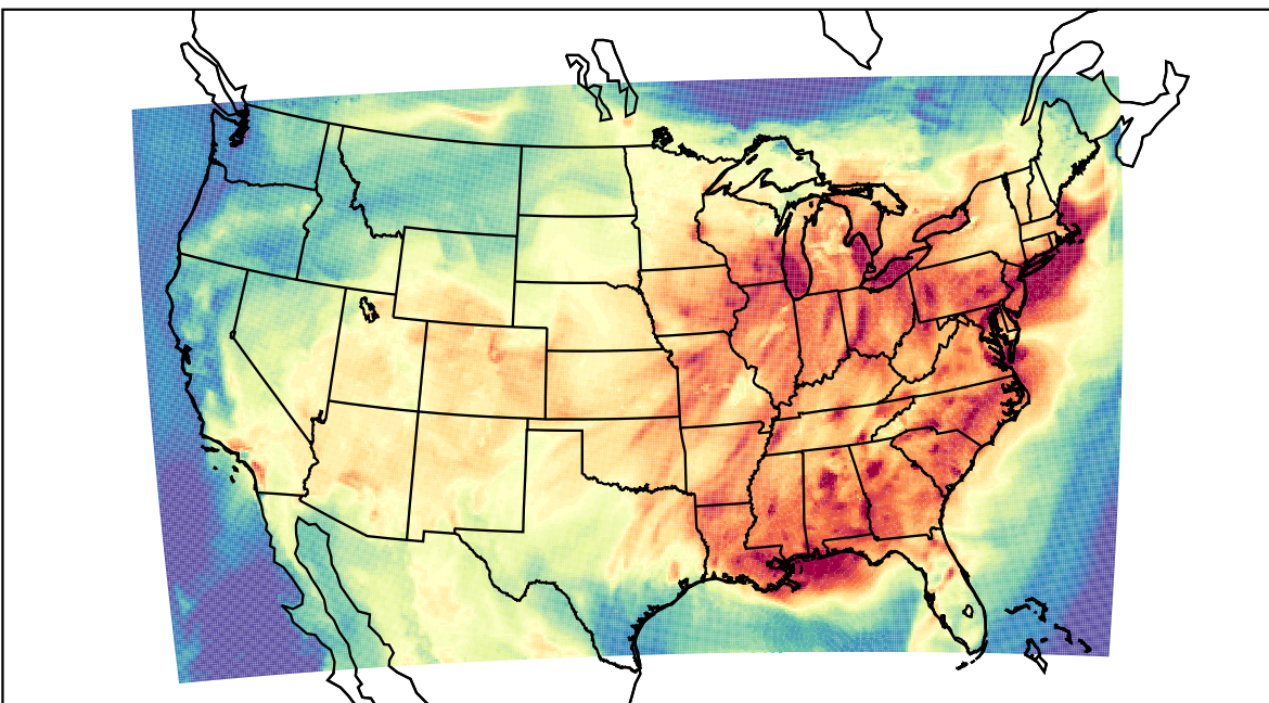
WRF (2023-07-26_18:00:00)
