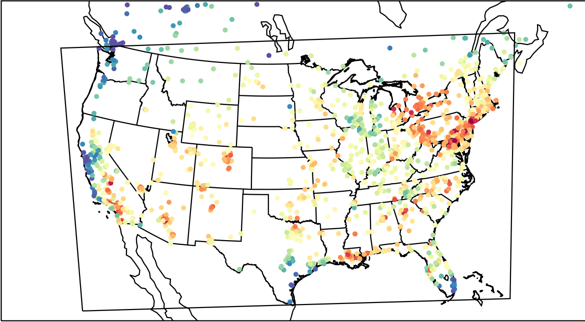
AirNOW (2023-07-26_18:00:00)
