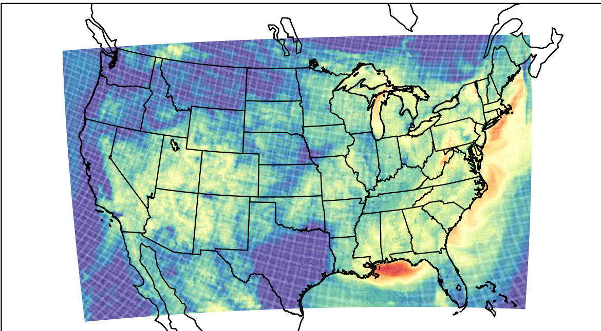
WRF (2023-07-26_13:00:00)
