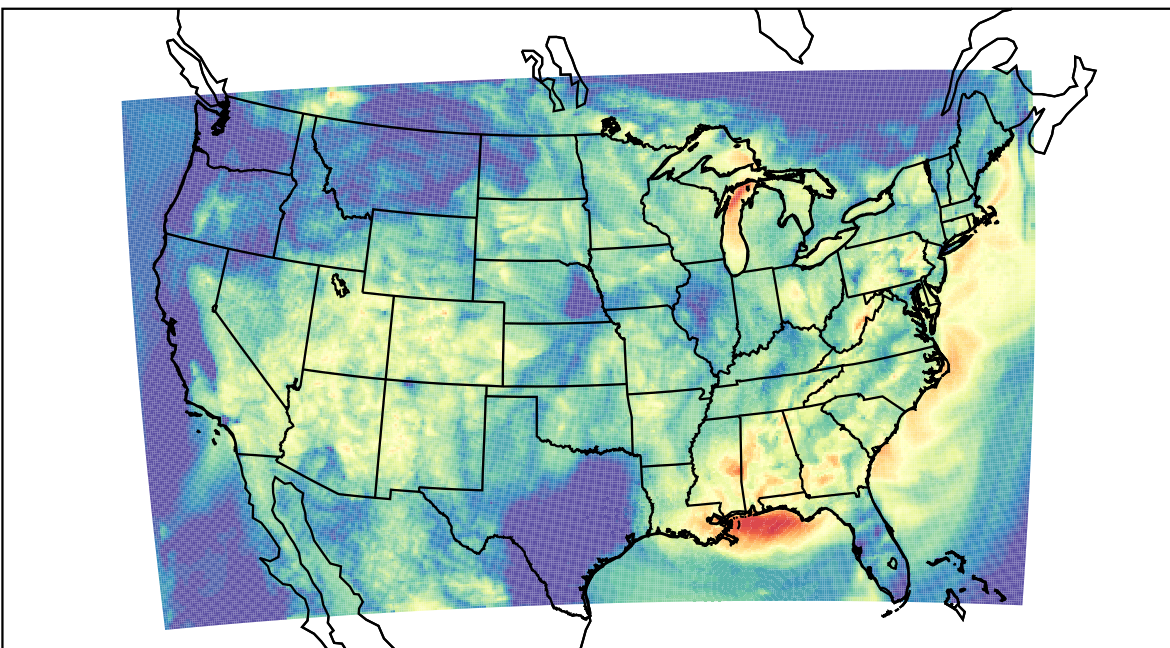
WRF (2023-07-26_10:00:00)
