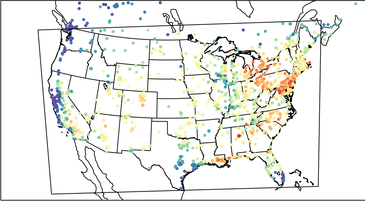
AirNOW (2023-07-26_16:00:00)
