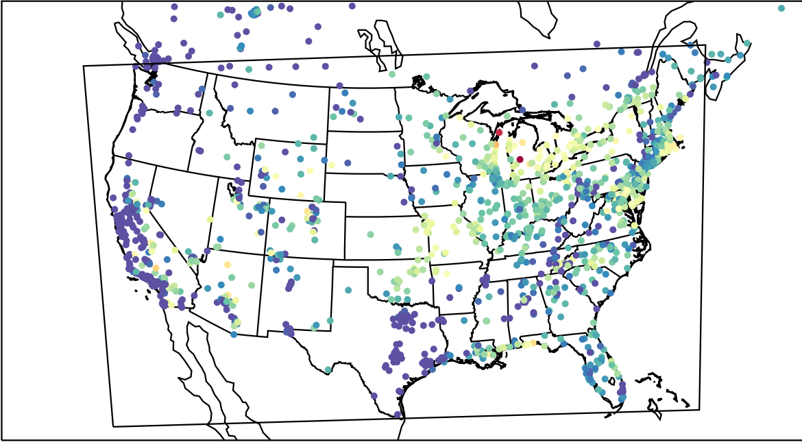
AirNOW (2023-07-26_13:00:00)
