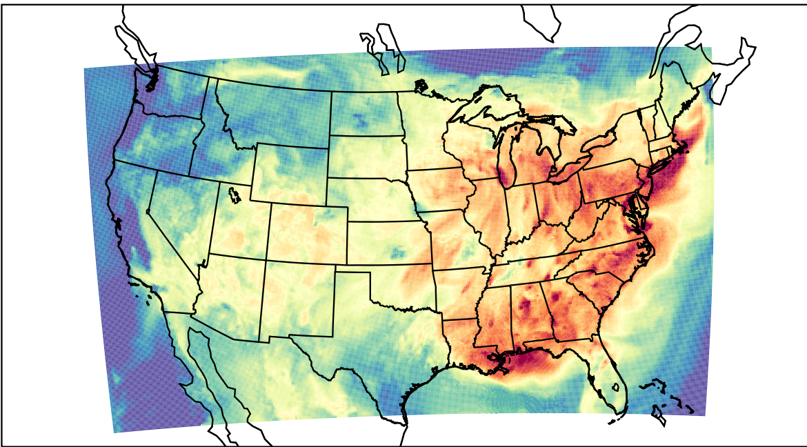
WRF (2023-07-26_16:00:00)
