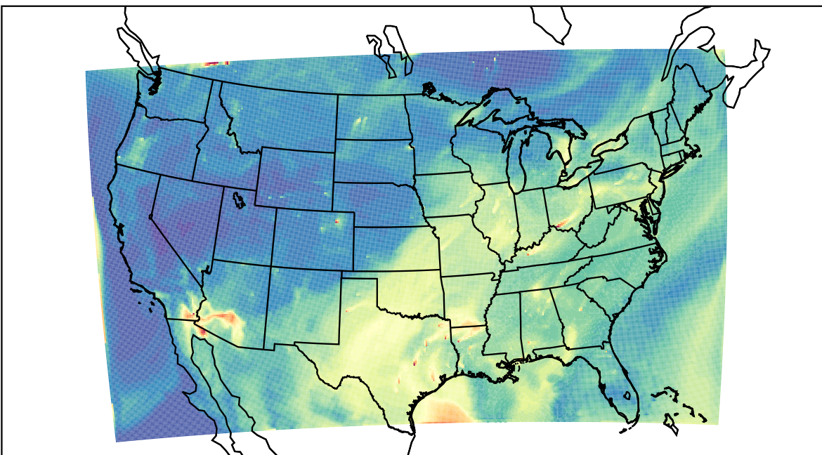
WRF 2023-07-28_16:00:00
