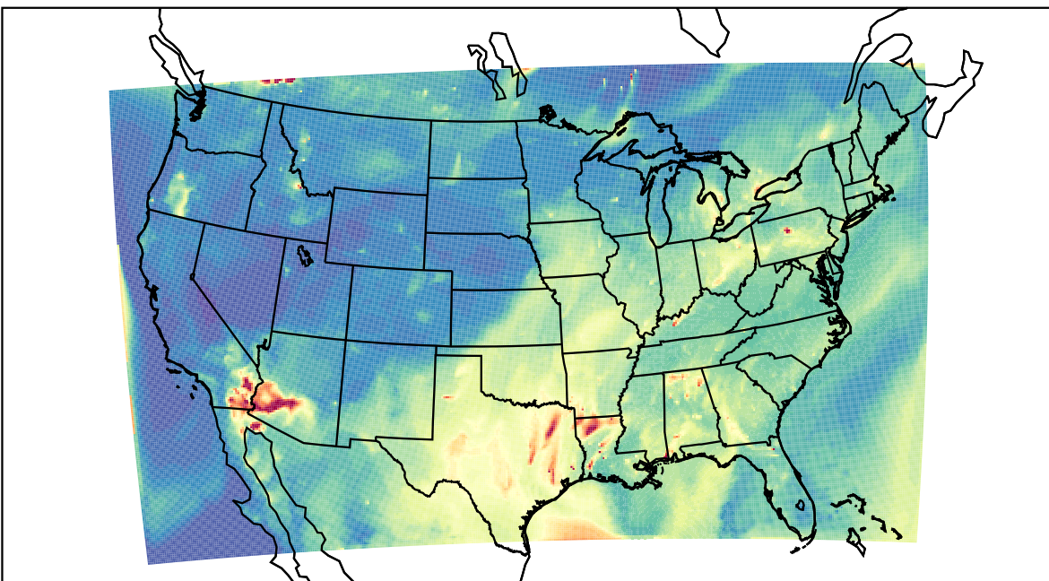
WRF 2023-07-28_11:00:00
