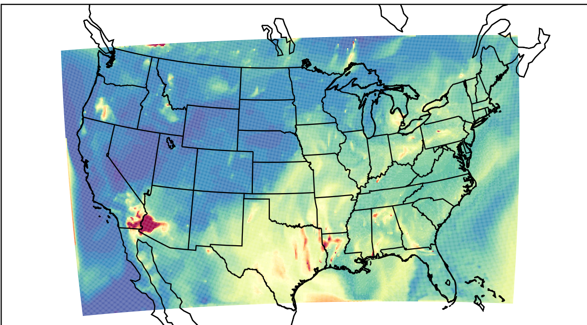
WRF 2023-07-28_08:00:00
