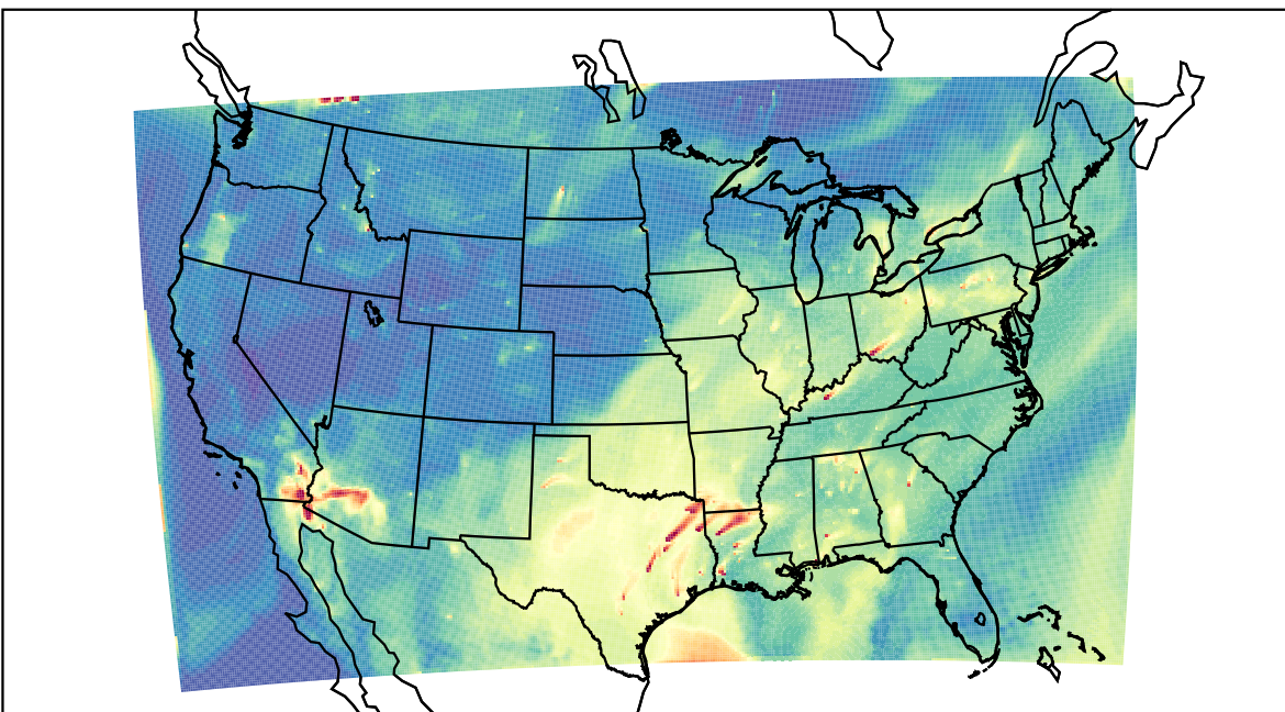
WRF 2023-07-28_14:00:00
