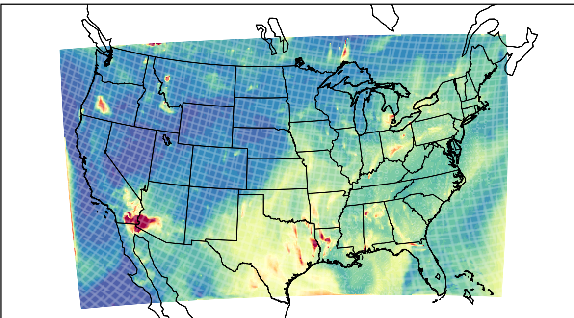
WRF 2023-07-28_06:00:00
