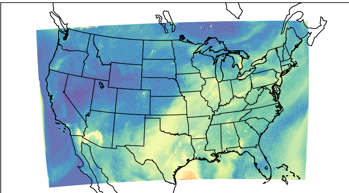
WRF 2023-07-28_18:00:00
