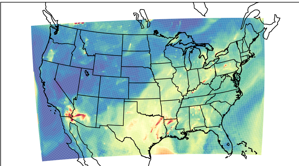
WRF 2023-07-28_13:00:00
