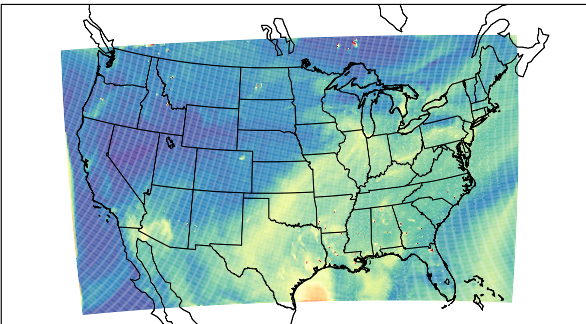
WRF 2023-07-28_20:00:00
