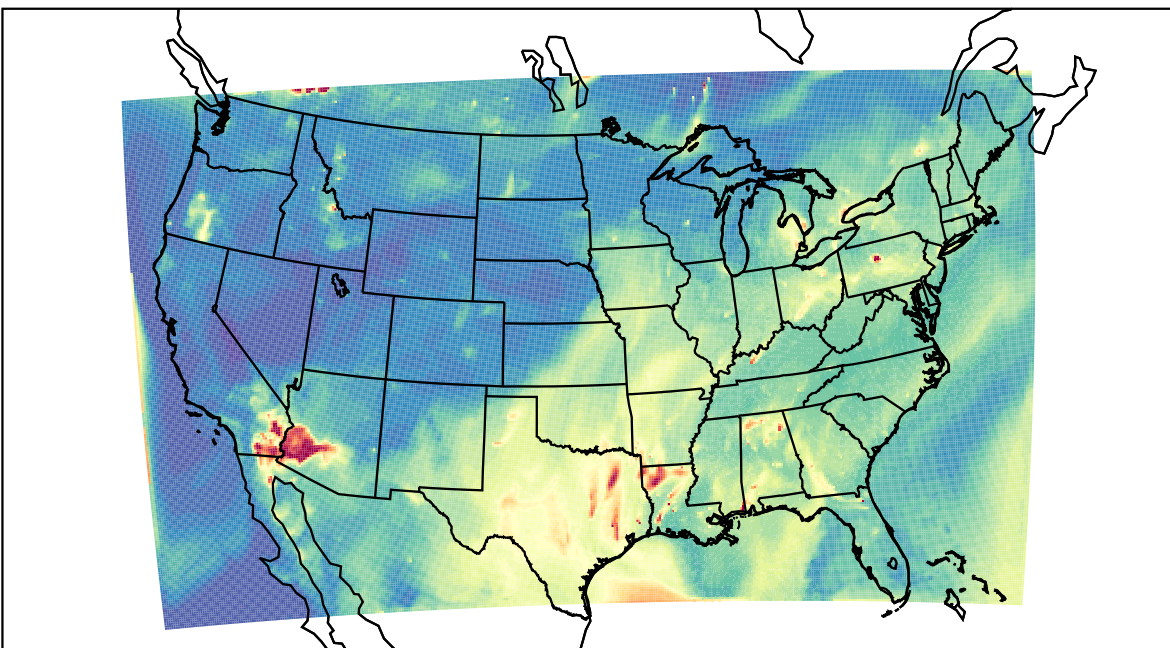
WRF 2023-07-28_10:00:00
