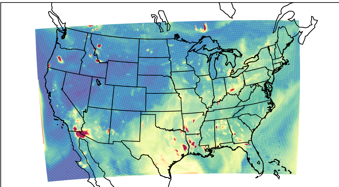
WRF 2023-07-28_03:00:00
