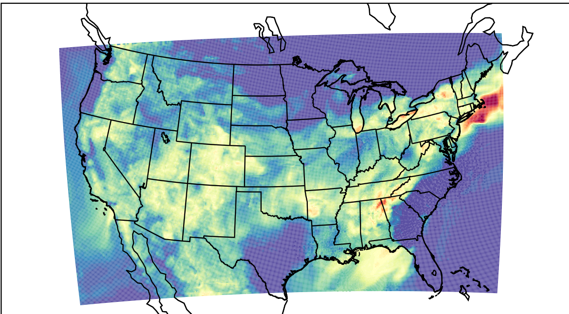
WRF (2023-07-29_10:00:00)
