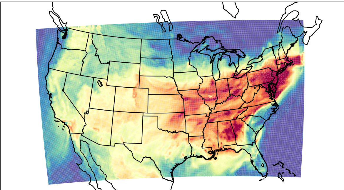
WRF (2023-07-29_18:00:00)
