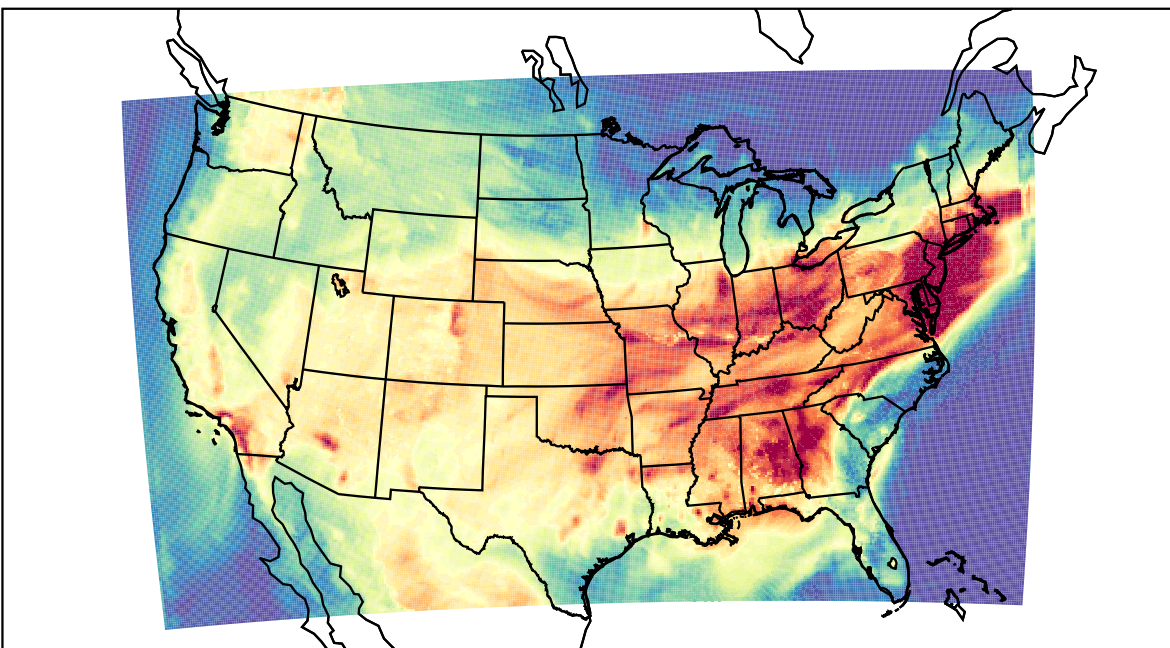
WRF (2023-07-29_20:00:00)
