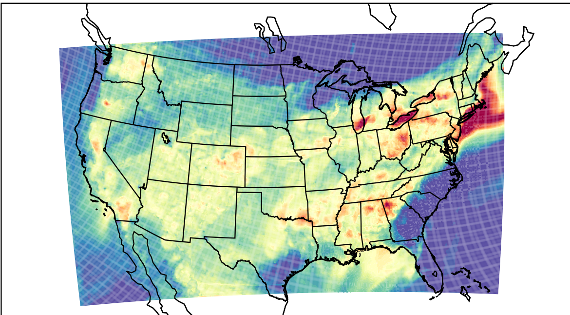
WRF (2023-07-29_03:00:00)
