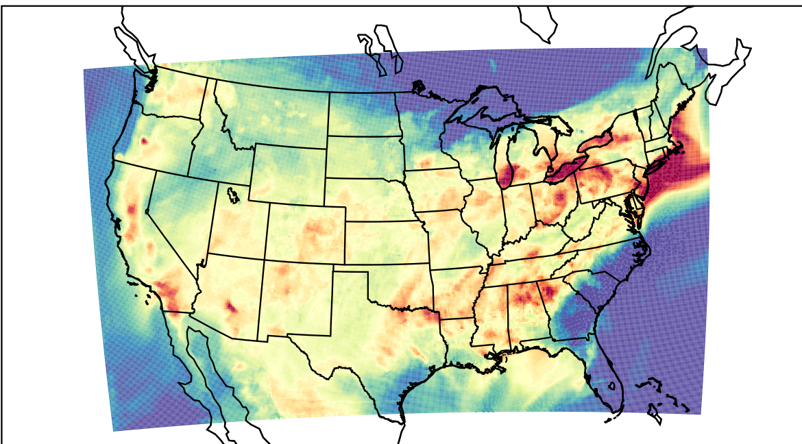
WRF (2023-07-29_01:00:00)
