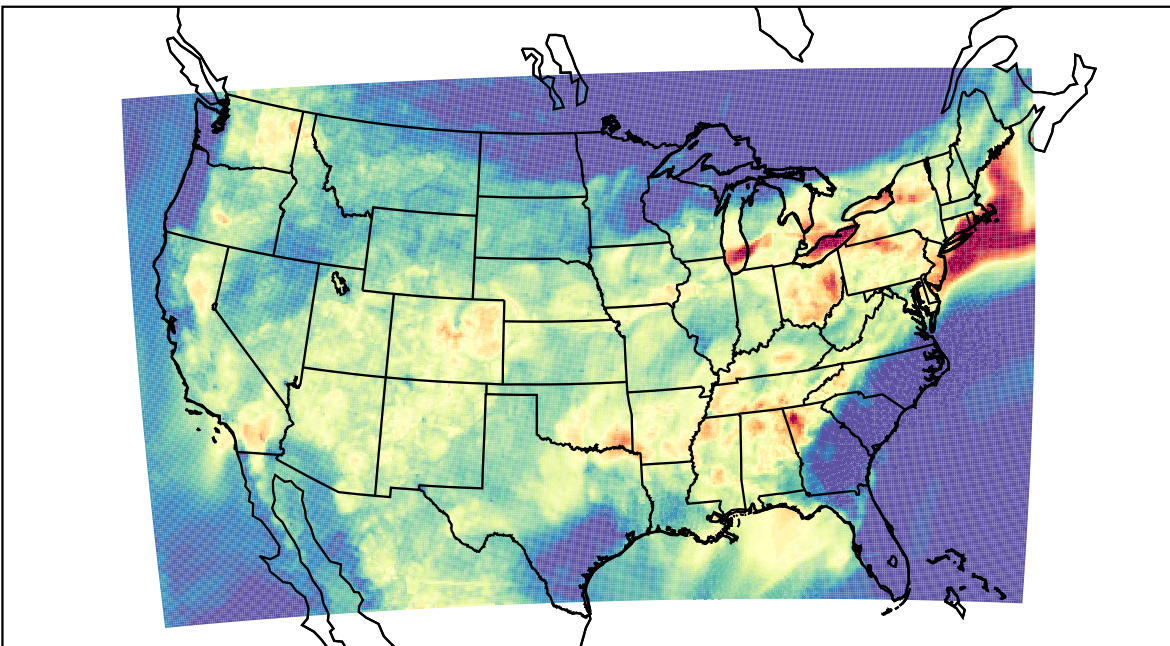
WRF (2023-07-29_04:00:00)
