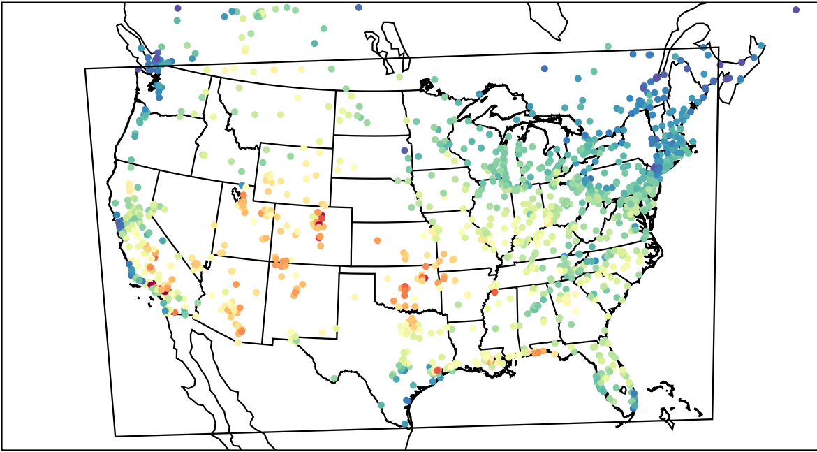
AirNOW (2023-07-30_18:00:00)
