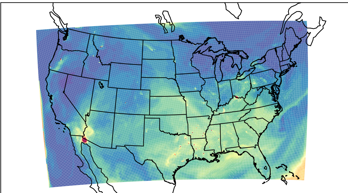
WRF 2023-07-30_20:00:00
