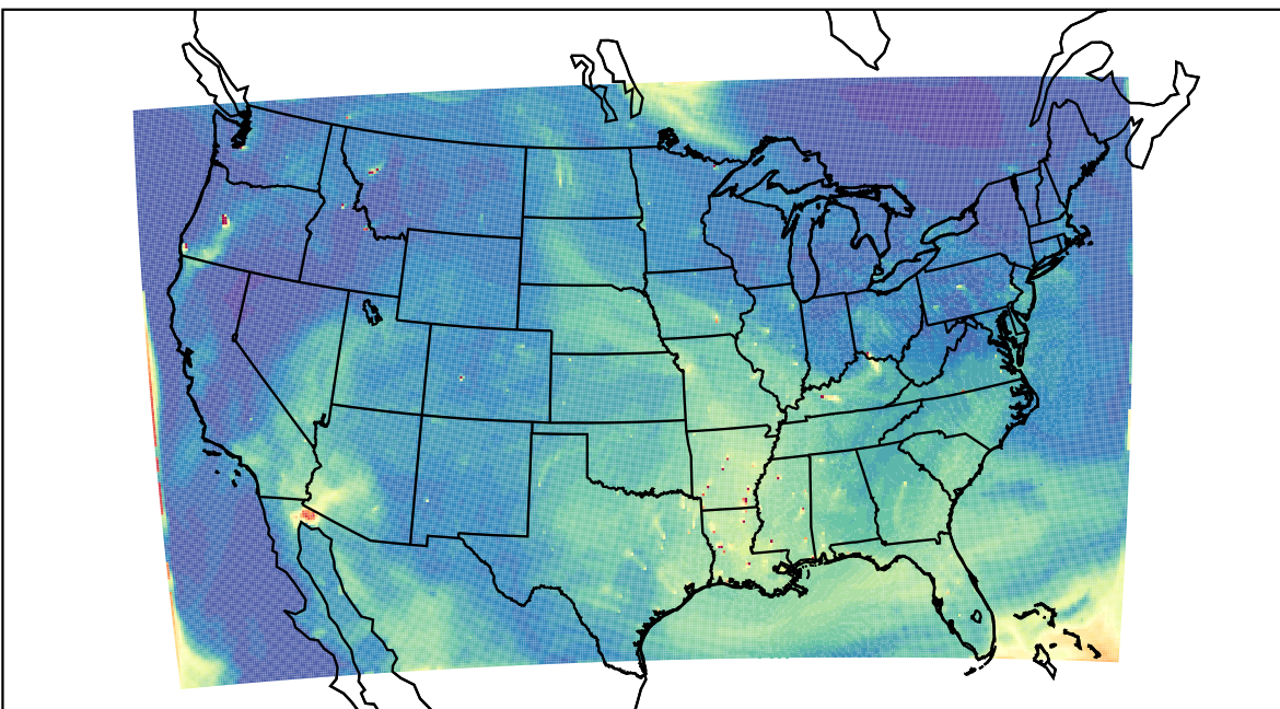
WRF 2023-07-31_22:00:00
