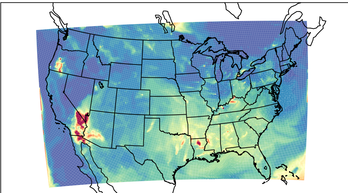
WRF 2023-07-31_10:00:00
