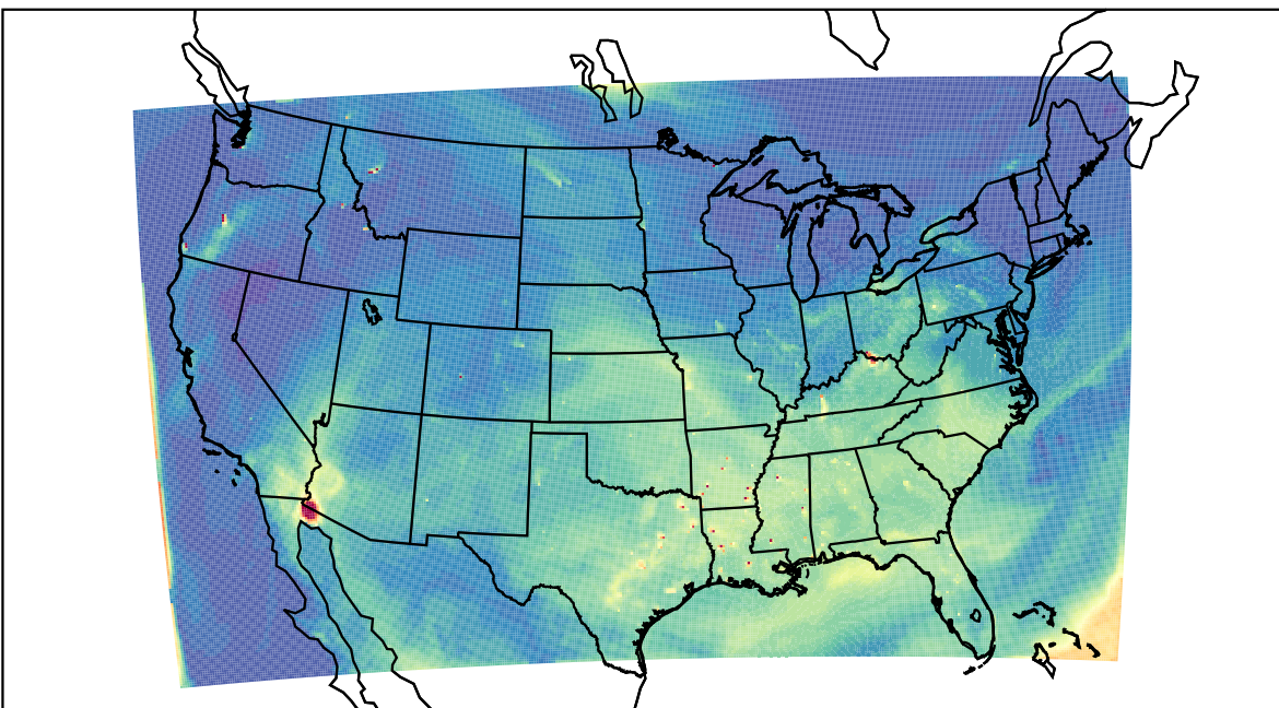
WRF 2023-07-30_21:00:00
