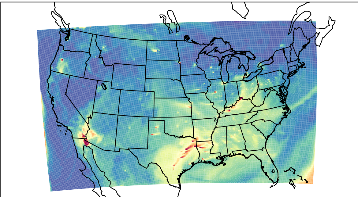
WRF 2023-07-30_14:00:00
