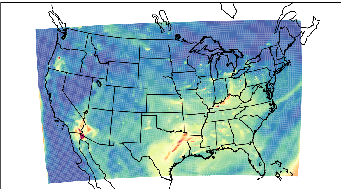
WRF 2023-07-30_13:00:00
