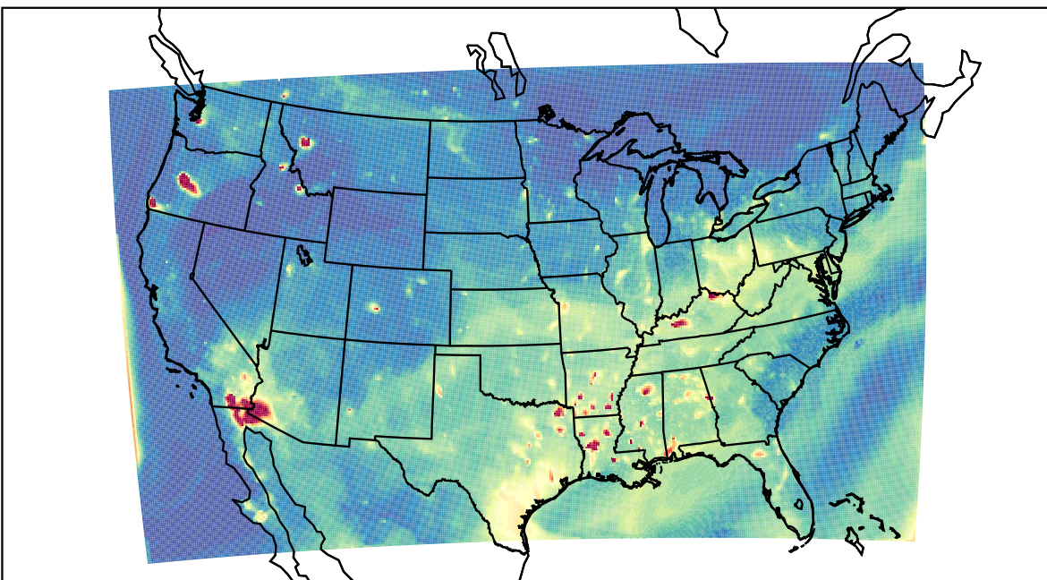
WRF 2023-07-30_03:00:00
