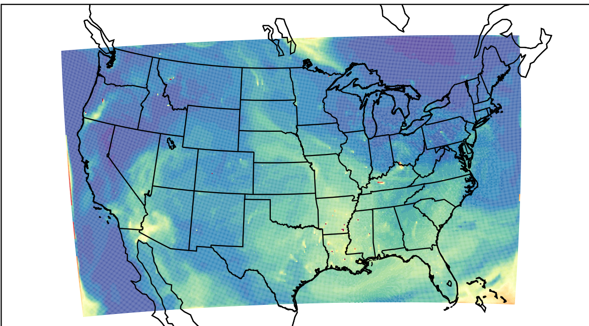
WRF 2023-07-31_20:00:00
