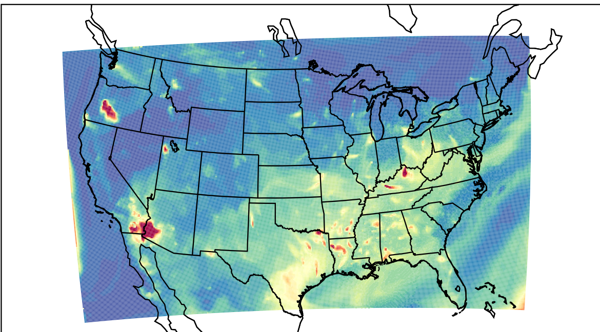
WRF 2023-07-30_06:00:00
