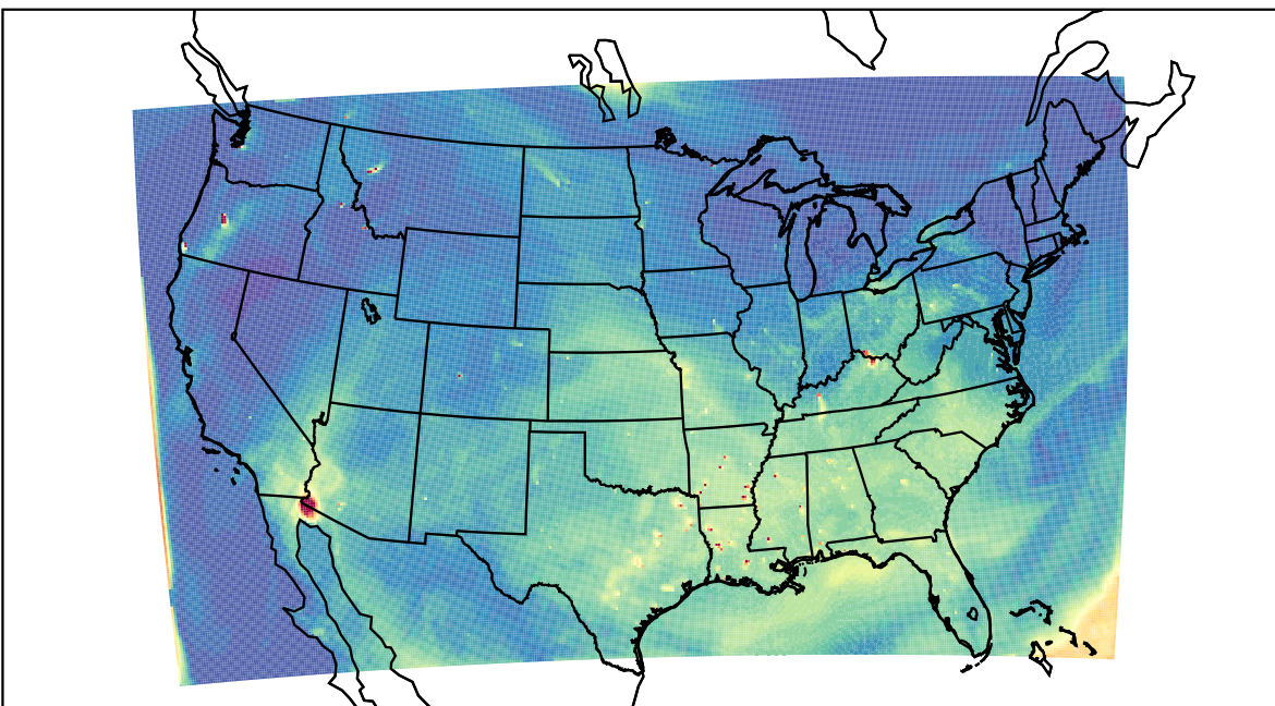
WRF 2023-07-30_22:00:00
