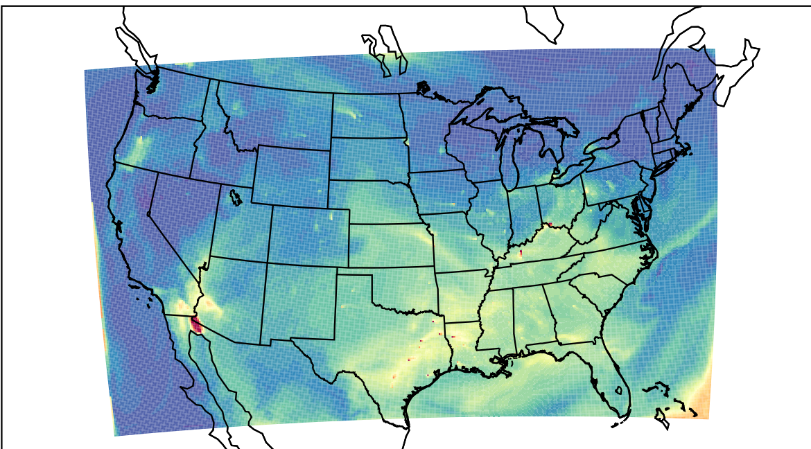
WRF 2023-07-30_17:00:00
