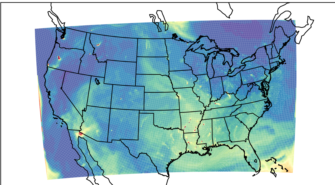
WRF 2023-07-31_23:00:00
