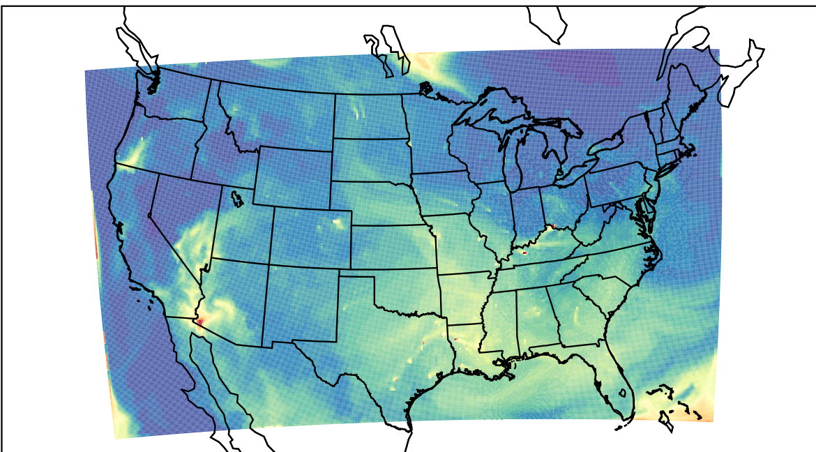
WRF 2023-07-31_17:00:00
