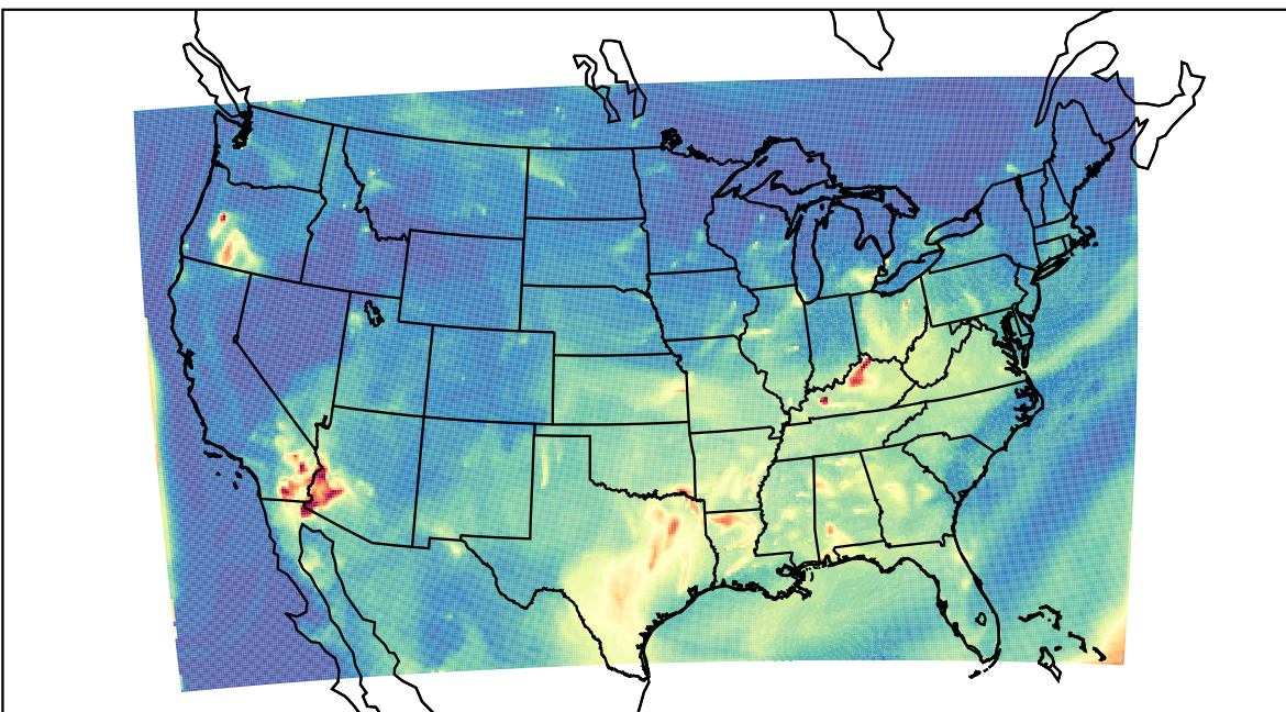
WRF 2023-07-30_09:00:00
