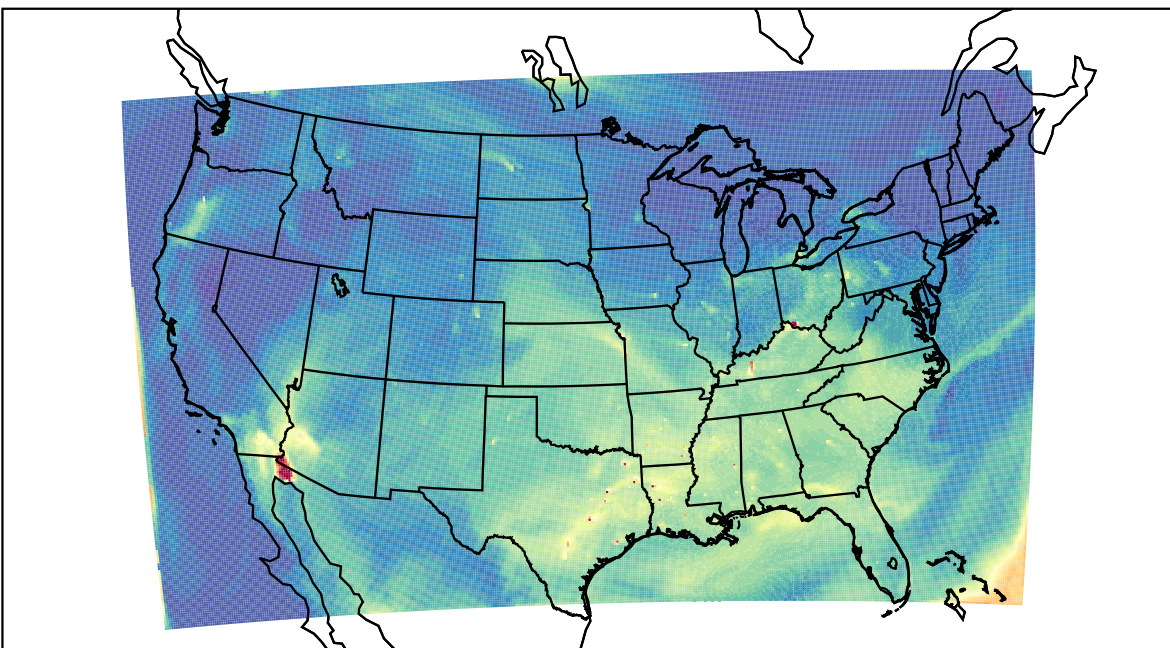
WRF 2023-07-30_18:00:00
