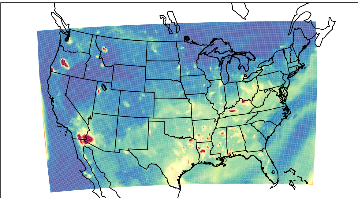
WRF 2023-07-30_04:00:00
