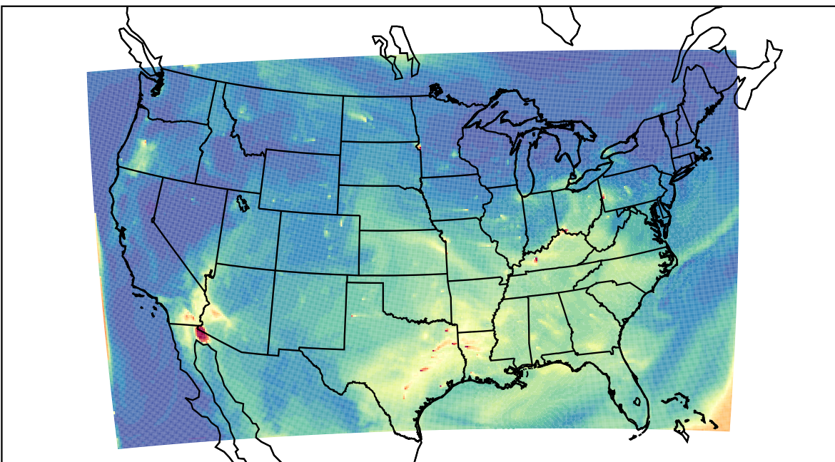
WRF 2023-07-30_16:00:00
