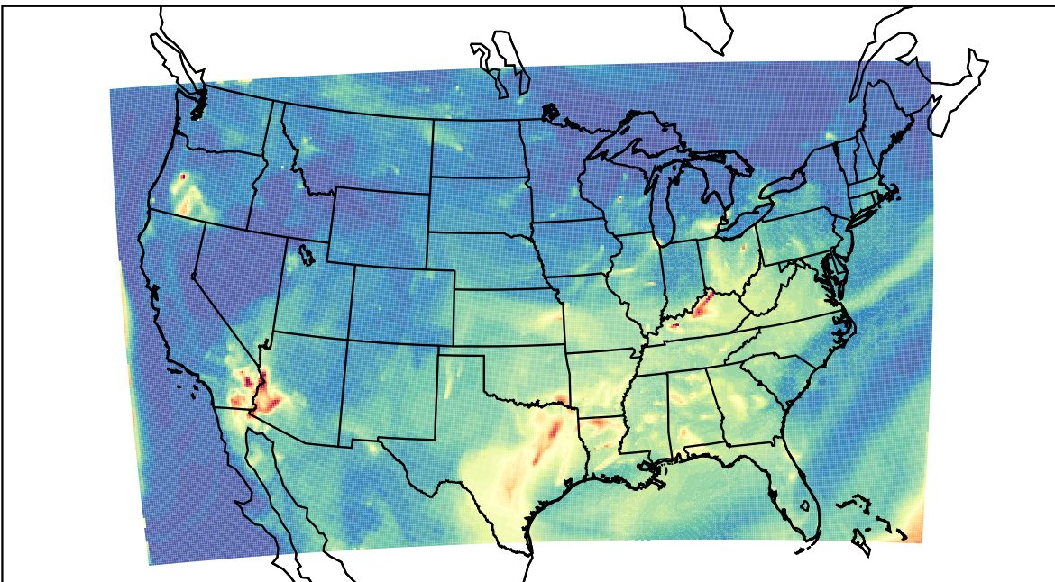
WRF 2023-07-30_10:00:00
