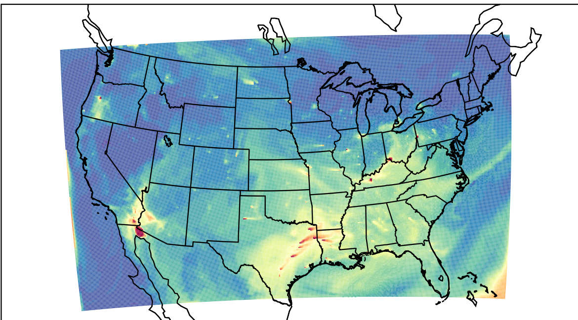
WRF 2023-07-30_15:00:00
