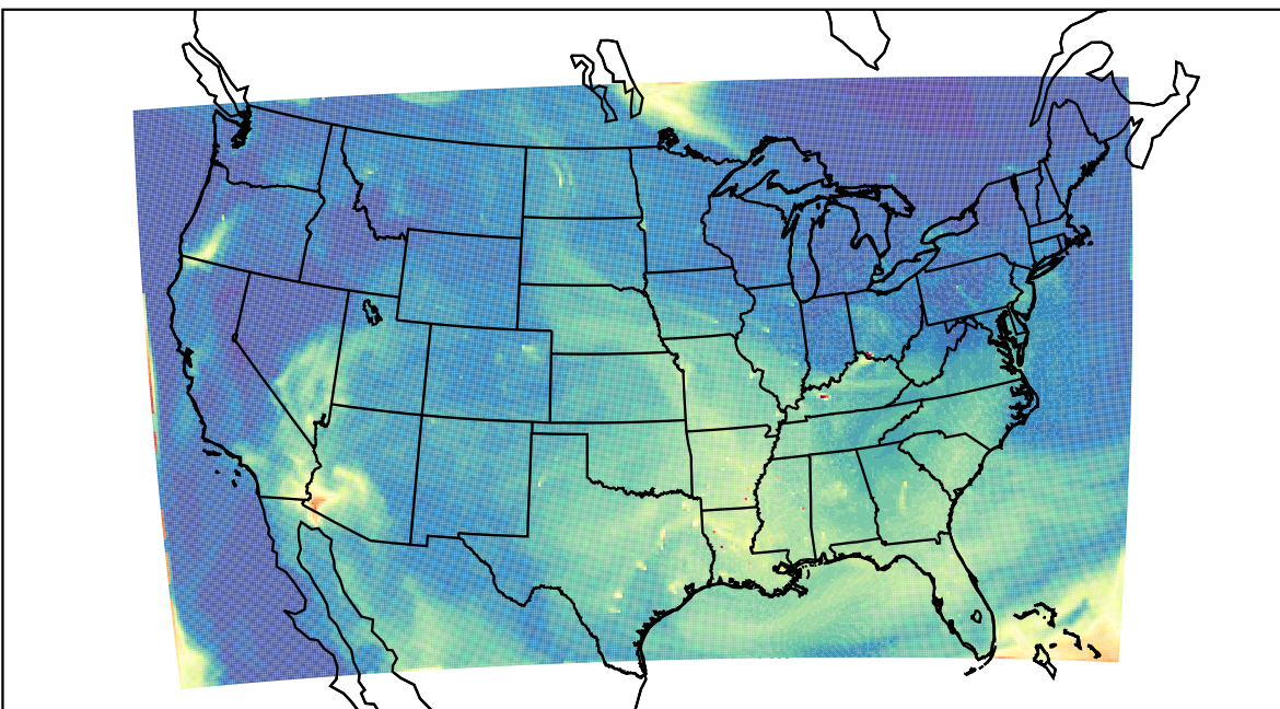
WRF 2023-07-31_18:00:00
