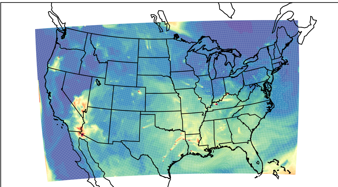
WRF 2023-07-31_15:00:00
