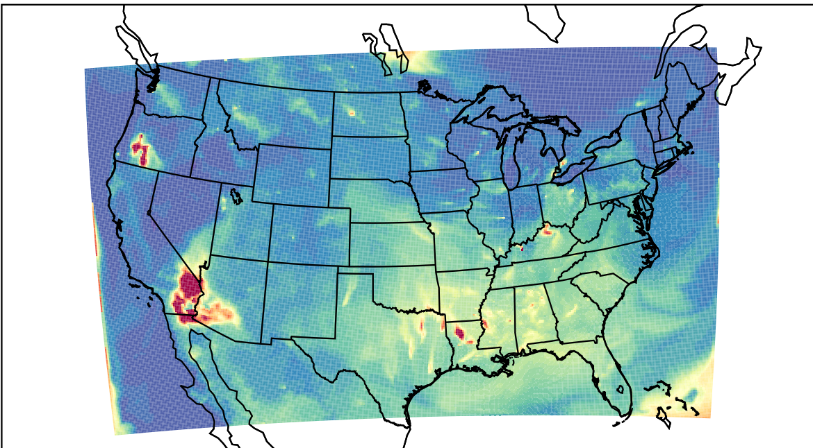
WRF 2023-07-31_08:00:00
