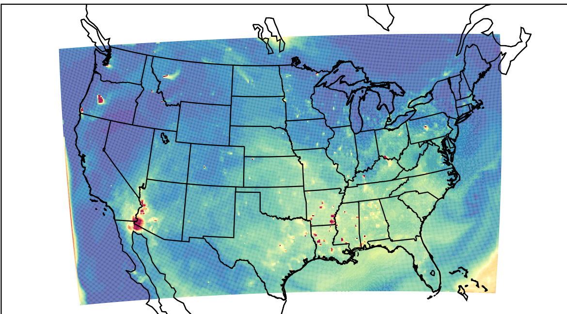
WRF 2023-07-31_01:00:00
