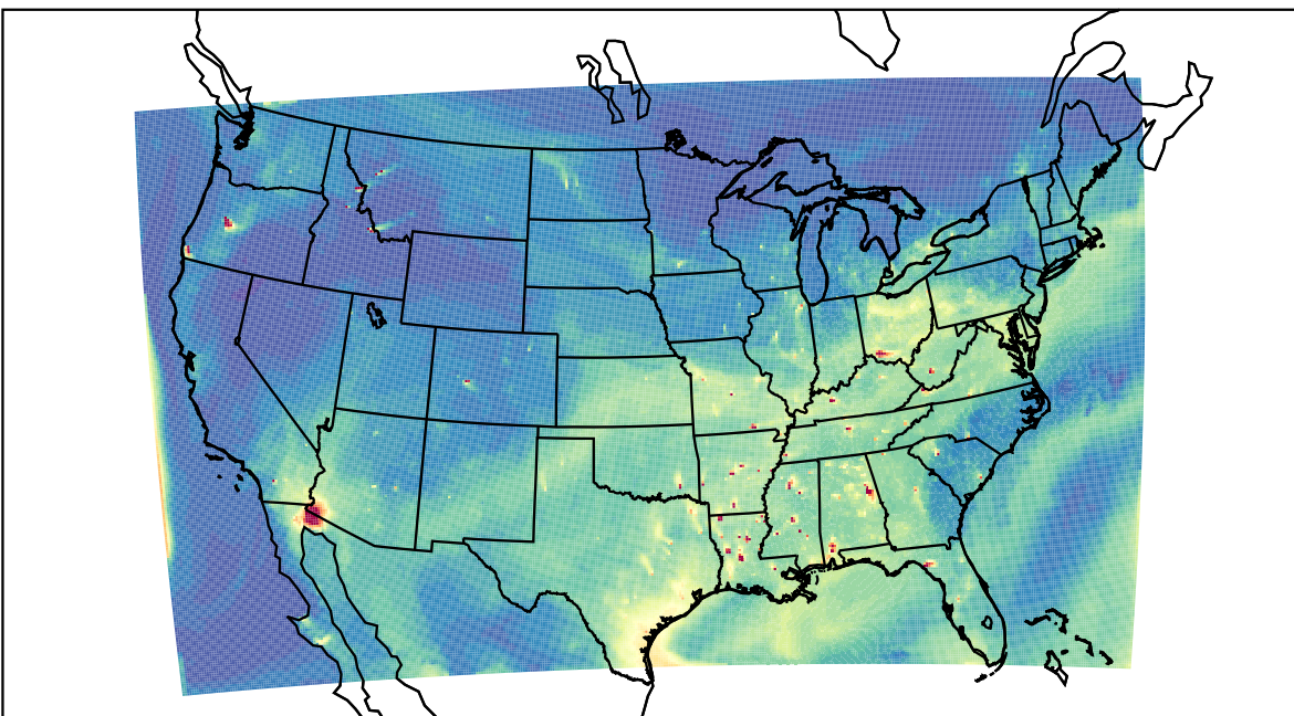
WRF 2023-07-30_00:00:00
