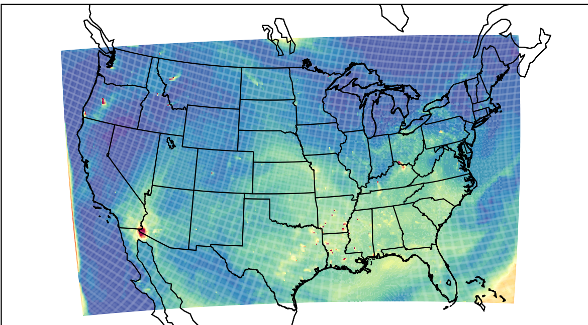
WRF 2023-07-30_23:00:00
