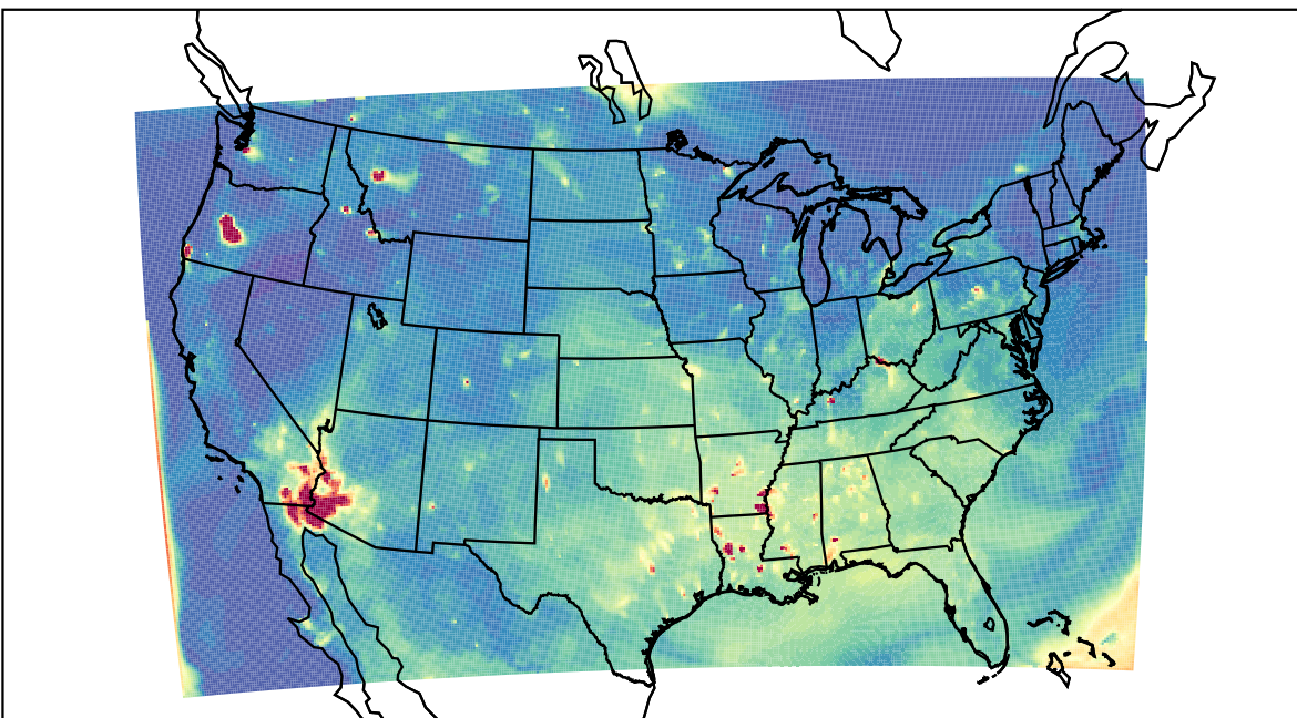
WRF 2023-07-31_03:00:00
