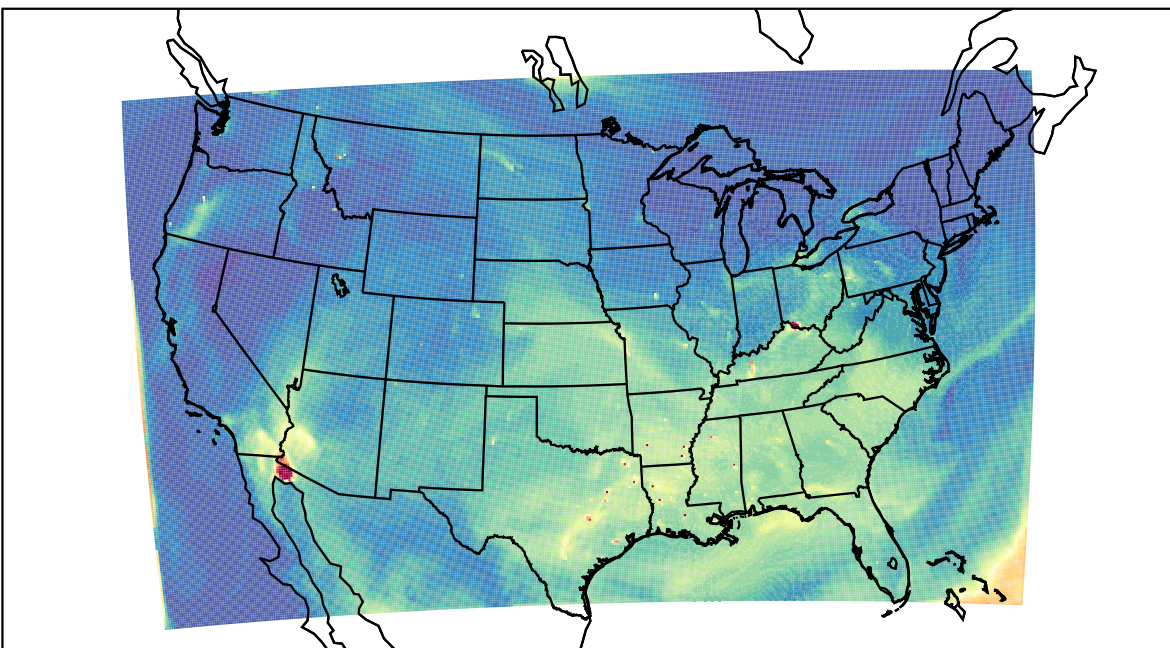
WRF 2023-07-30_19:00:00
