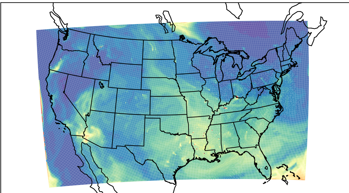
WRF 2023-07-31_19:00:00
