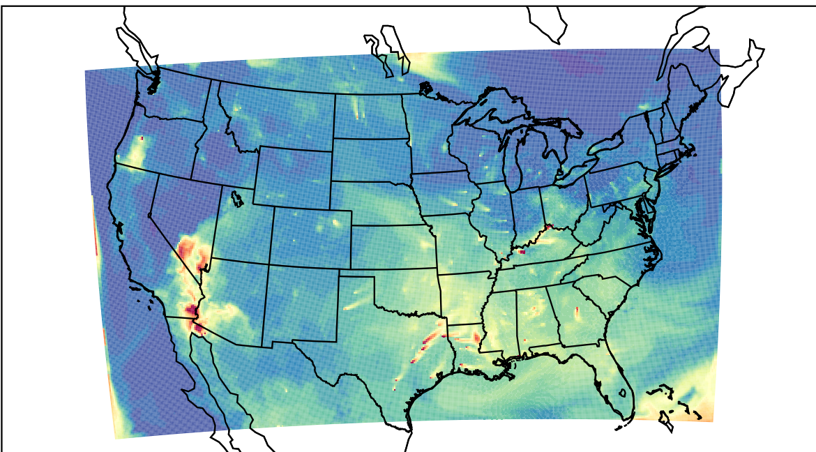
WRF 2023-07-31_14:00:00
