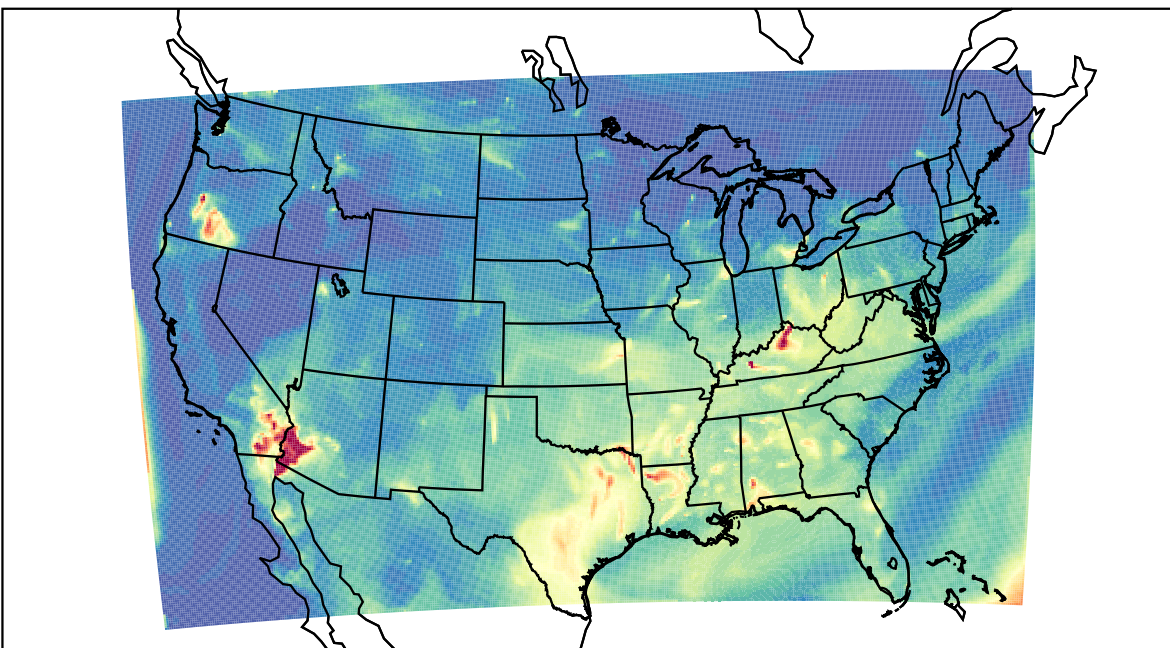
WRF 2023-07-30_08:00:00
