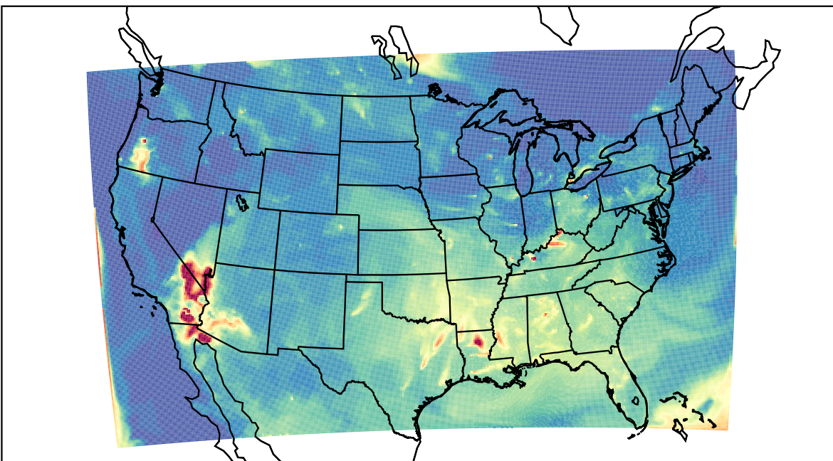
WRF 2023-07-31_11:00:00
