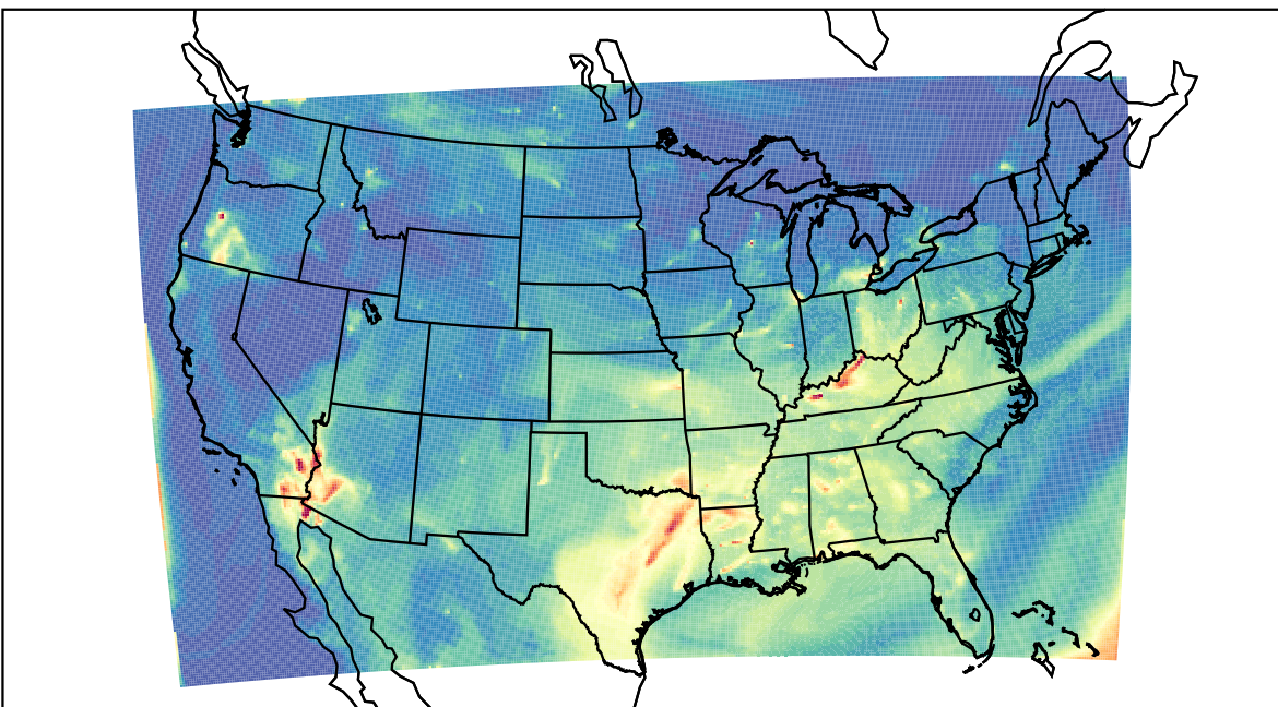
WRF 2023-07-30_11:00:00
