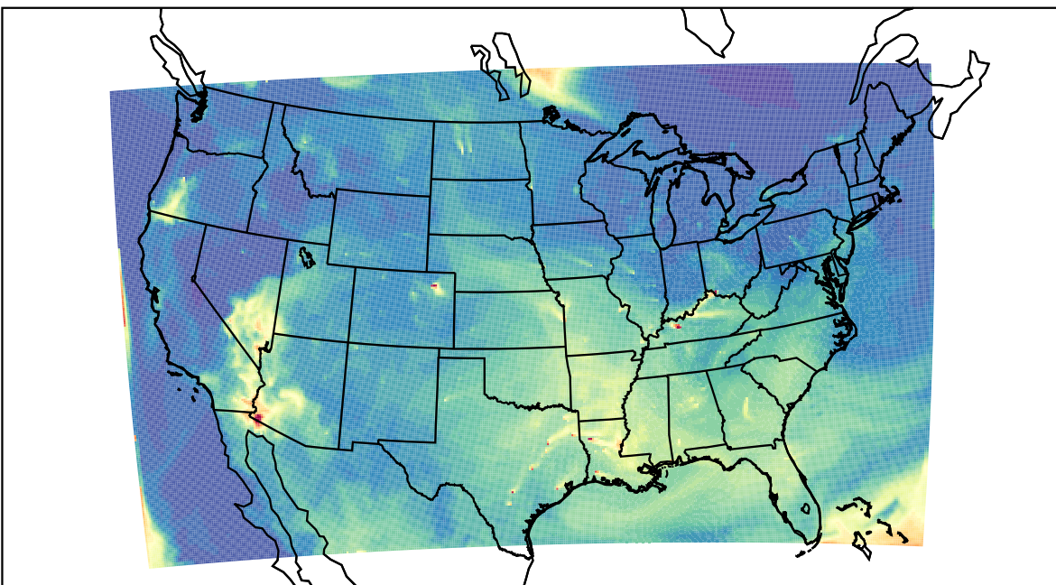
WRF 2023-07-31_16:00:00
