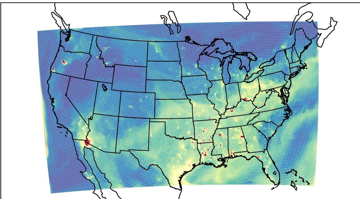
WRF 2023-07-30_01:00:00
