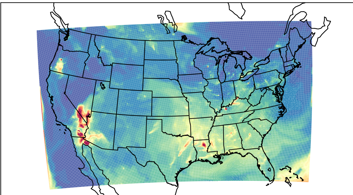
WRF 2023-07-31_12:00:00
