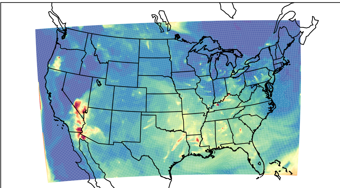
WRF 2023-07-31_13:00:00
