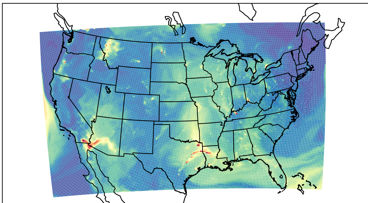
WRF 2023-08-02_15:00:00
