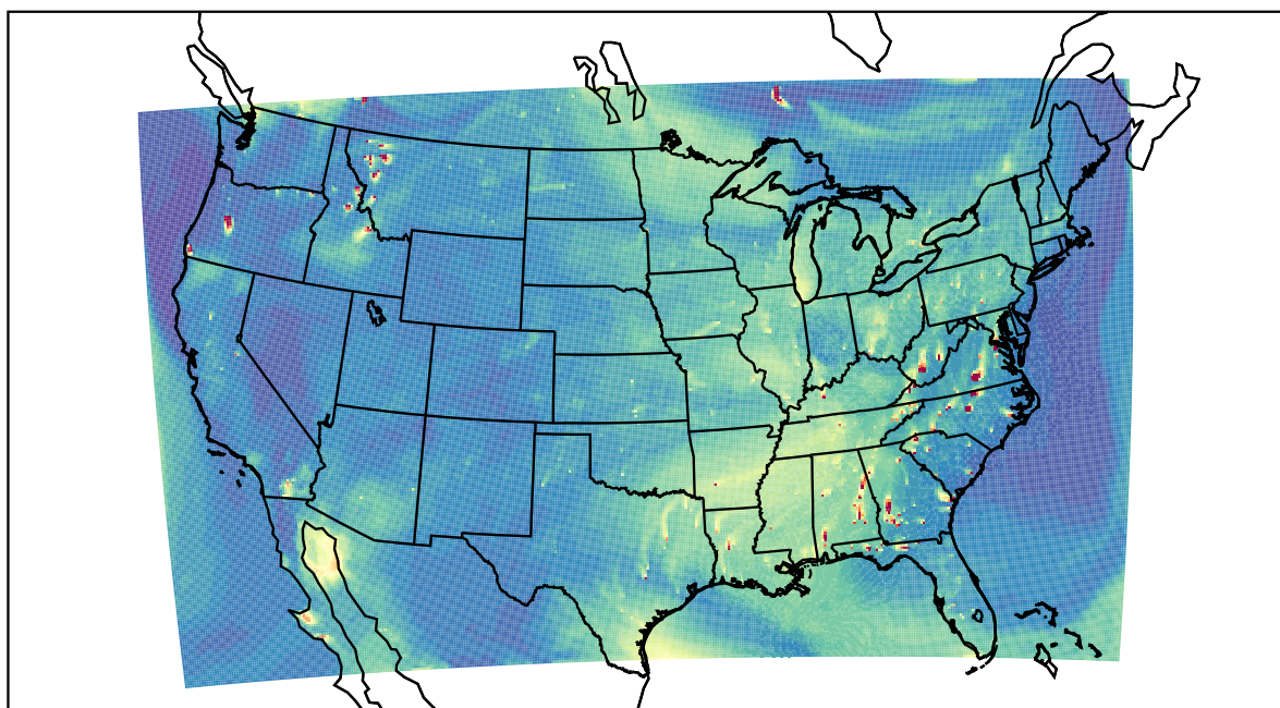
WRF 2023-08-03_23:00:00
