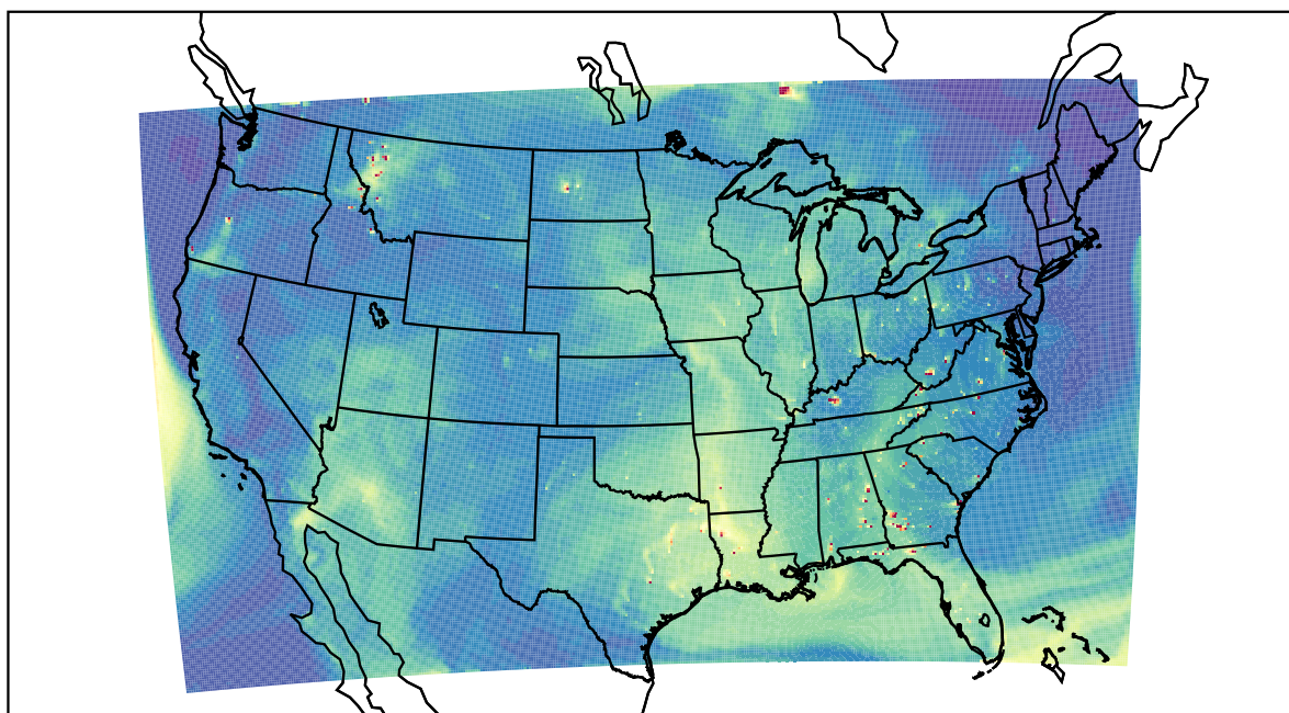
WRF 2023-08-02_20:00:00
