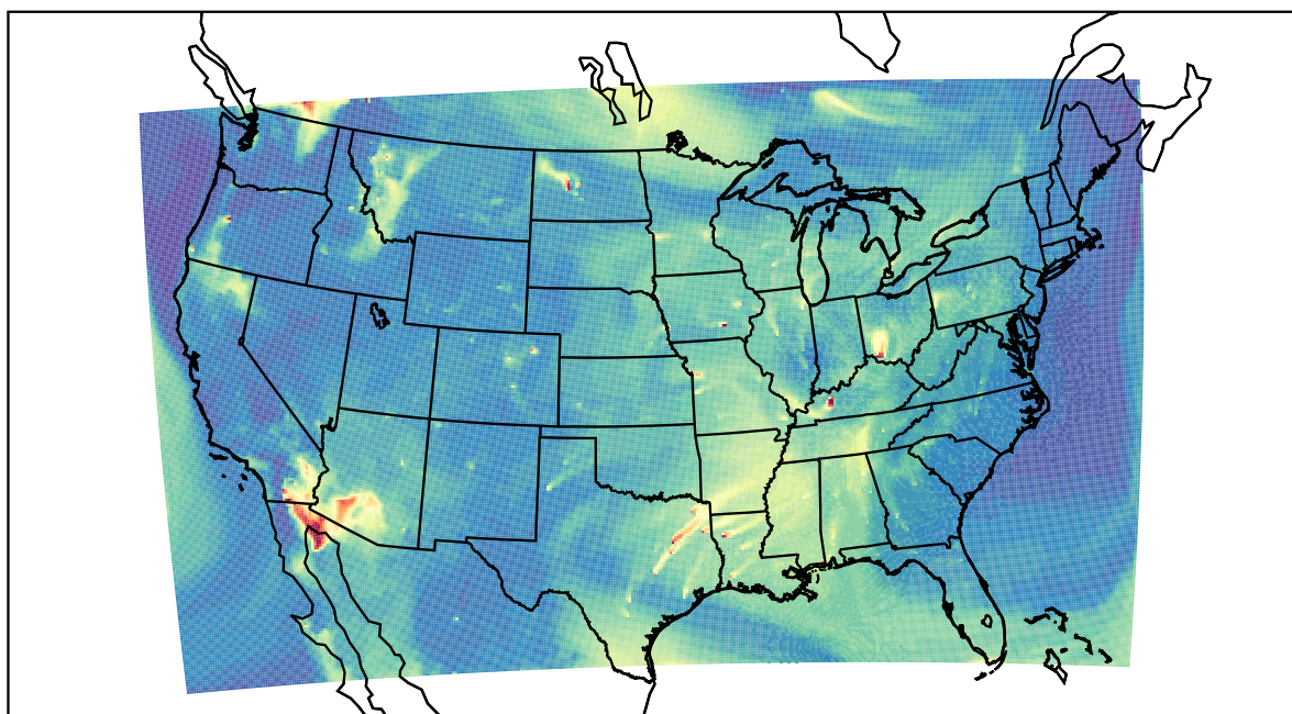
WRF 2023-08-03_15:00:00
