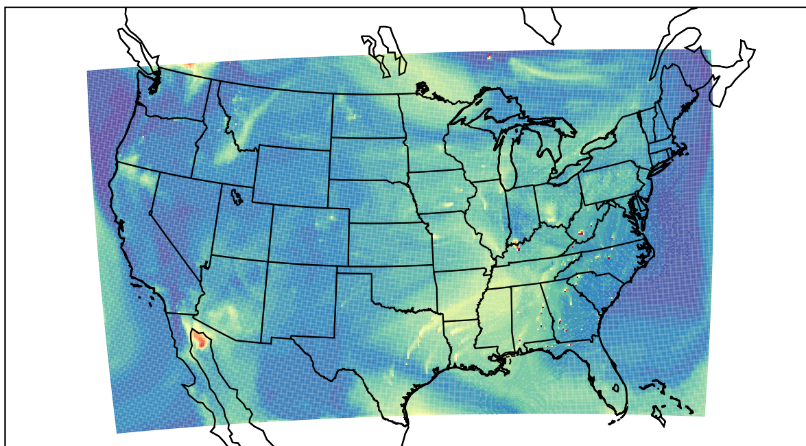
WRF 2023-08-03_18:00:00
