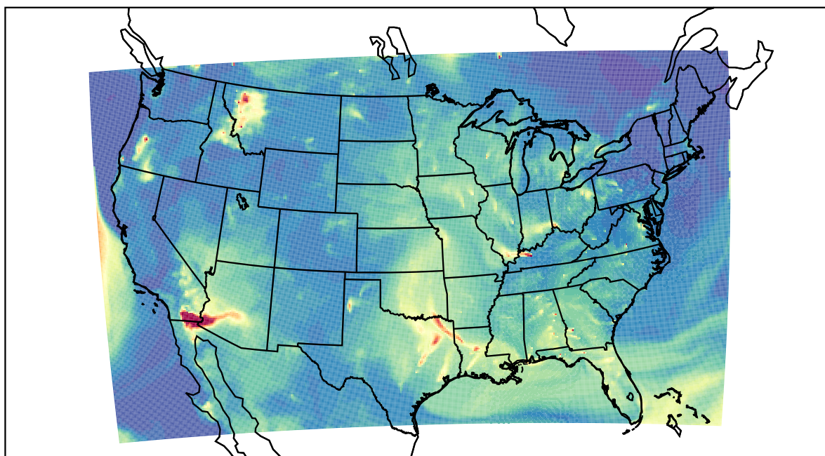
WRF 2023-08-02_10:00:00
