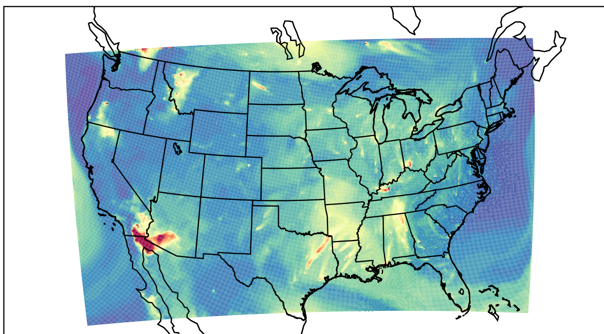
WRF 2023-08-03_12:00:00
