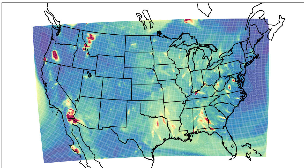
WRF 2023-08-03_04:00:00
