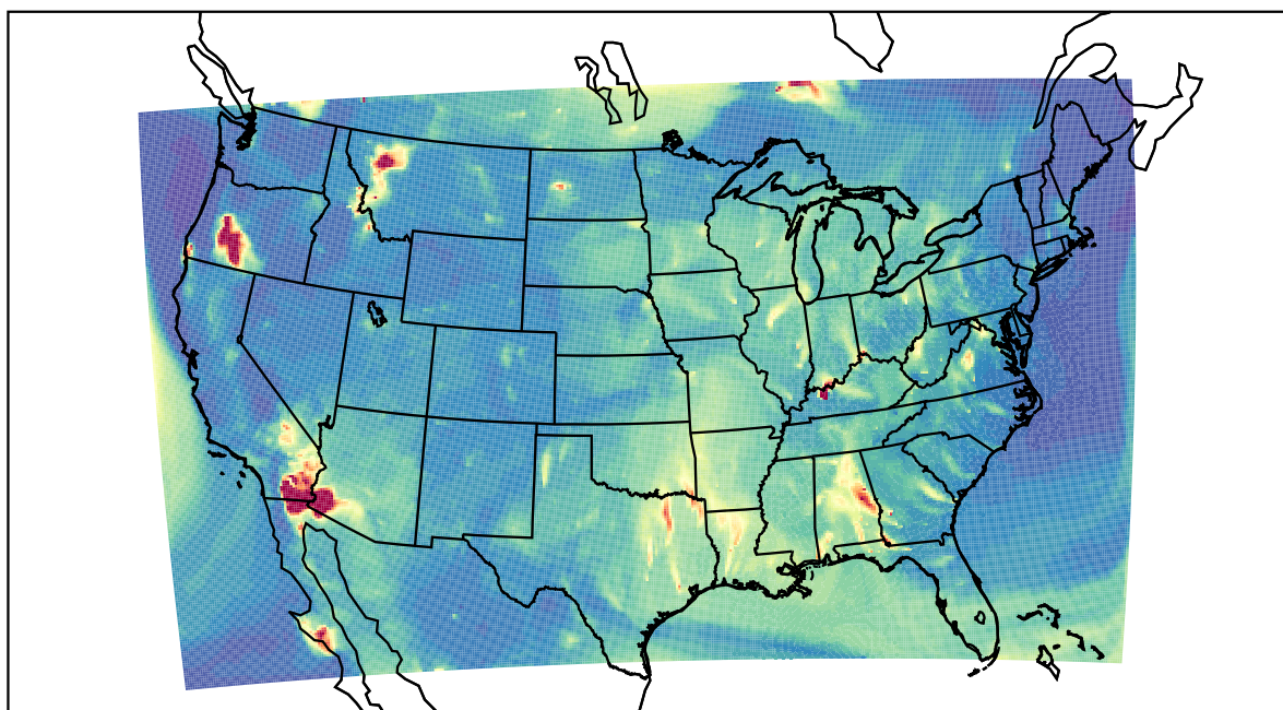
WRF 2023-08-03_06:00:00
