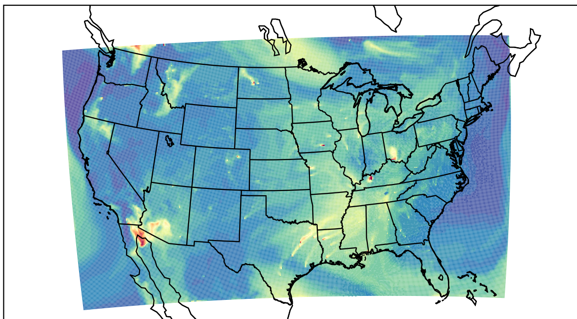
WRF 2023-08-03_16:00:00
