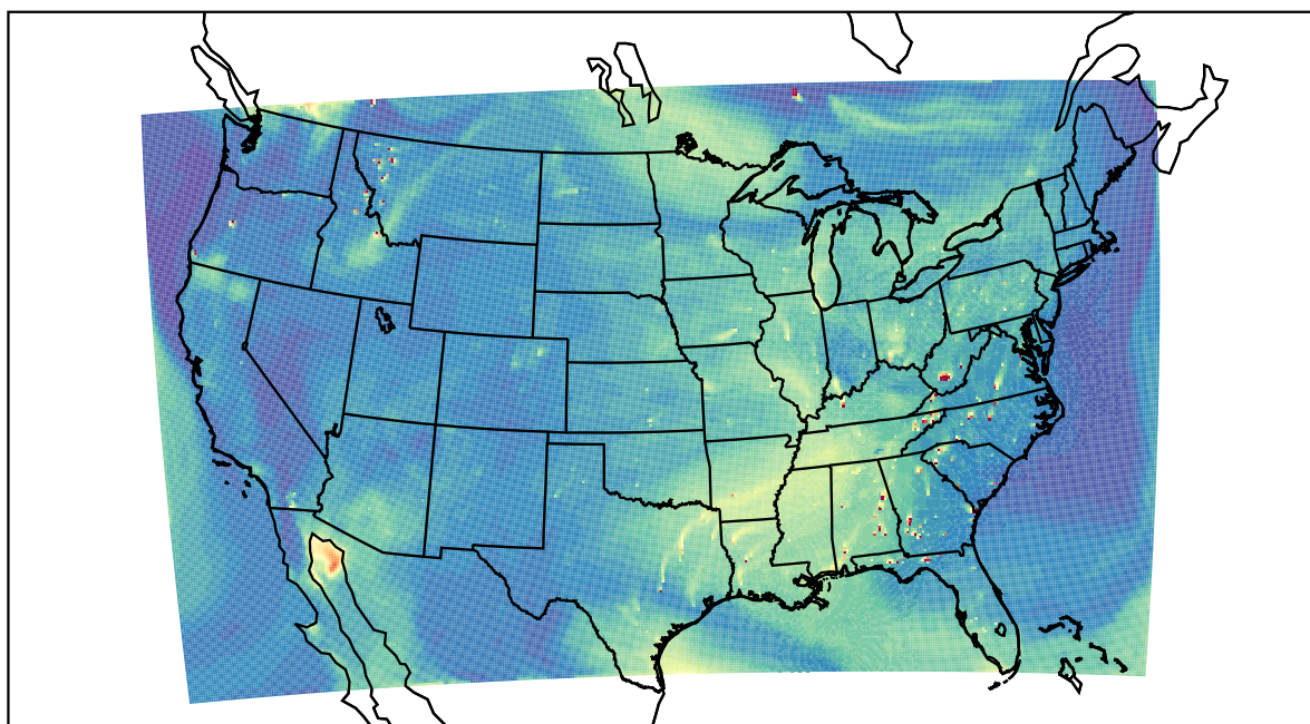
WRF 2023-08-03_20:00:00
