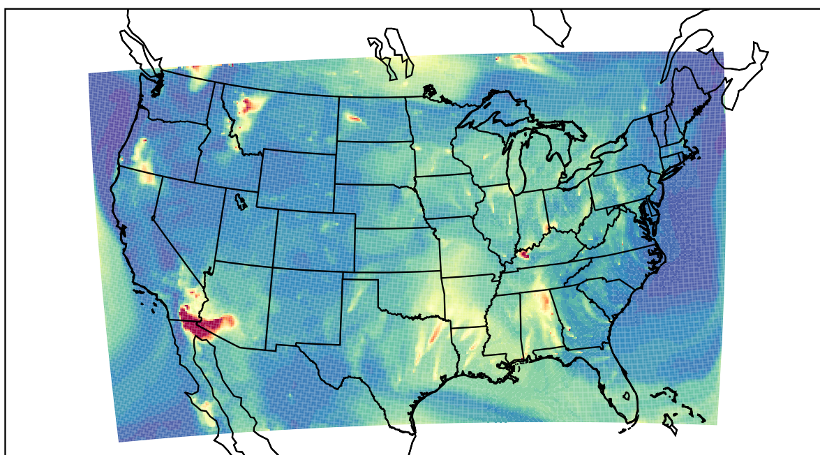
WRF 2023-08-03_10:00:00
