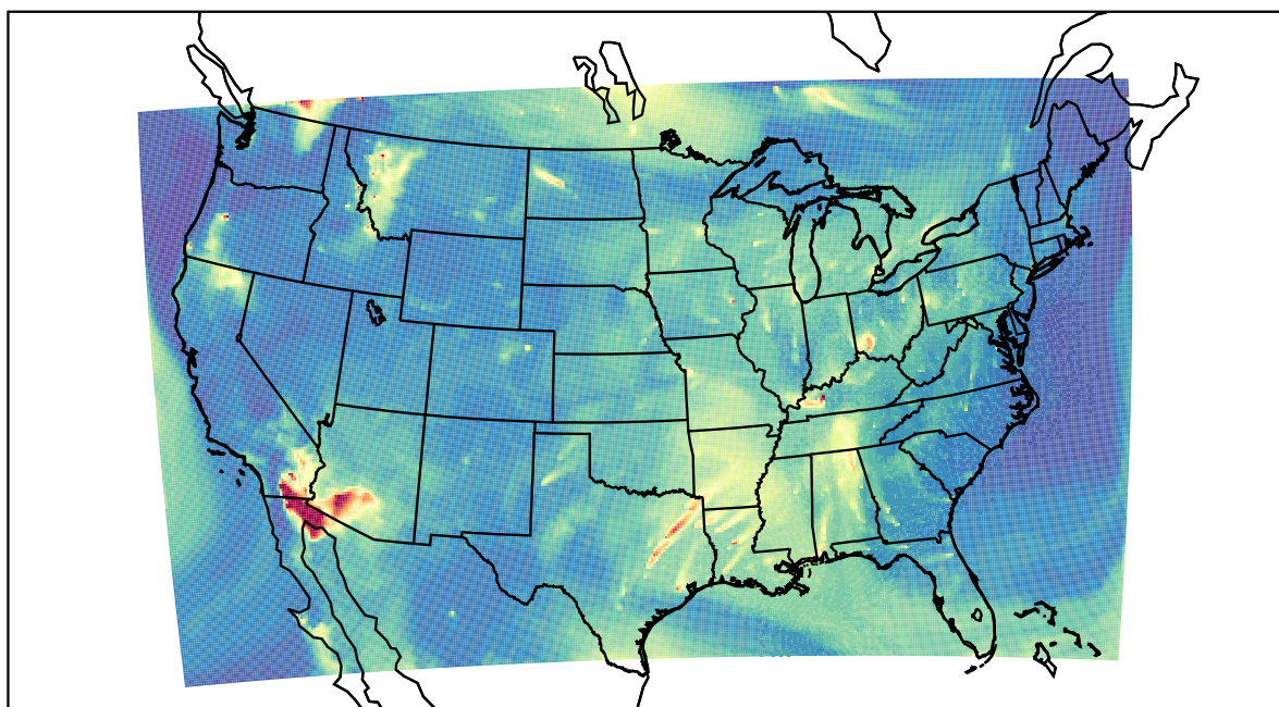
WRF 2023-08-03_13:00:00
