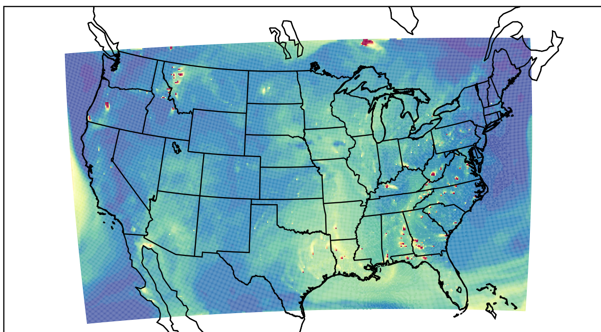
WRF 2023-08-02_23:00:00
