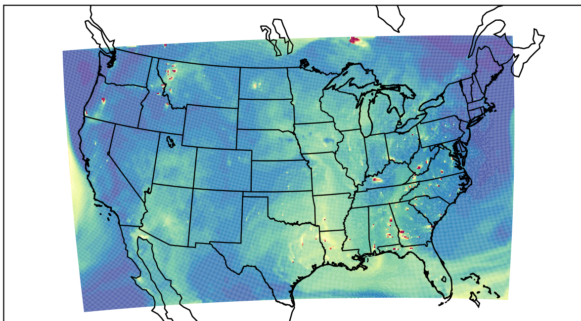
WRF 2023-08-02_22:00:00
