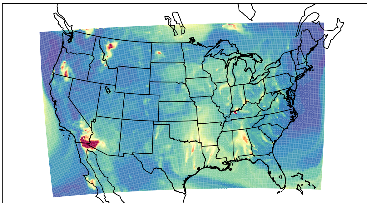
WRF 2023-08-03_08:00:00
