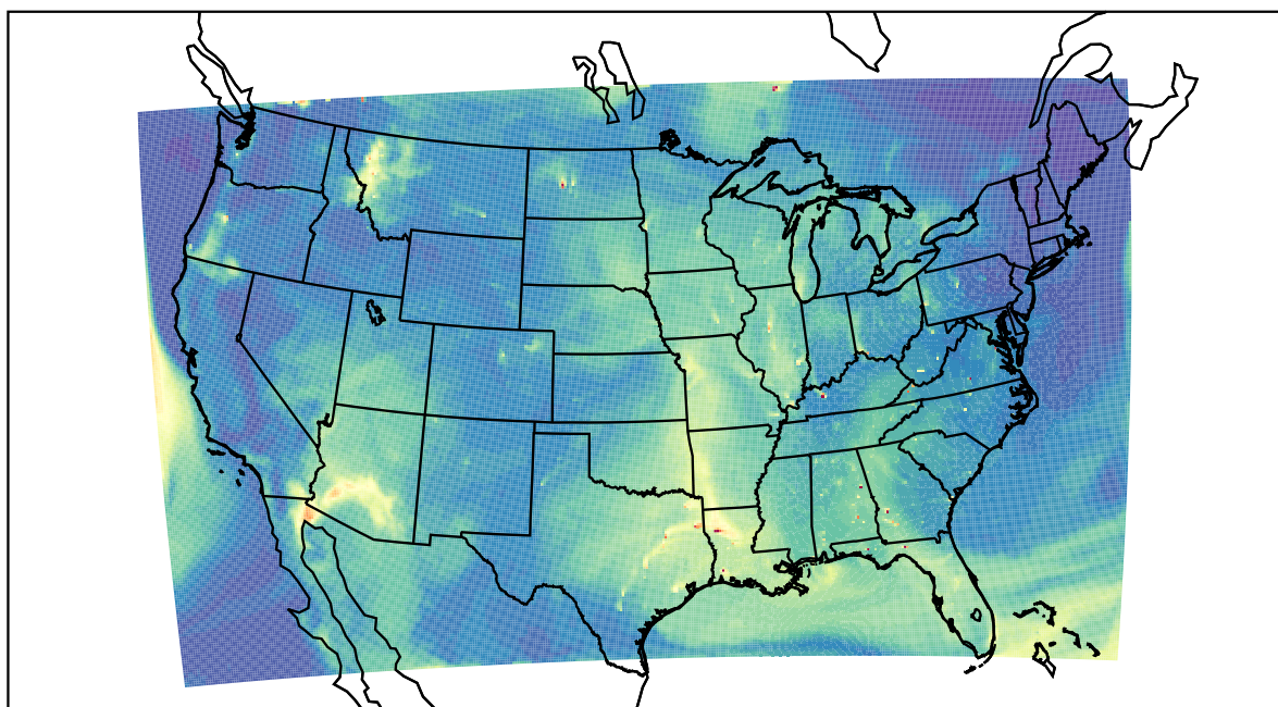
WRF 2023-08-02_17:00:00
