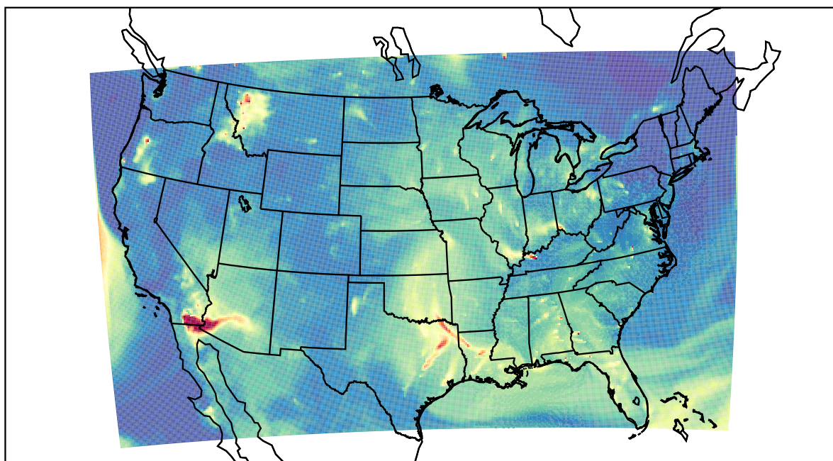
WRF 2023-08-02_11:00:00
