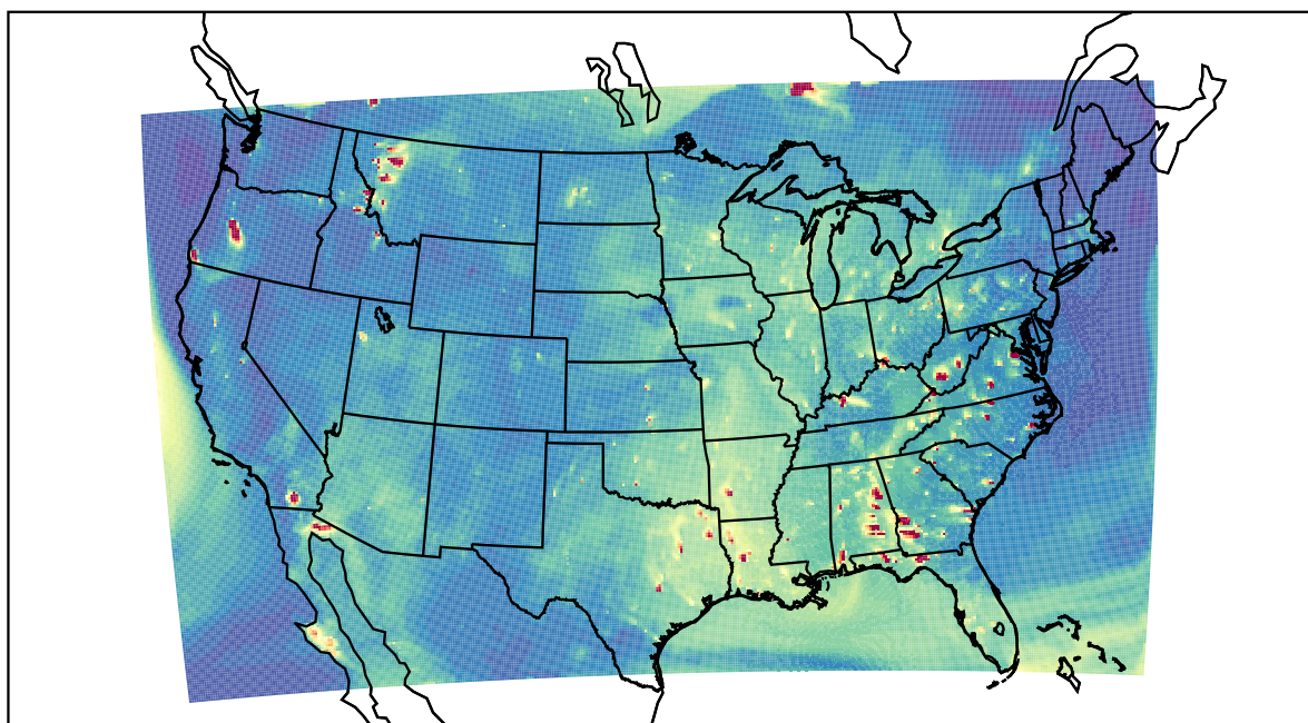
WRF 2023-08-03_01:00:00
