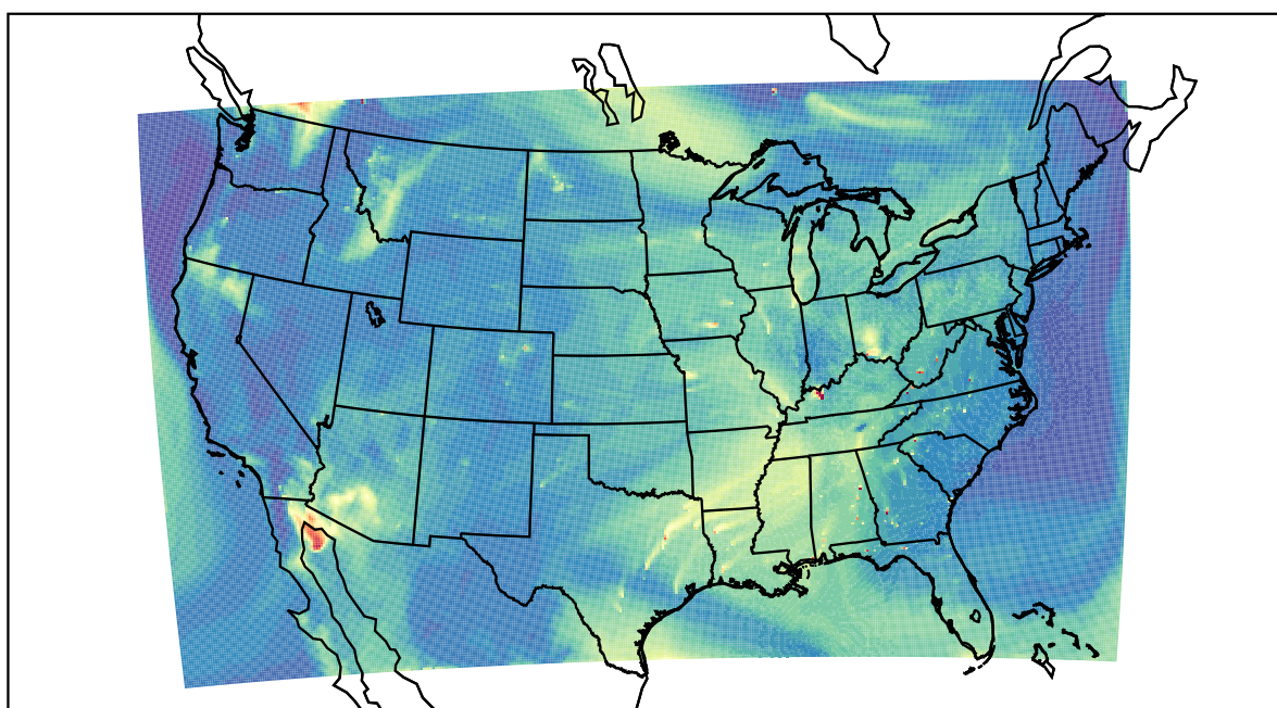
WRF 2023-08-03_17:00:00
