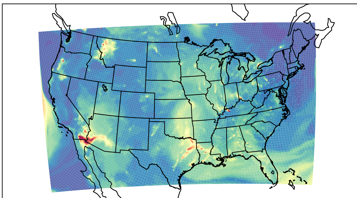
WRF 2023-08-02_13:00:00
