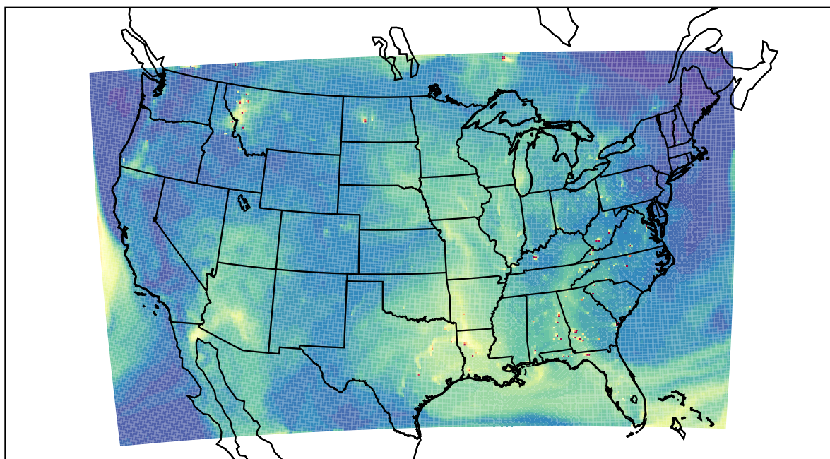
WRF 2023-08-02_19:00:00
