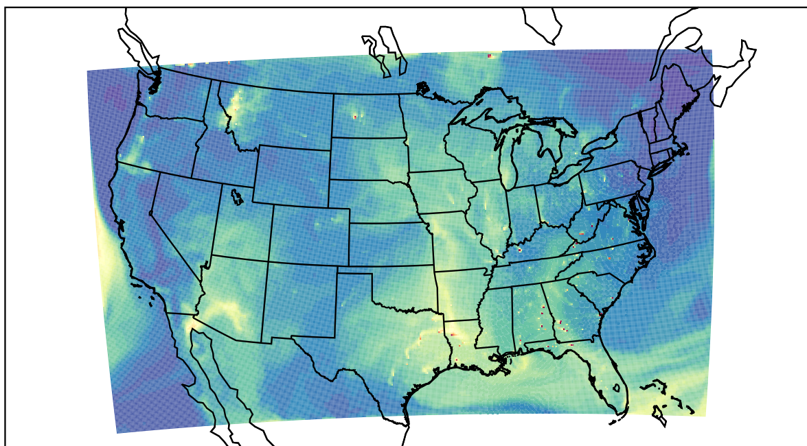
WRF 2023-08-02_18:00:00
