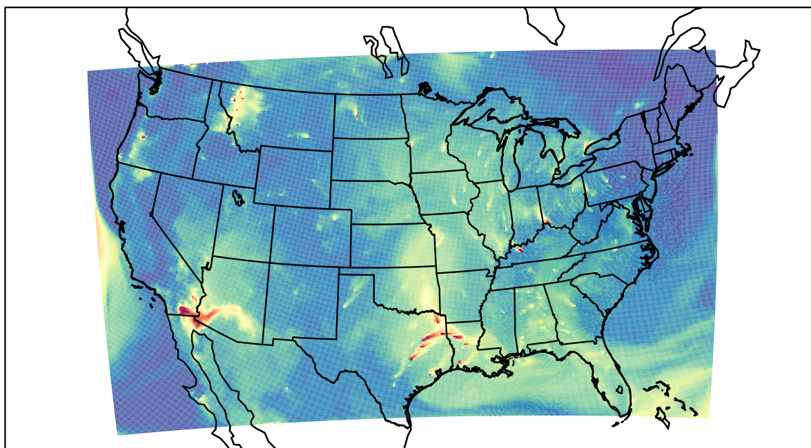
WRF 2023-08-02_14:00:00
