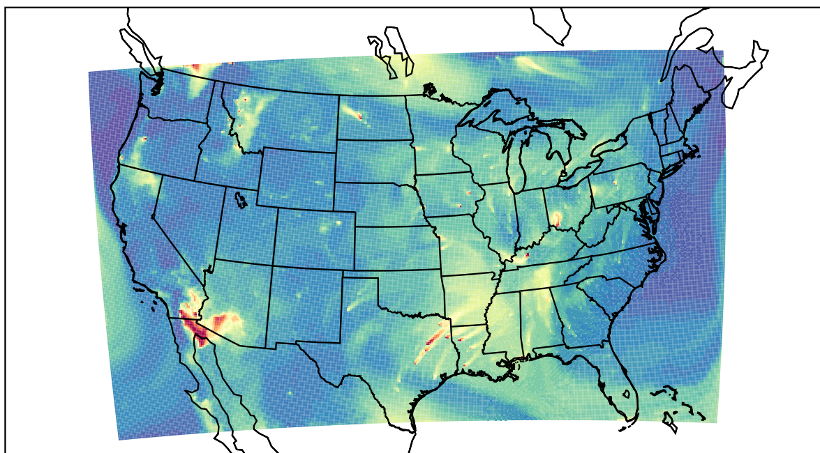
WRF 2023-08-03_14:00:00
