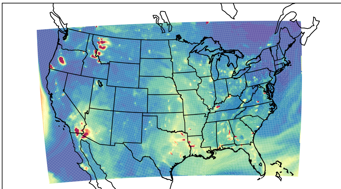
WRF 2023-08-02_03:00:00
