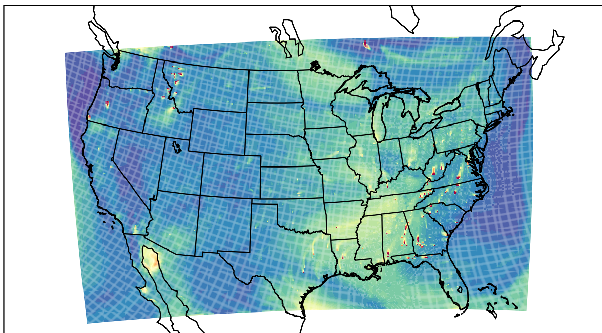
WRF 2023-08-03_22:00:00
