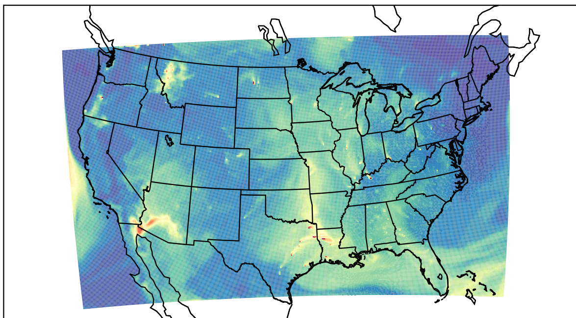
WRF 2023-08-02_16:00:00
