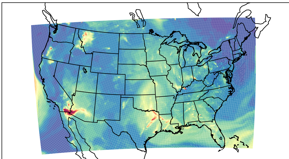
WRF 2023-08-02_12:00:00
