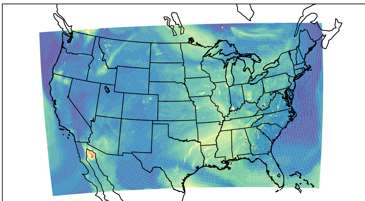
WRF 2023-08-03_19:00:00
