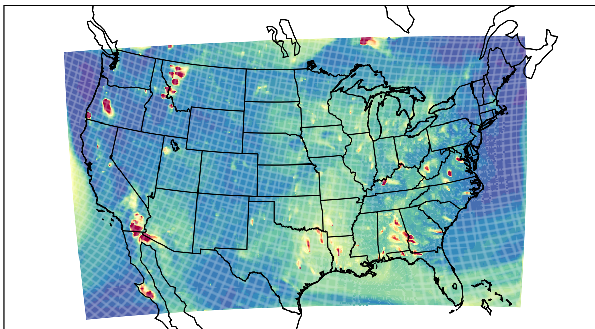
WRF 2023-08-03_03:00:00
