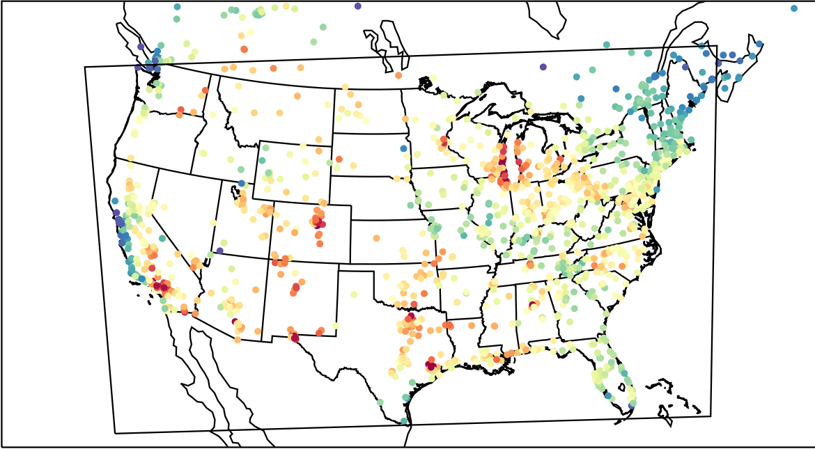
AirNOW (2023-08-02_20:00:00)
