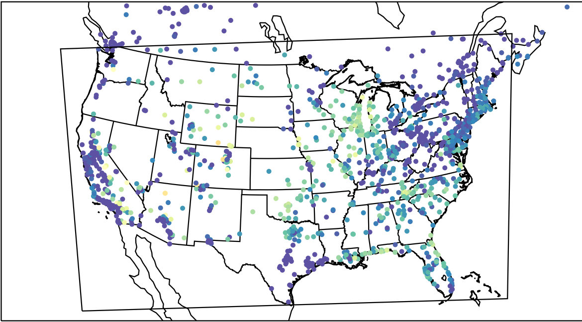
AirNOW (2023-08-02_13:00:00)
