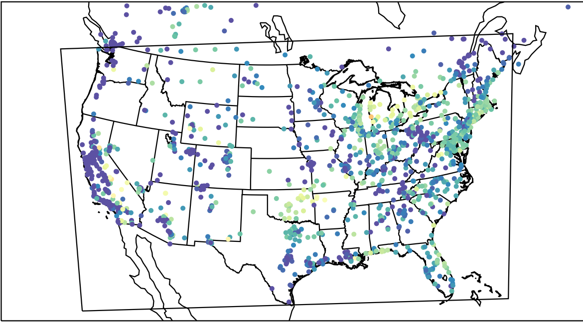
AirNOW (2023-08-03_13:00:00)
