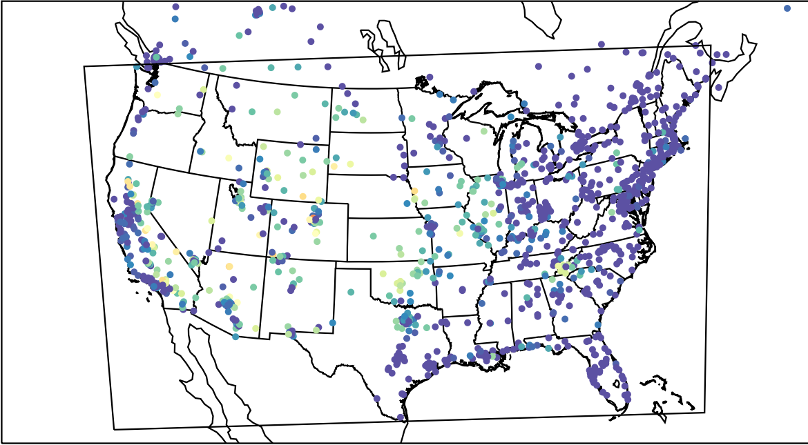
AirNOW (2023-08-02_10:00:00)
