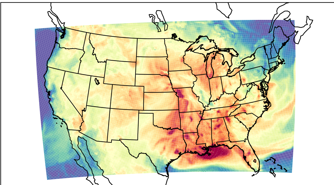
WRF (2023-08-02_18:00:00)
