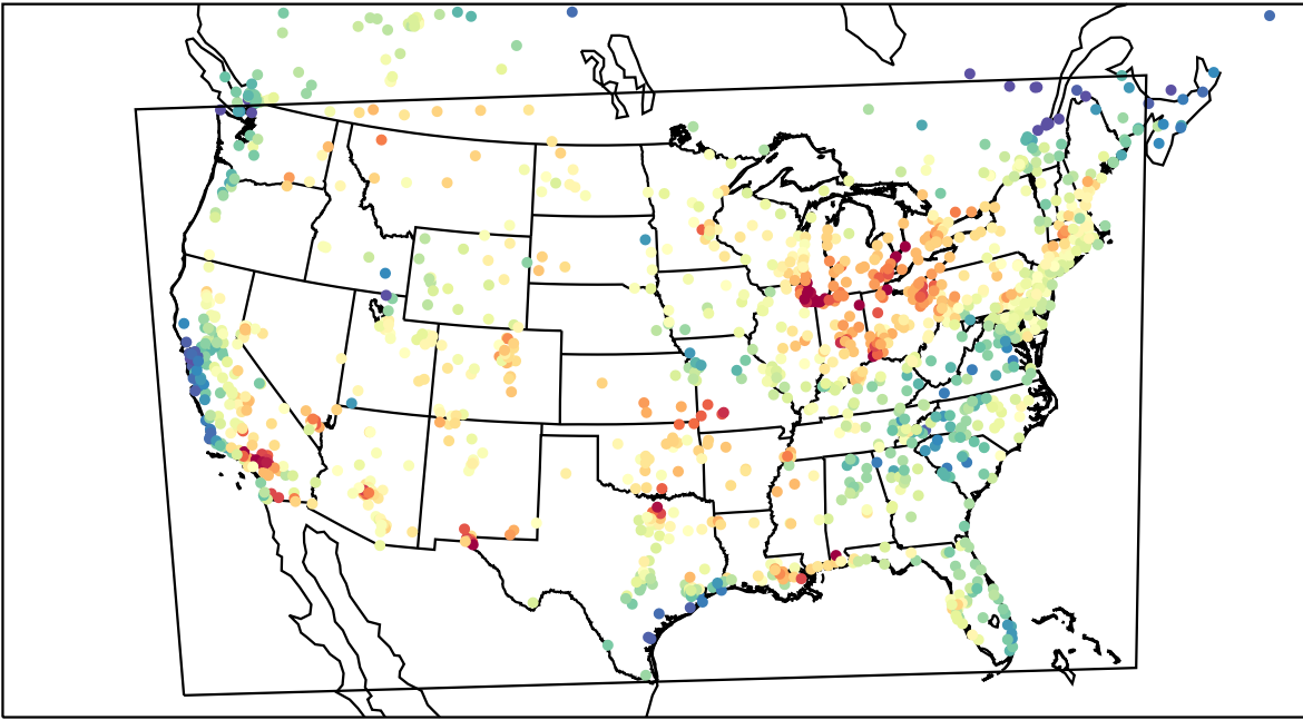
AirNOW (2023-08-03_20:00:00)
