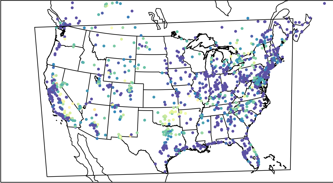
AirNOW (2023-08-03_10:00:00)
