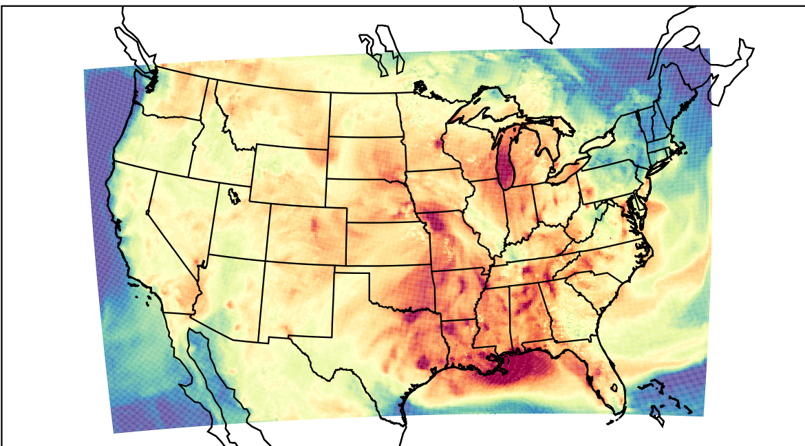
WRF (2023-08-02_20:00:00)
