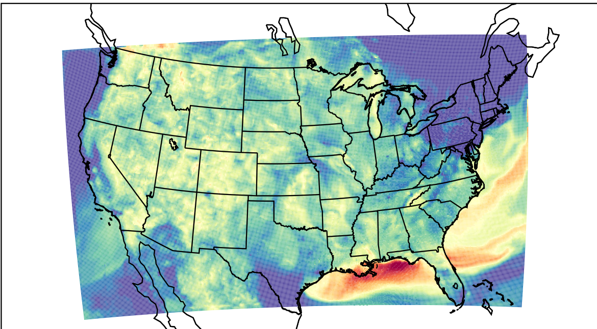
WRF (2023-08-02_10:00:00)
