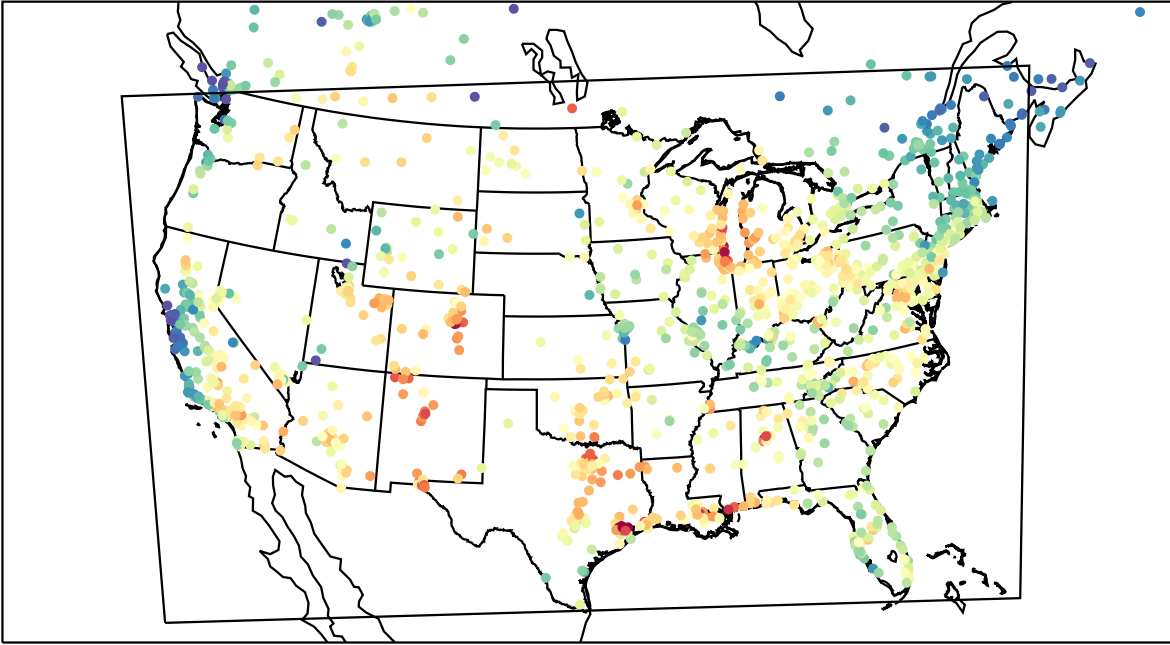
AirNOW (2023-08-02_18:00:00)
