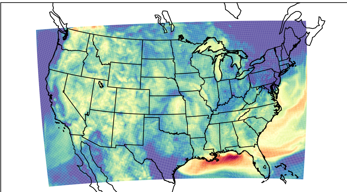
WRF (2023-08-02_13:00:00)
