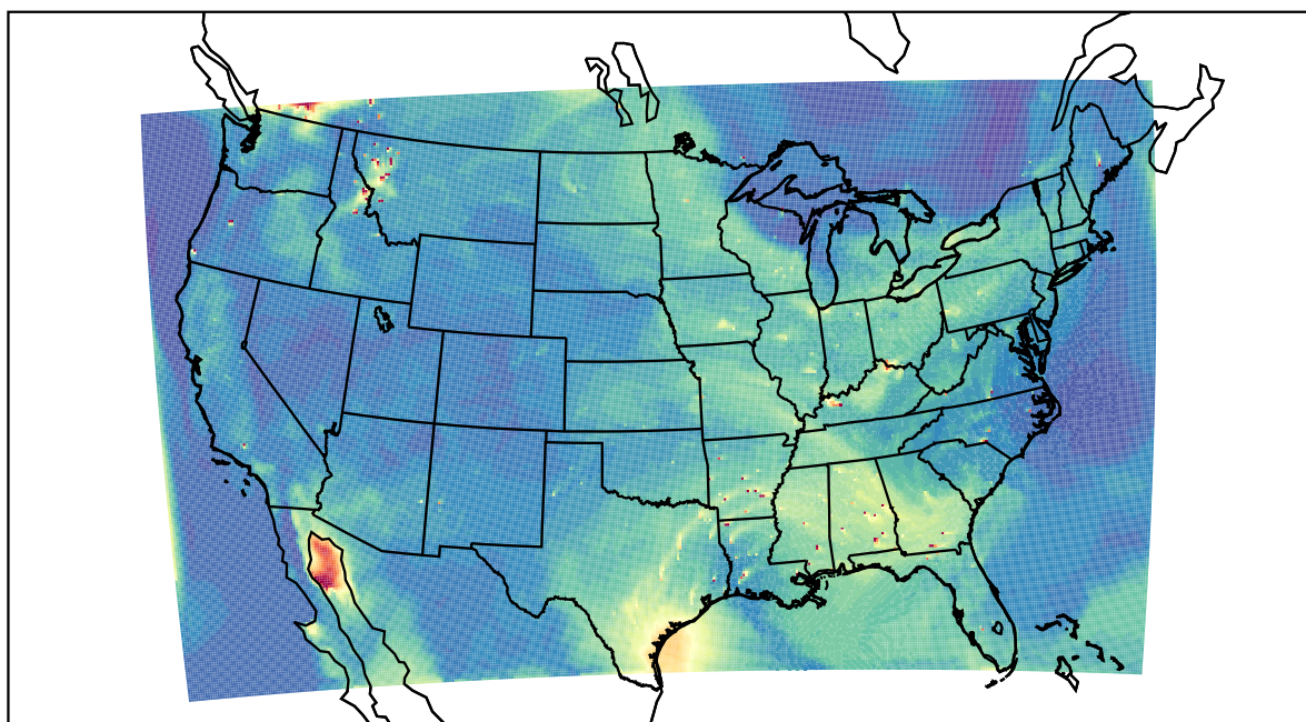
WRF 2023-08-04_20:00:00
