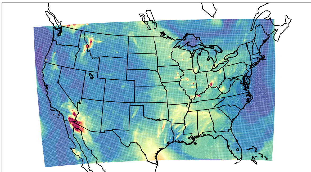
WRF 2023-08-04_10:00:00
