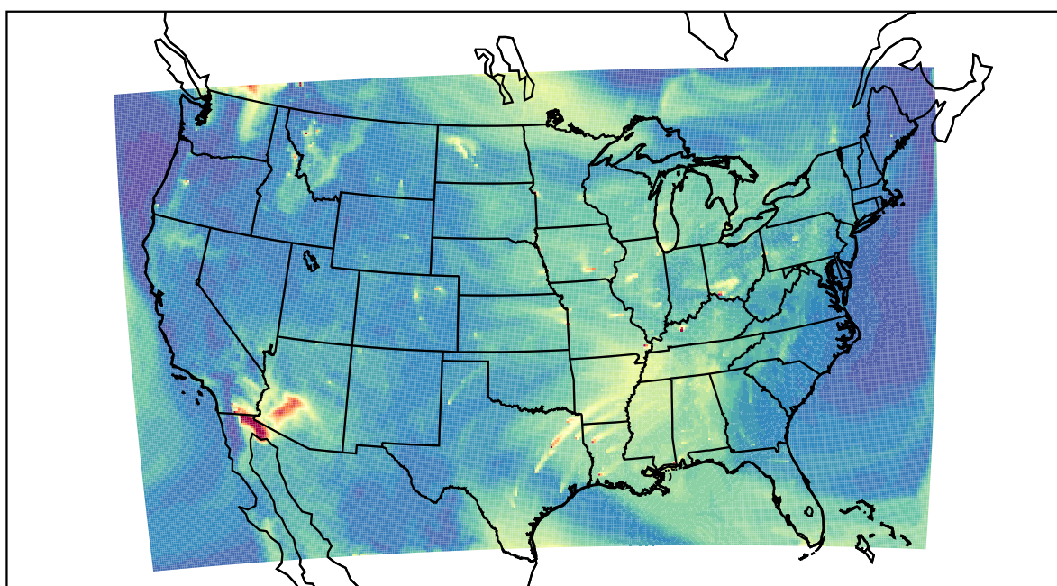
WRF 2023-08-03_16:00:00
