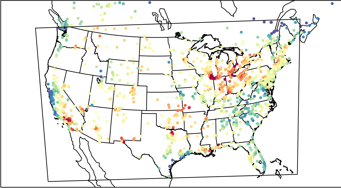
AirNOW (2023-08-03_20:00:00)
