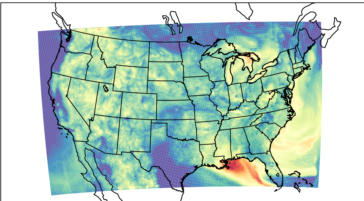
WRF (2023-08-03_13:00:00)
