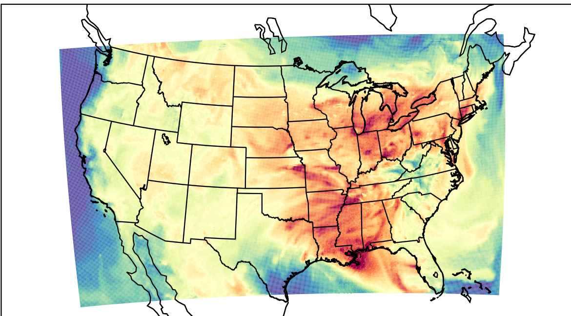
WRF (2023-08-03_18:00:00)
