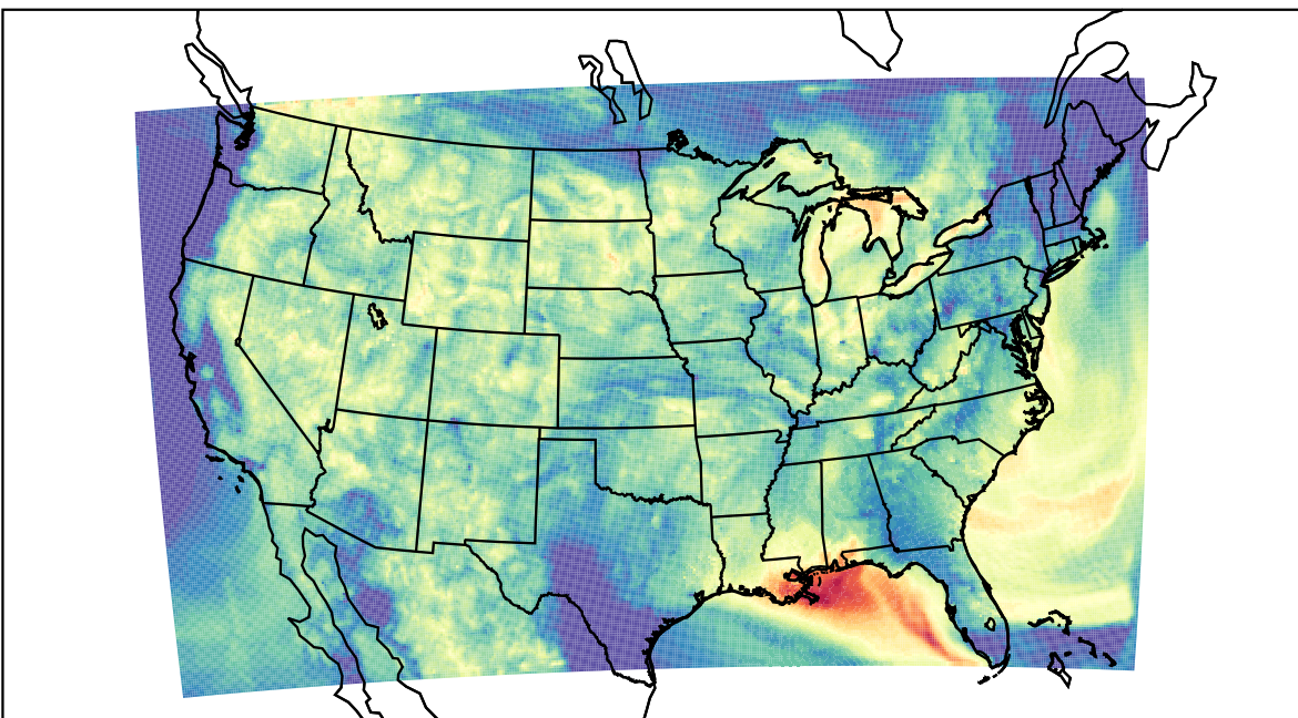
WRF (2023-08-03_10:00:00)
