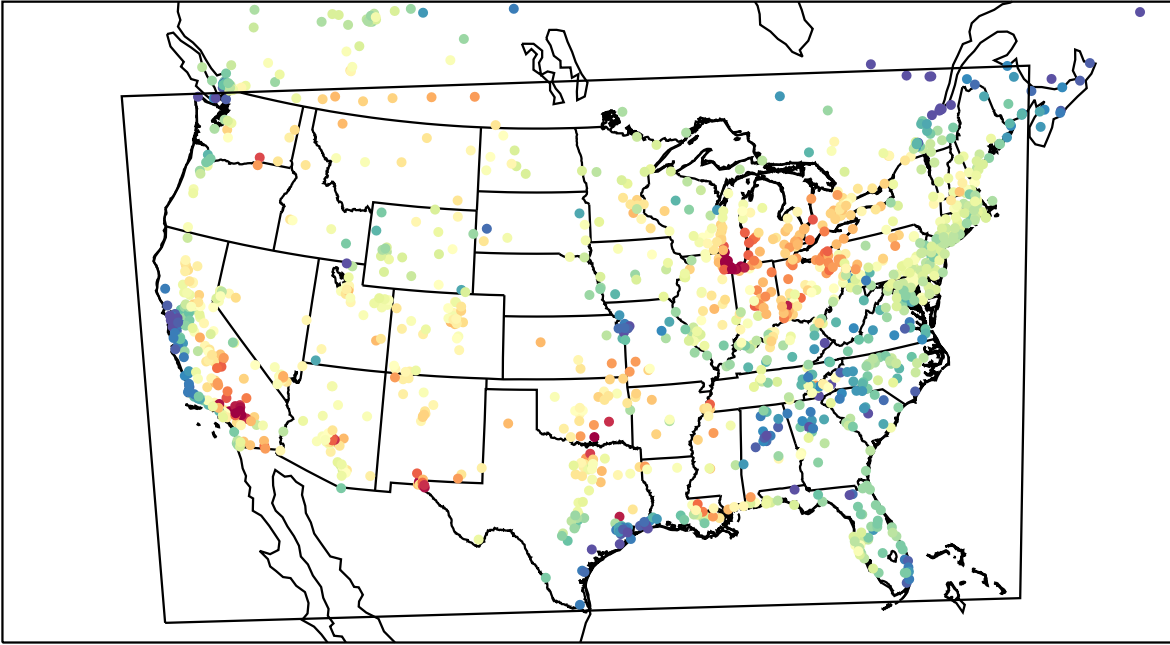
AirNOW (2023-08-03_23:00:00)
