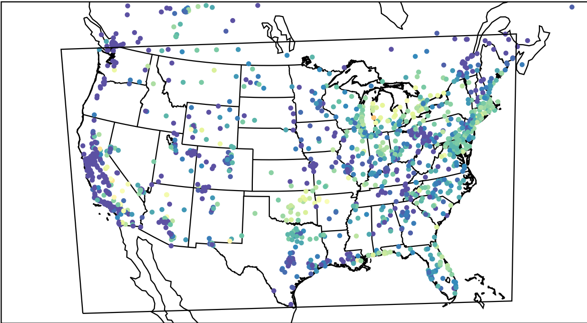
AirNOW (2023-08-03_13:00:00)
