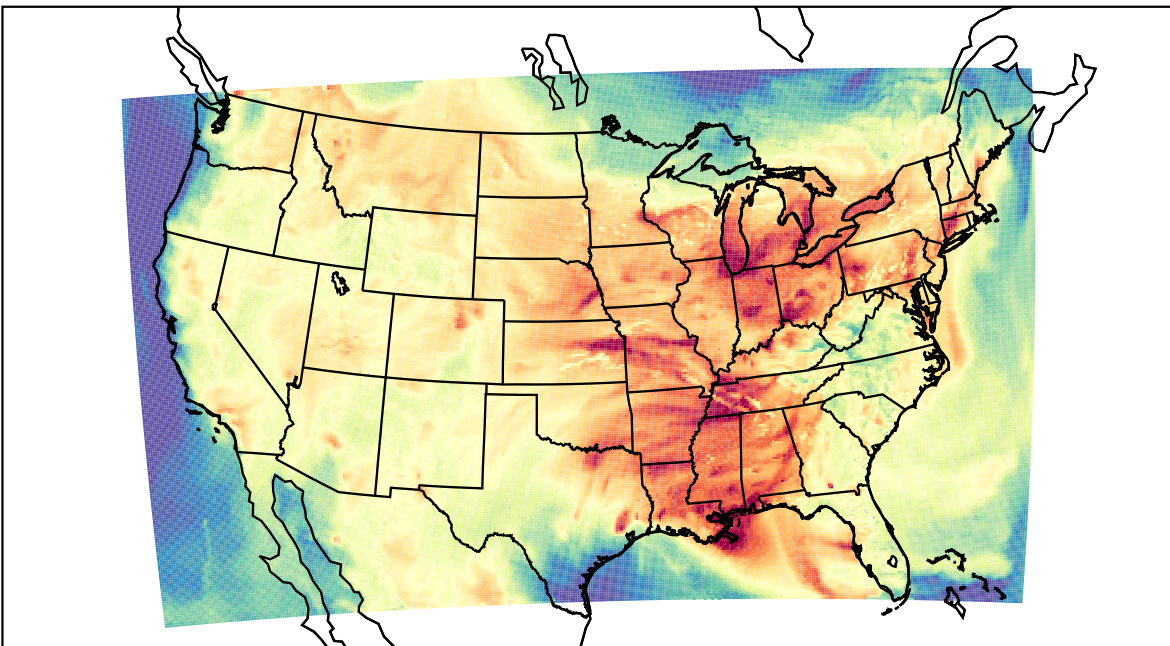
WRF (2023-08-03_20:00:00)
