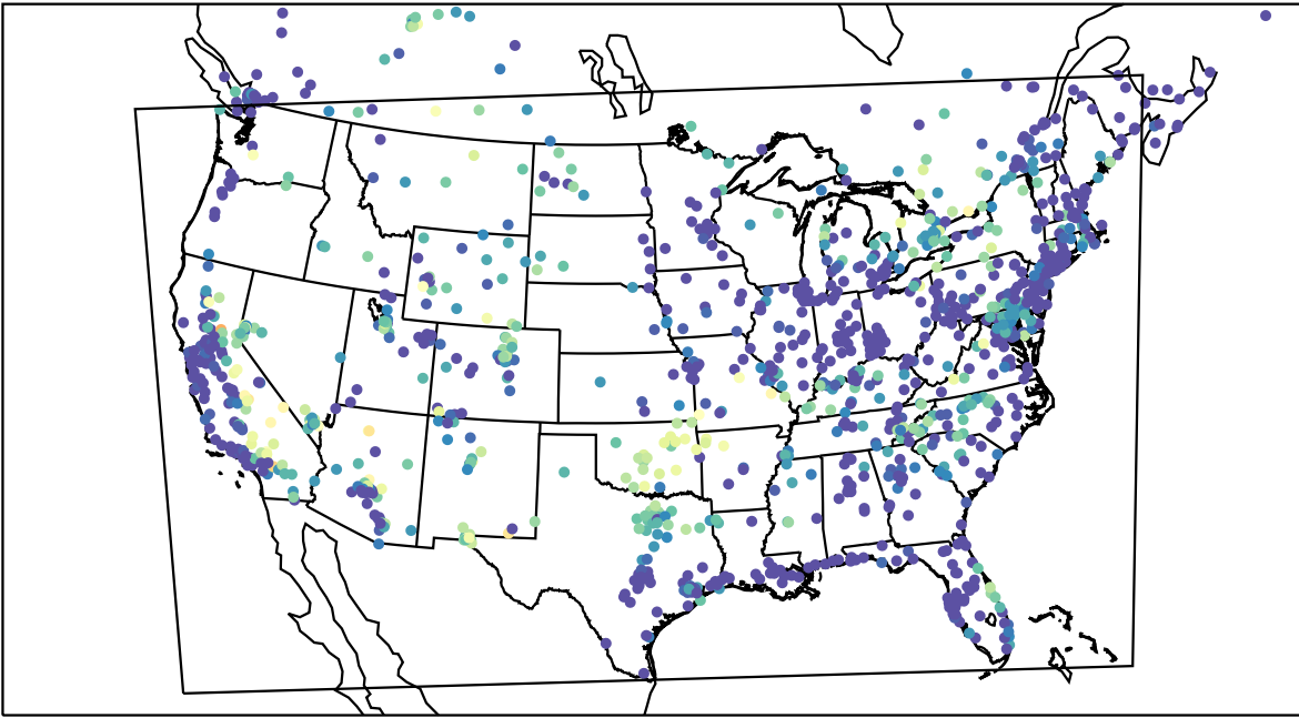
AirNOW (2023-08-03_10:00:00)
