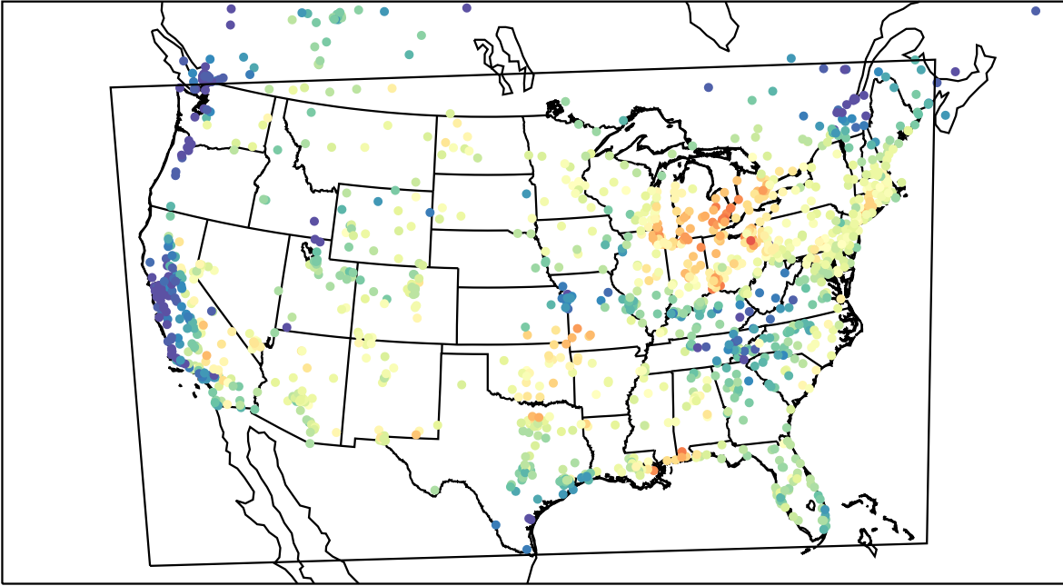
AirNOW (2023-08-03_16:00:00)
