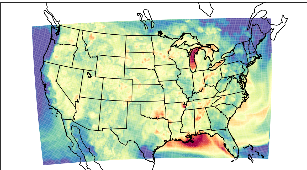
WRF (2023-08-03_03:00:00)
