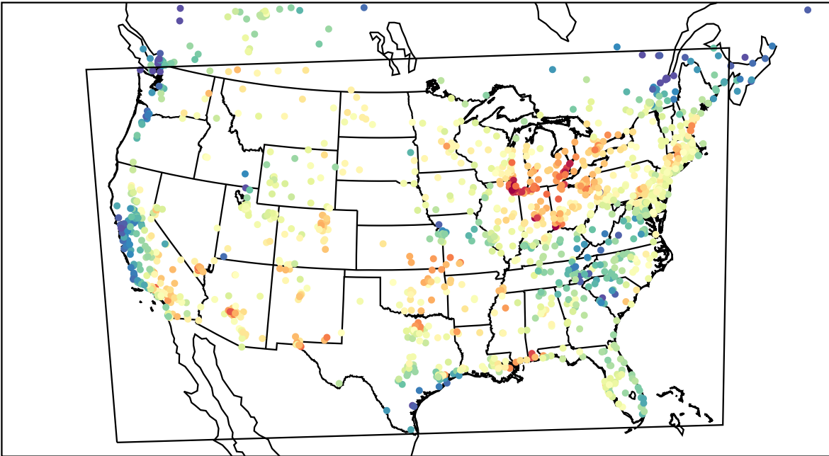
AirNOW (2023-08-03_18:00:00)
