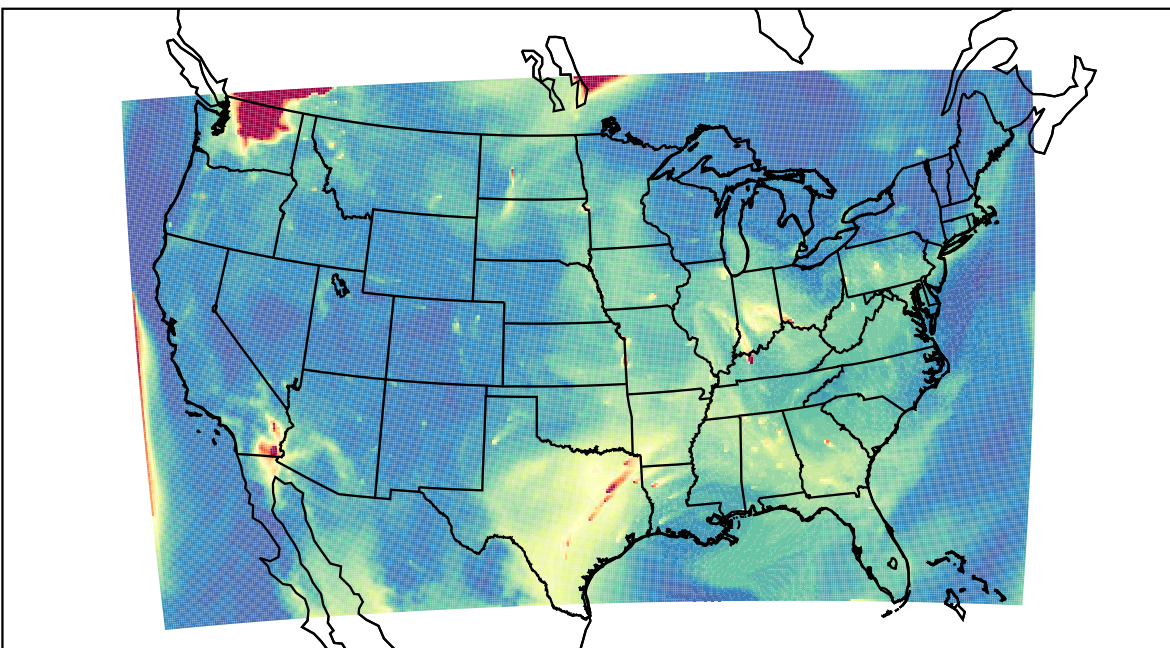
WRF 2023-08-05_15:00:00
