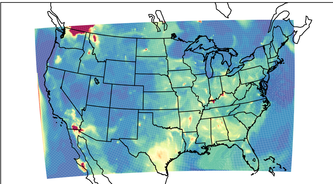
WRF 2023-08-05_06:00:00
