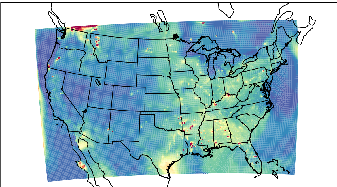
WRF 2023-08-05_01:00:00
