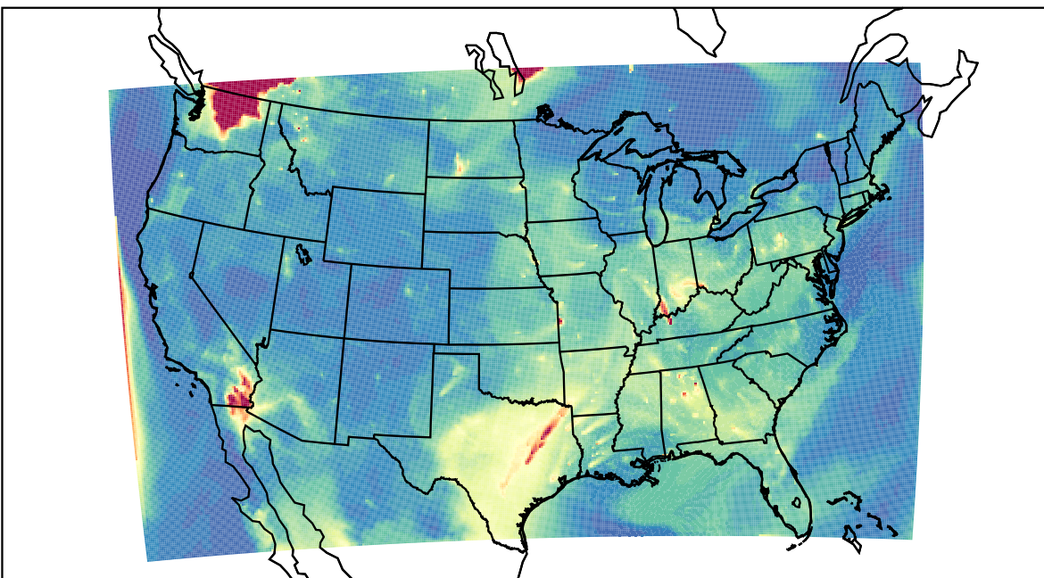
WRF 2023-08-05_13:00:00
