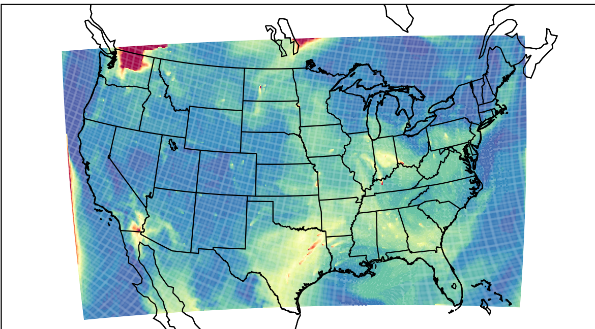
WRF 2023-08-05_16:00:00
