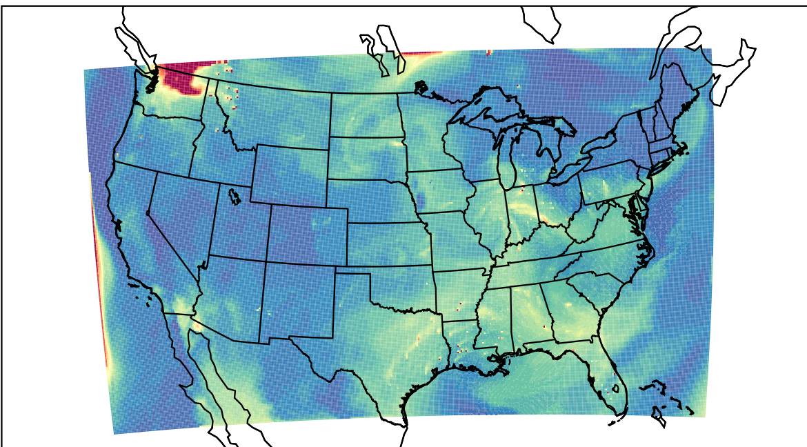
WRF 2023-08-05_20:00:00
