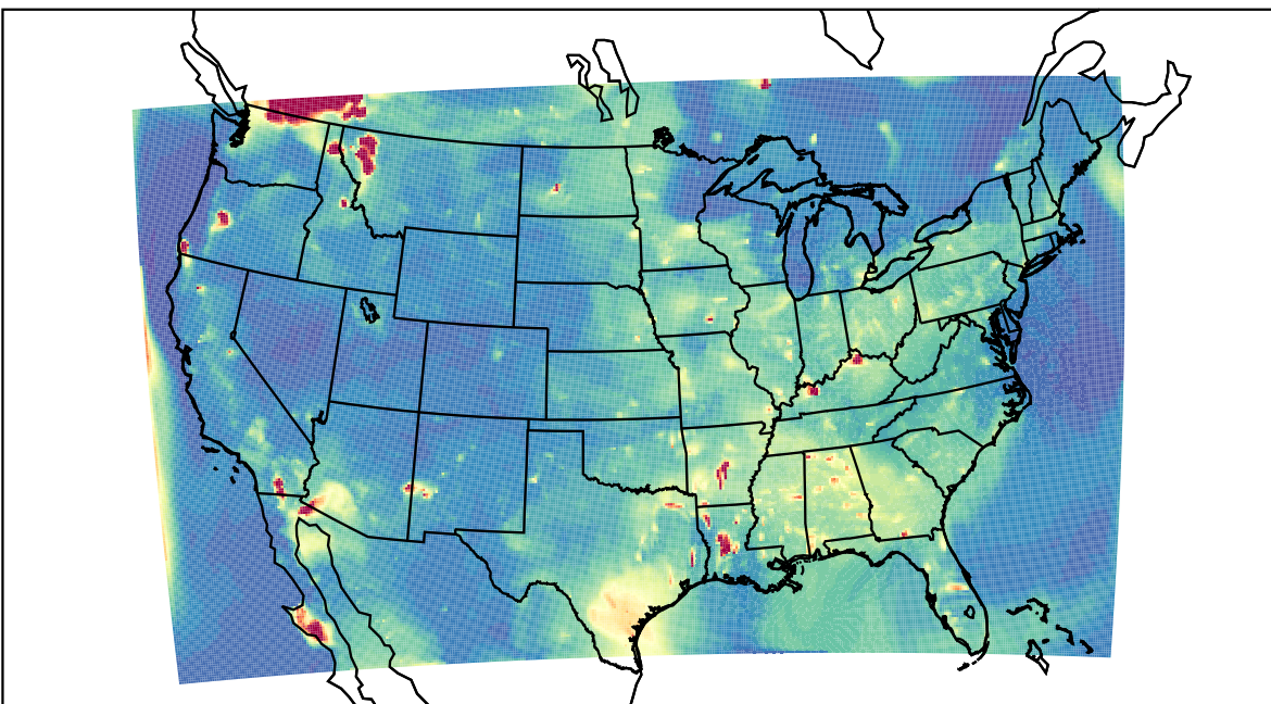
WRF 2023-08-05_03:00:00
