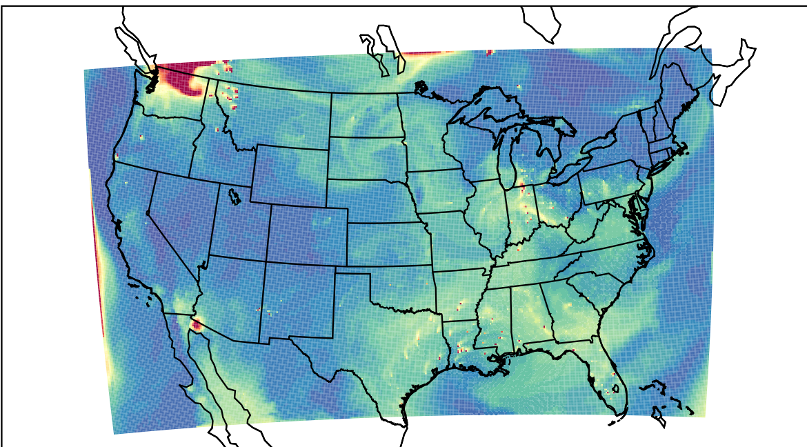
WRF 2023-08-05_22:00:00
