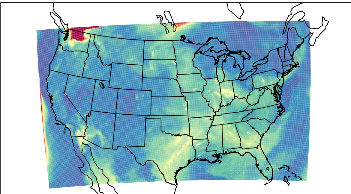
WRF 2023-08-05_17:00:00
