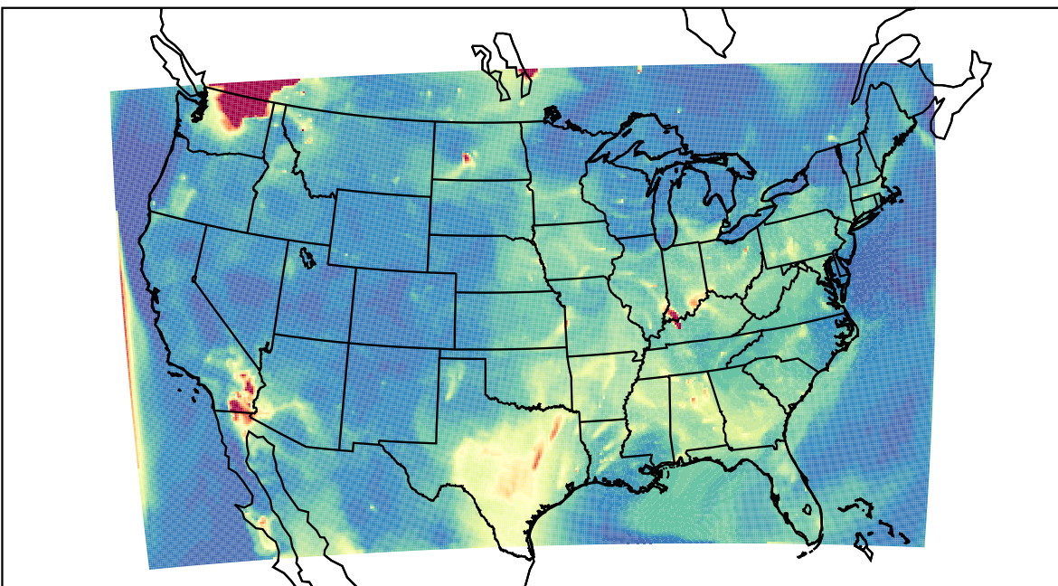
WRF 2023-08-05_10:00:00
