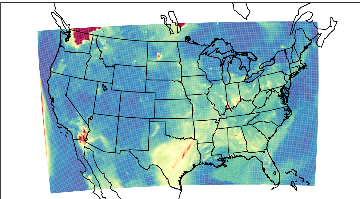
WRF 2023-08-05_12:00:00
