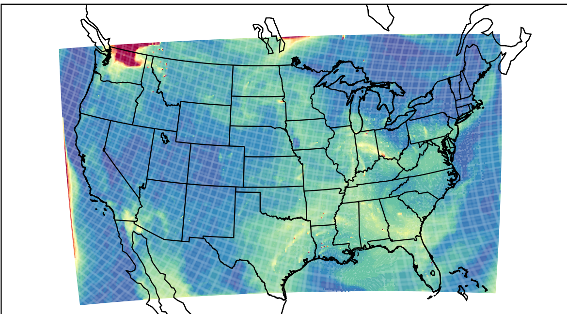
WRF 2023-08-05_19:00:00
