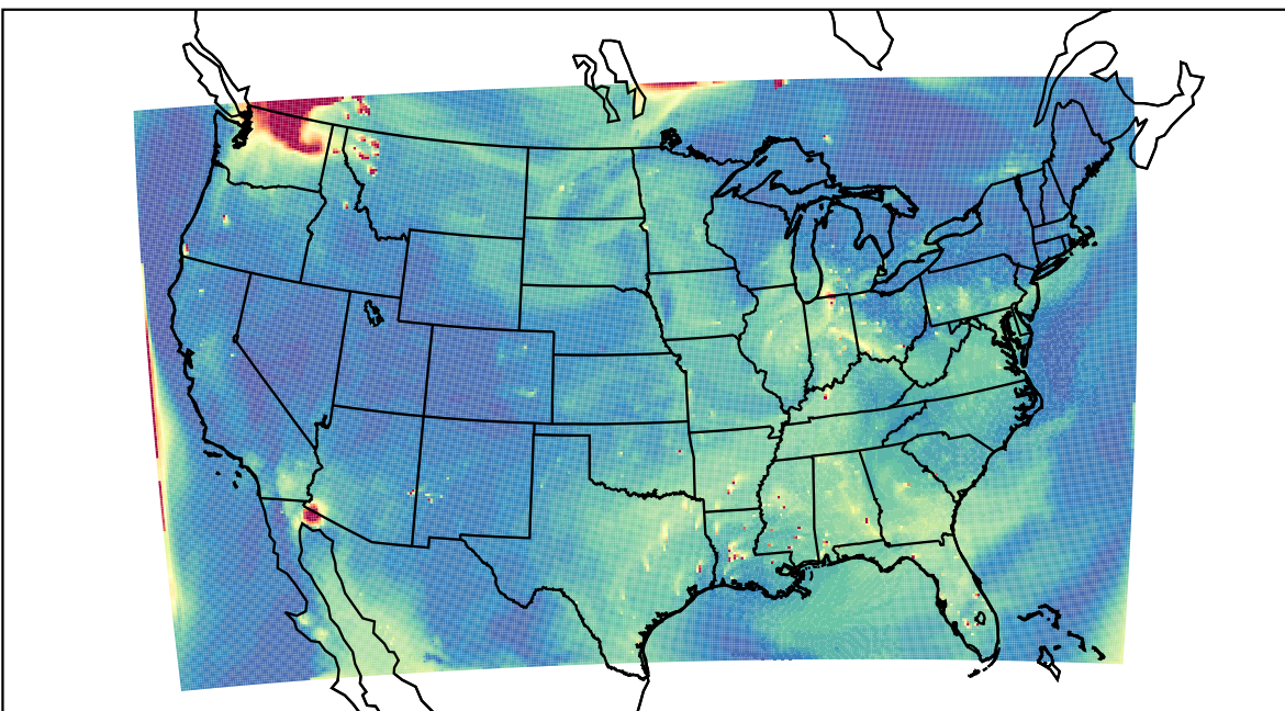
WRF 2023-08-05_23:00:00
