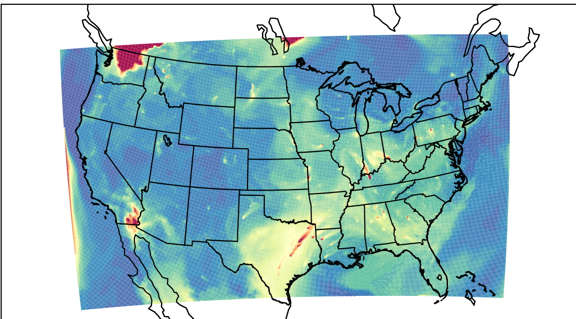
WRF 2023-08-05_14:00:00
