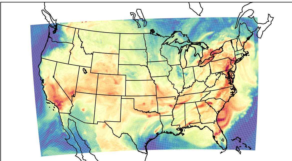
WRF (2023-08-07_20:00:00)
