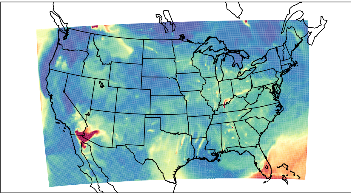
WRF 2023-08-09_11:00:00
