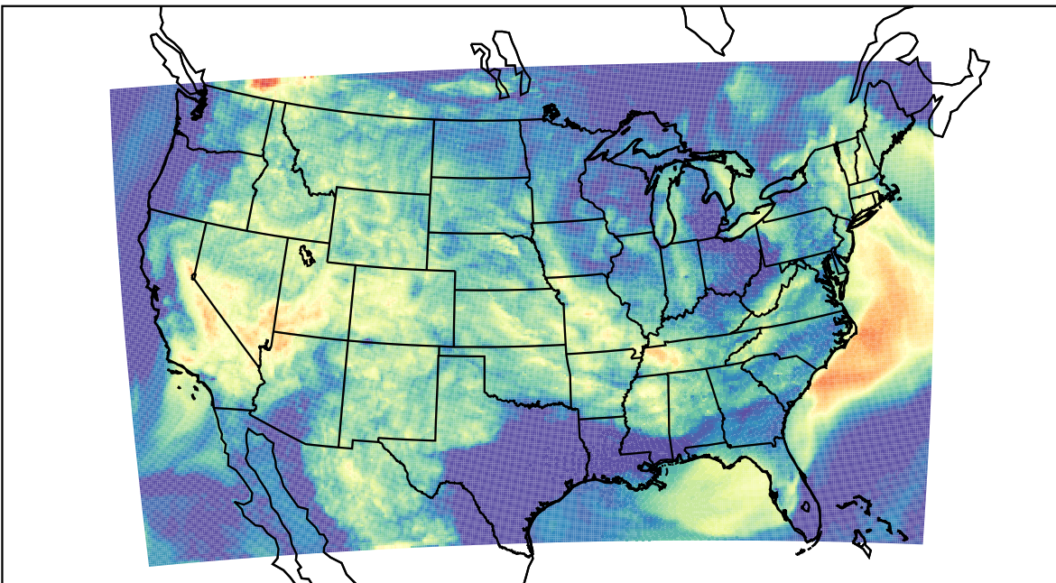
WRF (2023-08-08_10:00:00)
