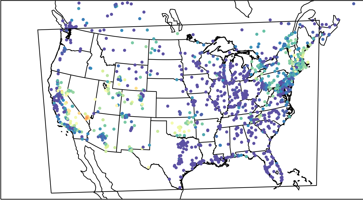
AirNOW (2023-08-08_10:00:00)
