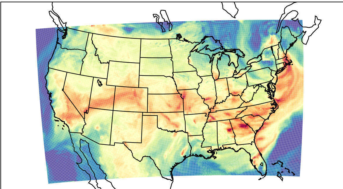
WRF (2023-08-08_20:00:00)
