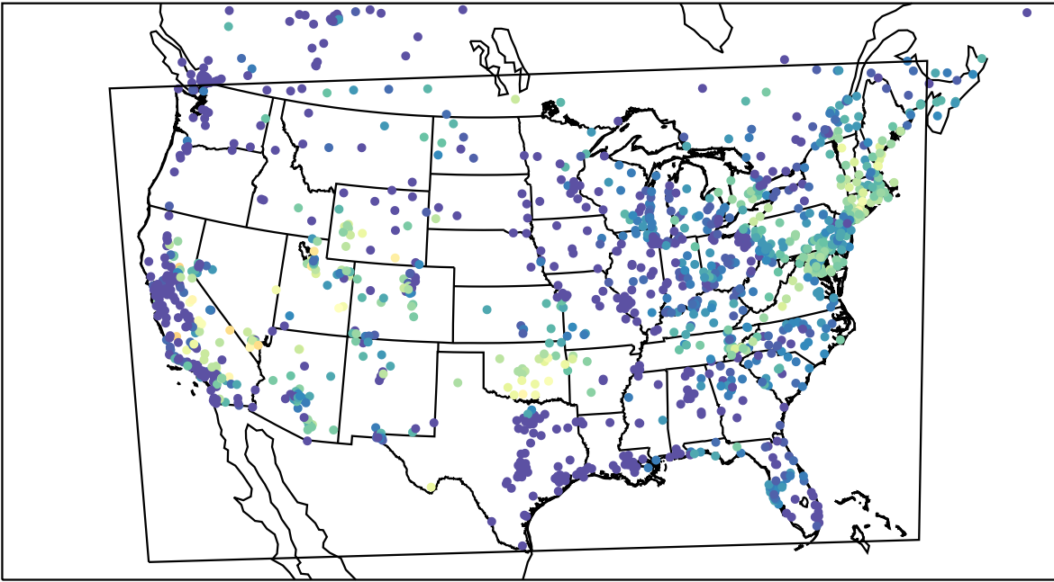
AirNOW (2023-08-08_13:00:00)
