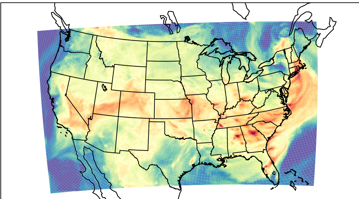
WRF (2023-08-08_18:00:00)
