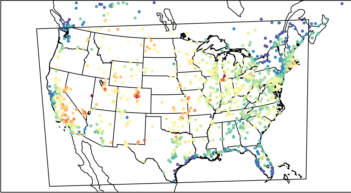
AirNOW (2023-08-08_20:00:00)
