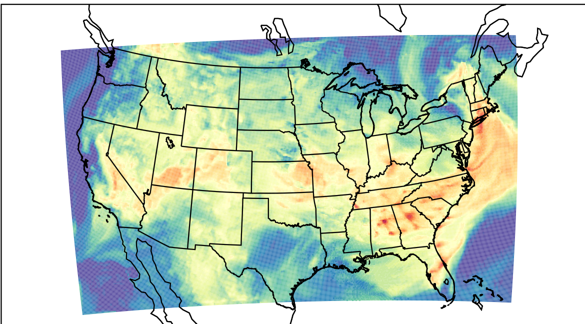
WRF (2023-08-08_16:00:00)
