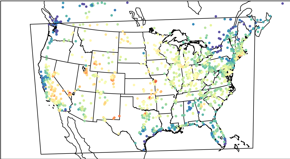
AirNOW (2023-08-08_18:00:00)
