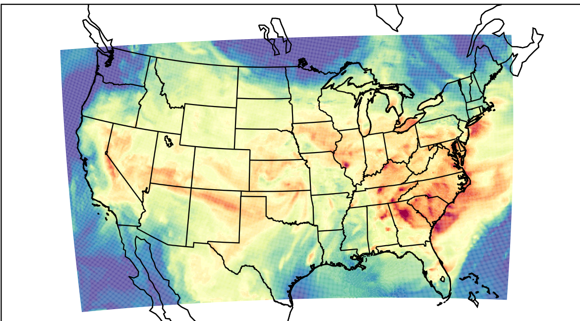
WRF (2023-08-09_18:00:00)
