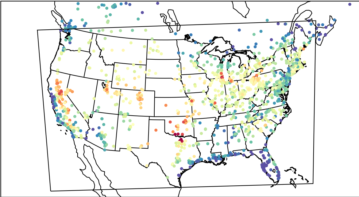
AirNOW (2023-08-10_23:00:00)
