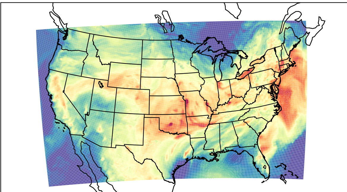
WRF (2023-08-10_22:00:00)
