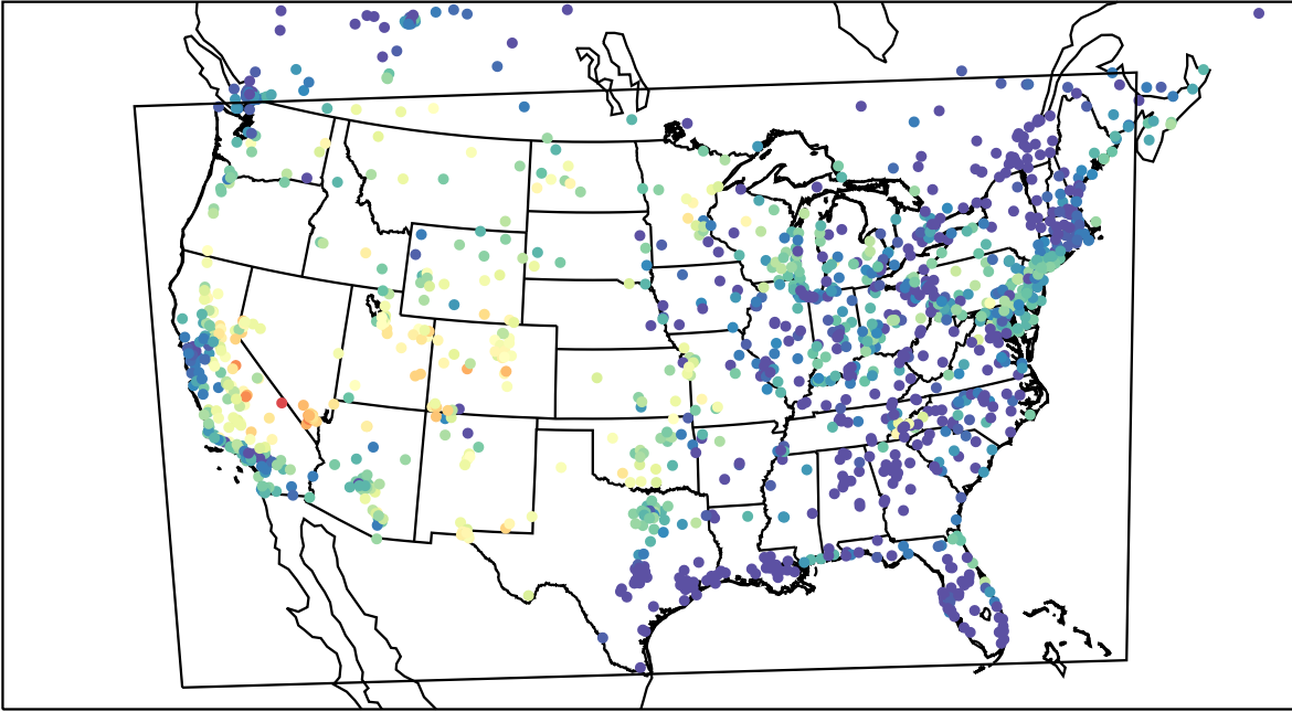
AirNOW (2023-08-09_03:00:00)
