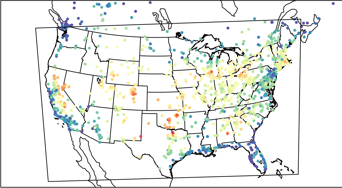
AirNOW (2023-08-10_18:00:00)
