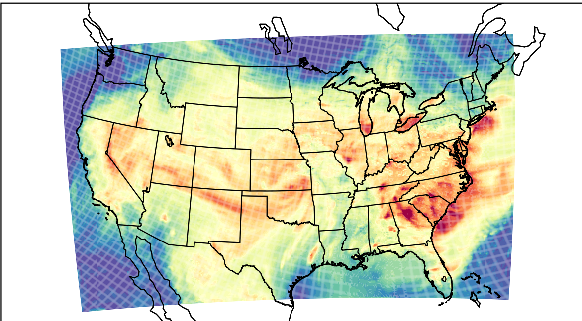
WRF (2023-08-09_20:00:00)
