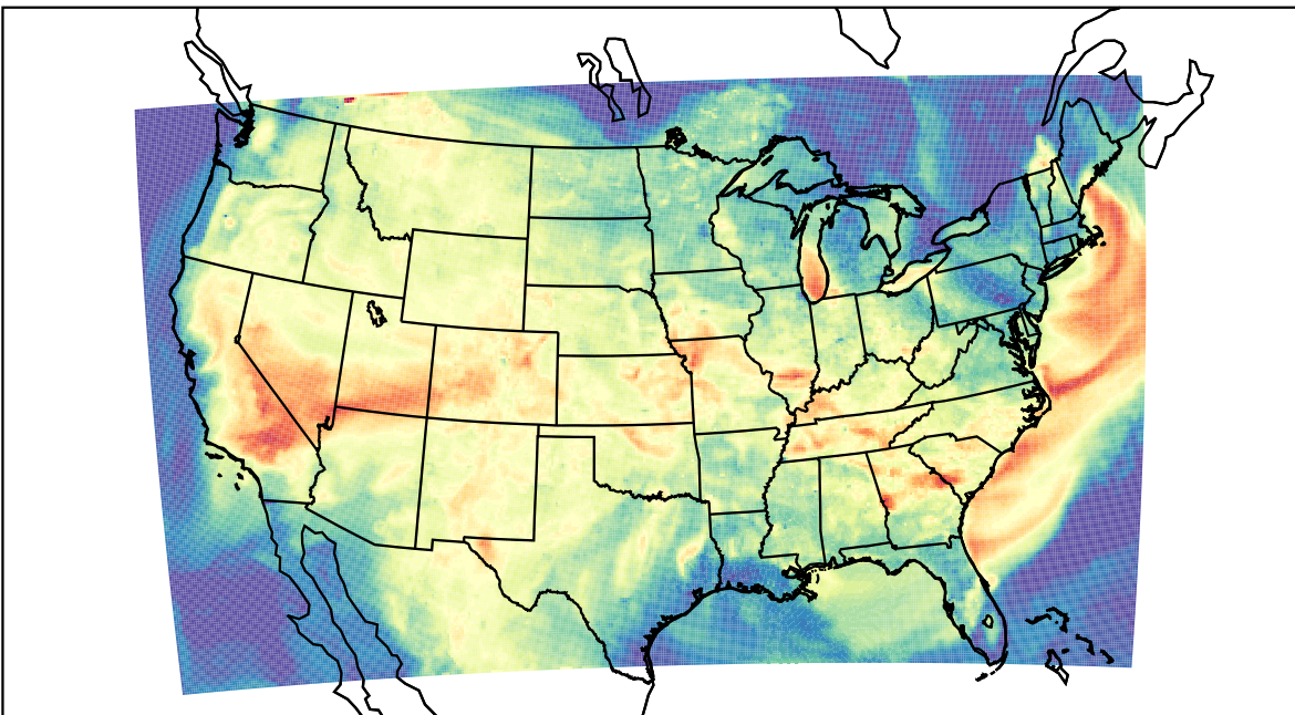
WRF (2023-08-09_01:00:00)
