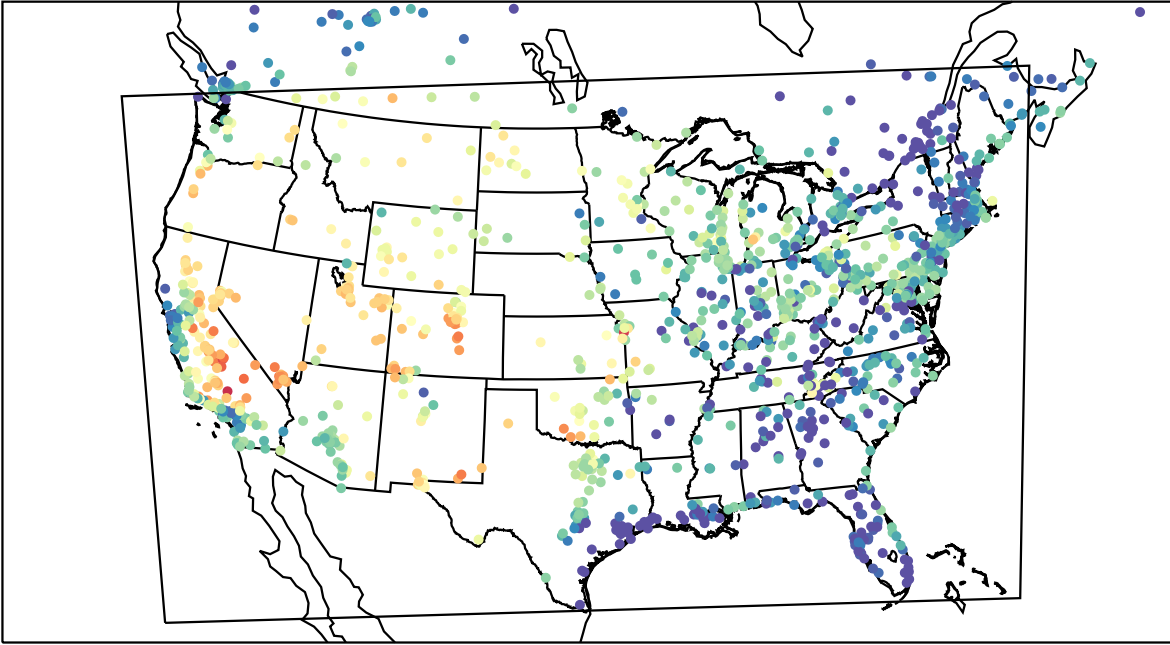
AirNOW (2023-08-09_01:00:00)
