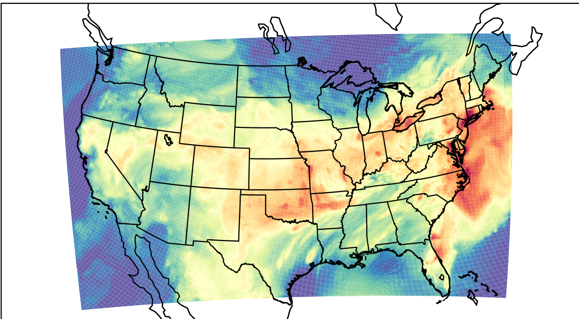
WRF (2023-08-10_18:00:00)
