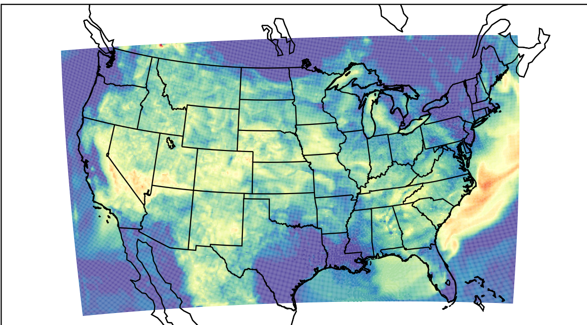
WRF (2023-08-09_08:00:00)
