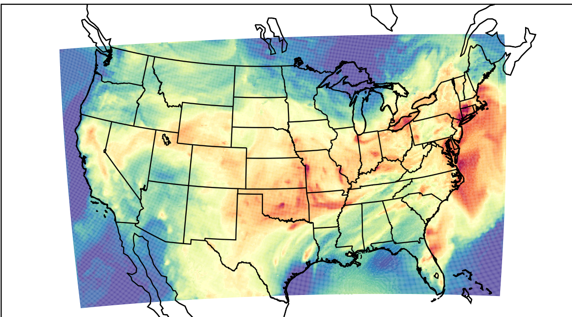
WRF (2023-08-10_20:00:00)
