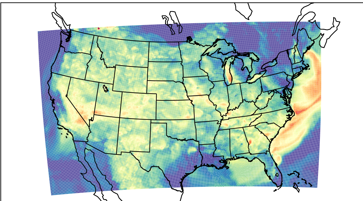
WRF (2023-08-09_04:00:00)
