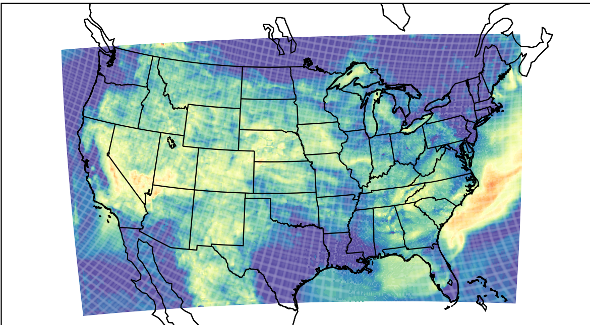
WRF (2023-08-09_10:00:00)
