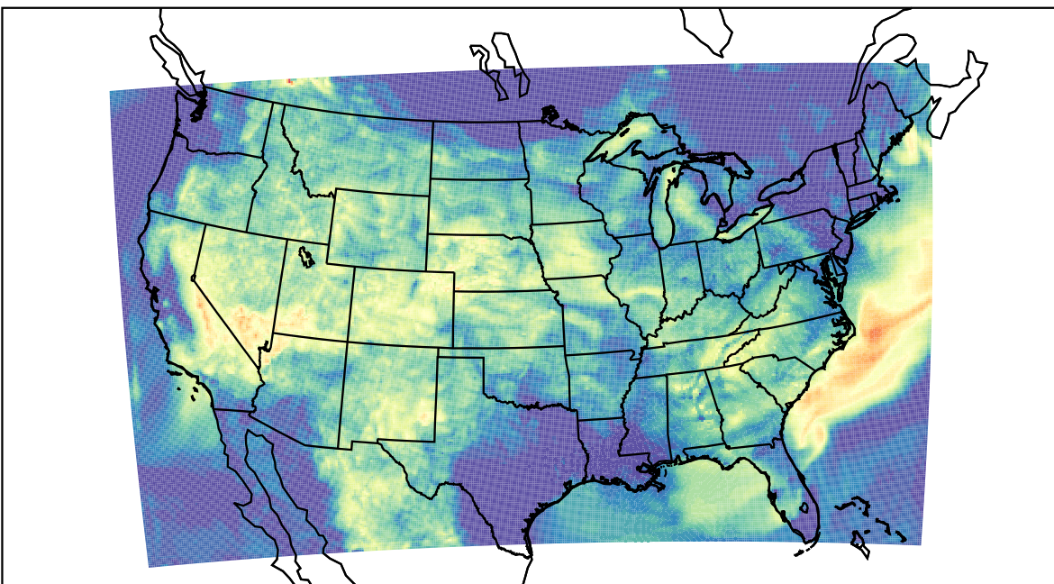
WRF (2023-08-09_09:00:00)
