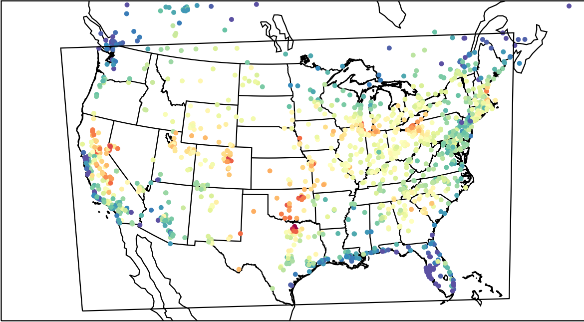
AirNOW (2023-08-10_20:00:00)
