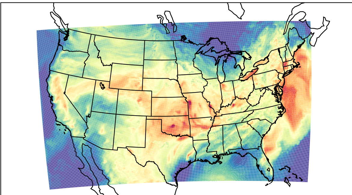
WRF (2023-08-10_23:00:00)
