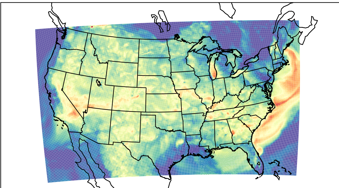
WRF (2023-08-09_03:00:00)
