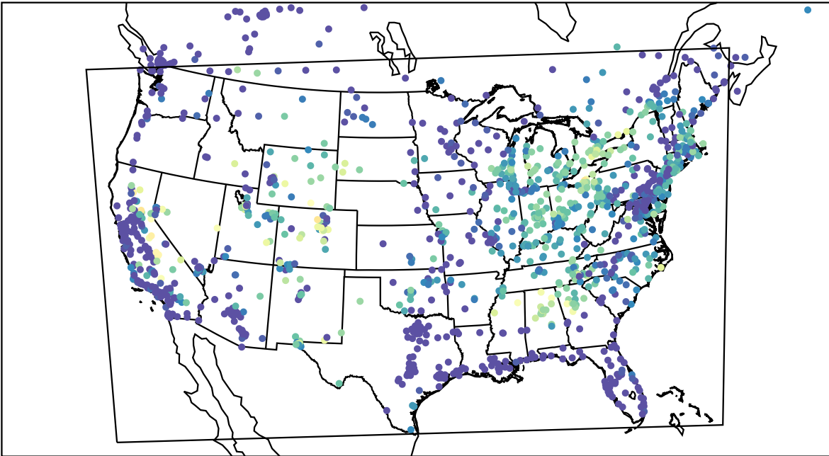
AirNOW (2023-08-10_13:00:00)
