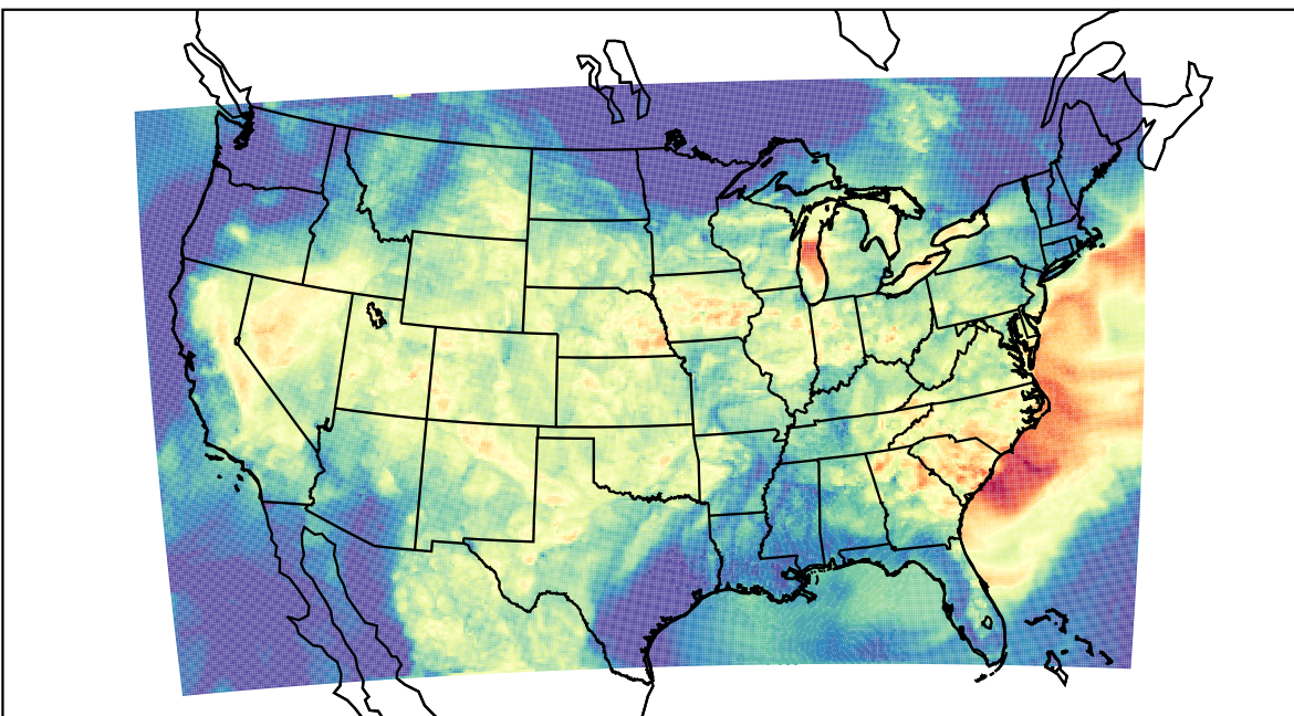
WRF (2023-08-10_03:00:00)
