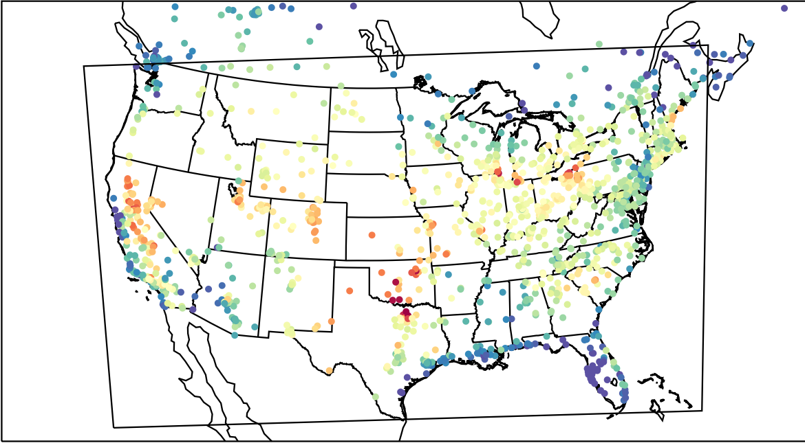
AirNOW (2023-08-10_22:00:00)
