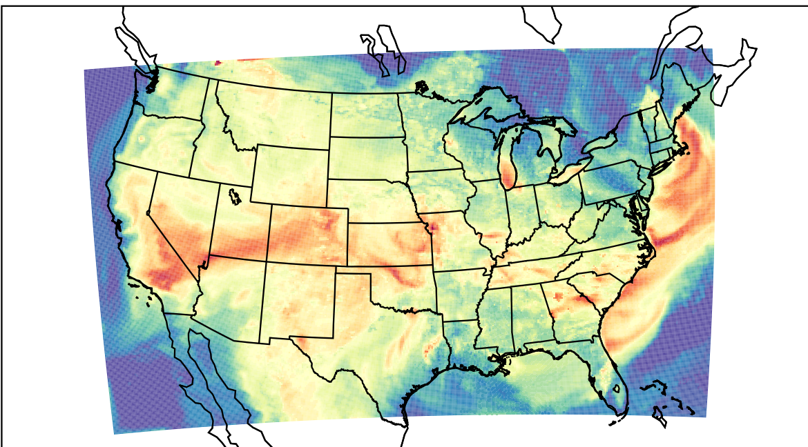
WRF (2023-08-09_00:00:00)
