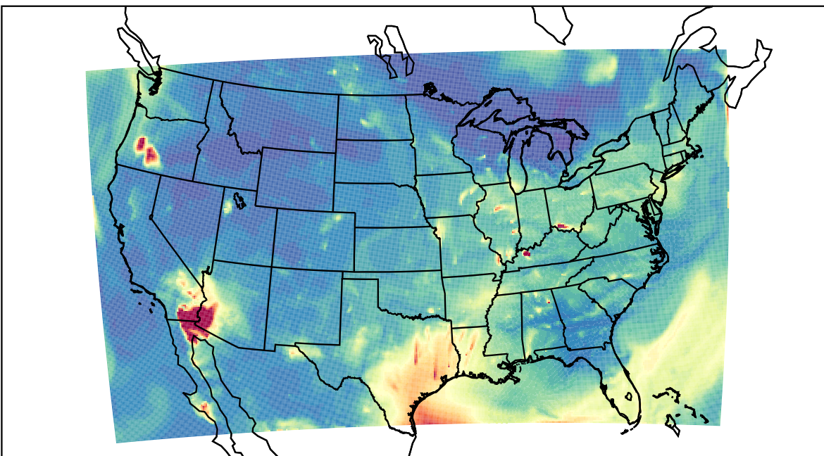
WRF 2023-08-11_06:00:00
