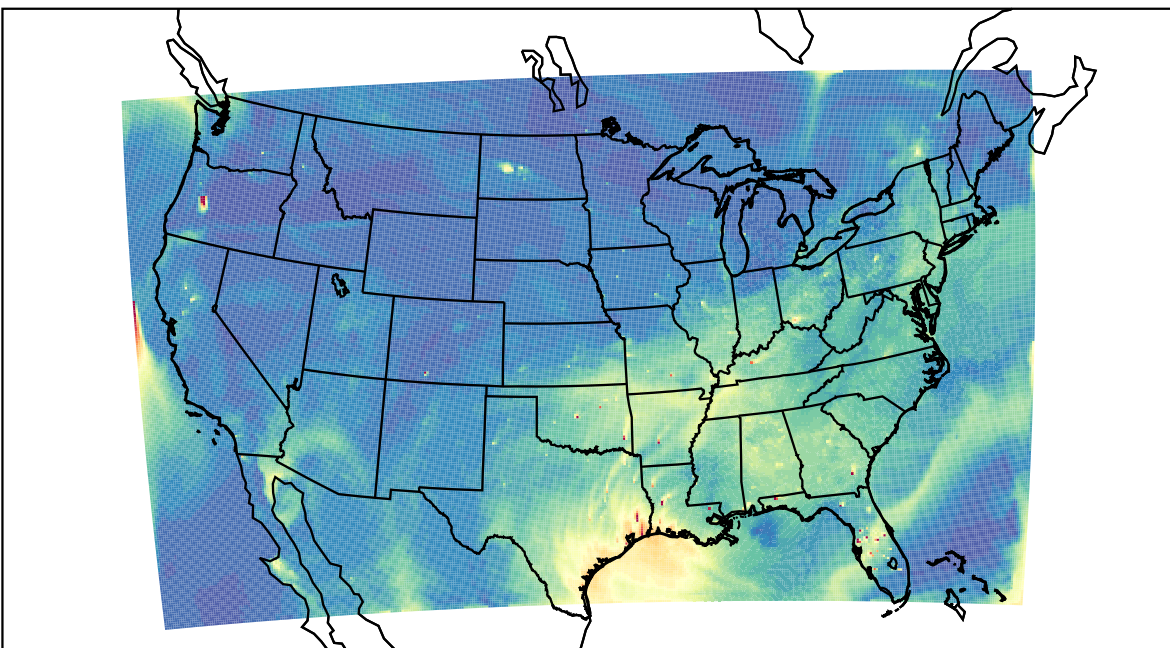
WRF 2023-08-12_23:00:00
