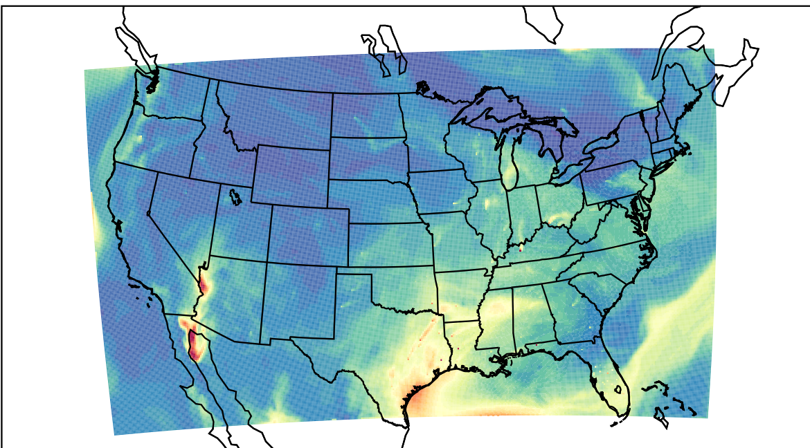
WRF 2023-08-11_18:00:00
