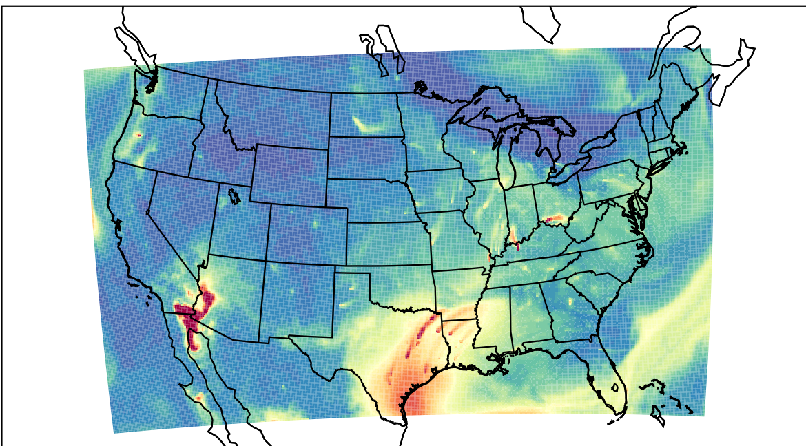
WRF 2023-08-11_14:00:00
