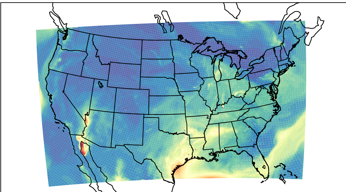
WRF 2023-08-11_19:00:00
