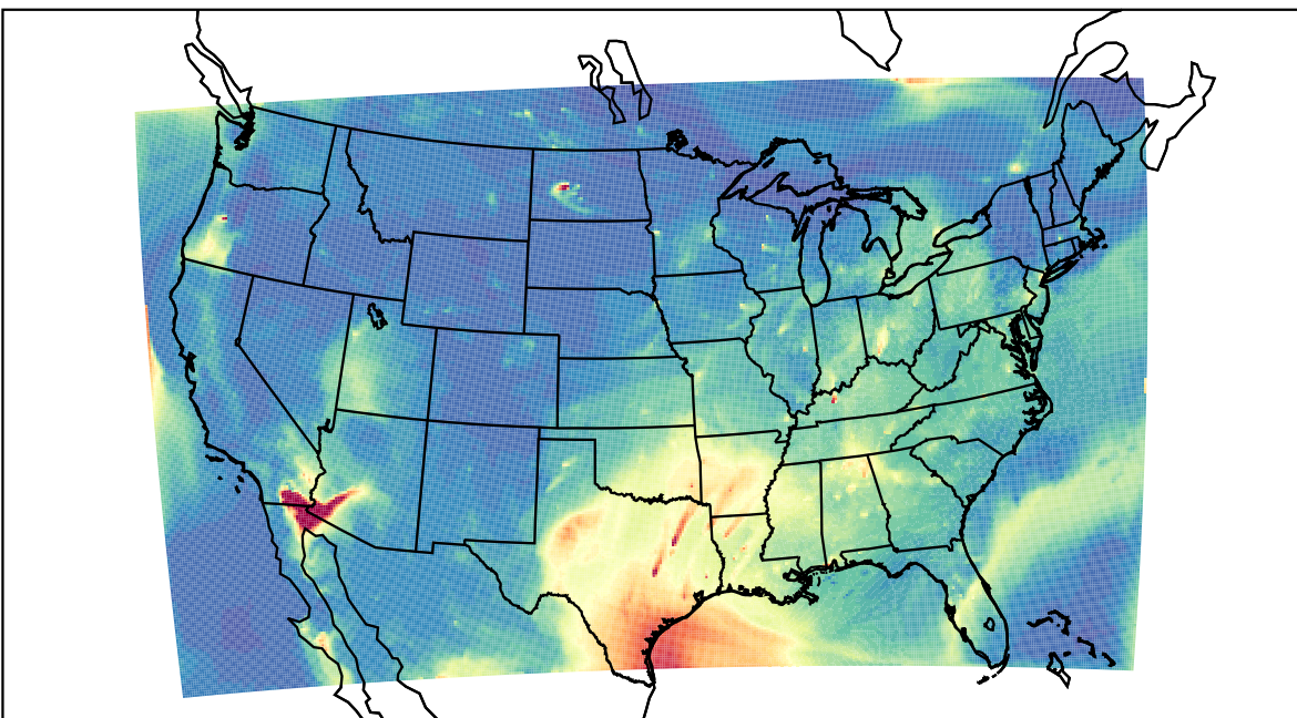
WRF 2023-08-12_12:00:00
