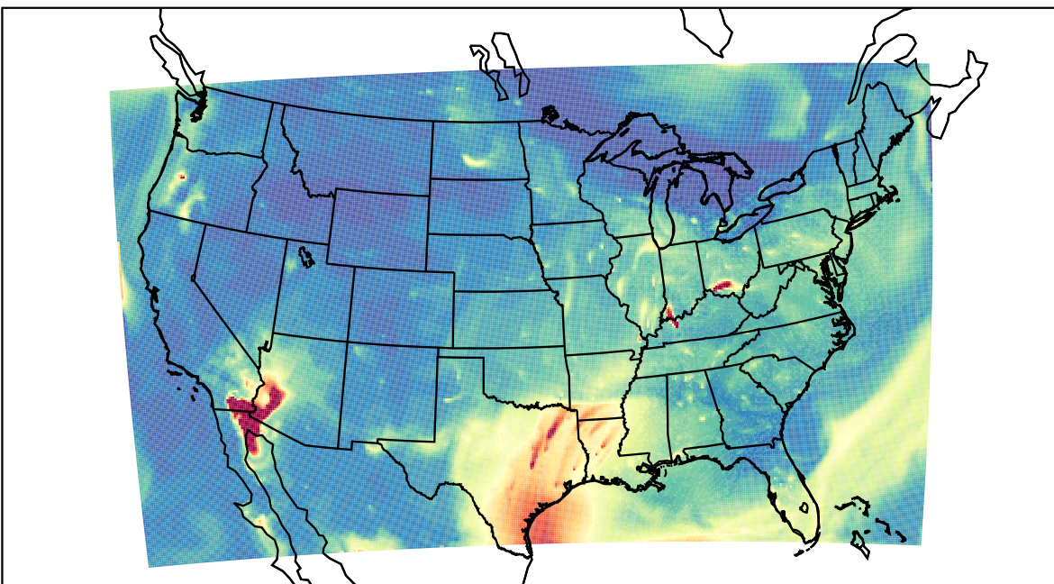
WRF 2023-08-11_12:00:00
