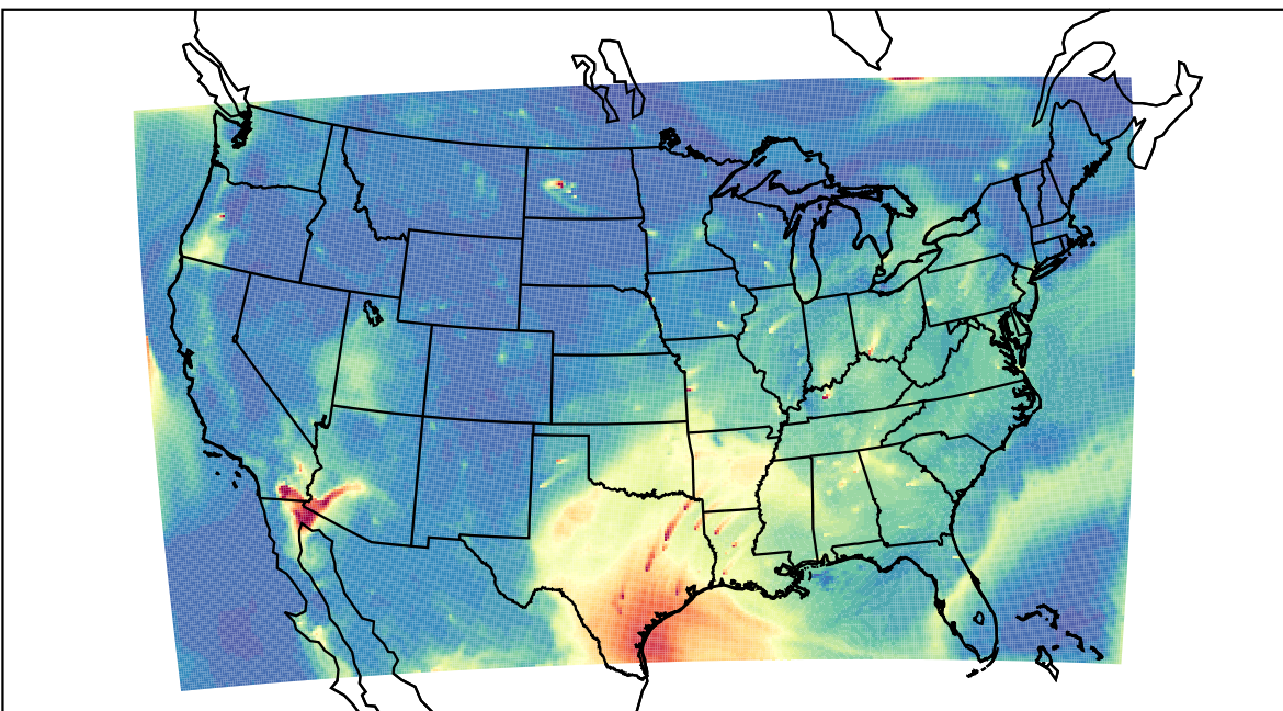
WRF 2023-08-12_14:00:00
