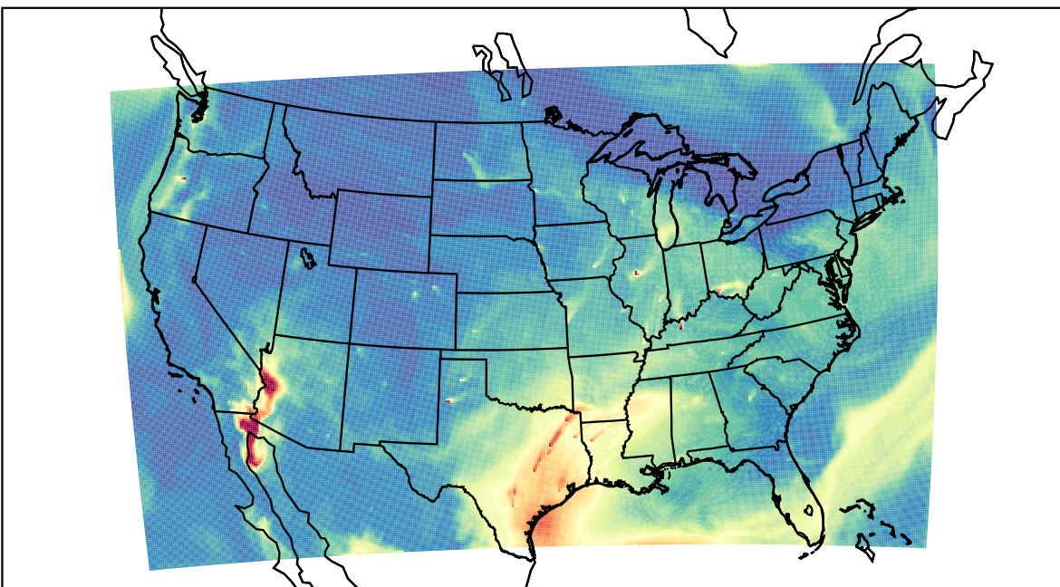
WRF 2023-08-11_16:00:00
