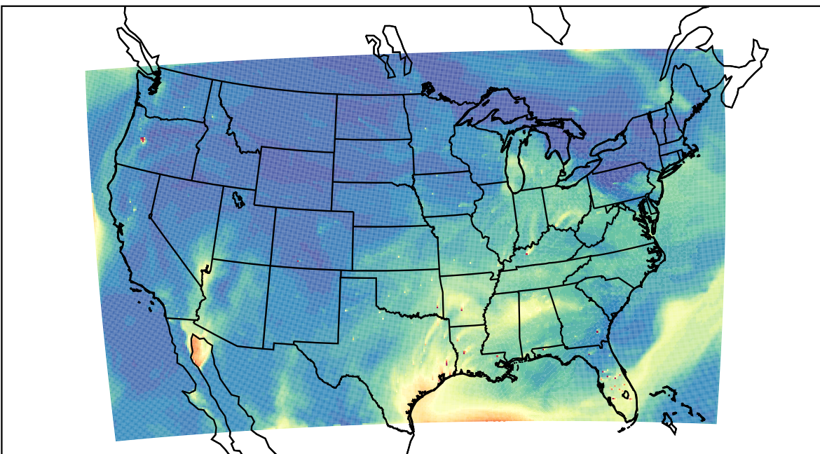
WRF 2023-08-11_22:00:00
