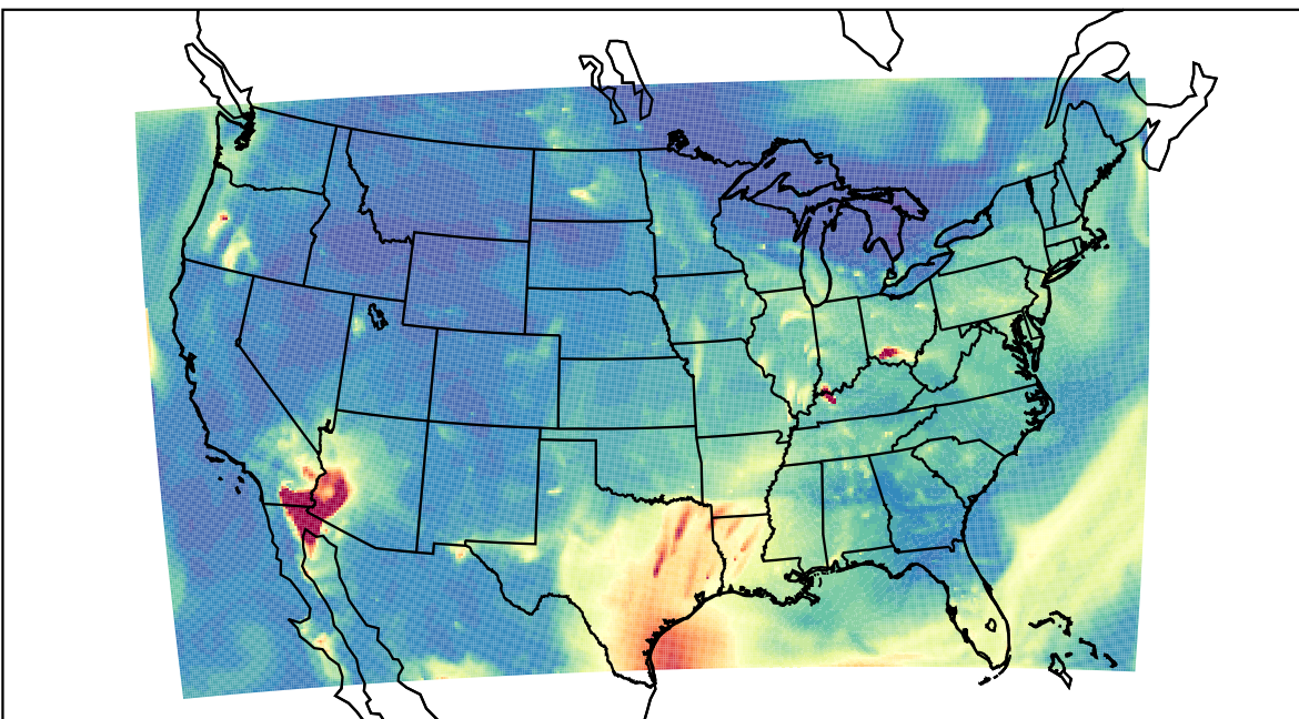
WRF 2023-08-11_10:00:00
