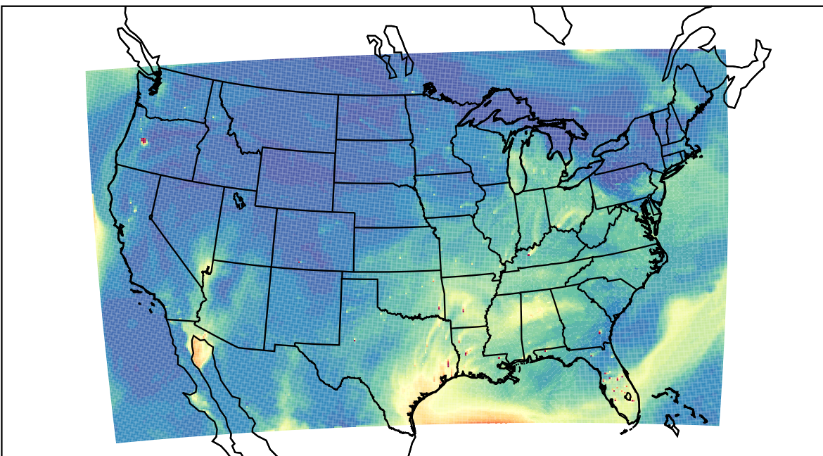
WRF 2023-08-11_23:00:00
