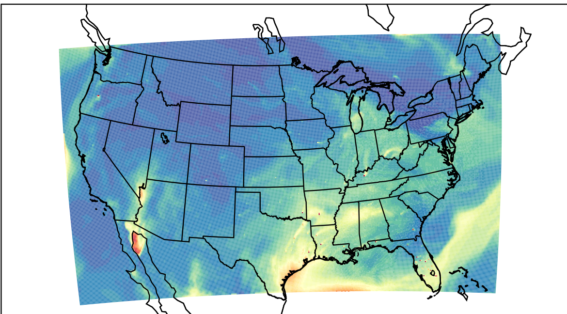
WRF 2023-08-11_20:00:00
