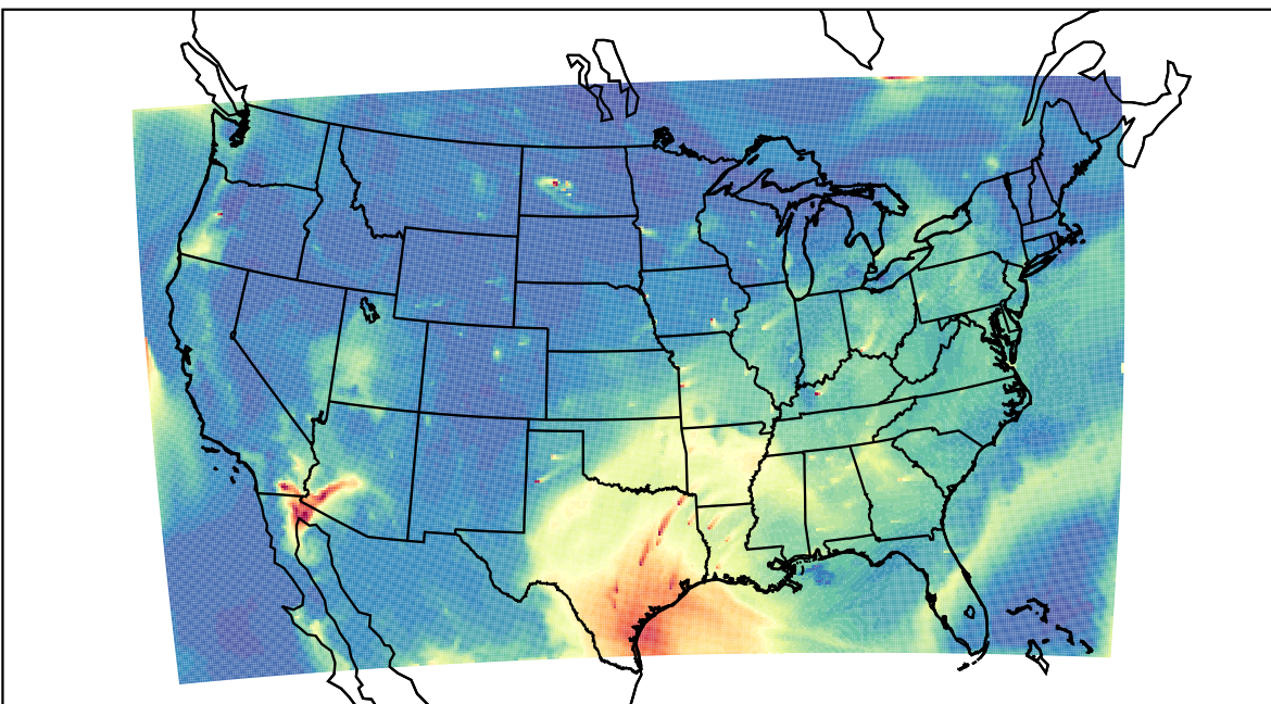
WRF 2023-08-12_15:00:00
