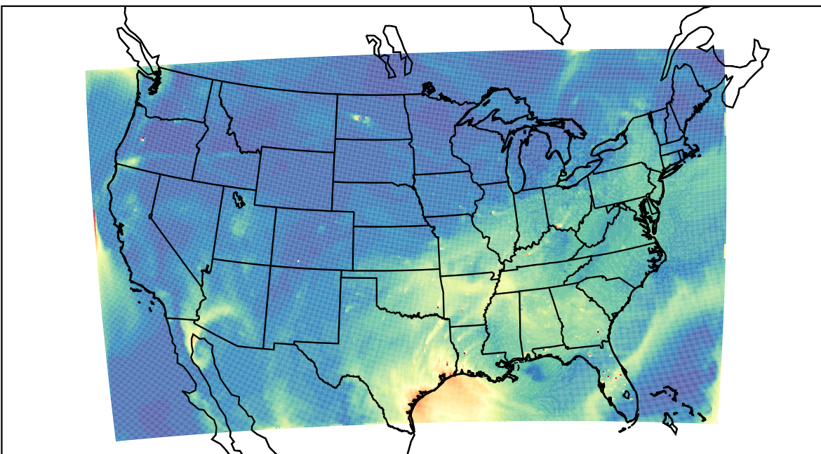
WRF 2023-08-12_20:00:00
