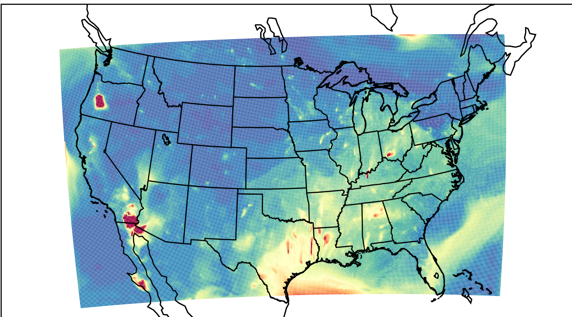
WRF 2023-08-12_04:00:00
