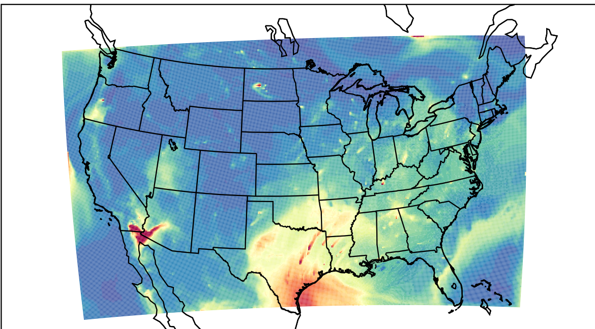
WRF 2023-08-12_13:00:00
