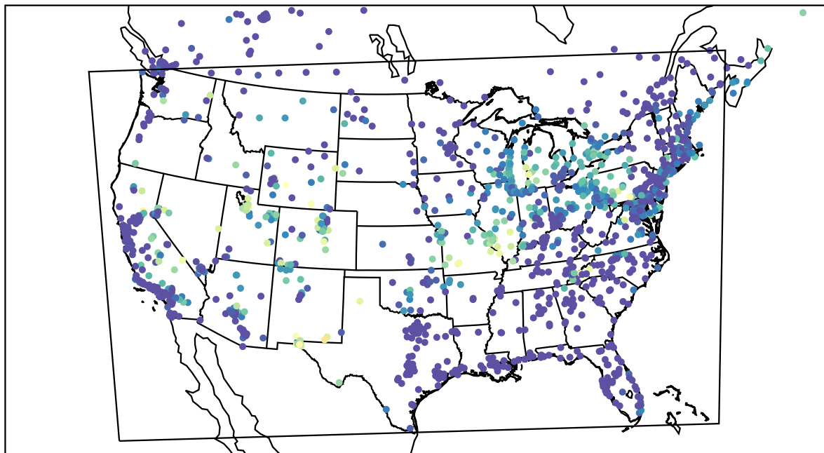
AirNOW (2023-08-12_12:00:00)
