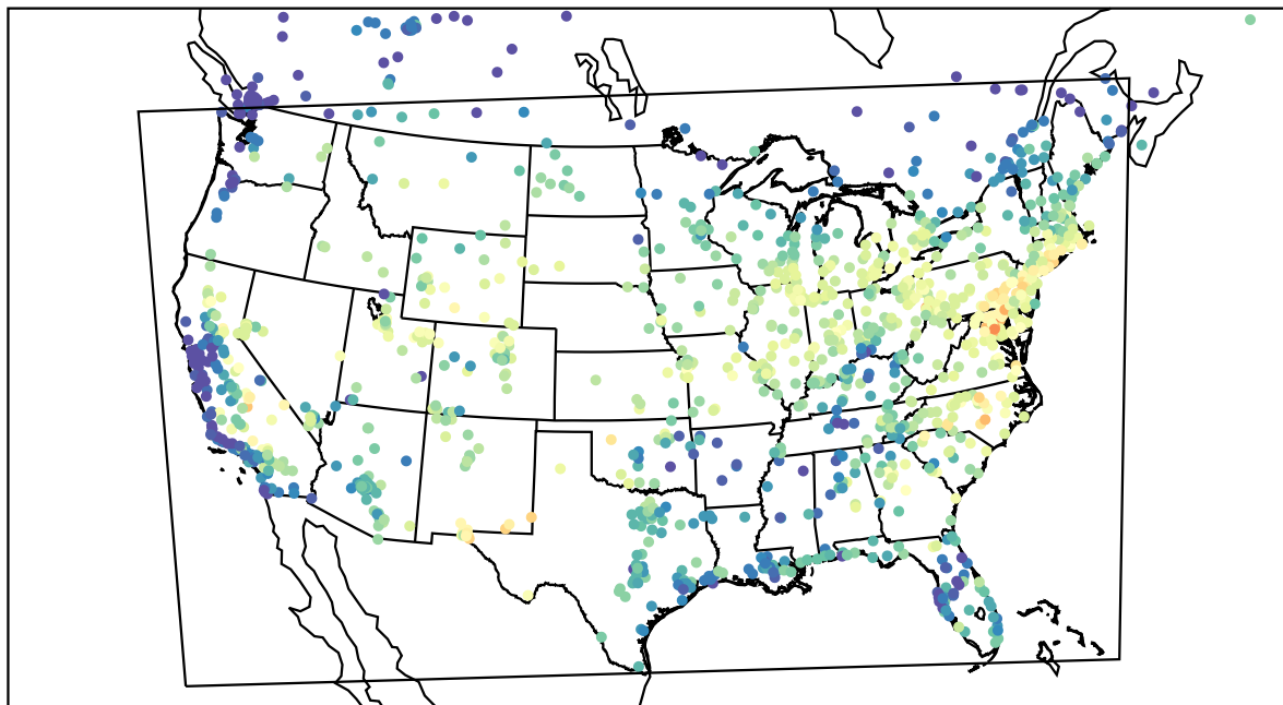
AirNOW (2023-08-12_16:00:00)
