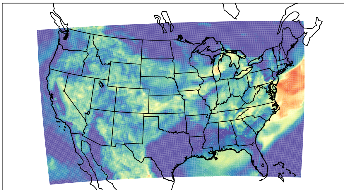
WRF (2023-08-12_10:00:00)
