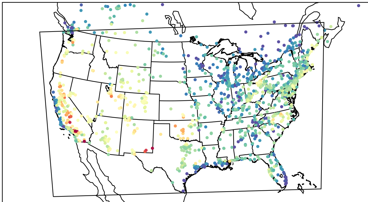
AirNOW (2023-08-13_23:00:00)
