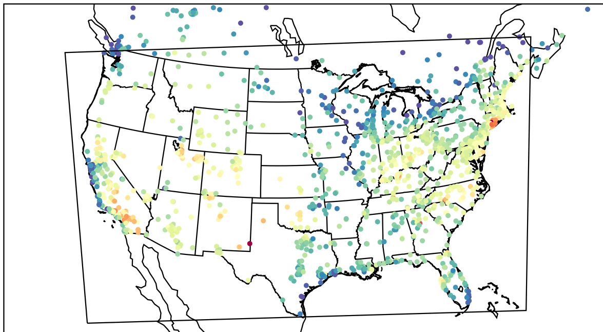
AirNOW (2023-08-13_18:00:00)
