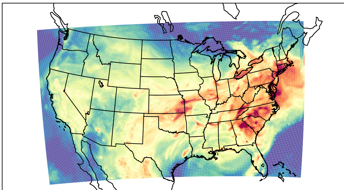
WRF (2023-08-12_20:00:00)
