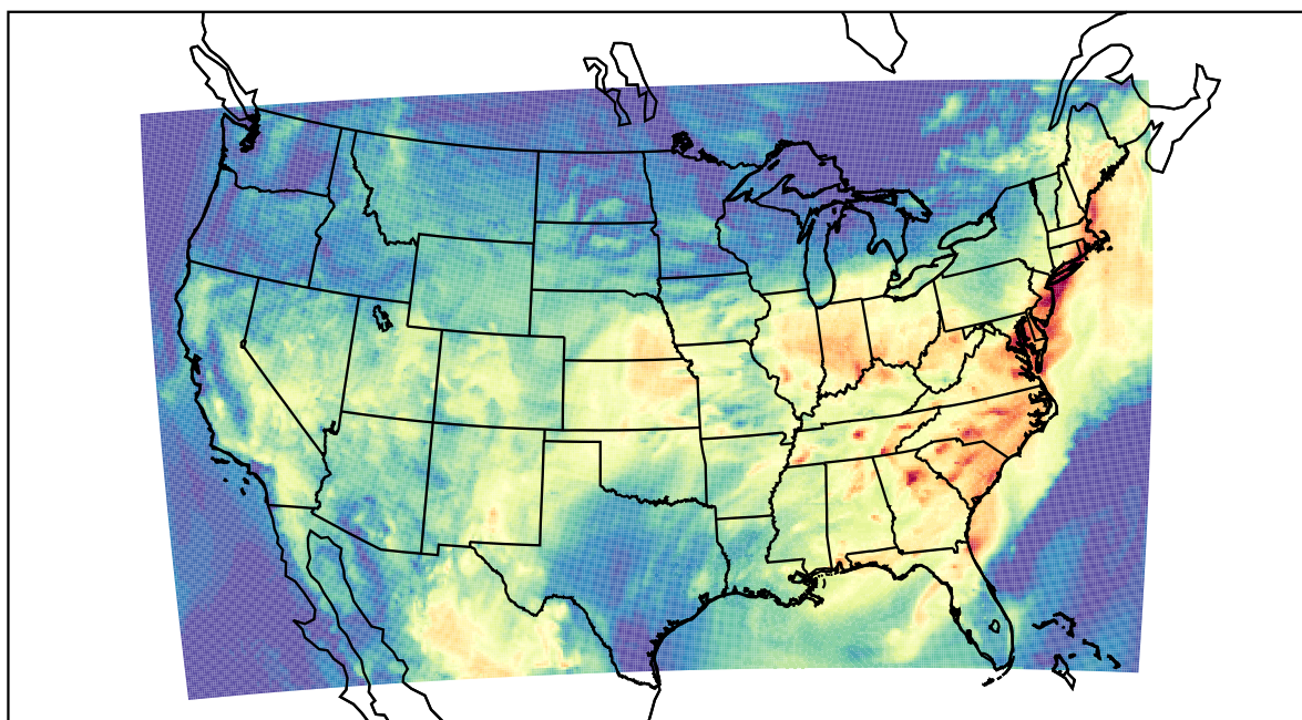
WRF (2023-08-13_16:00:00)
