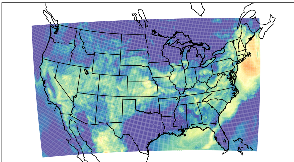
WRF (2023-08-13_10:00:00)
