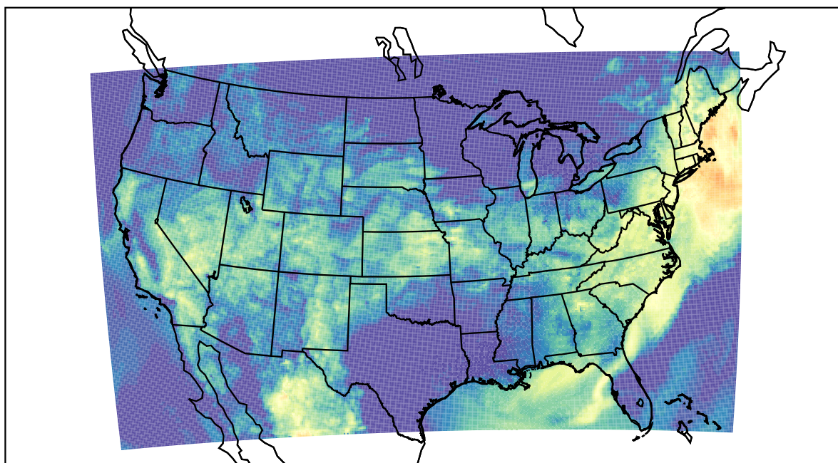
WRF (2023-08-13_13:00:00)
