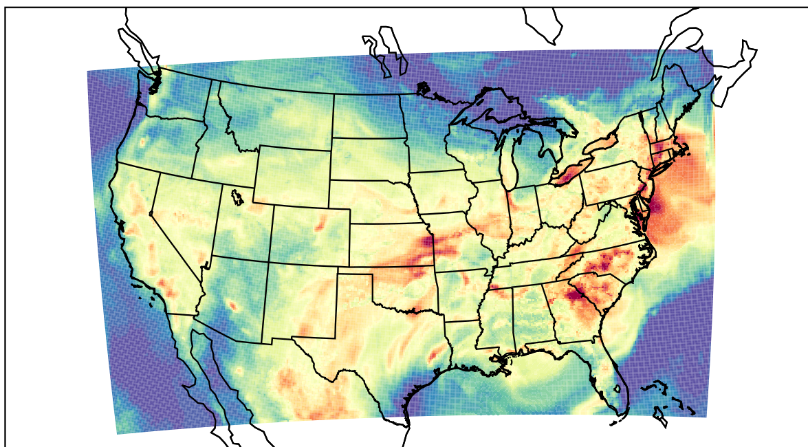
WRF (2023-08-12_23:00:00)
