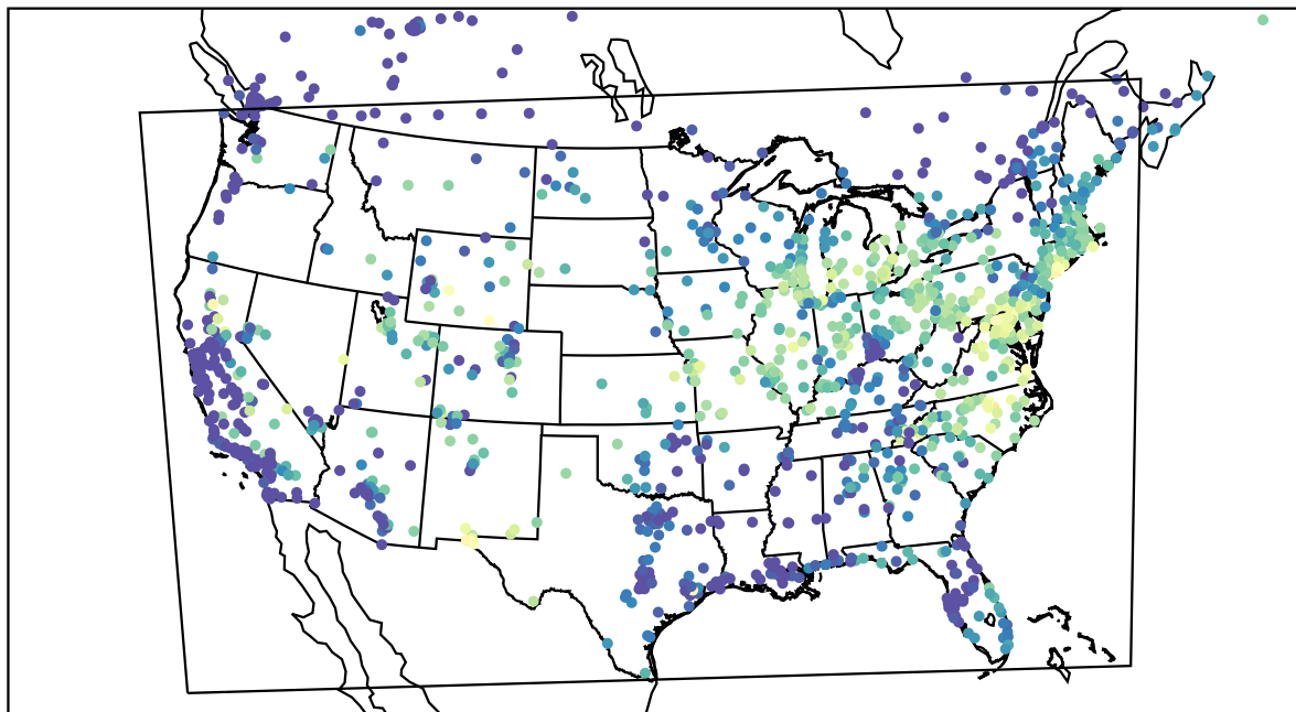
AirNOW (2023-08-12_14:00:00)
