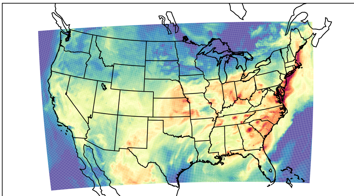
WRF (2023-08-13_18:00:00)
