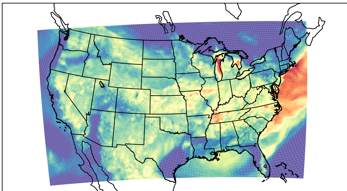
WRF (2023-08-12_03:00:00)
