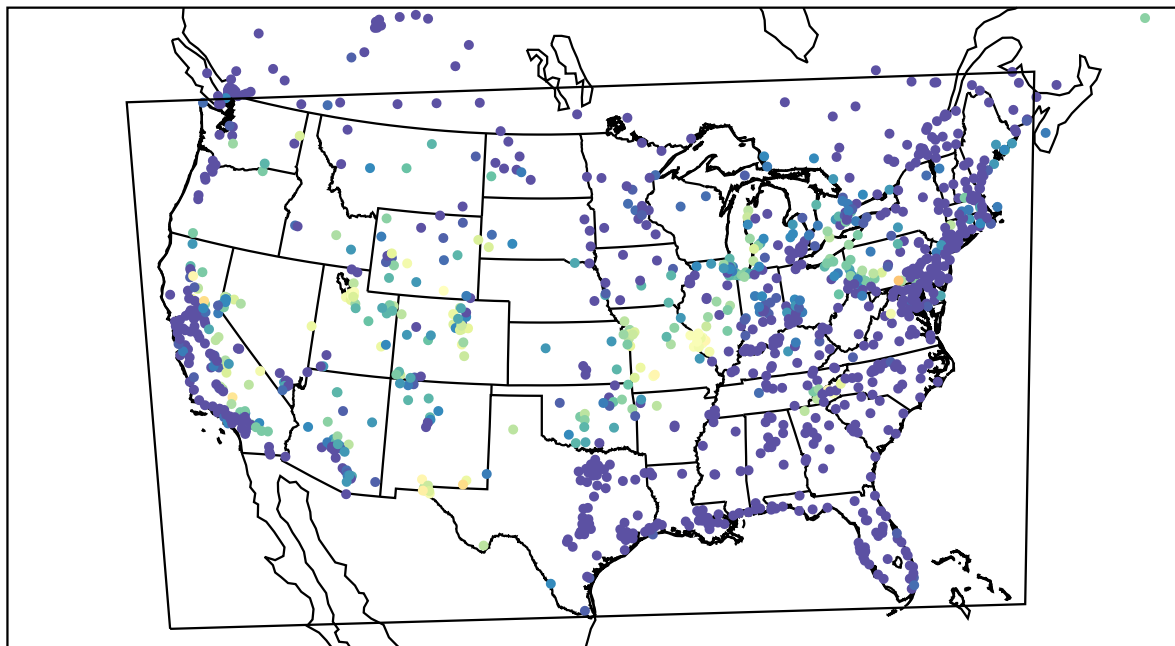
AirNOW (2023-08-12_10:00:00)
