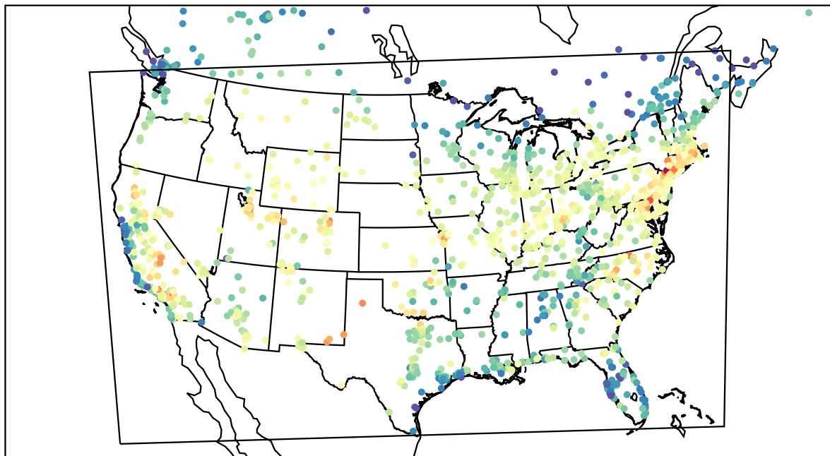
AirNOW (2023-08-12_19:00:00)
