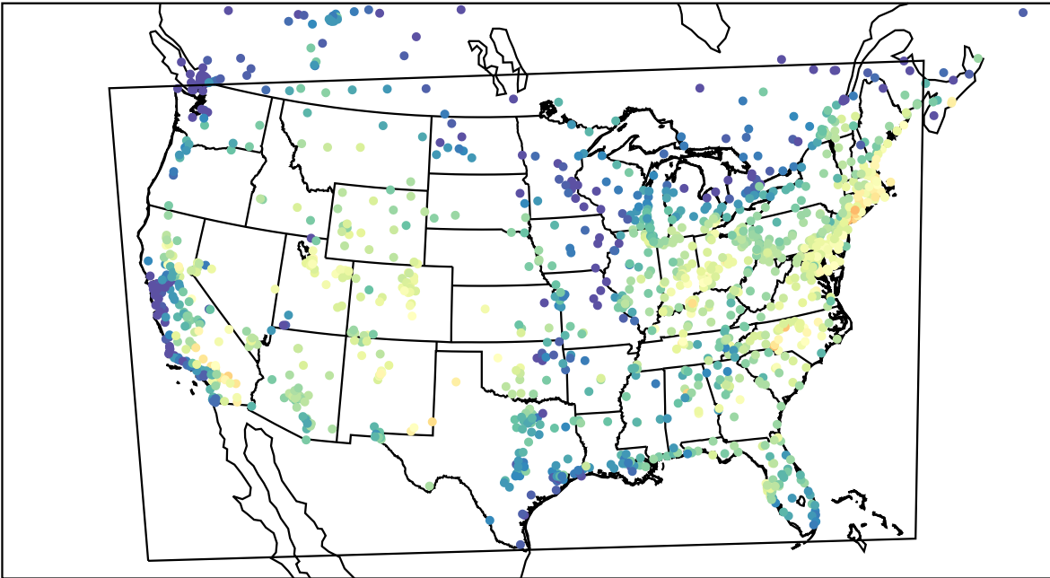
AirNOW (2023-08-13_16:00:00)
