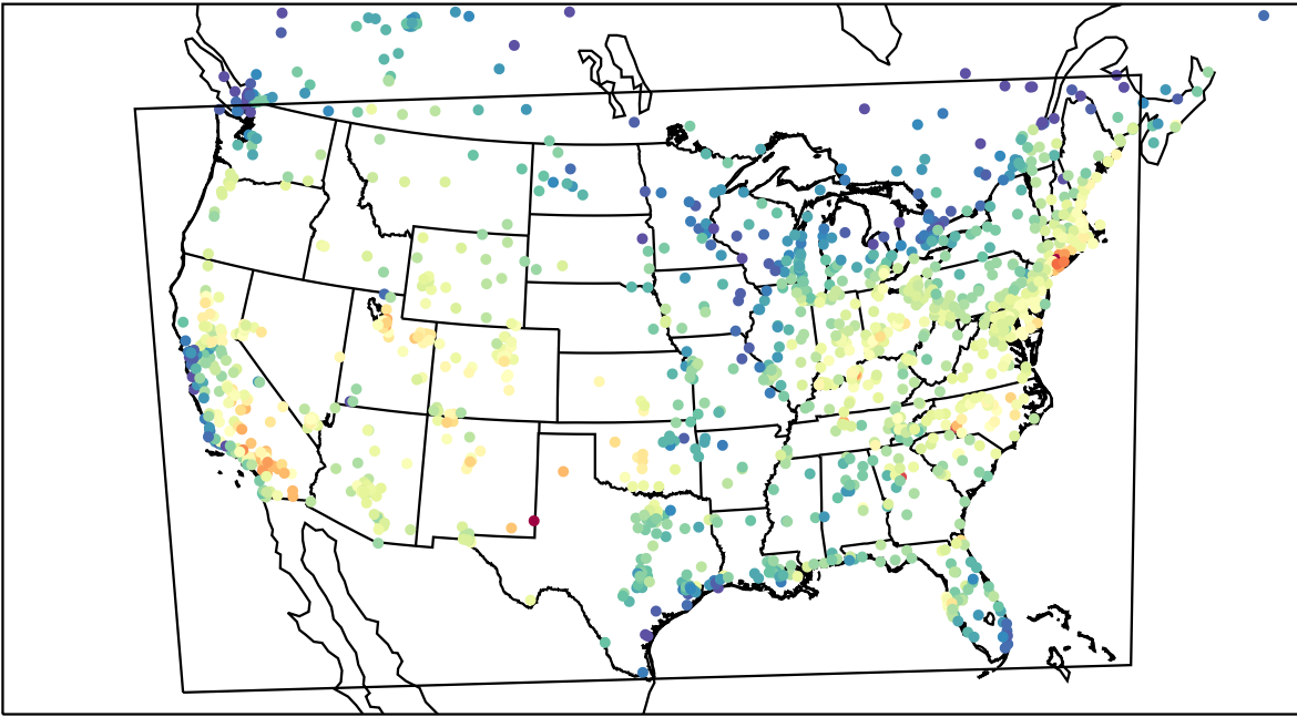
AirNOW (2023-08-13_18:00:00)
