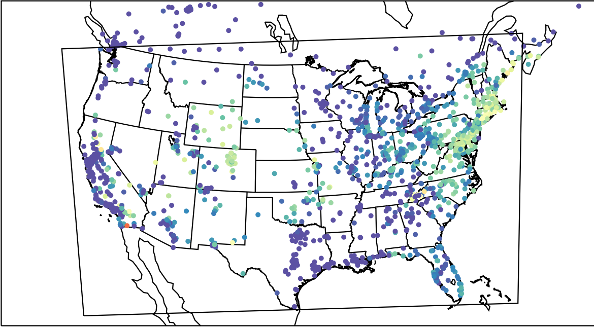
AirNOW (2023-08-13_13:00:00)
