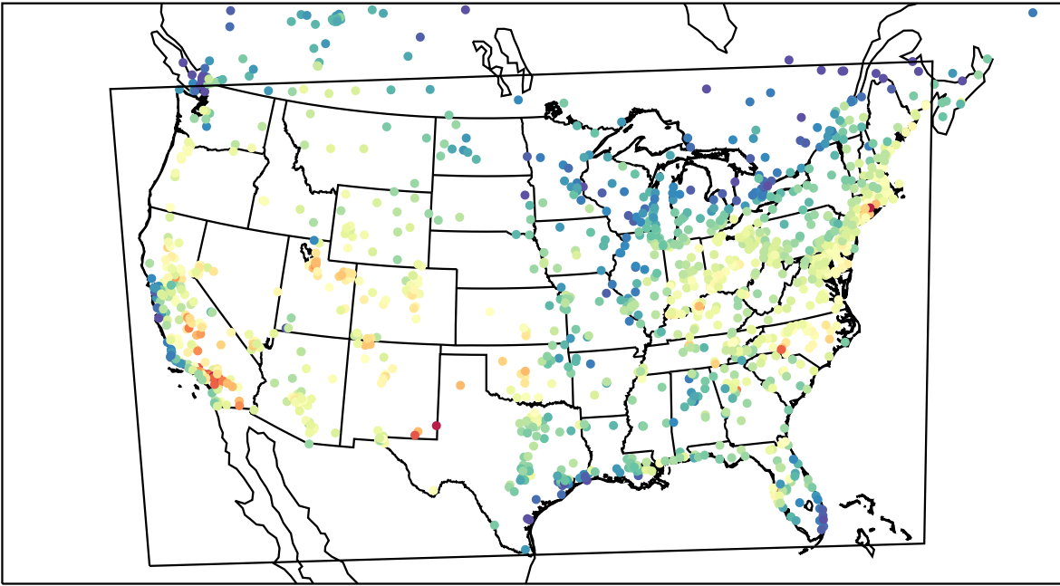
AirNOW (2023-08-13_19:00:00)
