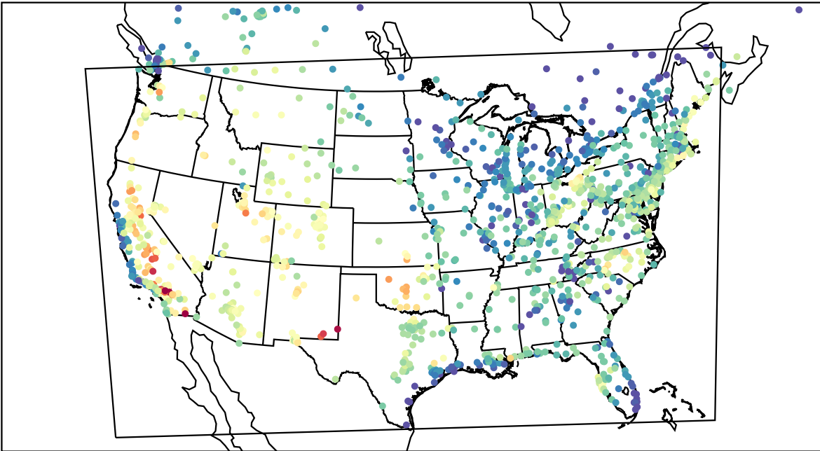
AirNOW (2023-08-13_23:00:00)
