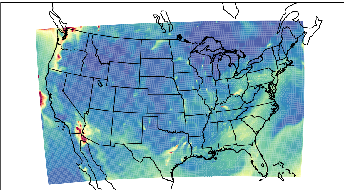
WRF 2023-08-15_13:00:00
