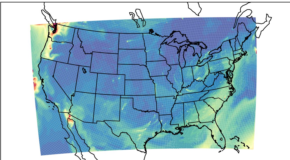
WRF 2023-08-15_18:00:00
