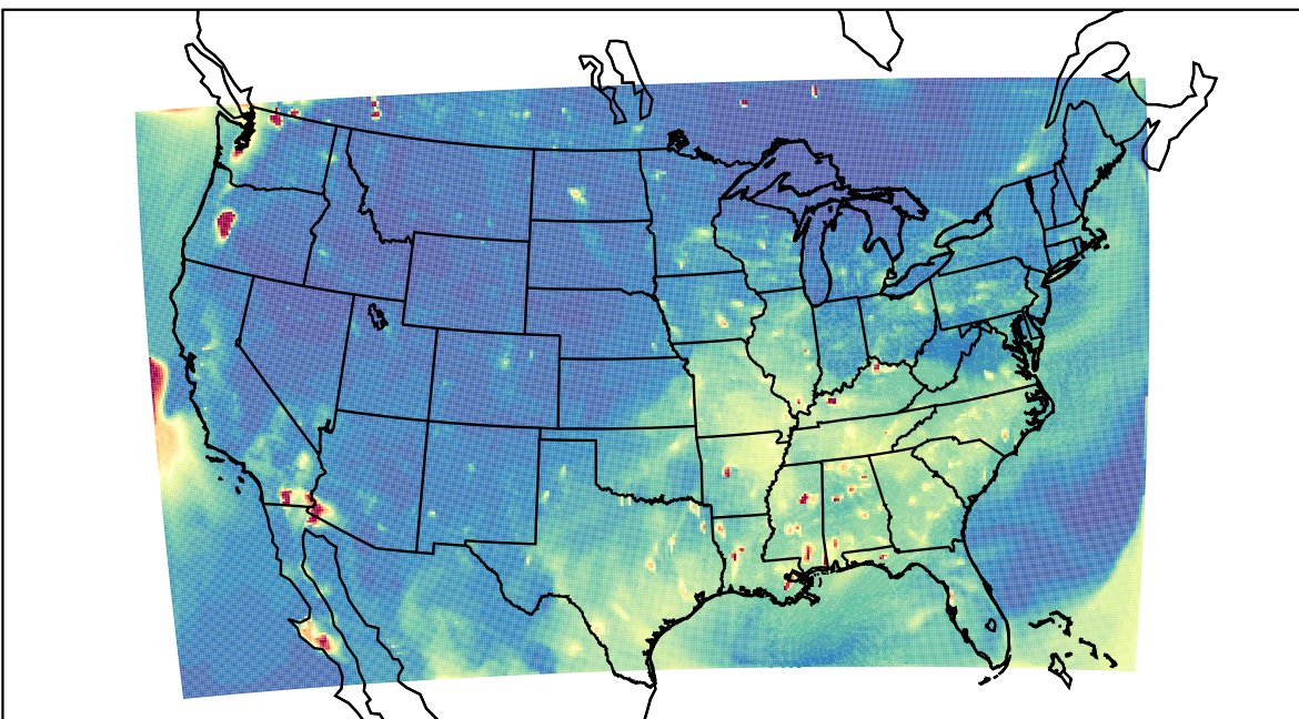
WRF 2023-08-14_03:00:00
