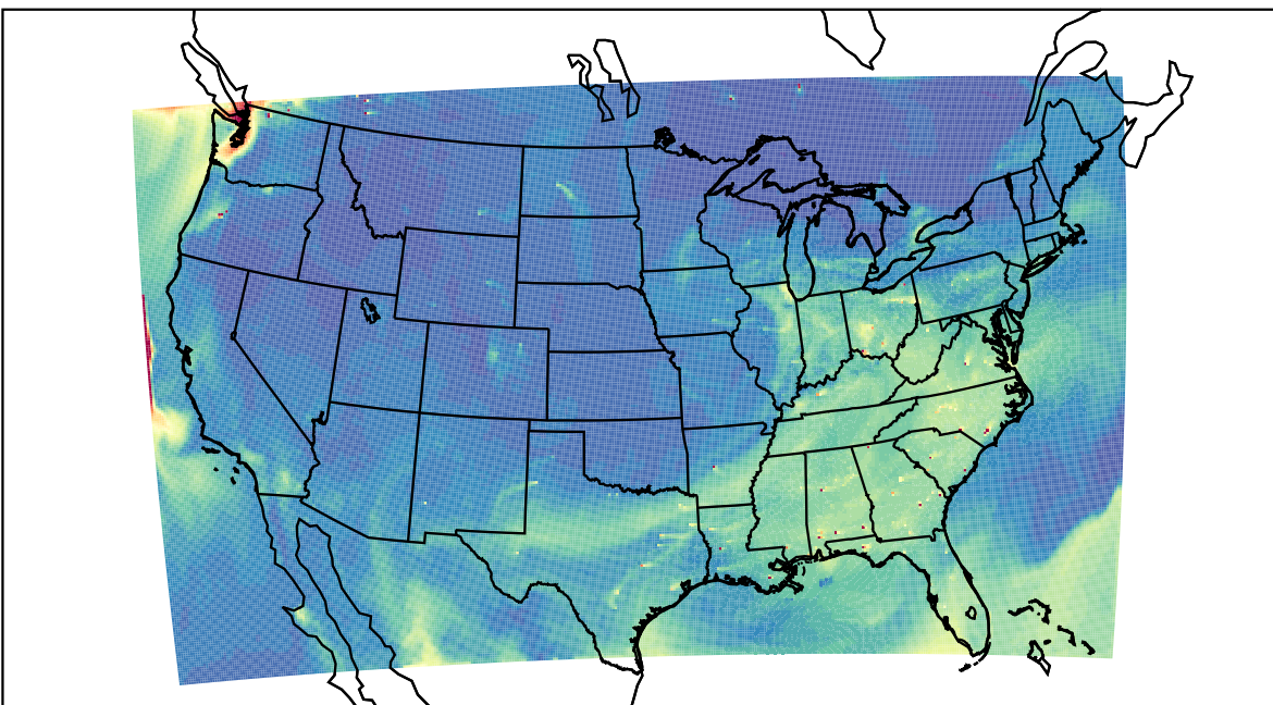
WRF 2023-08-14_20:00:00
