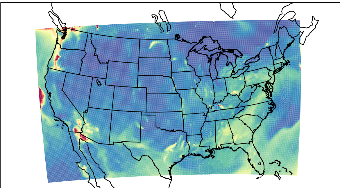
WRF 2023-08-15_10:00:00
