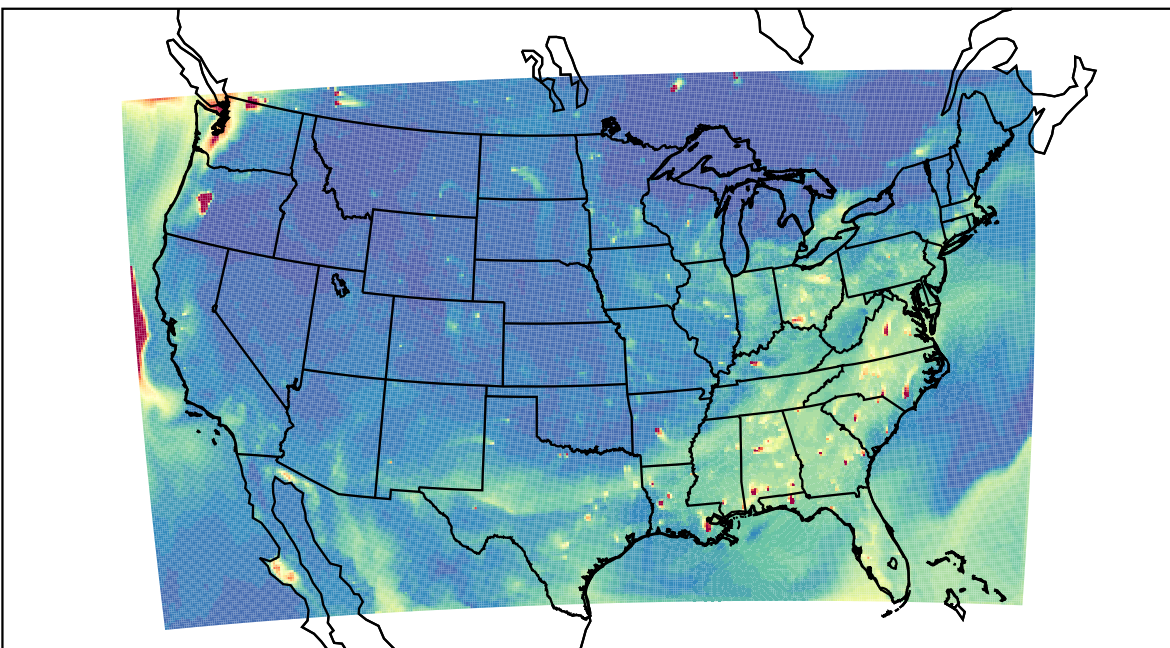
WRF 2023-08-15_01:00:00
