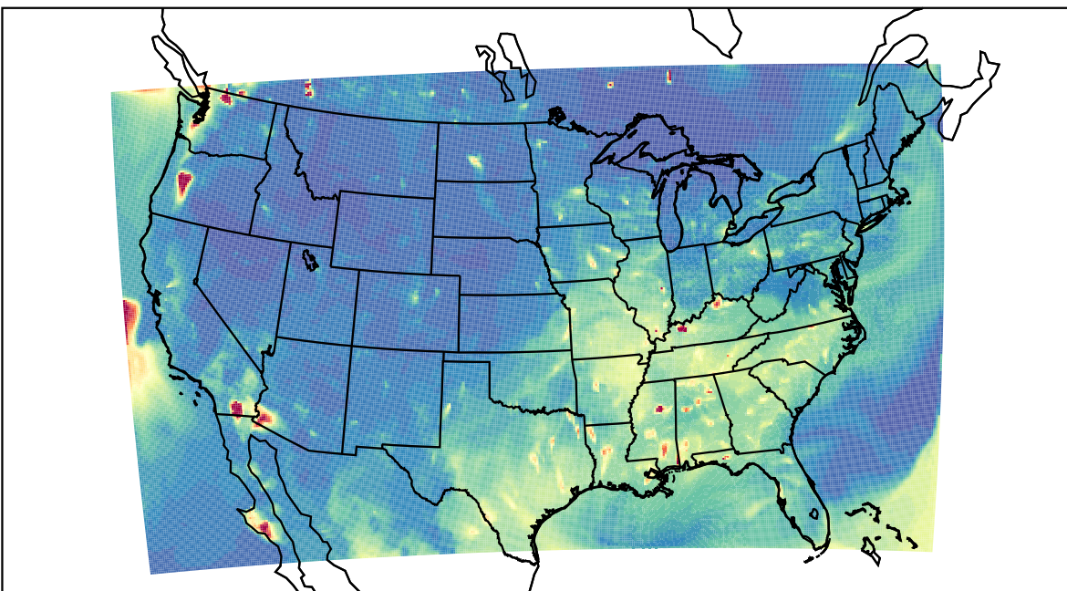
WRF 2023-08-14_04:00:00
