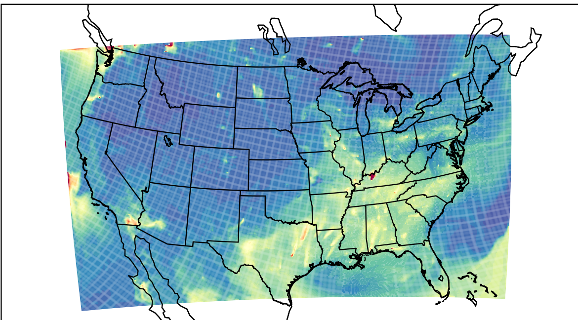
WRF 2023-08-14_10:00:00
