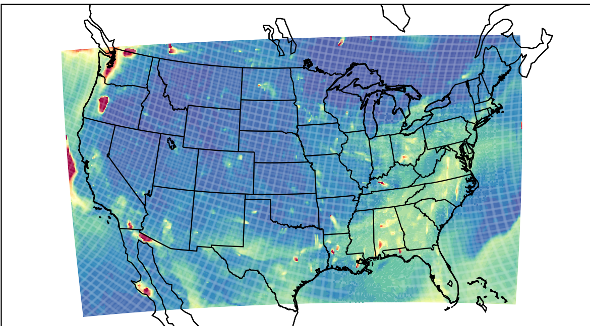
WRF 2023-08-15_03:00:00
