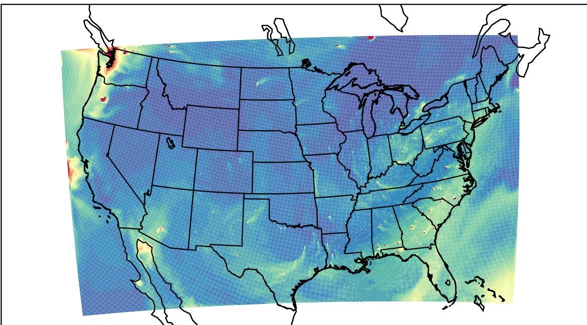
WRF 2023-08-15_22:00:00
