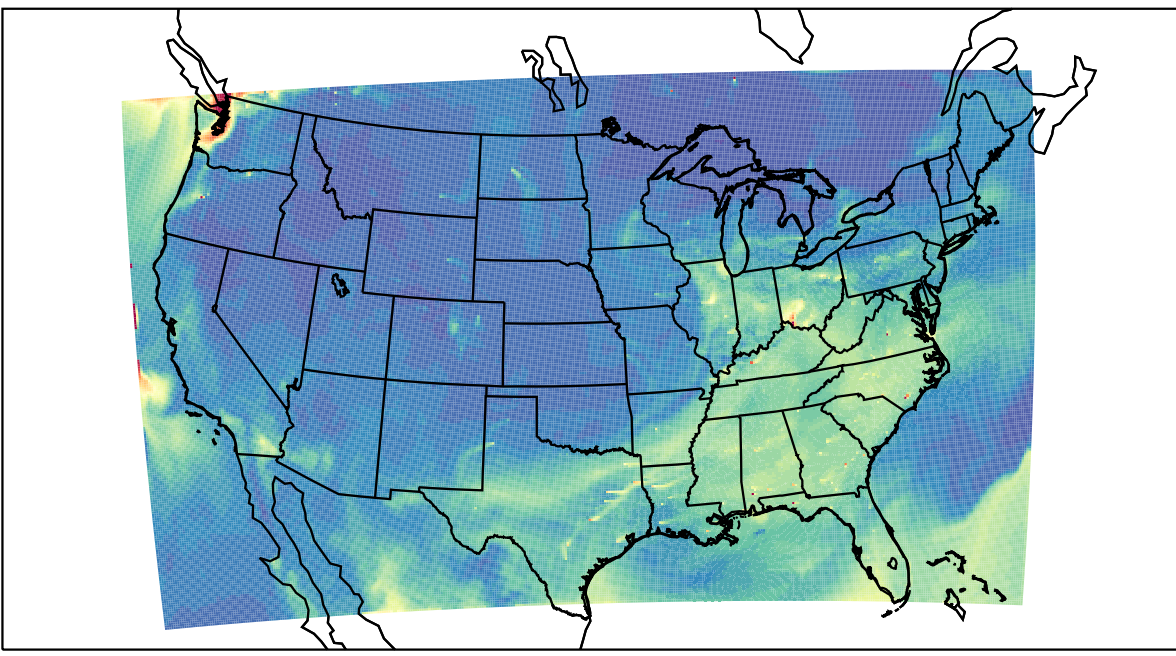
WRF 2023-08-14_18:00:00
