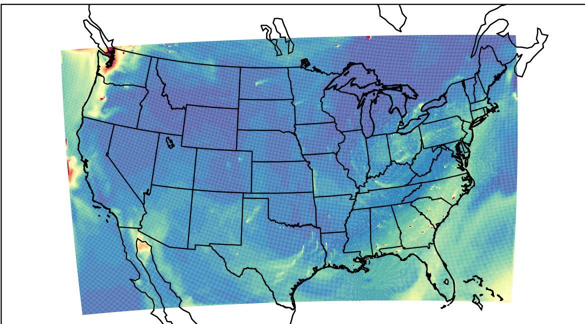
WRF 2023-08-15_20:00:00
