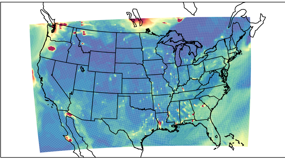
WRF 2023-08-16_02:00:00
