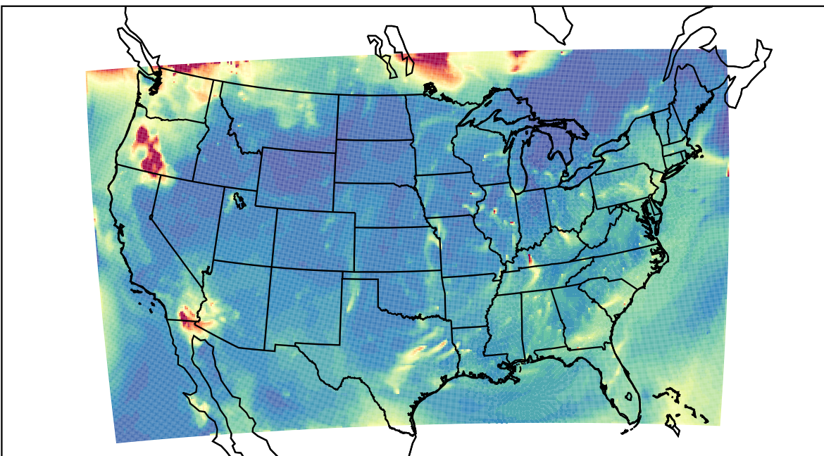
WRF 2023-08-16_10:00:00
