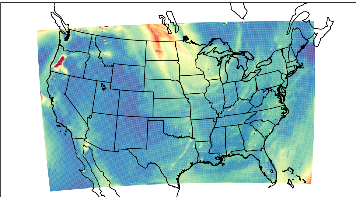
WRF 2023-08-17_20:00:00
