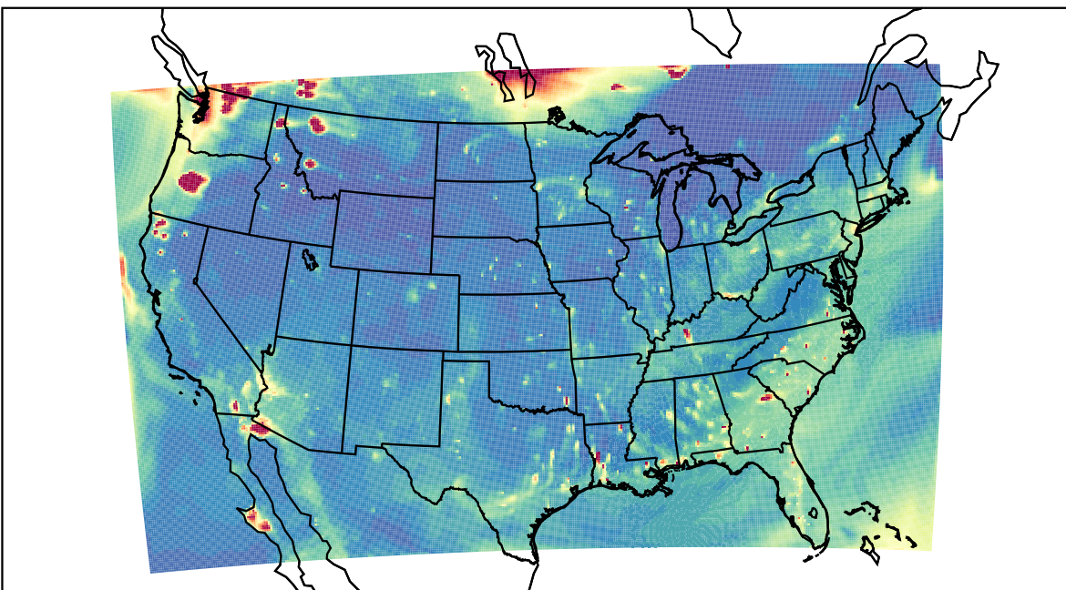
WRF 2023-08-16_02:00:00
