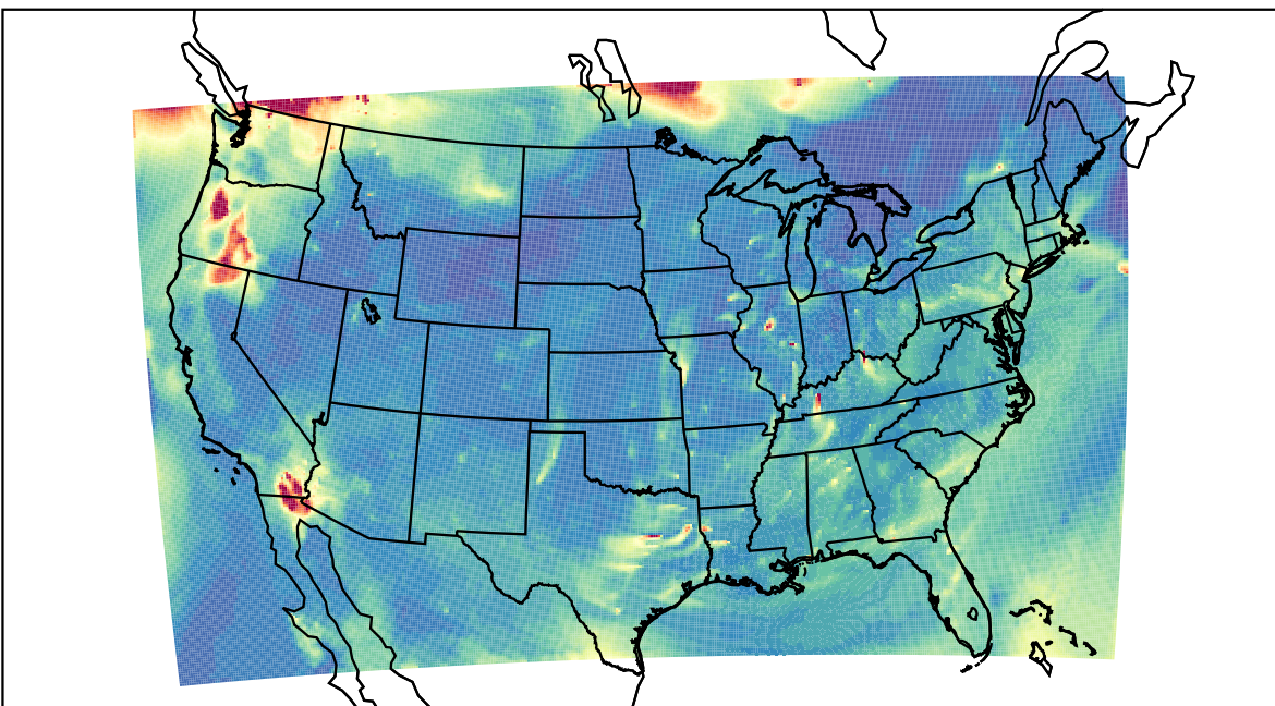
WRF 2023-08-16_13:00:00
