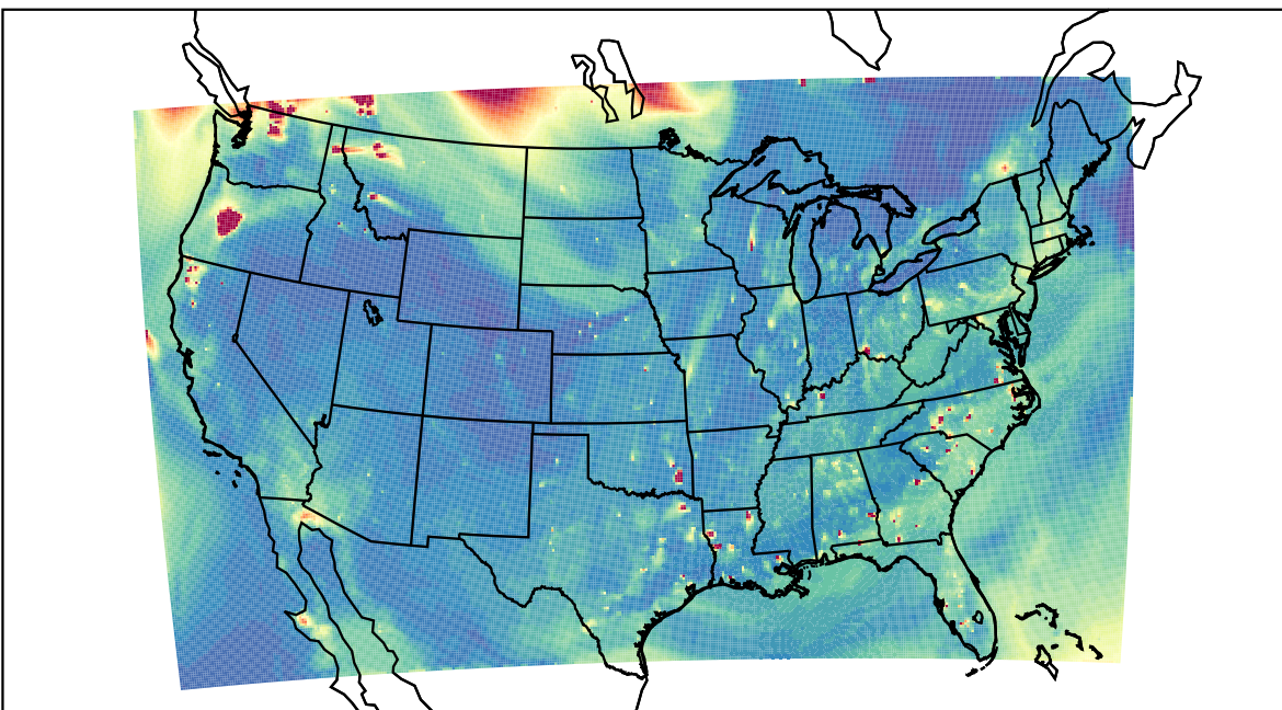
WRF 2023-08-17_01:00:00
