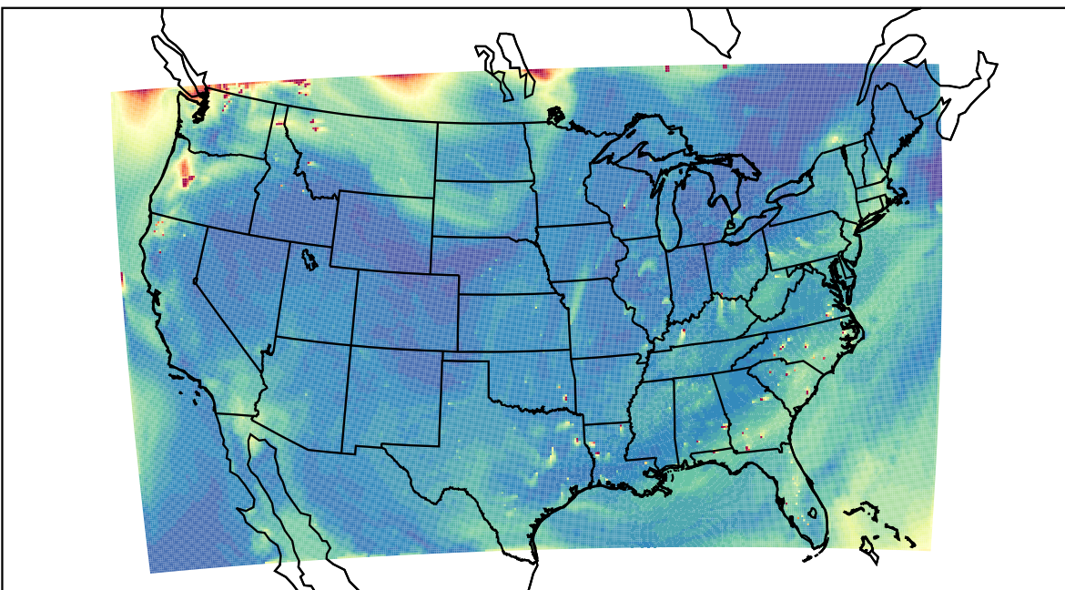
WRF 2023-08-16_21:00:00
