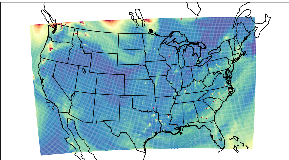
WRF 2023-08-16_22:00:00
