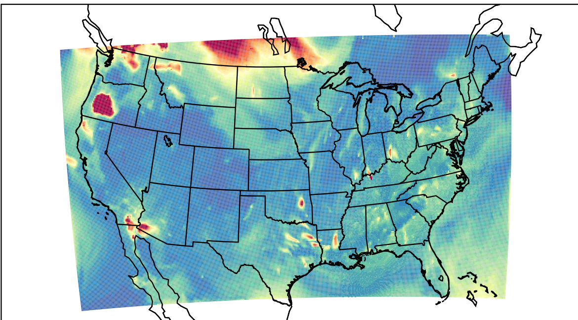
WRF 2023-08-17_06:00:00
