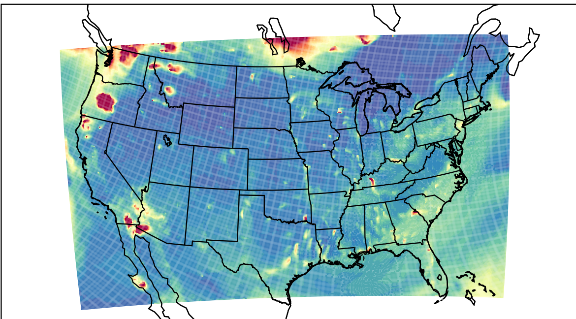
WRF 2023-08-16_04:00:00
