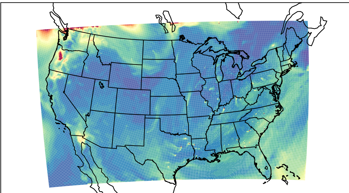
WRF 2023-08-16_18:00:00
