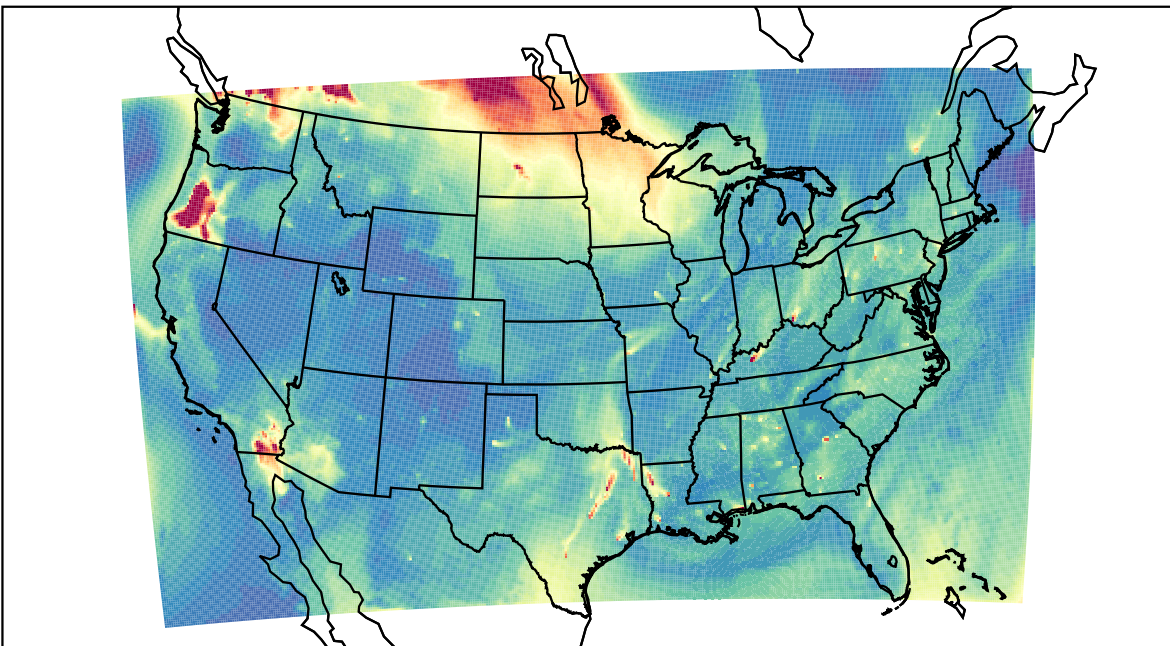
WRF 2023-08-17_14:00:00
