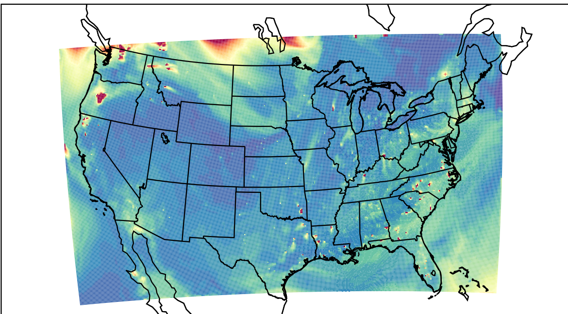
WRF 2023-08-17_00:00:00
