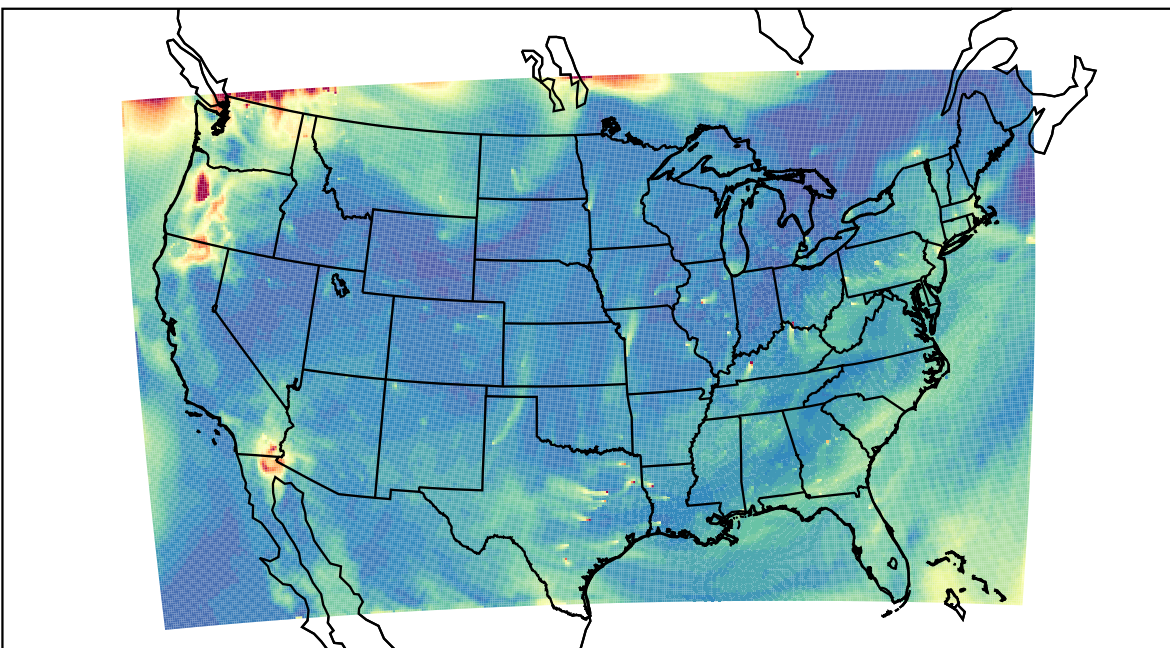
WRF 2023-08-16_16:00:00
