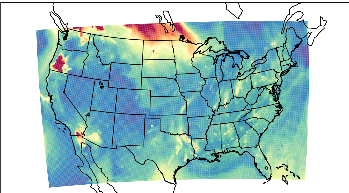
WRF 2023-08-17_12:00:00
