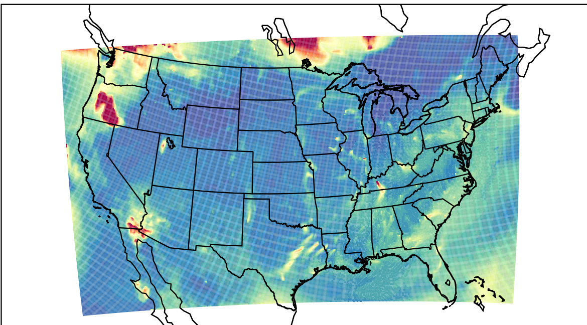
WRF 2023-08-16_08:00:00
