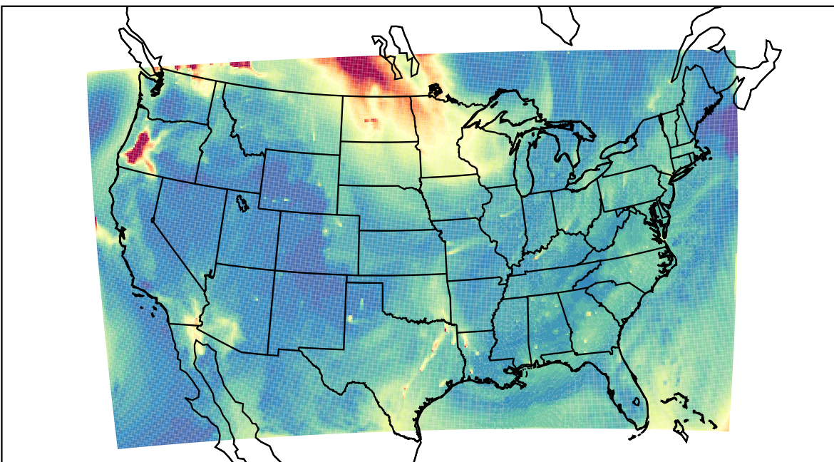
WRF 2023-08-17_16:00:00
