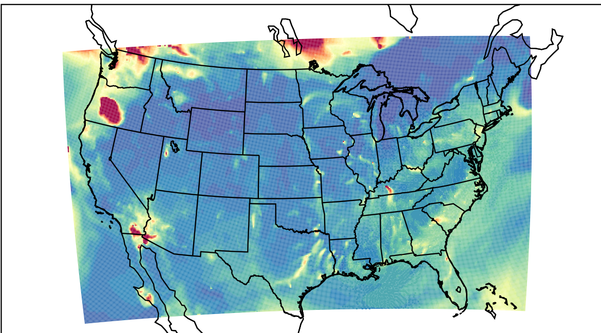
WRF 2023-08-16_06:00:00
