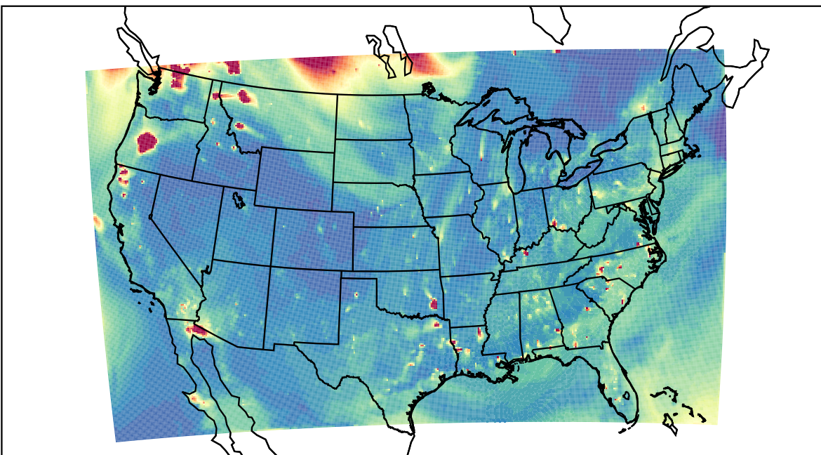
WRF 2023-08-17_02:00:00
