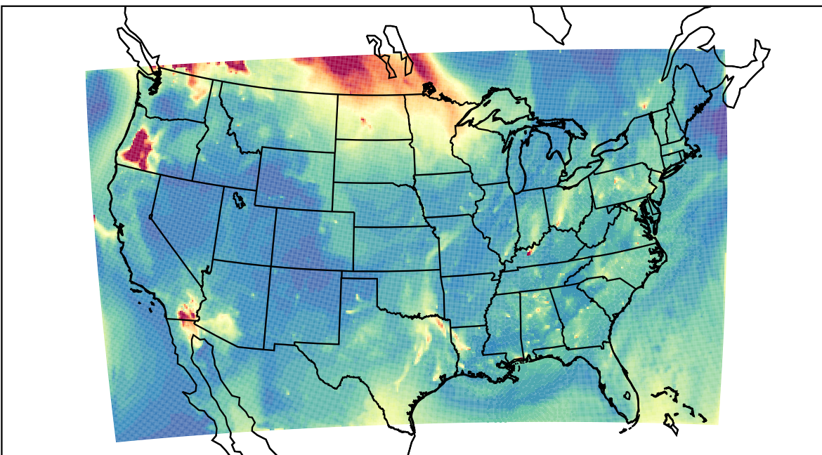
WRF 2023-08-17_13:00:00
