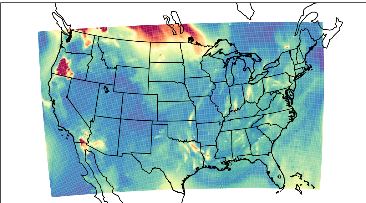
WRF 2023-08-17_10:00:00
