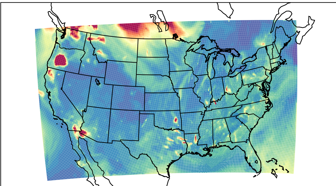
WRF 2023-08-17_05:00:00
