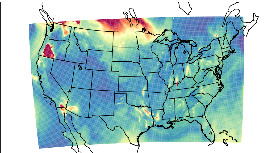
WRF 2023-08-17_09:00:00
