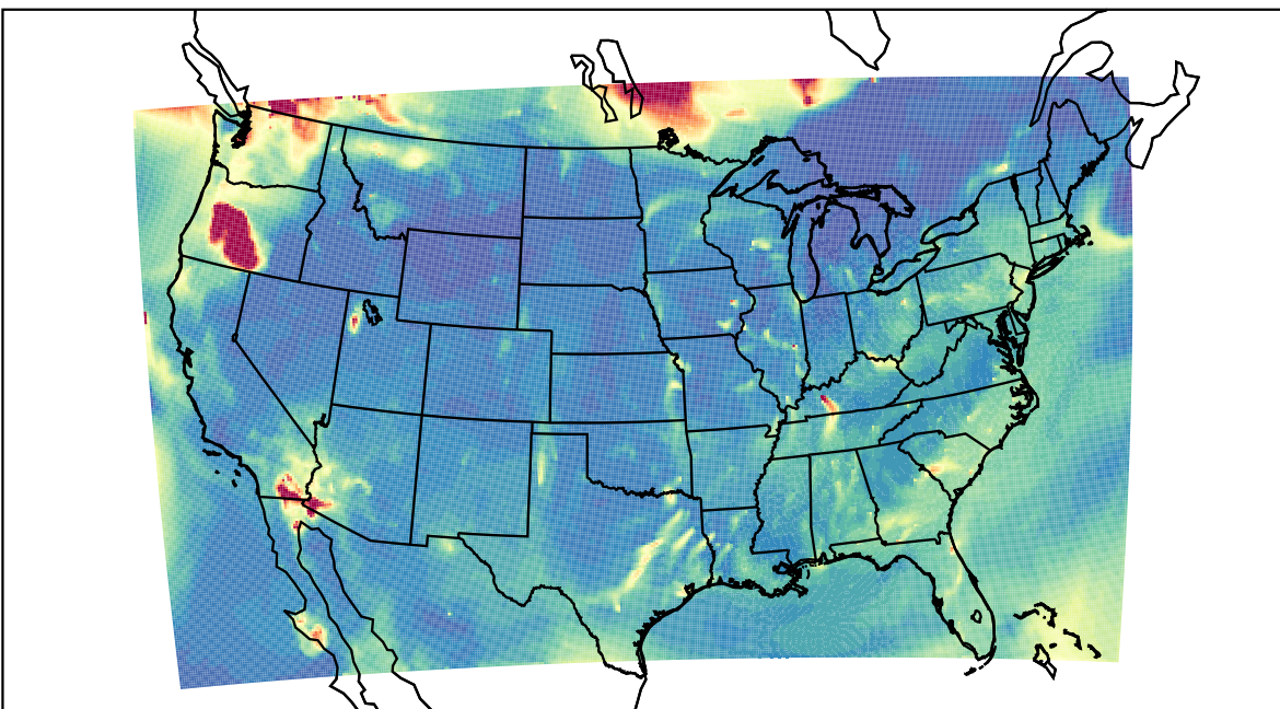
WRF 2023-08-16_07:00:00
