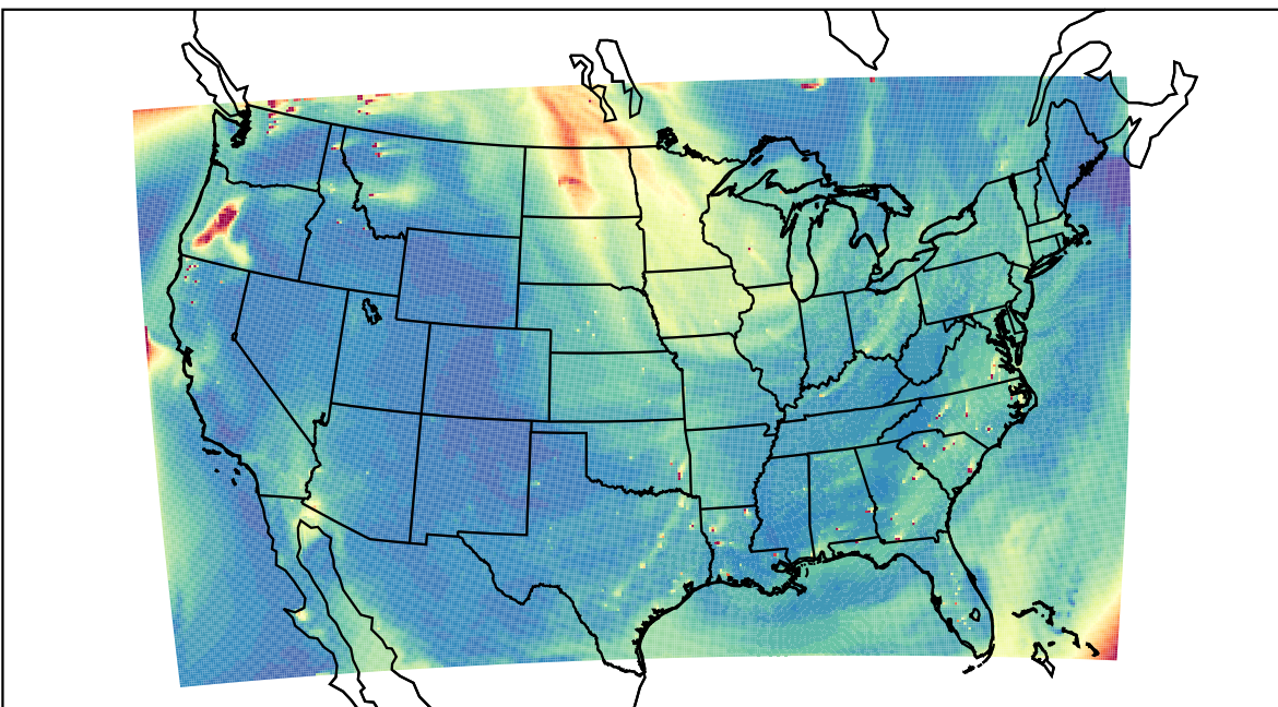
WRF 2023-08-17_22:00:00
