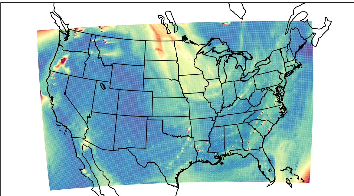
WRF 2023-08-17_23:00:00
