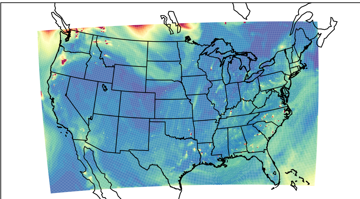
WRF 2023-08-16_23:00:00
