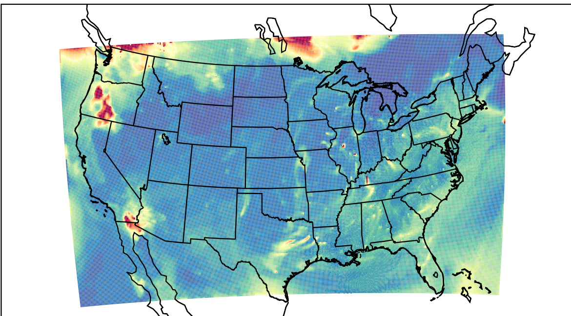
WRF 2023-08-16_11:00:00
