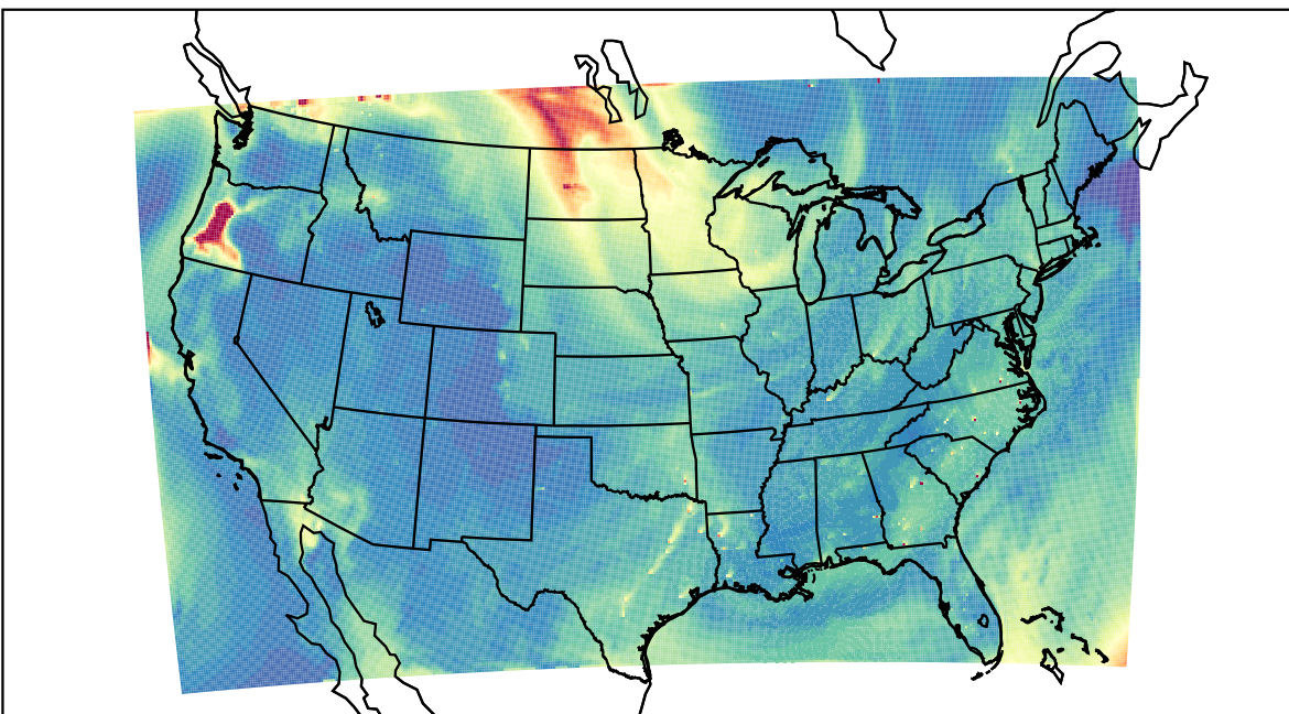
WRF 2023-08-17_18:00:00
