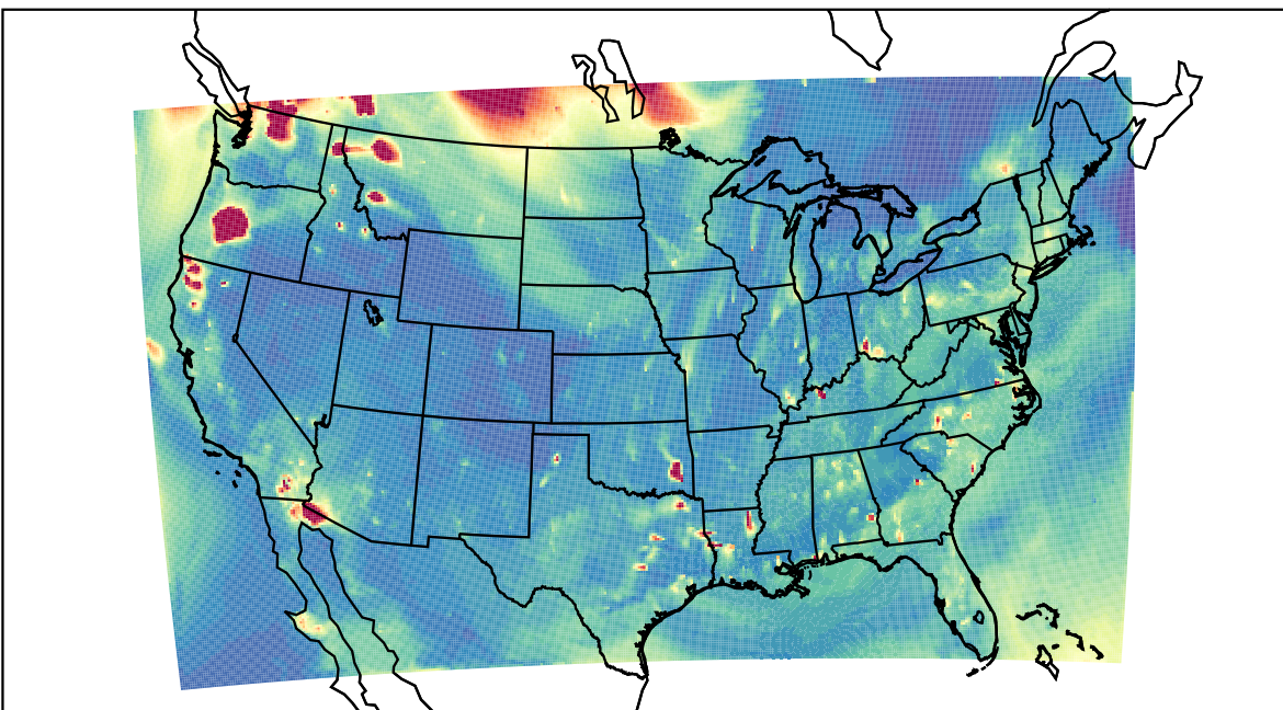
WRF 2023-08-17_03:00:00
