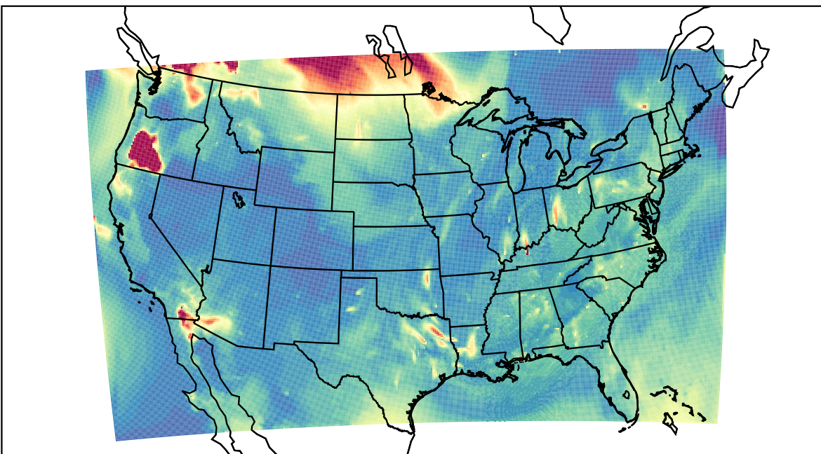
WRF 2023-08-17_08:00:00
