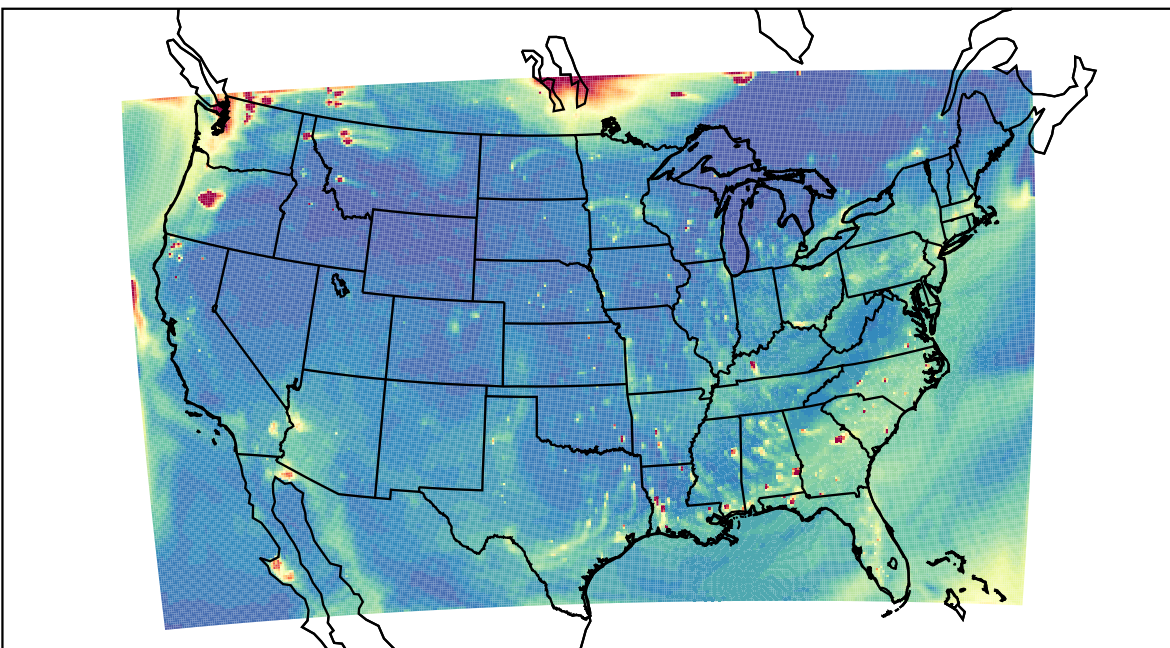
WRF 2023-08-16_01:00:00
