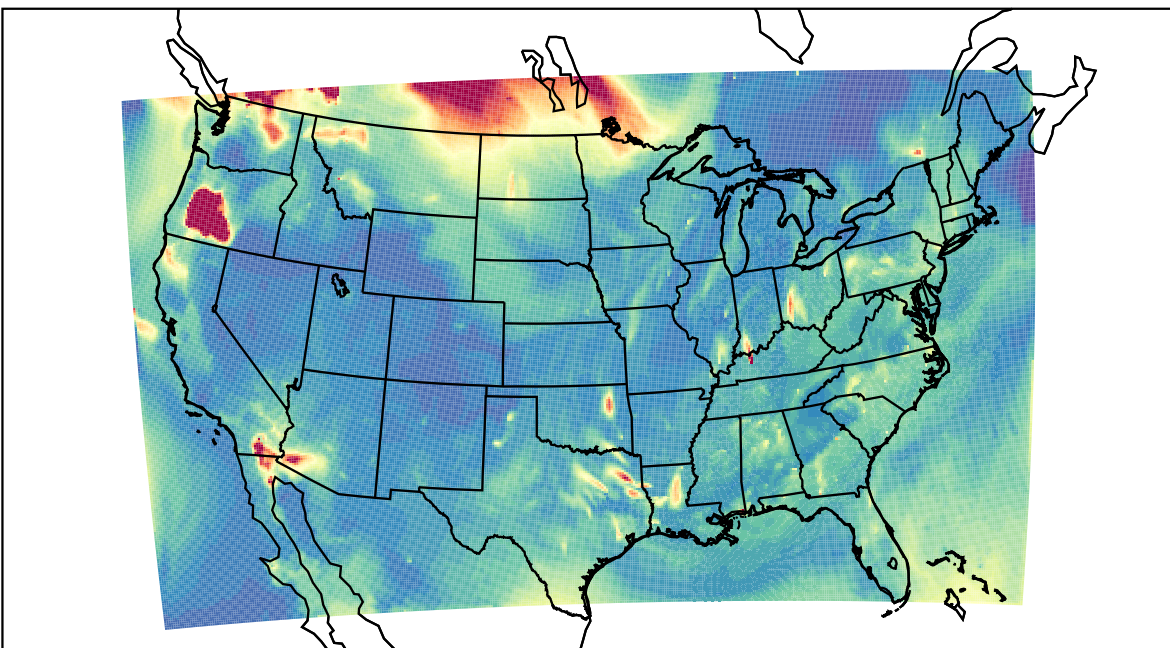
WRF 2023-08-17_07:00:00
