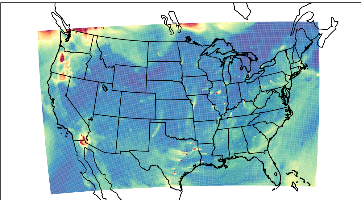
WRF 2023-08-16_15:00:00
