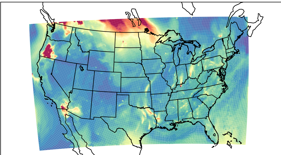
WRF 2023-08-17_11:00:00
