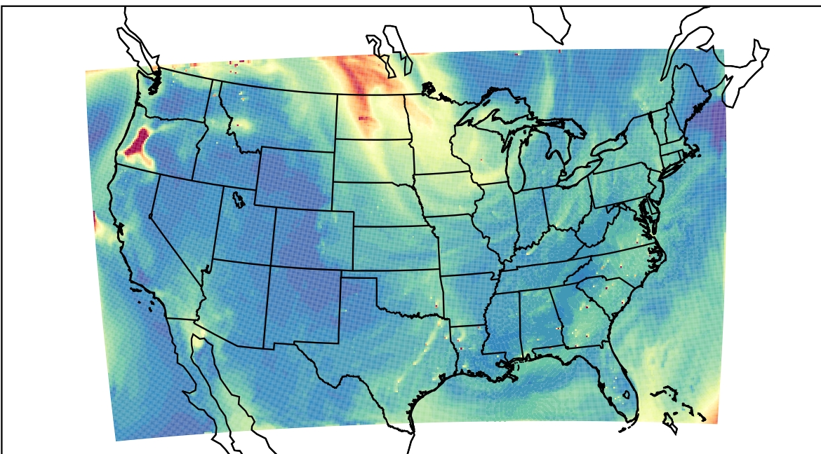
WRF 2023-08-17_19:00:00
