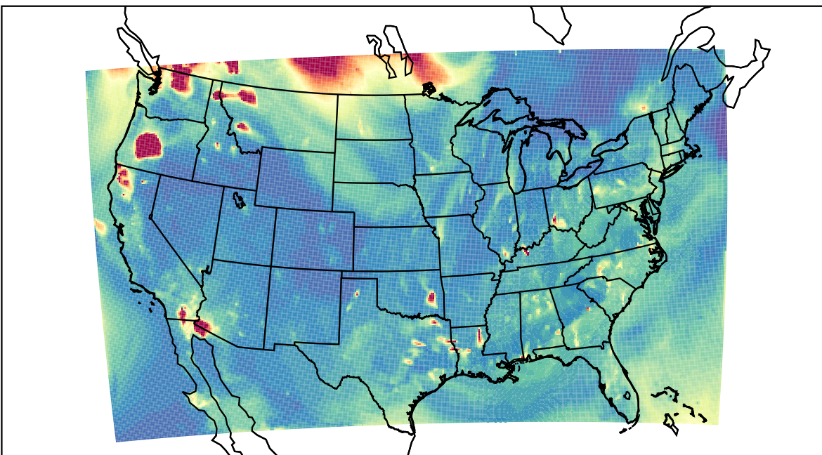
WRF 2023-08-17_04:00:00
