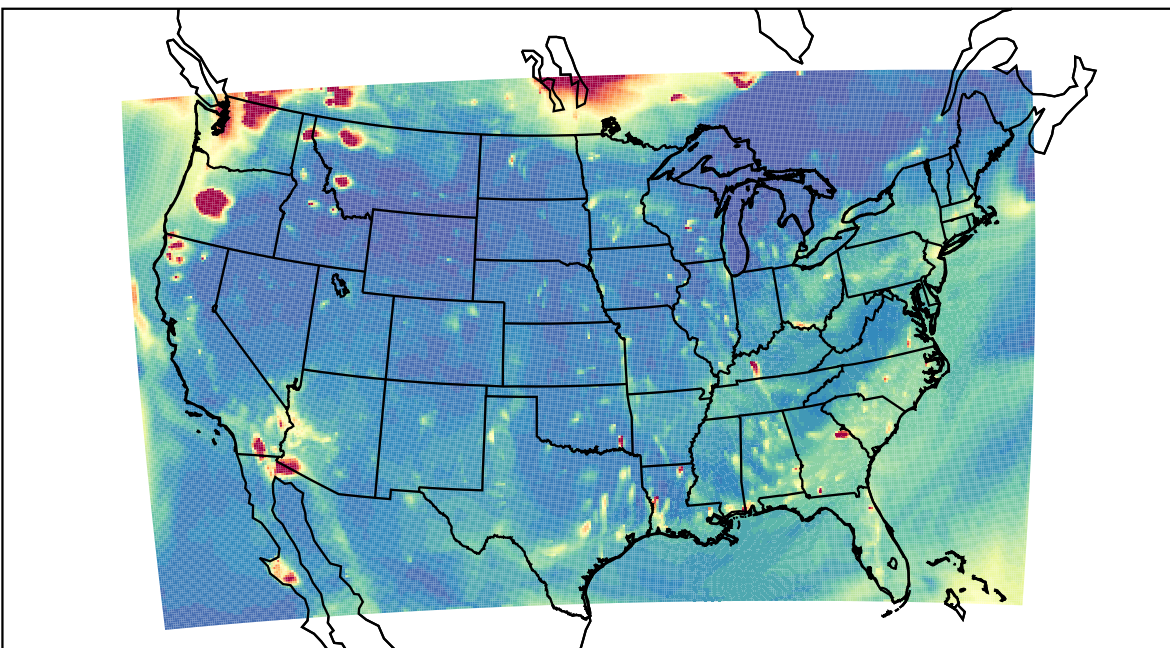
WRF 2023-08-16_03:00:00
