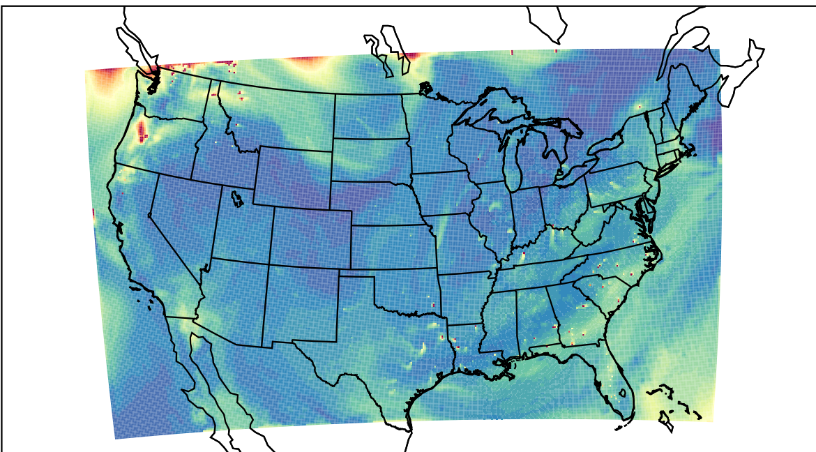
WRF 2023-08-16_20:00:00
