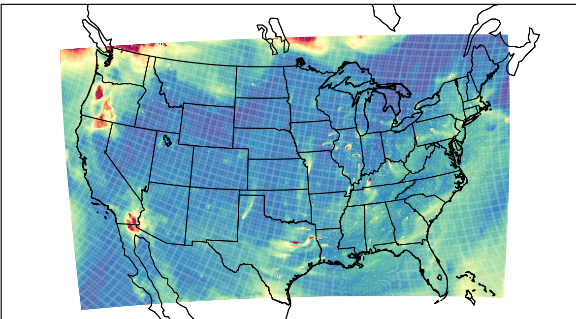
WRF 2023-08-16_14:00:00
