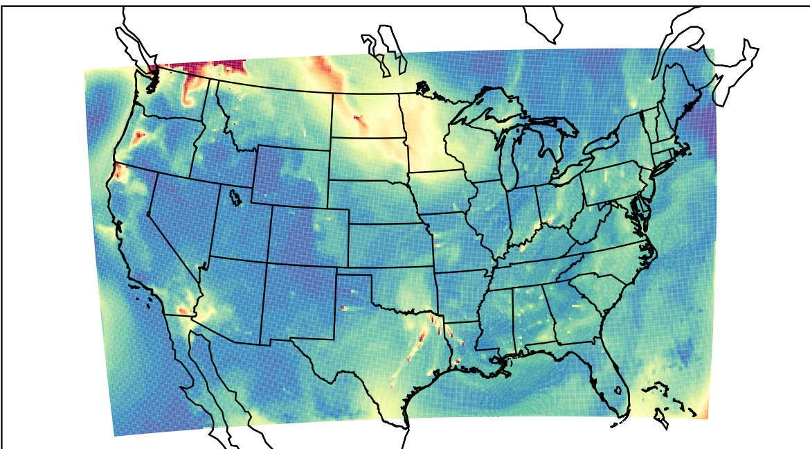
WRF 2023-08-17_15:00:00
