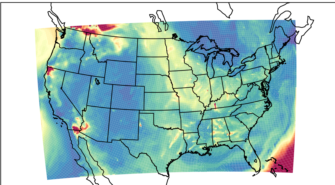
WRF 2023-08-18_11:00:00
