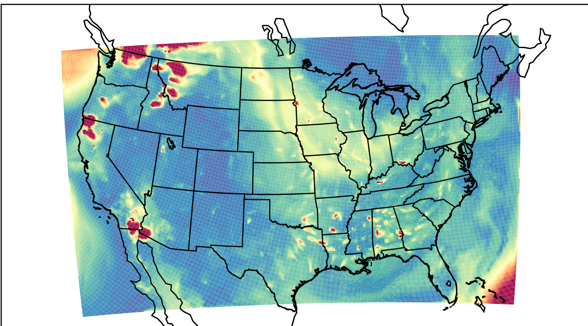
WRF 2023-08-18_04:00:00
