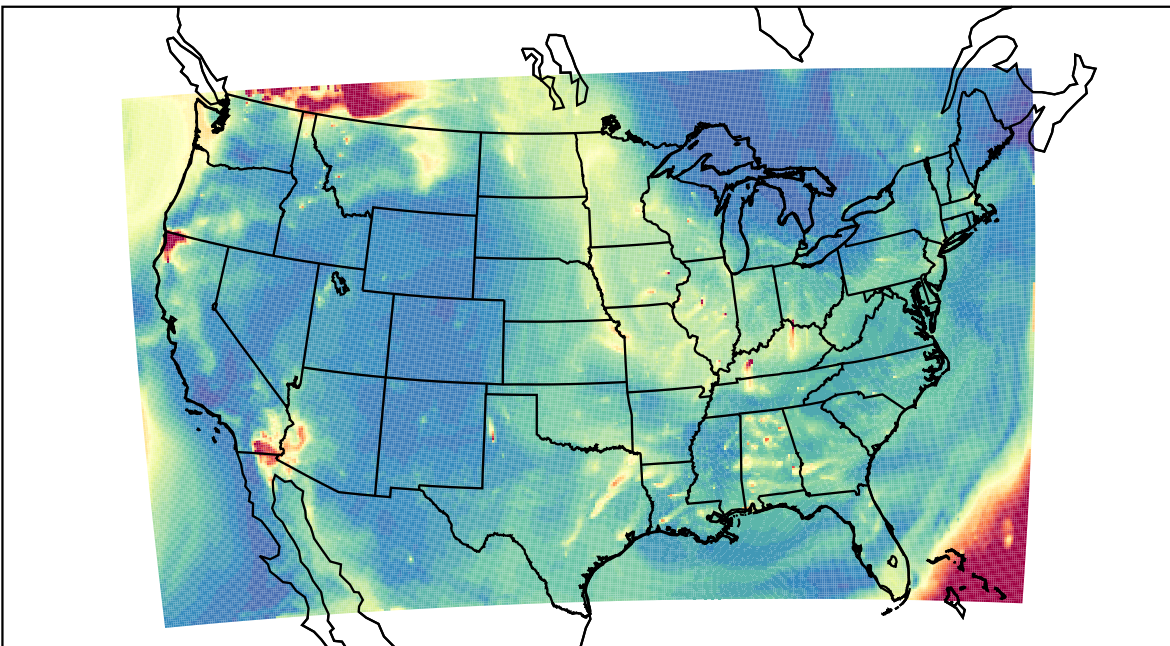
WRF 2023-08-18_13:00:00
