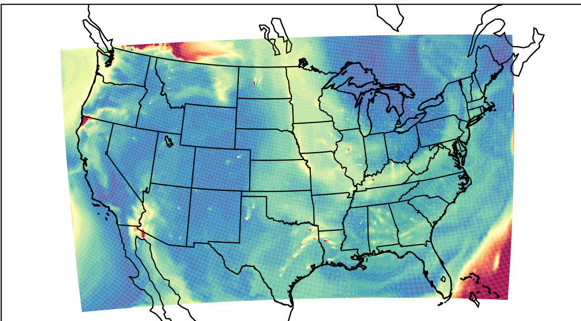
WRF 2023-08-18_16:00:00
