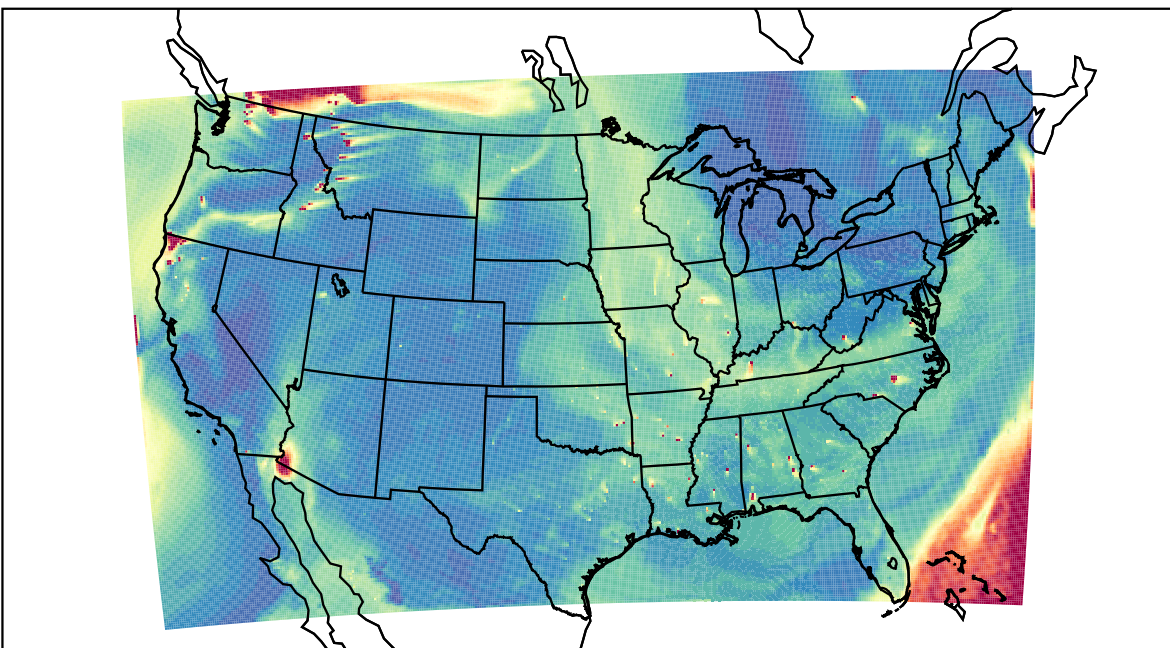
WRF 2023-08-18_23:00:00
