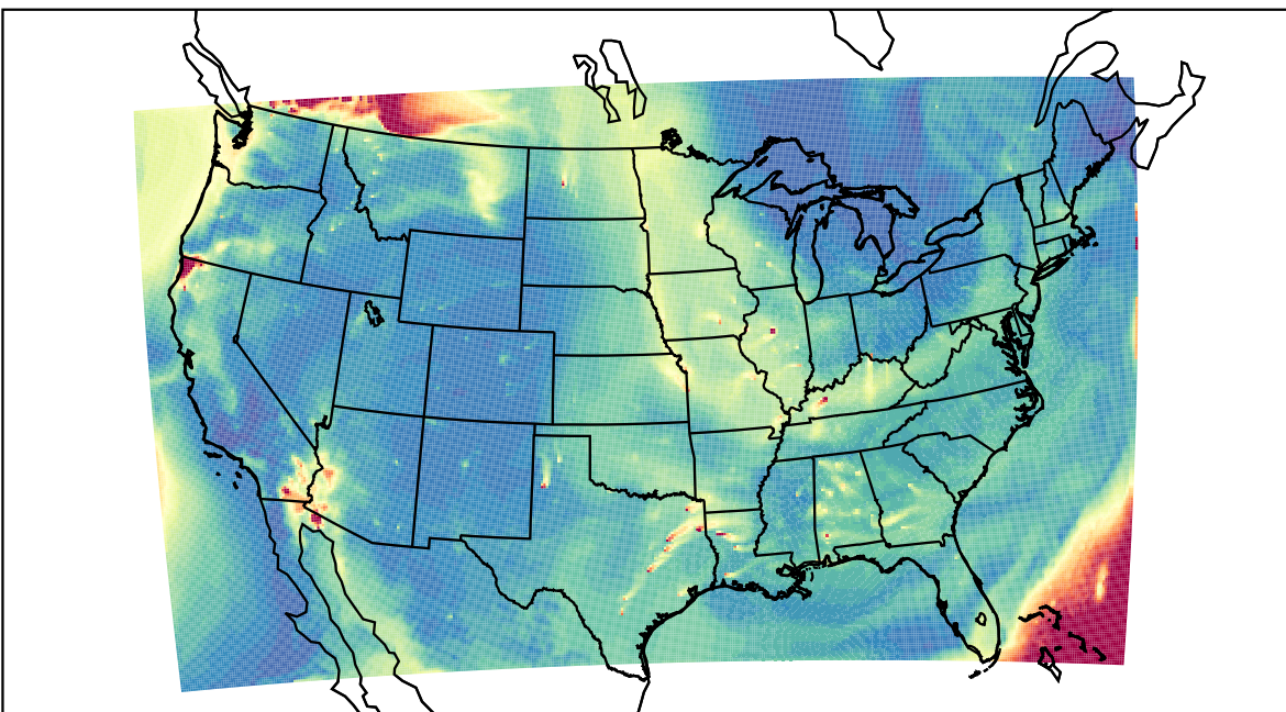
WRF 2023-08-18_15:00:00
