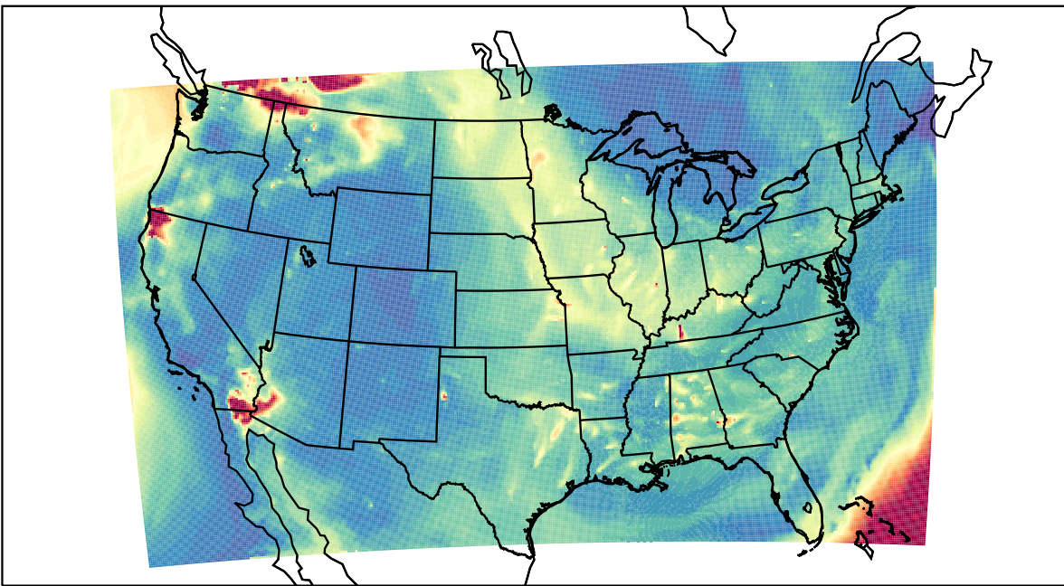
WRF 2023-08-18_10:00:00
