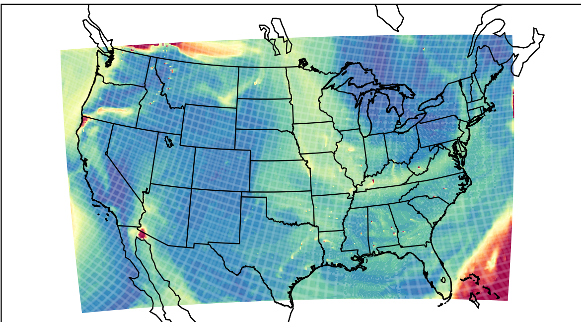
WRF 2023-08-18_19:00:00
