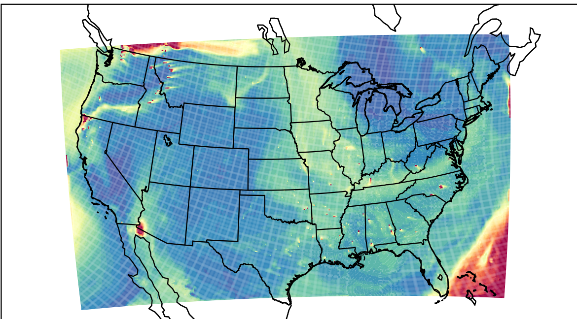
WRF 2023-08-18_22:00:00
