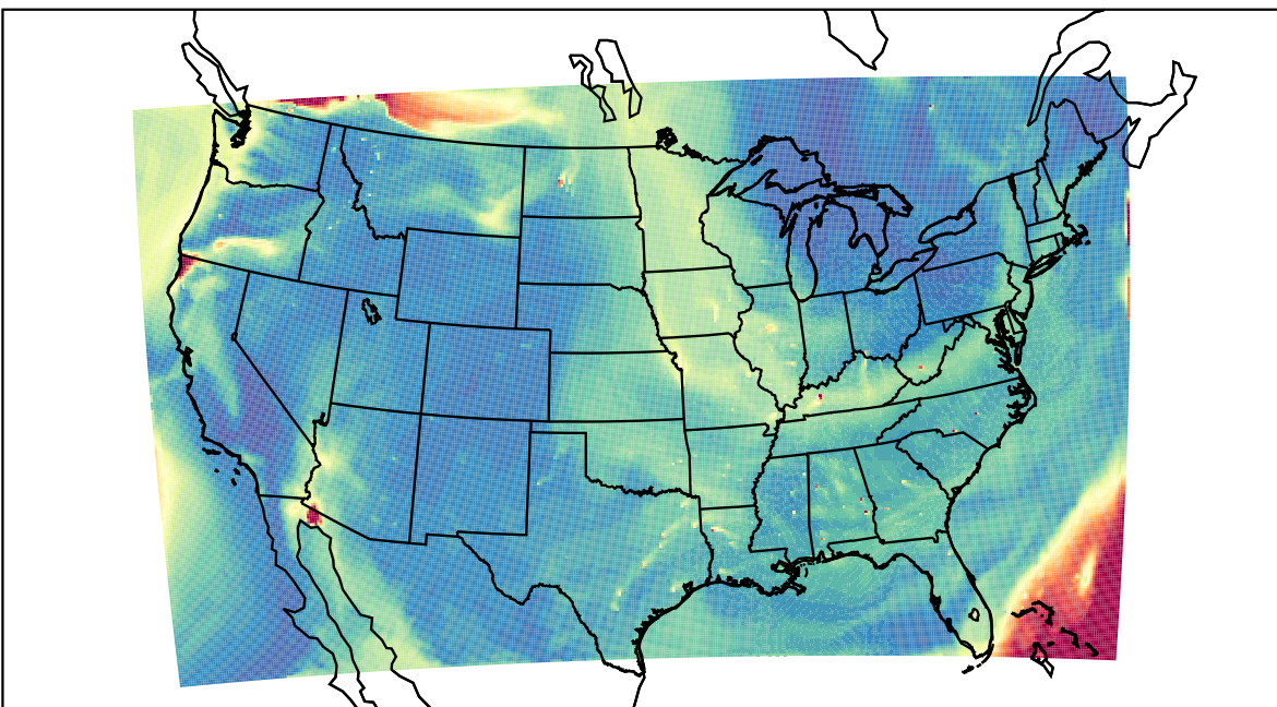
WRF 2023-08-18_18:00:00
