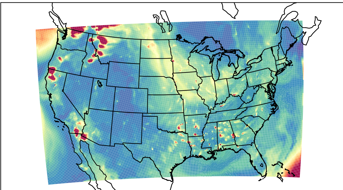
WRF 2023-08-18_03:00:00
