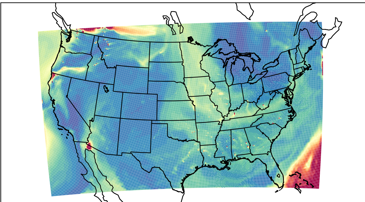
WRF 2023-08-18_20:00:00
