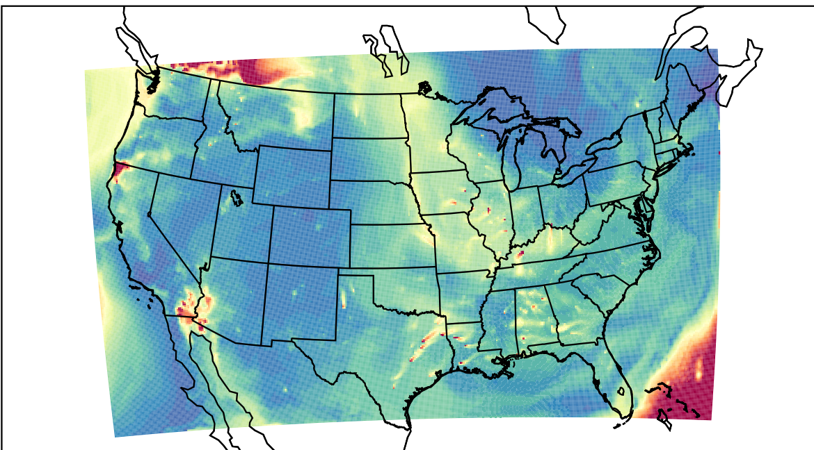
WRF 2023-08-18_14:00:00
