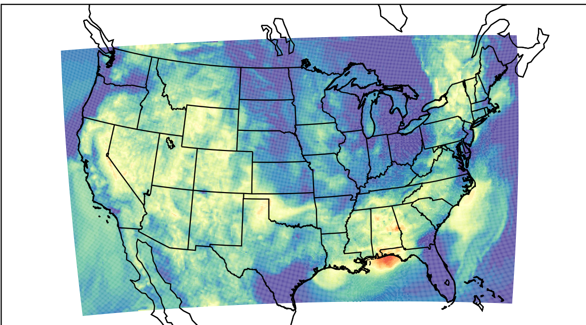
WRF (2023-08-18_10:00:00)
