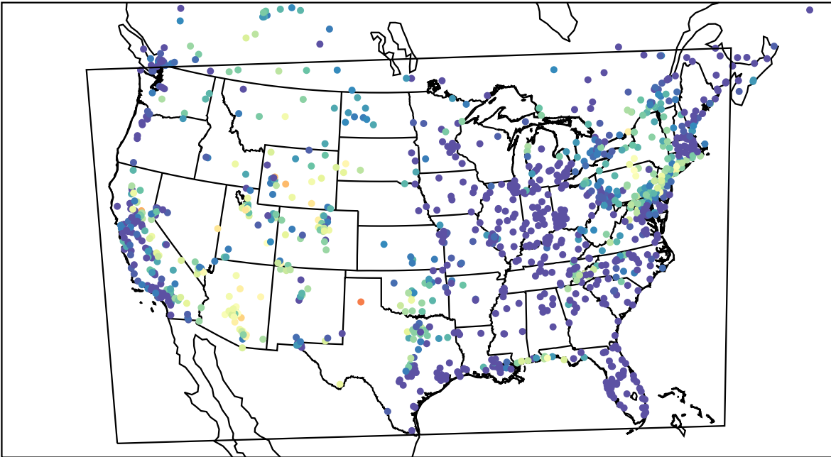
AirNOW (2023-08-18_10:00:00)
