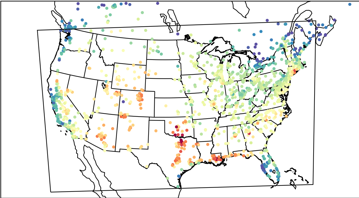
AirNOW (2023-08-18_18:00:00)
