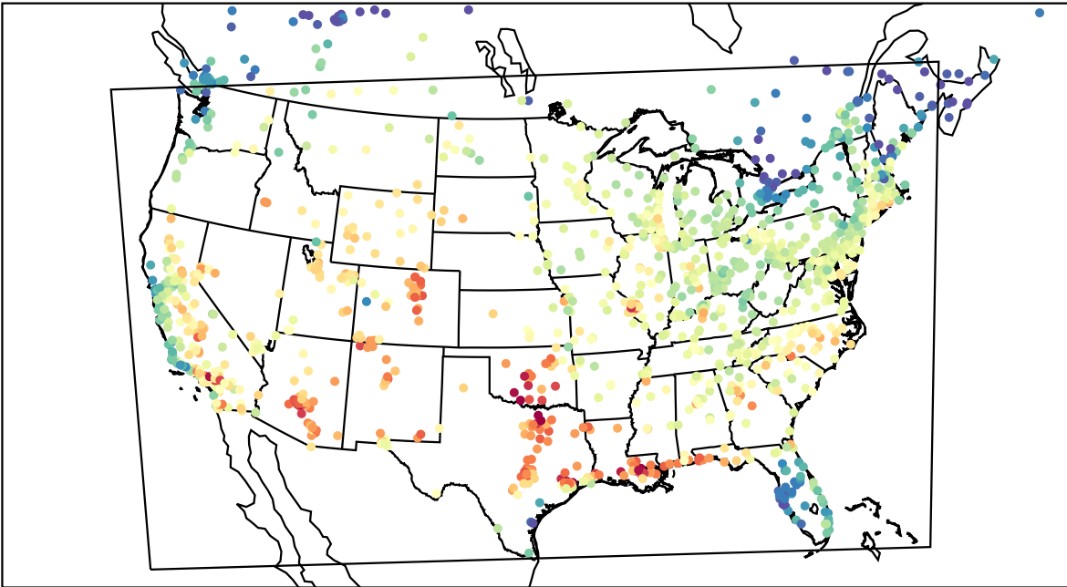
AirNOW (2023-08-18_20:00:00)
