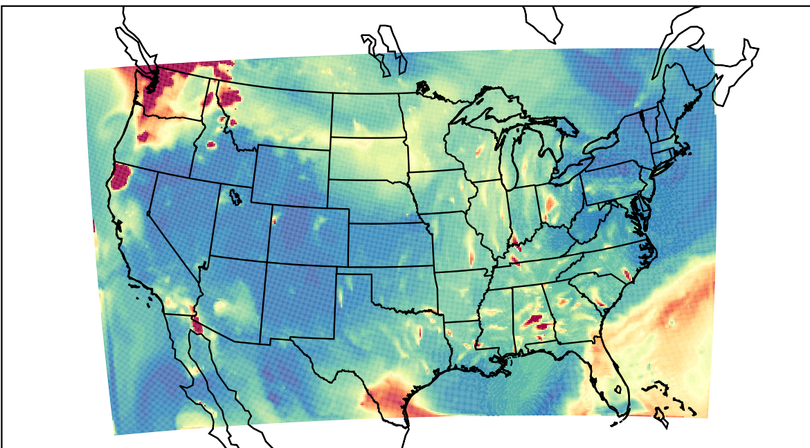
WRF 2023-08-20_04:00:00
