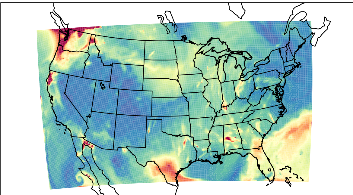
WRF 2023-08-20_08:00:00
