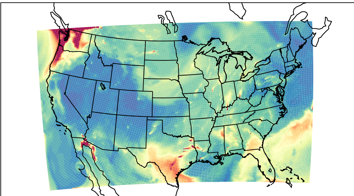
WRF 2023-08-20_14:00:00
