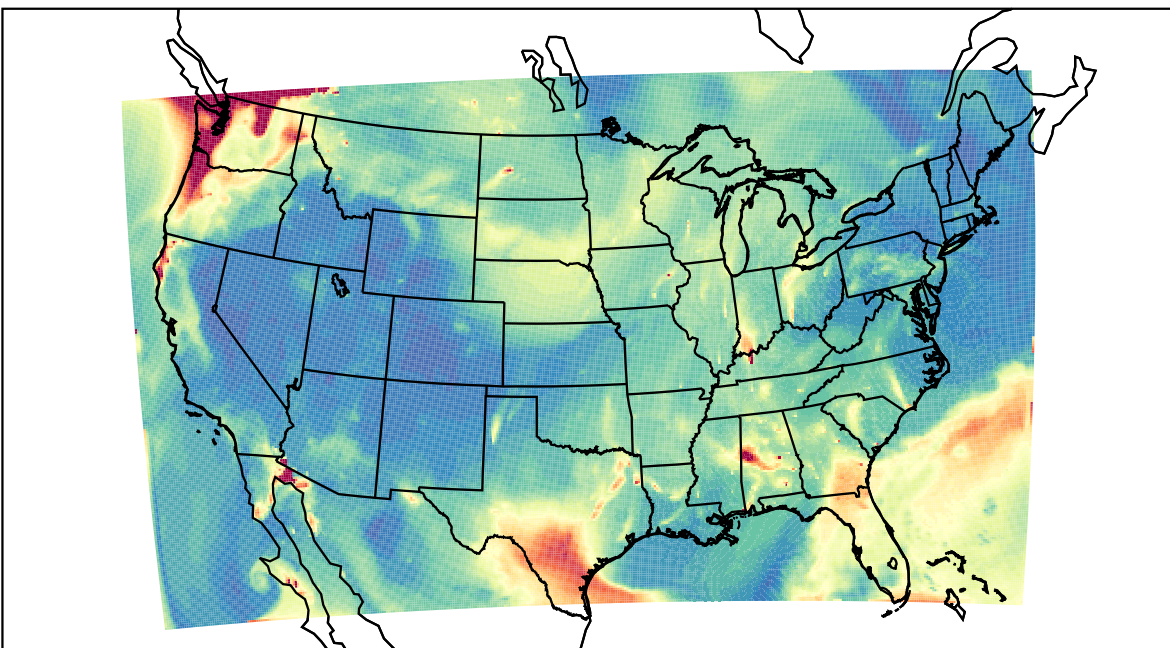
WRF 2023-08-20_10:00:00
