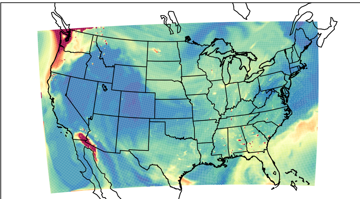
WRF 2023-08-20_20:00:00
