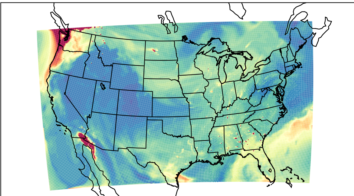
WRF 2023-08-20_19:00:00
