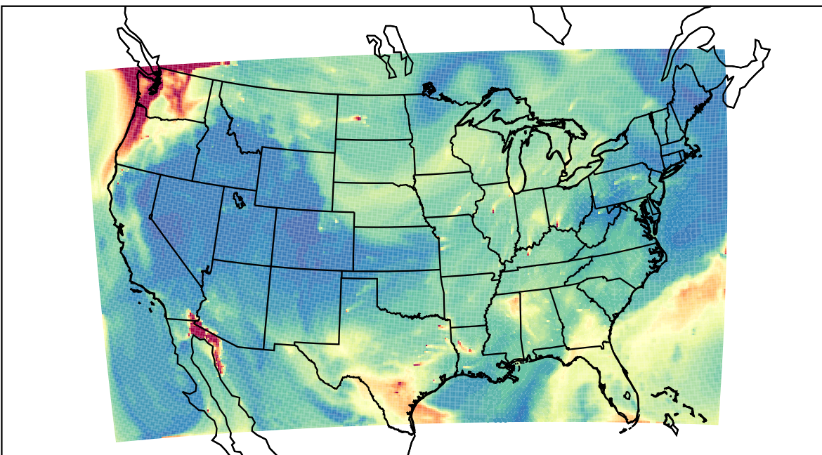
WRF 2023-08-20_16:00:00
