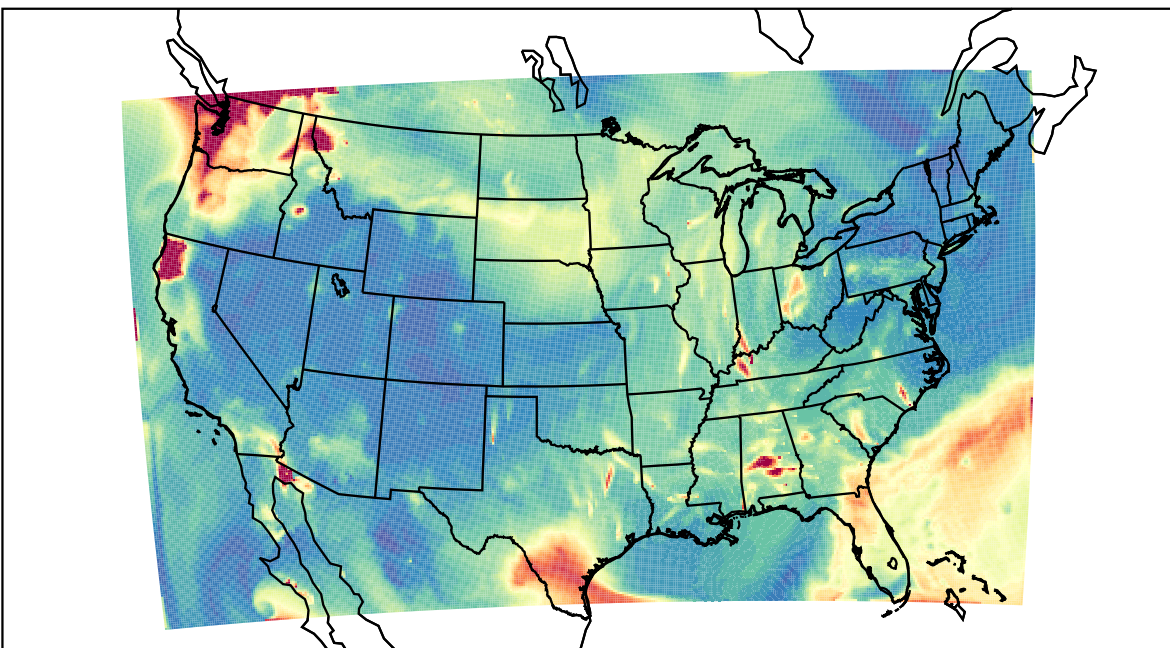
WRF 2023-08-20_06:00:00
