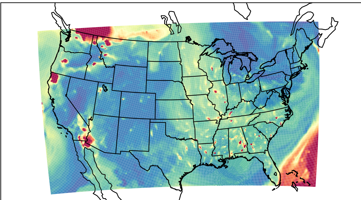
WRF 2023-08-19_03:00:00
