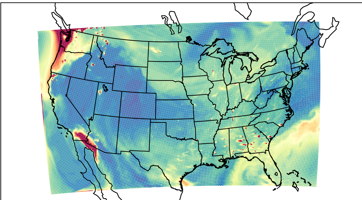
WRF 2023-08-20_22:00:00
