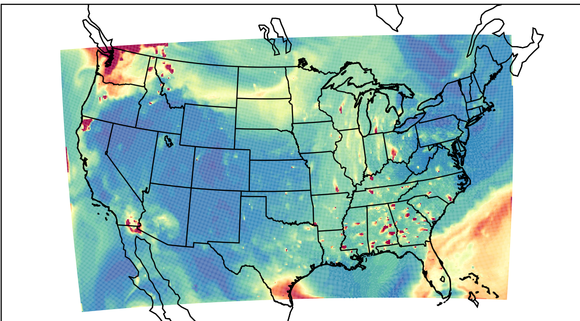
WRF 2023-08-20_01:00:00
