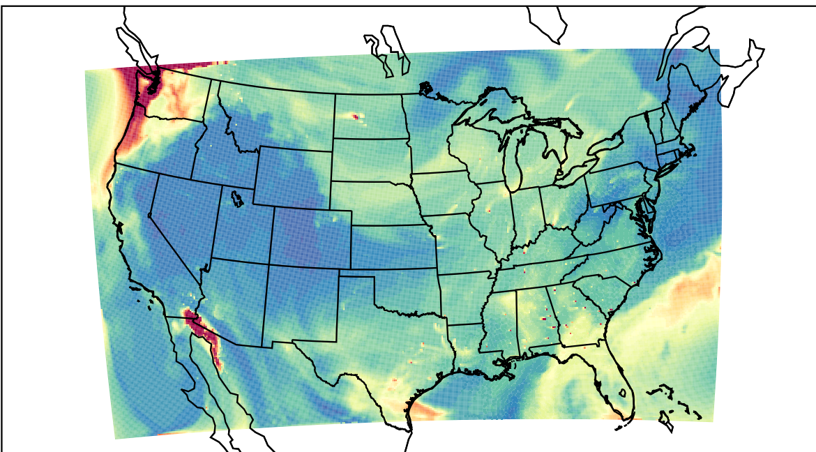
WRF 2023-08-20_18:00:00
