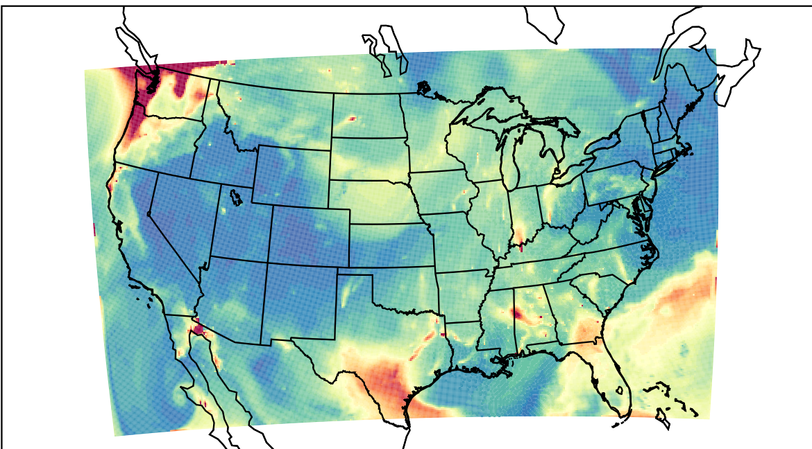
WRF 2023-08-20_11:00:00
