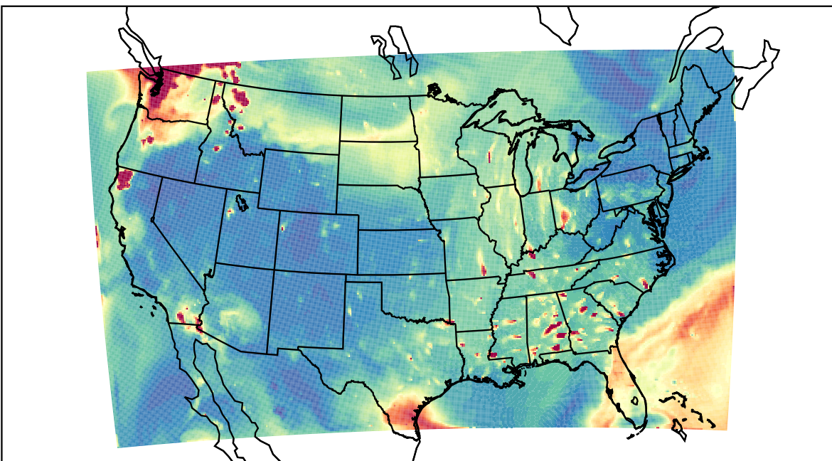
WRF 2023-08-20_02:00:00
