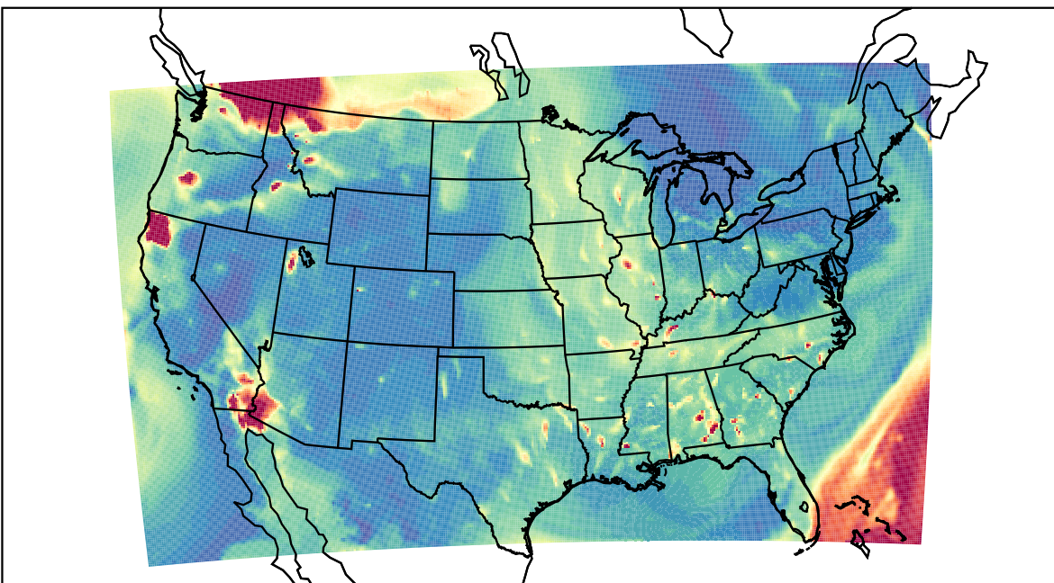
WRF 2023-08-19_04:00:00
