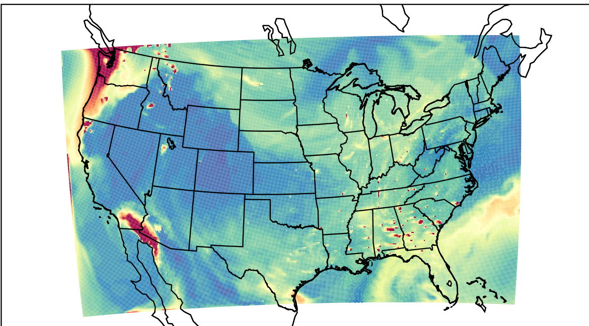
WRF 2023-08-20_23:00:00
