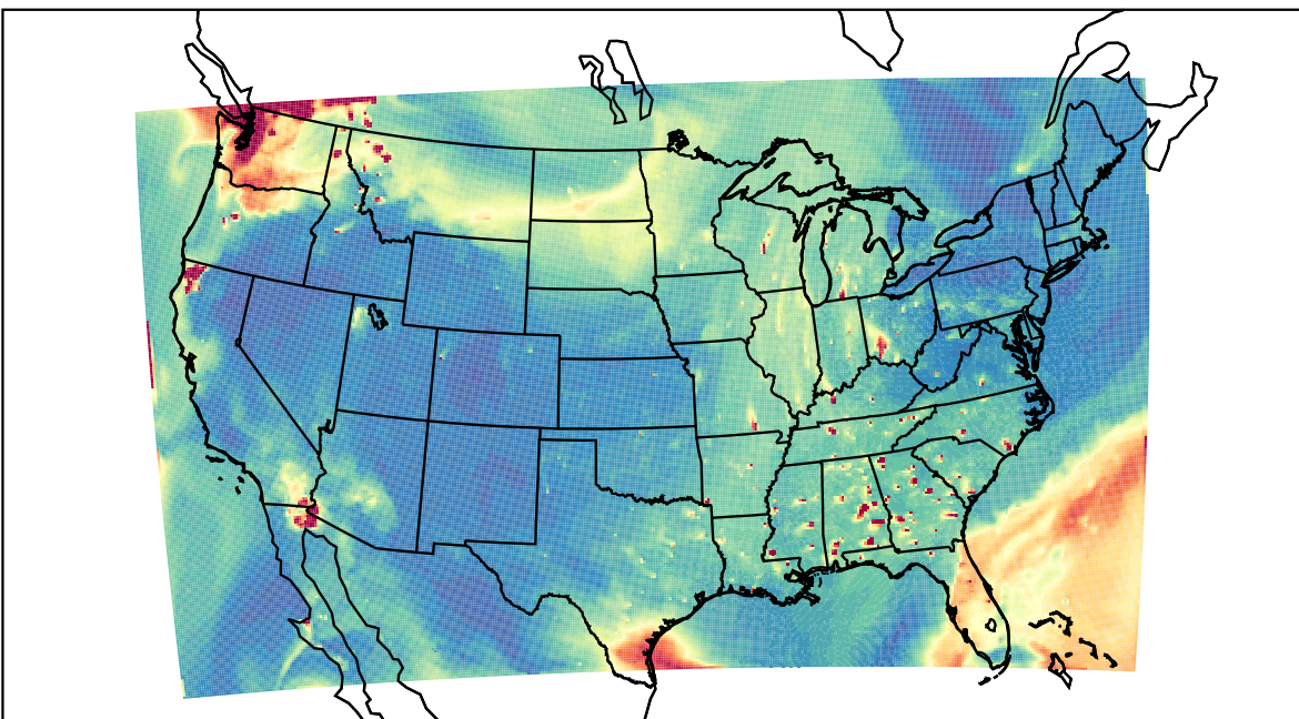
WRF 2023-08-20_00:00:00
