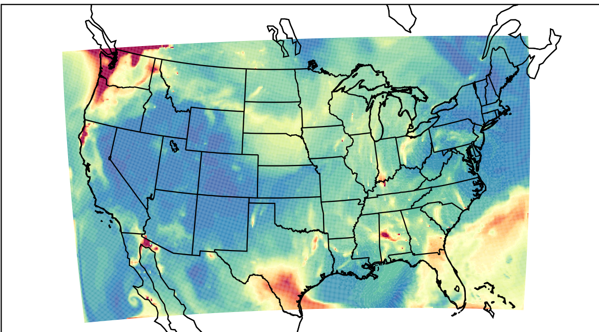
WRF 2023-08-20_09:00:00
