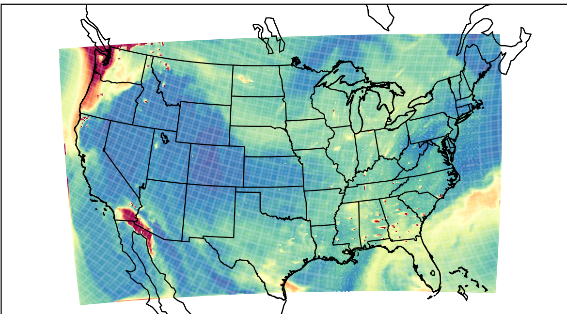
WRF 2023-08-20_21:00:00
