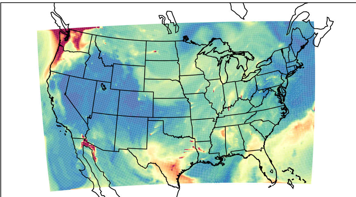
WRF 2023-08-20_15:00:00
