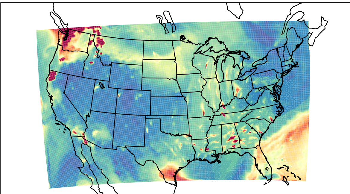
WRF 2023-08-20_03:00:00
