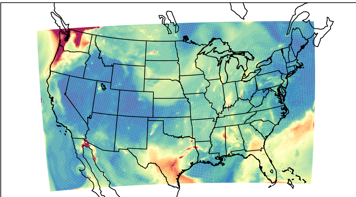
WRF 2023-08-20_13:00:00
