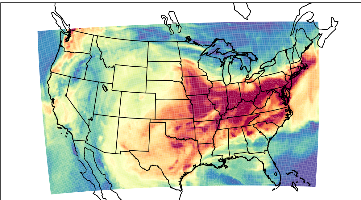
WRF (2023-08-21_19:00:00)
