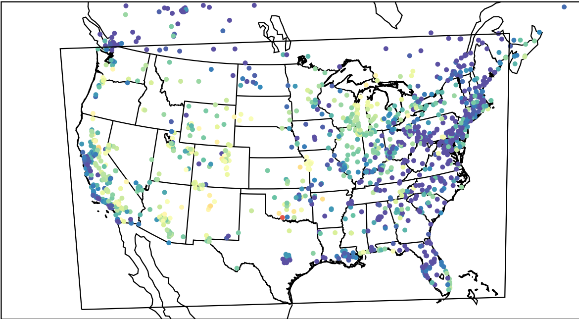
AirNOW (2023-08-20_04:00:00)
