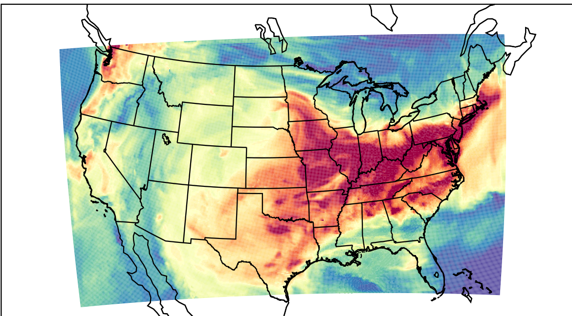
WRF (2023-08-21_20:00:00)
