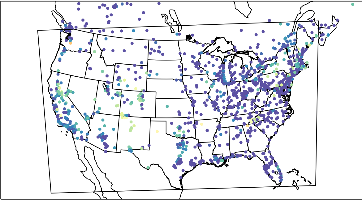
AirNOW (2023-08-21_11:00:00)
