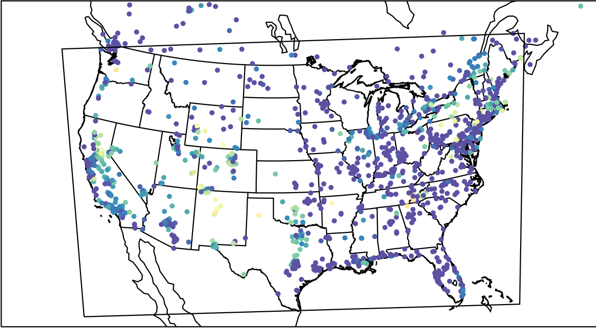
AirNOW (2023-08-21_10:00:00)
