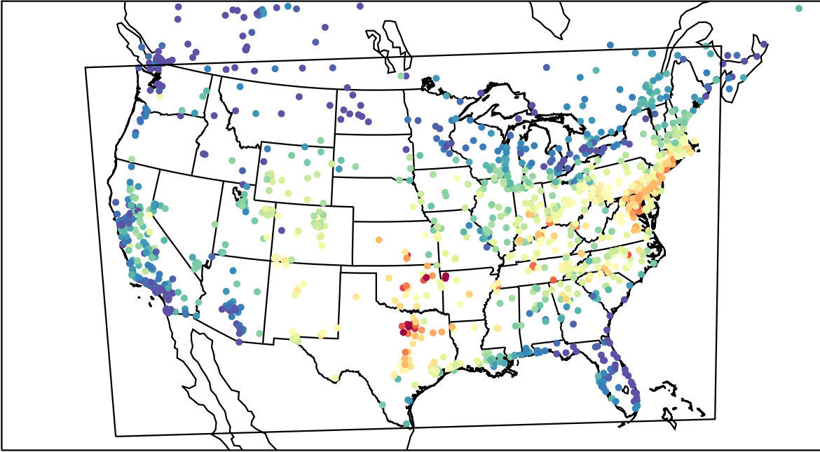
AirNOW (2023-08-21_16:00:00)
