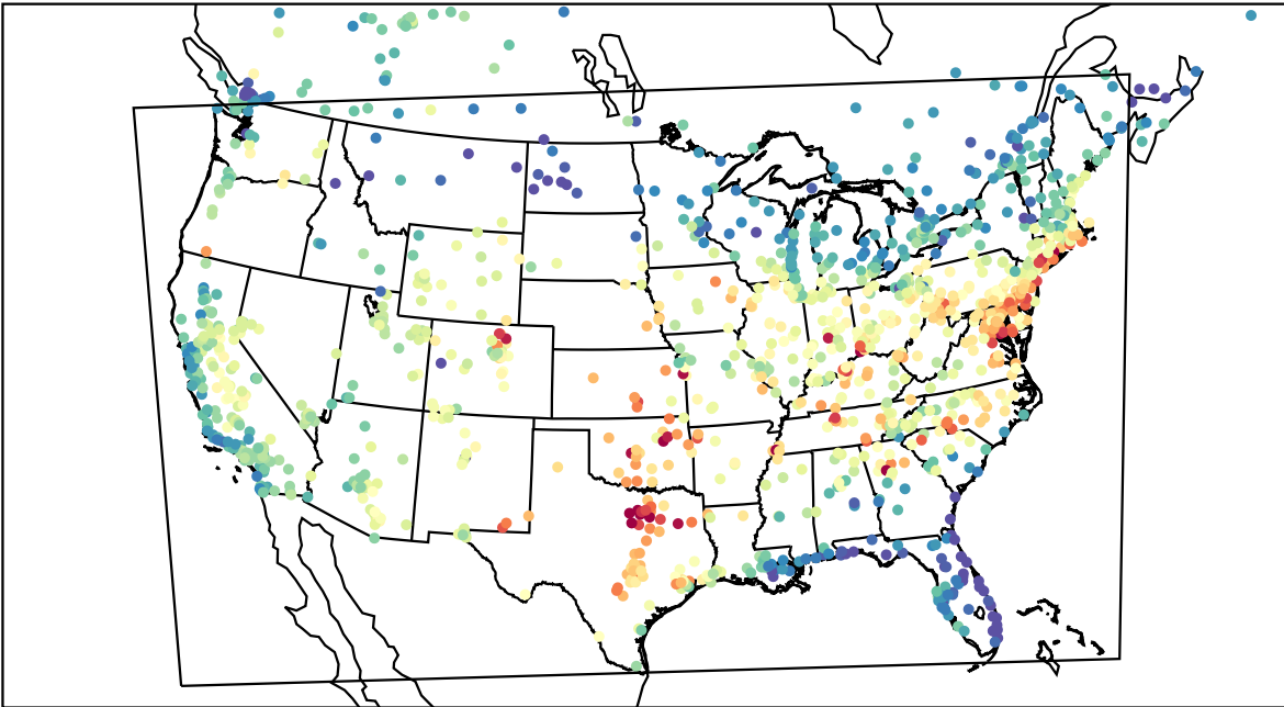
AirNOW (2023-08-21_20:00:00)
