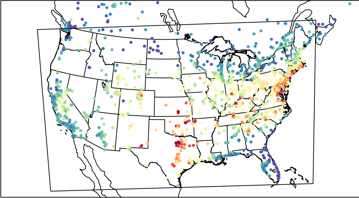
AirNOW (2023-08-21_18:00:00)
