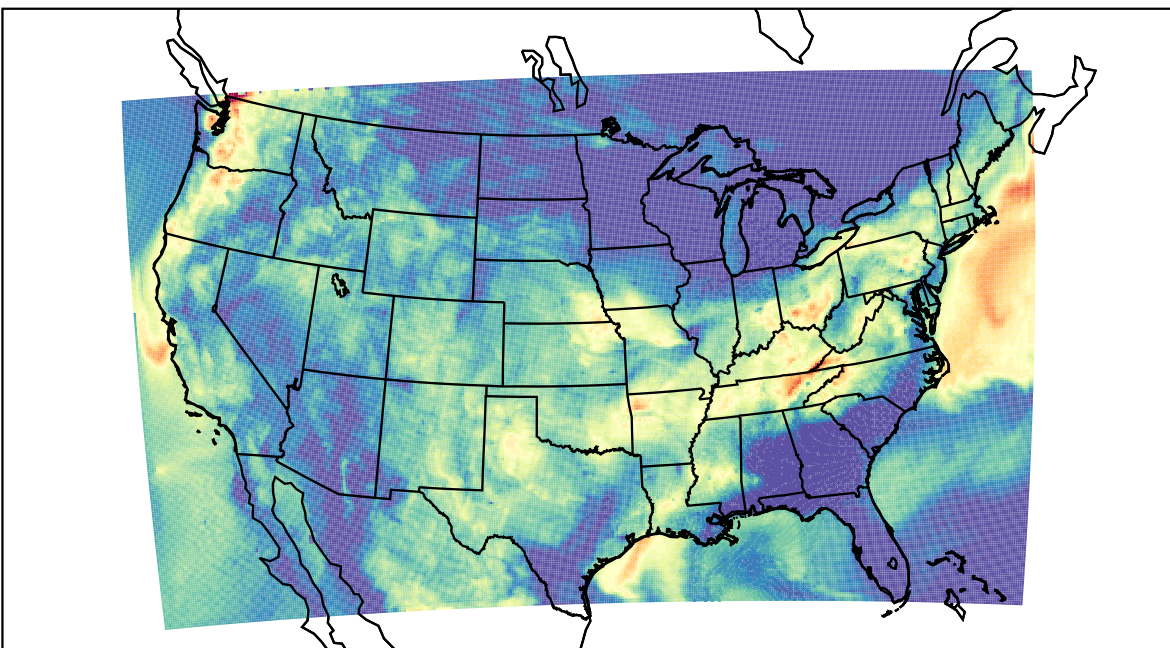
WRF (2023-08-21_11:00:00)
