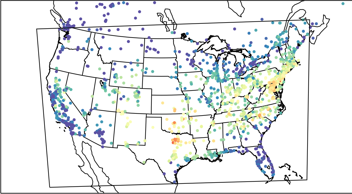
AirNOW (2023-08-21_15:00:00)
