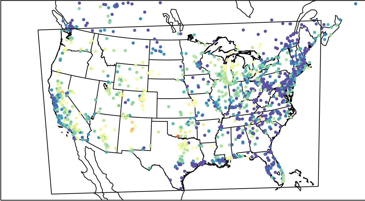
AirNOW (2023-08-20_03:00:00)
