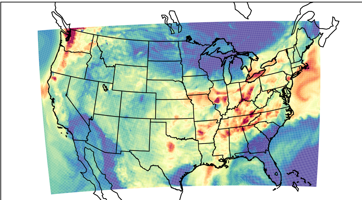
WRF (2023-08-21_03:00:00)
