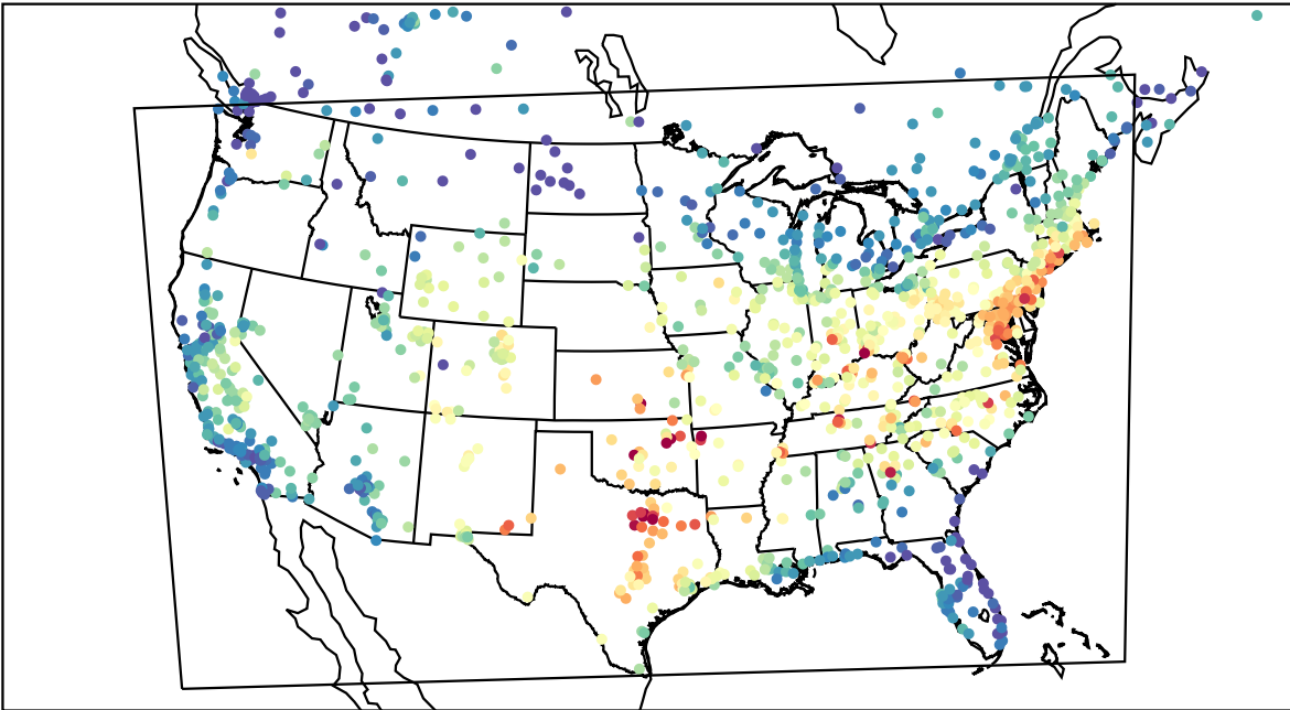
AirNOW (2023-08-21_17:00:00)
