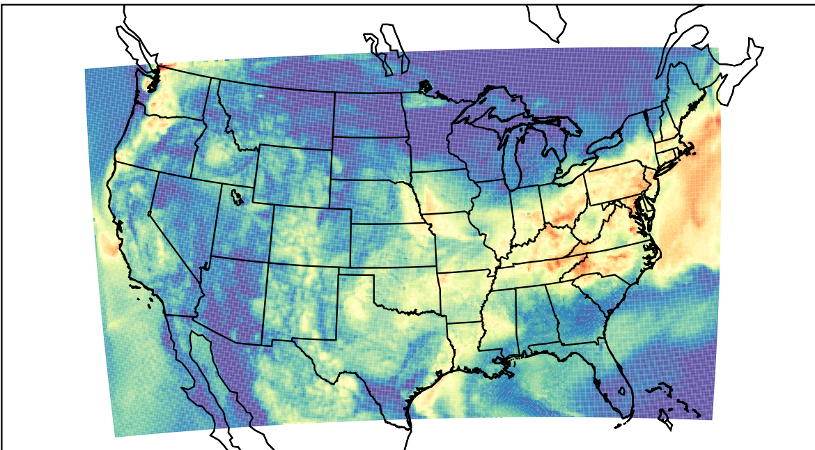
WRF (2023-08-21_14:00:00)
