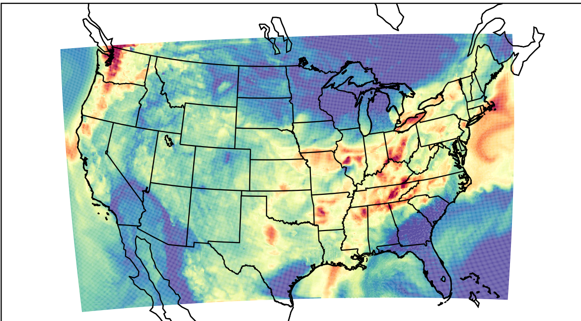
WRF (2023-08-21_04:00:00)
