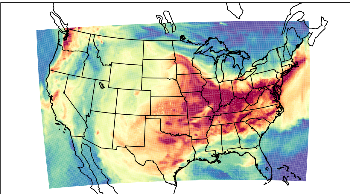
WRF (2023-08-21_22:00:00)
