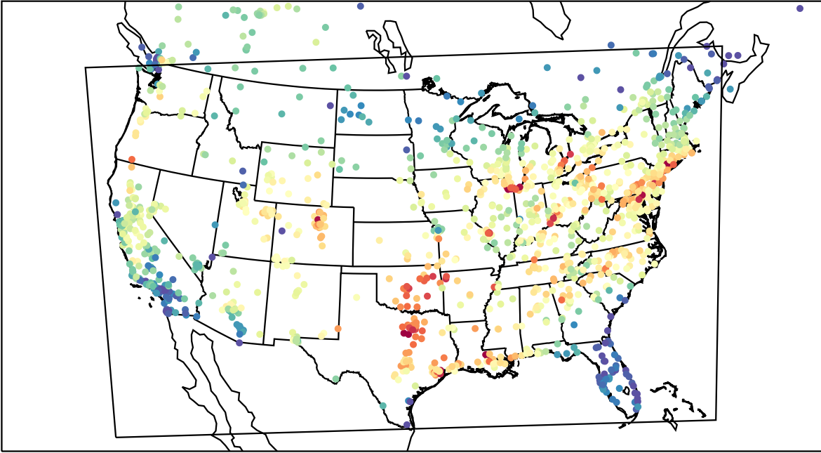
AirNOW (2023-08-20_20:00:00)
