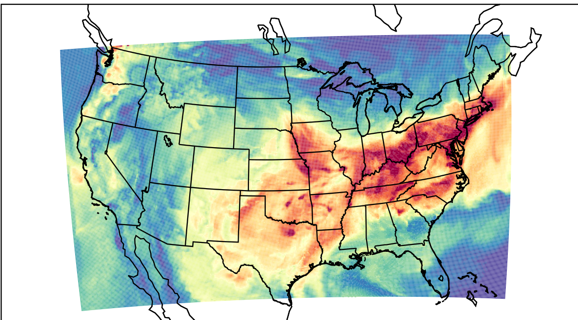
WRF (2023-08-21_16:00:00)
