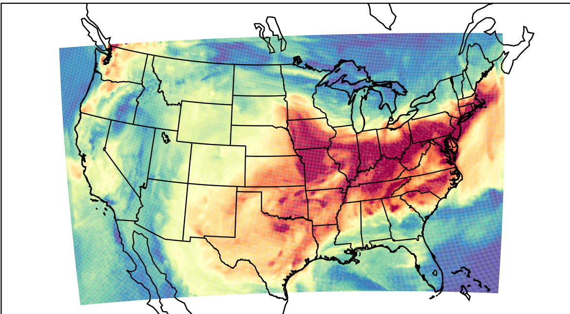
WRF (2023-08-21_18:00:00)
