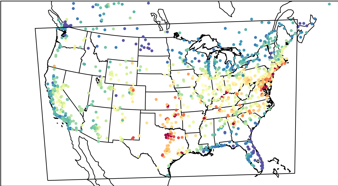
AirNOW (2023-08-21_19:00:00)
