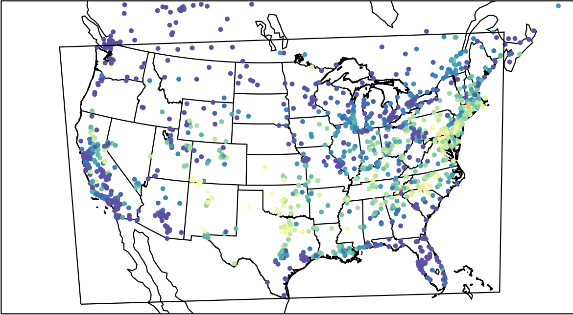
AirNOW (2023-08-21_14:00:00)
