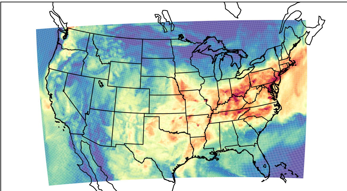
WRF (2023-08-21_15:00:00)
