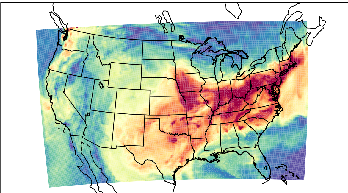
WRF (2023-08-21_17:00:00)
