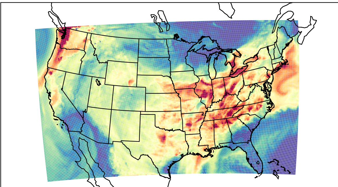
WRF (2023-08-21_01:00:00)
