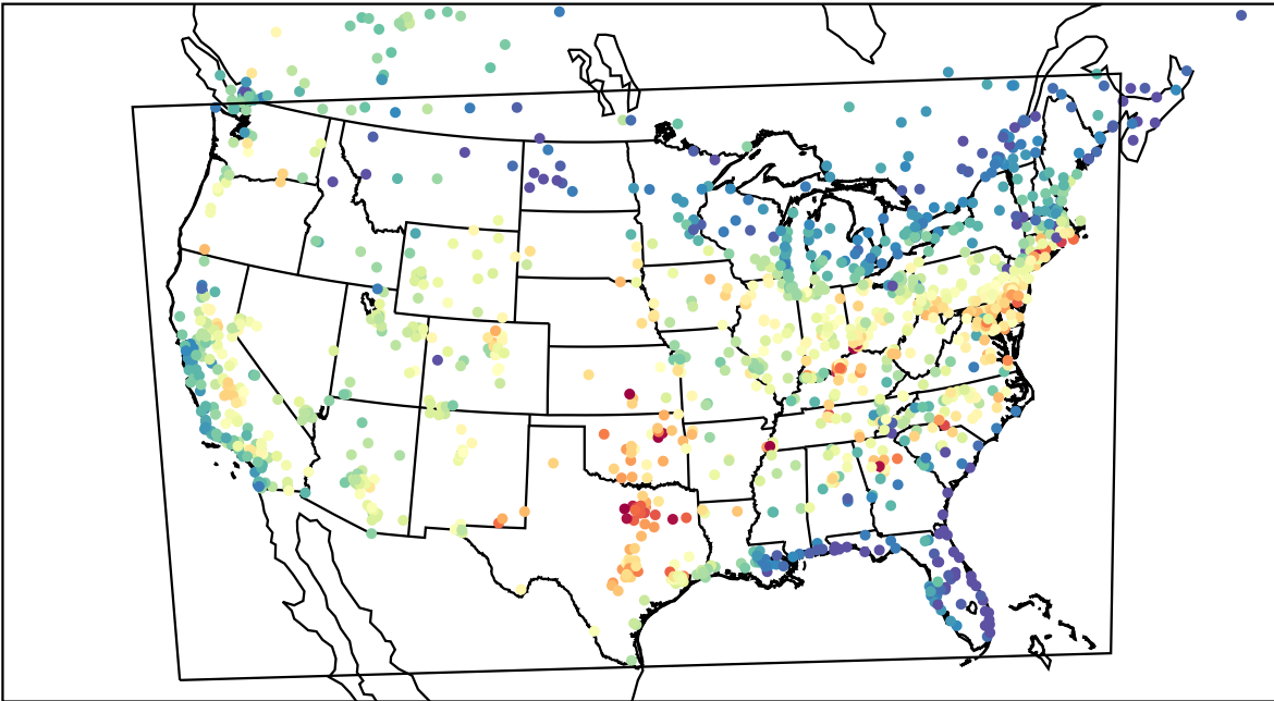
AirNOW (2023-08-21_22:00:00)
