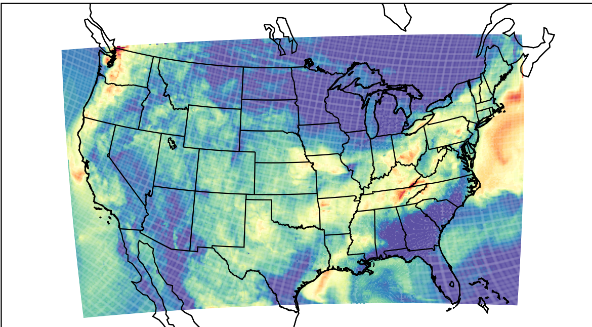
WRF (2023-08-21_10:00:00)
