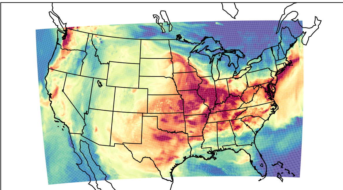
WRF (2023-08-21_23:00:00)
