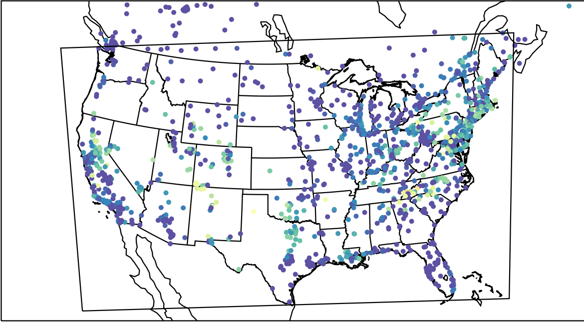
AirNOW (2023-08-21_13:00:00)
