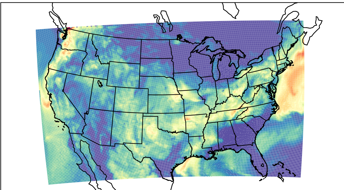
WRF (2023-08-21_12:00:00)
