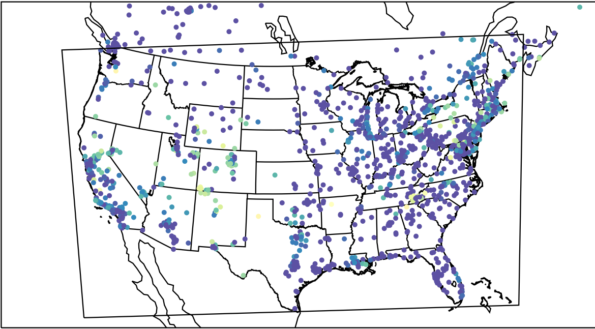
AirNOW (2023-08-21_12:00:00)
