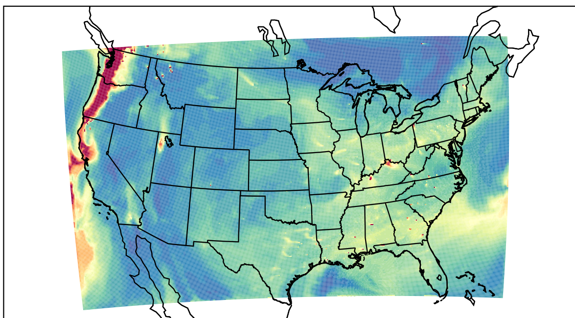
WRF 2023-08-21_20:00:00
