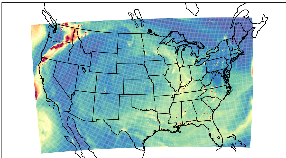
WRF 2023-08-22_23:00:00
