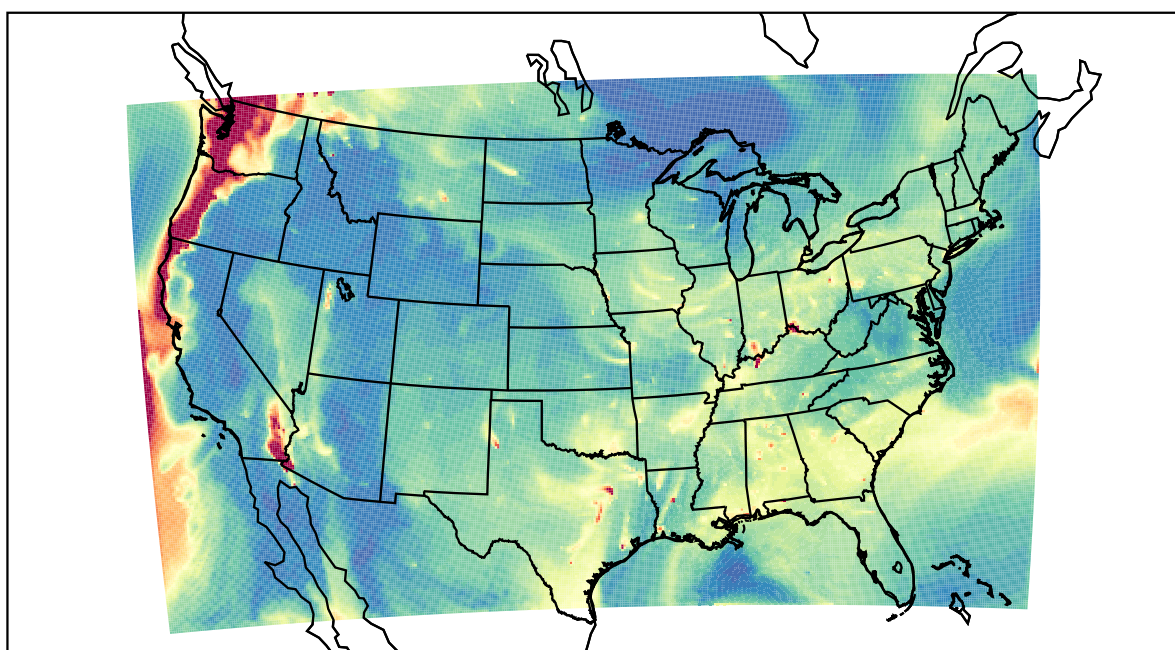
WRF 2023-08-21_13:00:00
