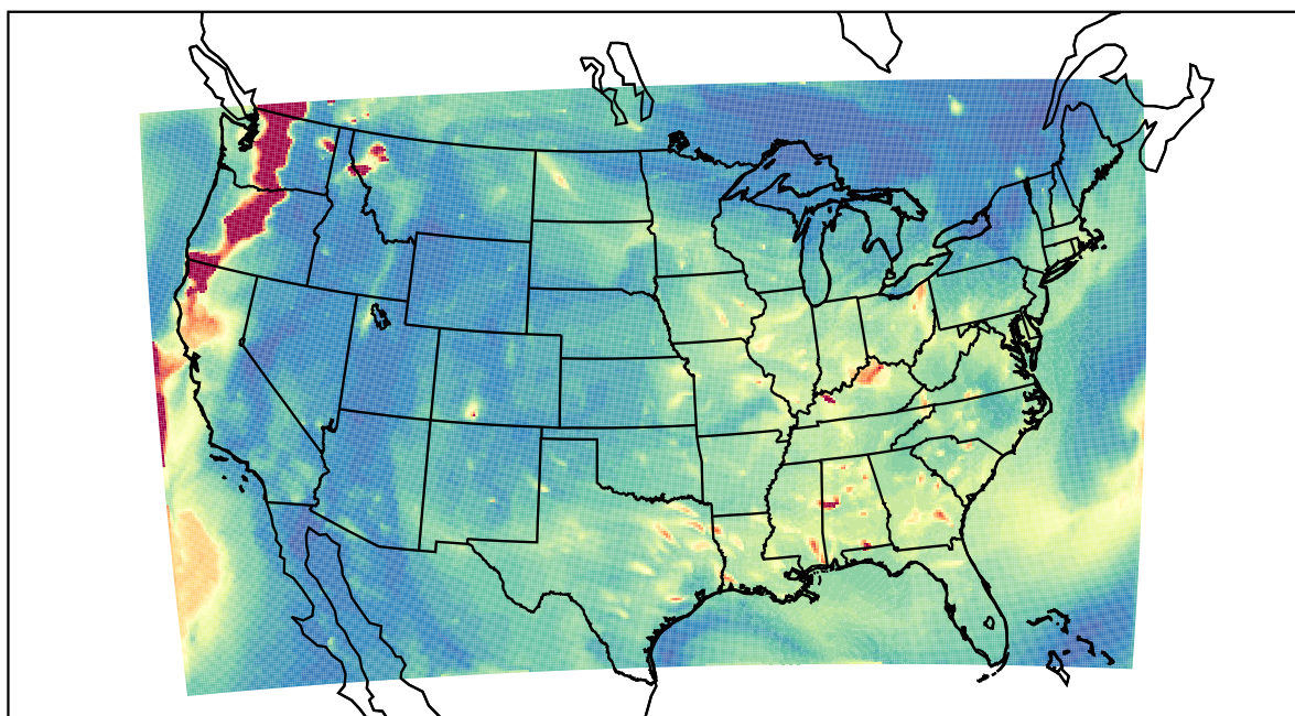
WRF 2023-08-22_04:00:00
