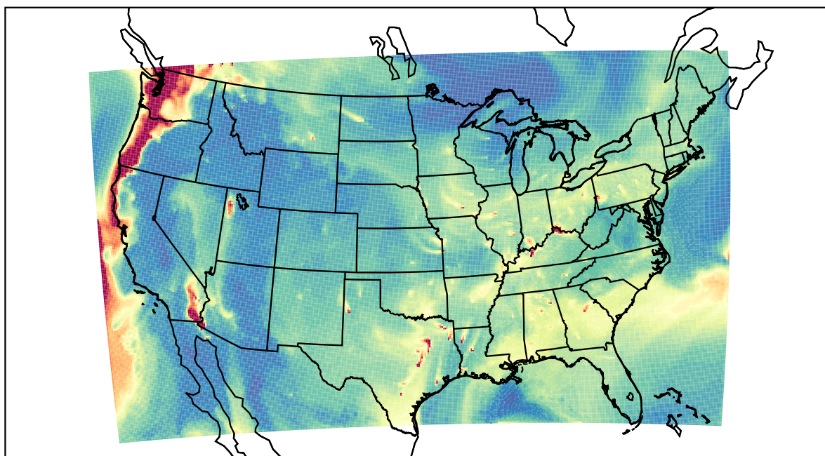
WRF 2023-08-21_14:00:00
