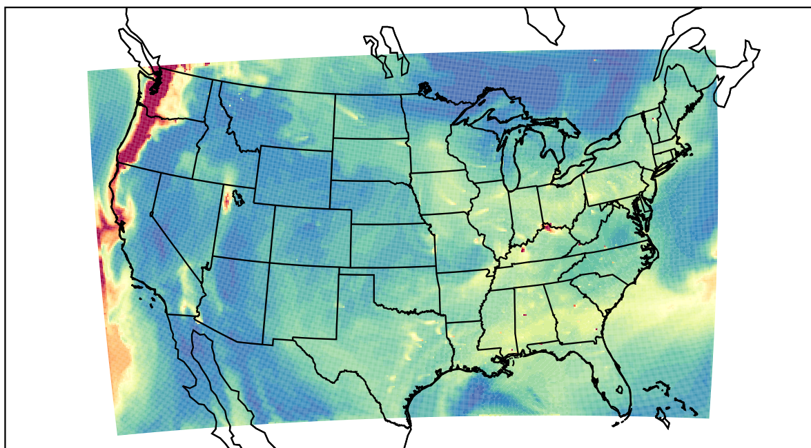
WRF 2023-08-21_18:00:00
