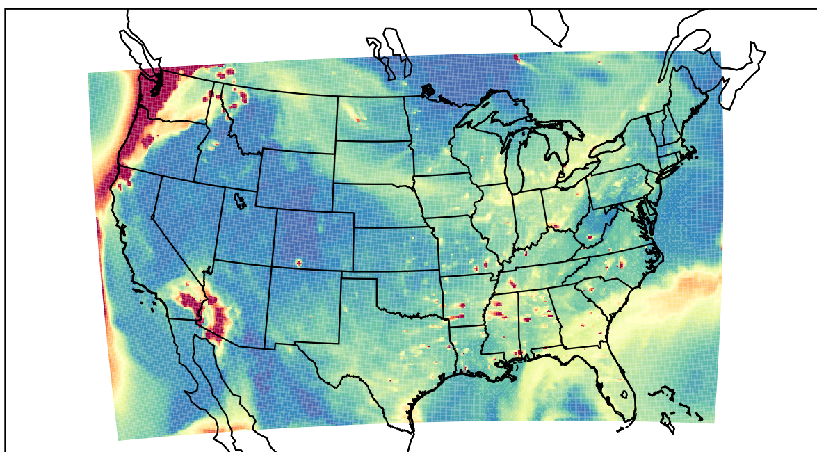
WRF 2023-08-21_01:00:00
