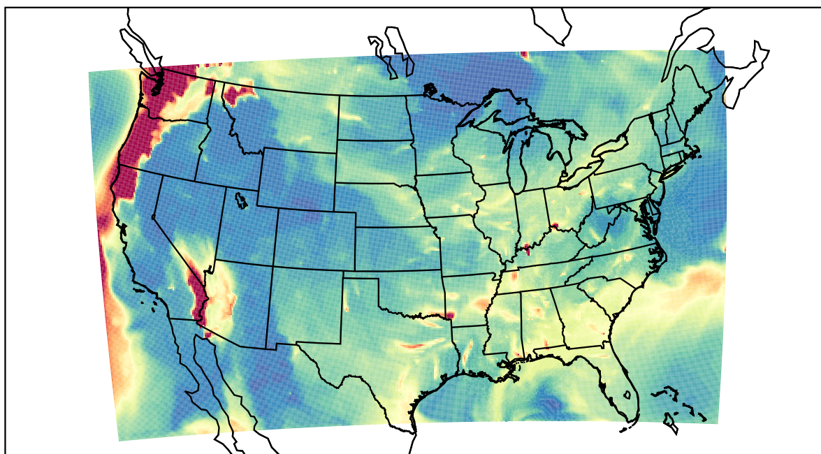
WRF 2023-08-21_07:00:00
