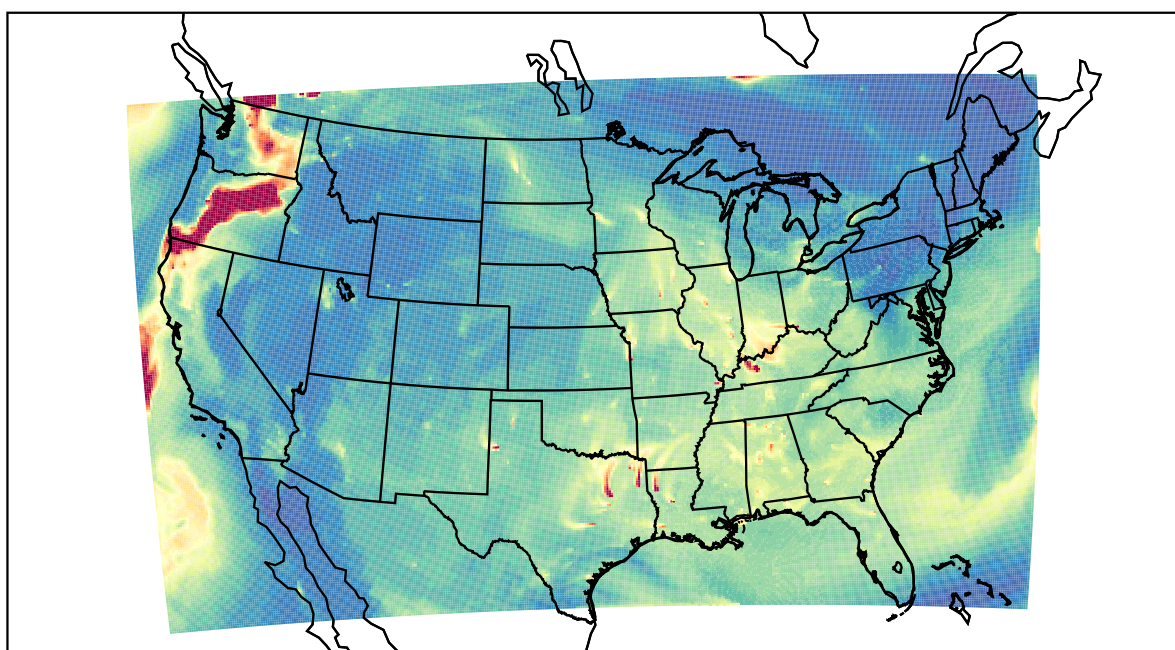
WRF 2023-08-22_14:00:00
