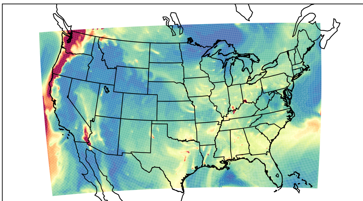
WRF 2023-08-21_12:00:00
