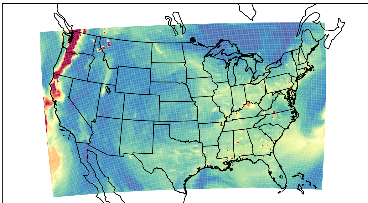
WRF 2023-08-21_23:00:00
