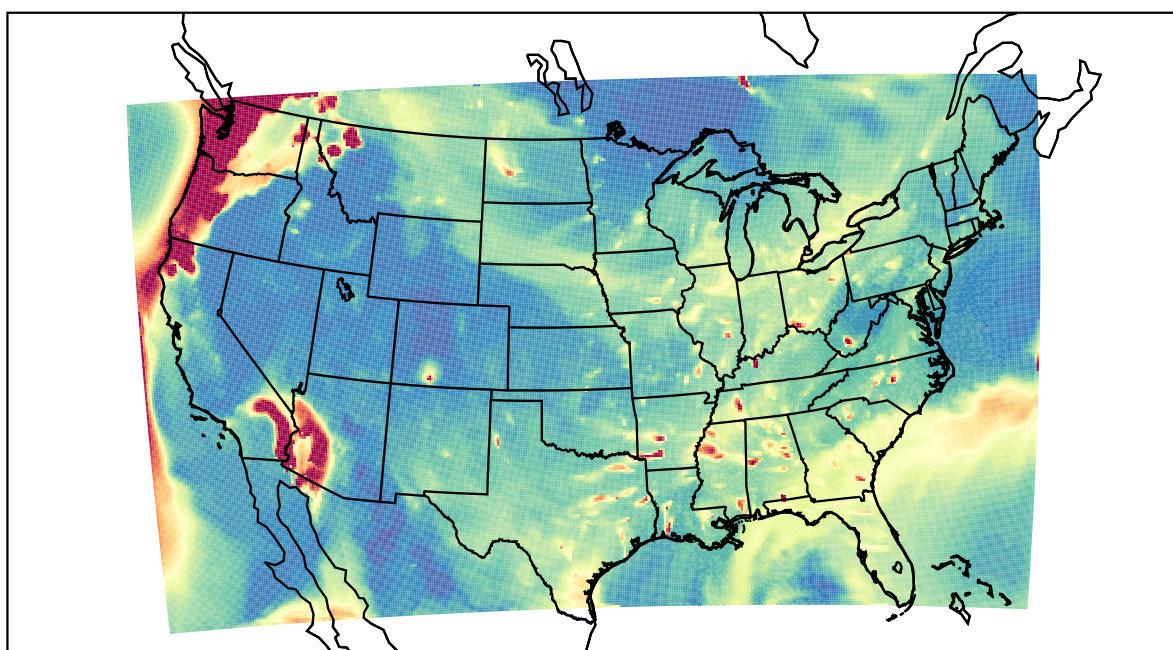
WRF 2023-08-21_03:00:00
