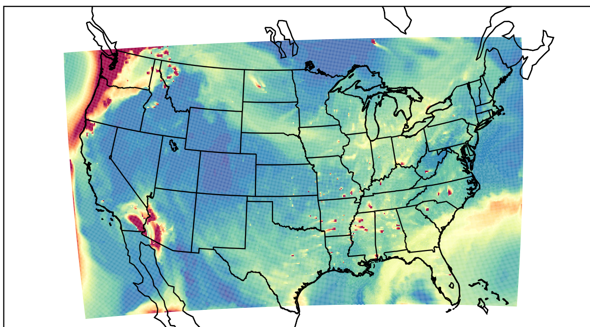
WRF 2023-08-21_00:00:00
