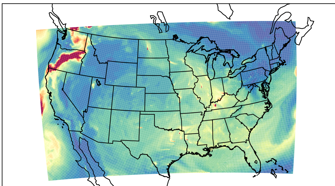
WRF 2023-08-22_16:00:00
