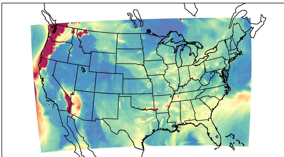
WRF 2023-08-21_06:00:00
