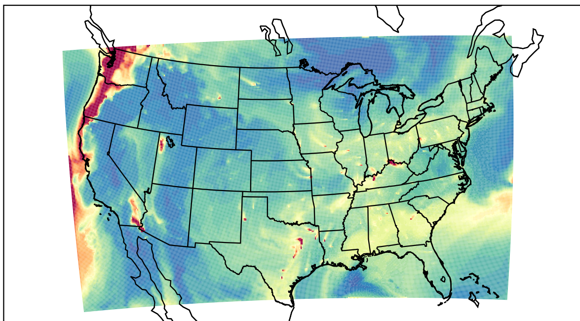
WRF 2023-08-21_15:00:00
