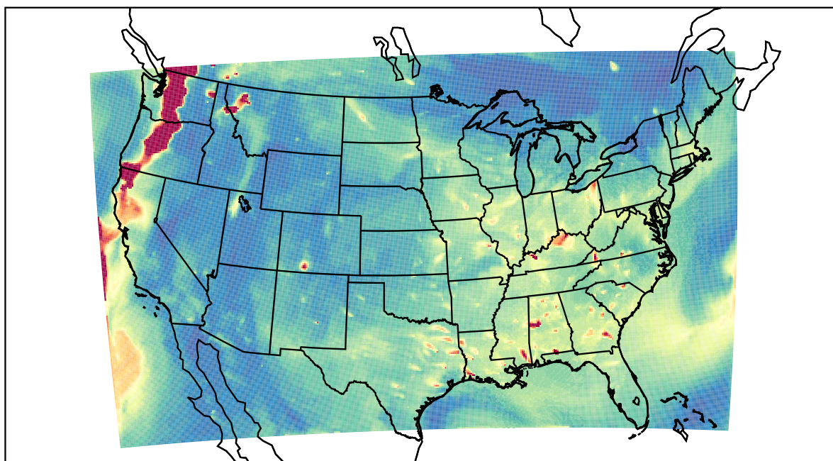
WRF 2023-08-22_03:00:00
