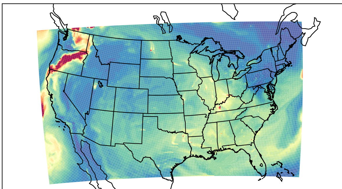
WRF 2023-08-22_17:00:00
