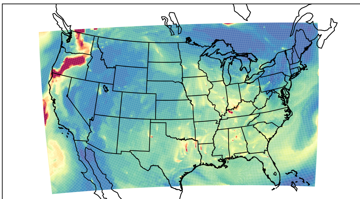
WRF 2023-08-22_13:00:00
