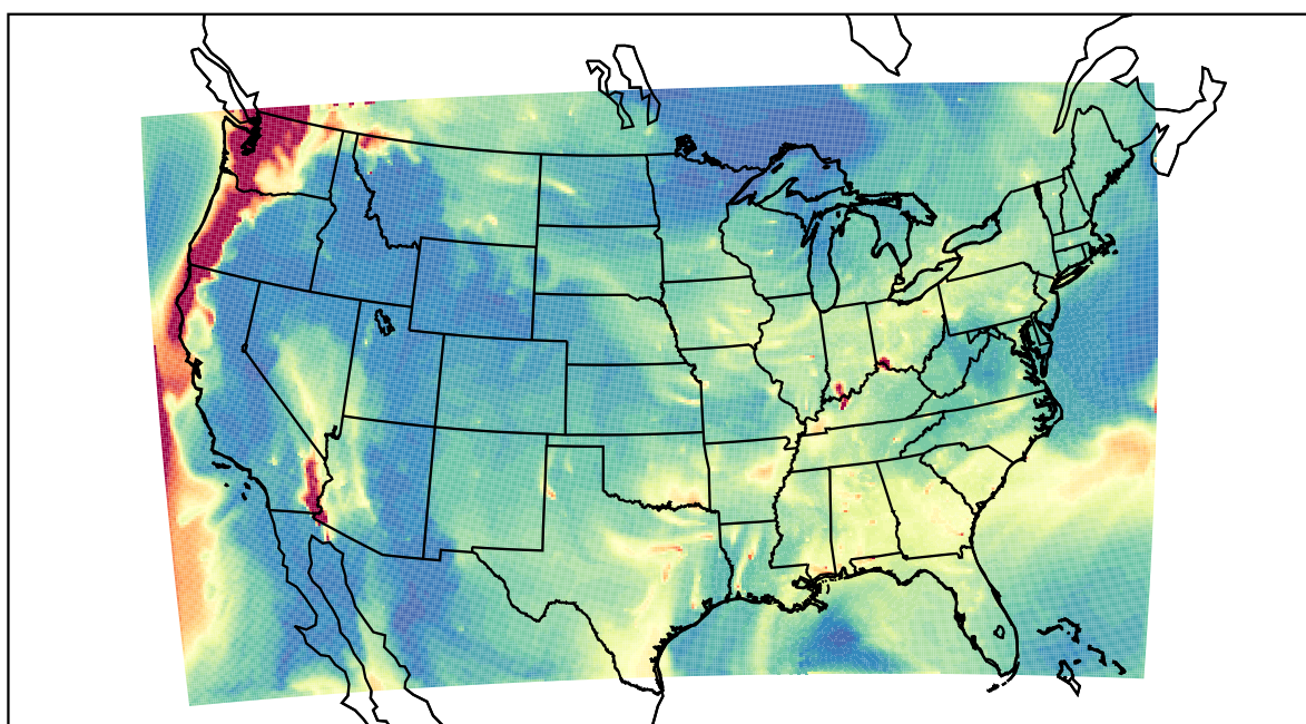
WRF 2023-08-21_11:00:00
