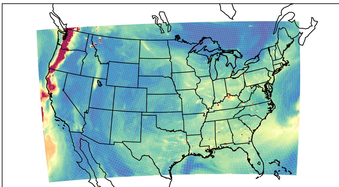
WRF 2023-08-21_22:00:00
