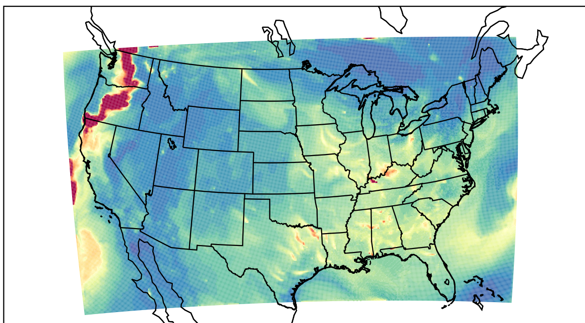
WRF 2023-08-22_08:00:00
