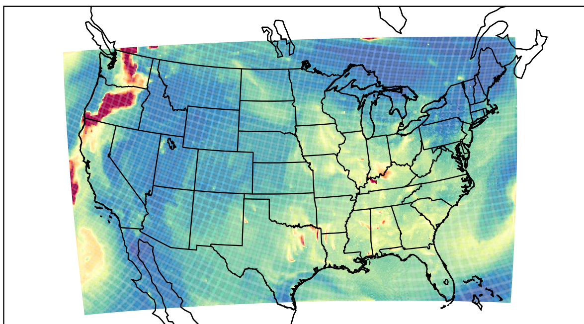
WRF 2023-08-22_11:00:00
