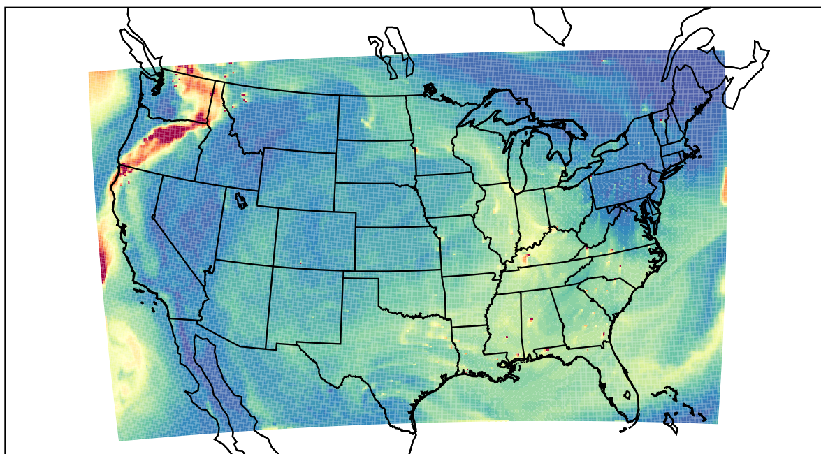
WRF 2023-08-22_20:00:00
