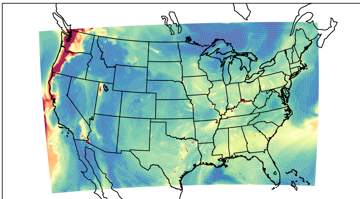
WRF 2023-08-21_16:00:00
