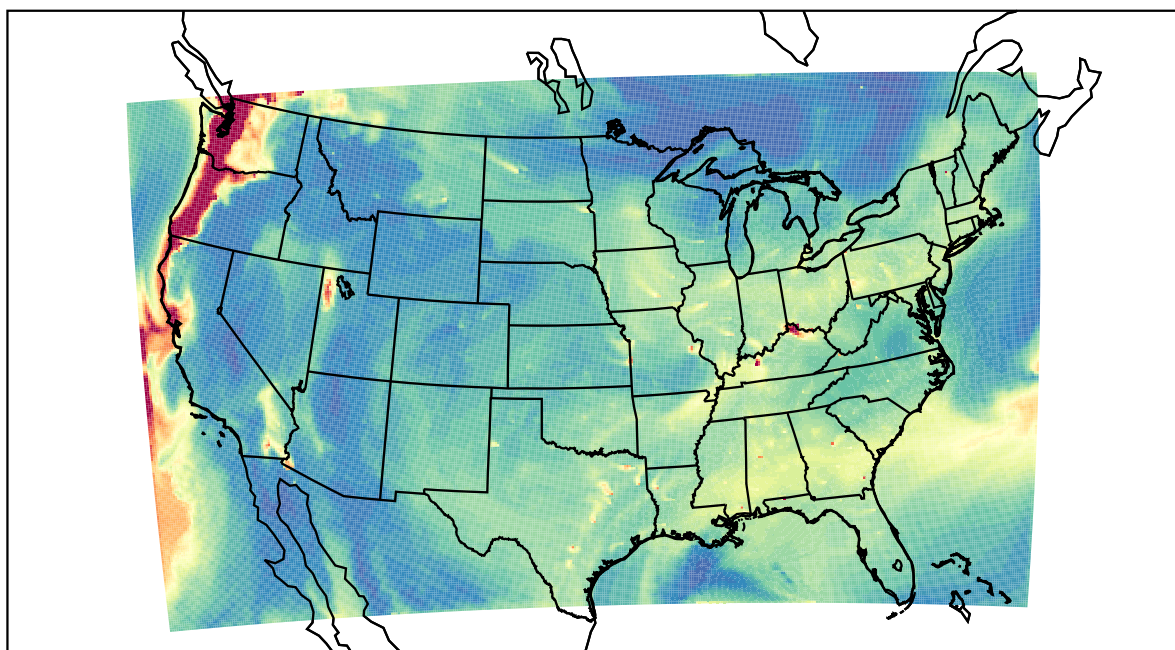
WRF 2023-08-21_17:00:00
