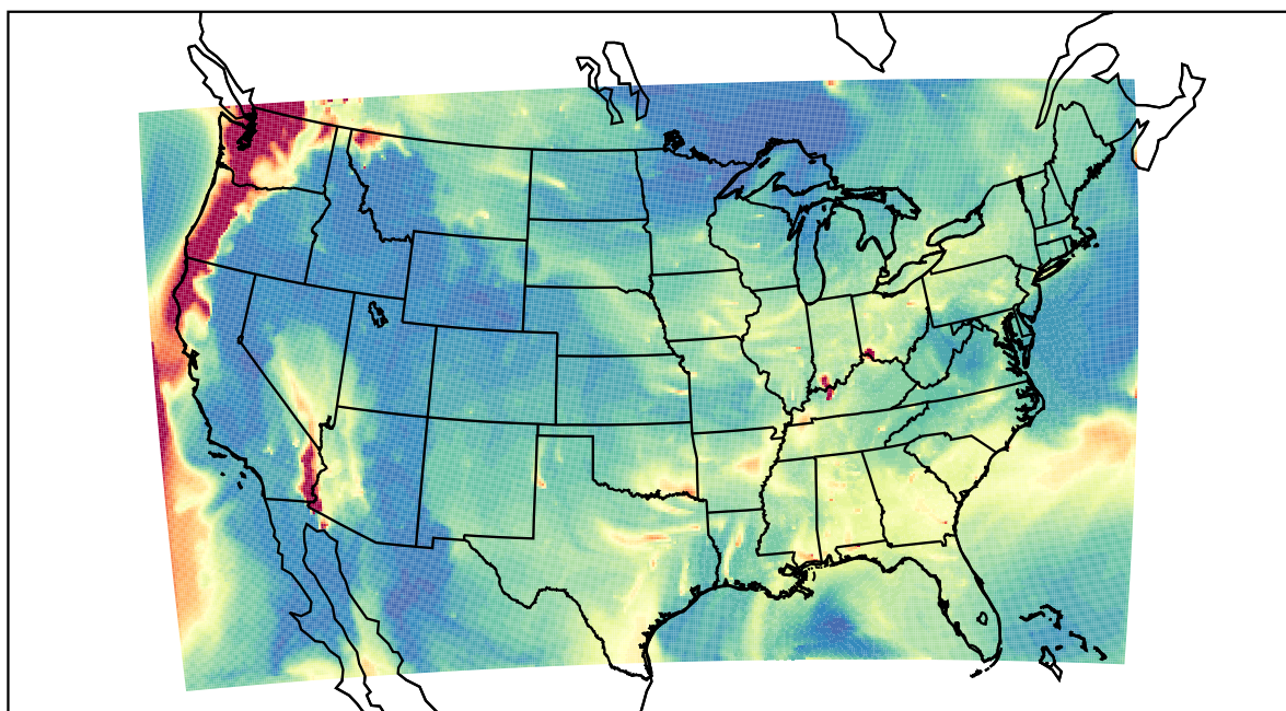
WRF 2023-08-21_10:00:00
