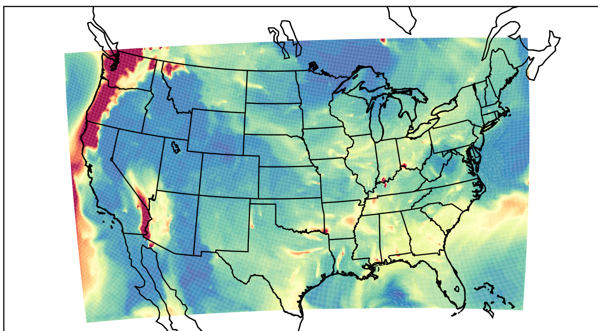
WRF 2023-08-21_08:00:00
