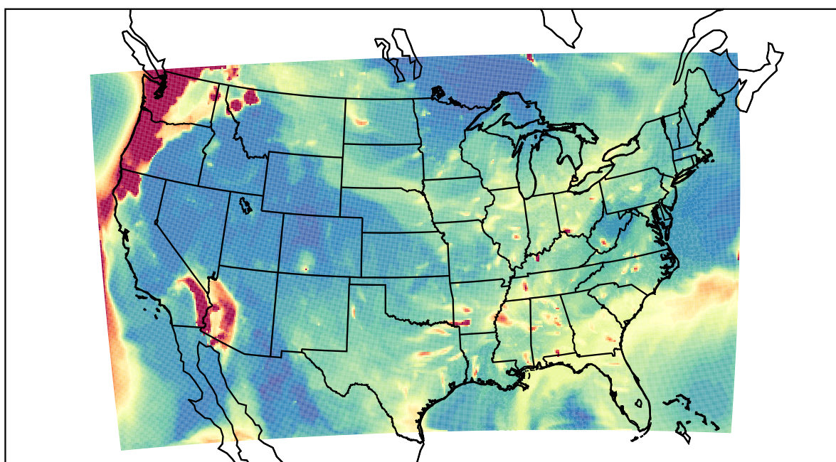
WRF 2023-08-21_04:00:00
