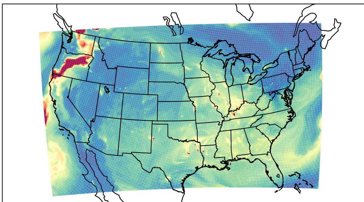
WRF 2023-08-22_15:00:00
