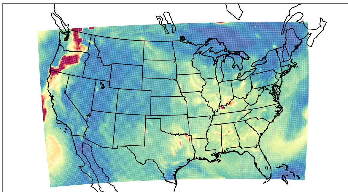
WRF 2023-08-22_10:00:00
