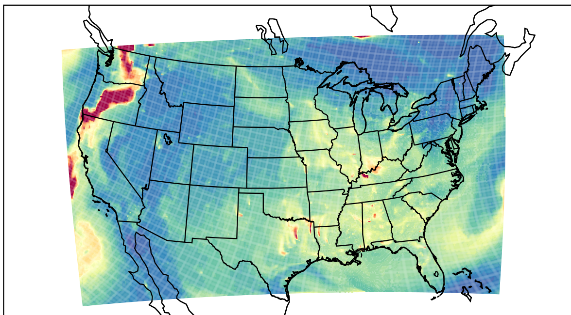
WRF 2023-08-22_12:00:00
