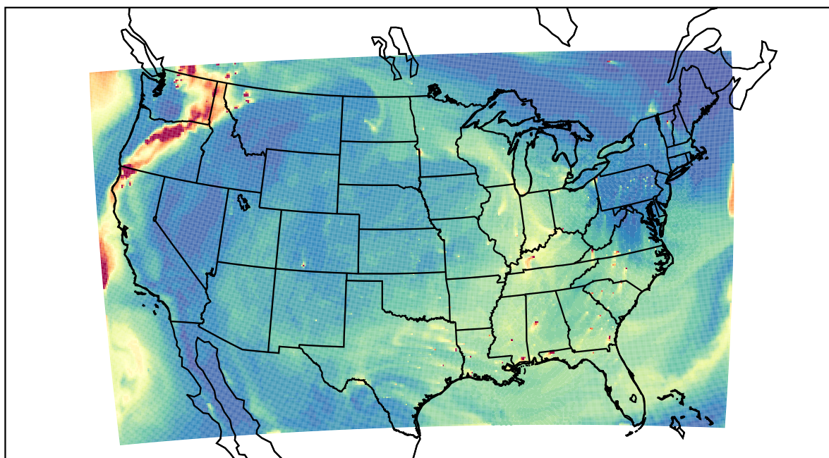
WRF 2023-08-22_22:00:00
