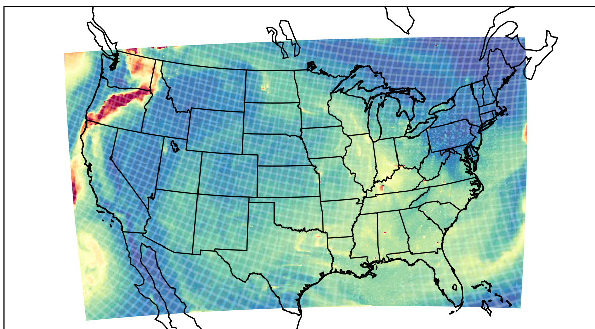
WRF 2023-08-22_18:00:00
