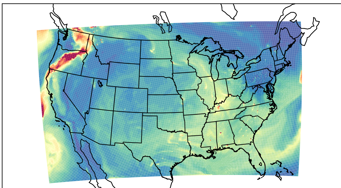
WRF 2023-08-22_19:00:00
