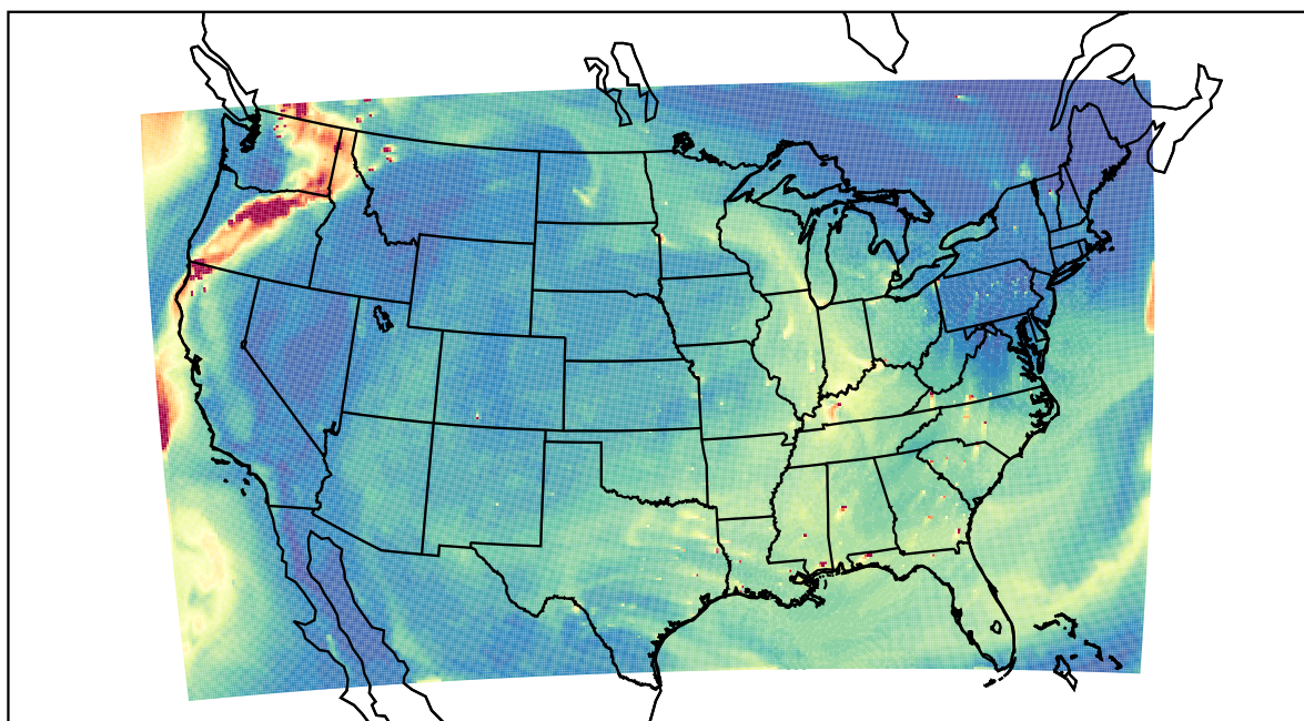
WRF 2023-08-22_21:00:00
