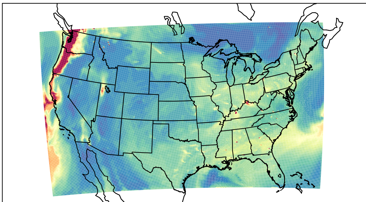
WRF 2023-08-21_19:00:00
