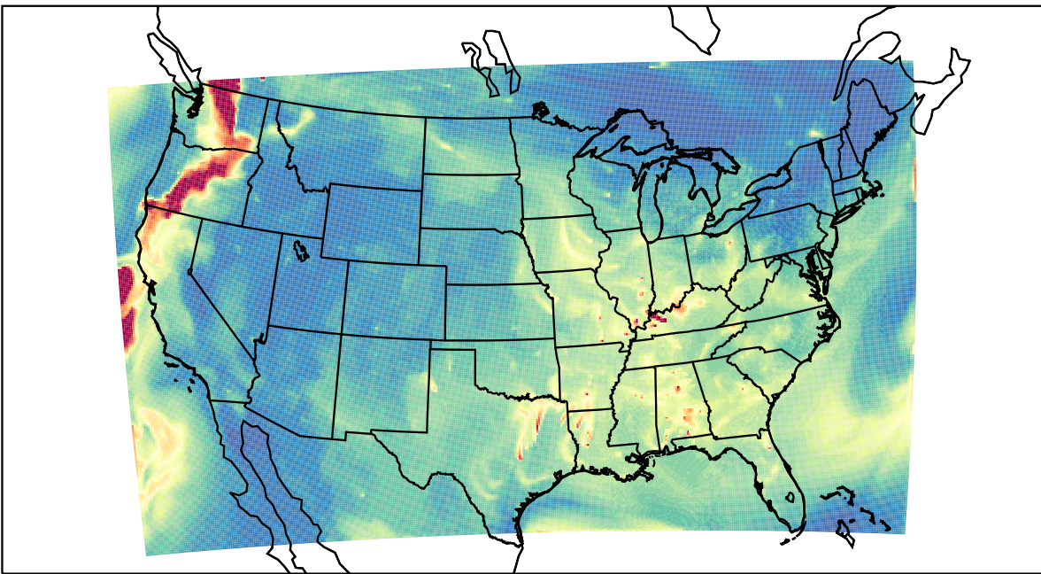
WRF 2023-08-22_11:00:00
