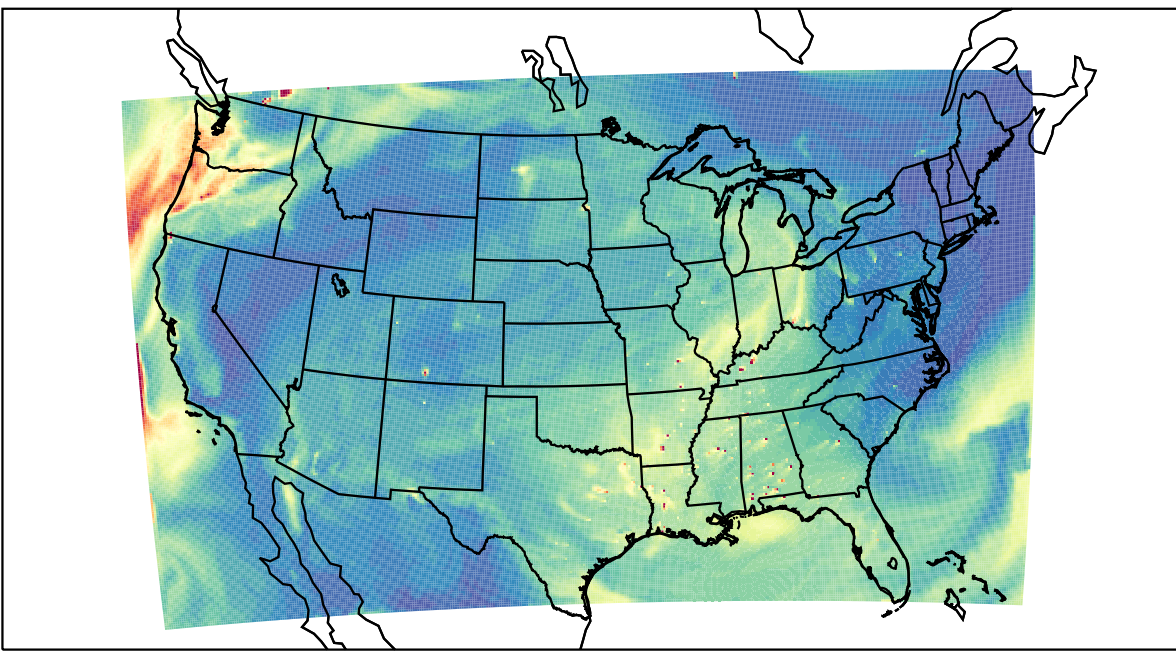
WRF 2023-08-23_20:00:00
