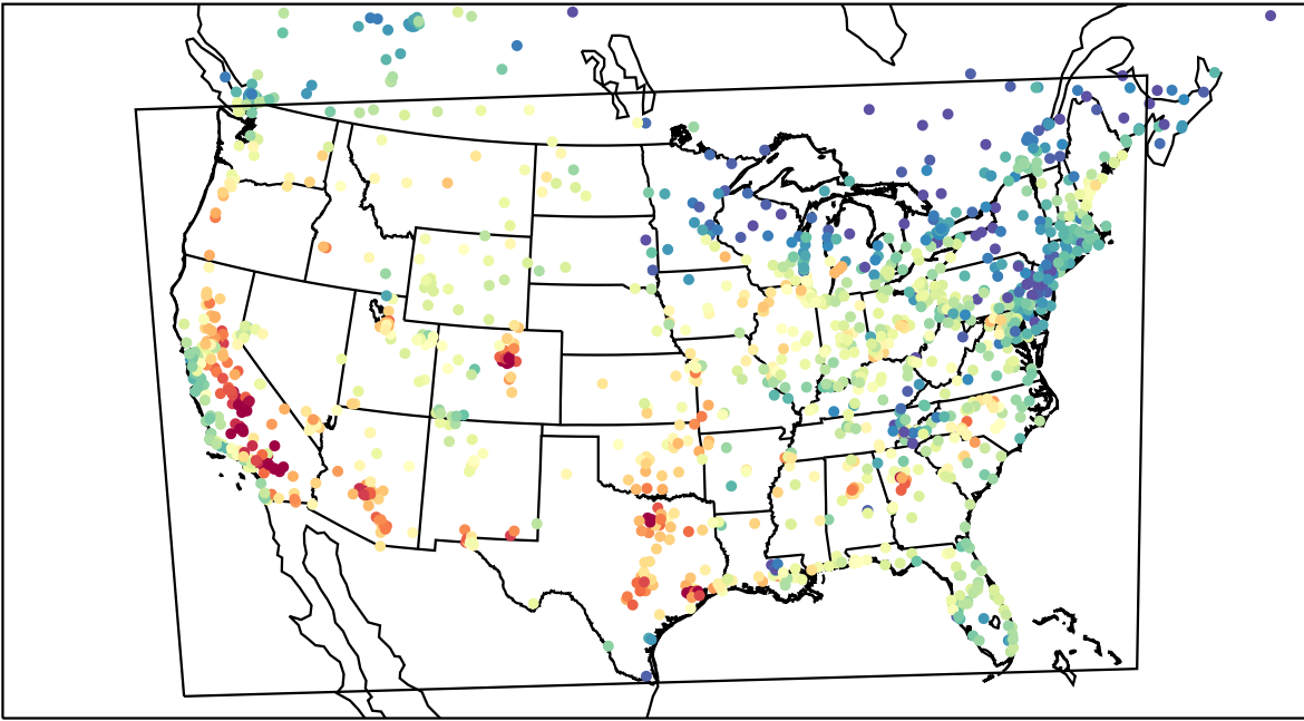
AirNOW (2023-08-24_23:00:00)
