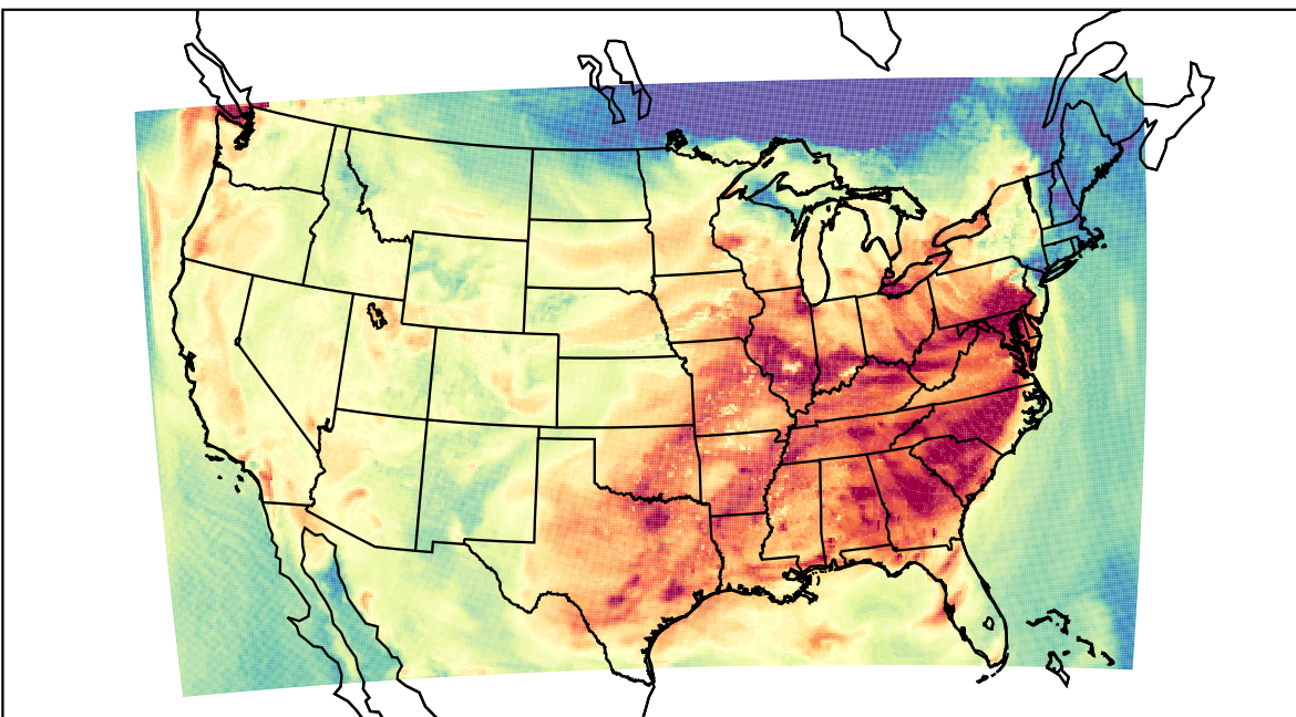
WRF (2023-08-25_20:00:00)
