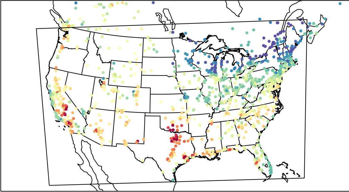
AirNOW (2023-08-26_20:00:00)
