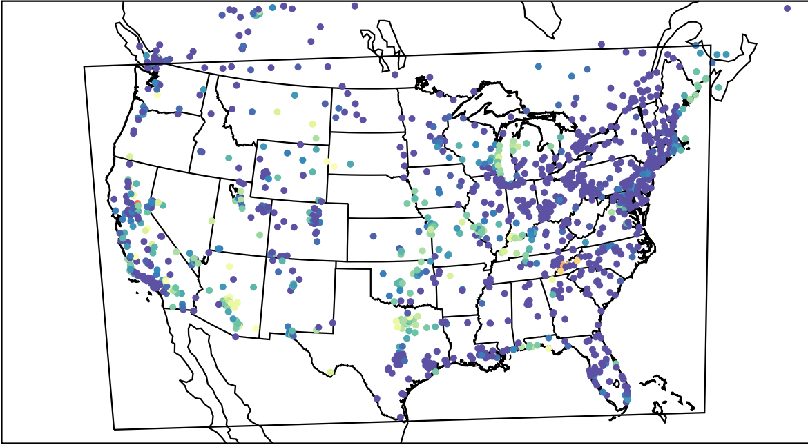
AirNOW (2023-08-26_11:00:00)
