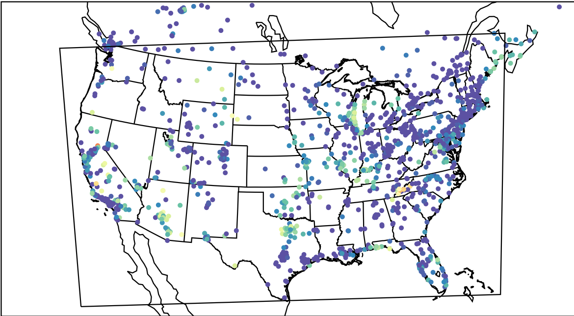
AirNOW (2023-08-26_12:00:00)
