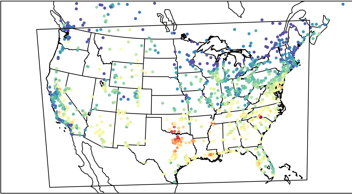
AirNOW (2023-08-26_16:00:00)
