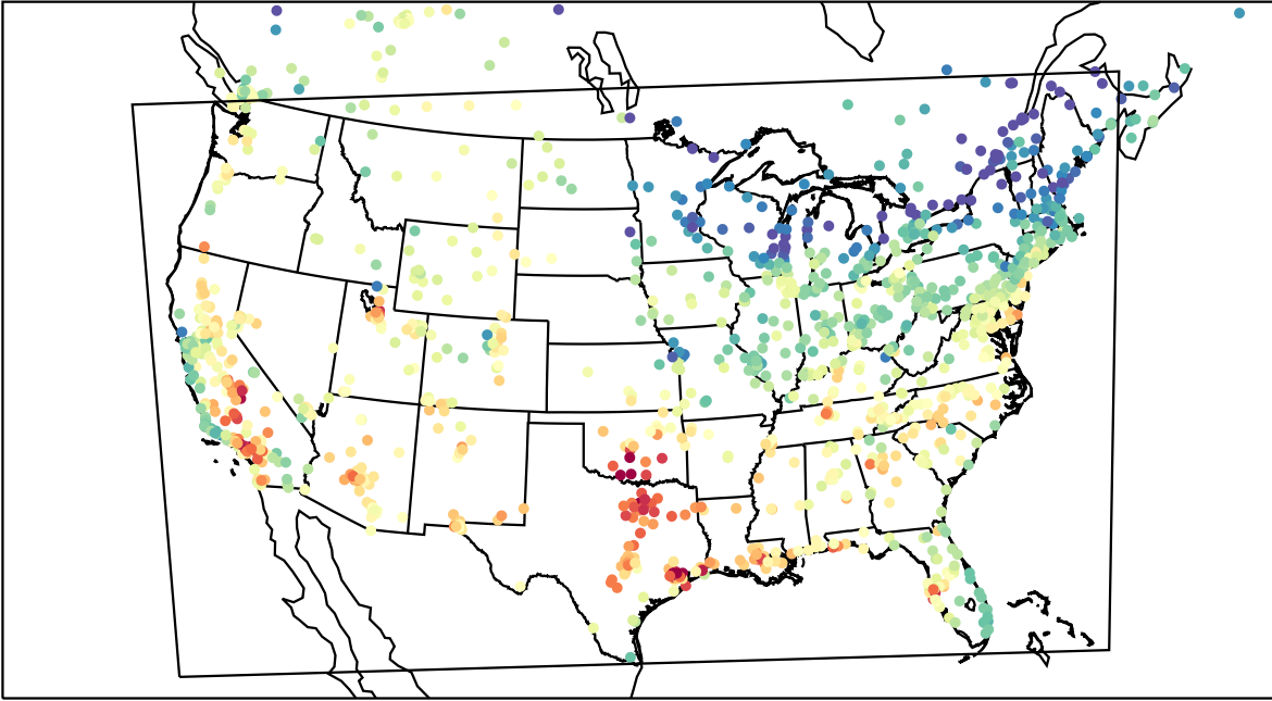
AirNOW (2023-08-26_19:00:00)
