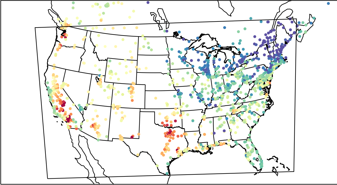
AirNOW (2023-08-26_23:00:00)
