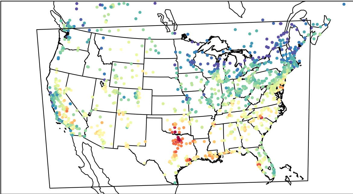
AirNOW (2023-08-26_17:00:00)
