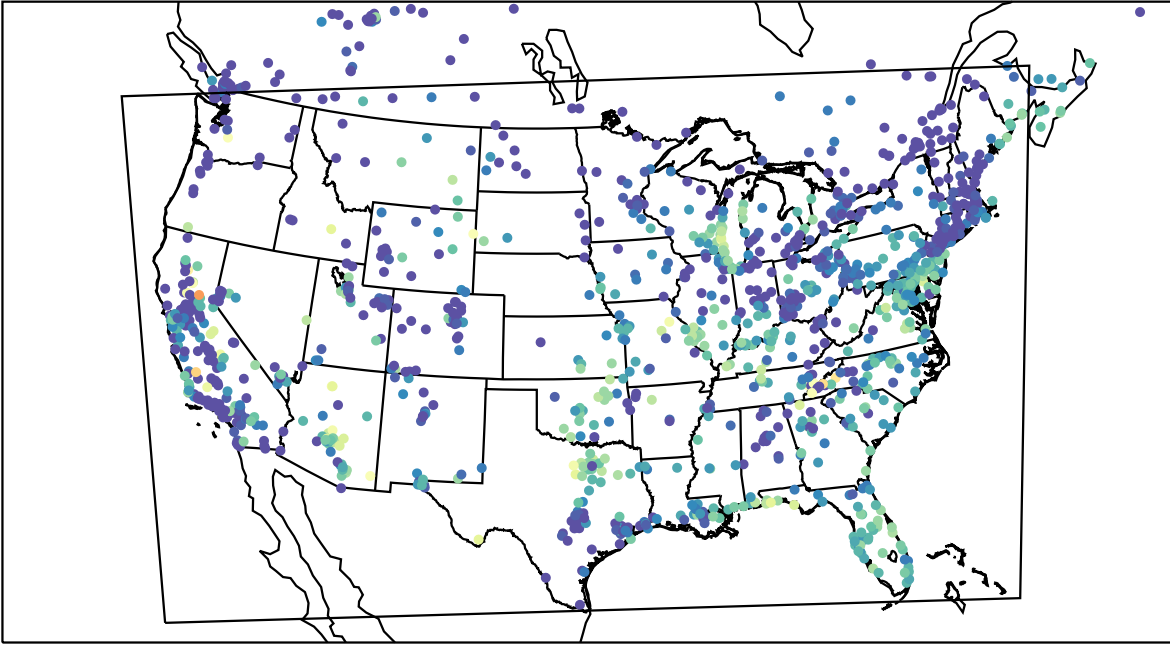
AirNOW (2023-08-26_13:00:00)
