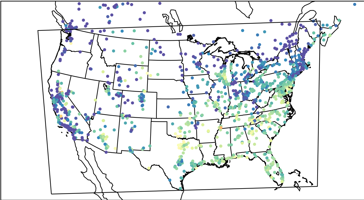
AirNOW (2023-08-26_14:00:00)
