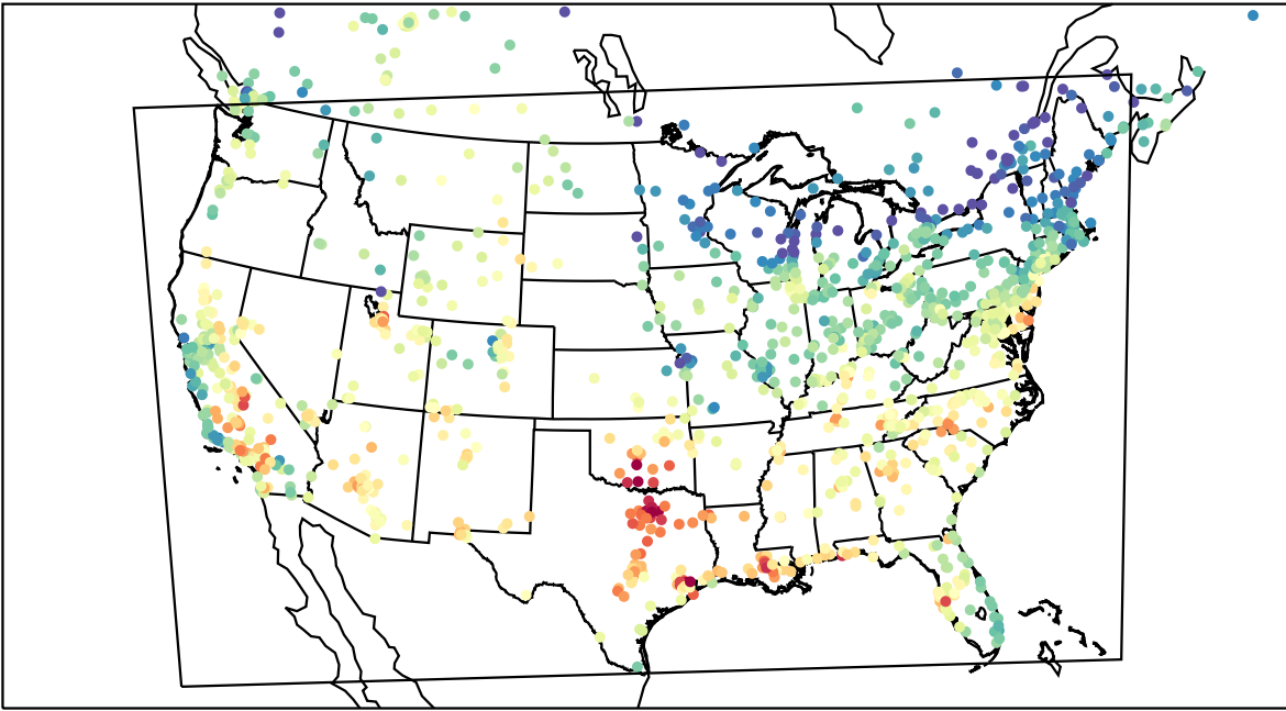
AirNOW (2023-08-26_18:00:00)
