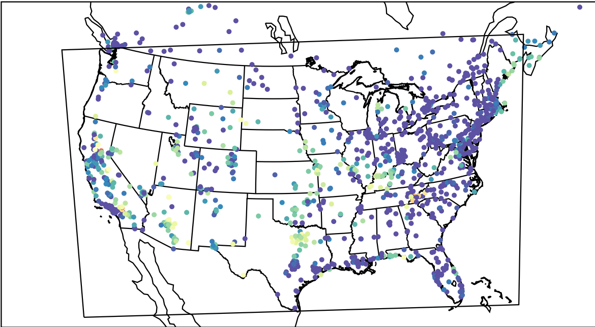
AirNOW (2023-08-26_10:00:00)
