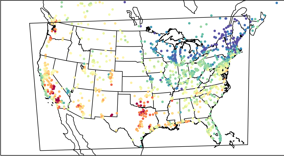
AirNOW (2023-08-26_22:00:00)
