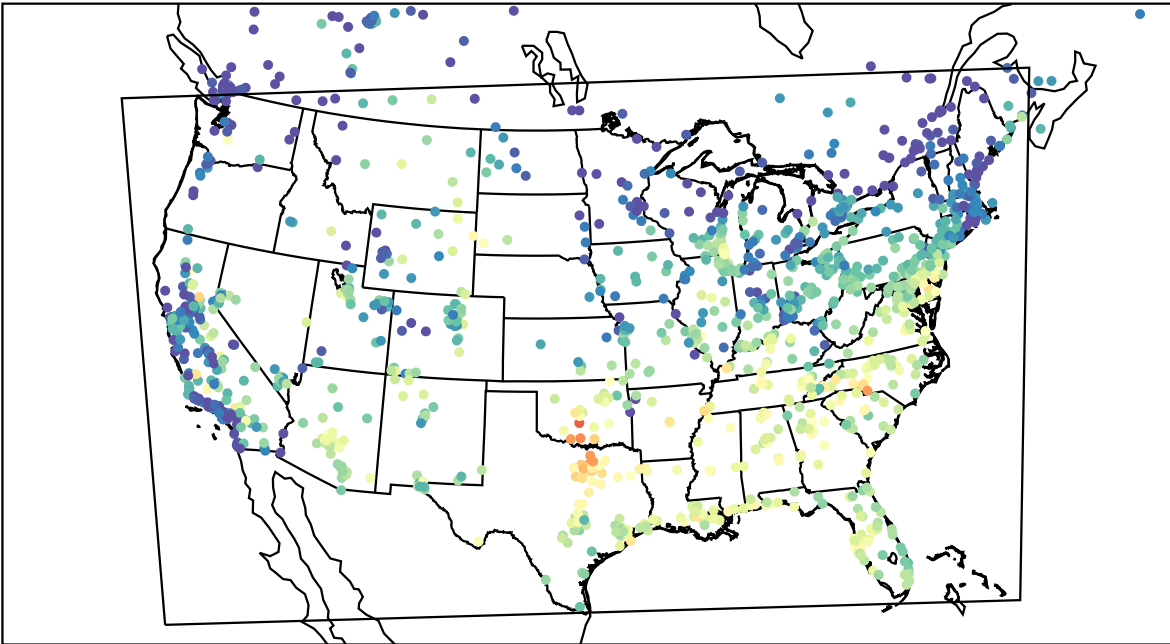
AirNOW (2023-08-26_15:00:00)
