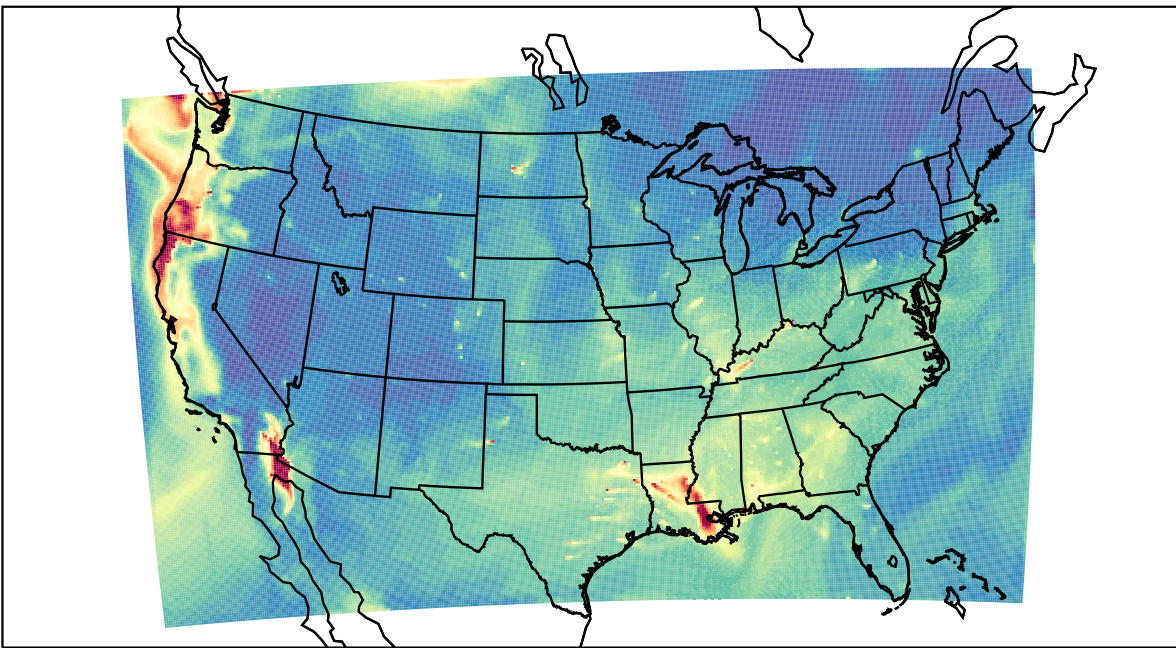
WRF 2023-08-27_16:00:00
