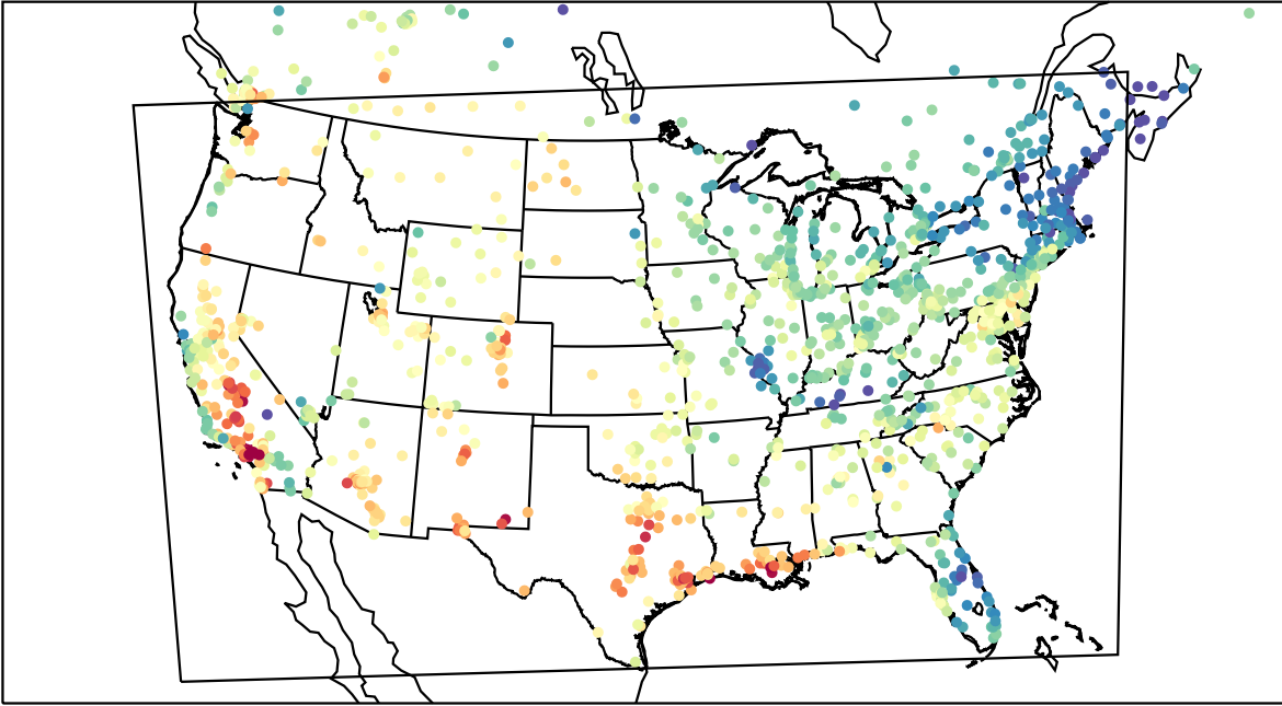
AirNOW (2023-08-27_20:00:00)
