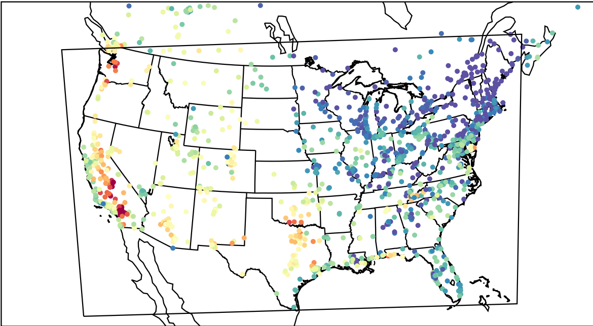
AirNOW (2023-08-27_01:00:00)
