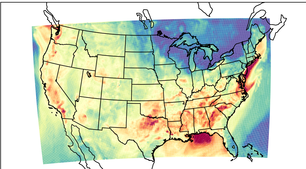
WRF (2023-08-27_01:00:00)
