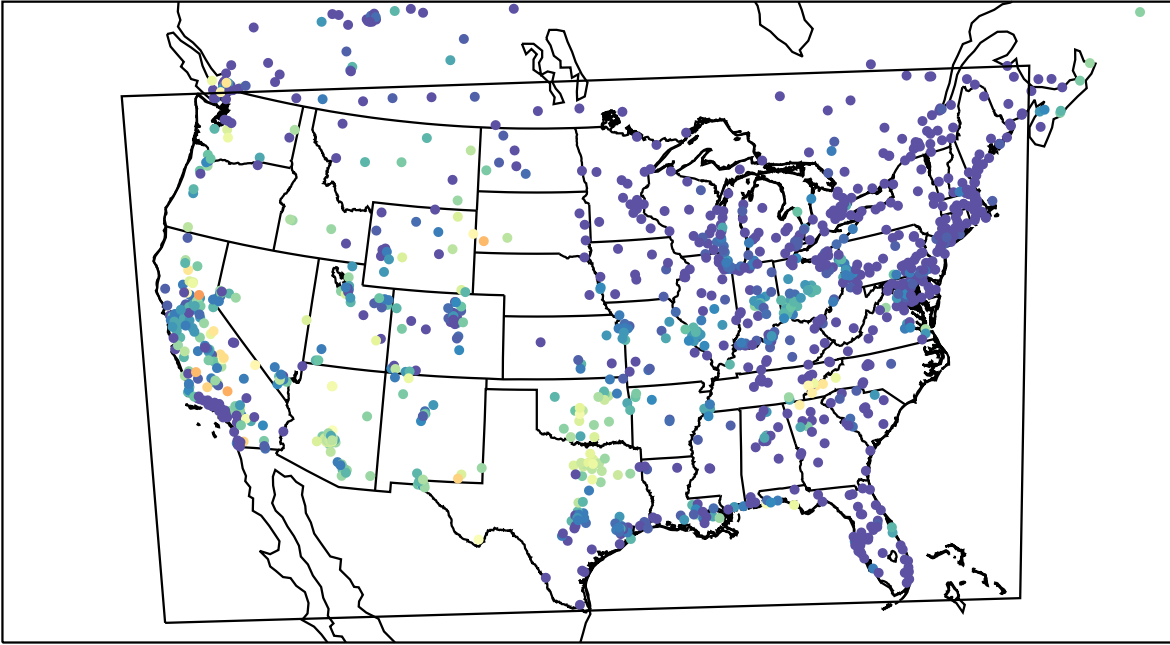
AirNOW (2023-08-27_08:00:00)
