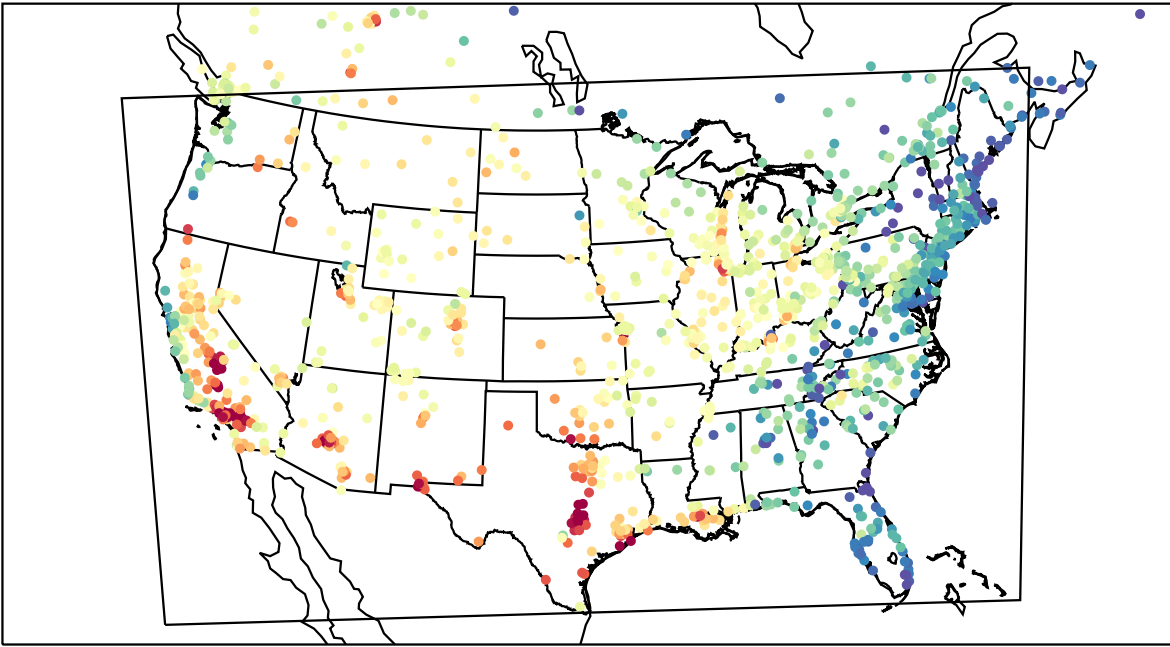
AirNOW (2023-08-28_22:00:00)
