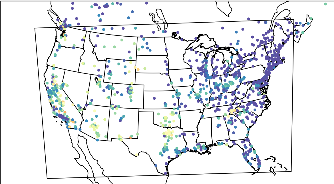
AirNOW (2023-08-27_06:00:00)
