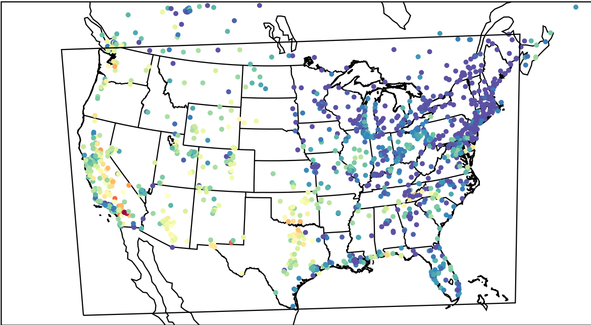
AirNOW (2023-08-27_03:00:00)
