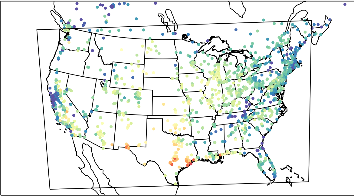
AirNOW (2023-08-28_16:00:00)
