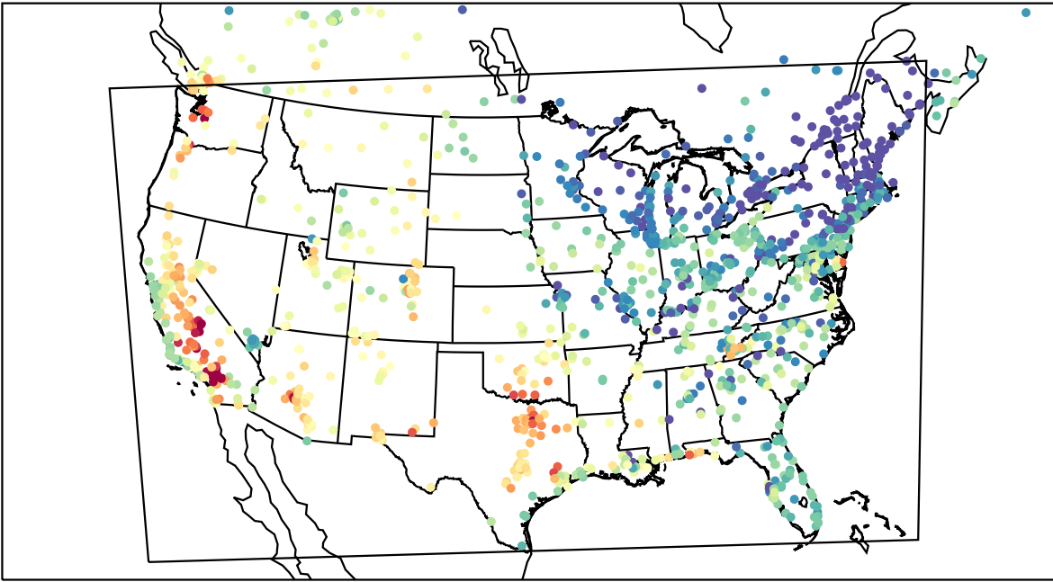
AirNOW (2023-08-27_00:00:00)
