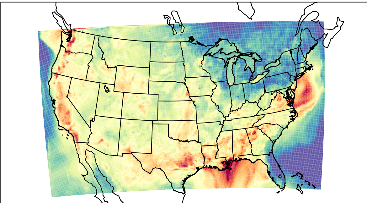
WRF (2023-08-28_01:00:00)
