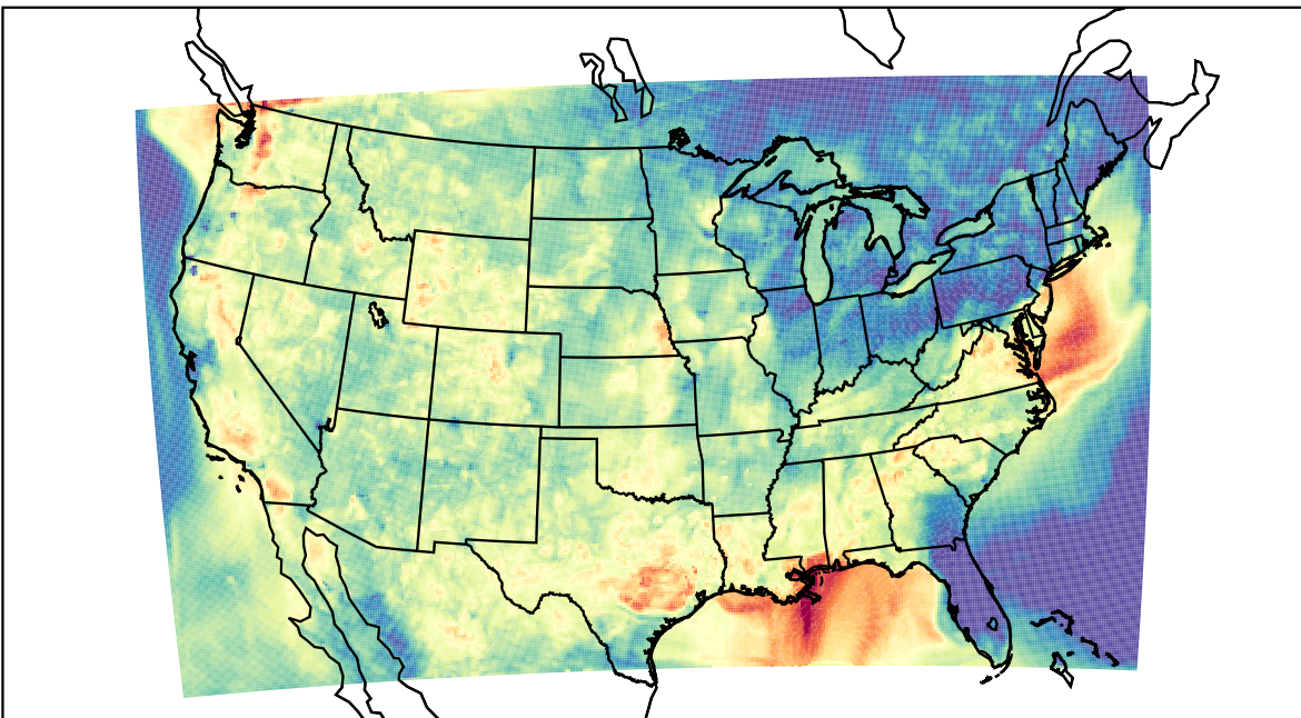
WRF (2023-08-28_04:00:00)
