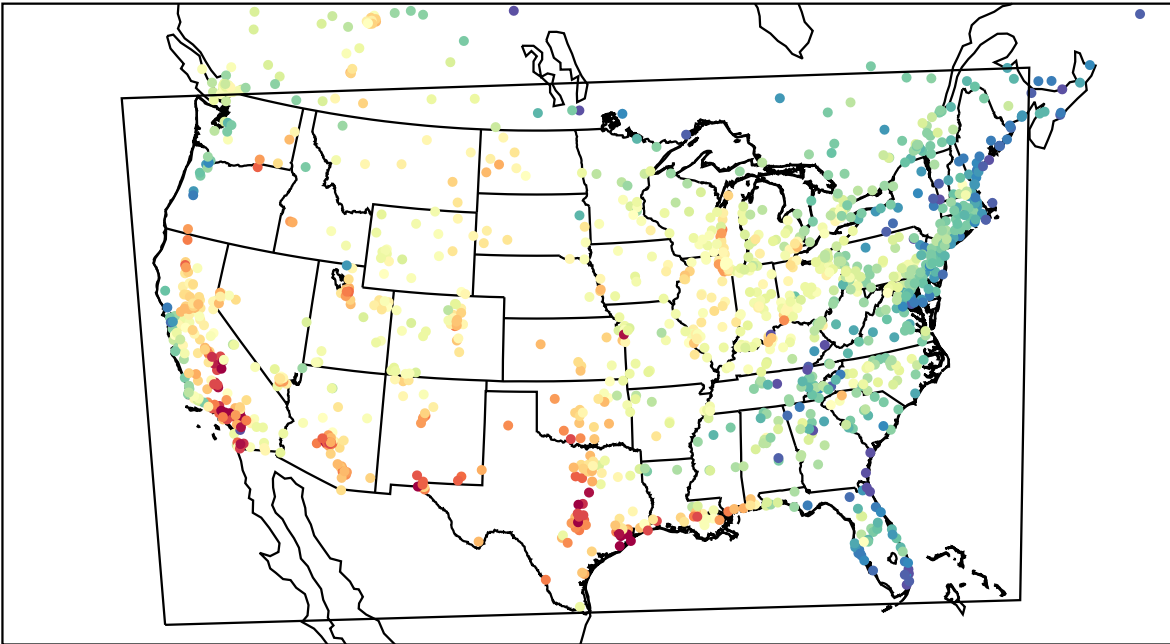
AirNOW (2023-08-28_20:00:00)
