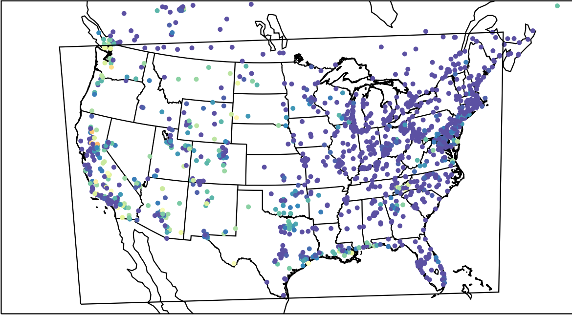
AirNOW (2023-08-28_11:00:00)
