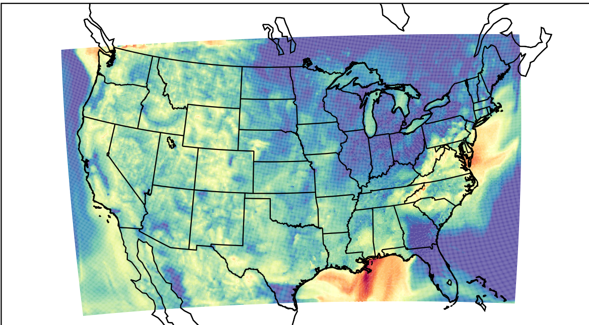
WRF (2023-08-28_13:00:00)
