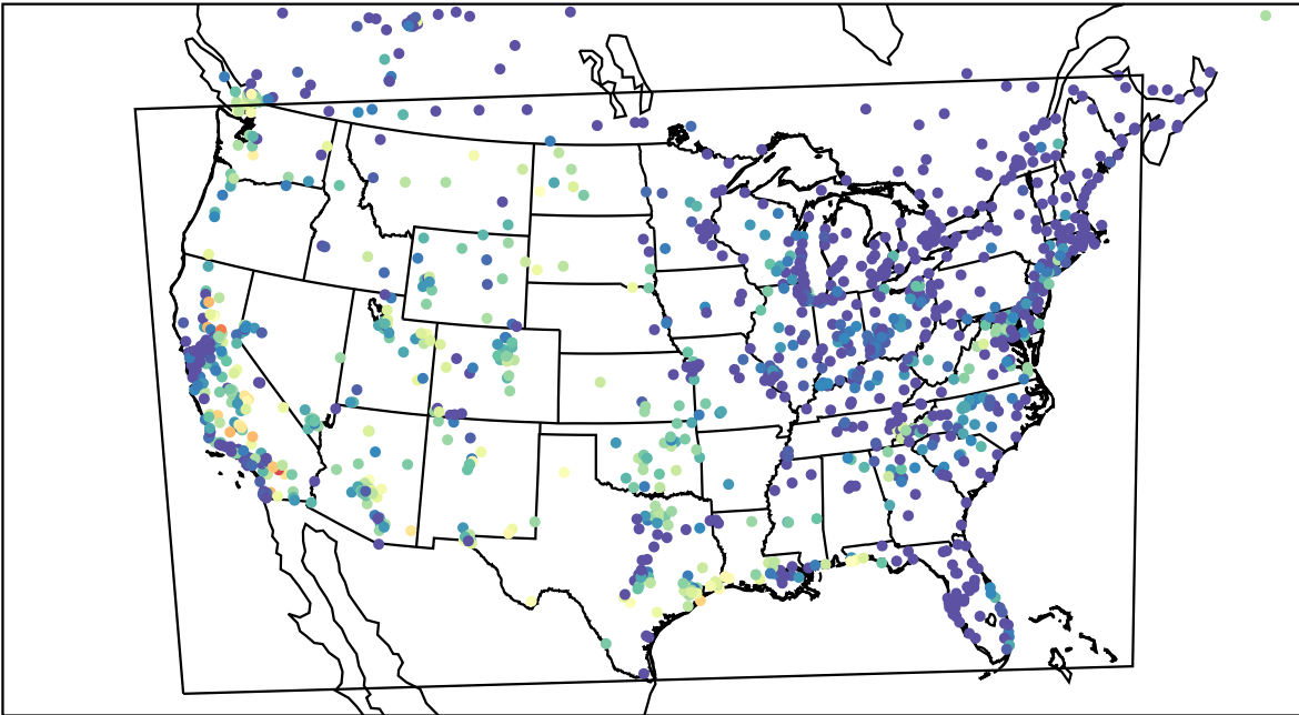
AirNOW (2023-08-28_06:00:00)
