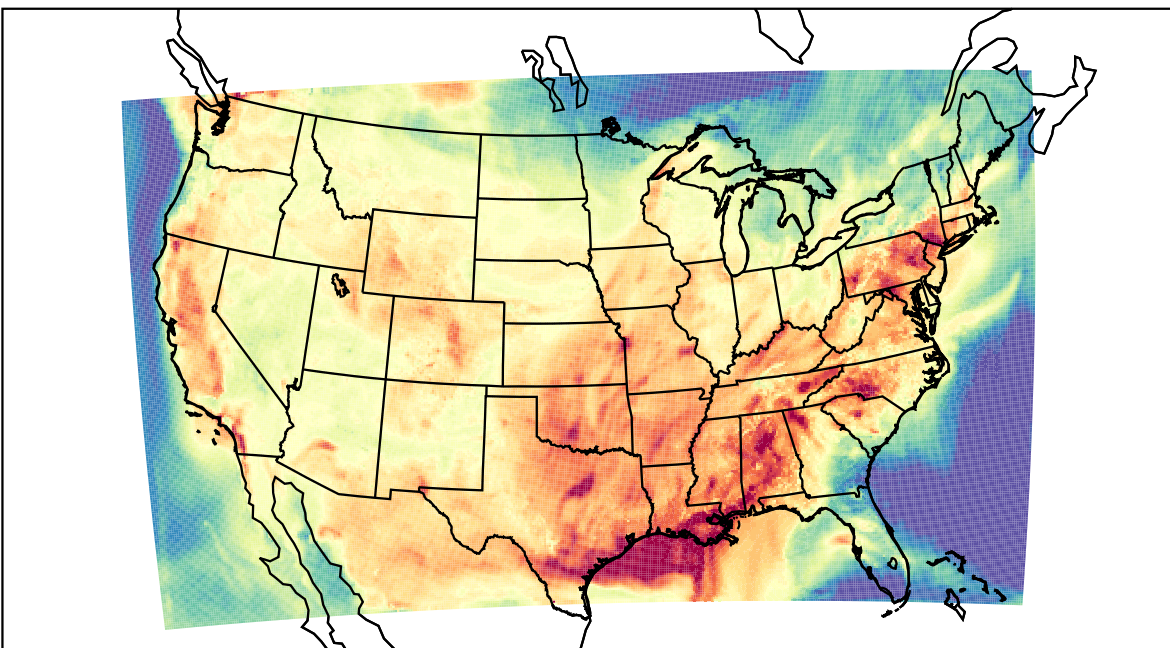
WRF (2023-08-28_20:00:00)
