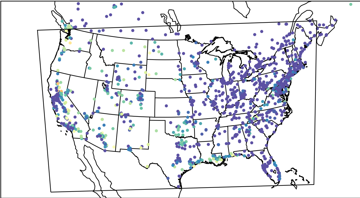
AirNOW (2023-08-28_10:00:00)
