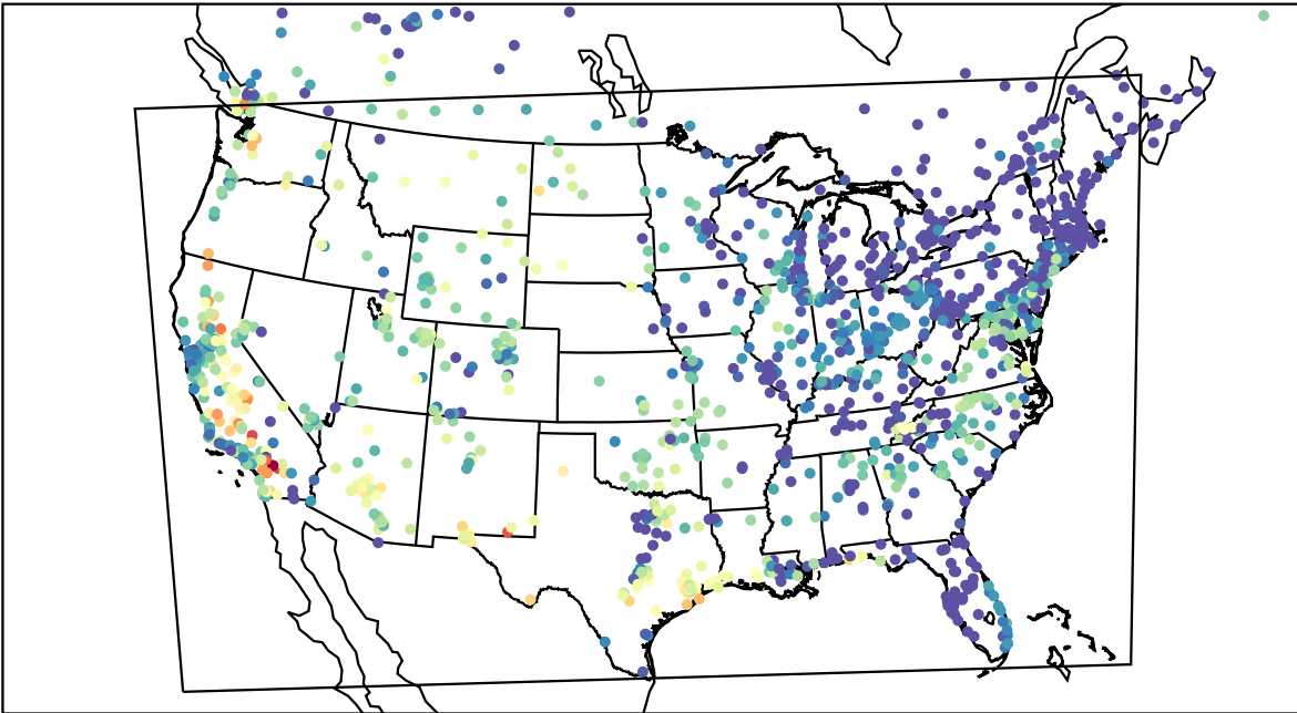
AirNOW (2023-08-28_03:00:00)
