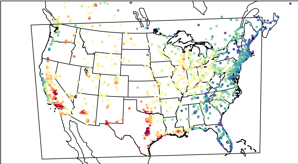
AirNOW (2023-08-28_22:00:00)
