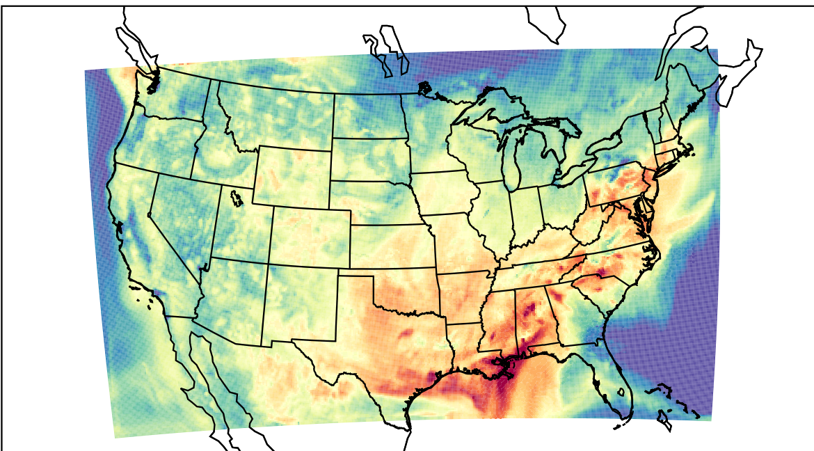
WRF (2023-08-28_16:00:00)
