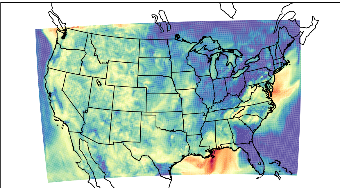
WRF (2023-08-28_11:00:00)
