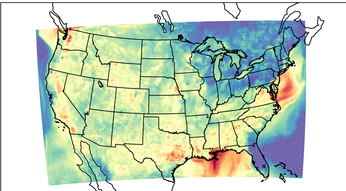
WRF (2023-08-28_03:00:00)
