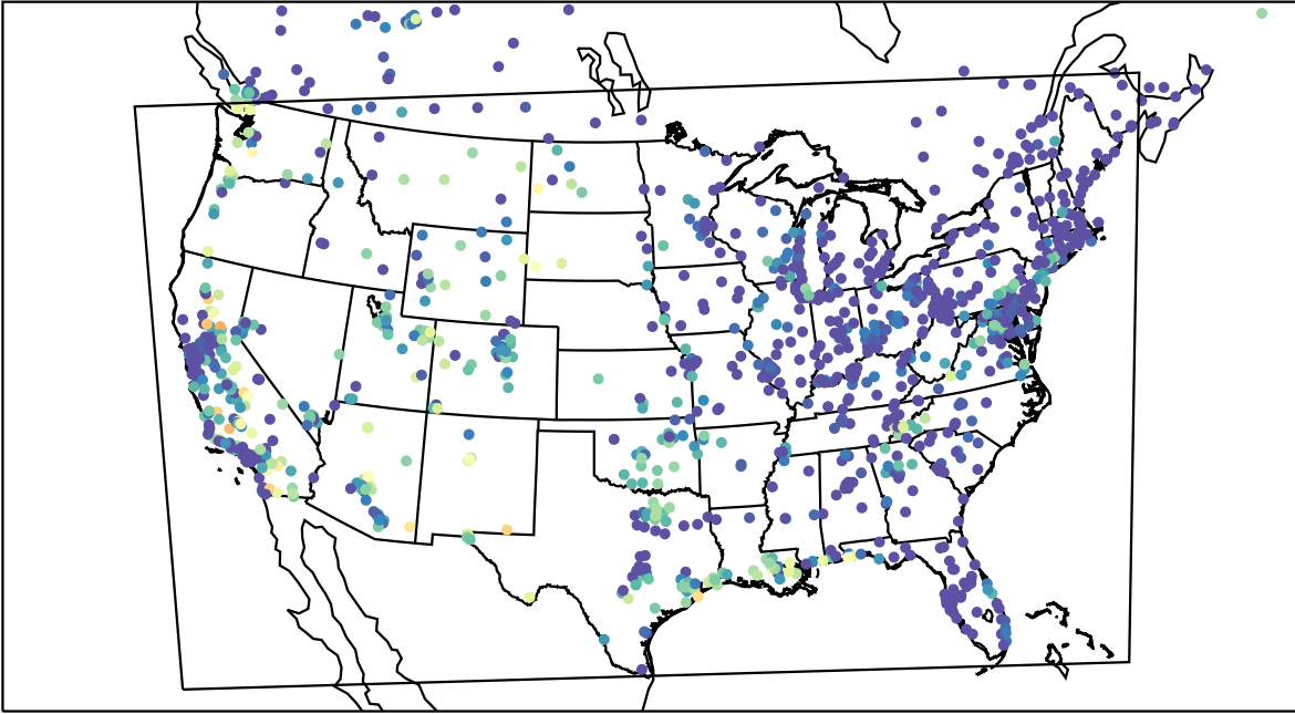
AirNOW (2023-08-28_08:00:00)
