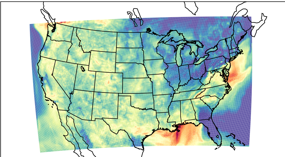
WRF (2023-08-28_08:00:00)
