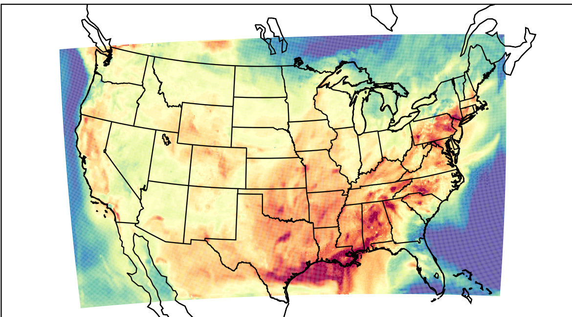
WRF (2023-08-28_19:00:00)
