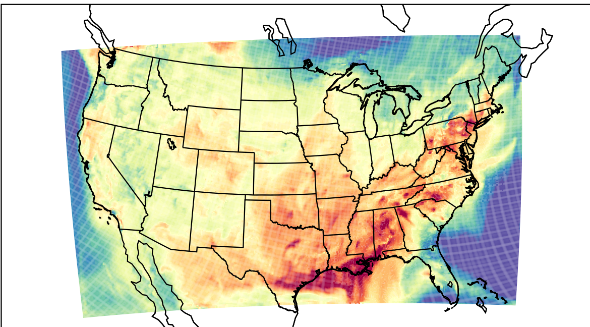
WRF (2023-08-28_18:00:00)
