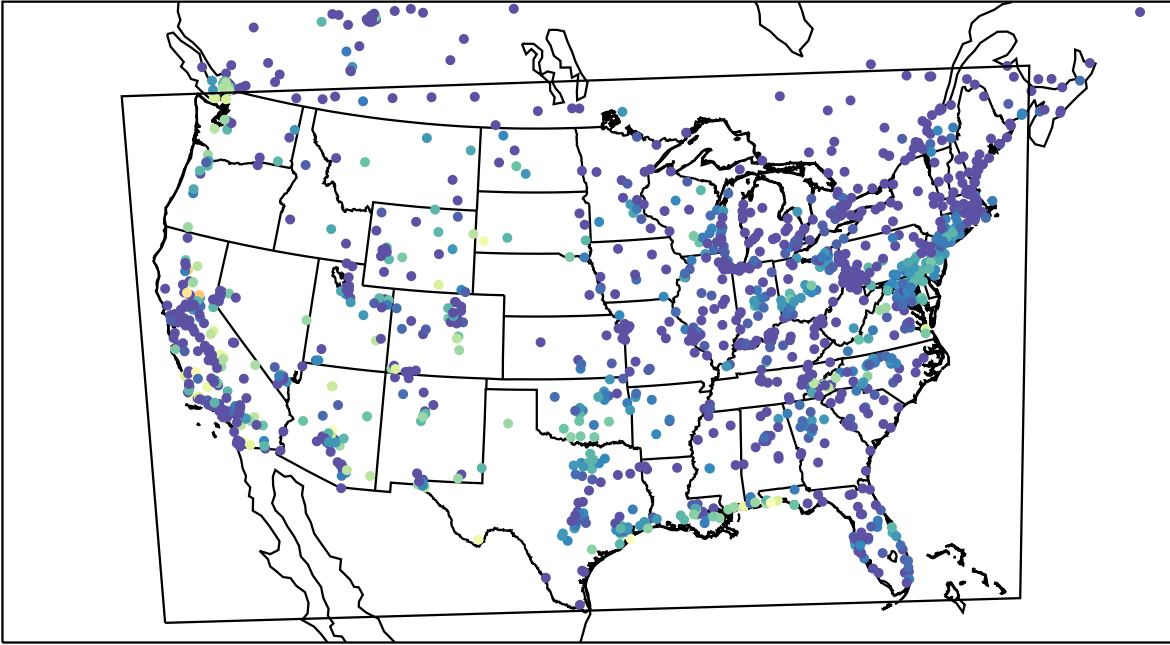
AirNOW (2023-08-28_13:00:00)
