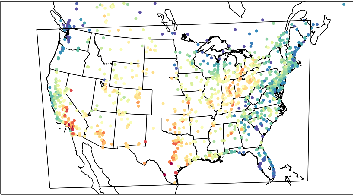
AirNOW (2023-08-29_18:00:00)
