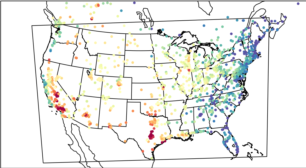
AirNOW (2023-08-28_23:00:00)
