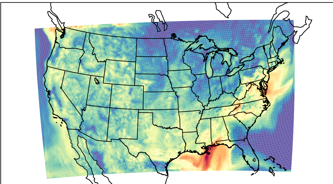
WRF (2023-08-28_14:00:00)
