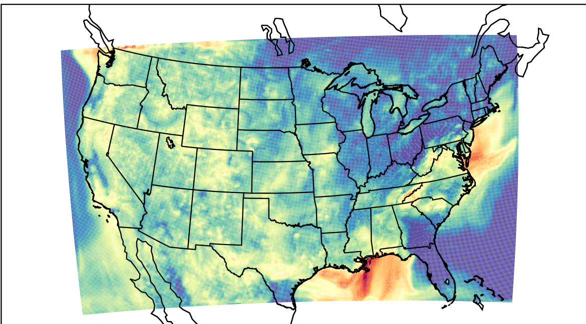
WRF (2023-08-28_10:00:00)
