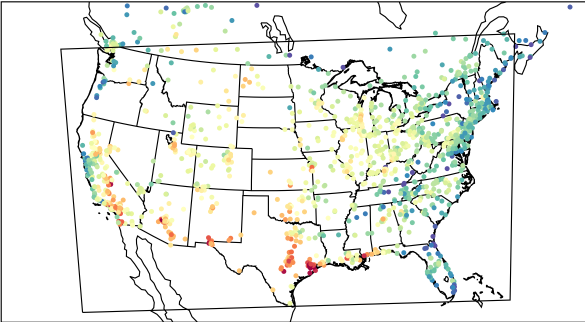
AirNOW (2023-08-28_18:00:00)
