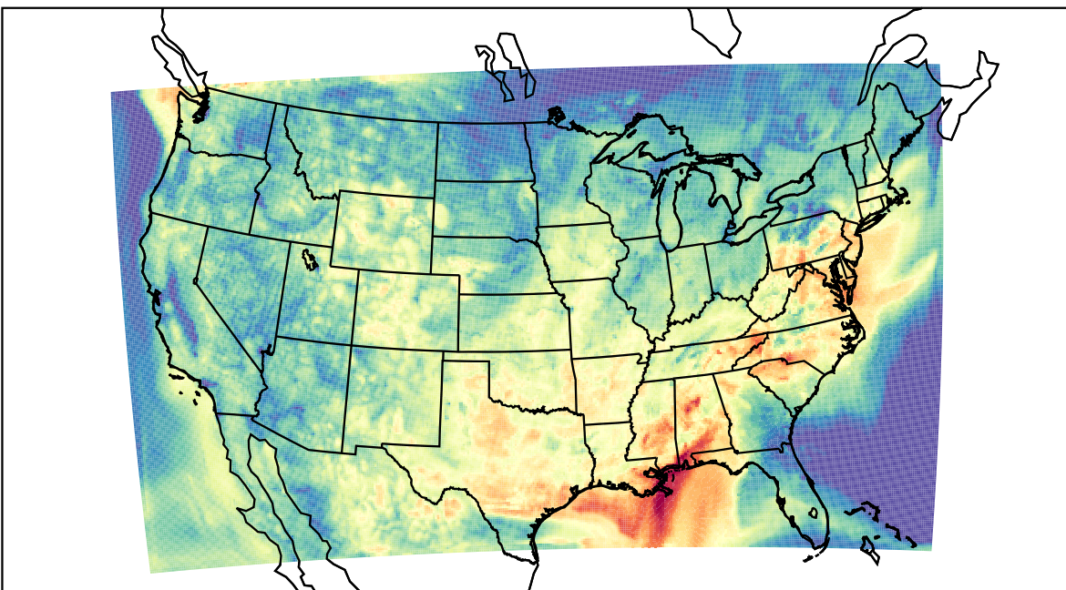
WRF (2023-08-28_15:00:00)
