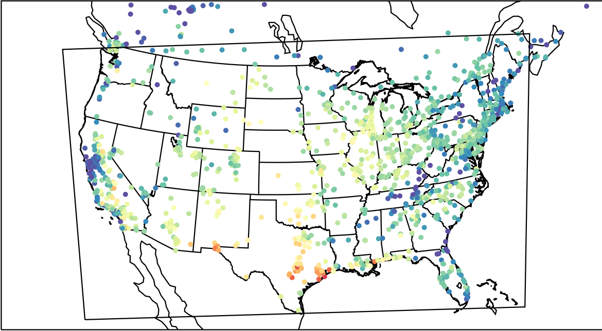
AirNOW (2023-08-28_16:00:00)
