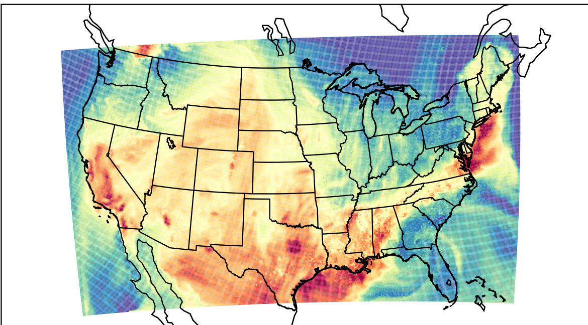
WRF (2023-08-30_23:00:00)
