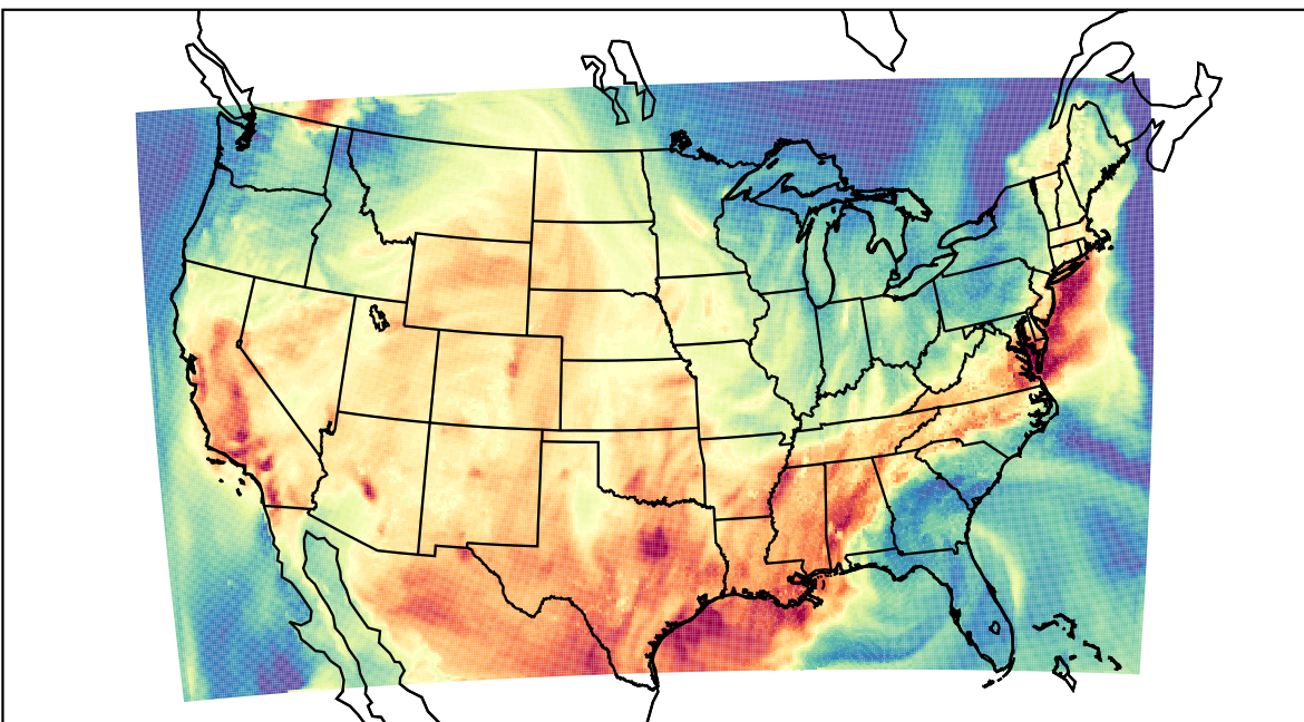
WRF (2023-08-30_22:00:00)
