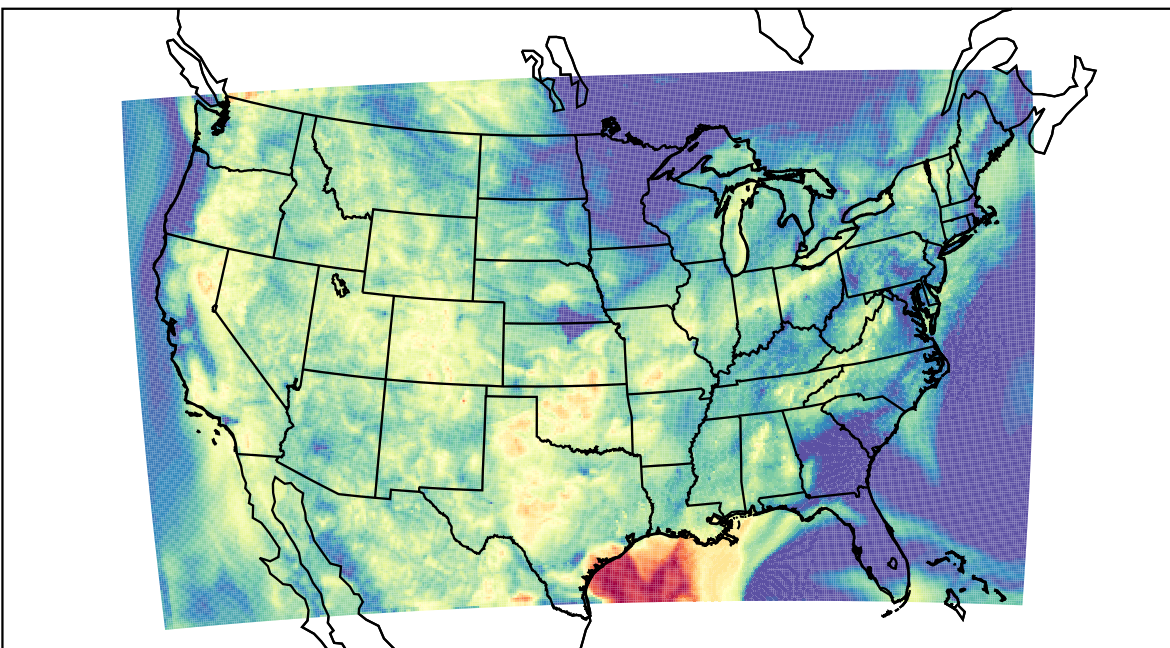
WRF (2023-08-29_10:00:00)
