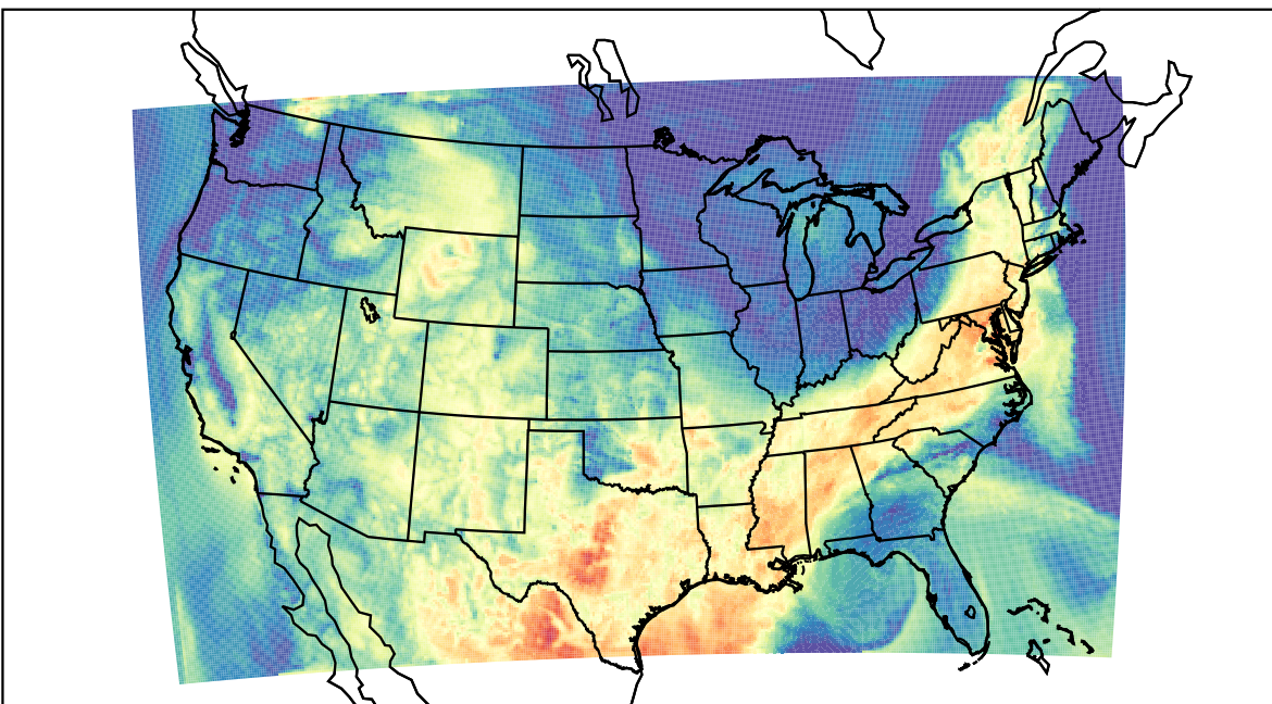
WRF (2023-08-30_15:00:00)
