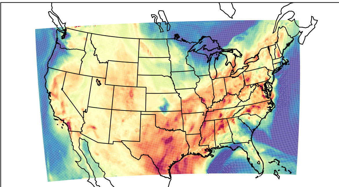
WRF (2023-08-29_20:00:00)
