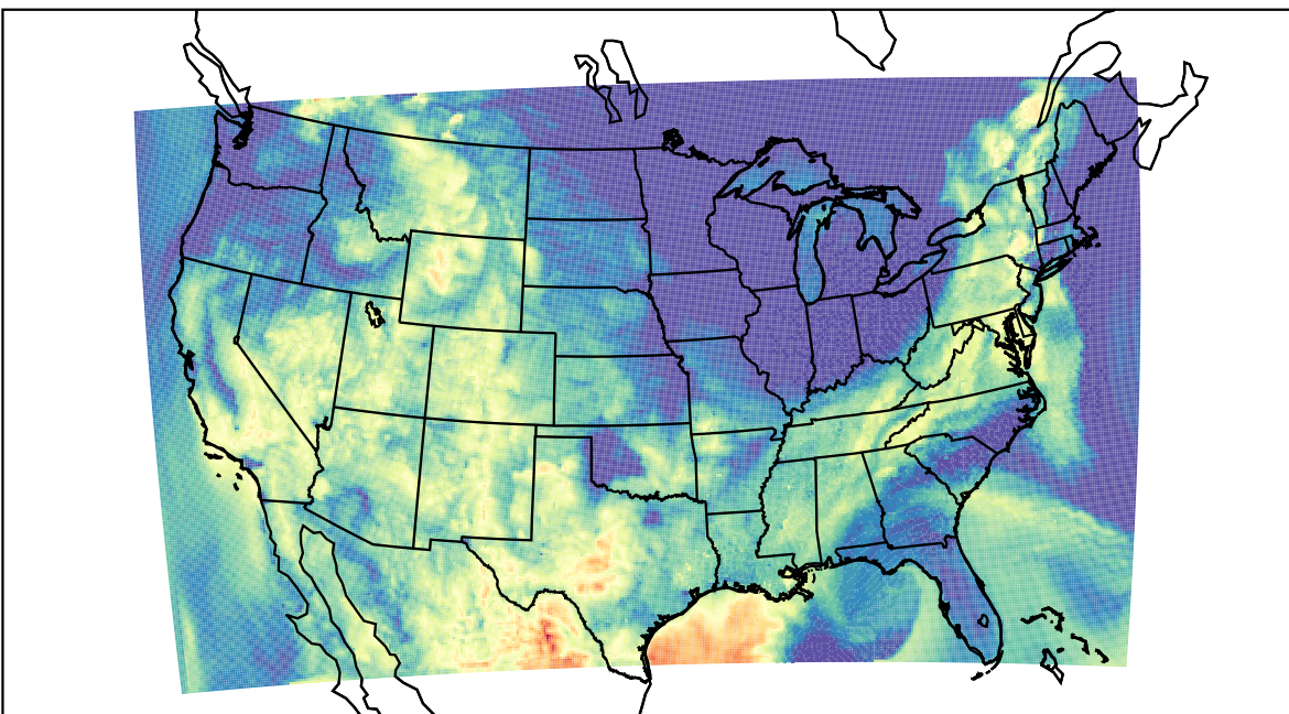
WRF (2023-08-30_13:00:00)
