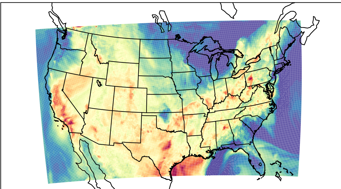
WRF (2023-08-30_01:00:00)
