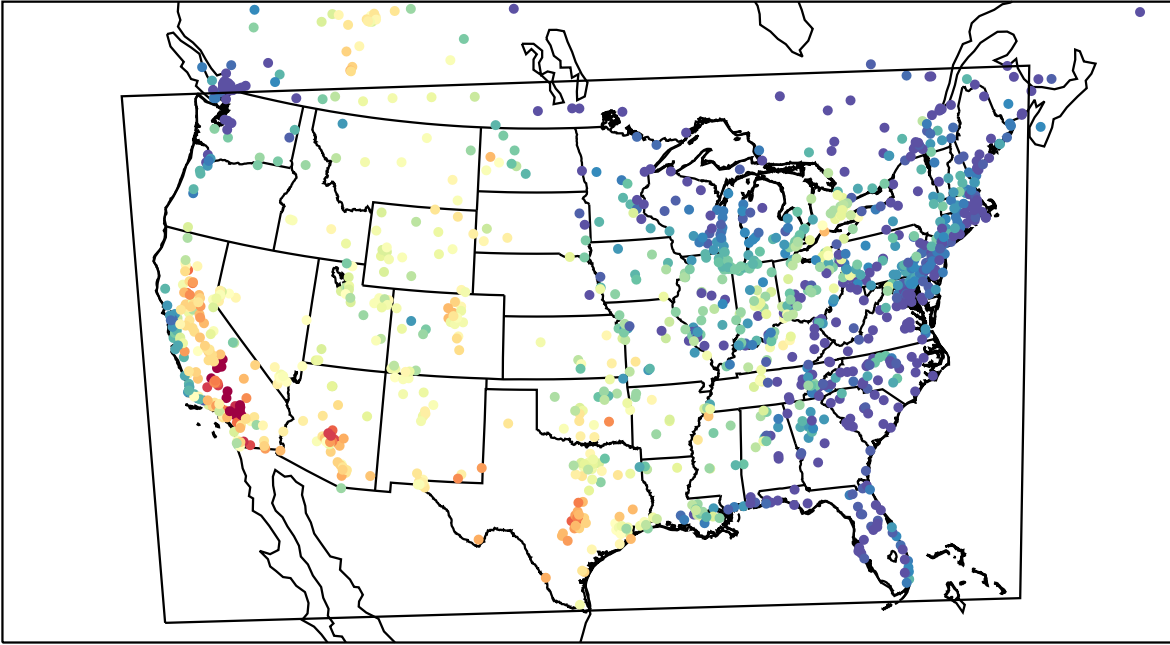
AirNOW (2023-08-30_01:00:00)
