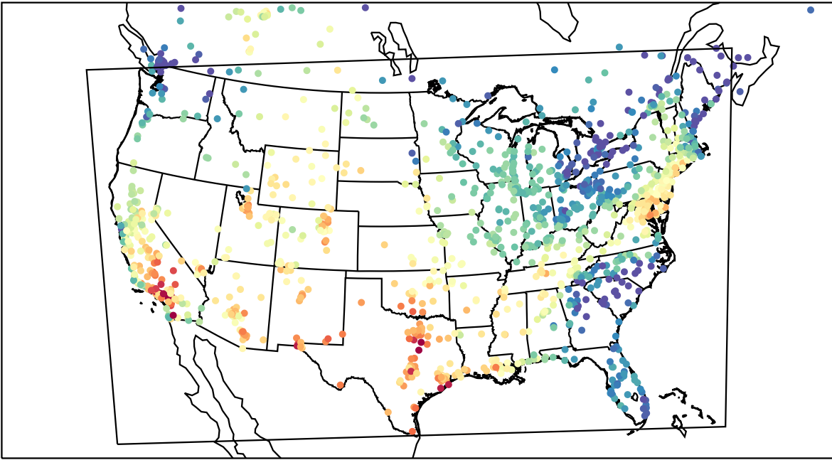
AirNOW (2023-08-30_18:00:00)
