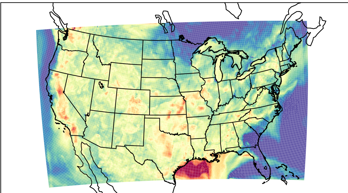
WRF (2023-08-29_03:00:00)
