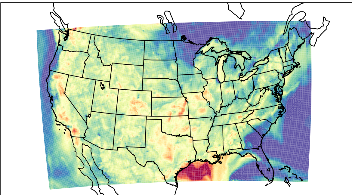
WRF (2023-08-29_04:00:00)
