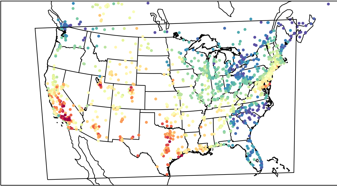
AirNOW (2023-08-30_20:00:00)
