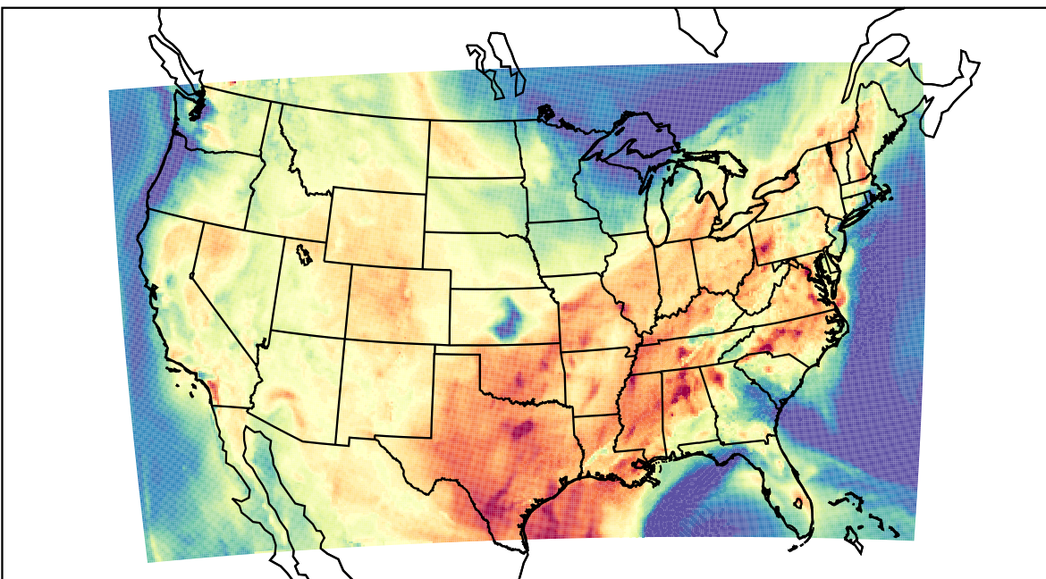
WRF (2023-08-29_18:00:00)
