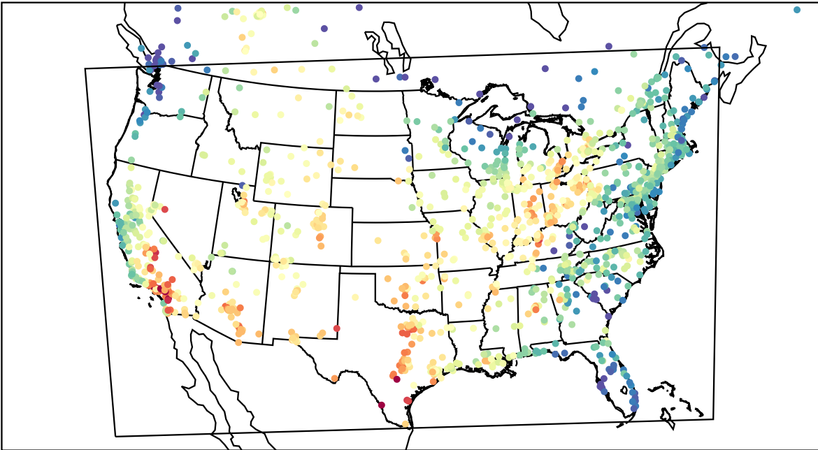
AirNOW (2023-08-29_18:00:00)
