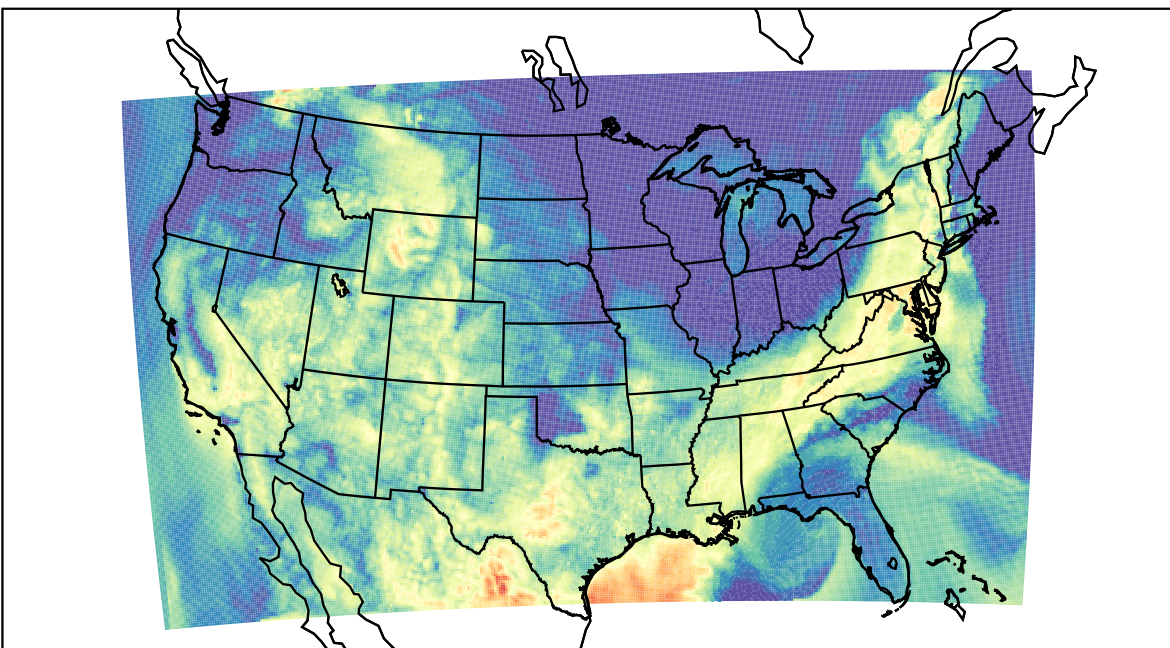
WRF (2023-08-30_14:00:00)
