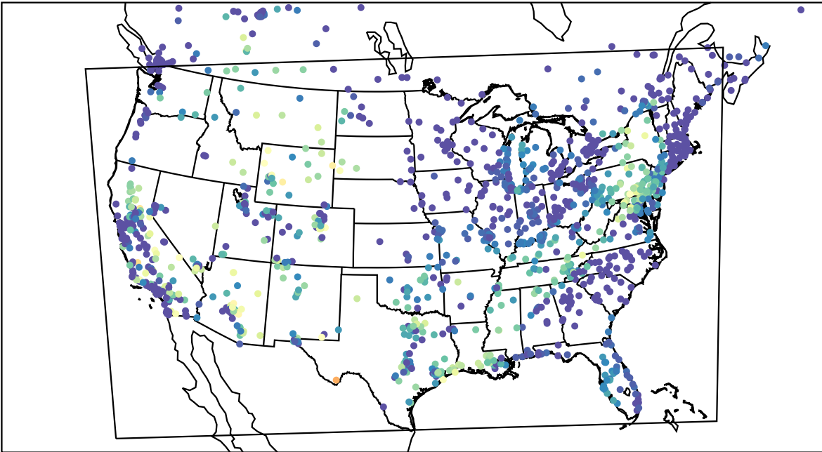
AirNOW (2023-08-30_13:00:00)
