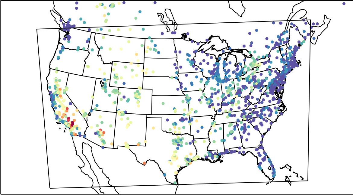
AirNOW (2023-08-30_03:00:00)
