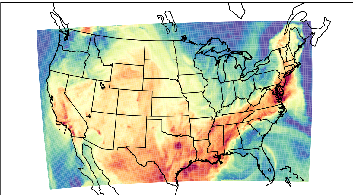
WRF (2023-08-30_20:00:00)
