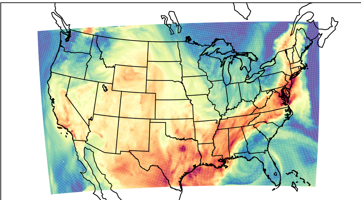
WRF (2023-08-30_19:00:00)
