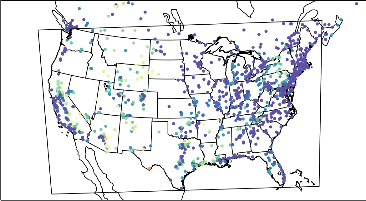
AirNOW (2023-08-30_10:00:00)
