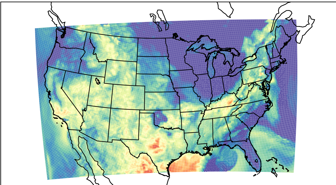
WRF (2023-08-30_10:00:00)
