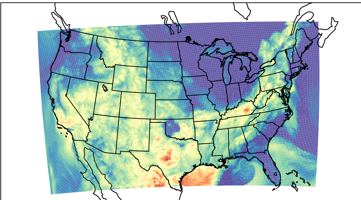
WRF (2023-08-30_09:00:00)
