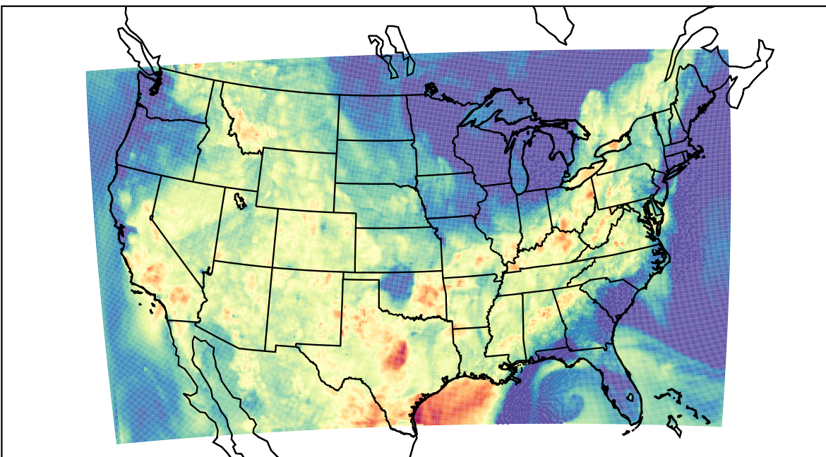
WRF (2023-08-30_04:00:00)
