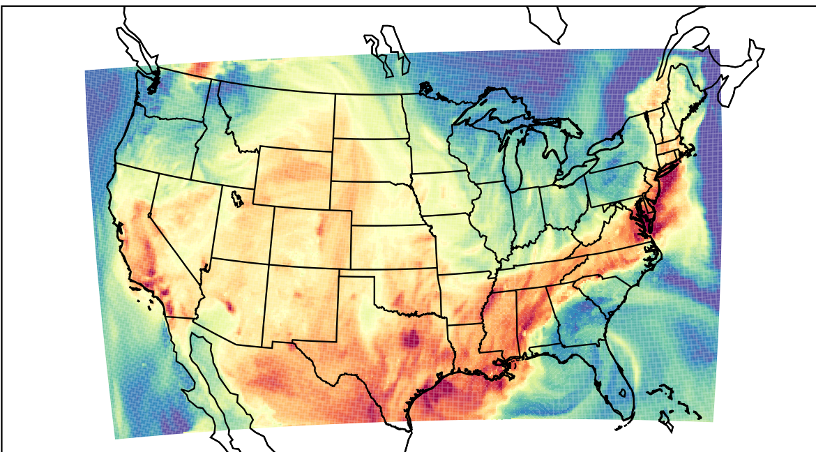
WRF (2023-08-30_21:00:00)
