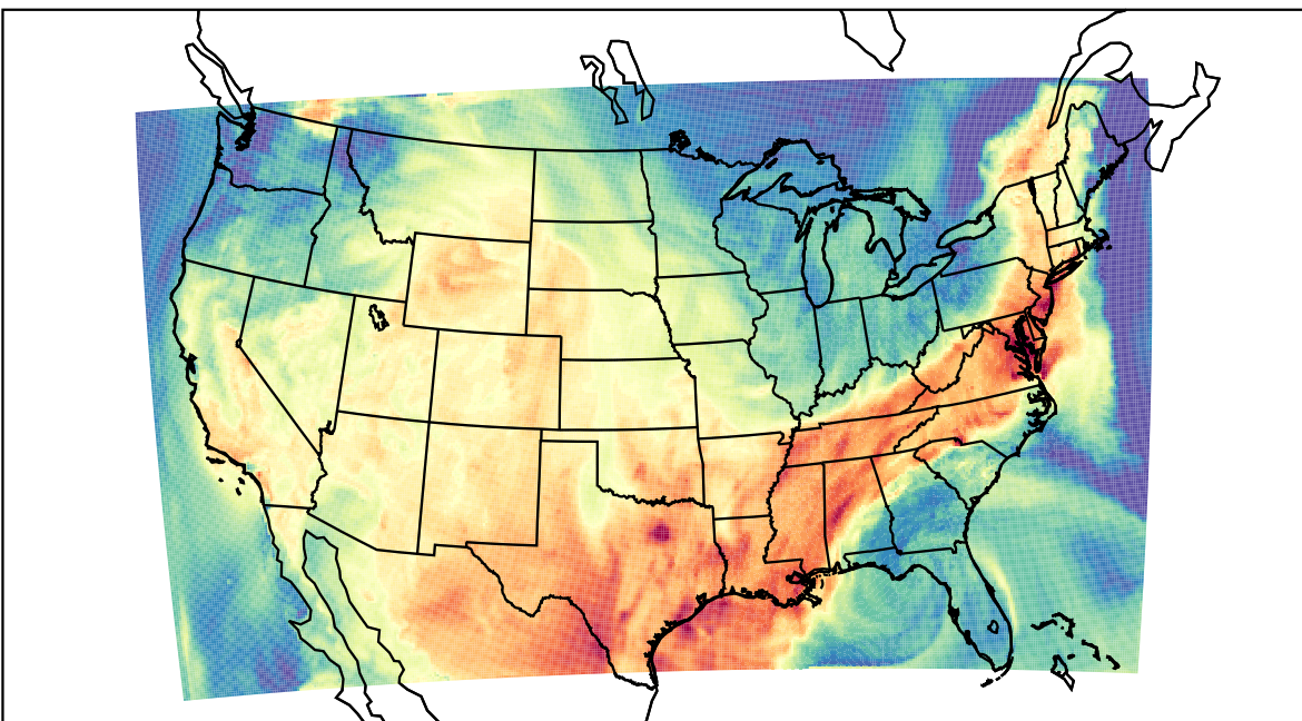
WRF (2023-08-30_18:00:00)
