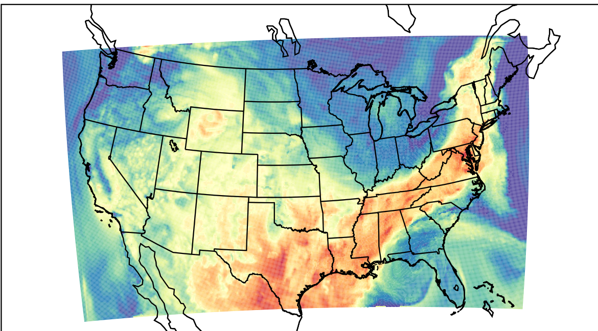
WRF (2023-08-30_16:00:00)
