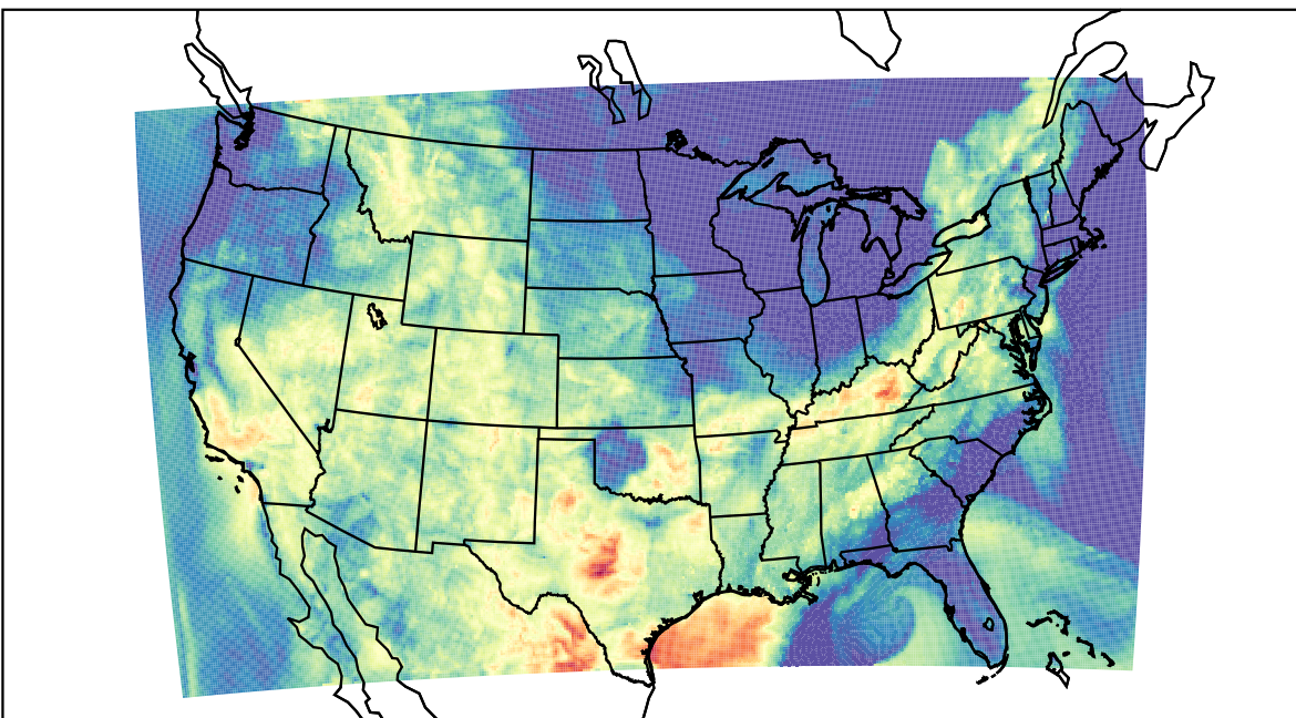
WRF (2023-08-30_08:00:00)
