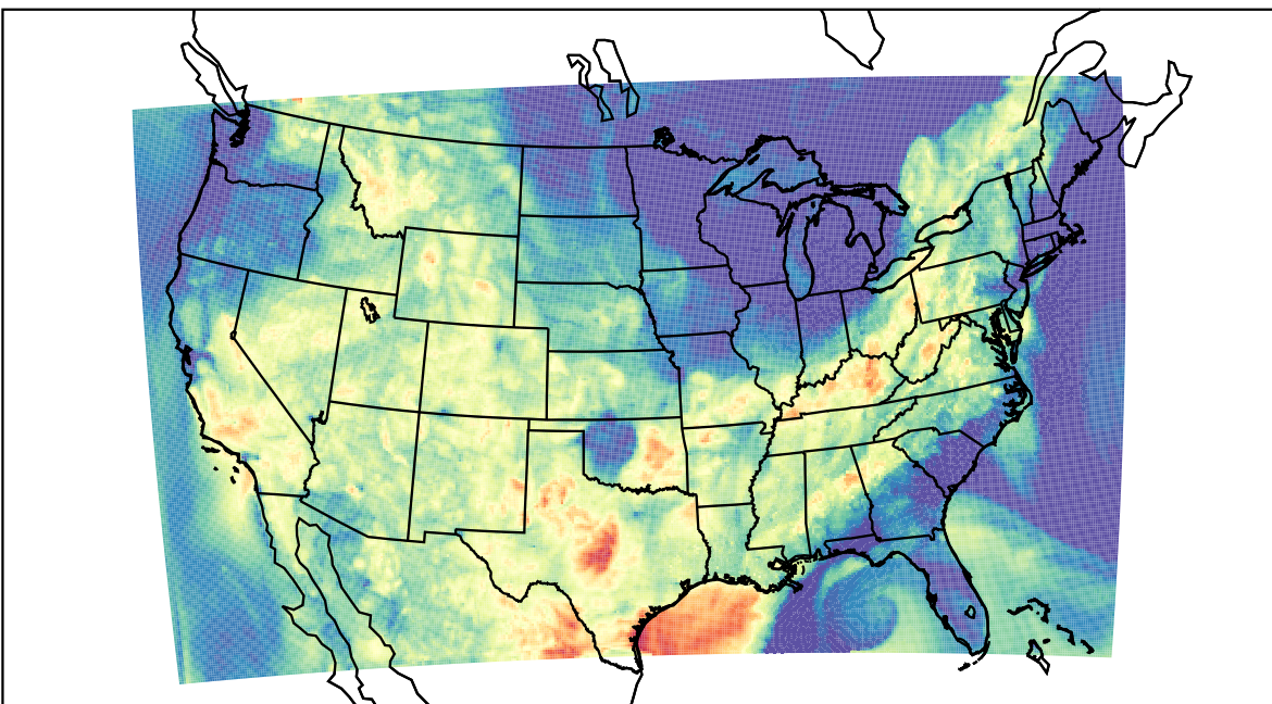
WRF (2023-08-30_06:00:00)
