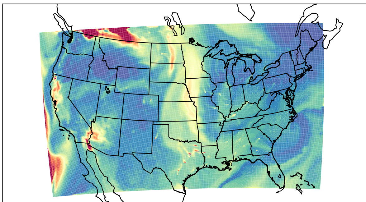
WRF 2023-08-31_16:00:00
