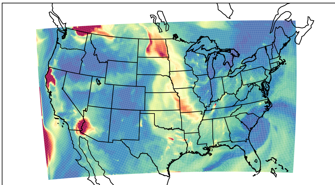
WRF 2023-08-31_06:00:00
