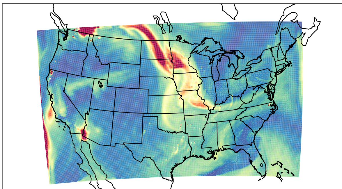
WRF 2023-08-30_21:00:00
