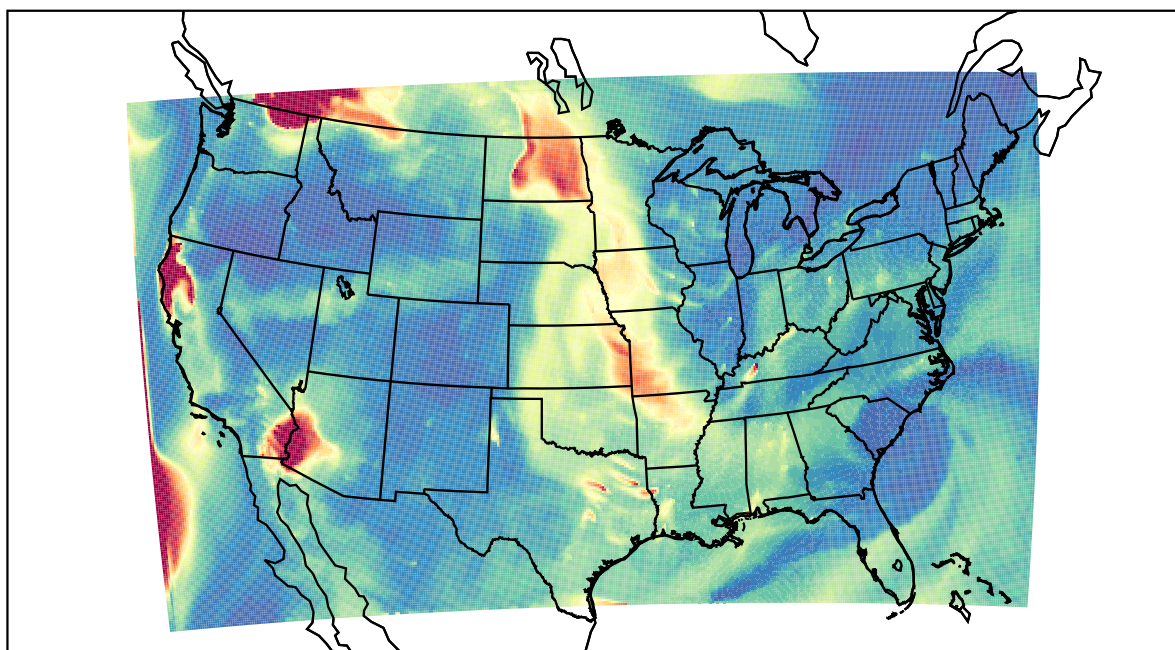
WRF 2023-08-31_07:00:00
