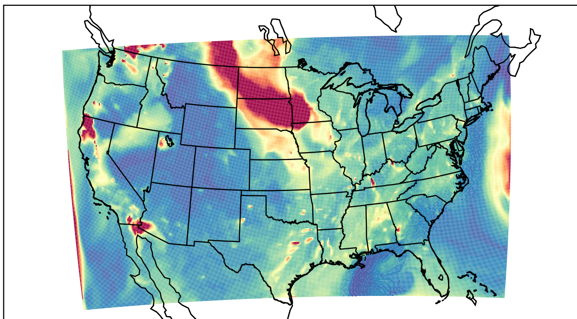
WRF 2023-08-30_04:00:00
