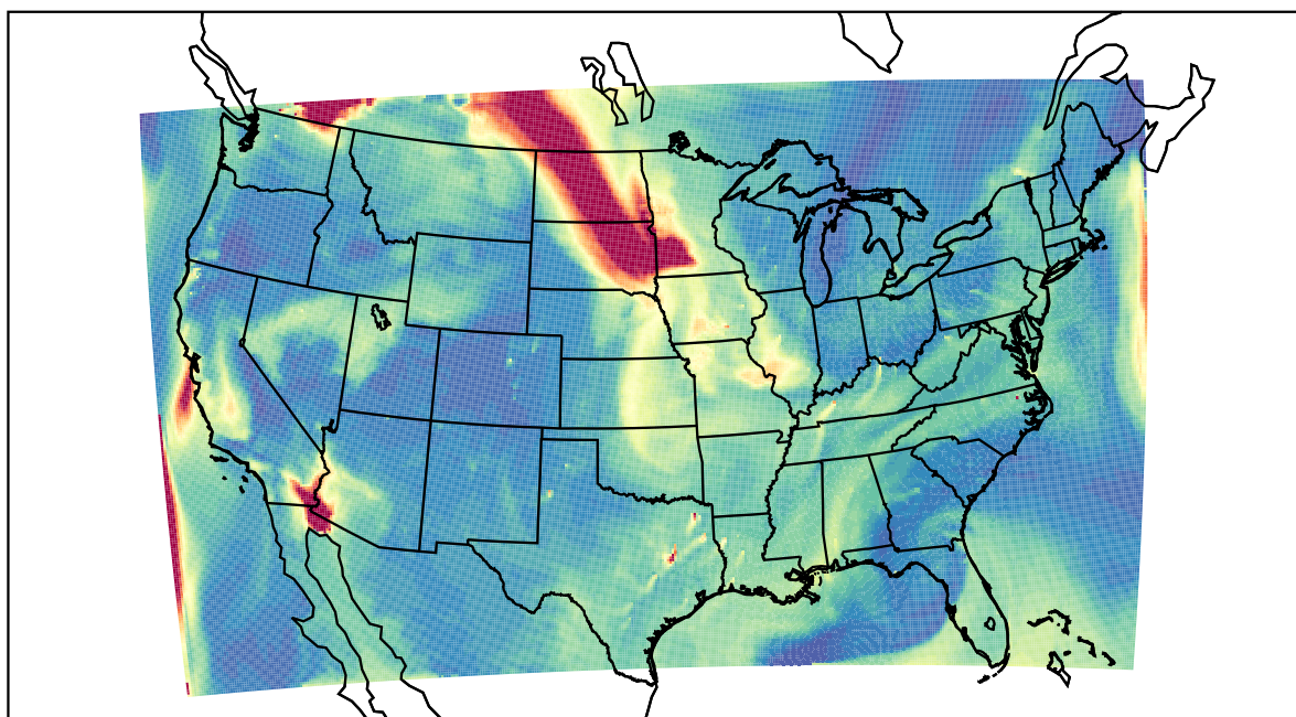
WRF 2023-08-30_17:00:00
