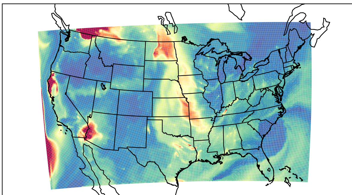
WRF 2023-08-31_08:00:00
