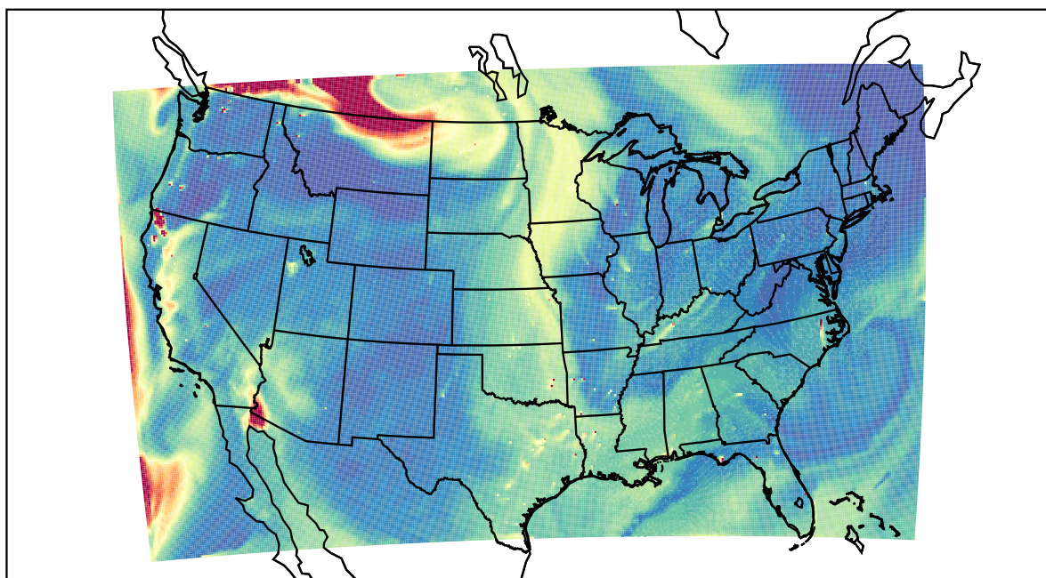
WRF 2023-08-31_22:00:00
