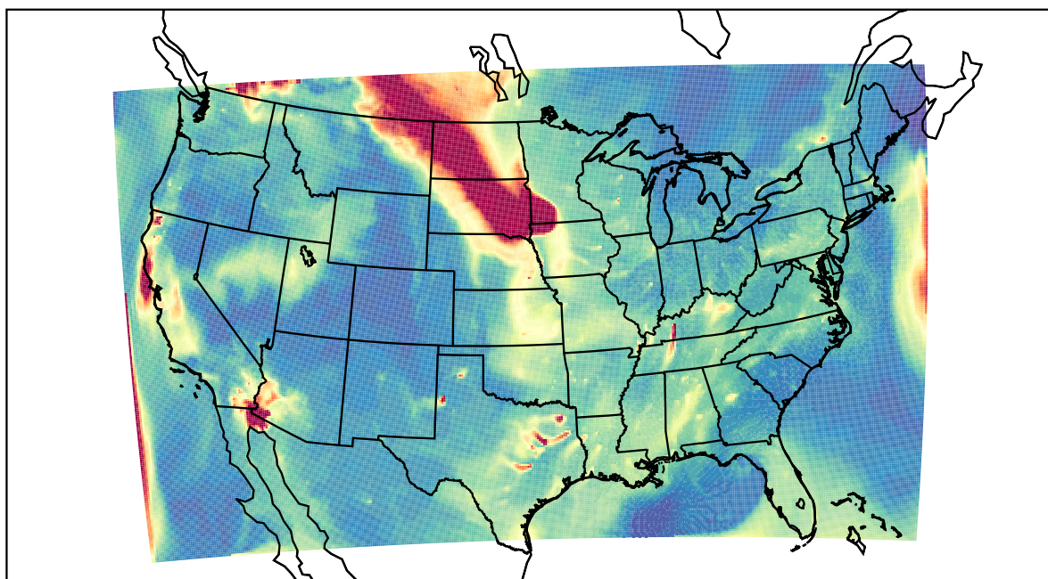
WRF 2023-08-30_12:00:00
