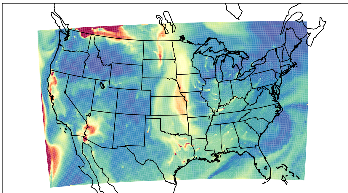
WRF 2023-08-31_14:00:00
