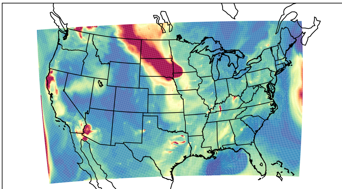
WRF 2023-08-30_09:00:00
