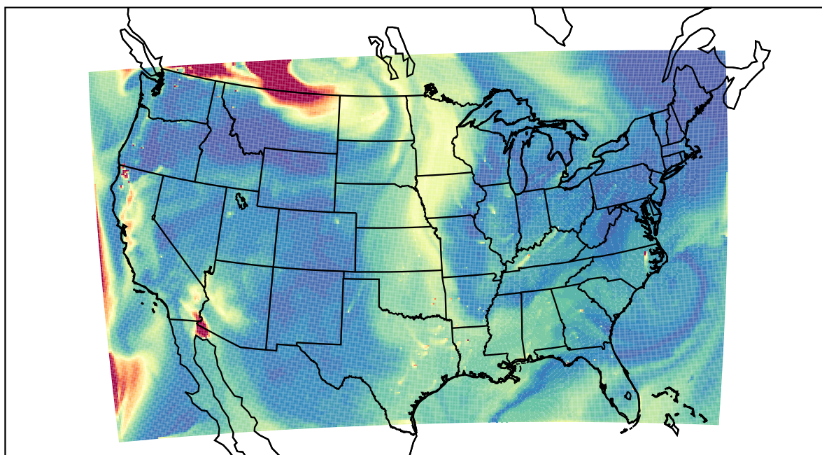
WRF 2023-08-31_20:00:00
