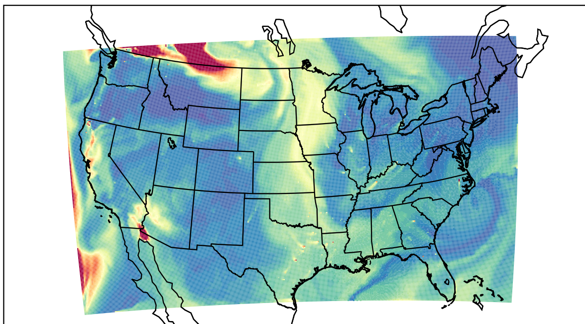
WRF 2023-08-31_19:00:00
