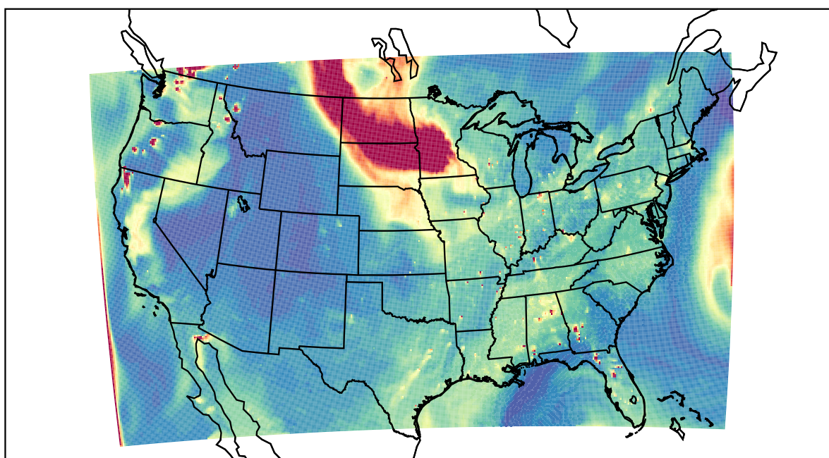
WRF 2023-08-30_00:00:00
