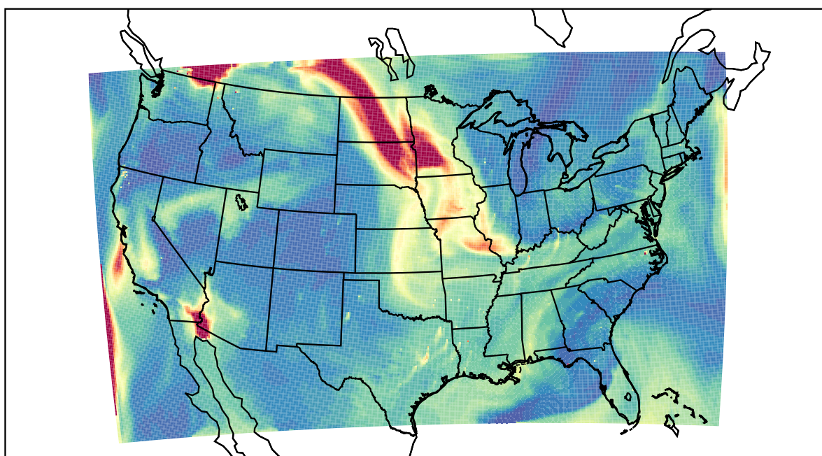
WRF 2023-08-30_19:00:00
