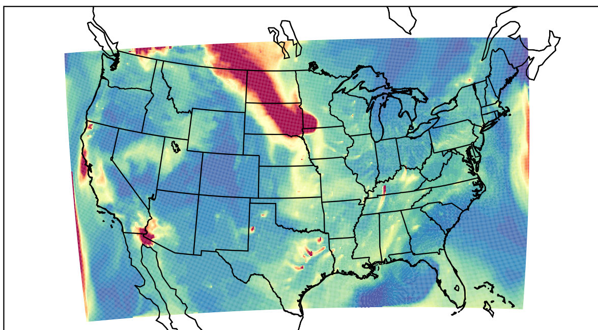
WRF 2023-08-30_13:00:00
