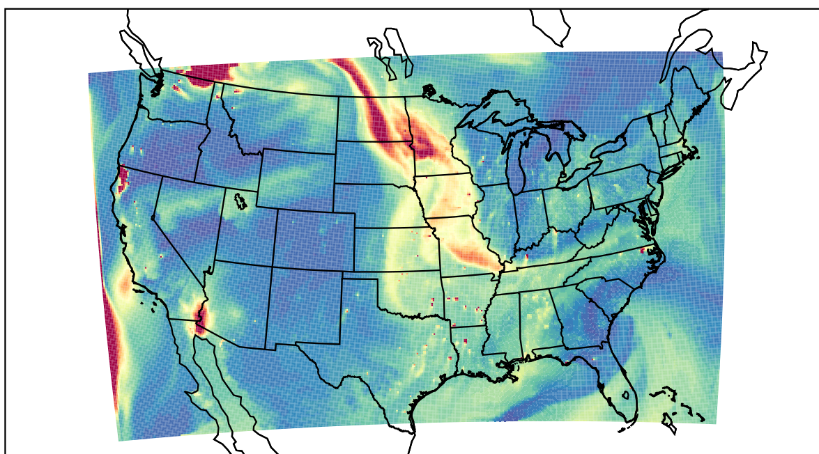
WRF 2023-08-31_00:00:00
