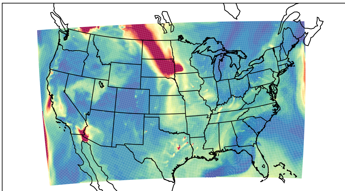
WRF 2023-08-30_16:00:00
