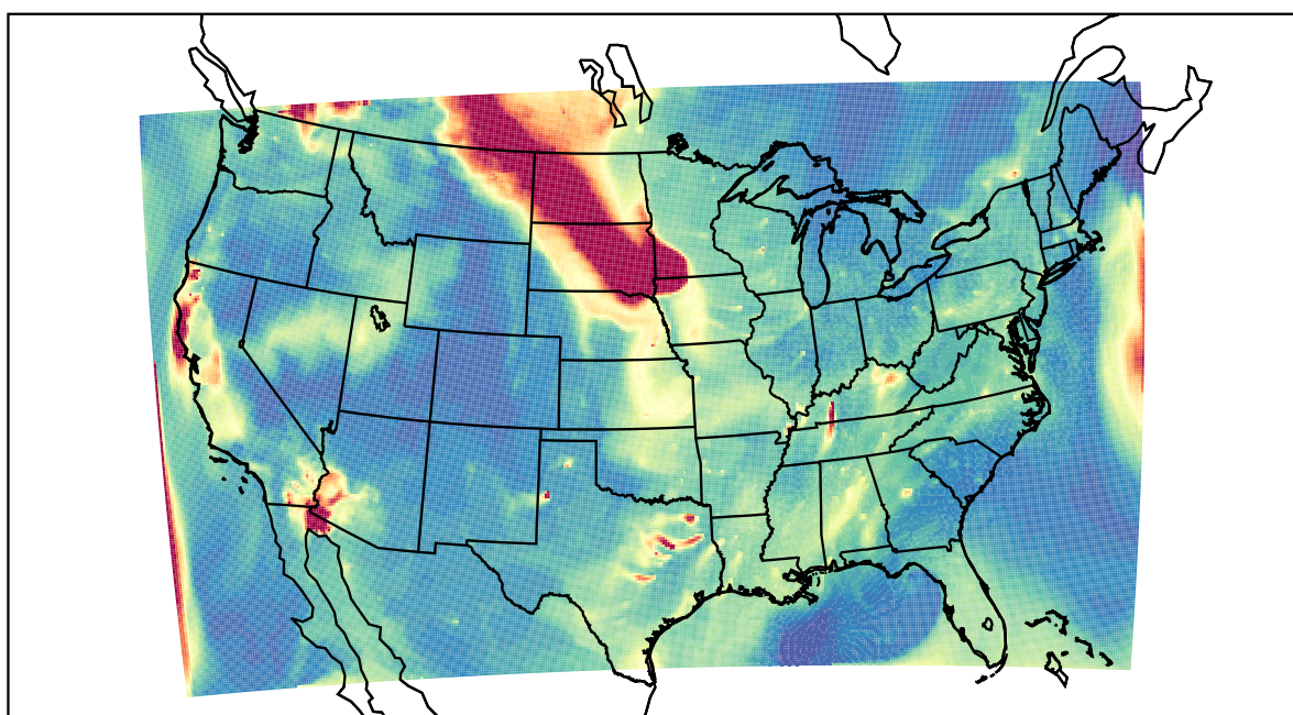
WRF 2023-08-30_11:00:00
