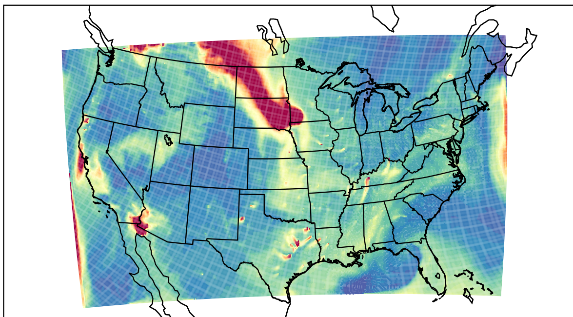
WRF 2023-08-30_14:00:00
