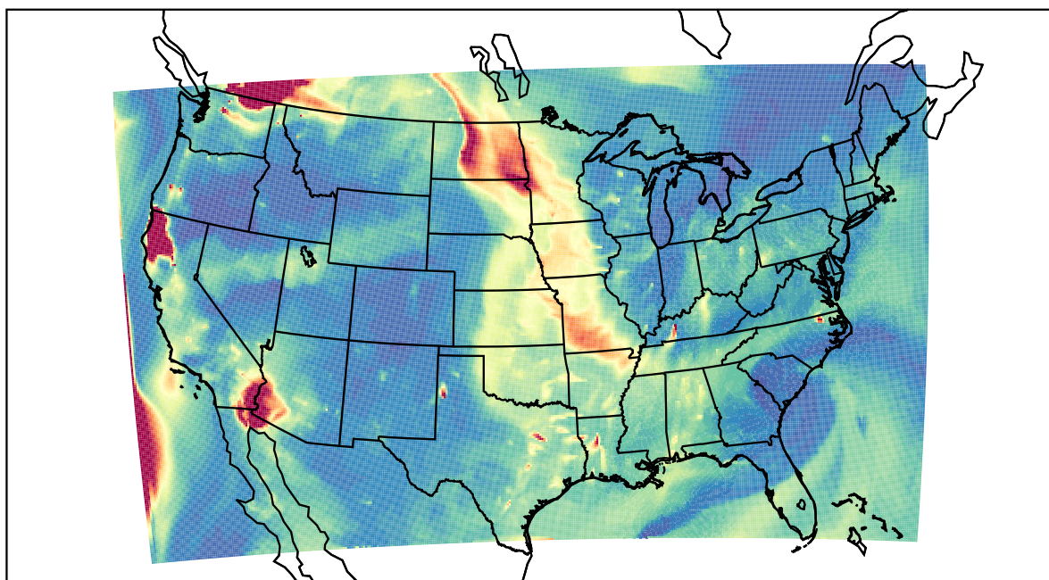
WRF 2023-08-31_04:00:00
