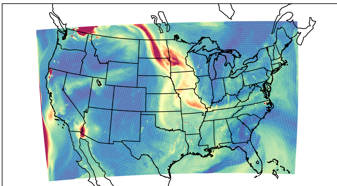
WRF 2023-08-30_23:00:00
