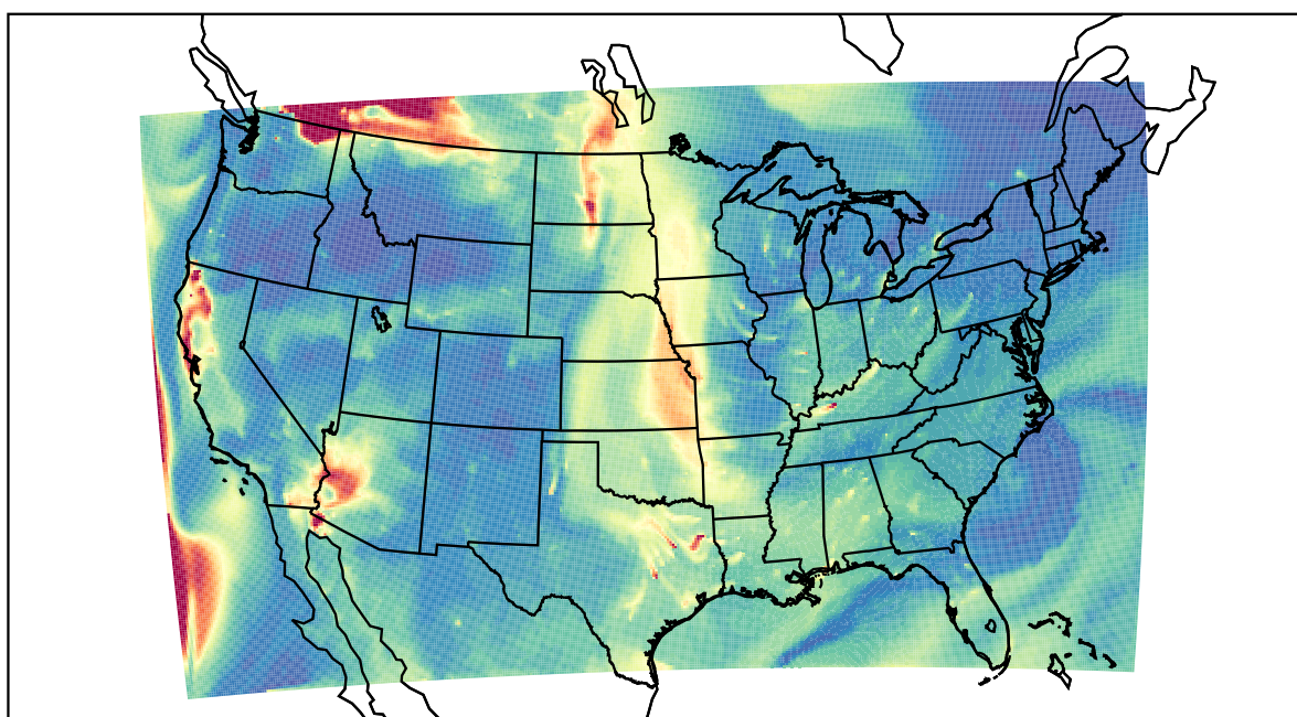
WRF 2023-08-31_13:00:00
