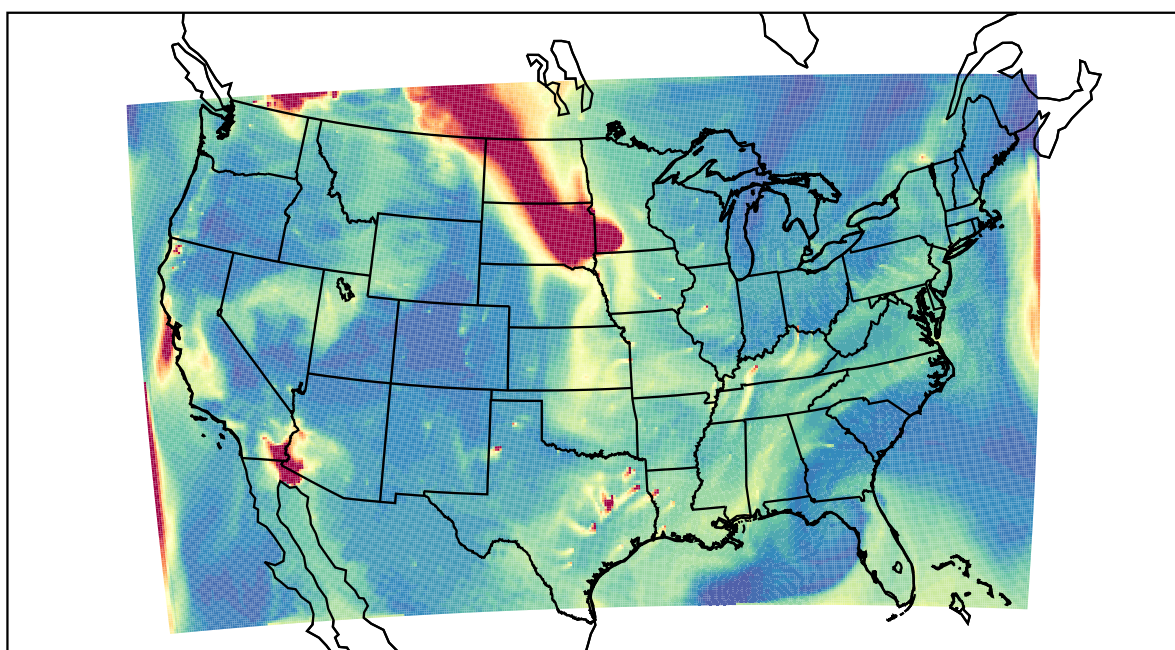
WRF 2023-08-30_15:00:00
