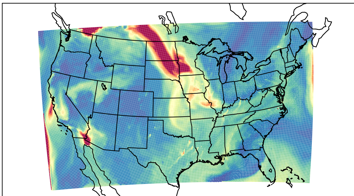
WRF 2023-08-30_18:00:00
