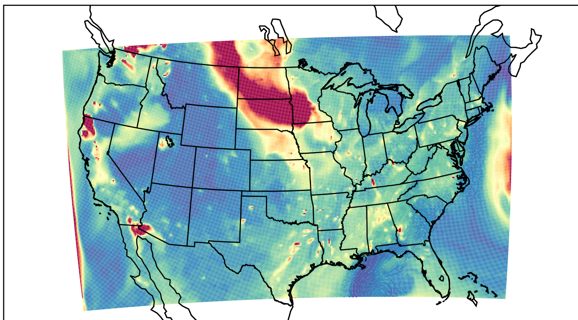
WRF 2023-08-30_03:00:00
