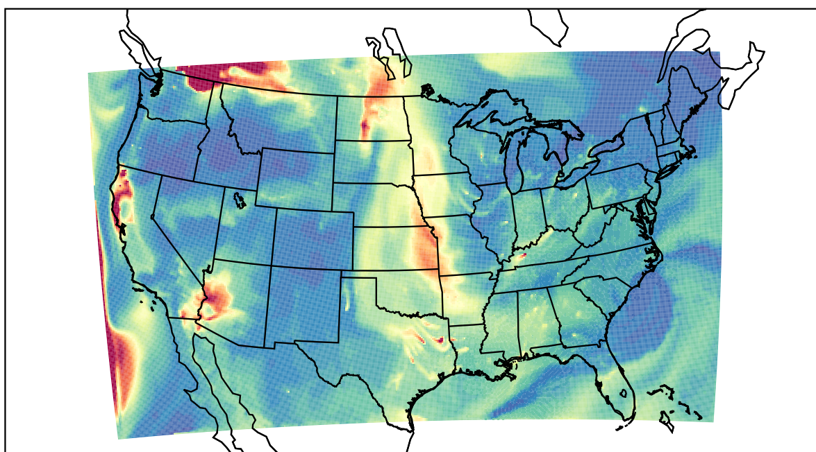
WRF 2023-08-31_11:00:00
