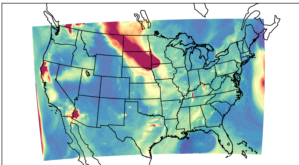
WRF 2023-08-30_08:00:00
