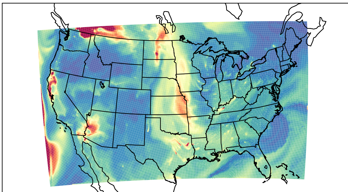
WRF 2023-08-31_12:00:00
