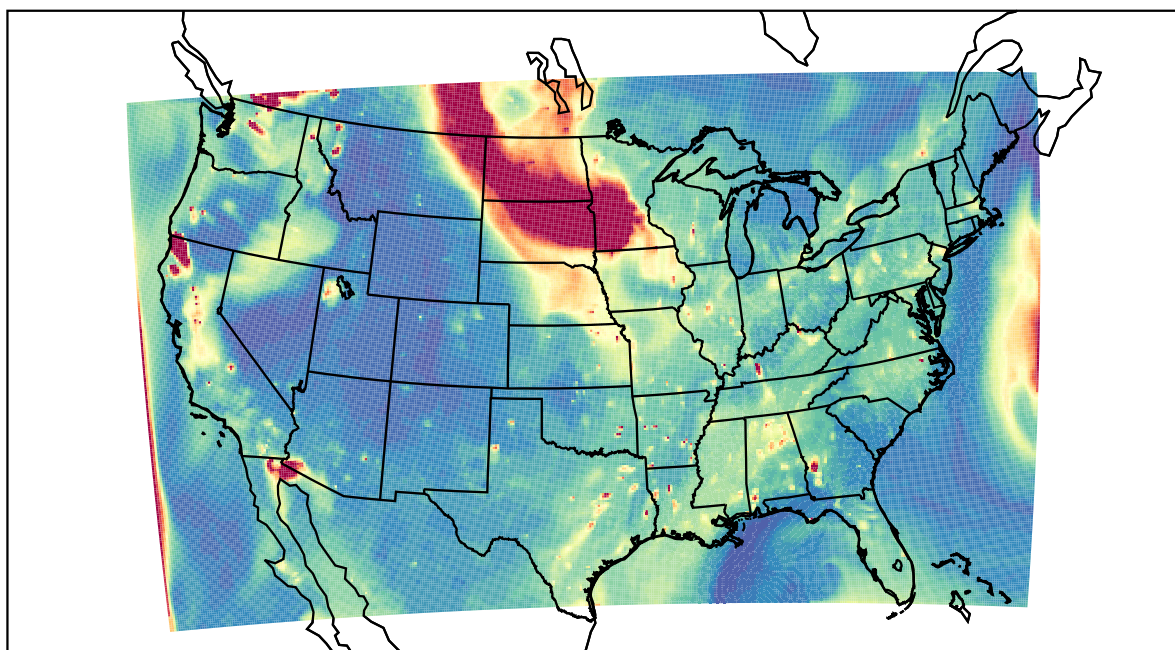
WRF 2023-08-30_02:00:00
