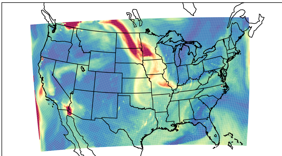
WRF 2023-08-30_20:00:00
