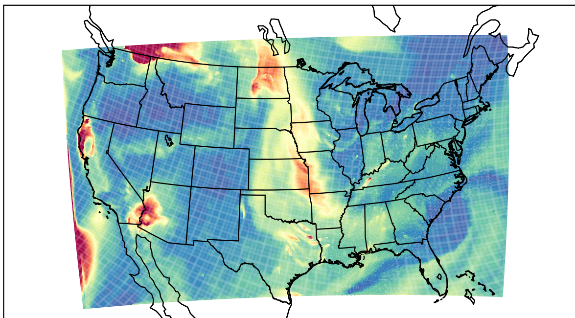
WRF 2023-08-31_09:00:00
