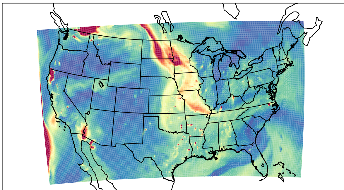
WRF 2023-08-31_01:00:00
