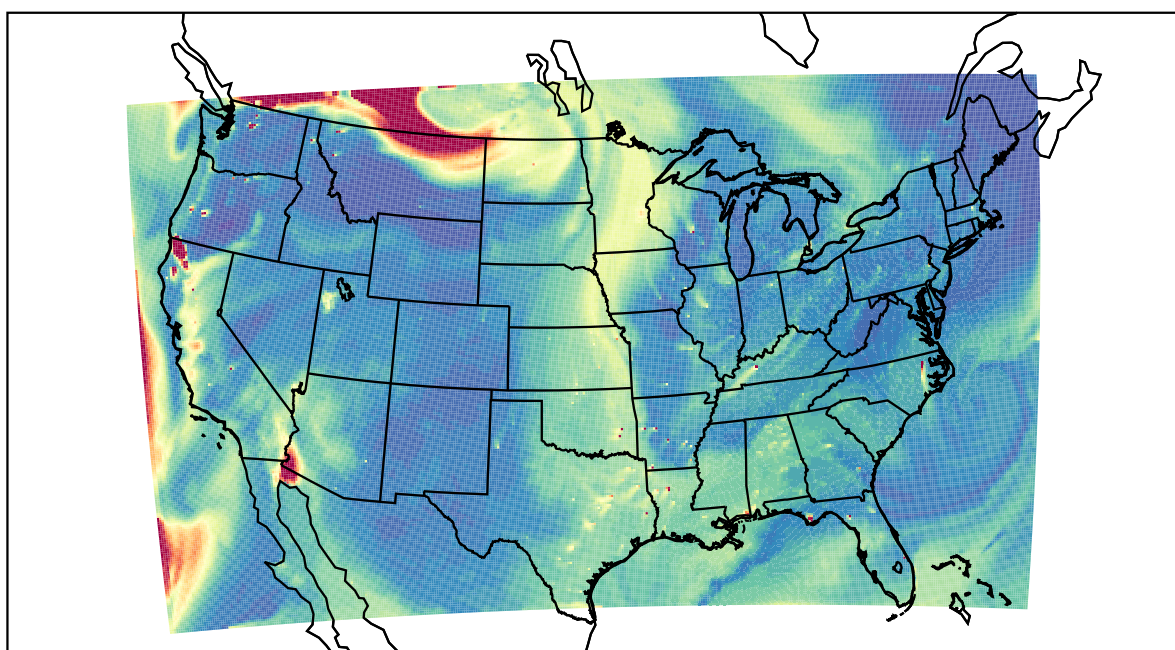
WRF 2023-08-31_23:00:00
