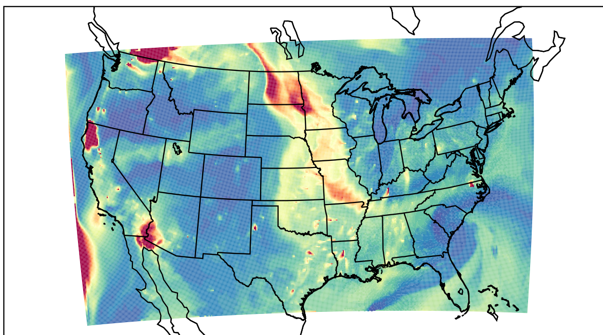
WRF 2023-08-31_03:00:00
