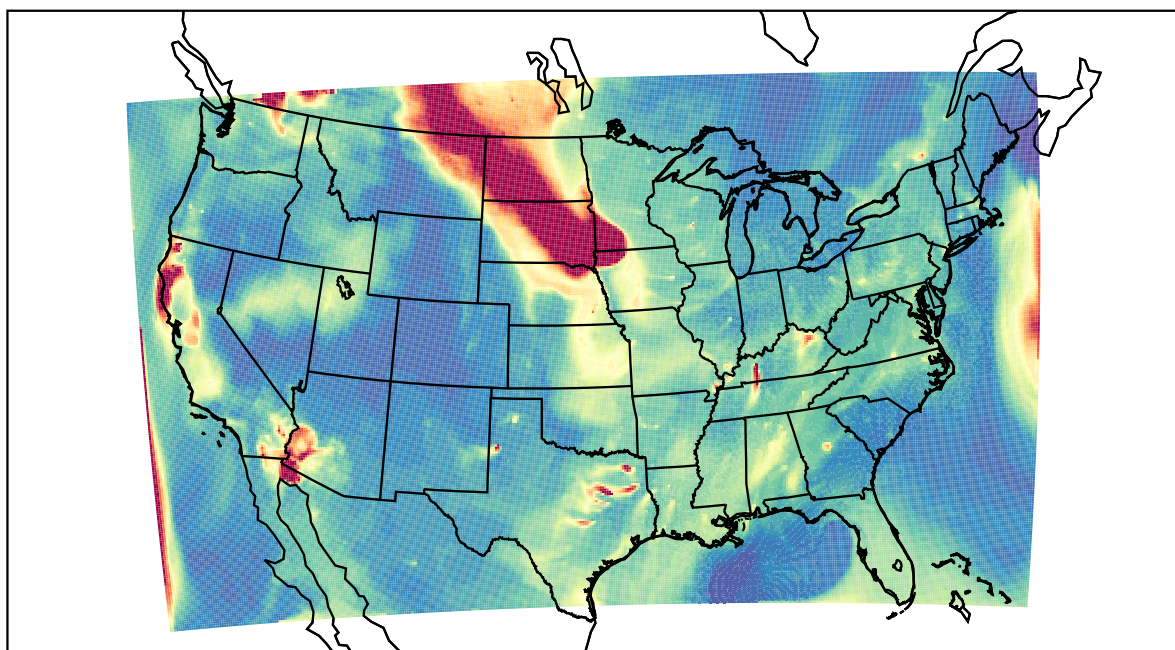
WRF 2023-08-30_10:00:00
