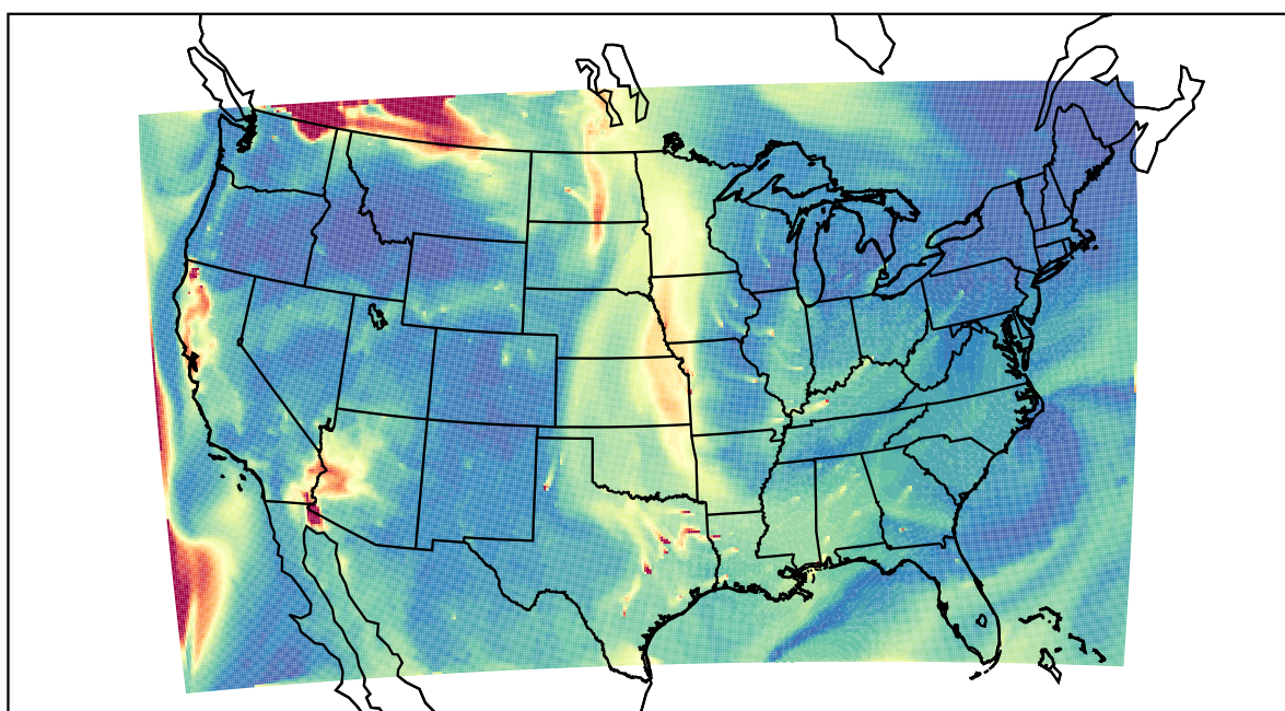
WRF 2023-08-31_15:00:00
