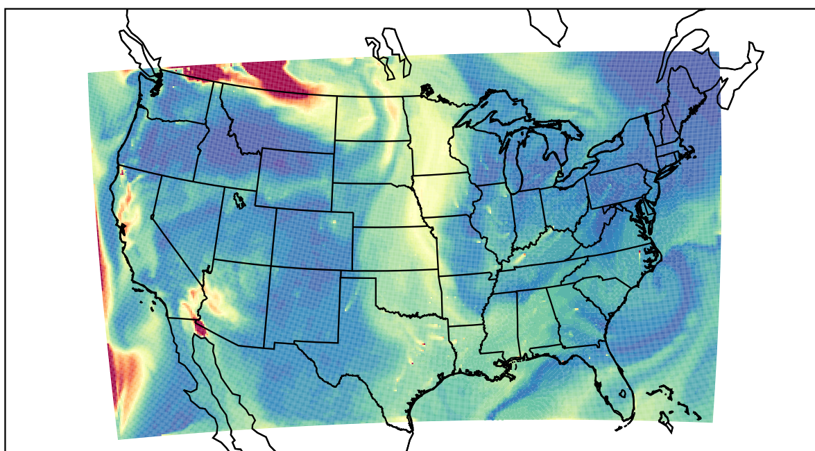
WRF 2023-08-31_18:00:00
