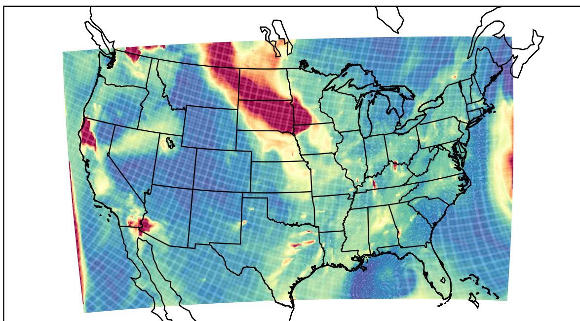
WRF 2023-08-30_06:00:00
