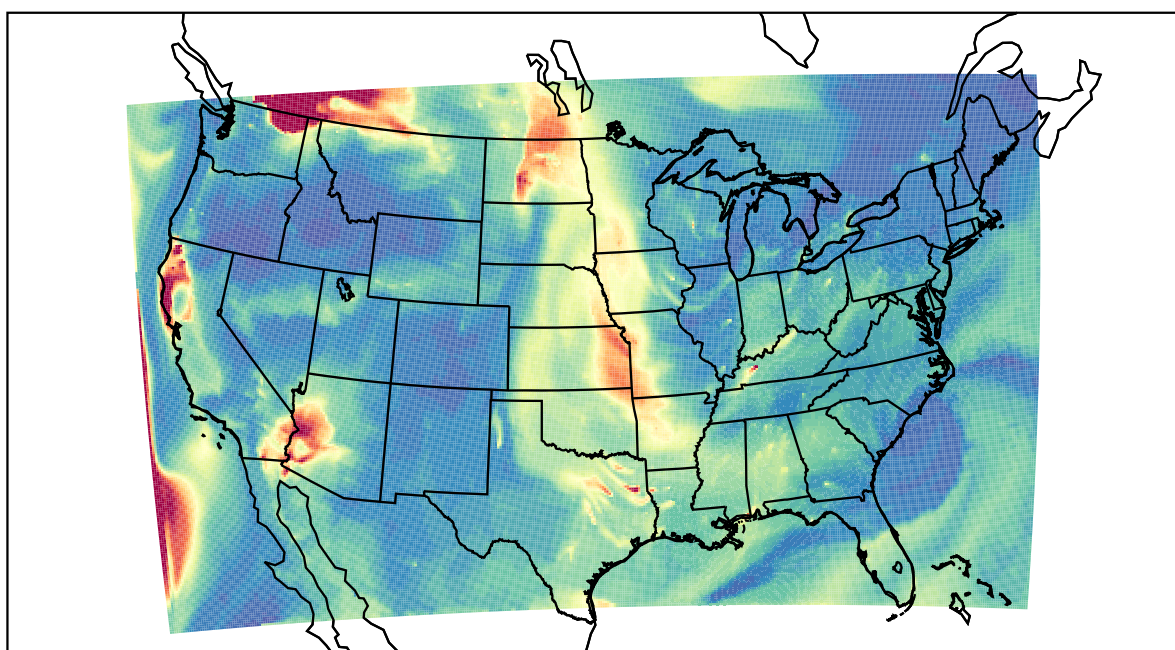
WRF 2023-08-31_10:00:00
