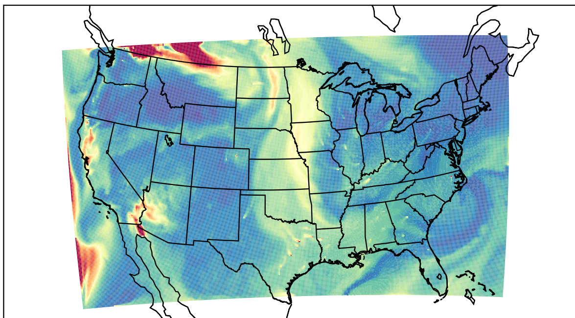
WRF 2023-08-31_17:00:00
