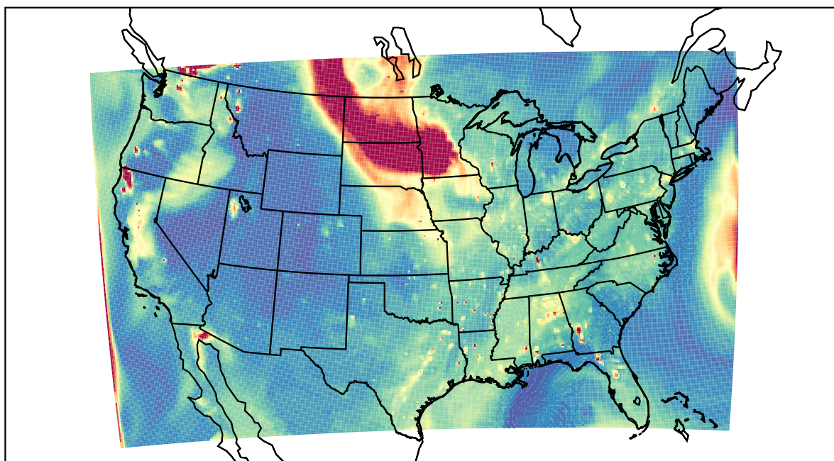
WRF 2023-08-30_01:00:00
