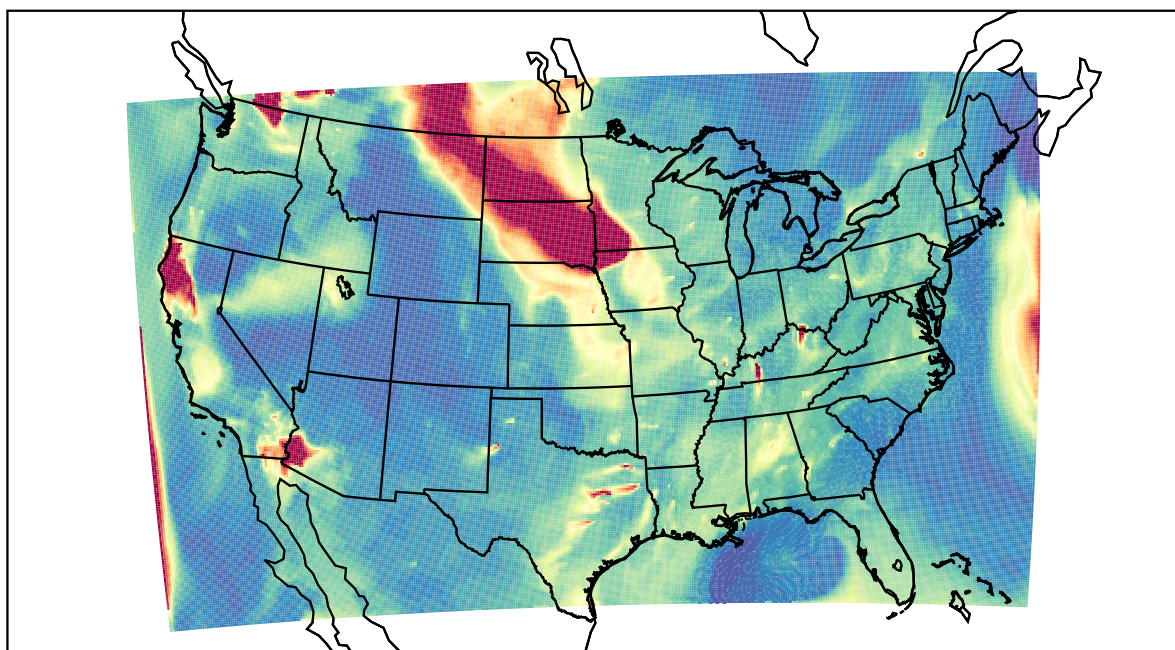
WRF 2023-08-30_07:00:00
