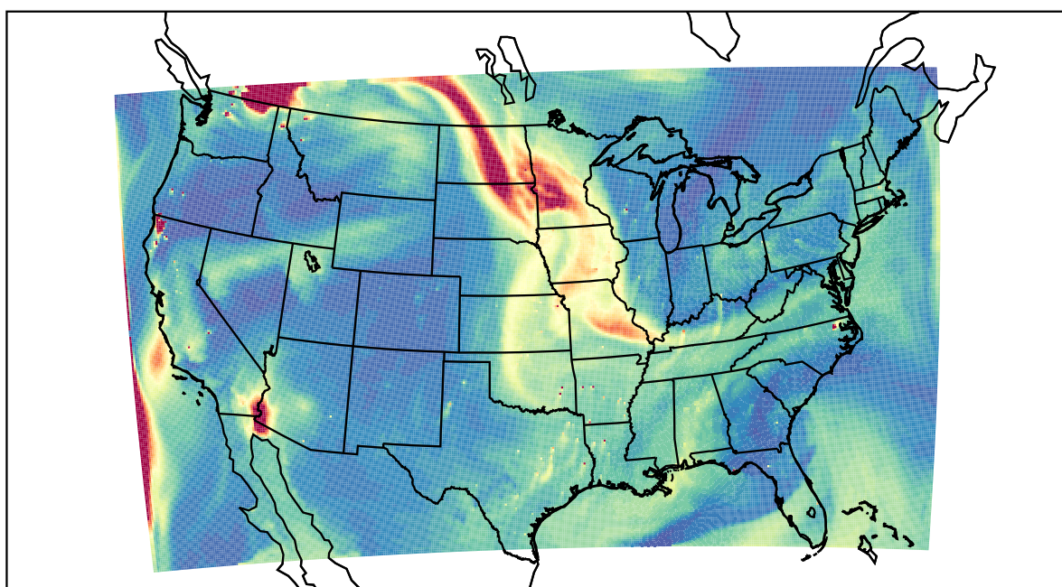
WRF 2023-08-30_22:00:00
