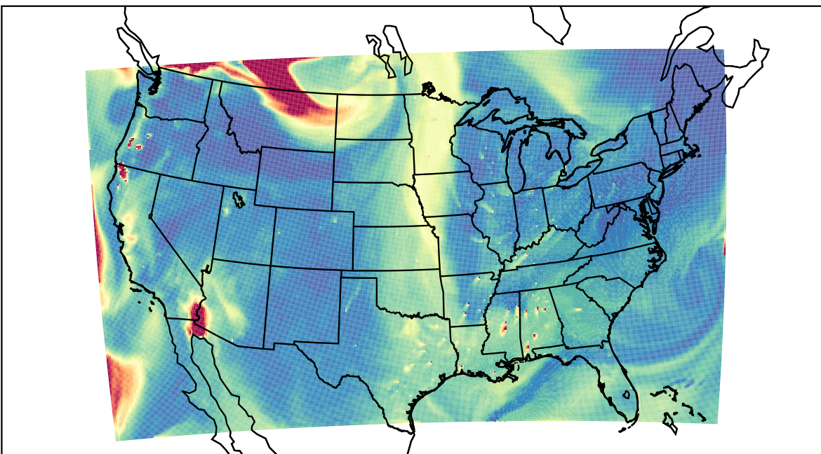
WRF 2023-08-31_22:00:00
