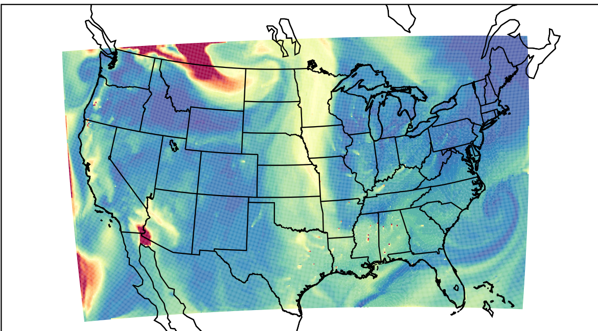
WRF 2023-08-31_19:00:00
