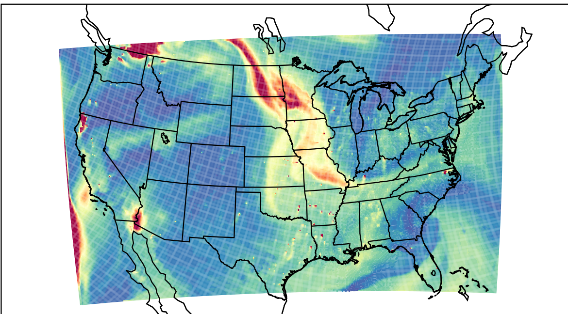
WRF 2023-08-31_00:00:00
