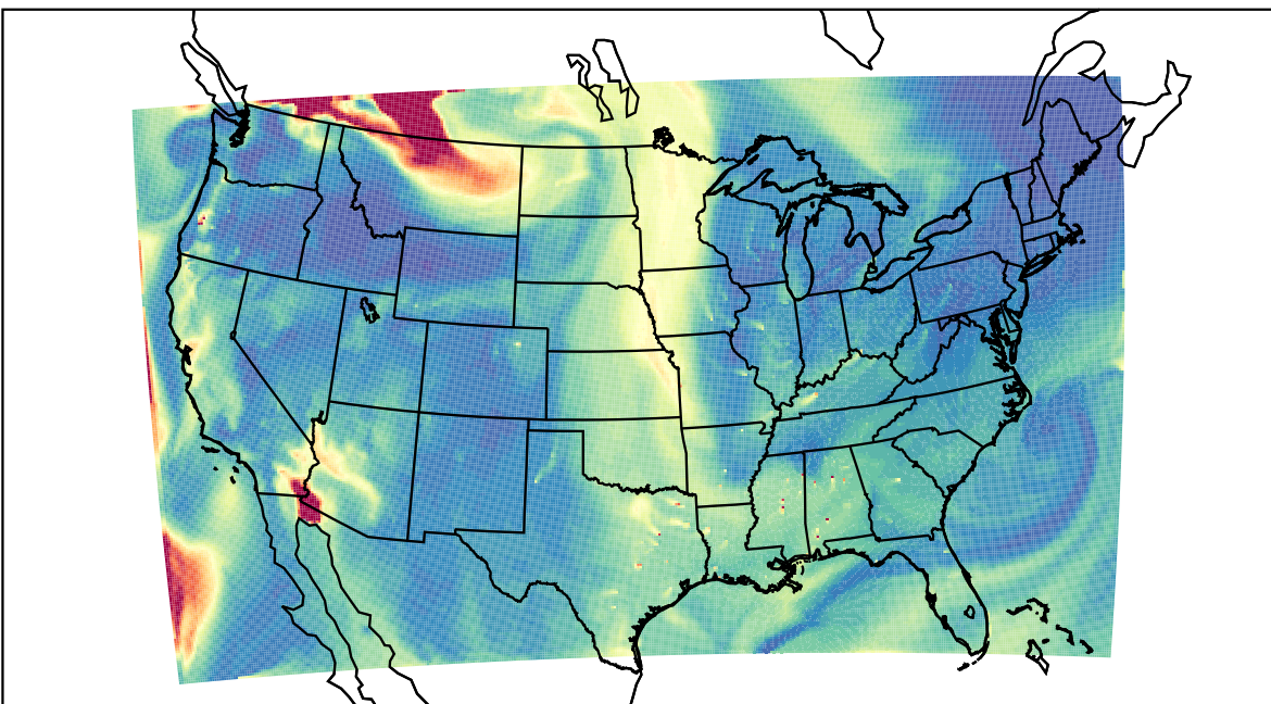
WRF 2023-08-31_18:00:00
