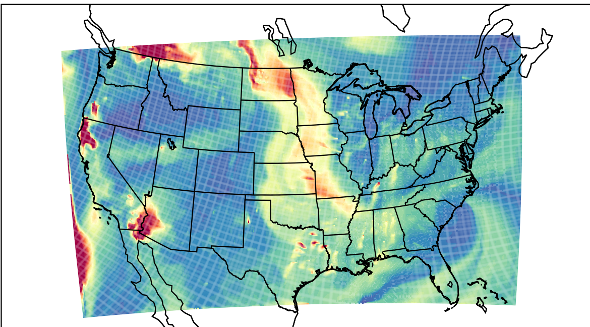
WRF 2023-08-31_06:00:00
