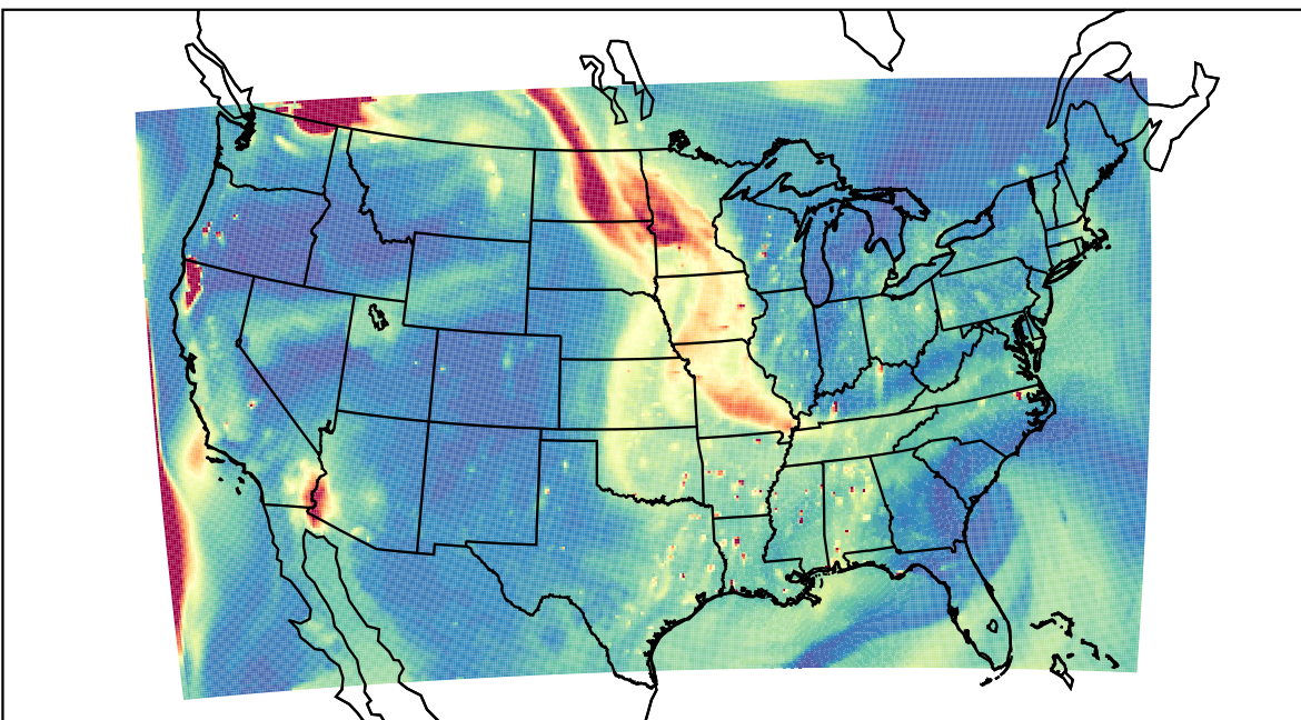
WRF 2023-08-31_01:00:00
