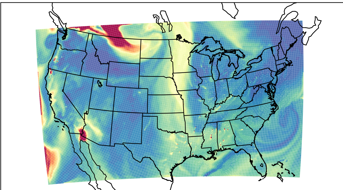
WRF 2023-08-31_20:00:00
