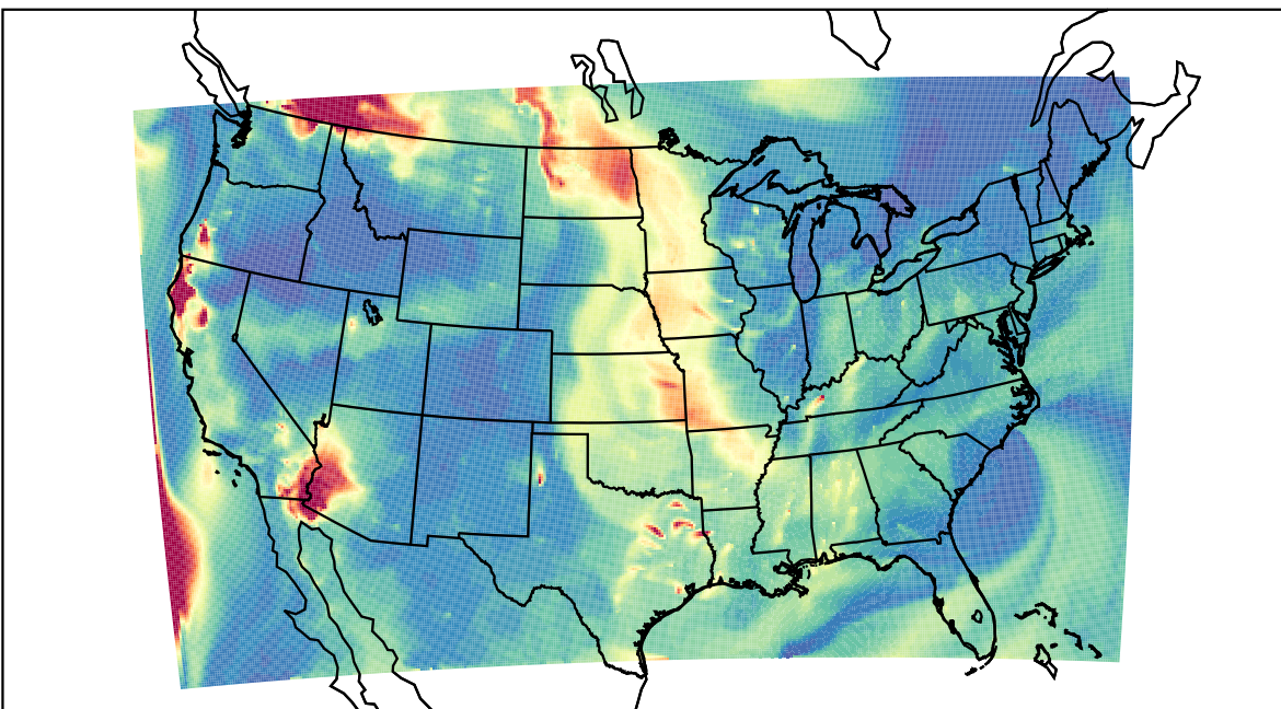
WRF 2023-08-31_07:00:00
