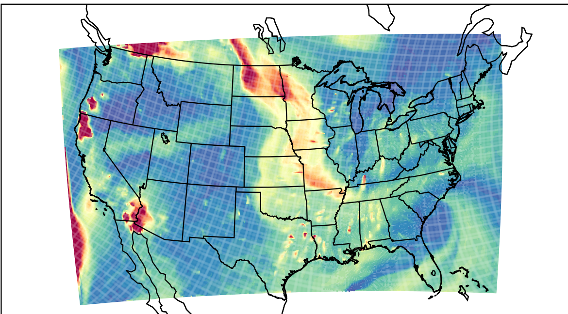
WRF 2023-08-31_04:00:00
