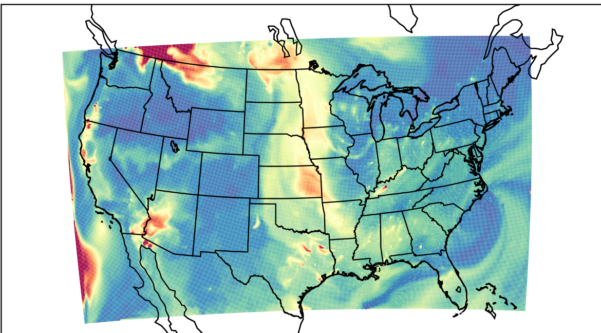
WRF 2023-08-31_11:00:00
