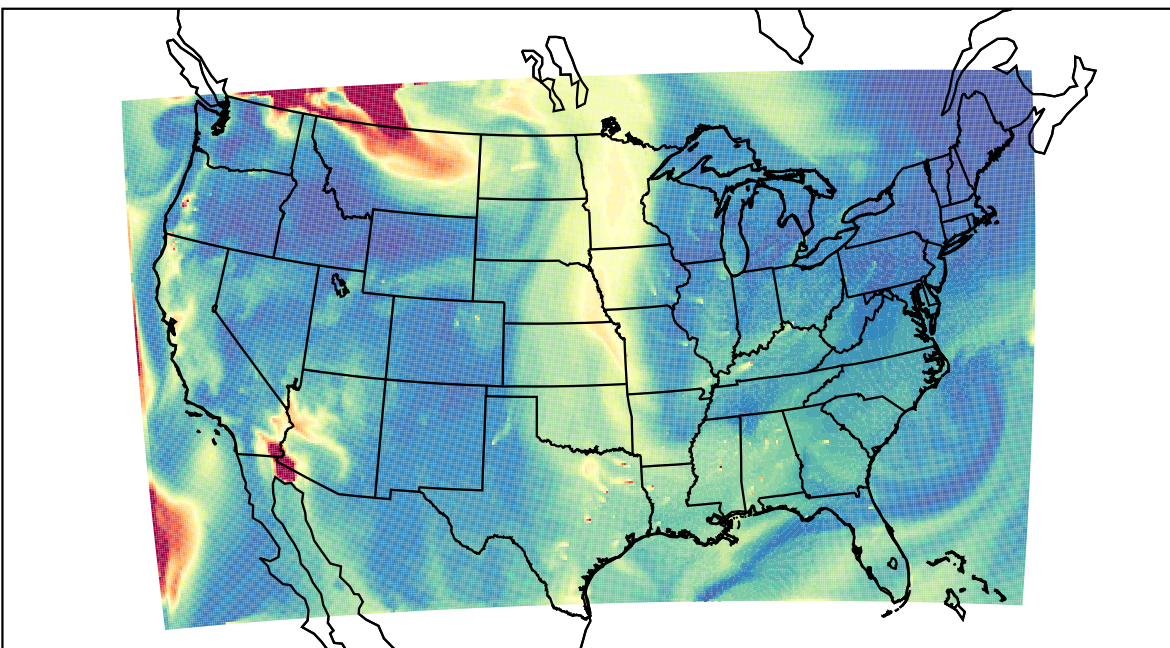
WRF 2023-08-31_17:00:00
