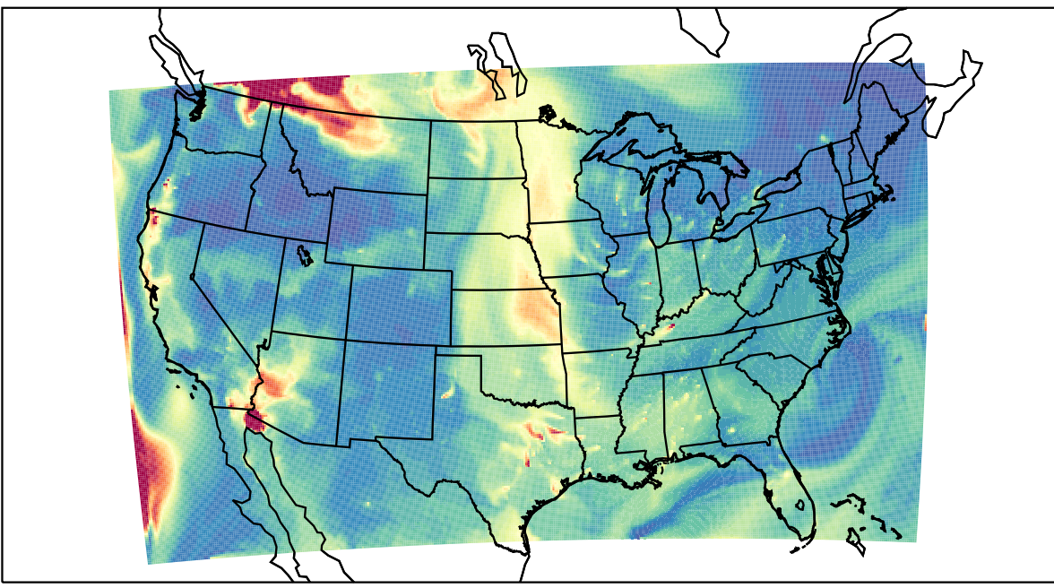
WRF 2023-08-31_13:00:00
