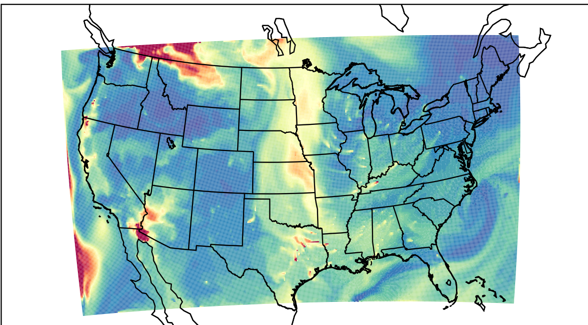
WRF 2023-08-31_14:00:00
