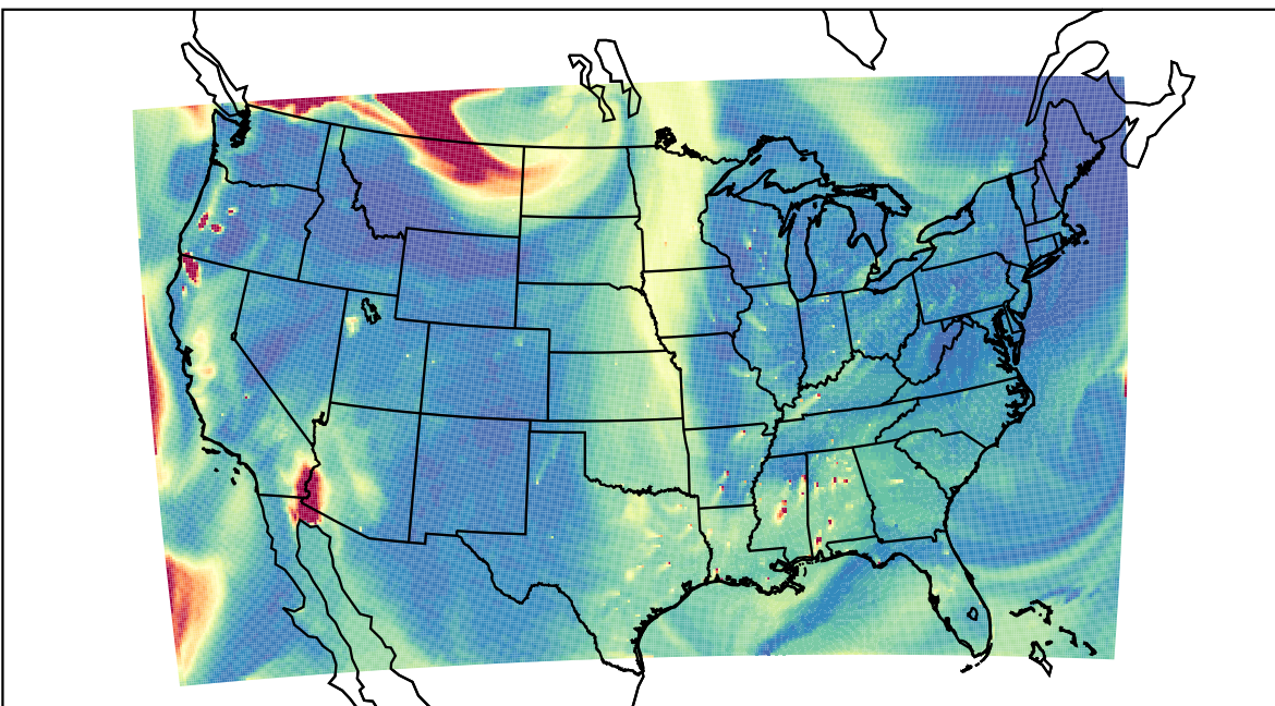
WRF 2023-08-31_23:00:00
