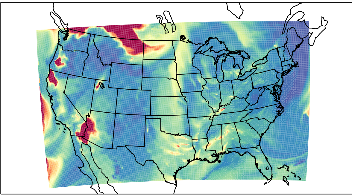
WRF 2023-09-01_06:00:00
