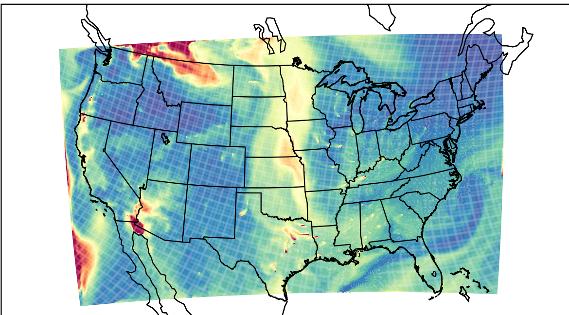
WRF 2023-08-31_15:00:00
