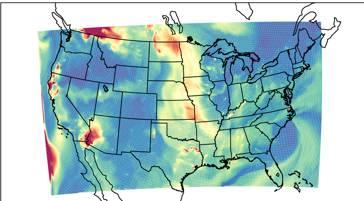
WRF 2023-08-31_08:00:00
