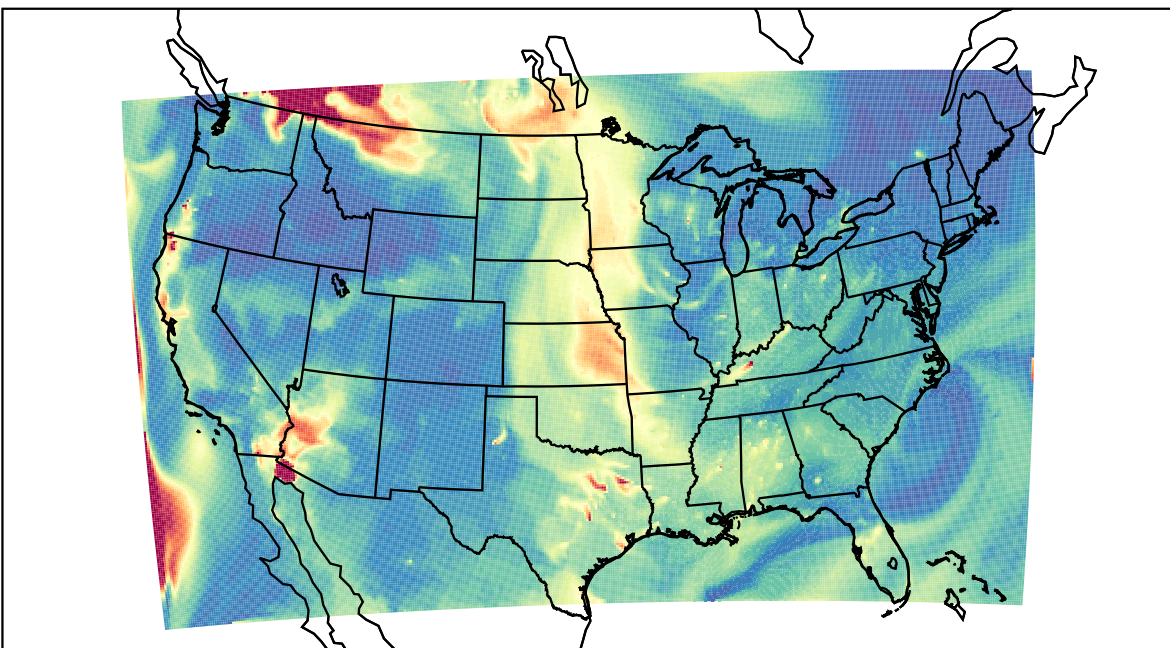
WRF 2023-08-31_12:00:00
