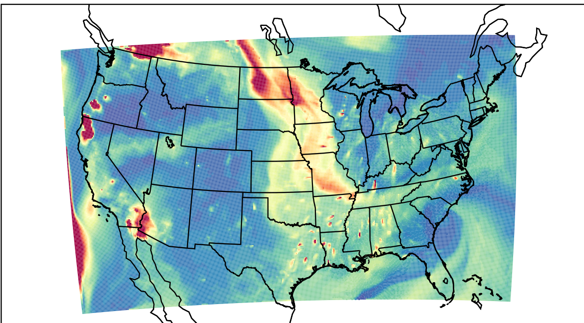
WRF 2023-08-31_03:00:00
