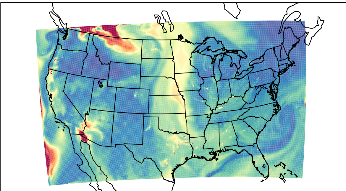
WRF 2023-08-31_16:00:00
