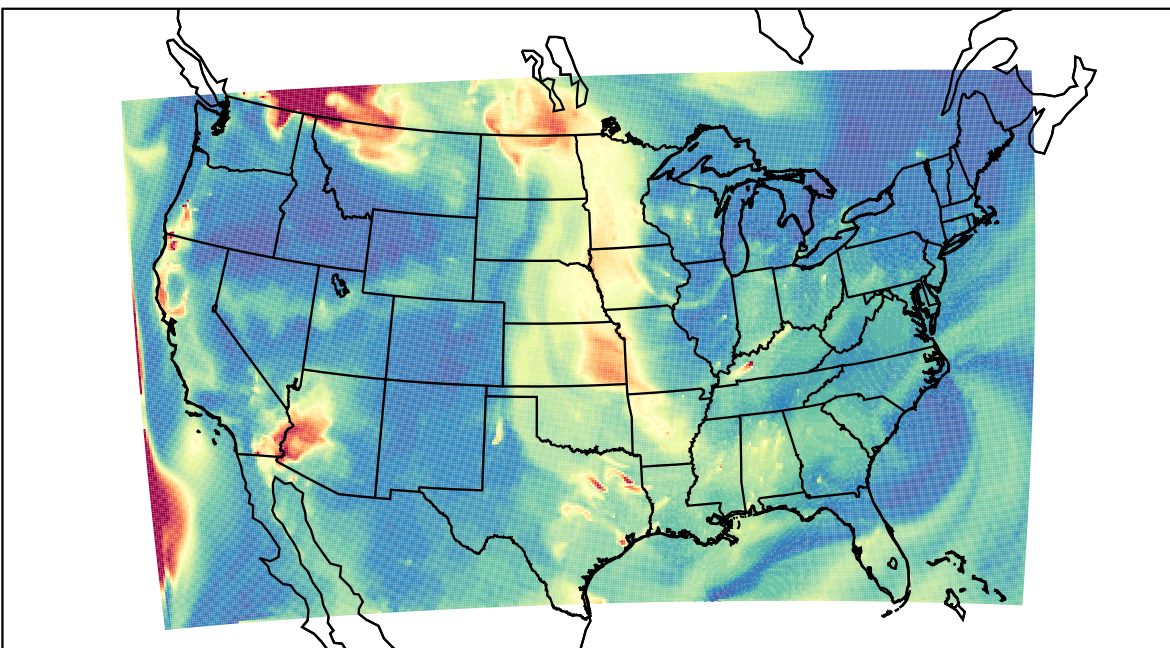
WRF 2023-08-31_10:00:00
