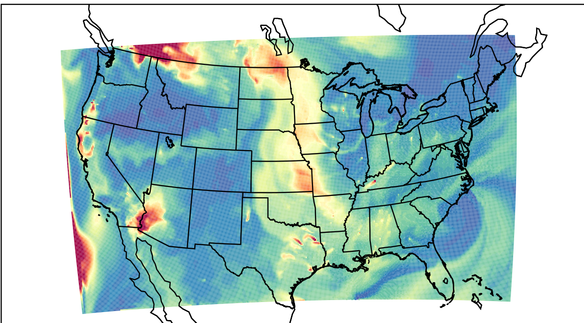
WRF 2023-08-31_09:00:00
