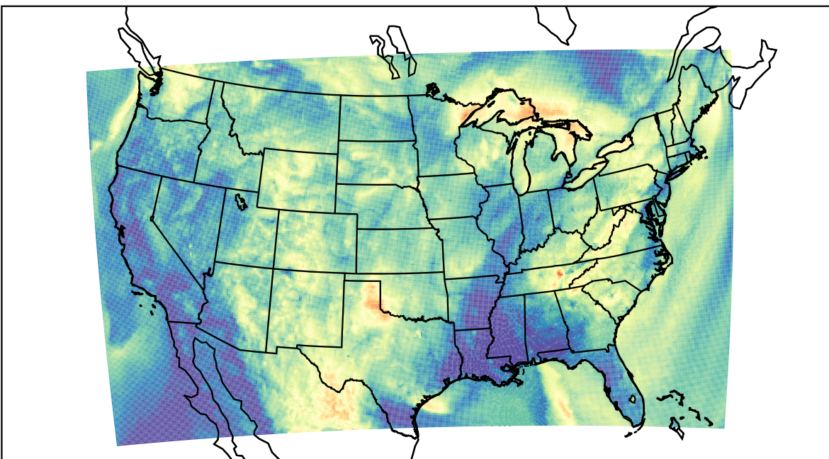
WRF (2023-09-03_10:00:00)
