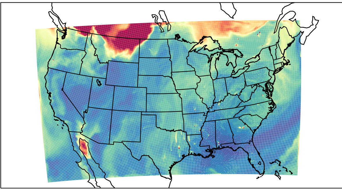
WRF 2023-09-04_20:00:00
