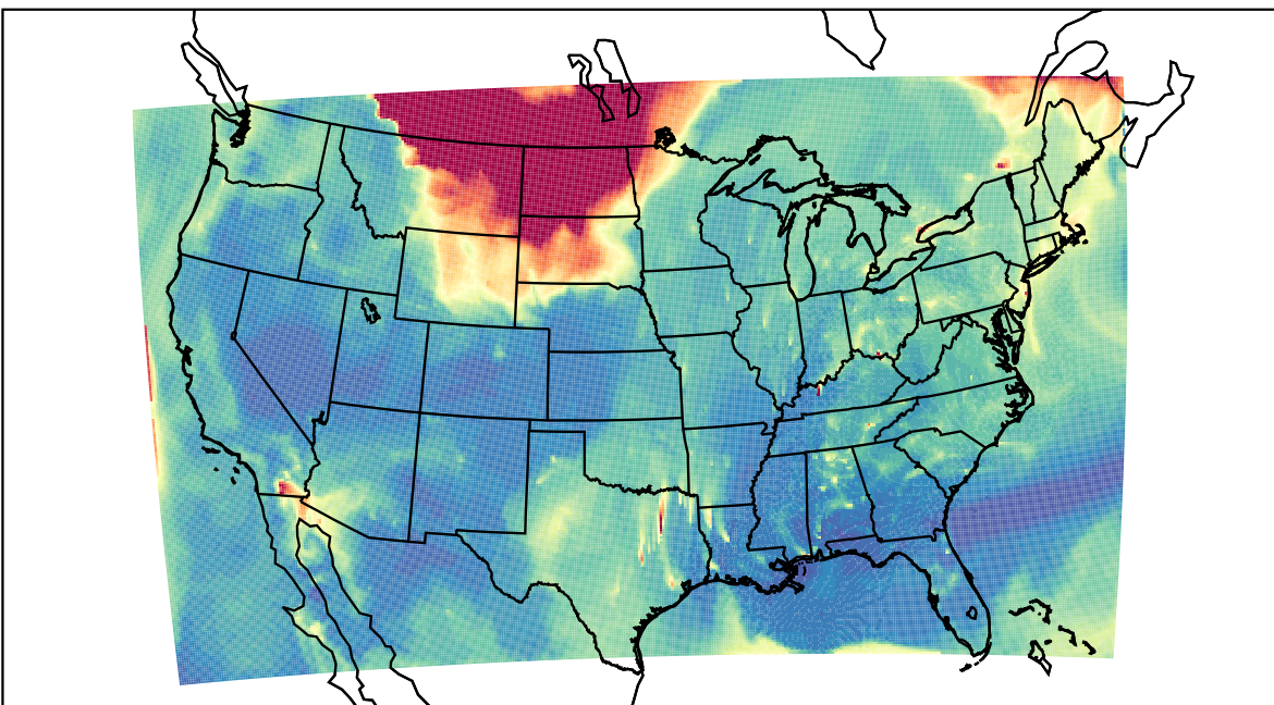
WRF 2023-09-05_13:00:00
