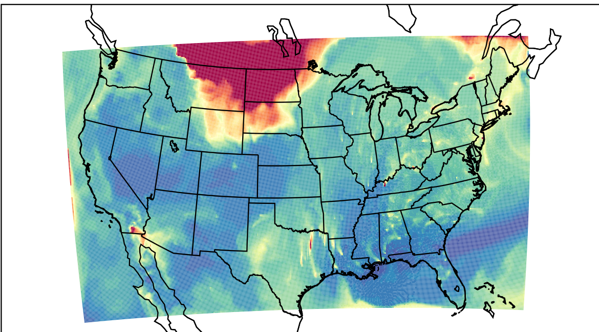
WRF 2023-09-05_12:00:00
