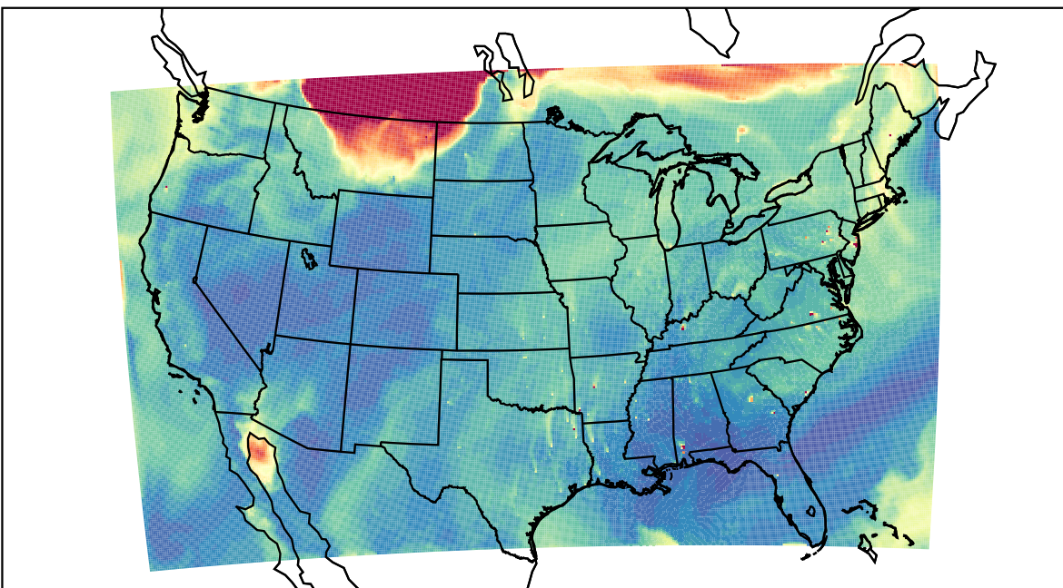
WRF 2023-09-04_22:00:00
