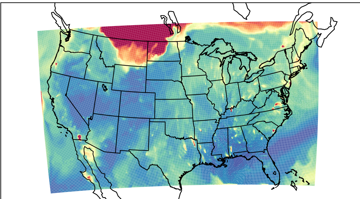
WRF 2023-09-05_03:00:00
