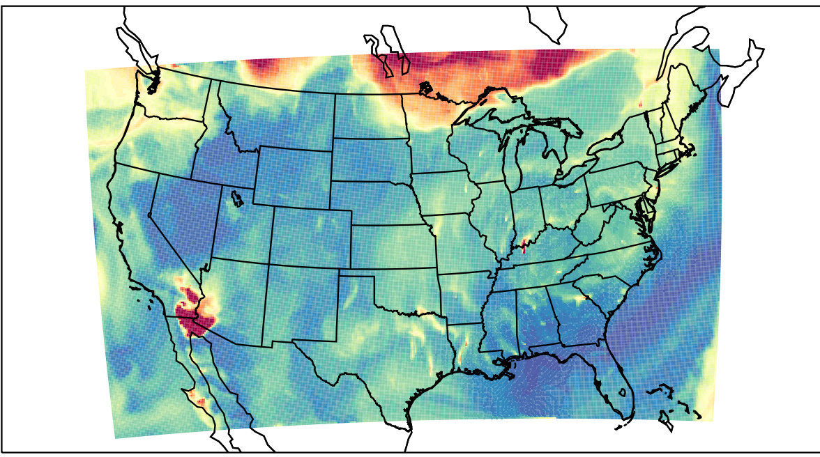
WRF 2023-09-04_08:00:00
