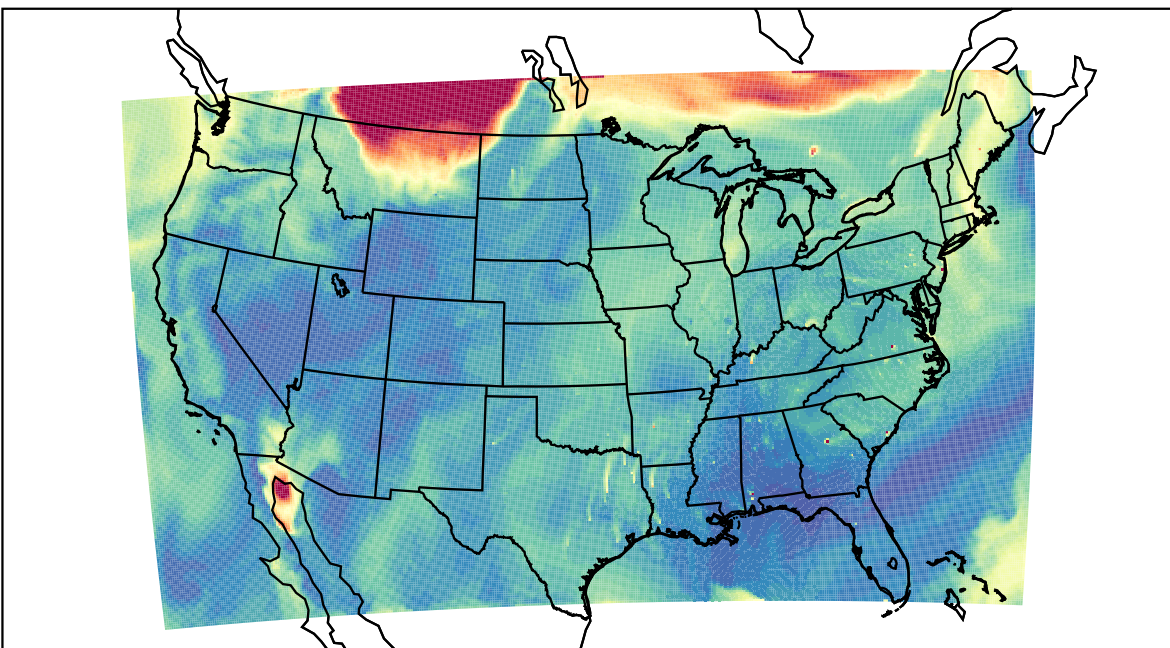
WRF 2023-09-04_19:00:00
