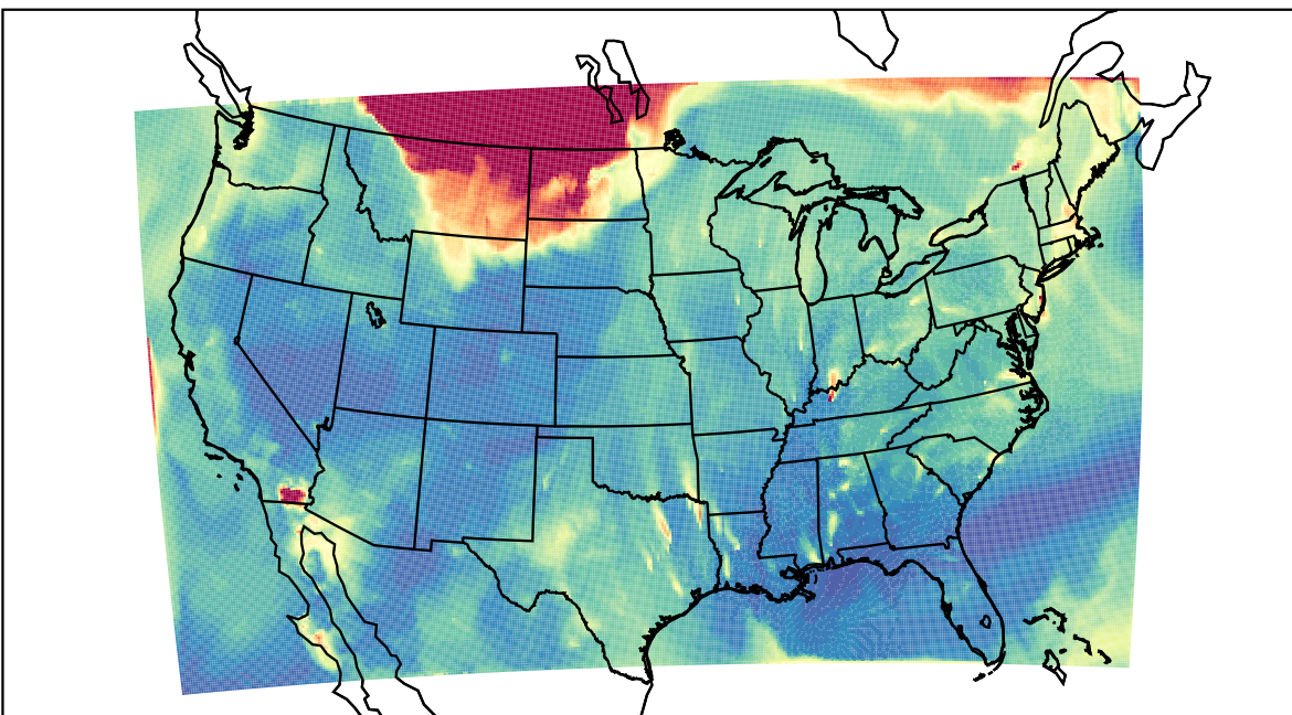
WRF 2023-09-05_06:00:00
