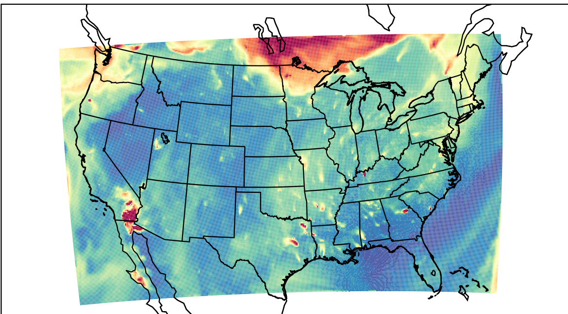
WRF 2023-09-04_03:00:00
