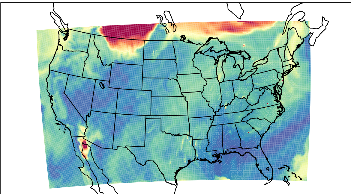
WRF 2023-09-04_18:00:00
