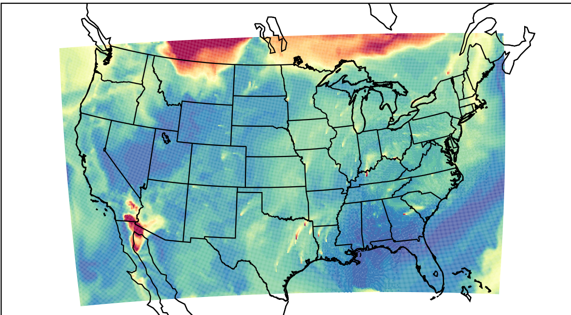
WRF 2023-09-04_15:00:00
