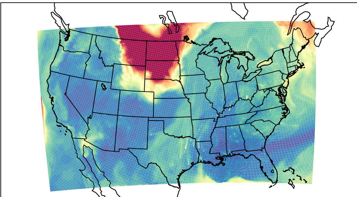
WRF 2023-09-05_18:00:00
