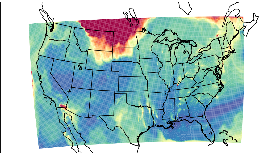
WRF 2023-09-05_09:00:00
