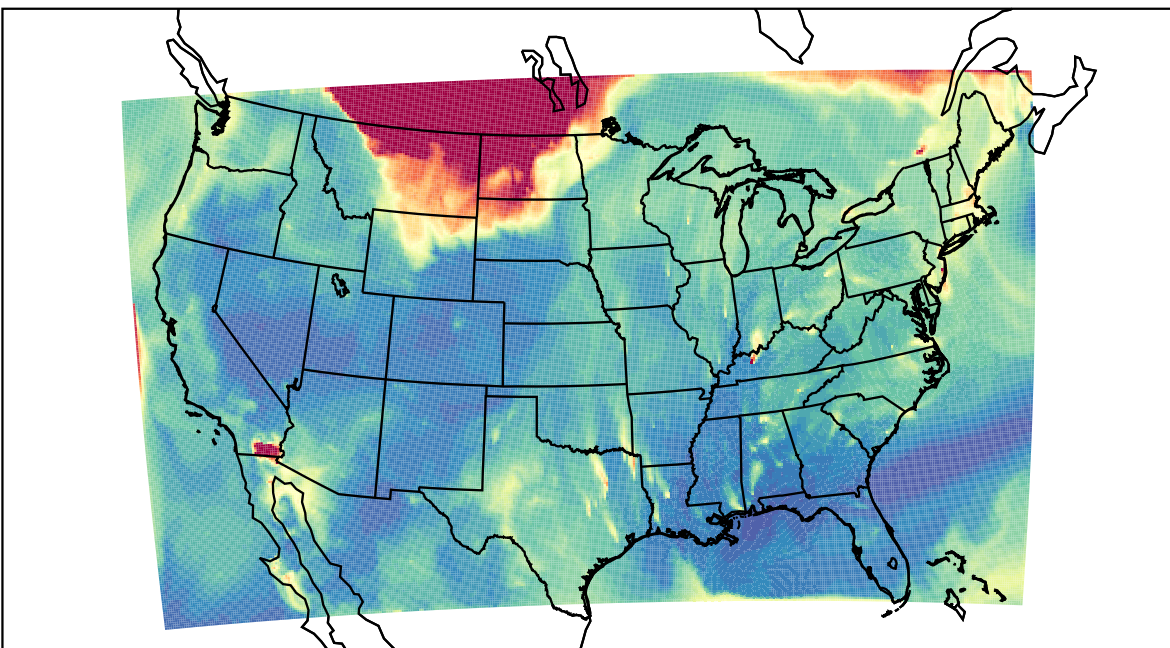
WRF 2023-09-05_07:00:00
