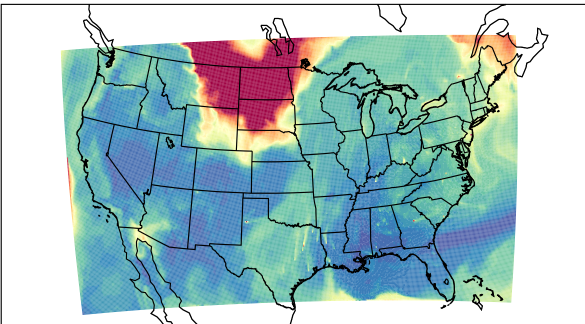
WRF 2023-09-05_17:00:00
