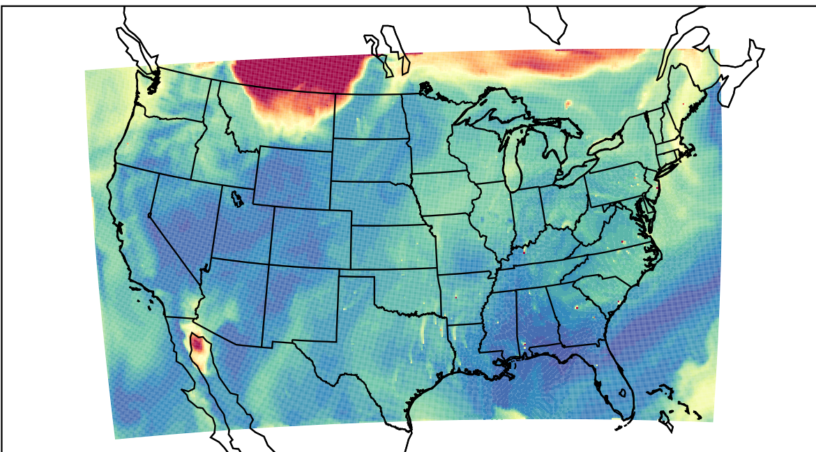
WRF 2023-09-04_20:00:00
