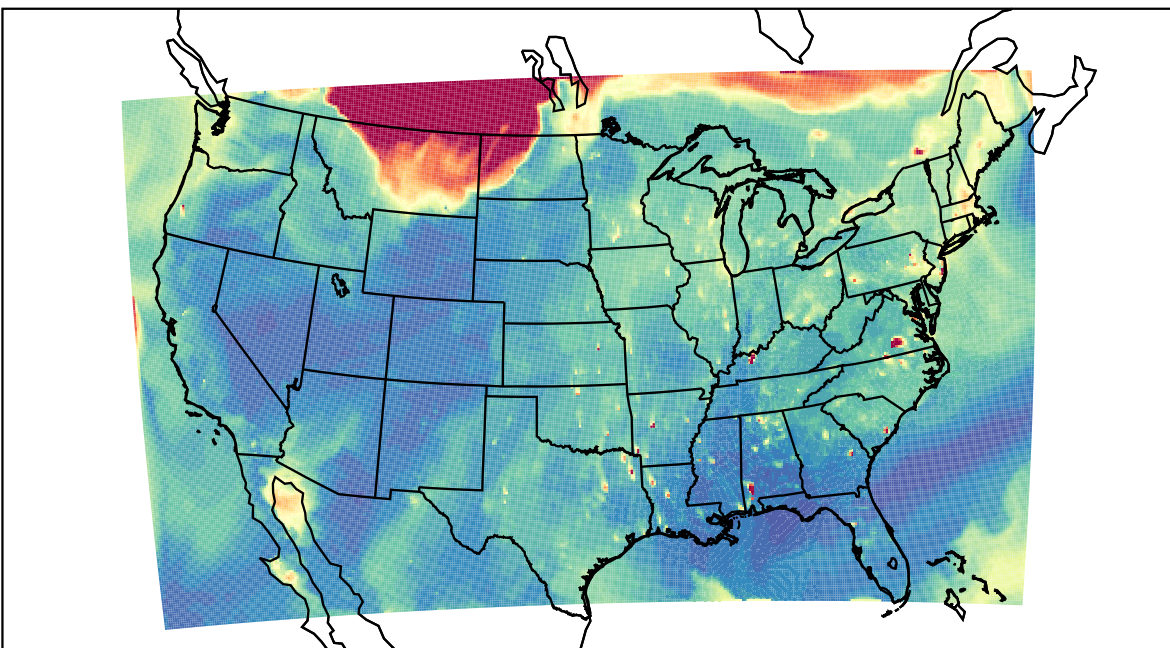
WRF 2023-09-05_01:00:00
