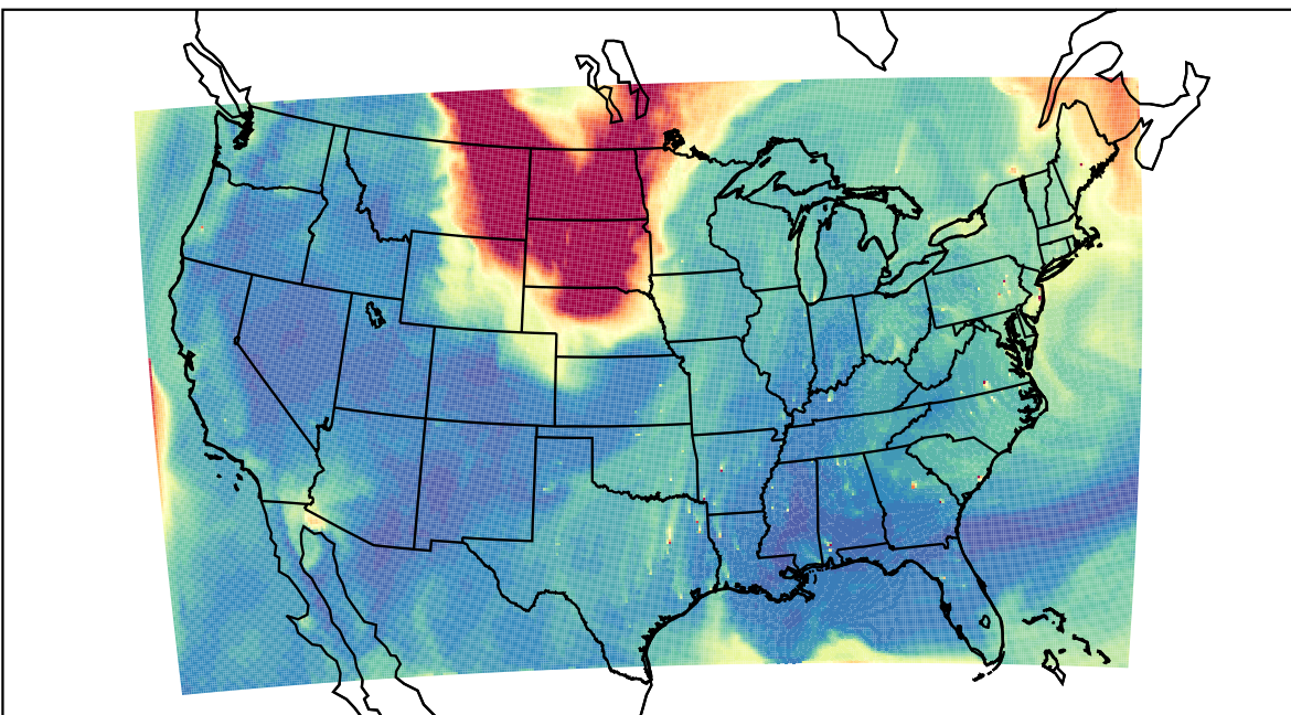
WRF 2023-09-05_21:00:00
