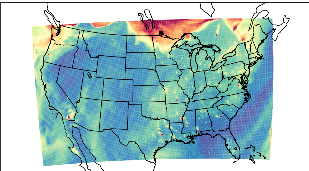
WRF 2023-09-04_00:00:00
