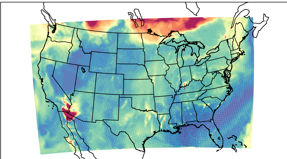
WRF 2023-09-04_10:00:00
