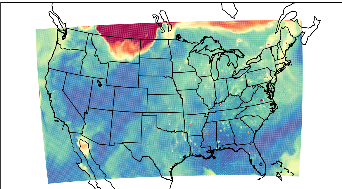
WRF 2023-09-05_00:00:00
