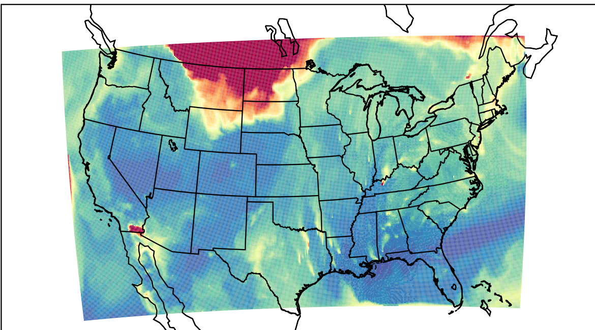
WRF 2023-09-05_08:00:00
