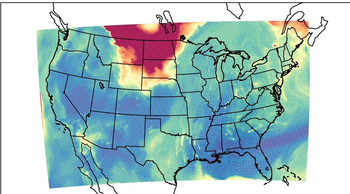
WRF 2023-09-05_15:00:00
