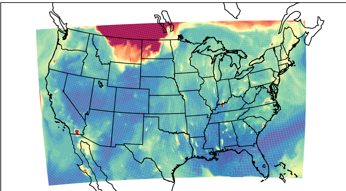
WRF 2023-09-05_04:00:00
