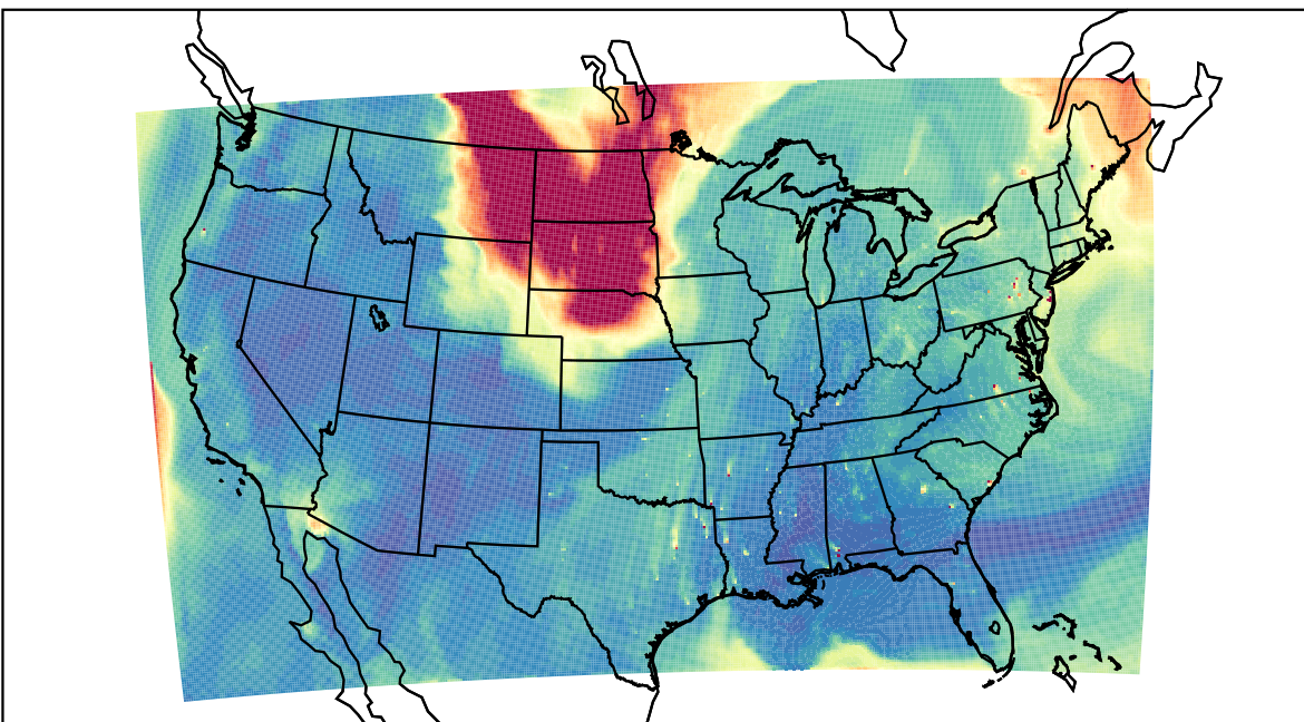
WRF 2023-09-05_22:00:00
