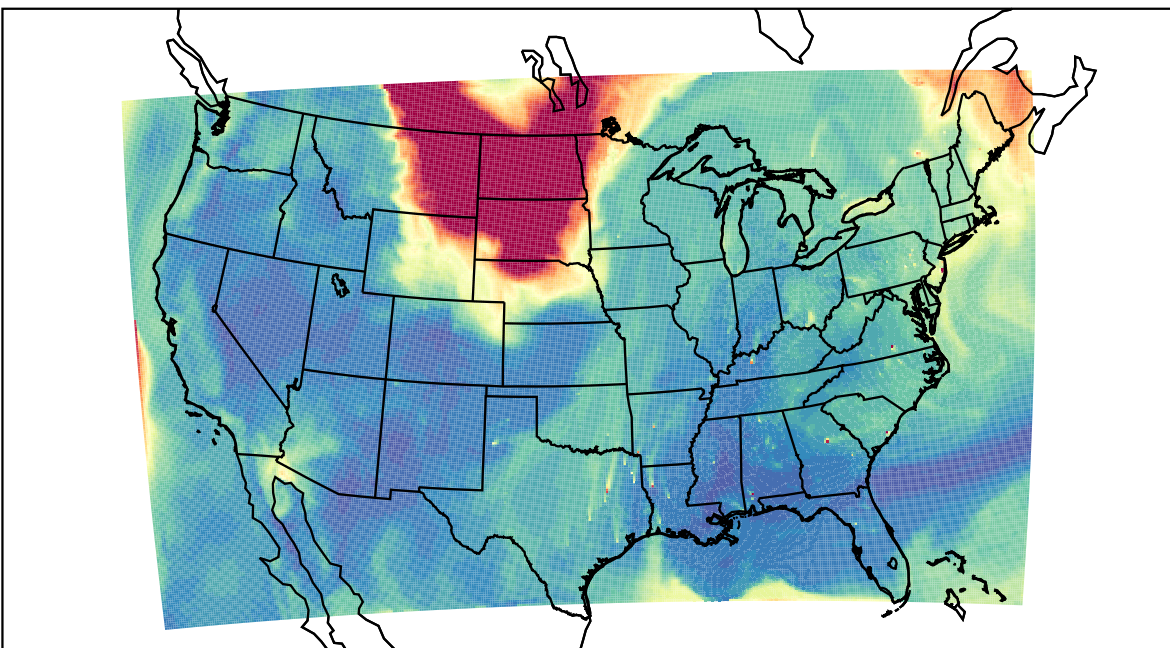
WRF 2023-09-05_19:00:00
