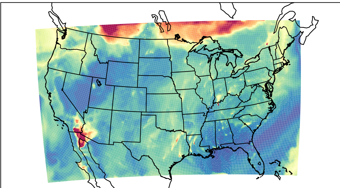
WRF 2023-09-04_13:00:00
