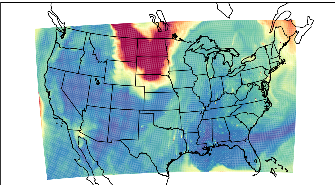
WRF 2023-09-05_20:00:00
