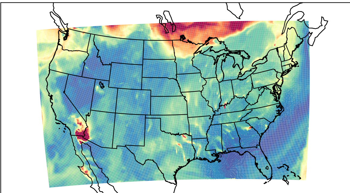
WRF 2023-09-04_06:00:00
