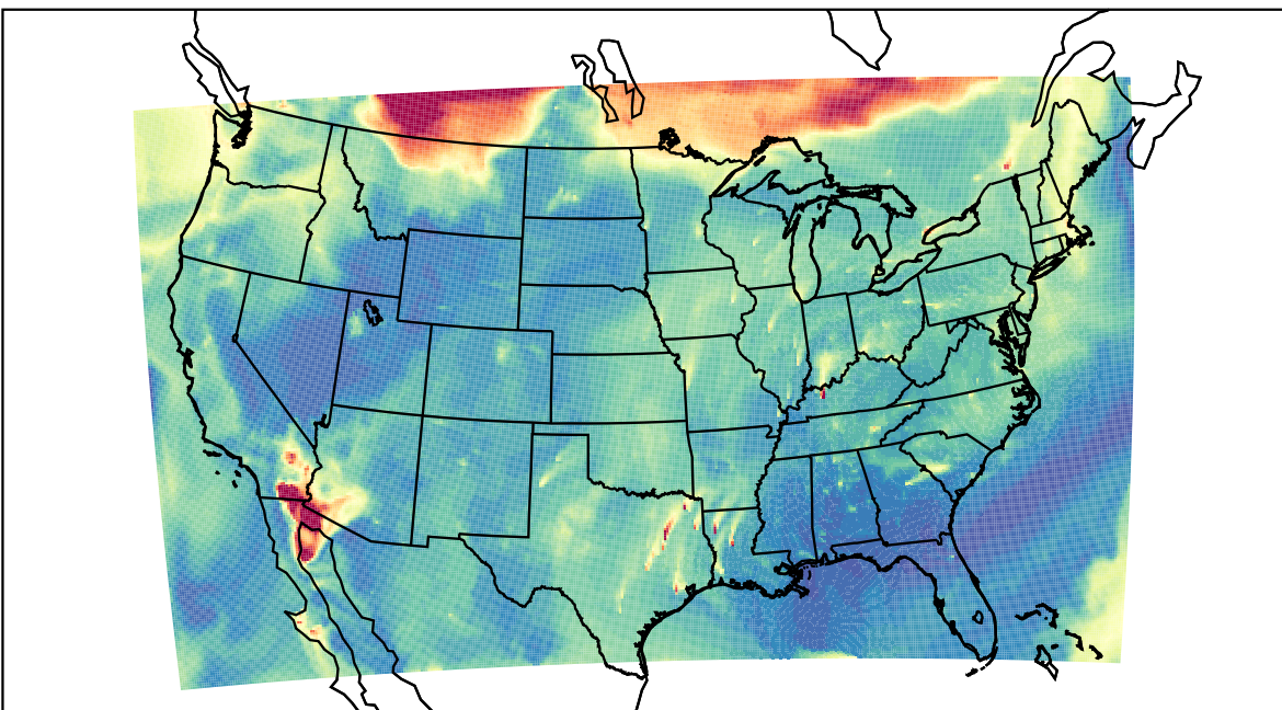
WRF 2023-09-04_14:00:00
