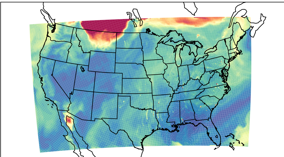
WRF 2023-09-04_21:00:00
