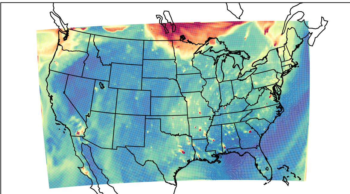
WRF 2023-09-04_01:00:00
