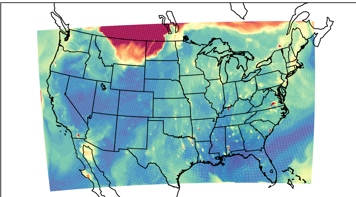
WRF 2023-09-05_02:00:00
