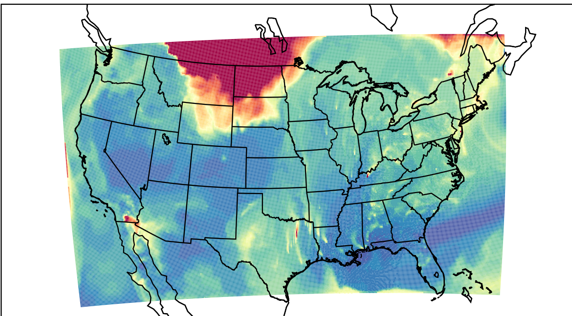
WRF 2023-09-05_11:00:00
