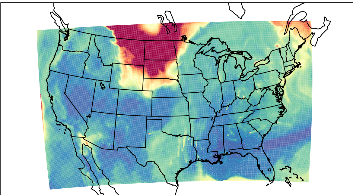
WRF 2023-09-05_16:00:00
