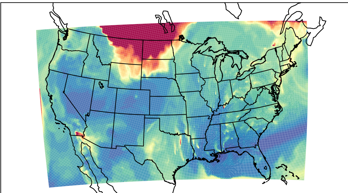
WRF 2023-09-05_10:00:00
