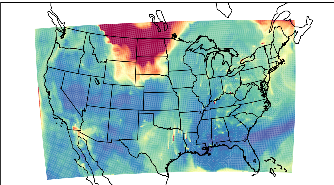
WRF 2023-09-05_14:00:00
