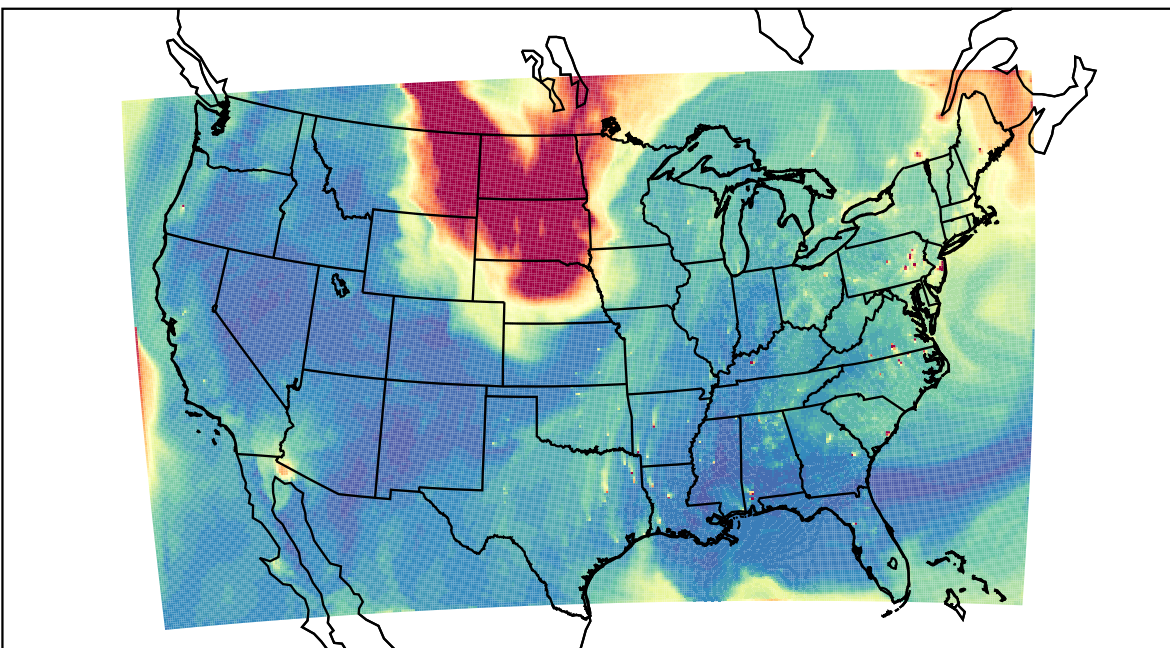
WRF 2023-09-05_23:00:00
