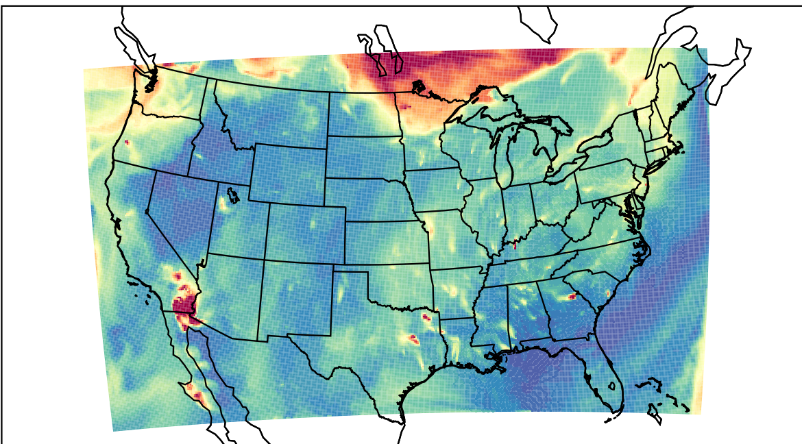
WRF 2023-09-04_04:00:00
