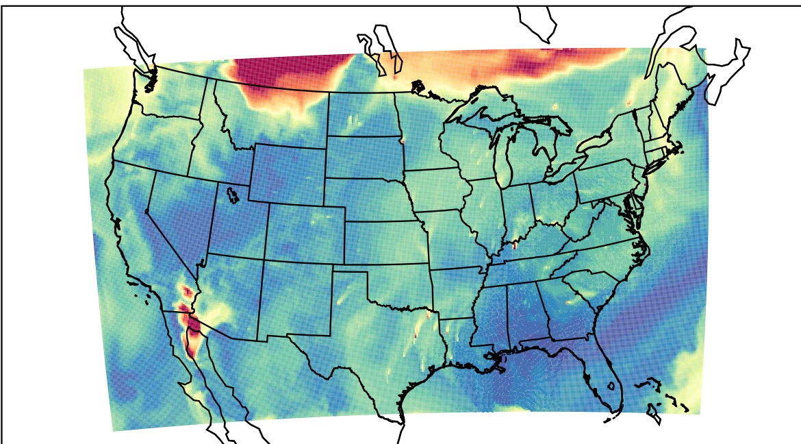
WRF 2023-09-04_16:00:00
