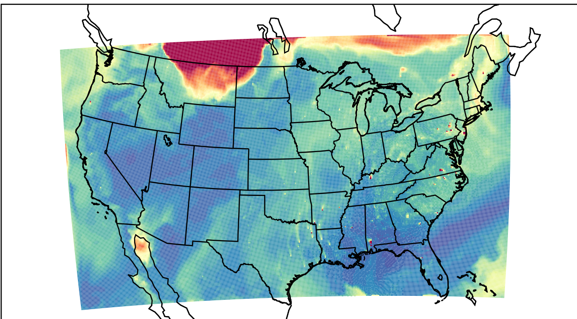
WRF 2023-09-04_23:00:00
