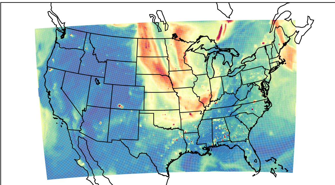
WRF 2023-09-07_01:00:00
