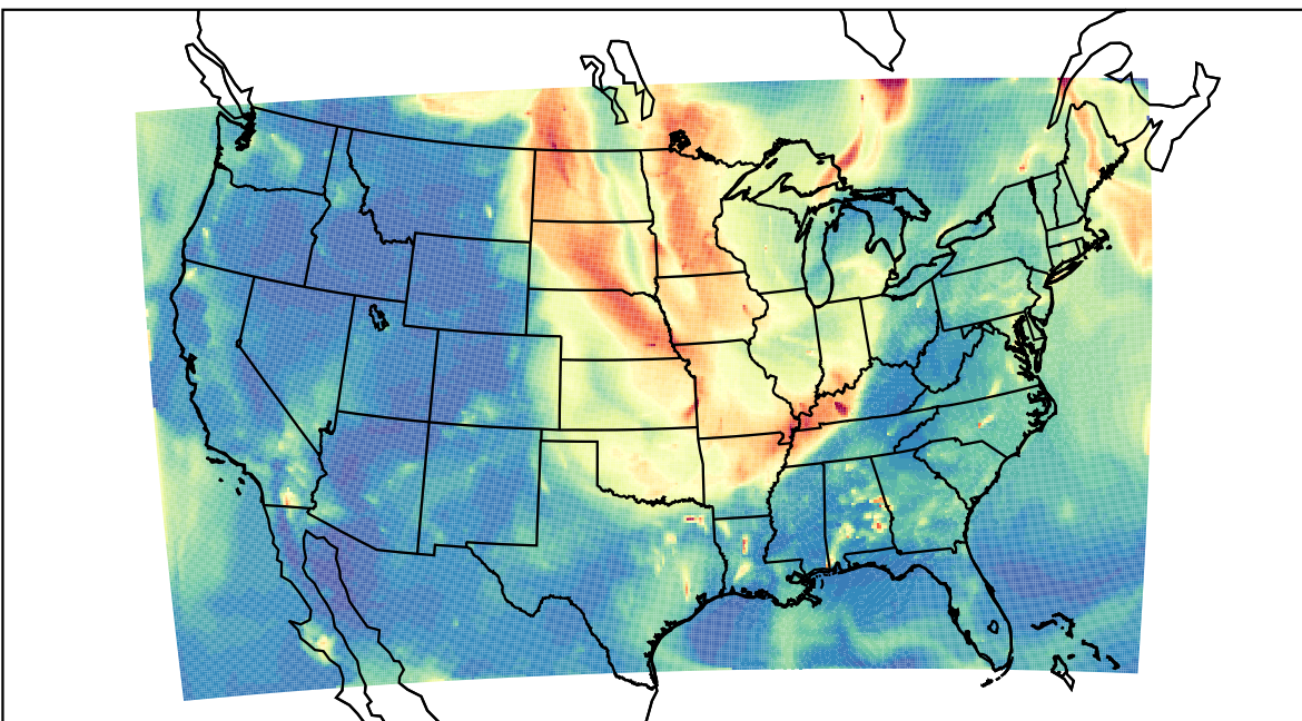
WRF 2023-09-07_06:00:00
