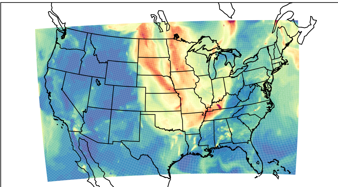
WRF 2023-09-07_08:00:00
