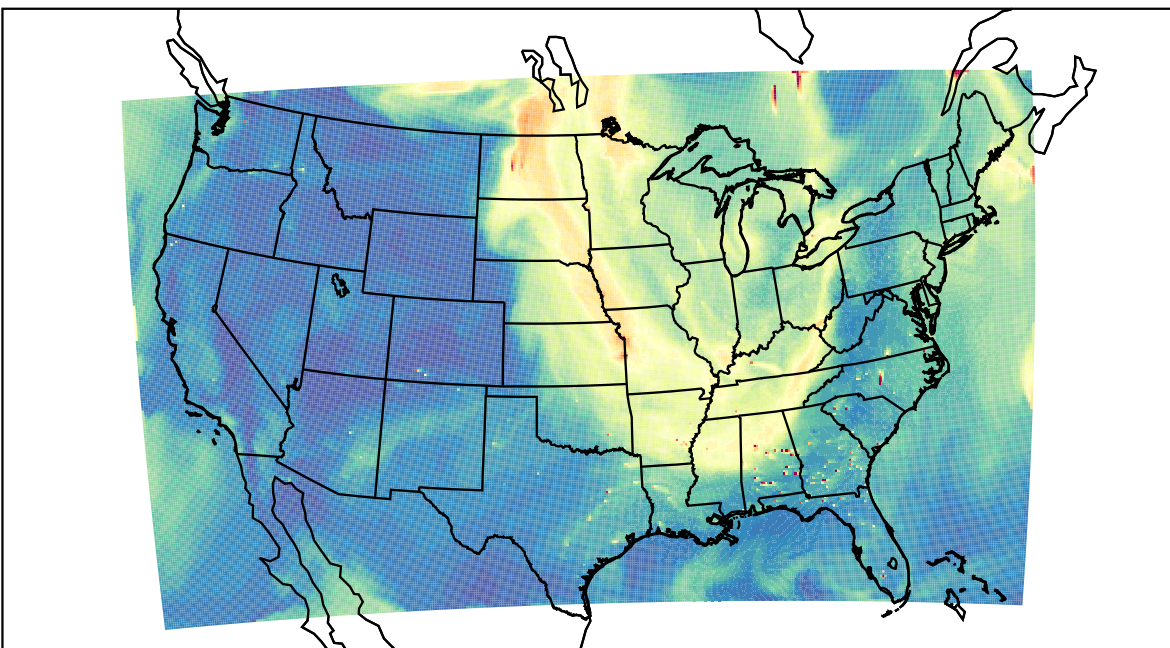
WRF 2023-09-07_20:00:00
