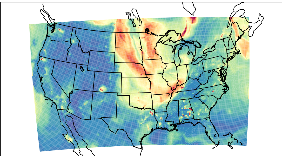
WRF 2023-09-07_04:00:00
