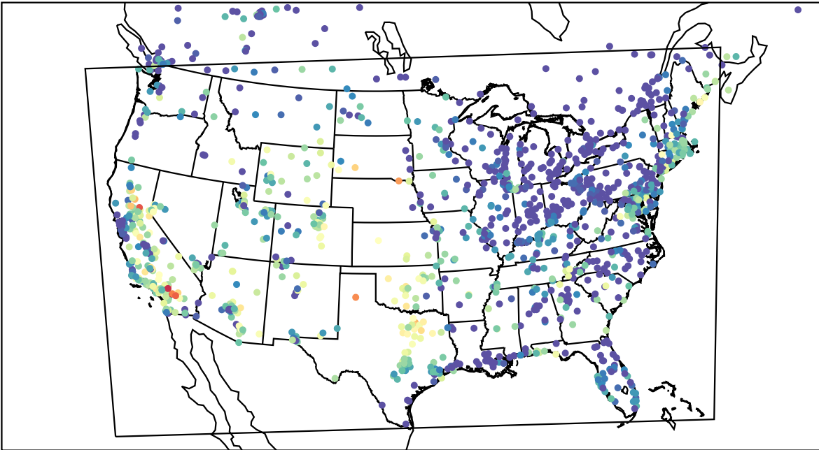
AirNOW (2023-09-09_04:00:00)
