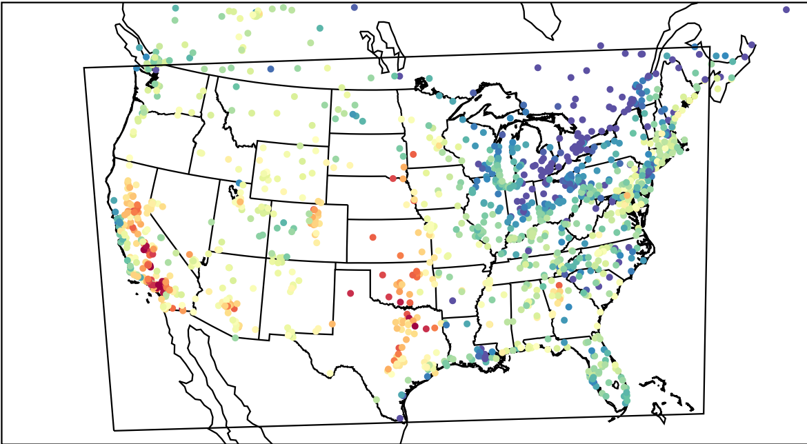
AirNOW (2023-09-08_23:00:00)
