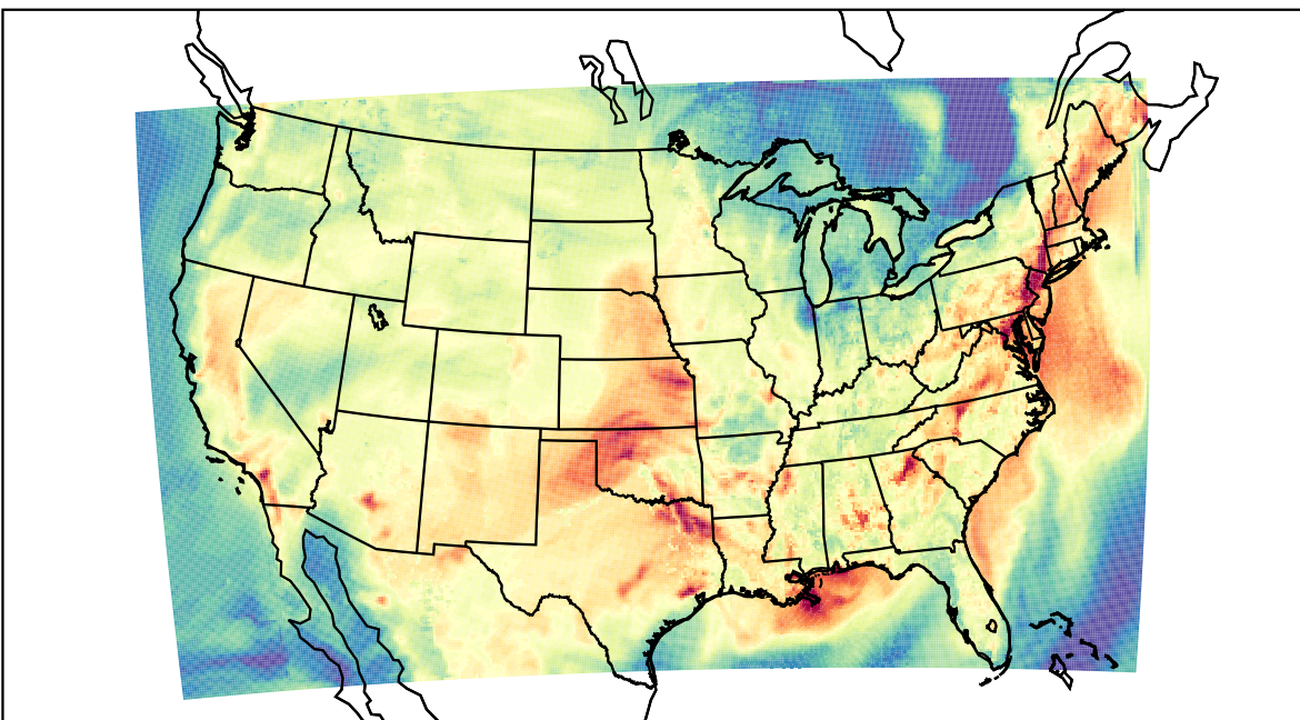
WRF (2023-09-08_23:00:00)
