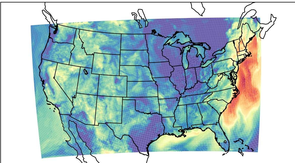
WRF (2023-09-08_13:00:00)
