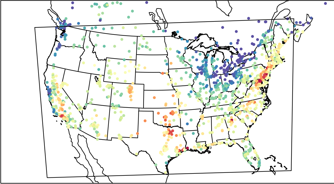
AirNOW (2023-09-08_18:00:00)
