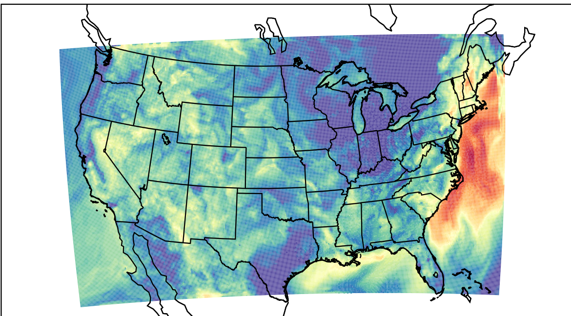
WRF (2023-09-08_11:00:00)
