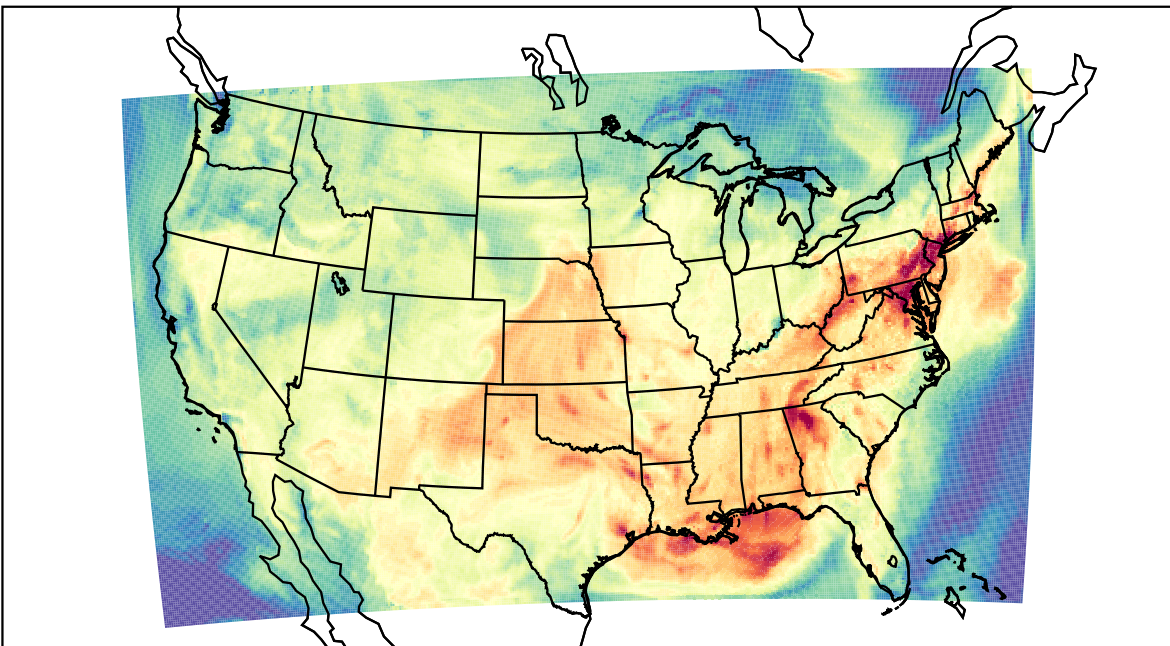
WRF (2023-09-09_18:00:00)
