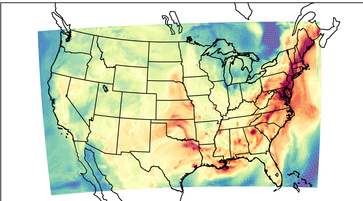
WRF (2023-09-08_19:00:00)
