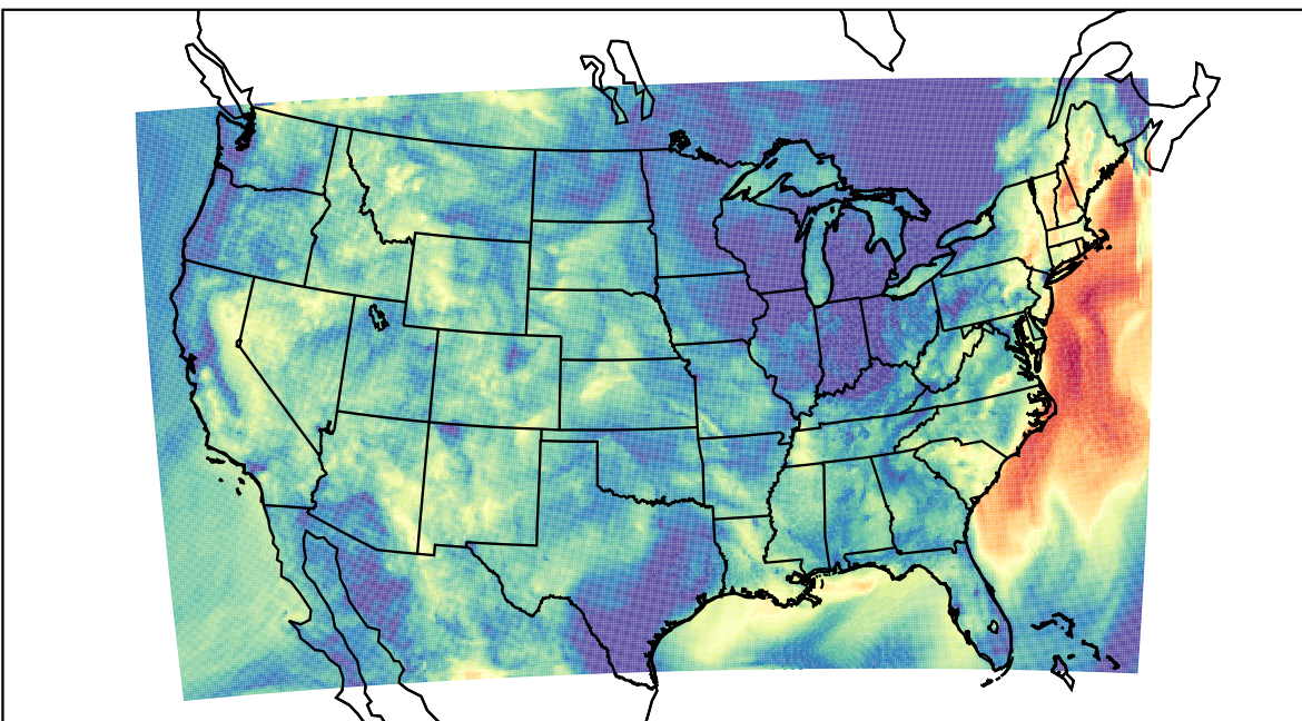
WRF (2023-09-08_10:00:00)
