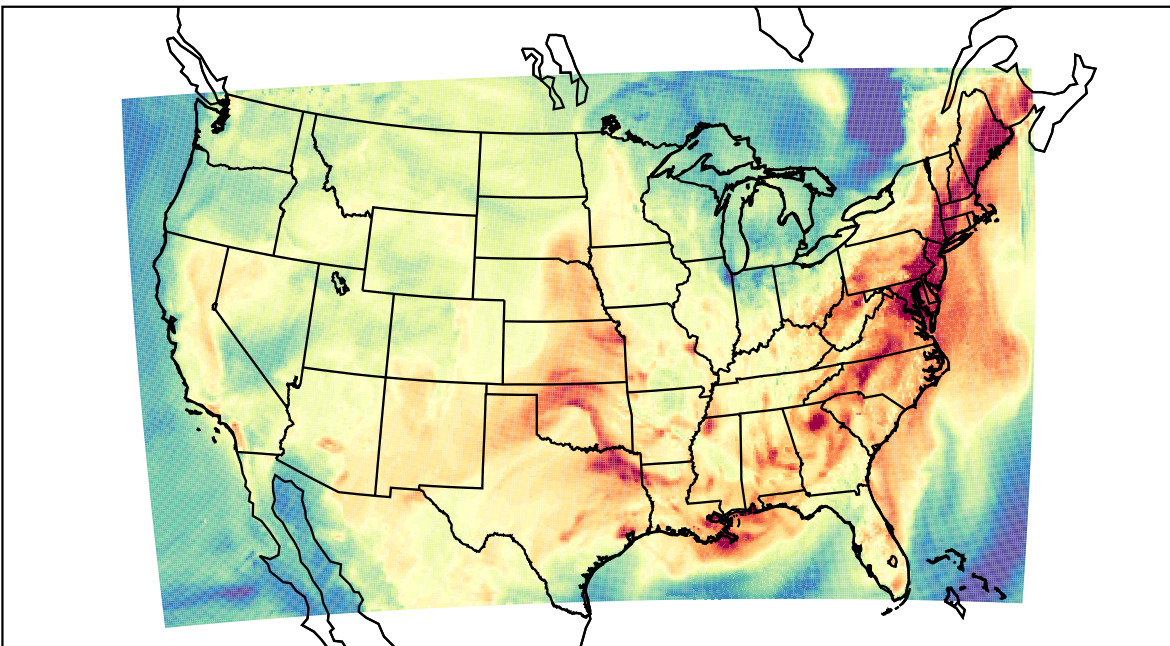
WRF (2023-09-08_20:00:00)
