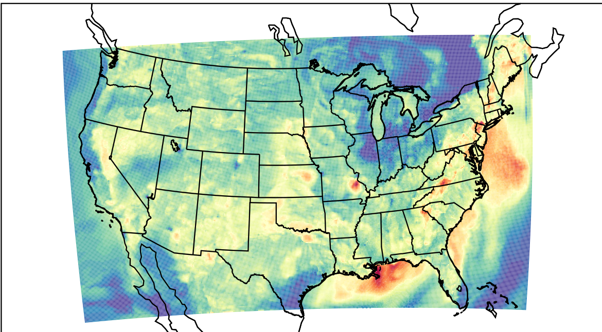
WRF (2023-09-09_03:00:00)
