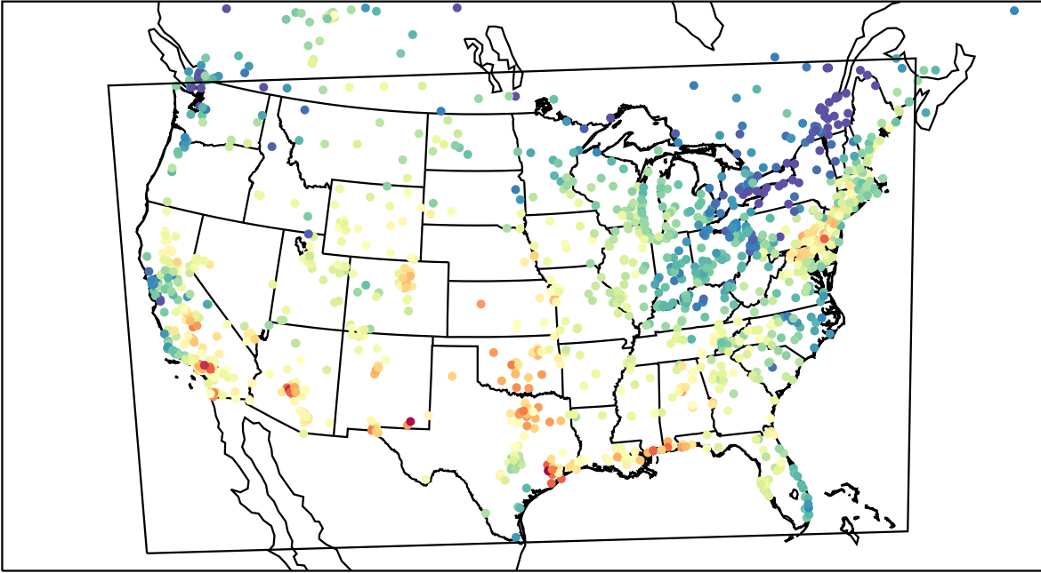
AirNOW (2023-09-09_18:00:00)
