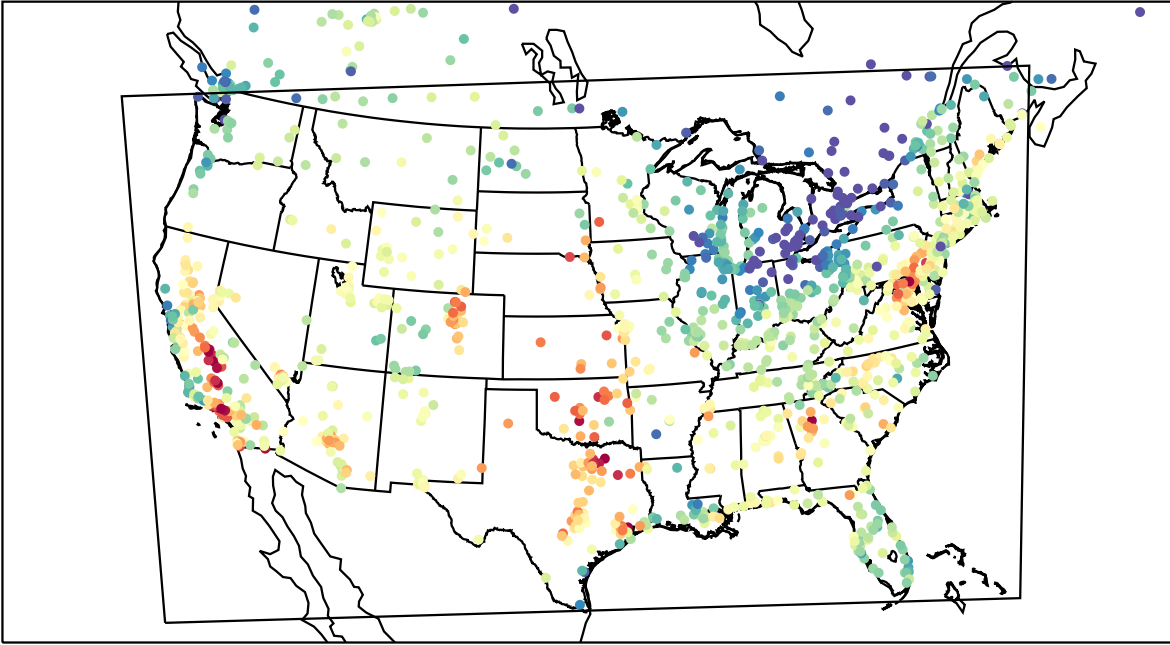
AirNOW (2023-09-08_20:00:00)
