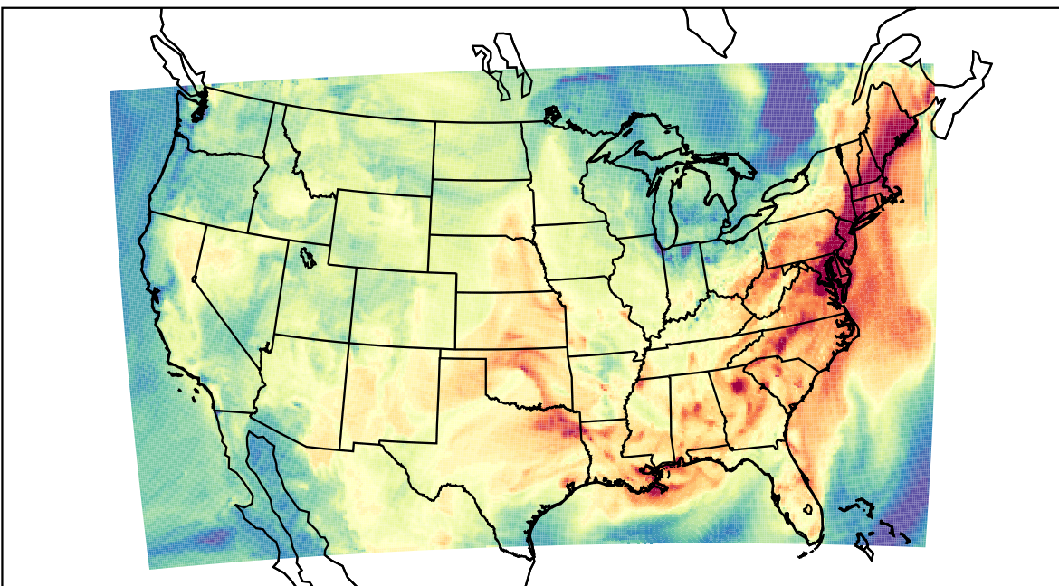
WRF (2023-09-08_18:00:00)
