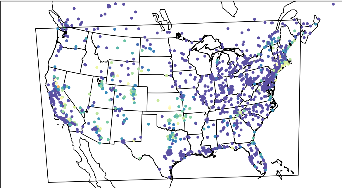
AirNOW (2023-09-08_10:00:00)
