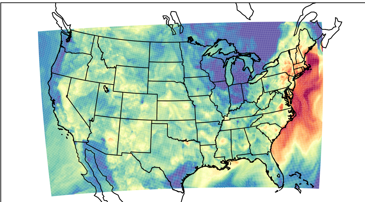
WRF (2023-09-08_04:00:00)
