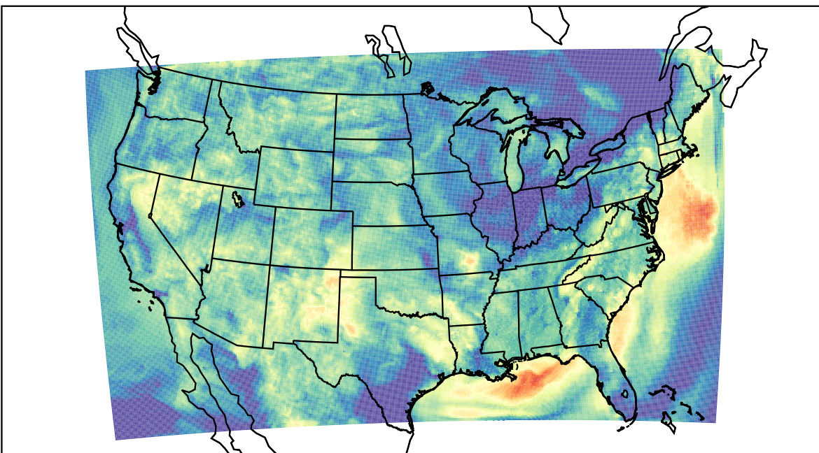
WRF (2023-09-09_10:00:00)
