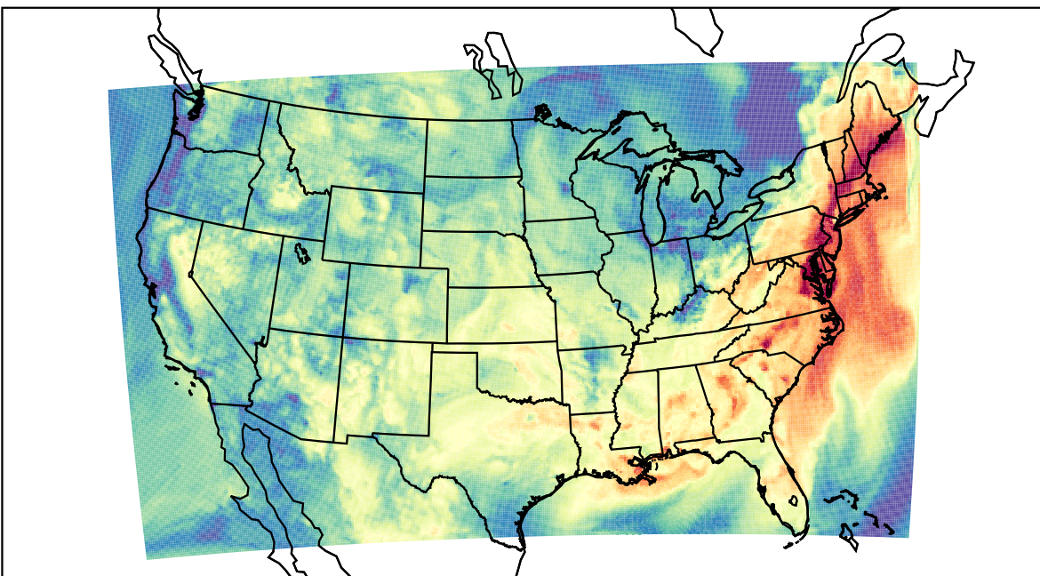
WRF (2023-09-08_16:00:00)
