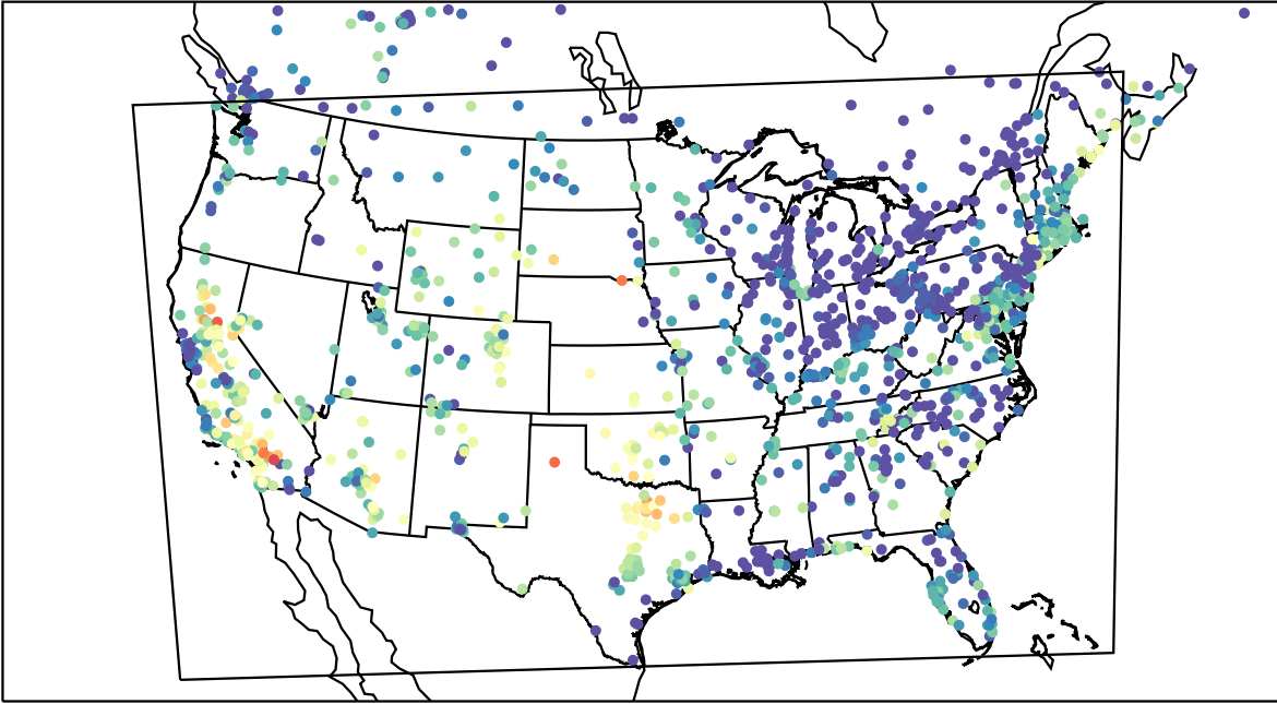
AirNOW (2023-09-09_03:00:00)
