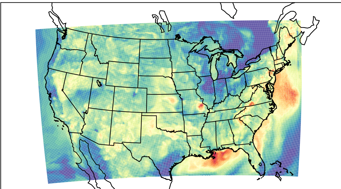
WRF (2023-09-09_04:00:00)
