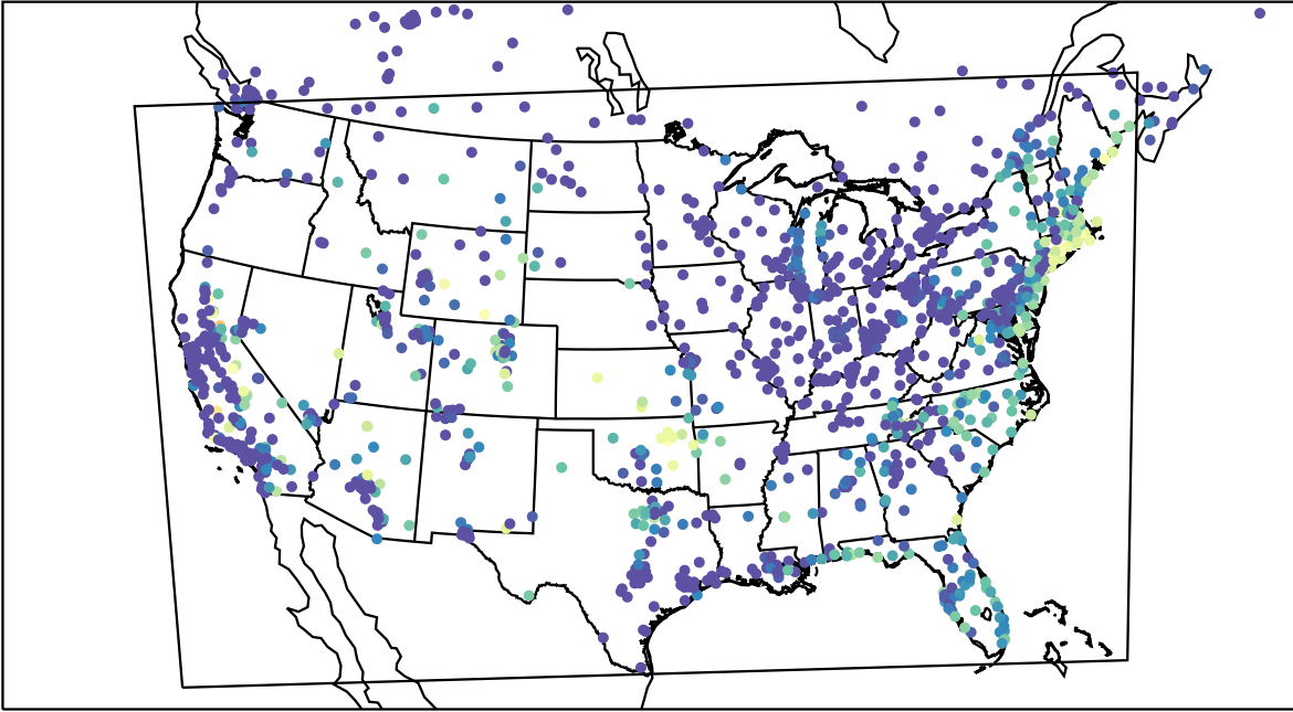
AirNOW (2023-09-08_13:00:00)
