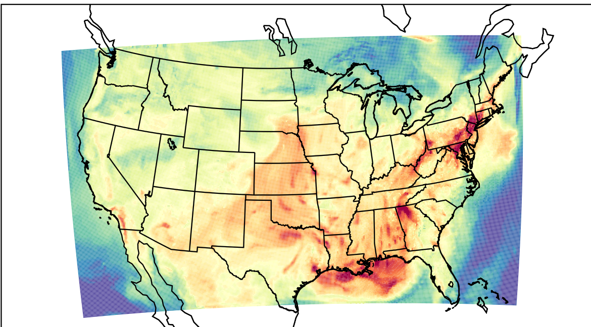
WRF (2023-09-09_20:00:00)
