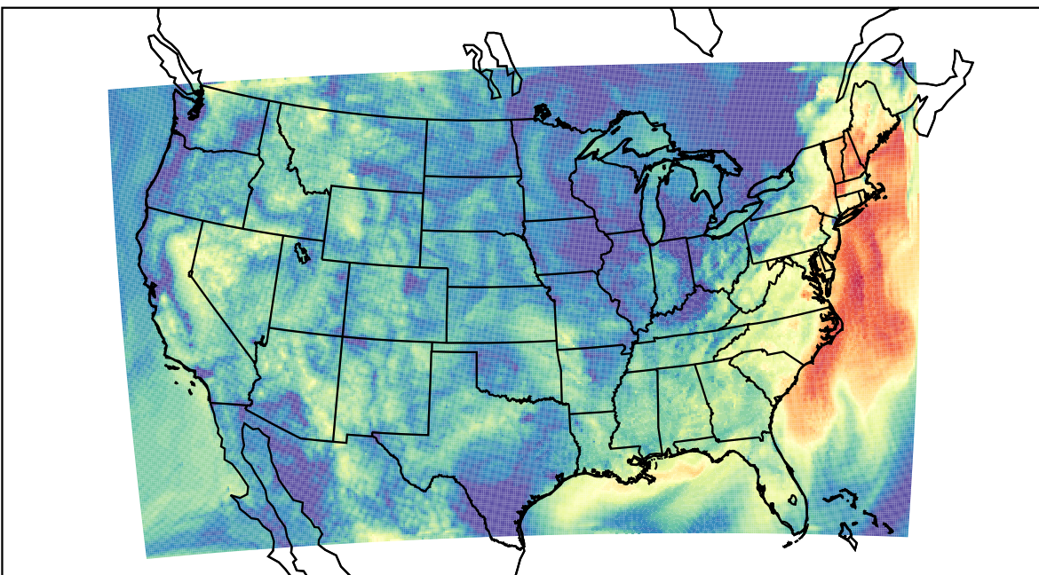
WRF (2023-09-08_14:00:00)
