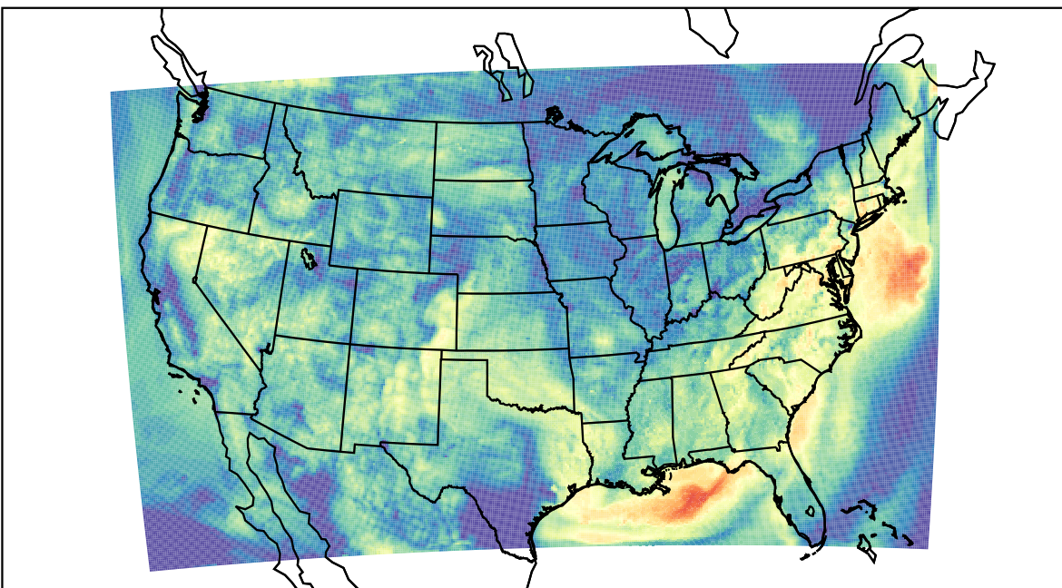
WRF (2023-09-09_14:00:00)
