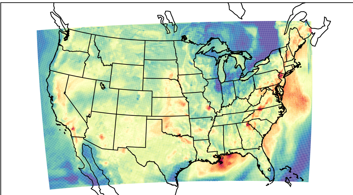
WRF (2023-09-09_01:00:00)
