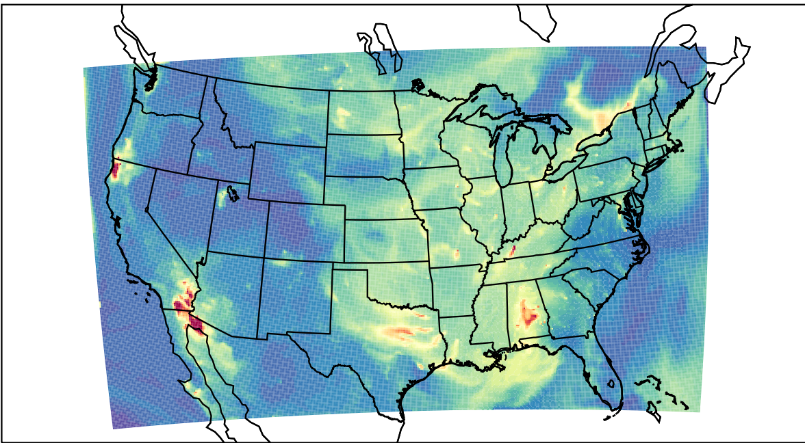
WRF 2023-09-10_09:00:00
