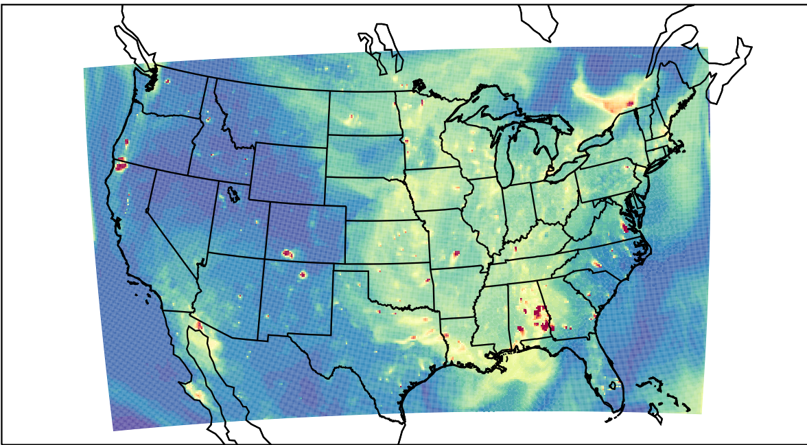
WRF 2023-09-10_01:00:00
