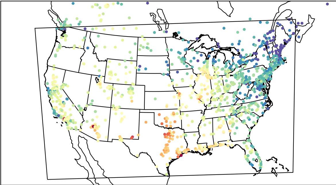
AirNOW (2023-09-10_19:00:00)
