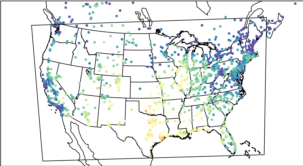
AirNOW (2023-09-10_16:00:00)
