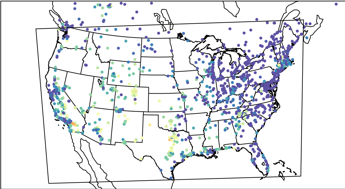
AirNOW (2023-09-10_06:00:00)
