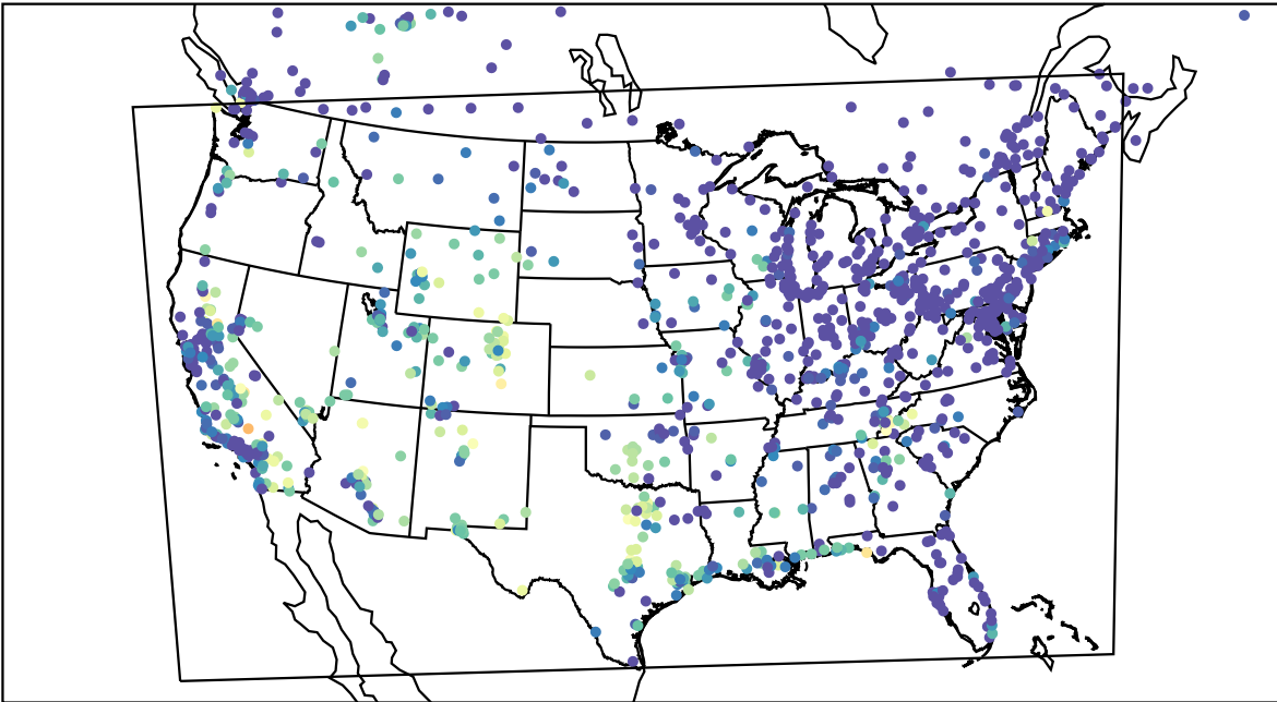
AirNOW (2023-09-10_08:00:00)
