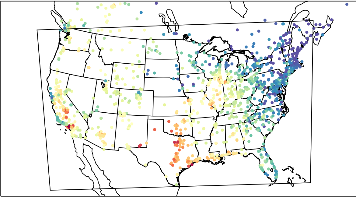
AirNOW (2023-09-10_22:00:00)
