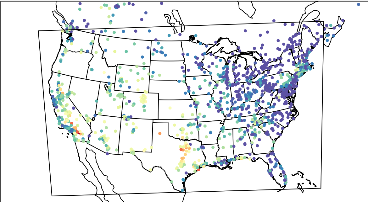
AirNOW (2023-09-10_03:00:00)
