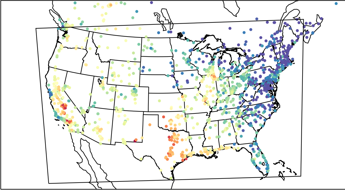
AirNOW (2023-09-10_23:00:00)
