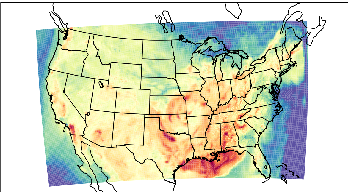
WRF (2023-09-10_22:00:00)
