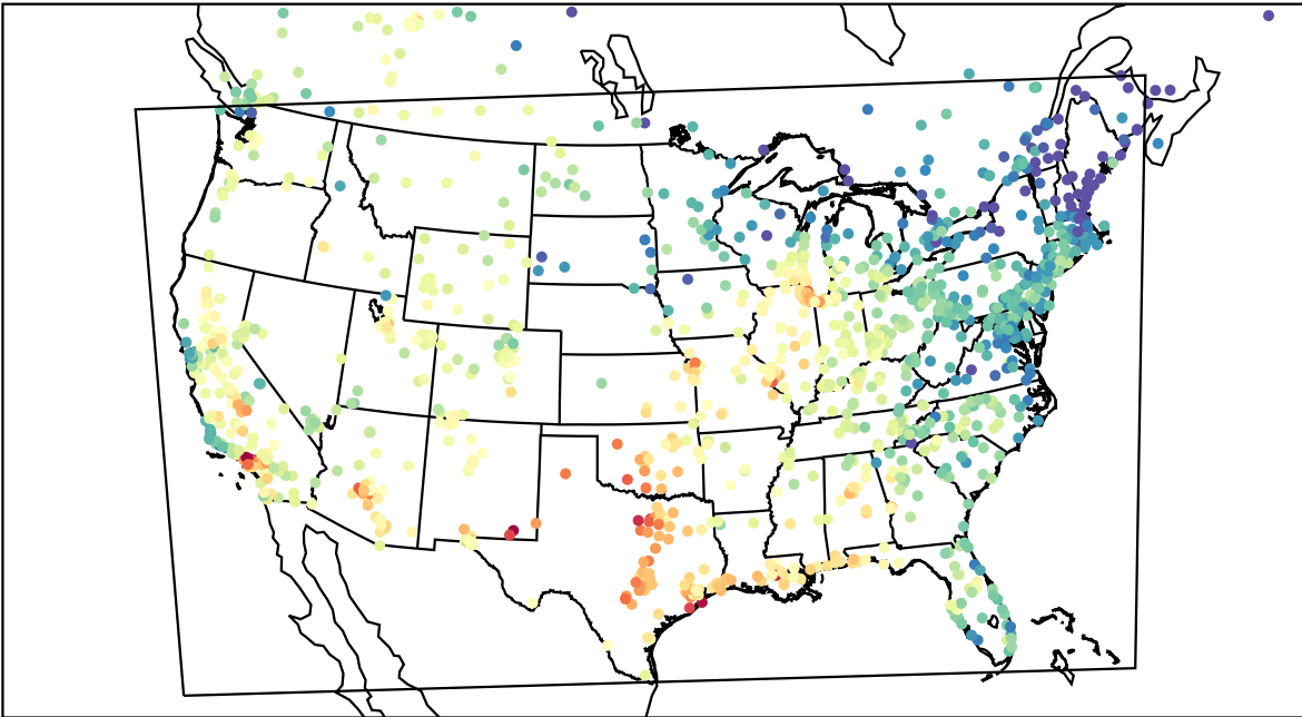
AirNOW (2023-09-10_20:00:00)
