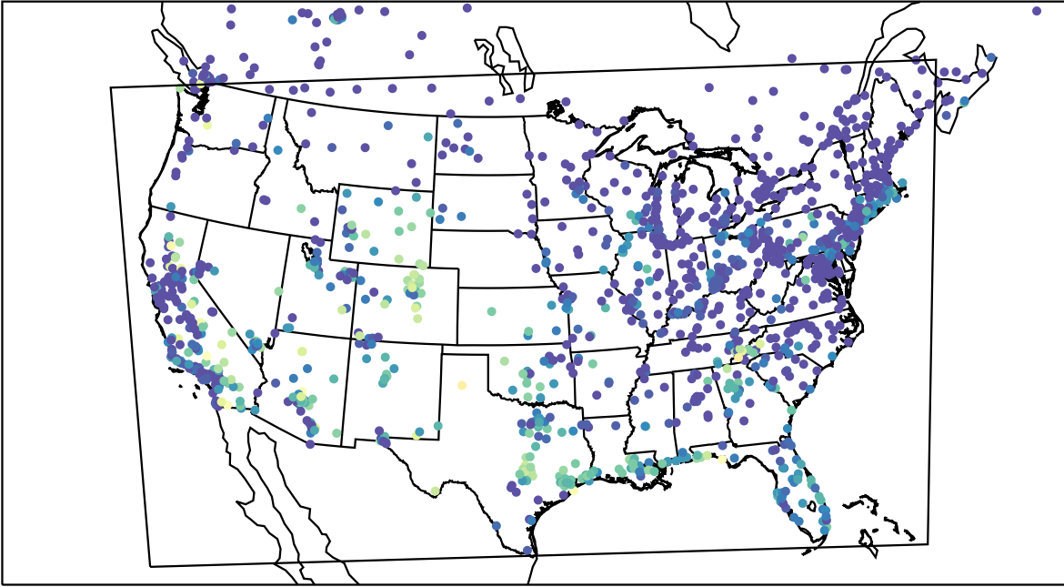
AirNOW (2023-09-10_13:00:00)
