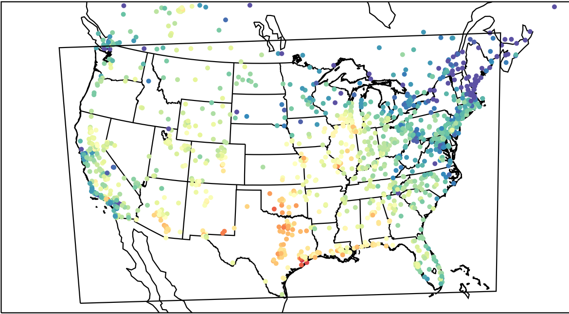
AirNOW (2023-09-10_18:00:00)
