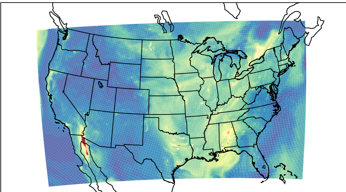
WRF 2023-09-10_18:00:00
