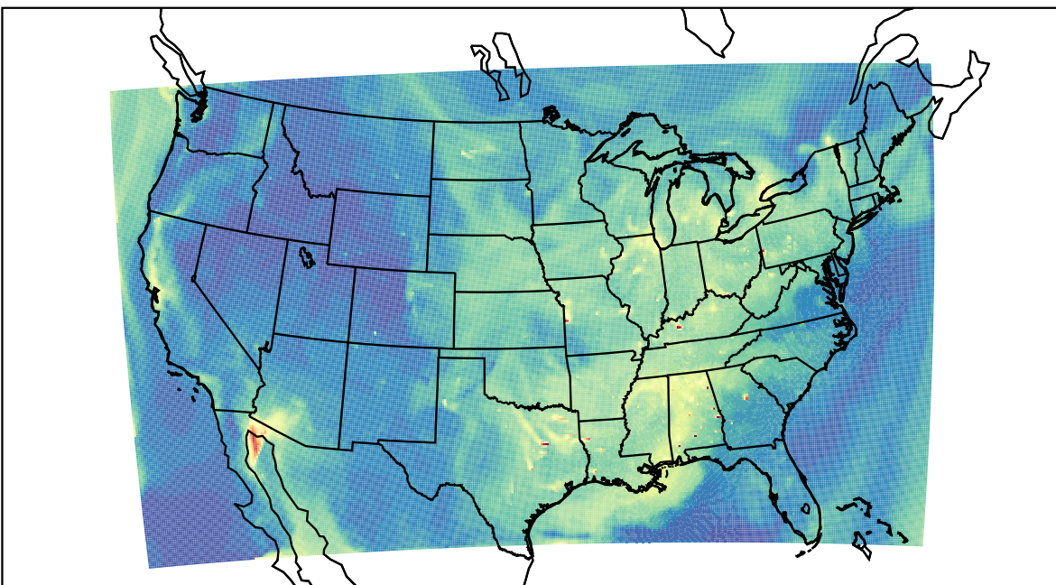
WRF 2023-09-11_18:00:00
