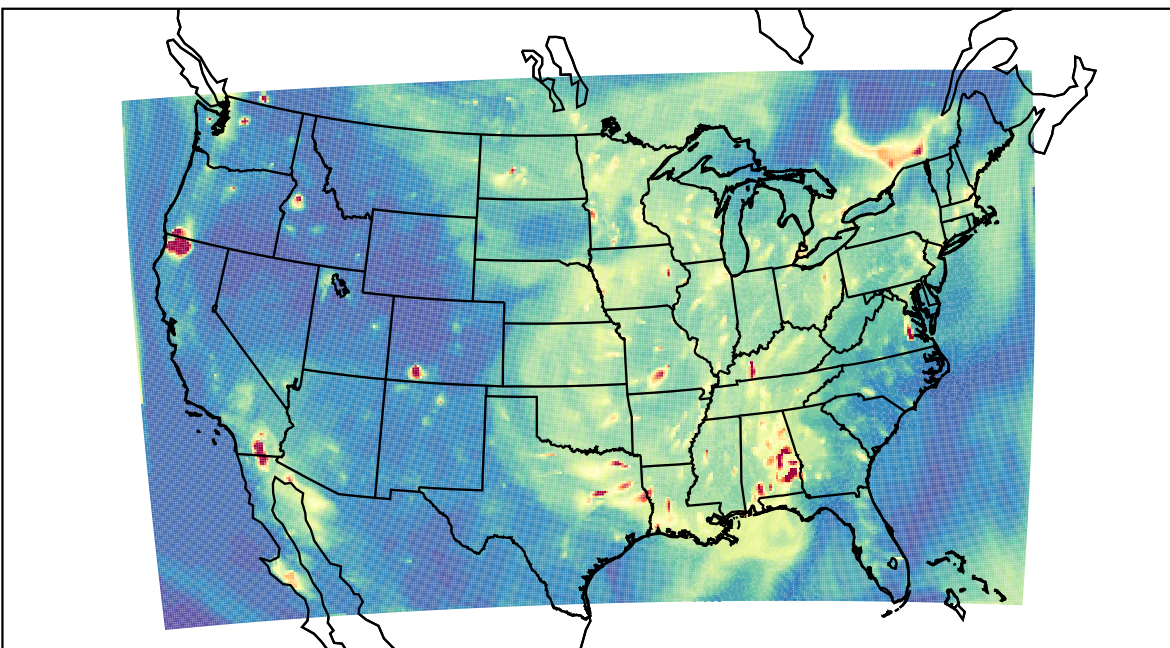
WRF 2023-09-10_03:00:00
