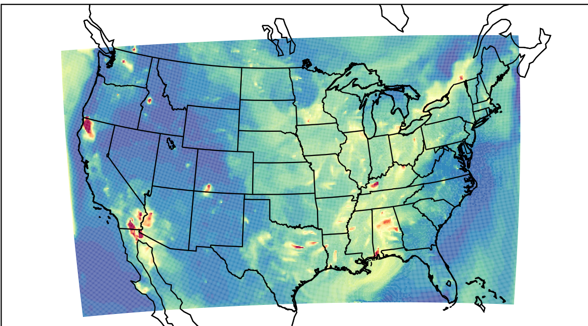
WRF 2023-09-11_04:00:00
