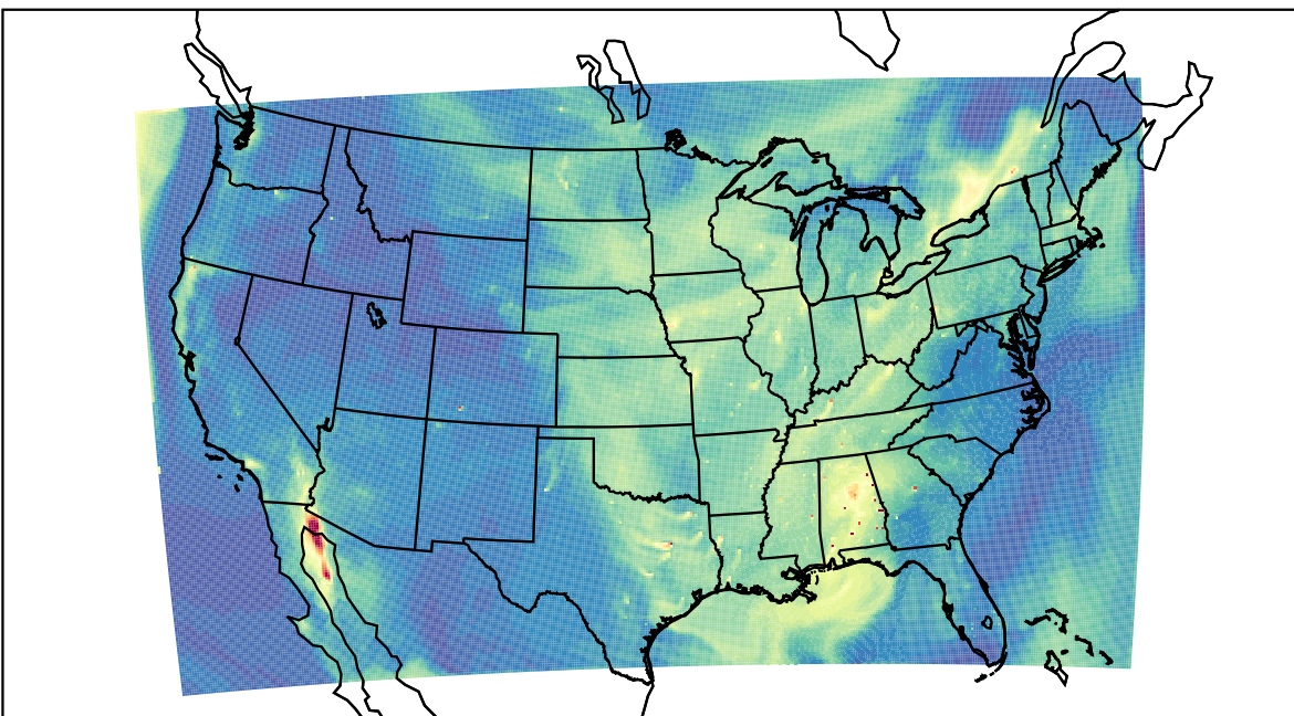
WRF 2023-09-10_19:00:00
