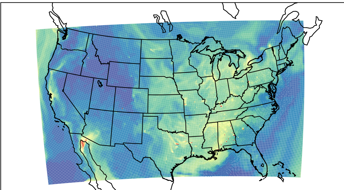
WRF 2023-09-11_19:00:00
