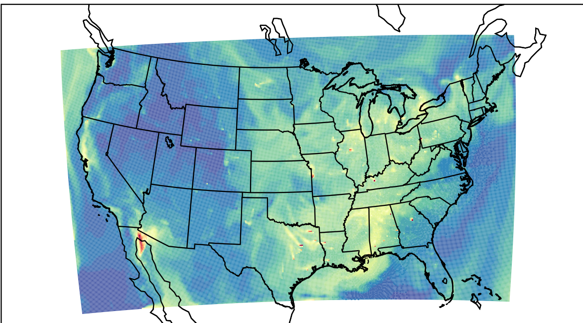
WRF 2023-09-11_17:00:00
