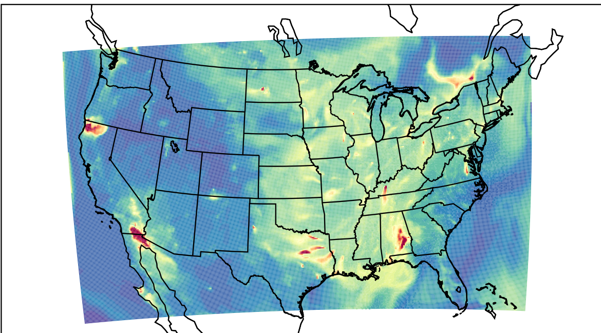
WRF 2023-09-10_06:00:00
