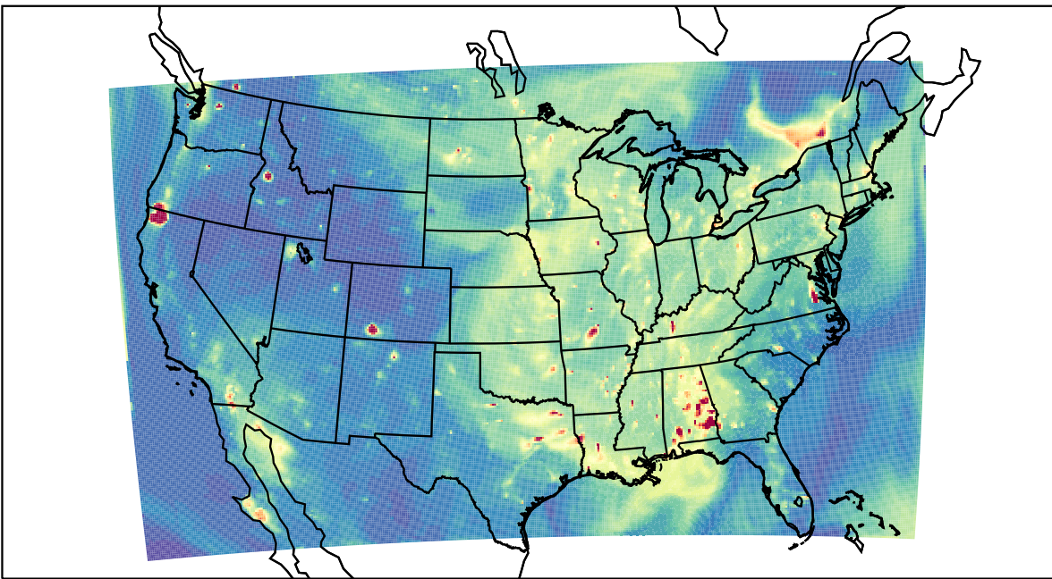
WRF 2023-09-10_02:00:00
