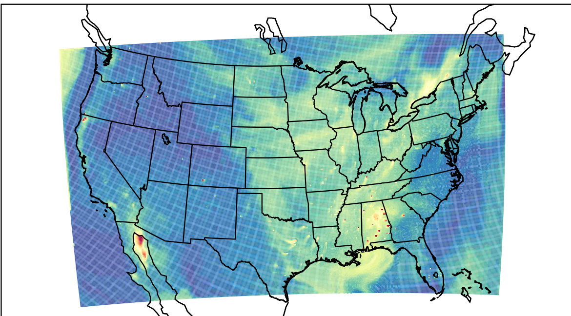
WRF 2023-09-10_21:00:00
