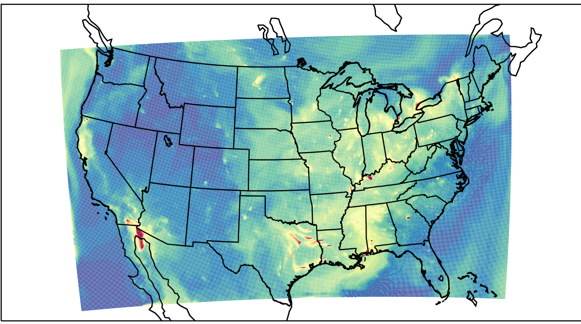
WRF 2023-09-11_14:00:00
