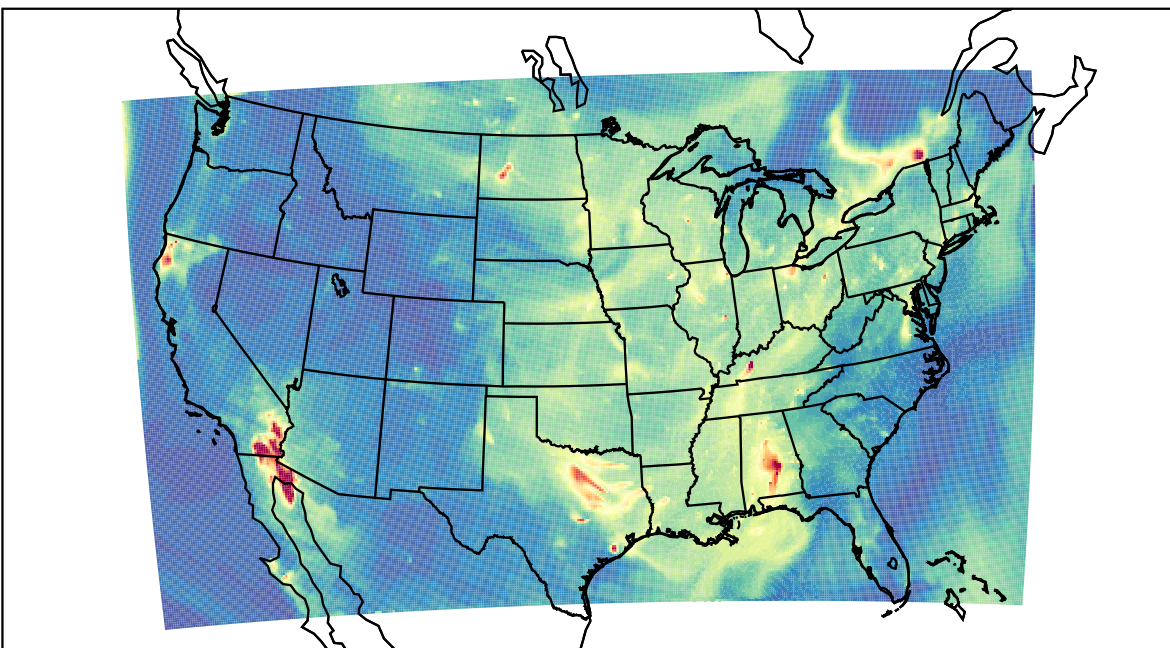
WRF 2023-09-10_11:00:00
