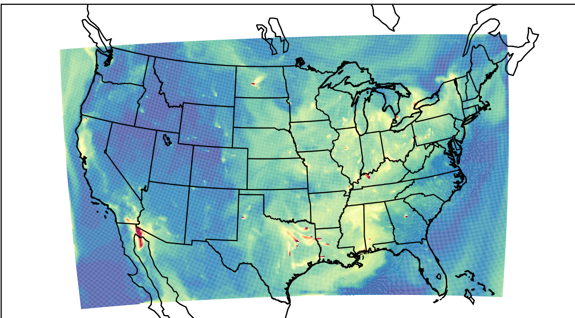
WRF 2023-09-11_15:00:00
