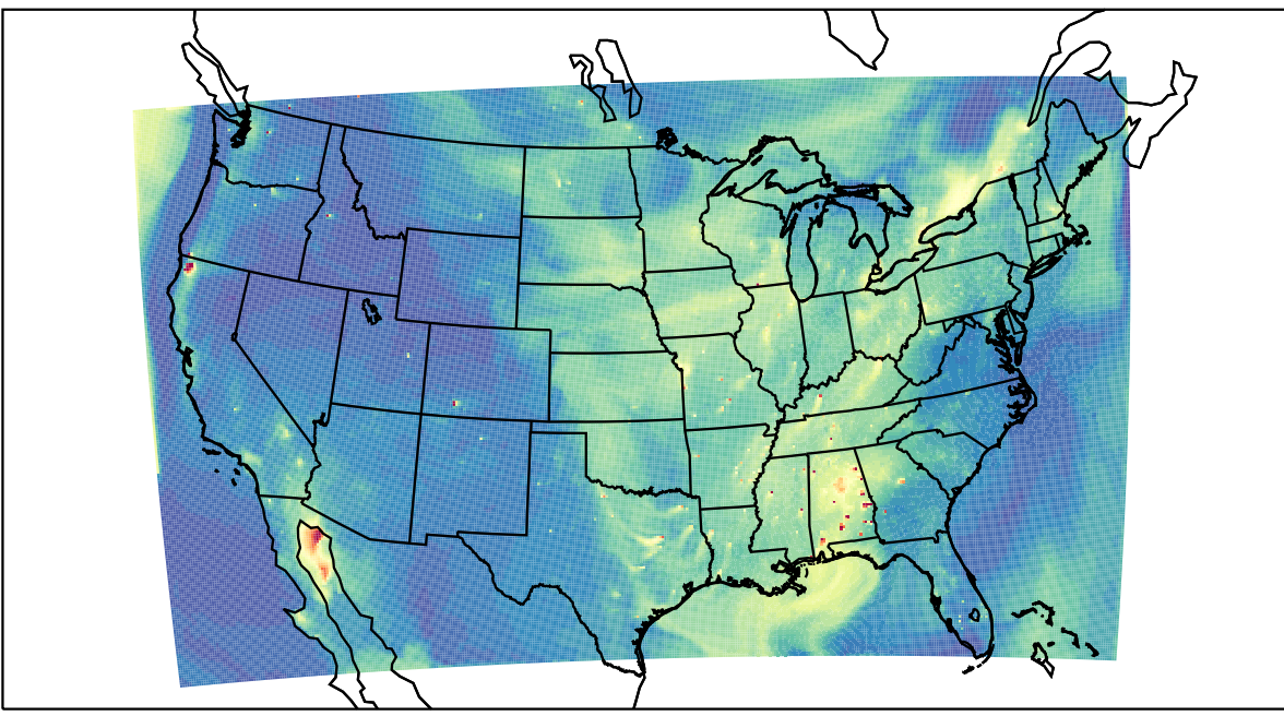
WRF 2023-09-10_22:00:00
