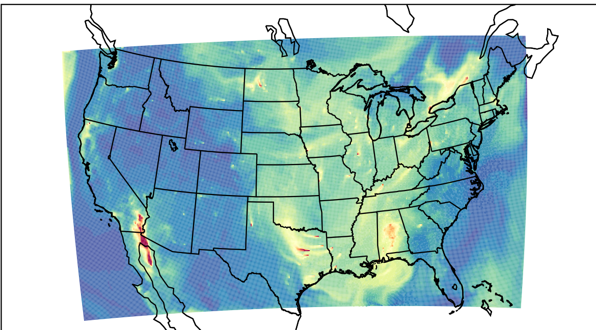
WRF 2023-09-10_16:00:00
