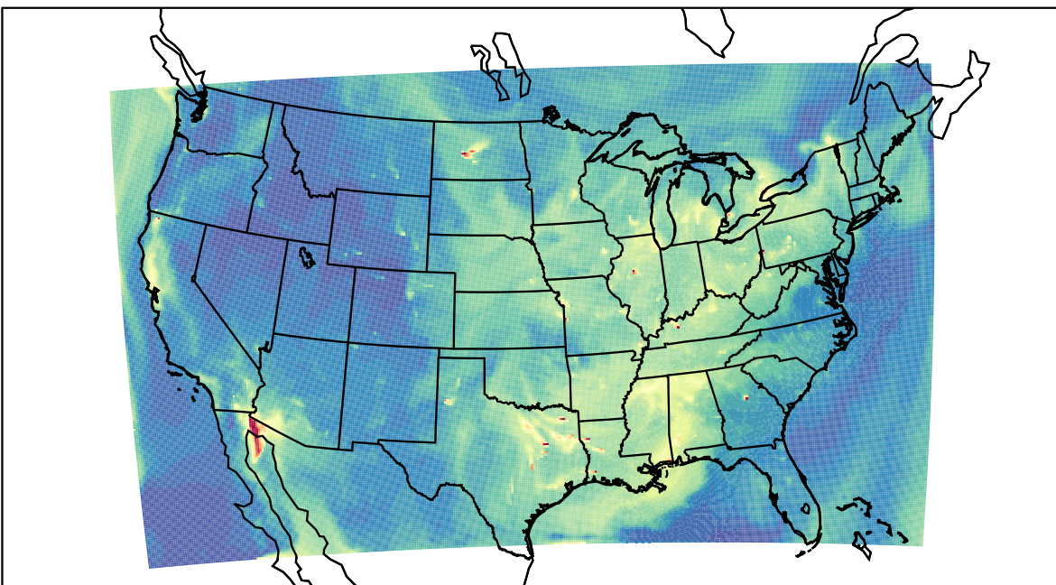
WRF 2023-09-11_16:00:00
