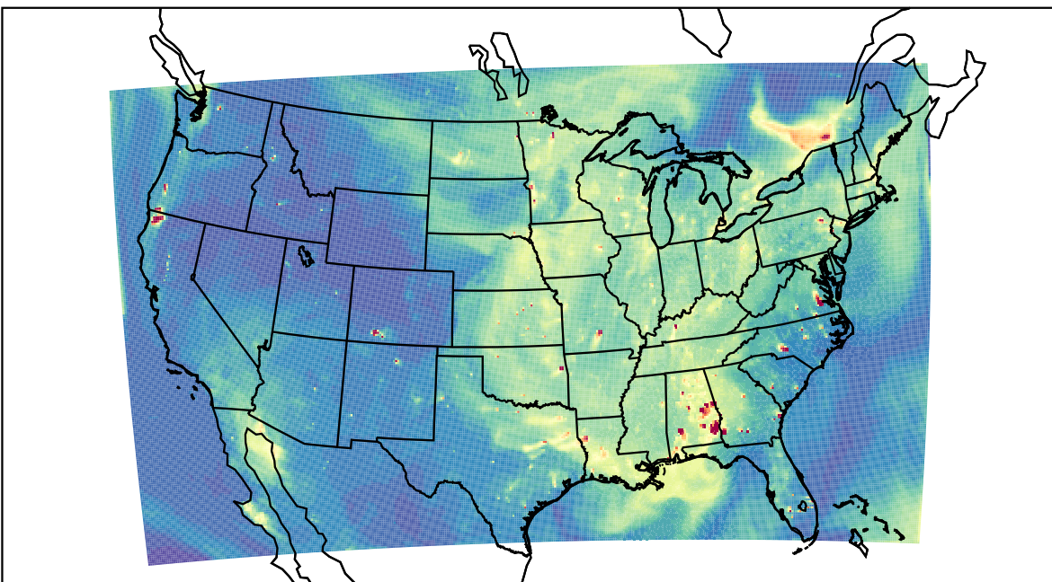
WRF 2023-09-10_00:00:00
