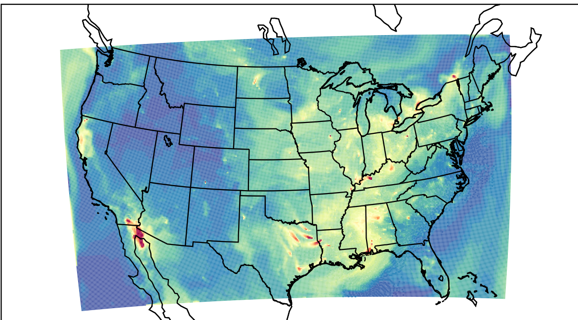
WRF 2023-09-11_12:00:00
