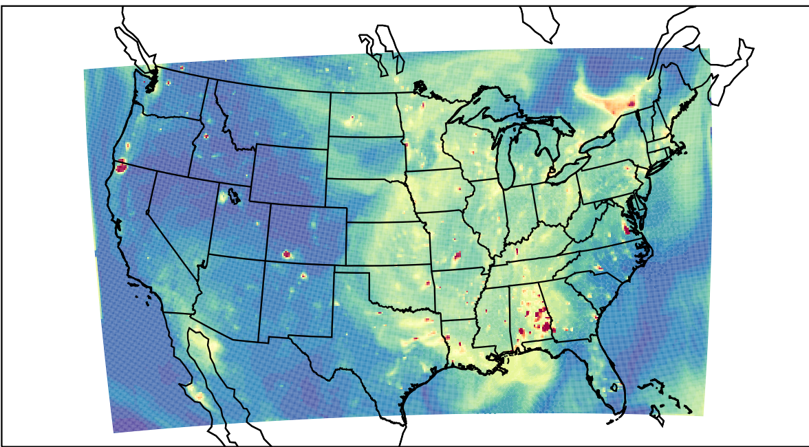
WRF 2023-09-10_01:00:00
