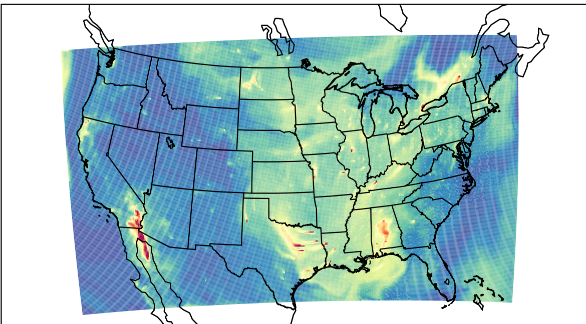
WRF 2023-09-10_15:00:00
