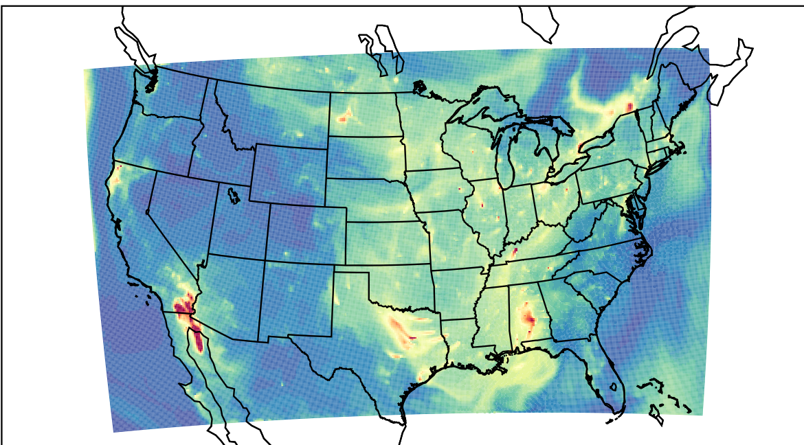
WRF 2023-09-10_13:00:00
