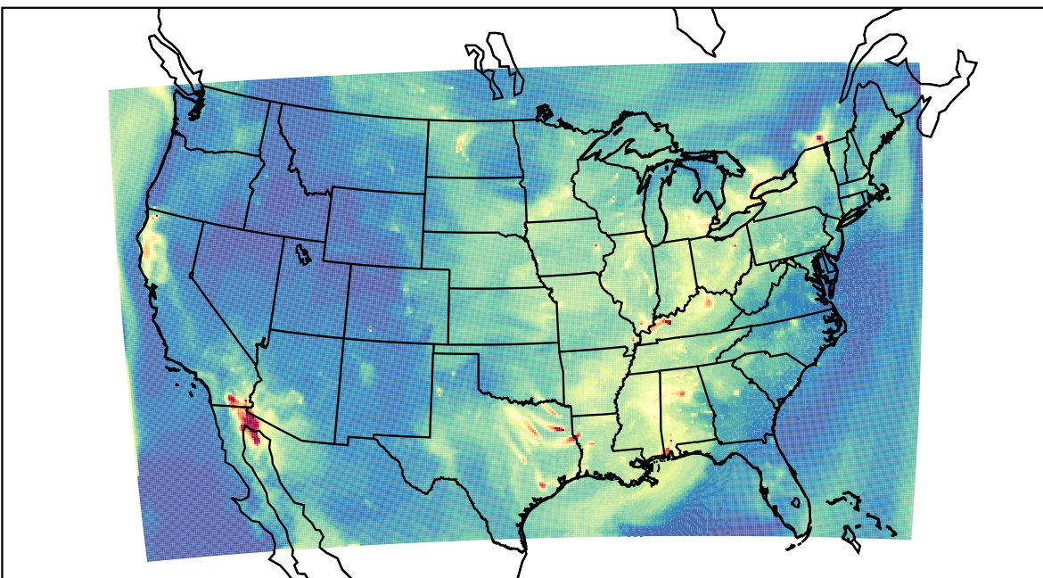
WRF 2023-09-11_11:00:00
