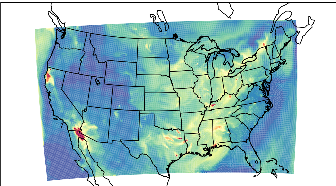
WRF 2023-09-11_08:00:00
