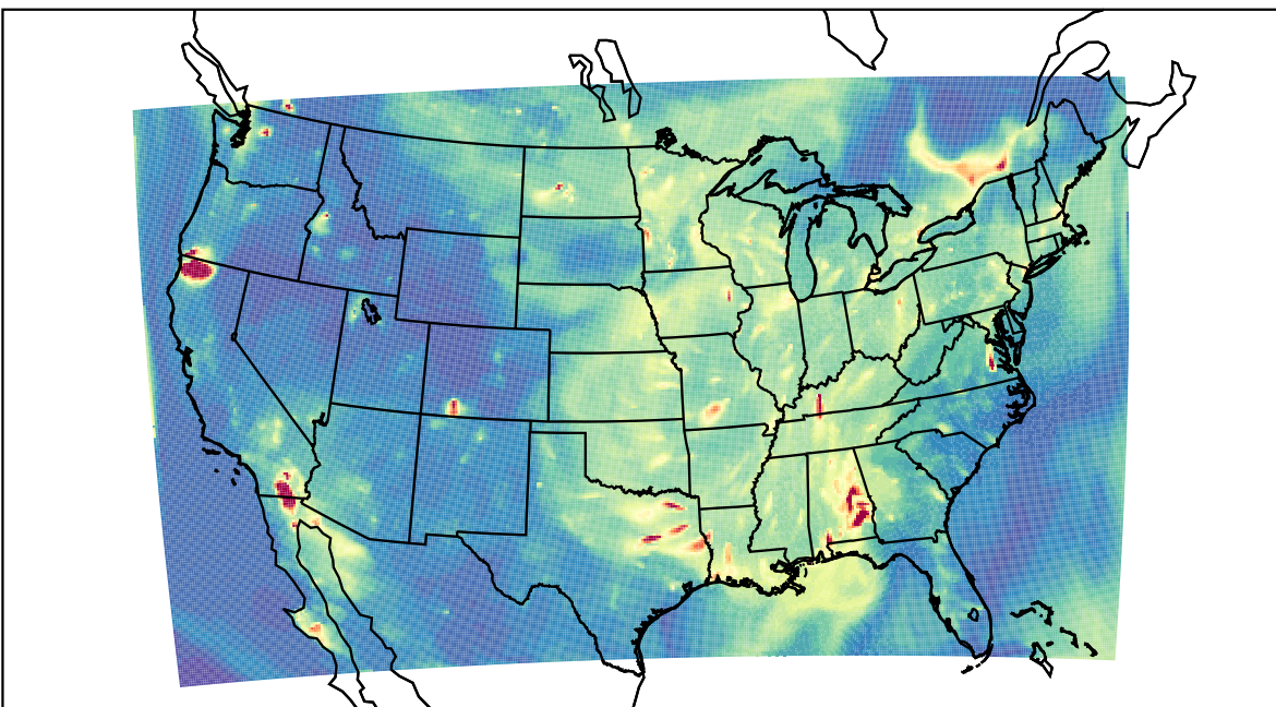
WRF 2023-09-10_04:00:00
