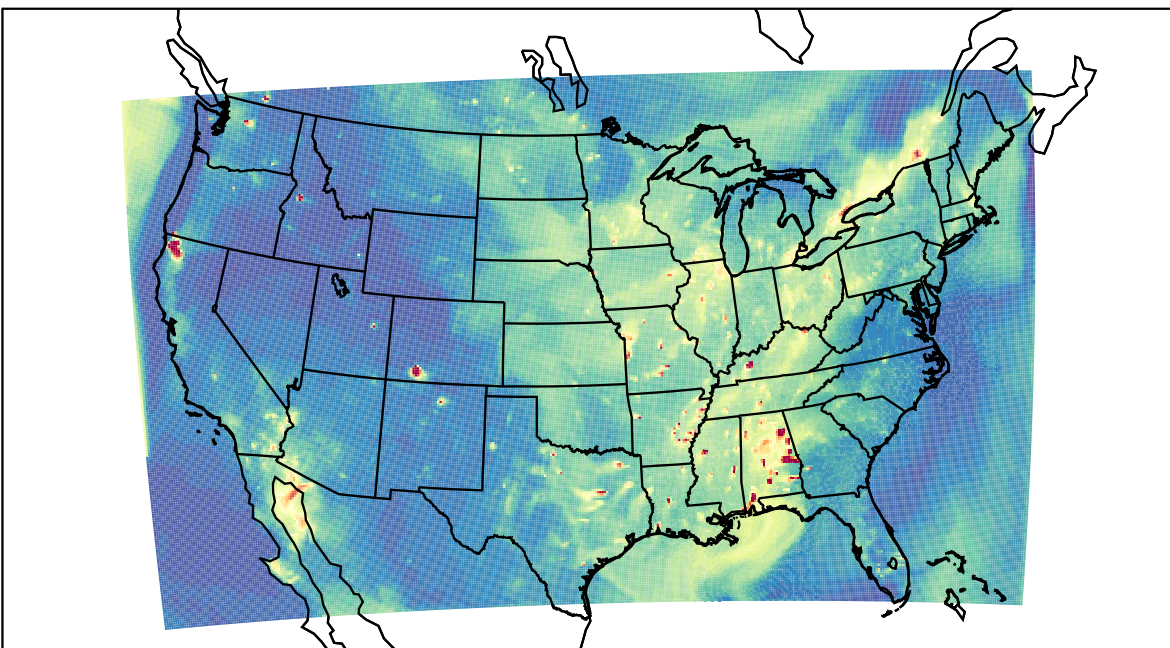
WRF 2023-09-11_01:00:00
