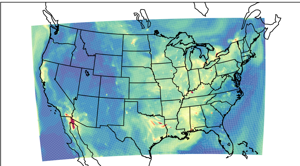
WRF 2023-09-11_13:00:00
