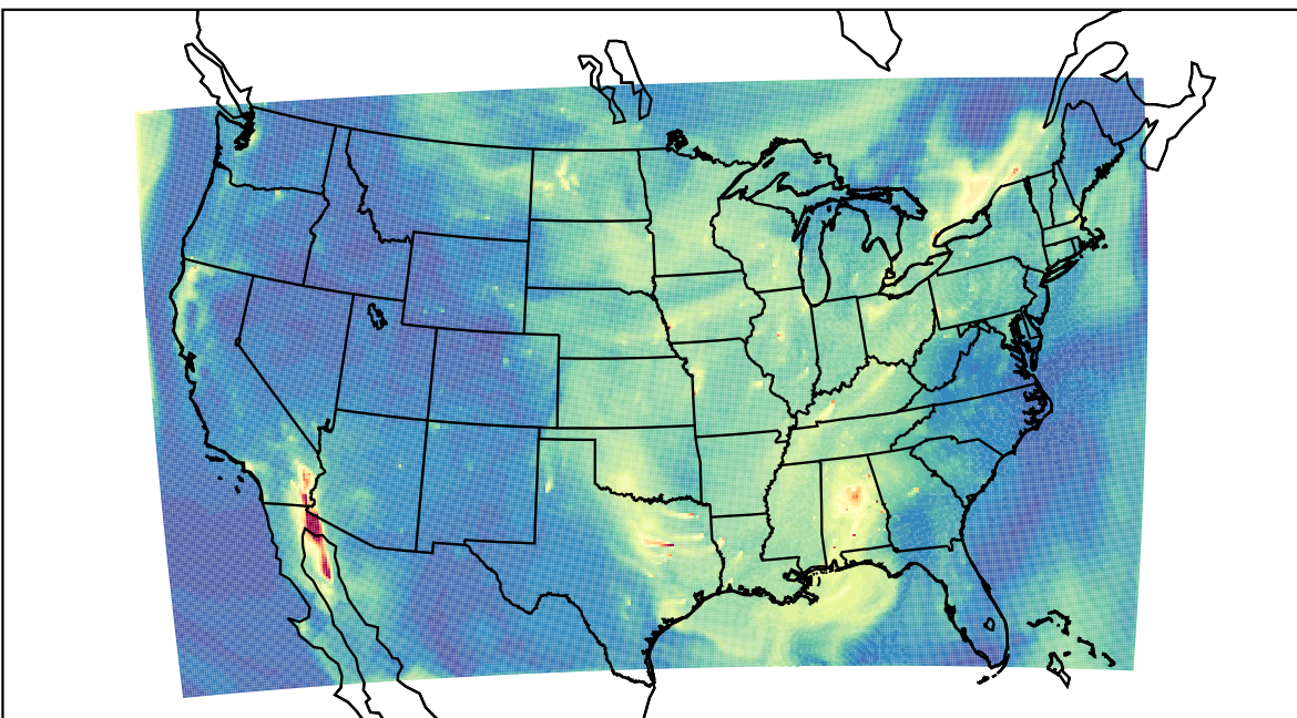
WRF 2023-09-10_17:00:00
