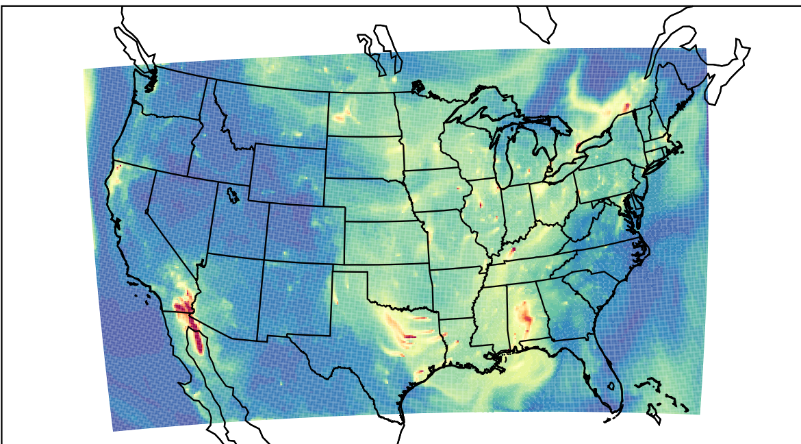
WRF 2023-09-10_14:00:00
