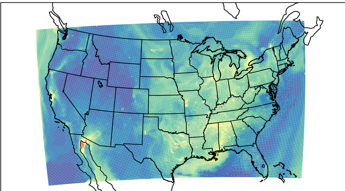
WRF 2023-09-11_20:00:00
