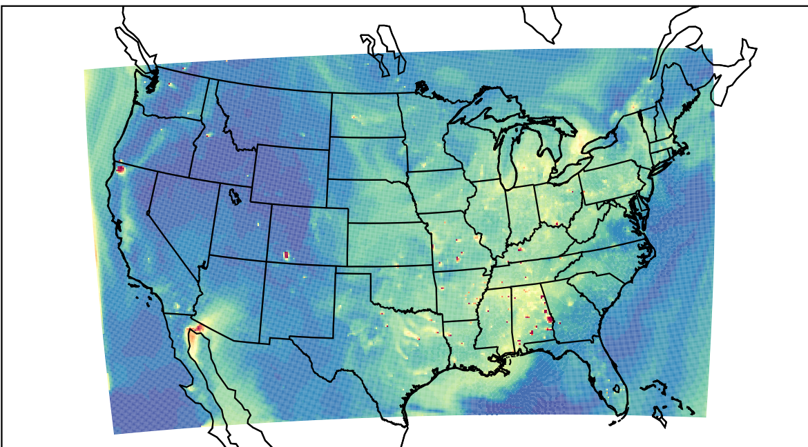
WRF 2023-09-11_23:00:00
