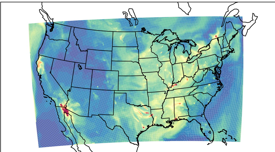
WRF 2023-09-11_10:00:00
