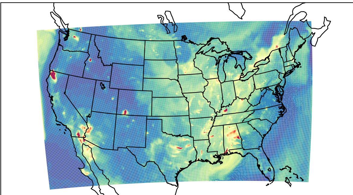
WRF 2023-09-11_03:00:00
