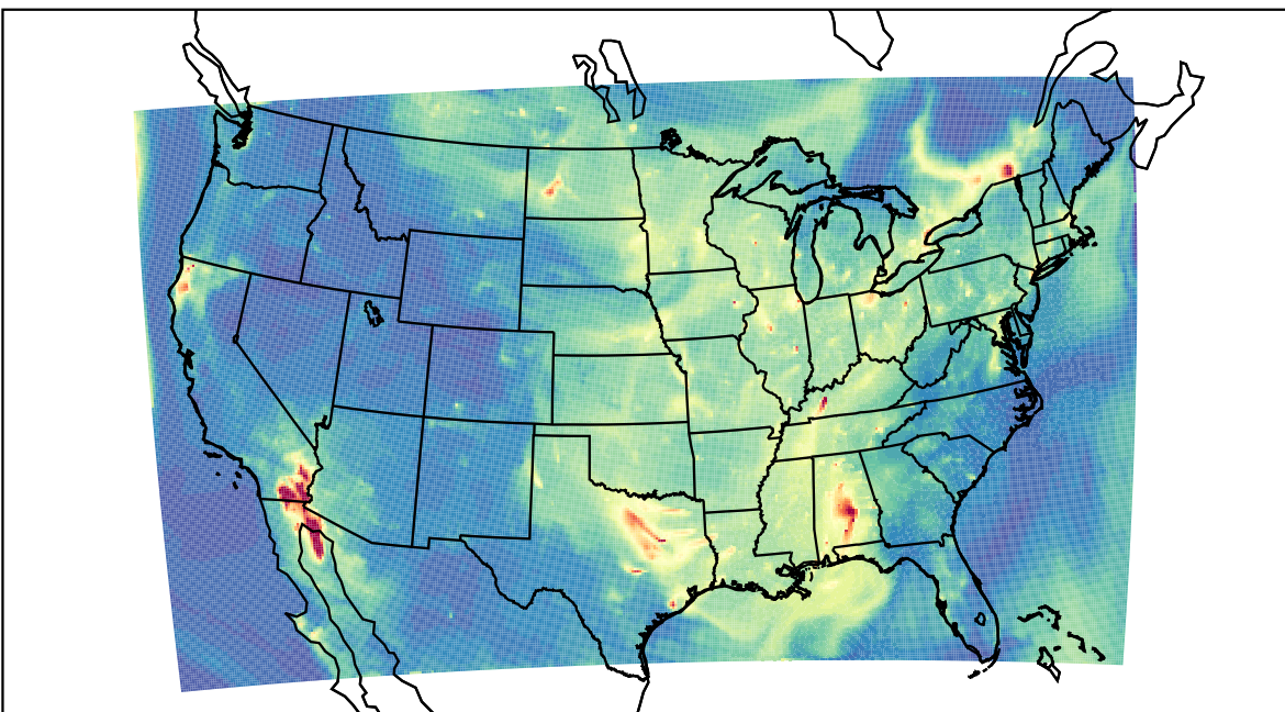
WRF 2023-09-10_12:00:00
