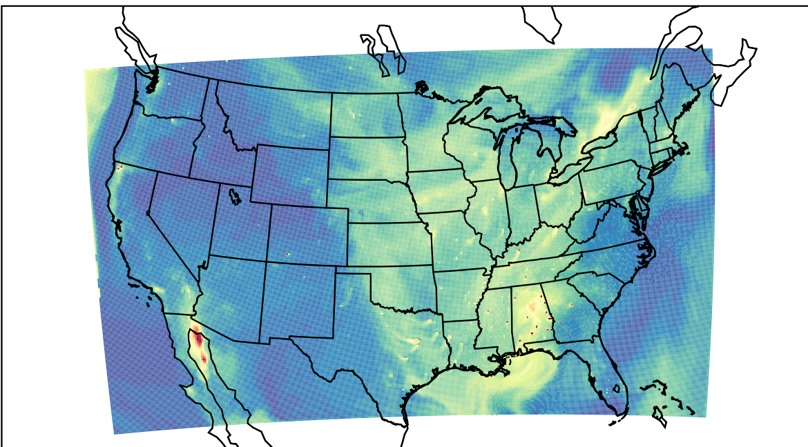
WRF 2023-09-10_20:00:00
