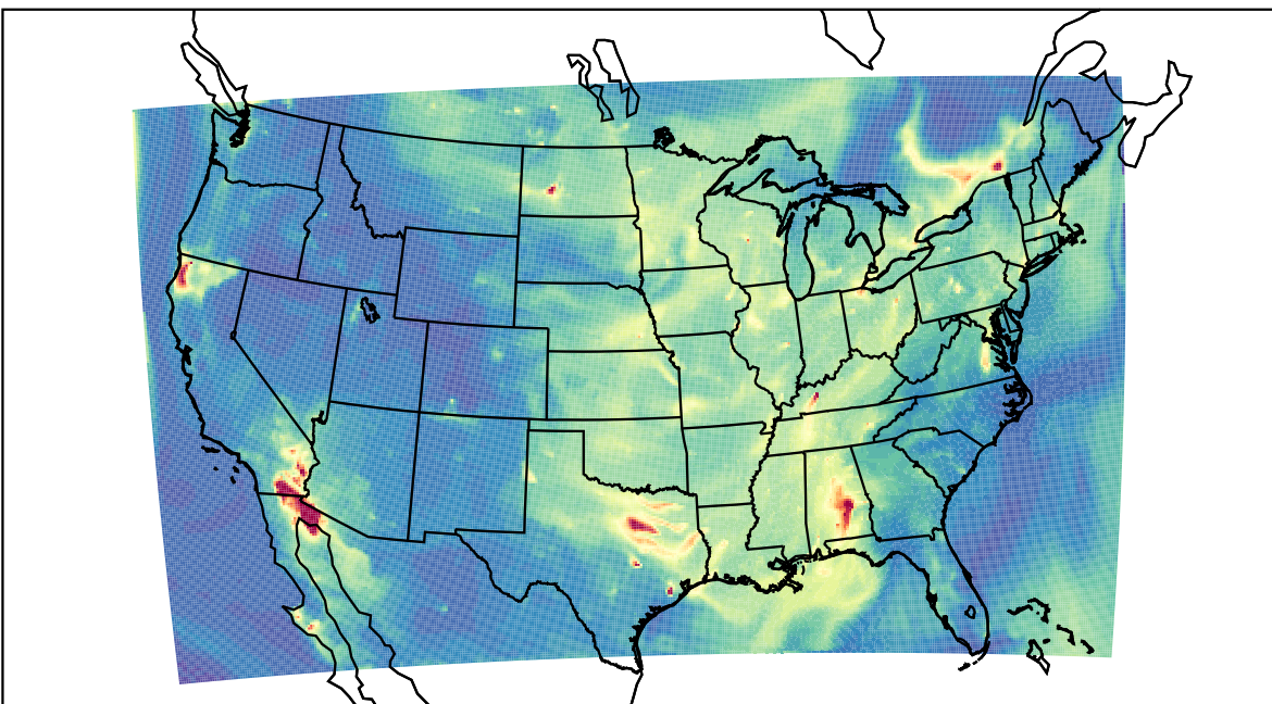
WRF 2023-09-10_09:00:00
