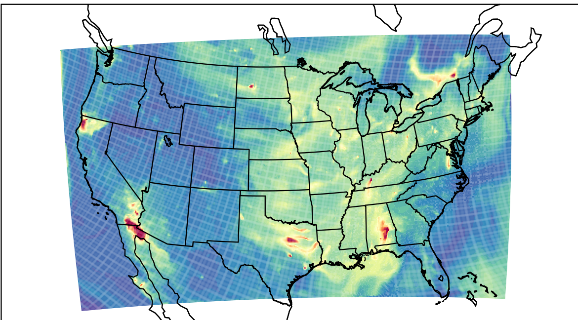
WRF 2023-09-10_08:00:00
