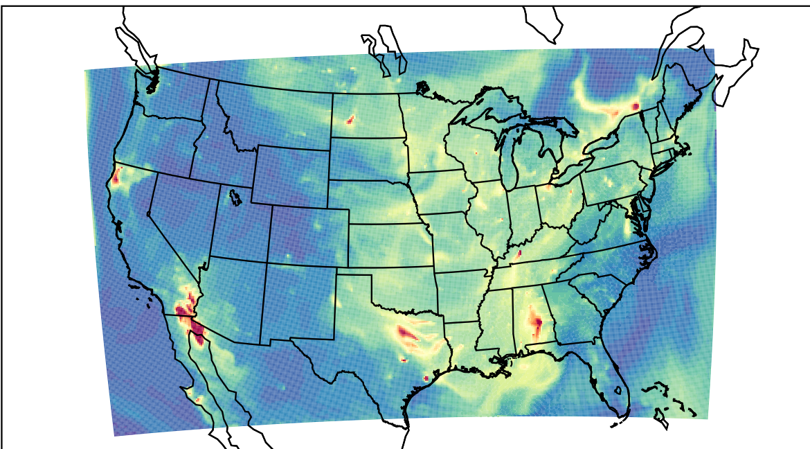
WRF 2023-09-10_10:00:00
