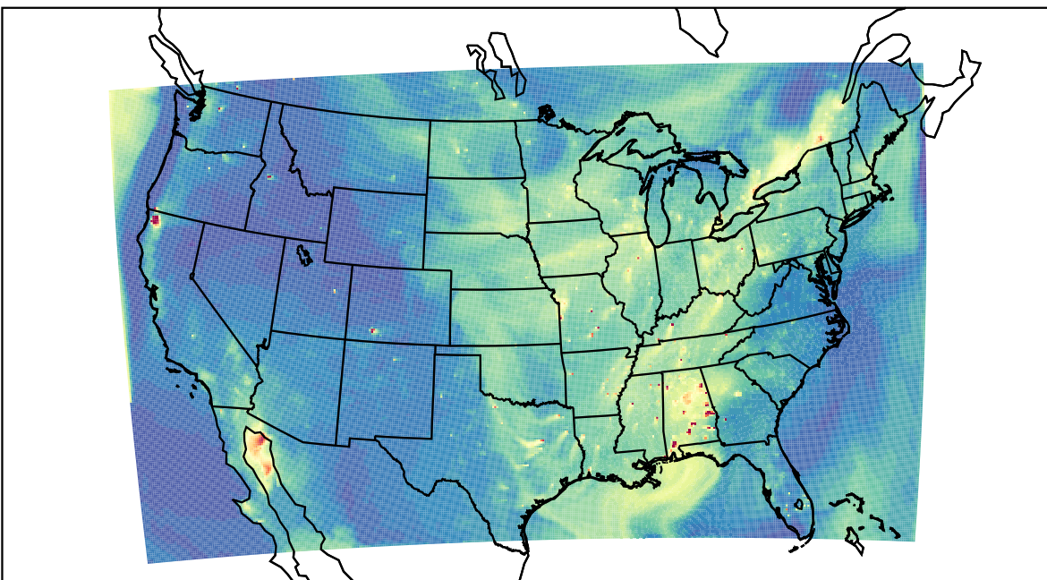
WRF 2023-09-10_23:00:00
