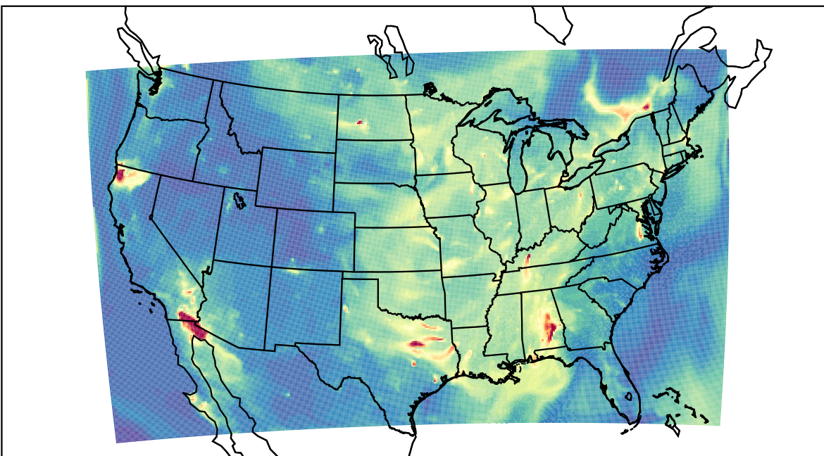
WRF 2023-09-10_07:00:00
