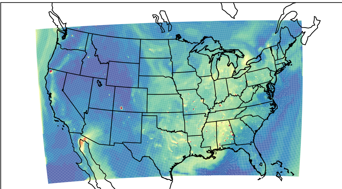
WRF 2023-09-11_22:00:00
