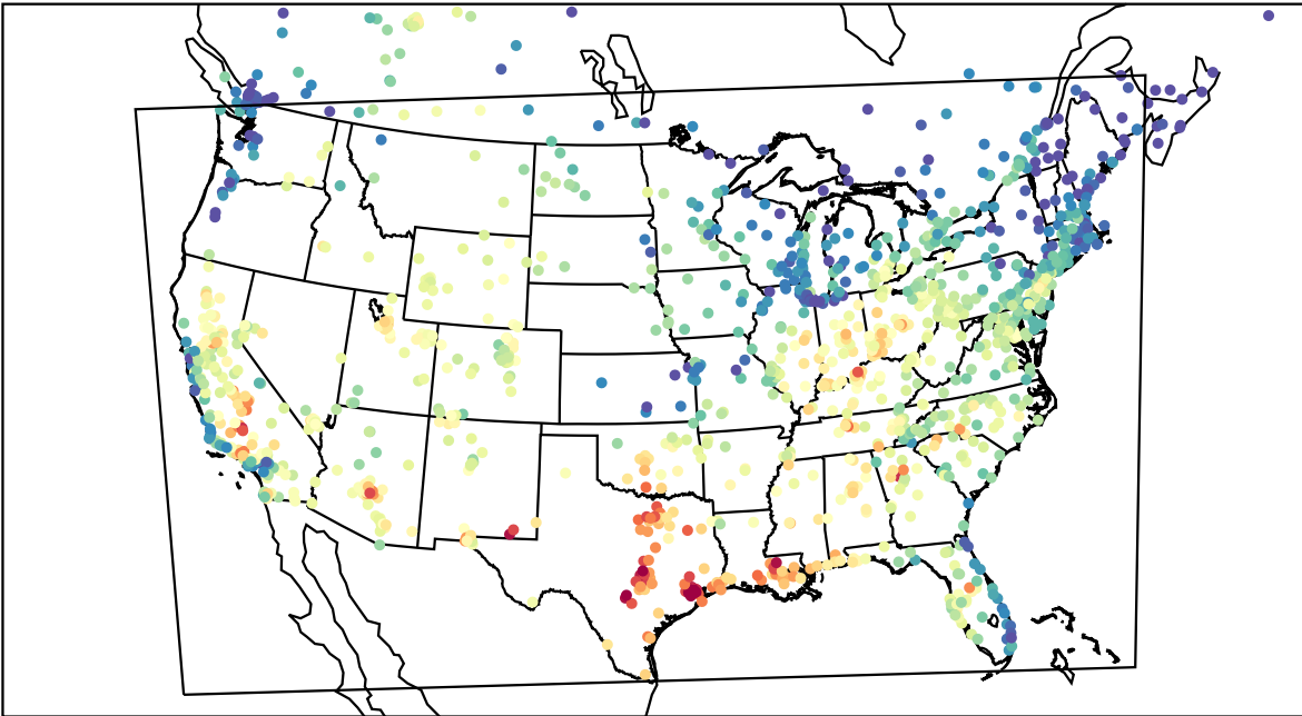
AirNOW (2023-09-11_19:00:00)
