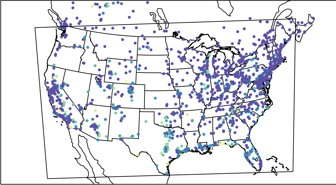
AirNOW (2023-09-11_13:00:00)
