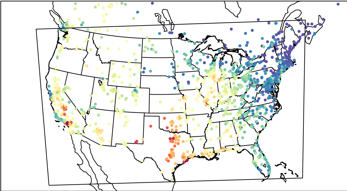
AirNOW (2023-09-10_22:00:00)
