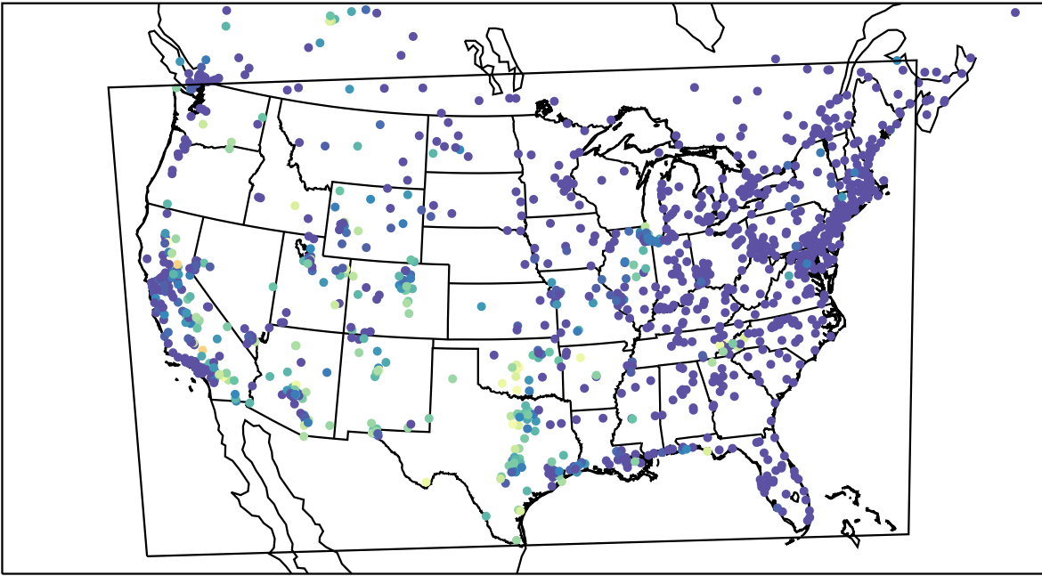
AirNOW (2023-09-11_10:00:00)
