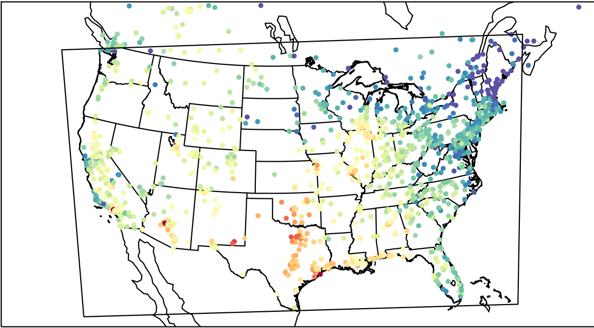
AirNOW (2023-09-10_19:00:00)
