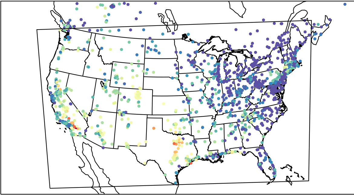
AirNOW (2023-09-10_03:00:00)
