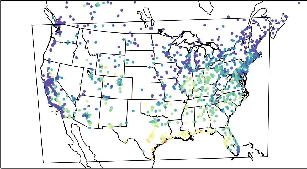
AirNOW (2023-09-11_15:00:00)
