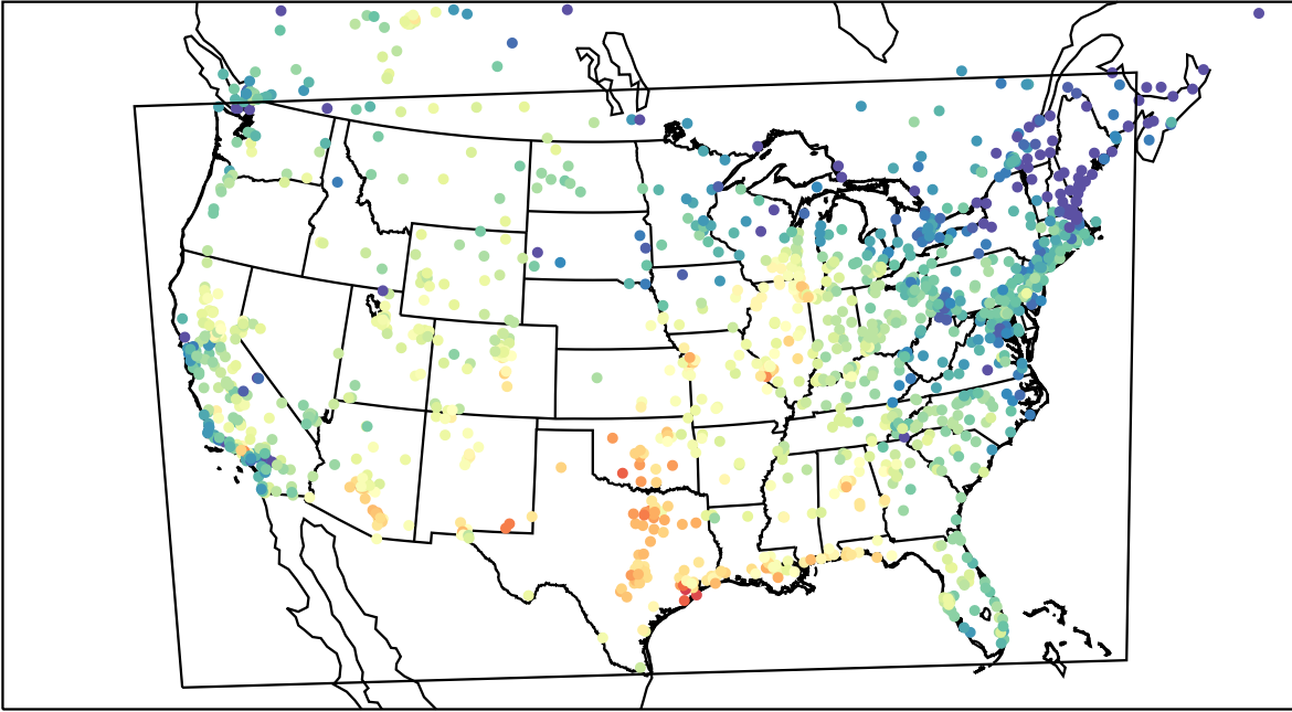
AirNOW (2023-09-10_18:00:00)
