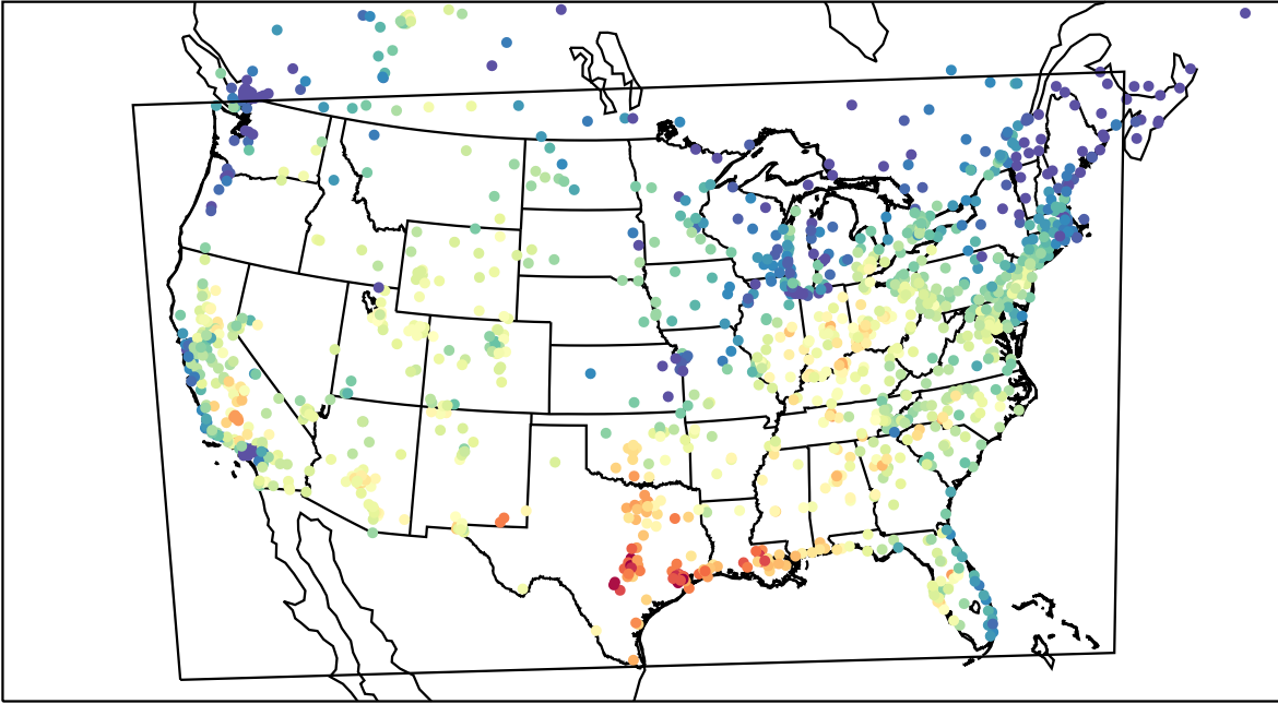
AirNOW (2023-09-11_18:00:00)
