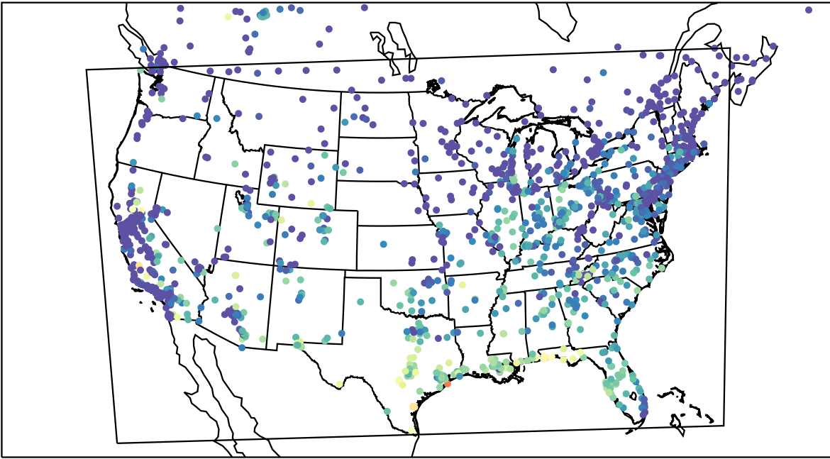
AirNOW (2023-09-11_14:00:00)
