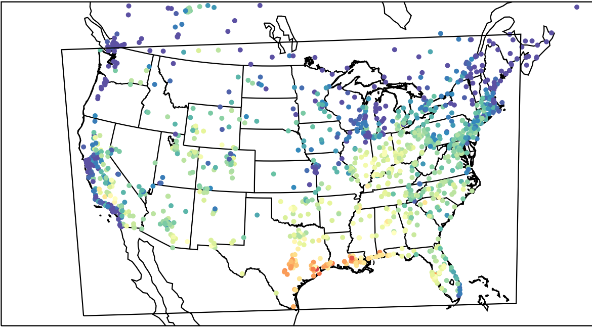
AirNOW (2023-09-11_16:00:00)
