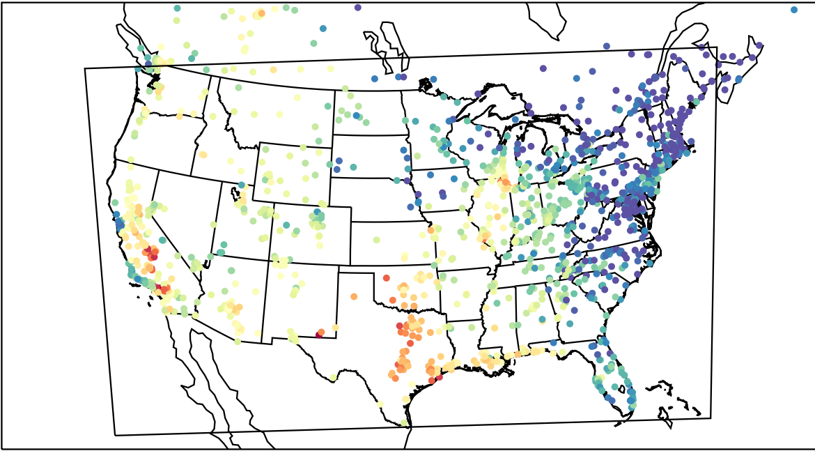
AirNOW (2023-09-10_23:00:00)
