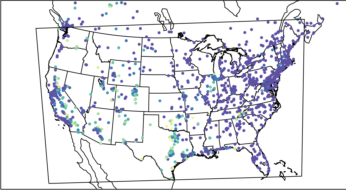
AirNOW (2023-09-11_10:00:00)
