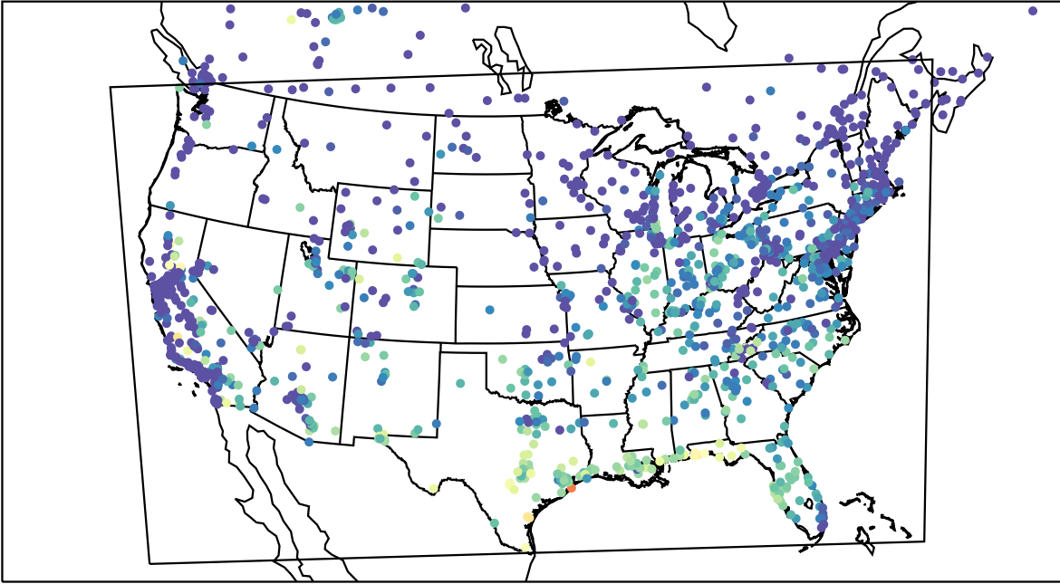
AirNOW (2023-09-11_14:00:00)
