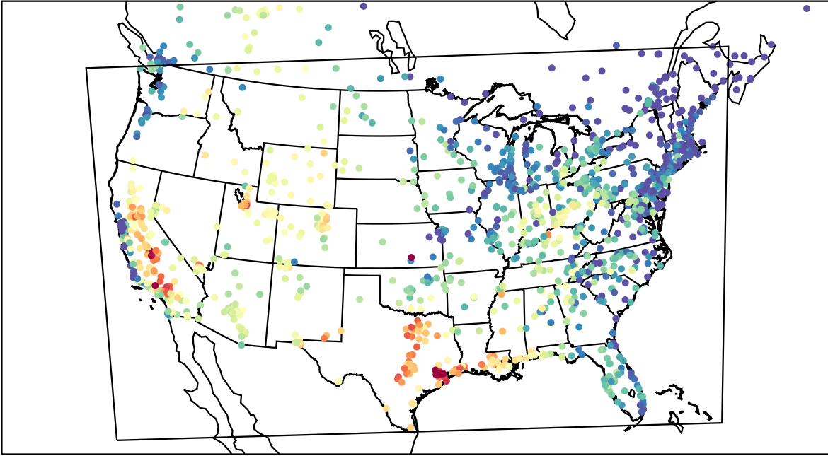
AirNOW (2023-09-11_23:00:00)
