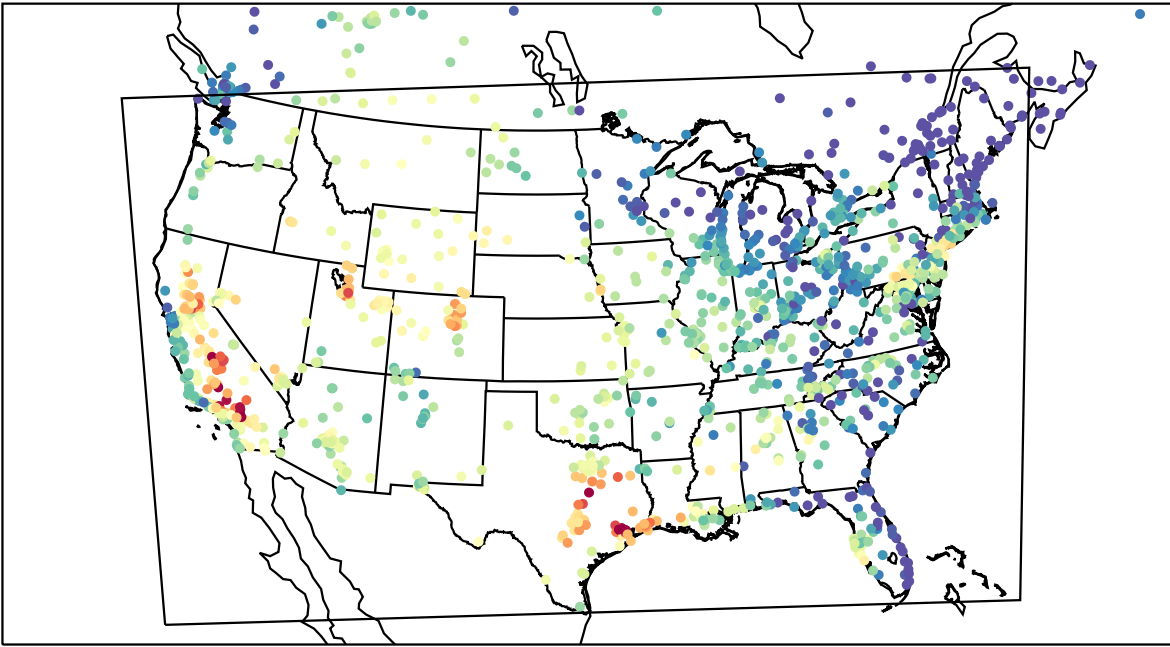
AirNOW (2023-09-12_23:00:00)
