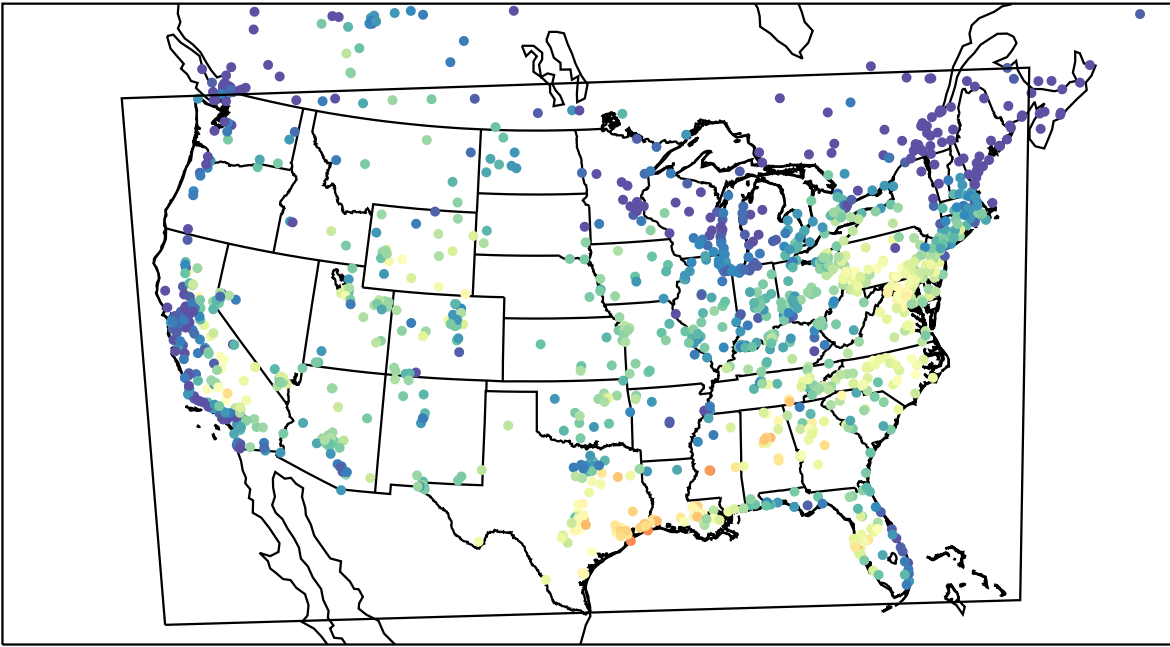
AirNOW (2023-09-12_16:00:00)
