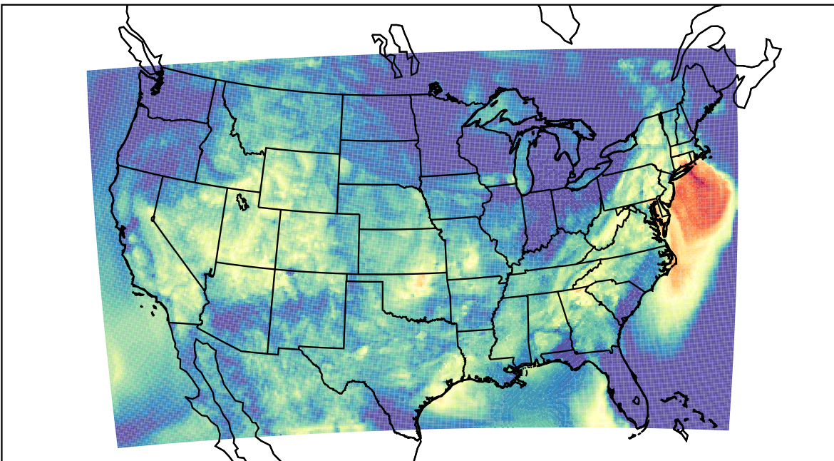
WRF (2023-09-13_10:00:00)
