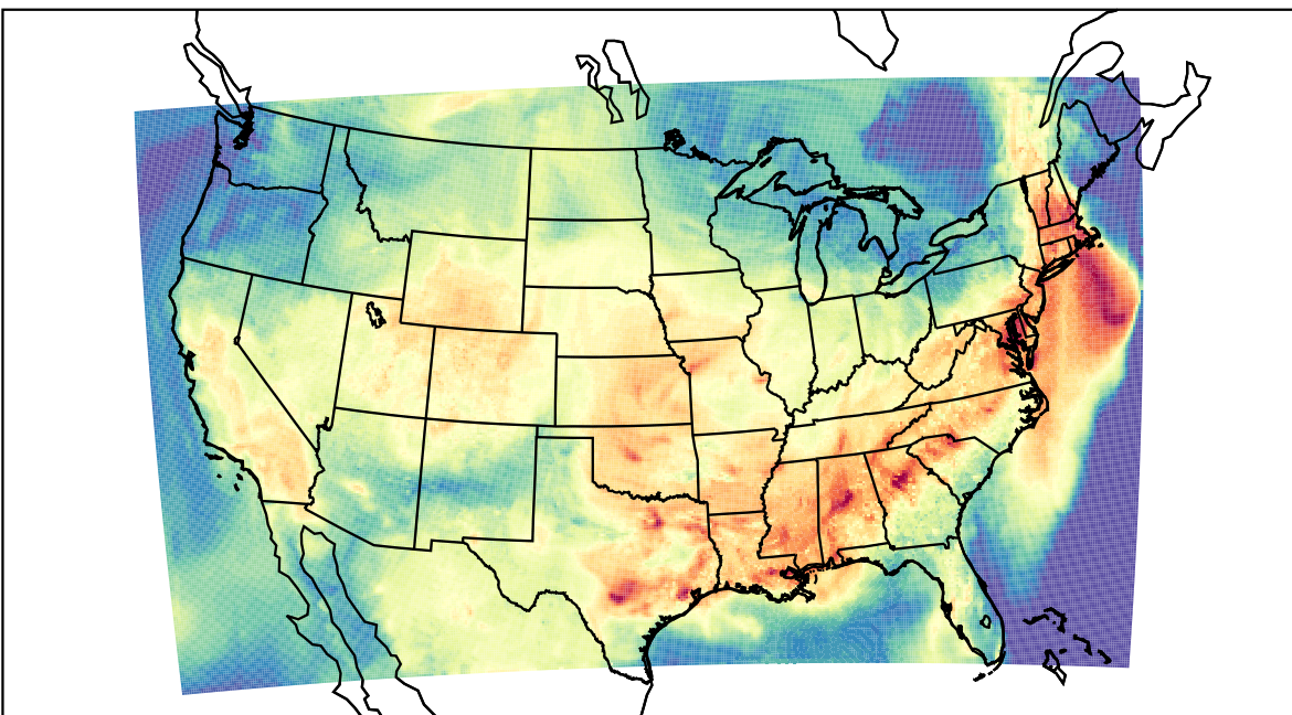
WRF (2023-09-13_20:00:00)
