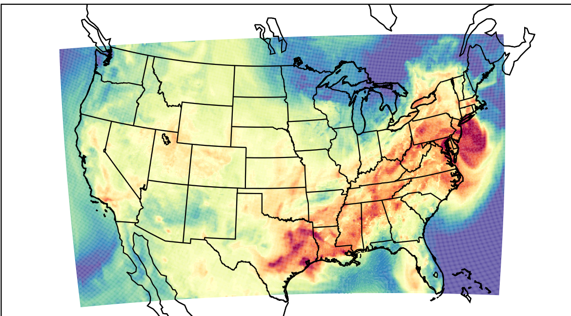
WRF (2023-09-12_20:00:00)
