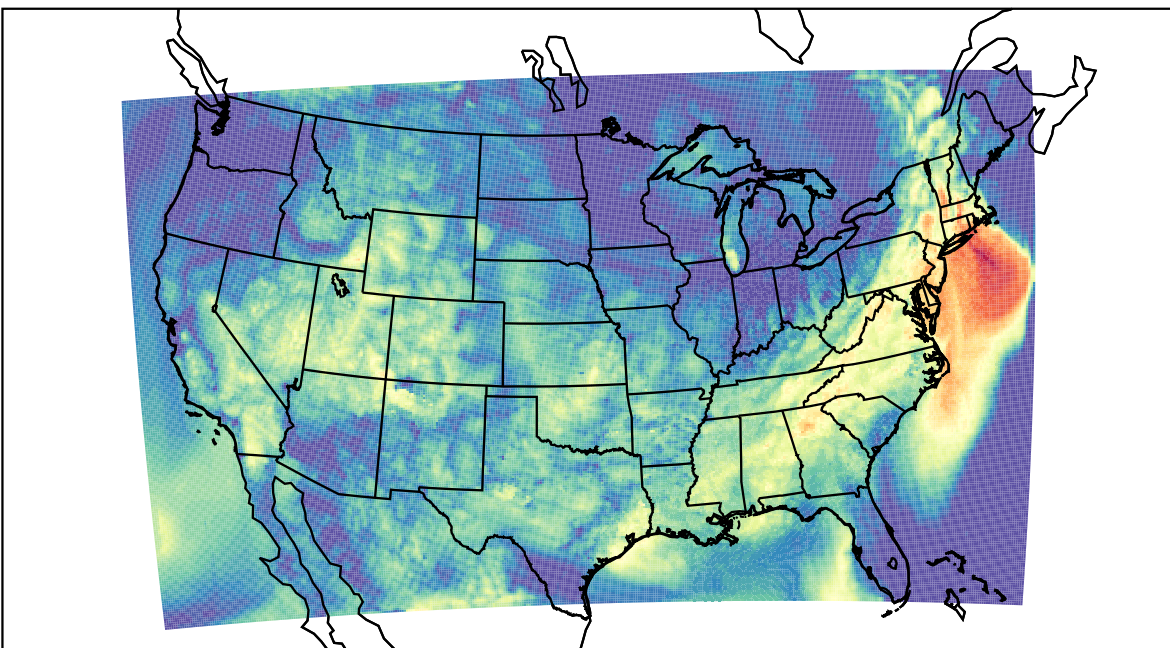
WRF (2023-09-13_14:00:00)
