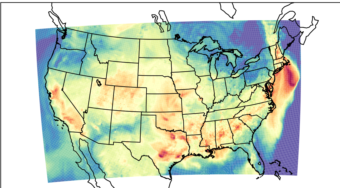
WRF (2023-09-13_23:00:00)
