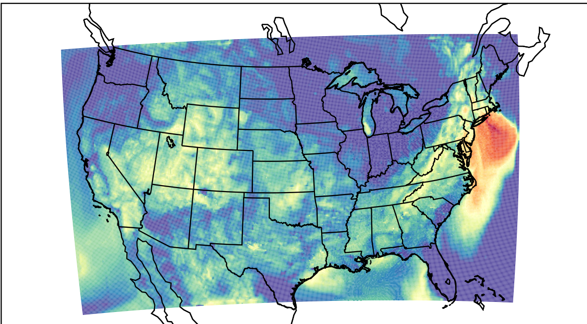
WRF (2023-09-13_13:00:00)
