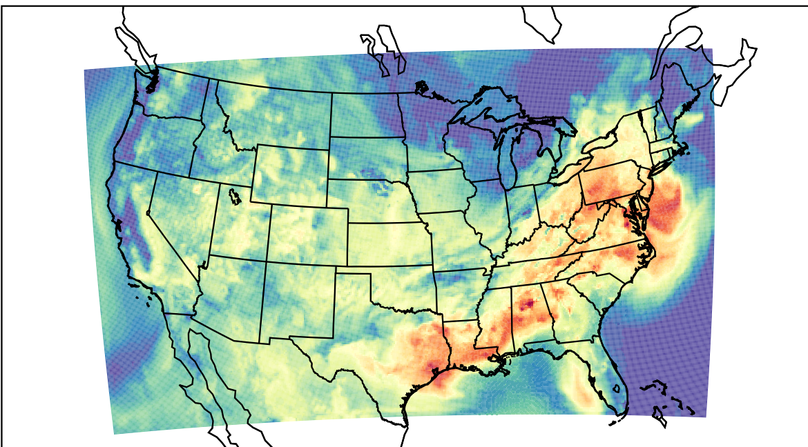
WRF (2023-09-12_16:00:00)
