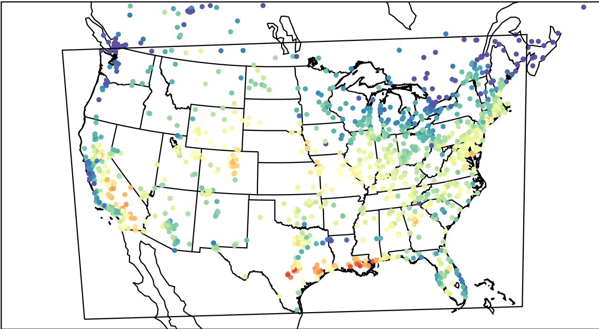
AirNOW (2023-09-13_18:00:00)
