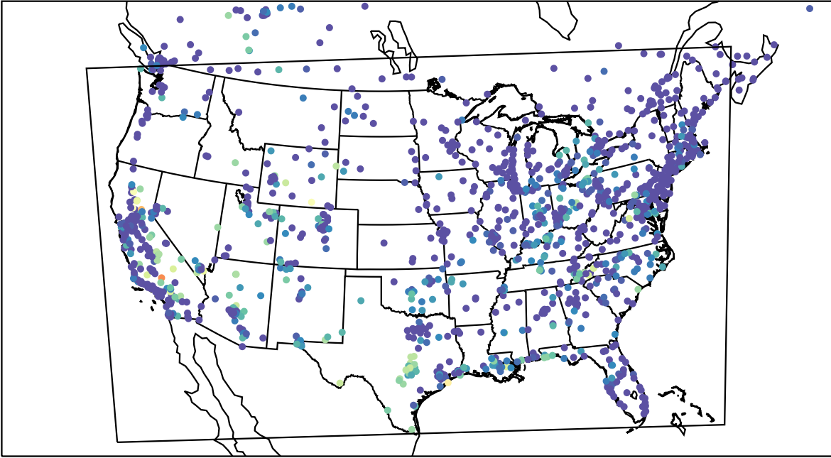
AirNOW (2023-09-12_13:00:00)
