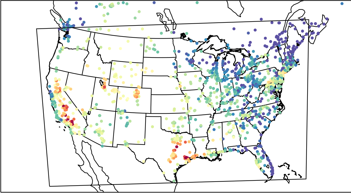
AirNOW (2023-09-12_23:00:00)
