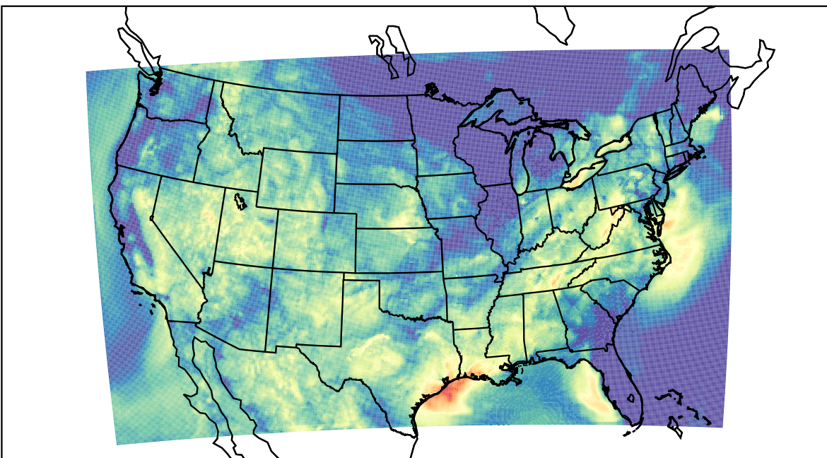
WRF (2023-09-12_10:00:00)
