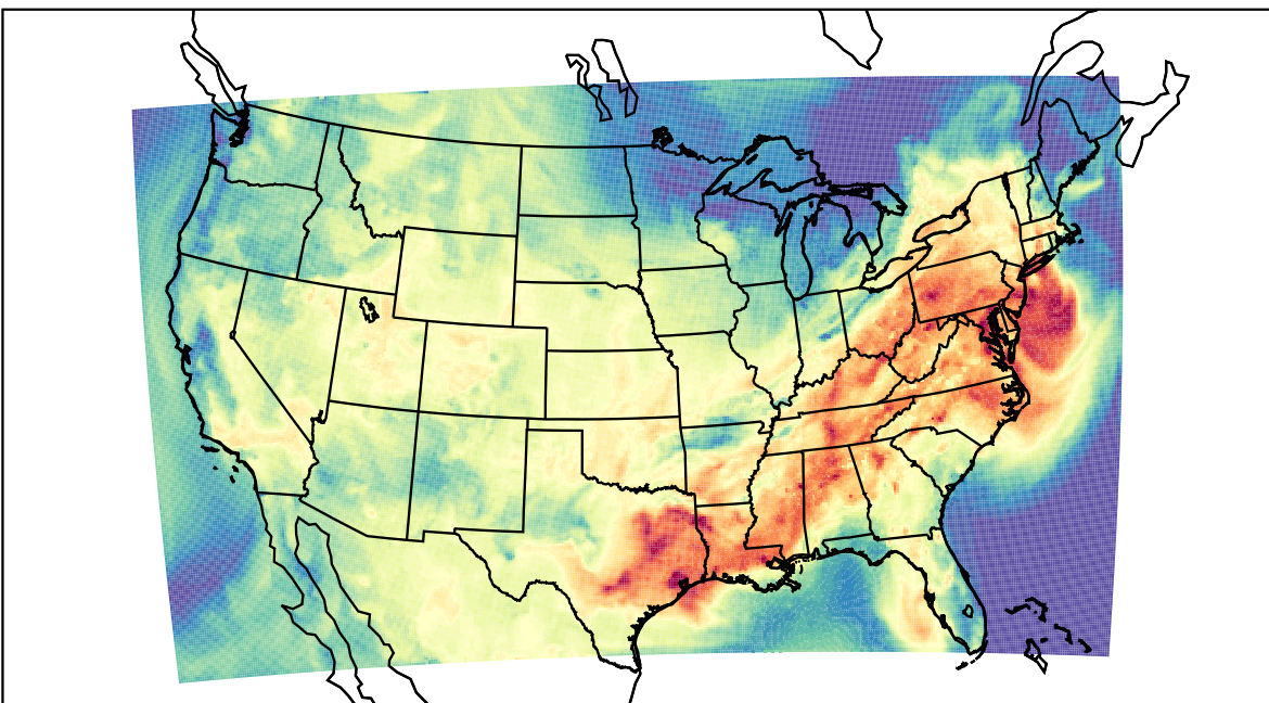
WRF (2023-09-12_18:00:00)
