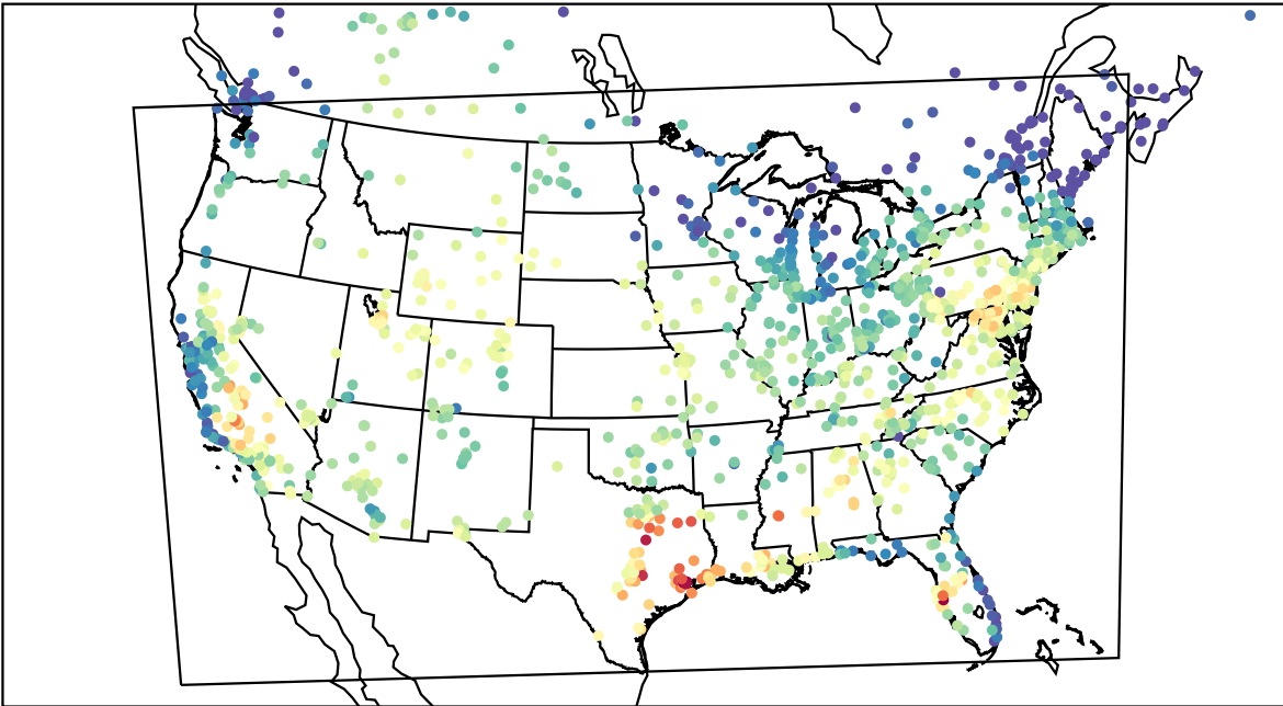
AirNOW (2023-09-12_18:00:00)
