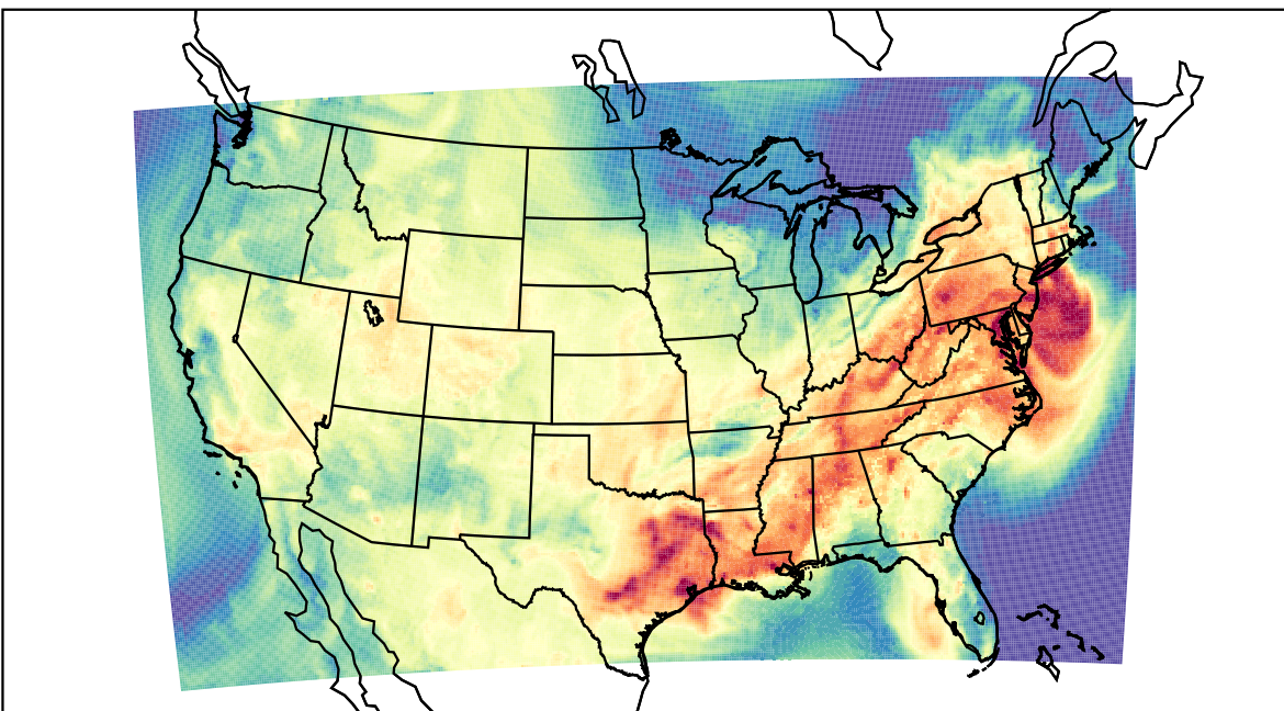
WRF (2023-09-12_19:00:00)
