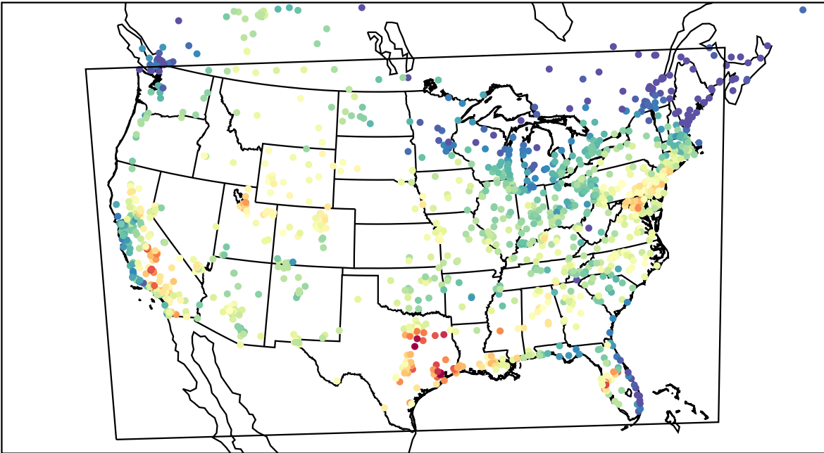
AirNOW (2023-09-12_19:00:00)
