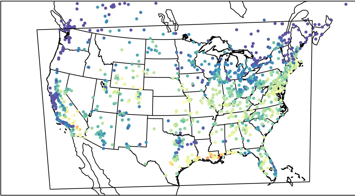
AirNOW (2023-09-13_16:00:00)
