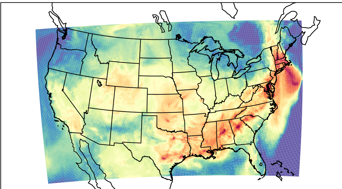
WRF (2023-09-13_19:00:00)
