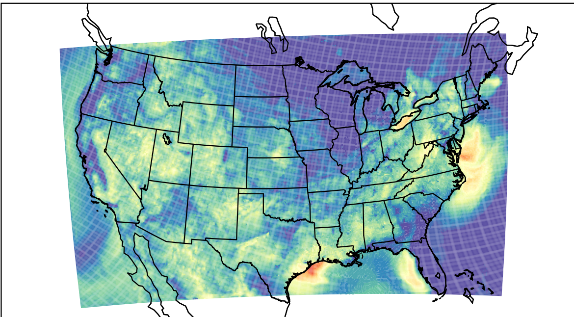
WRF (2023-09-12_13:00:00)
