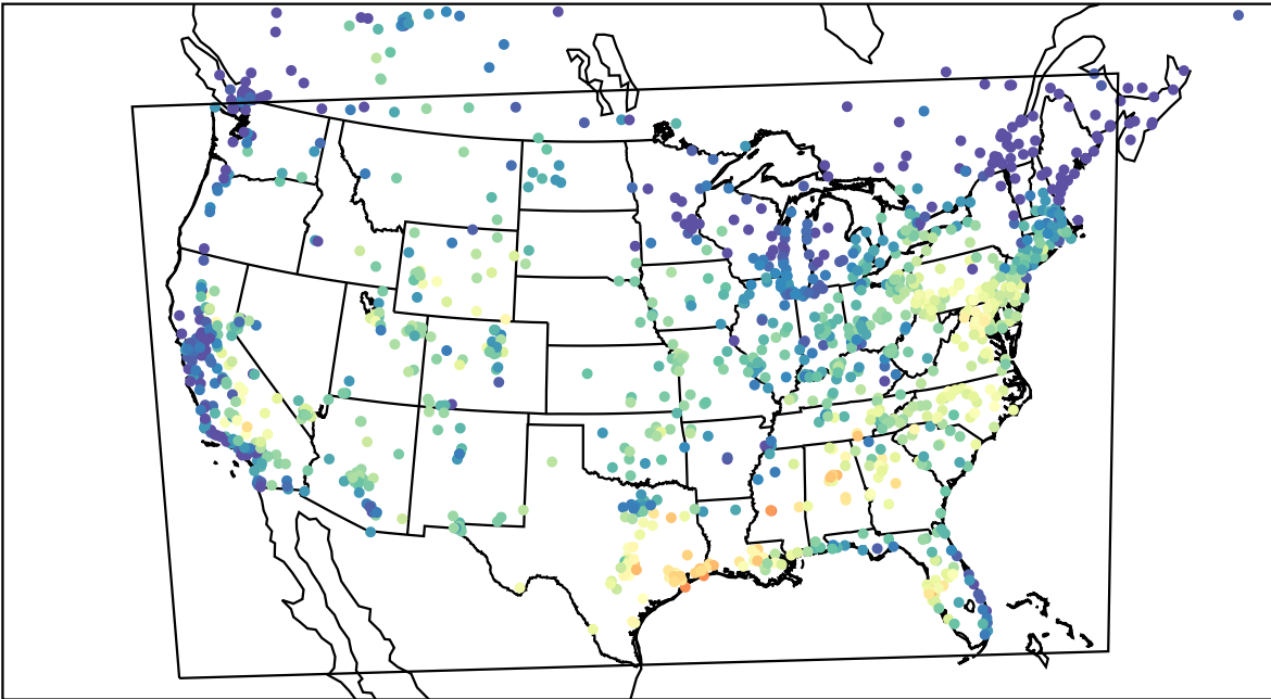
AirNOW (2023-09-12_16:00:00)
