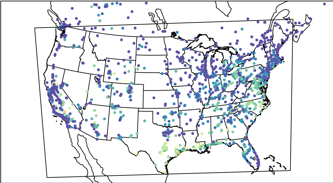
AirNOW (2023-09-12_14:00:00)
