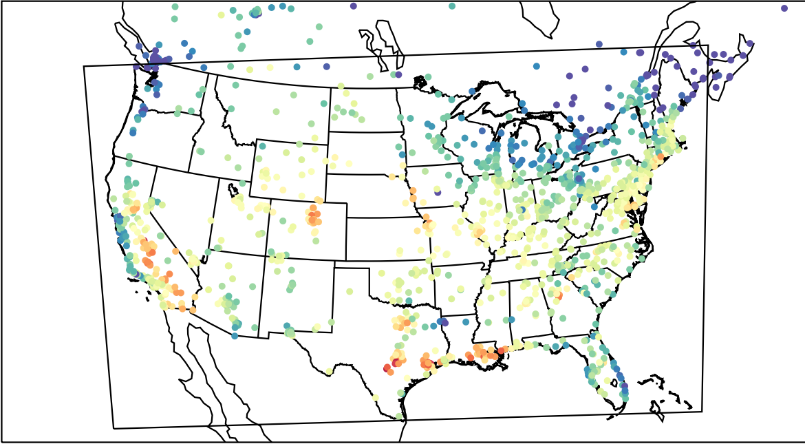
AirNOW (2023-09-13_19:00:00)
