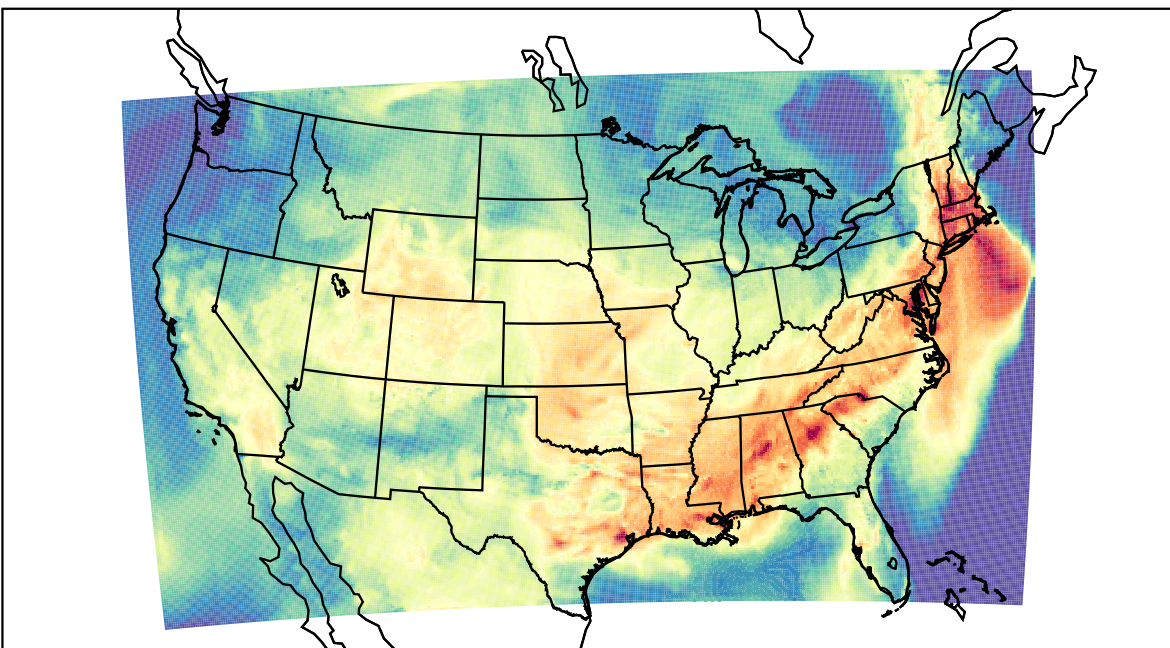
WRF (2023-09-13_18:00:00)
