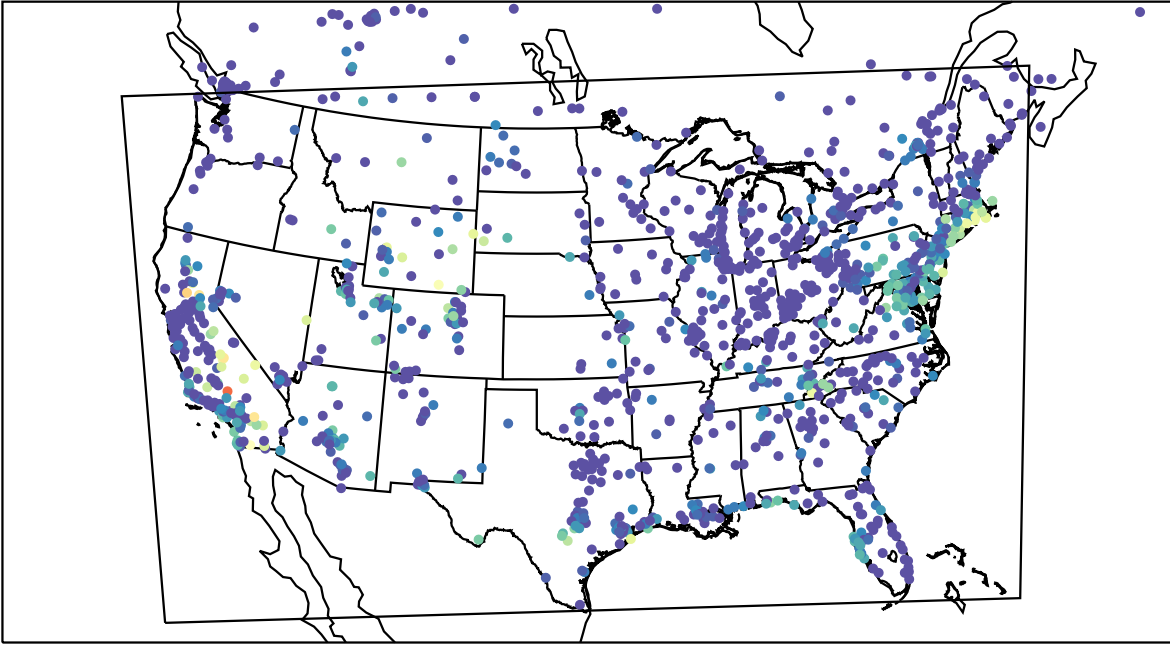
AirNOW (2023-09-13_13:00:00)
