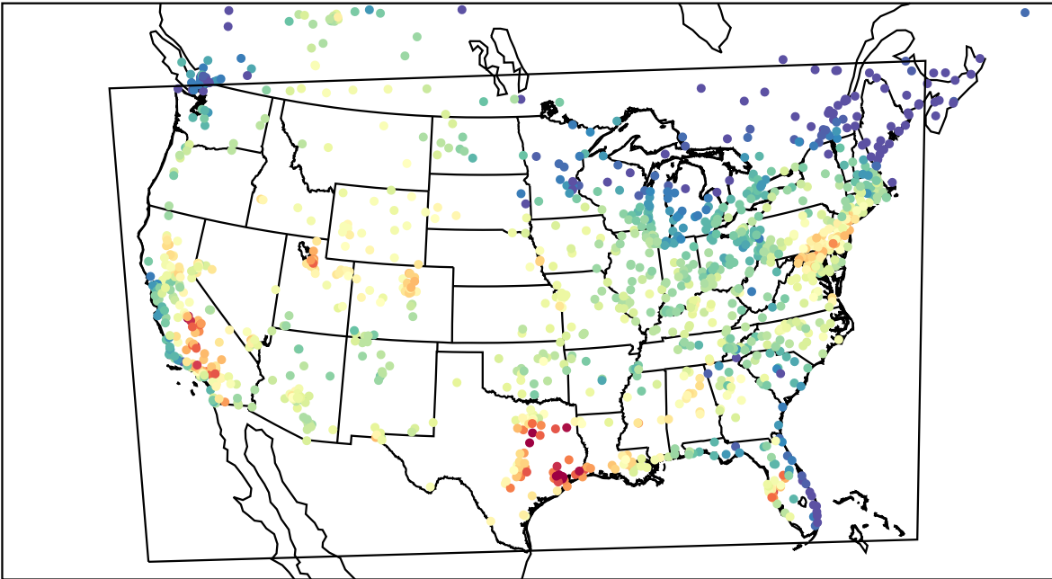
AirNOW (2023-09-12_20:00:00)
