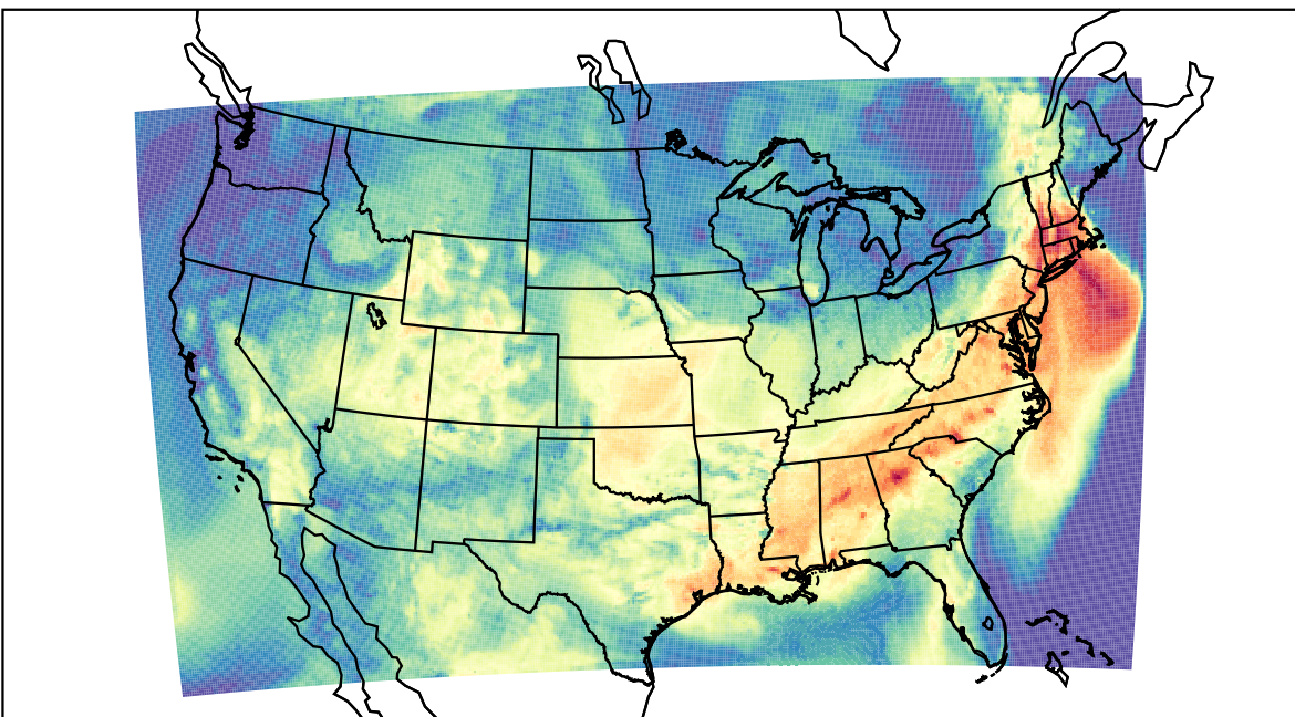
WRF (2023-09-13_16:00:00)
