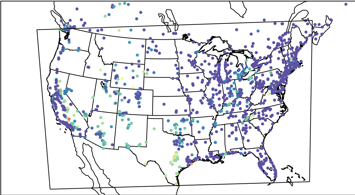
AirNOW (2023-09-12_10:00:00)
