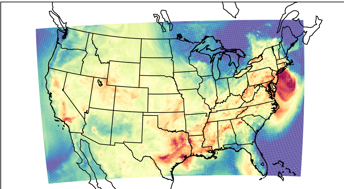
WRF (2023-09-12_23:00:00)
